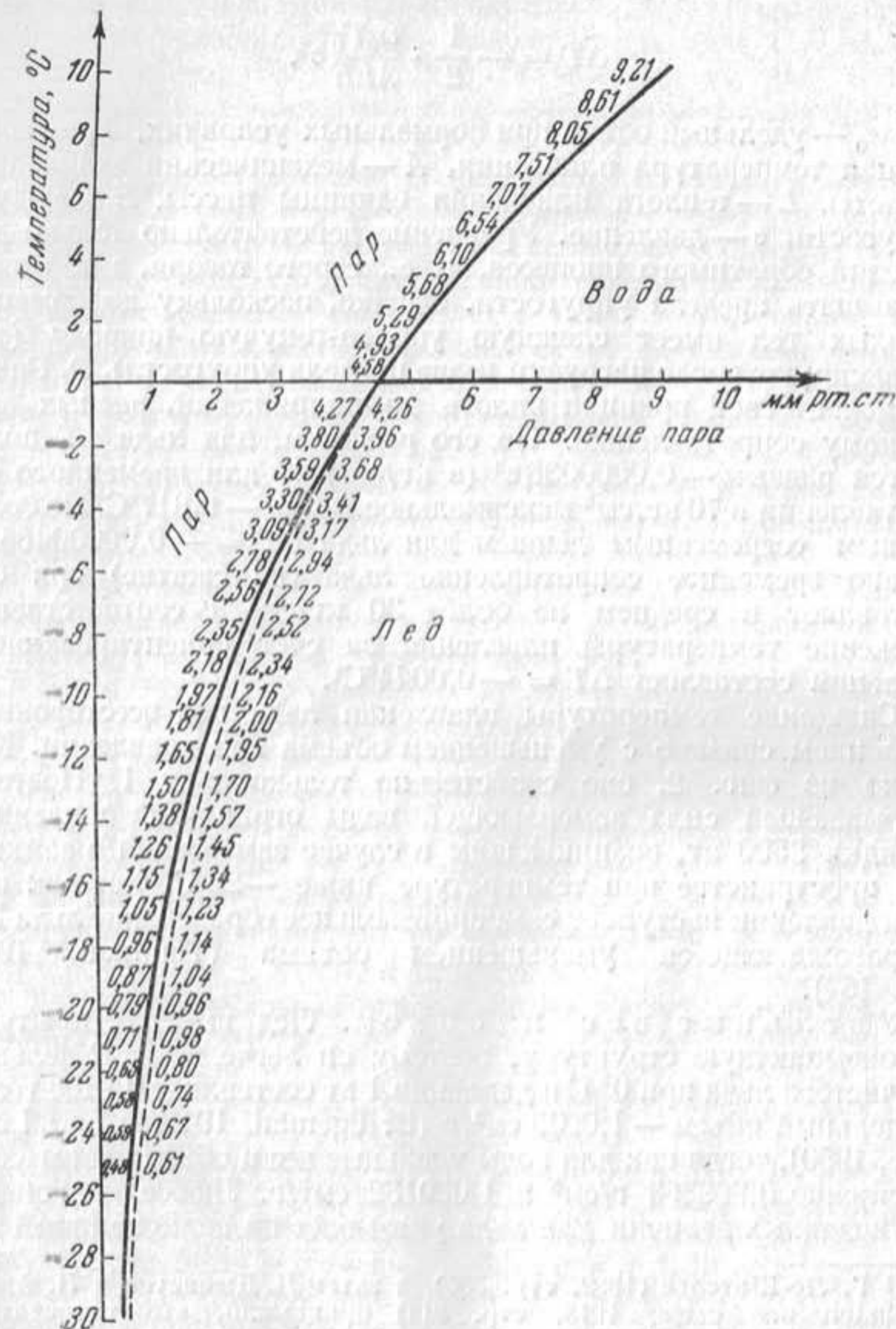
Фиг. 6. Давление насыщающих паров льда I и воды при атмосферном давлении. (Пунктиром показана кривая равновесия пара и переохлажденной воды.)
