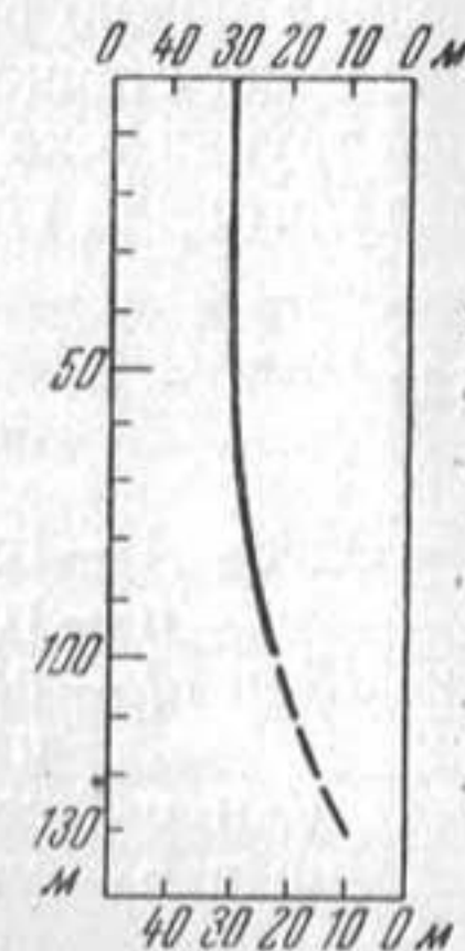
Фиг. 90. Движение в вертикальном профиле Юнгфрауфирна за 14 мес.
