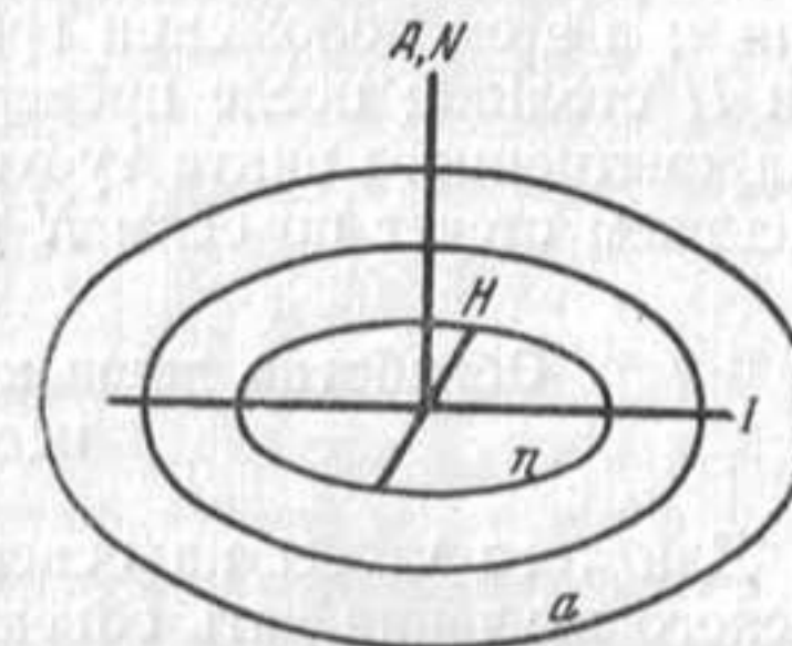
Фиг. 26. Схема осей федоровского столика в исходном положении.
