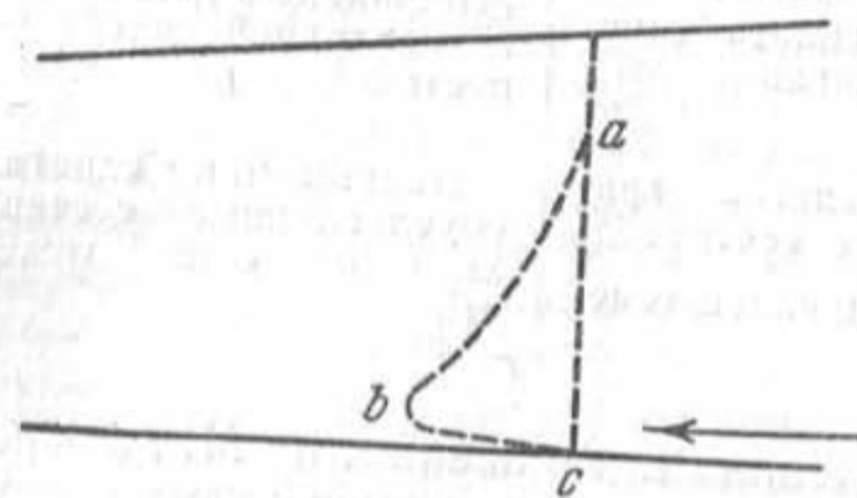
Фиг. 95. Эпюра скорости «течения выдавливания». (По М. Demorest, 1943)
