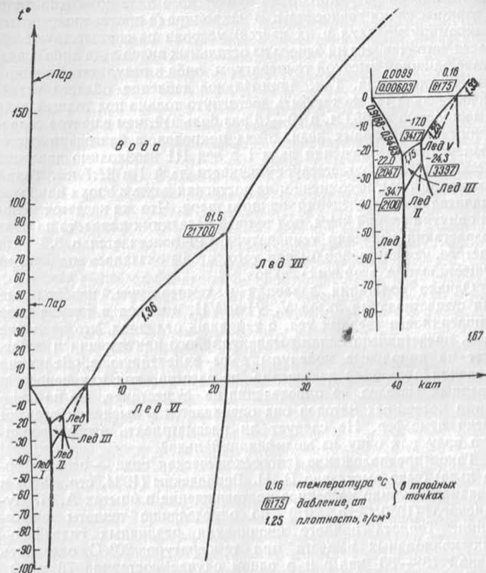
Фиг. 2. Фазовая диаграмма H_2O .
