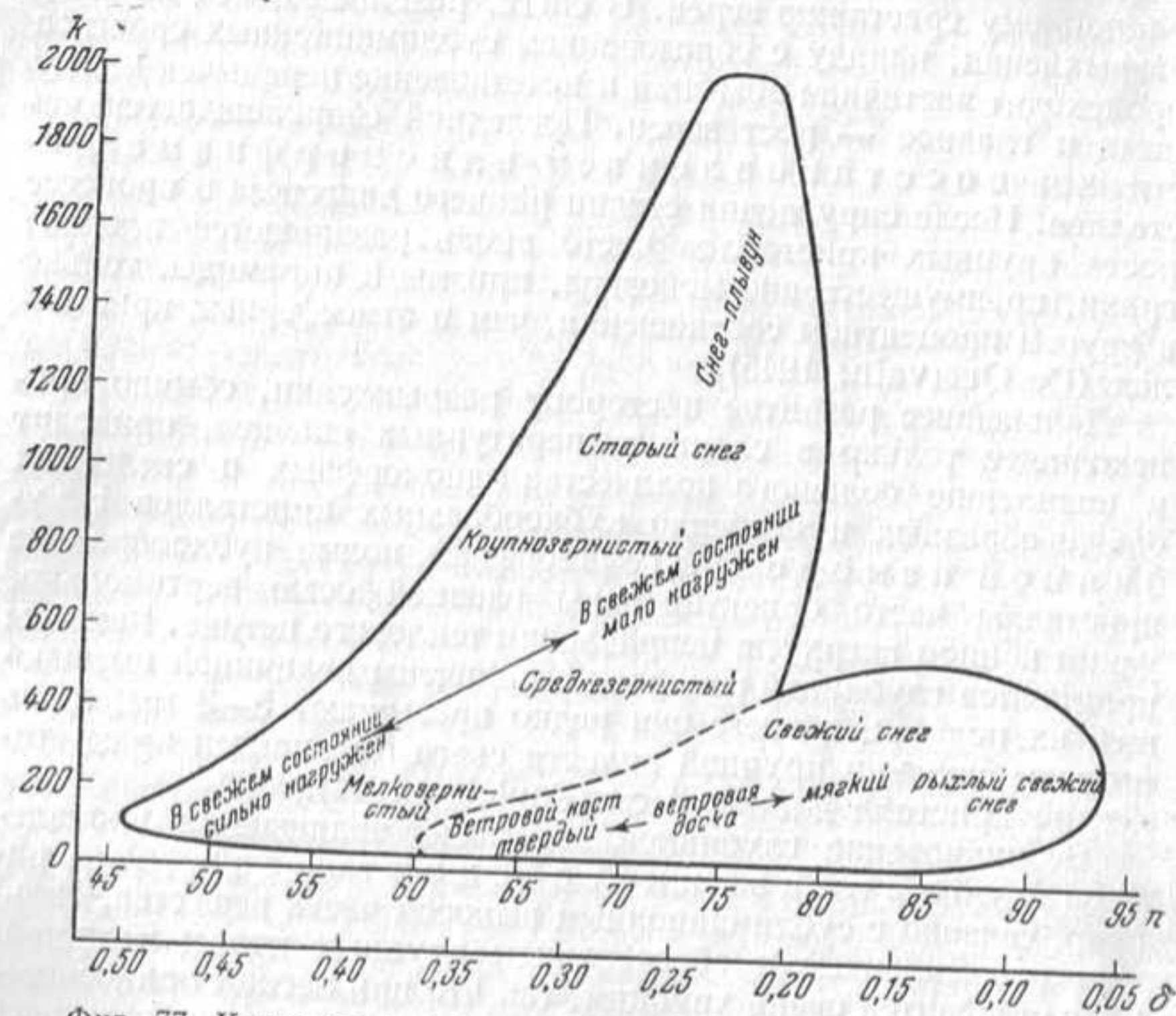
Фиг. 77. Классификация снега по соотношению пористости n с воздухопроницаемостью k . (По G. Bader, 1939)
