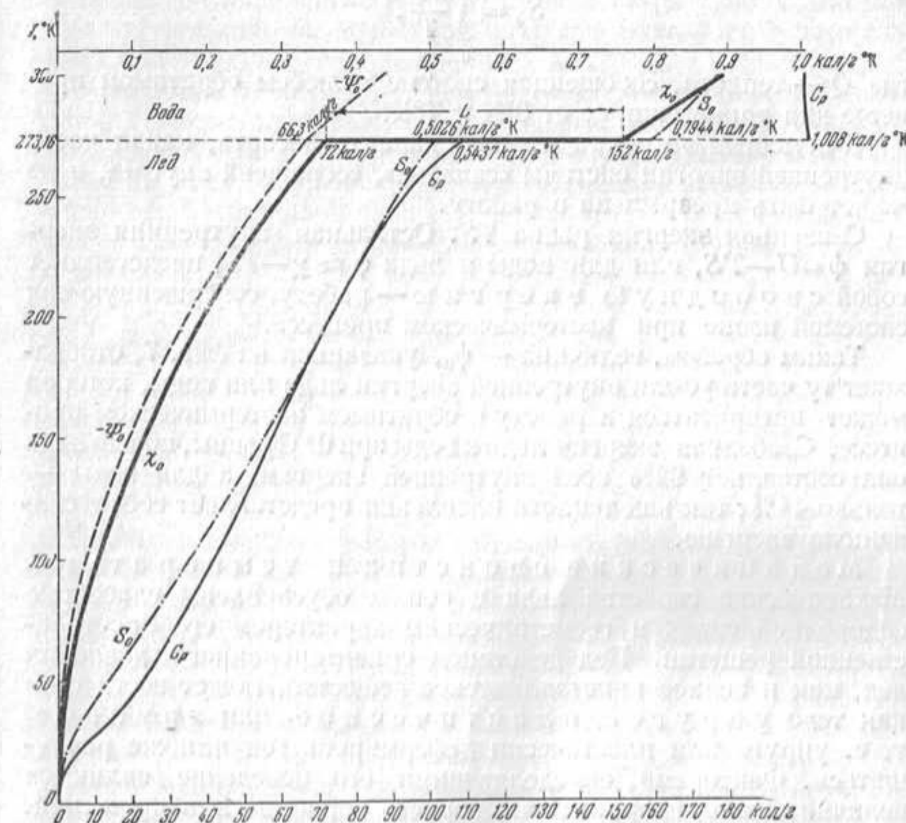
Фиг. 7. Калорические свойства и тепловая энергия льда при давлении в 1 ат.
