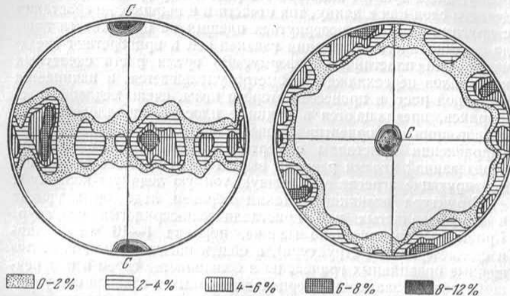
Фиг. 31. Стереогрaмма кристаллографической ориентировки первичного слоя конжеляционного льда на поверхности спокойной воды (52 кристалла). (Обычный случай.)
