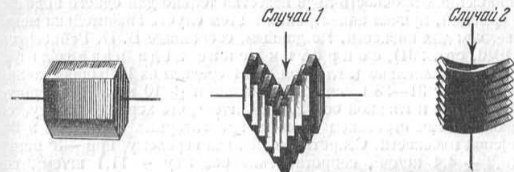
Фиг. 8. Схема опытов О. Мюгге по деформированию льда.
