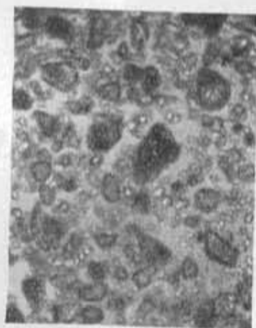
Фиг. 44. Минеральные частицы в кристалле льда. \times 100 . (Фото Б. И. Втюрина)
