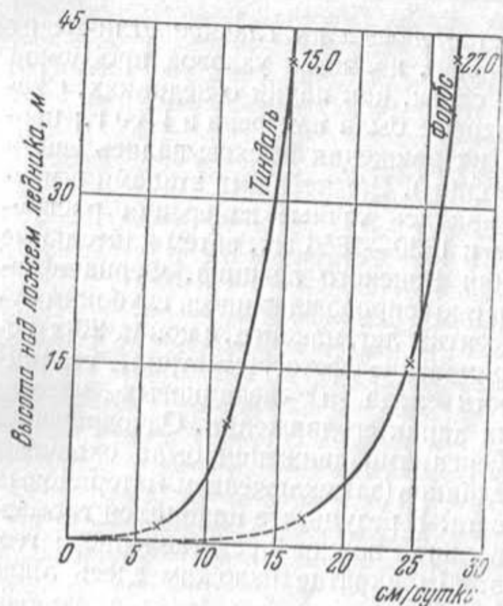
Фиг. 89. Эпюра скорости движения льда в вертикальном профиле ледника Мер де Глас по фронтальной стене по измерениям Д. Д. Форбса в 1846 г. и по боковой стене по измерениям Д. Тиндаля в 1857 г.
