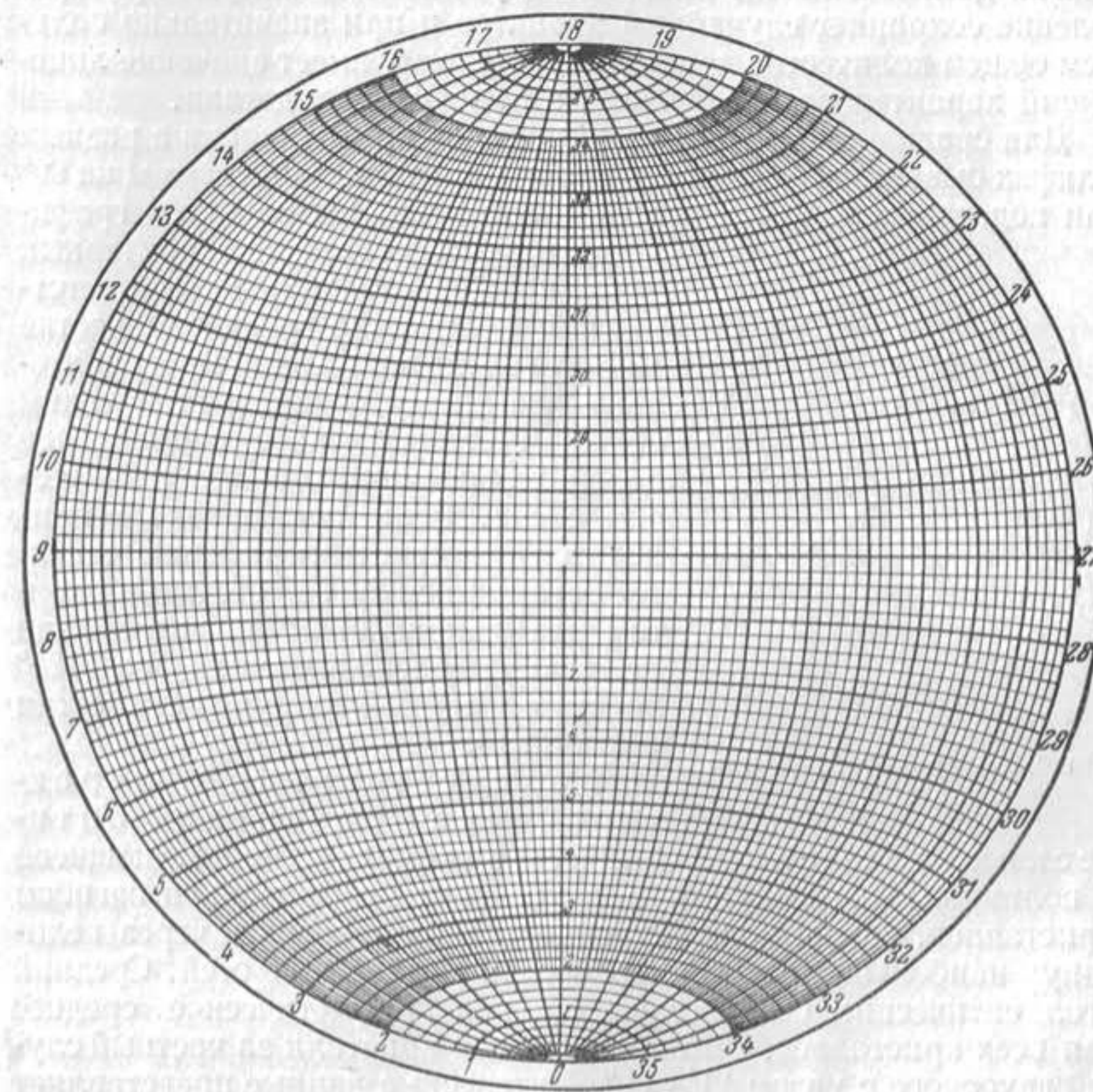
Фиг. 28. Сетка Шмидта. Уменьшена в 2 раза.
