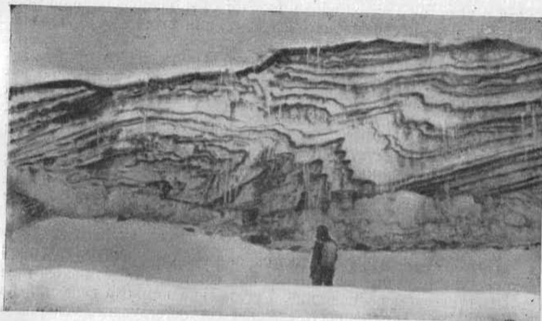
Фиг. 92. Складчатость в обрыве ледника. (Фото Н. В. Черепанова)
