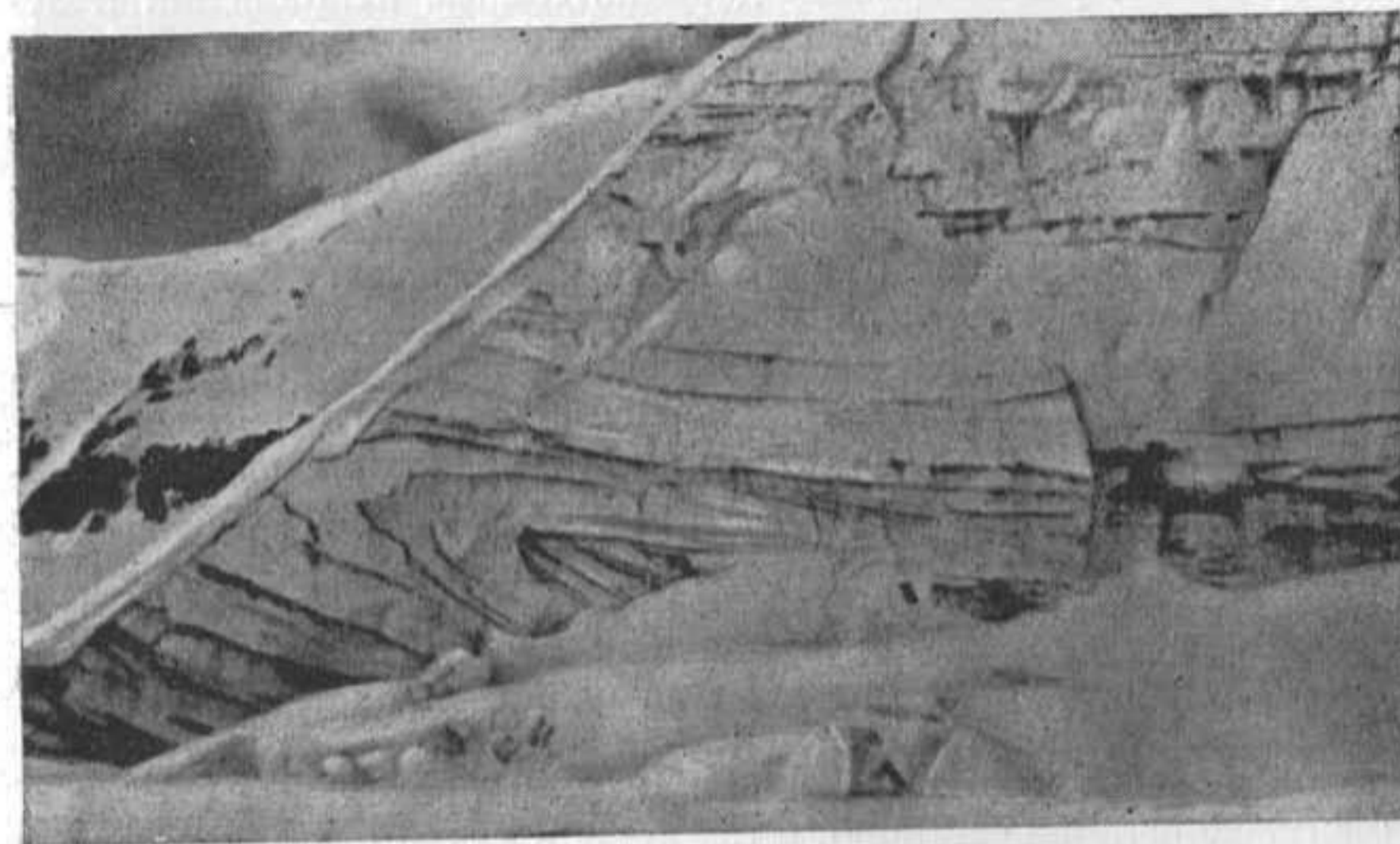
Фиг. 93. Антиклинальная складка, осложненная в замке пloidчатостью, с разрывом и волочением вдоль верхнего крыла. Масштаб 1 см \approx 5 м. (Фото Н. В. Черепанова)
