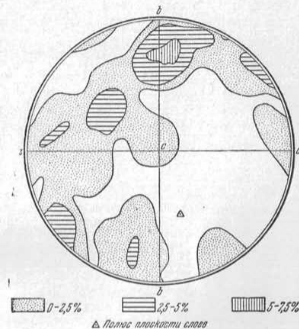
Фиг. 117. Стереогрaмма кристаллографической ориентировки льда, вмещающего голубую ленту, показанную на фиг. 115 и 116.
