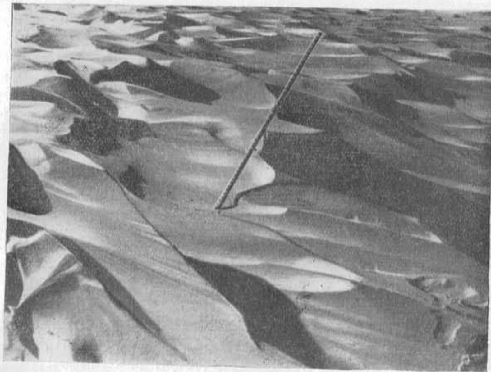
Фиг. 75. Свежие продольные снежные дюны. (Фото Н. В. Черепанова)
