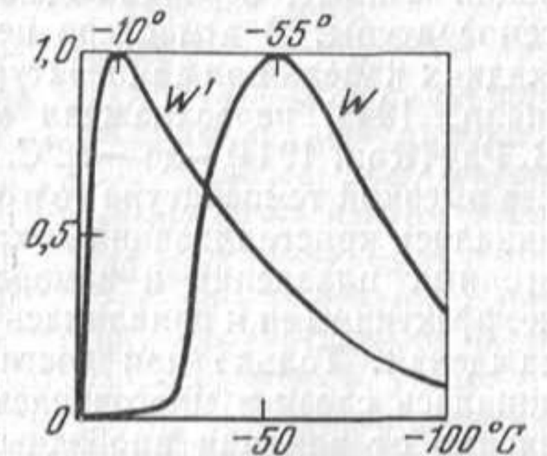
Фиг. 12. Температурная зависимость вероятности самопроизвольного образования объемных W и плоскостных W' зародышей кристаллов льда в переохлажденной воде.
