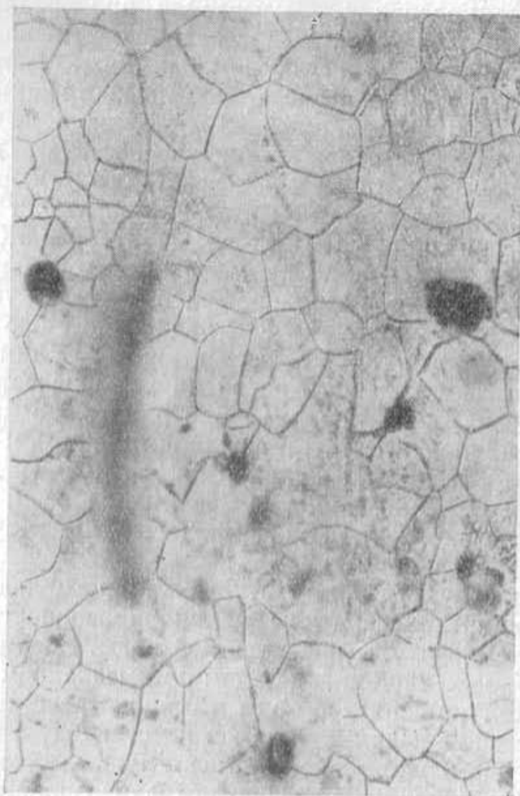
Фиг. 46. Полость по оси вертикальной жилы в ледниковом льду. По структуре жильный лед не отличается от вмещающего. Овальные темные пятна — пузырьки воздуха в ледниковом льду.
