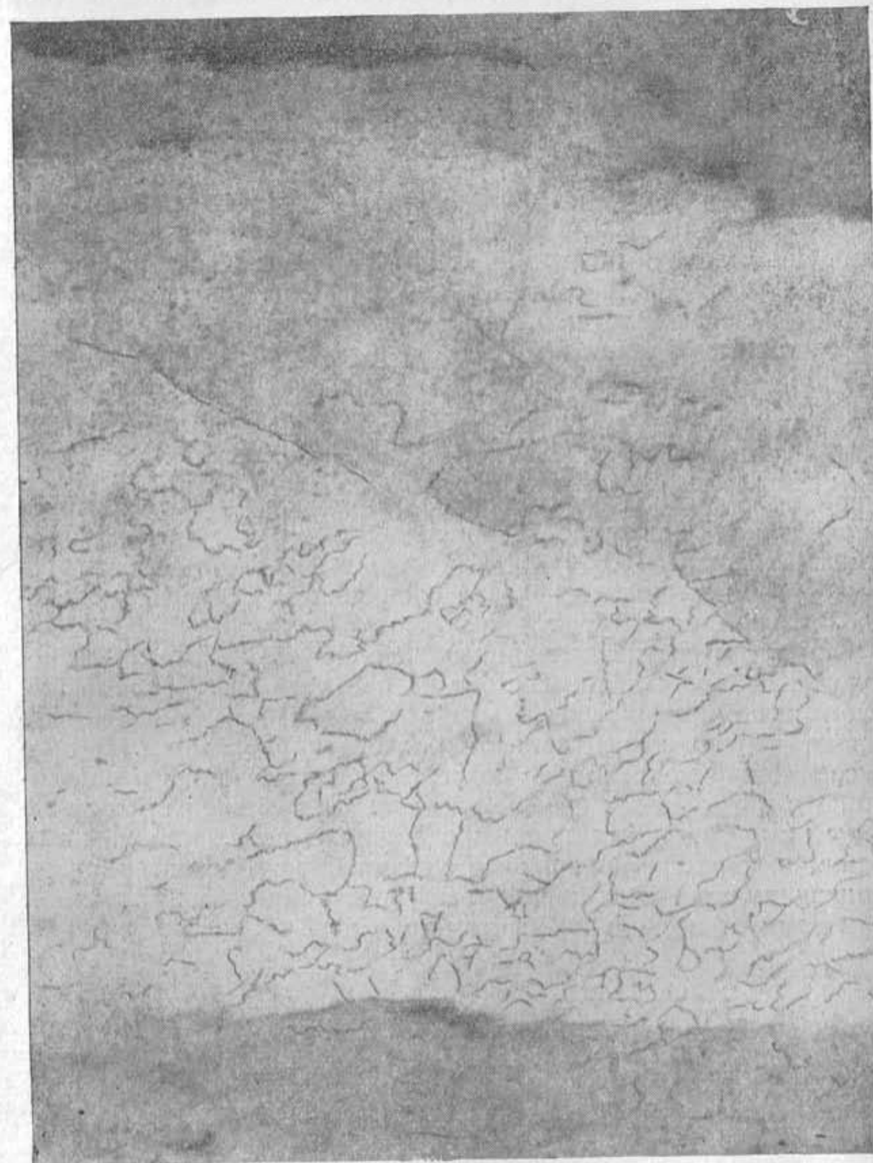
Фиг. 119. Апофиза мощной линзы «хрустального» льда среди перекристаллизованного инфильтрационно-рекристаллизационного с флюидальной текстурой.
