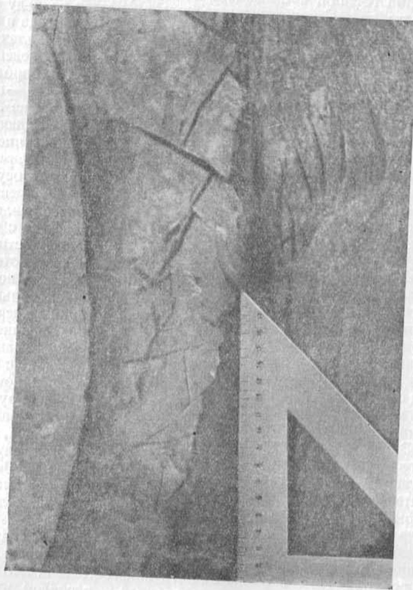
Фиг. 105. Вертикальное сечение контакта повторной ледяной жилы с вмещающей мерзлой породой. Темное—лед, светлое—мерзлая порода. Серия поперечных сбоев между главным телом жилы и апофизой. (Фото Б. И. Втюрина)
