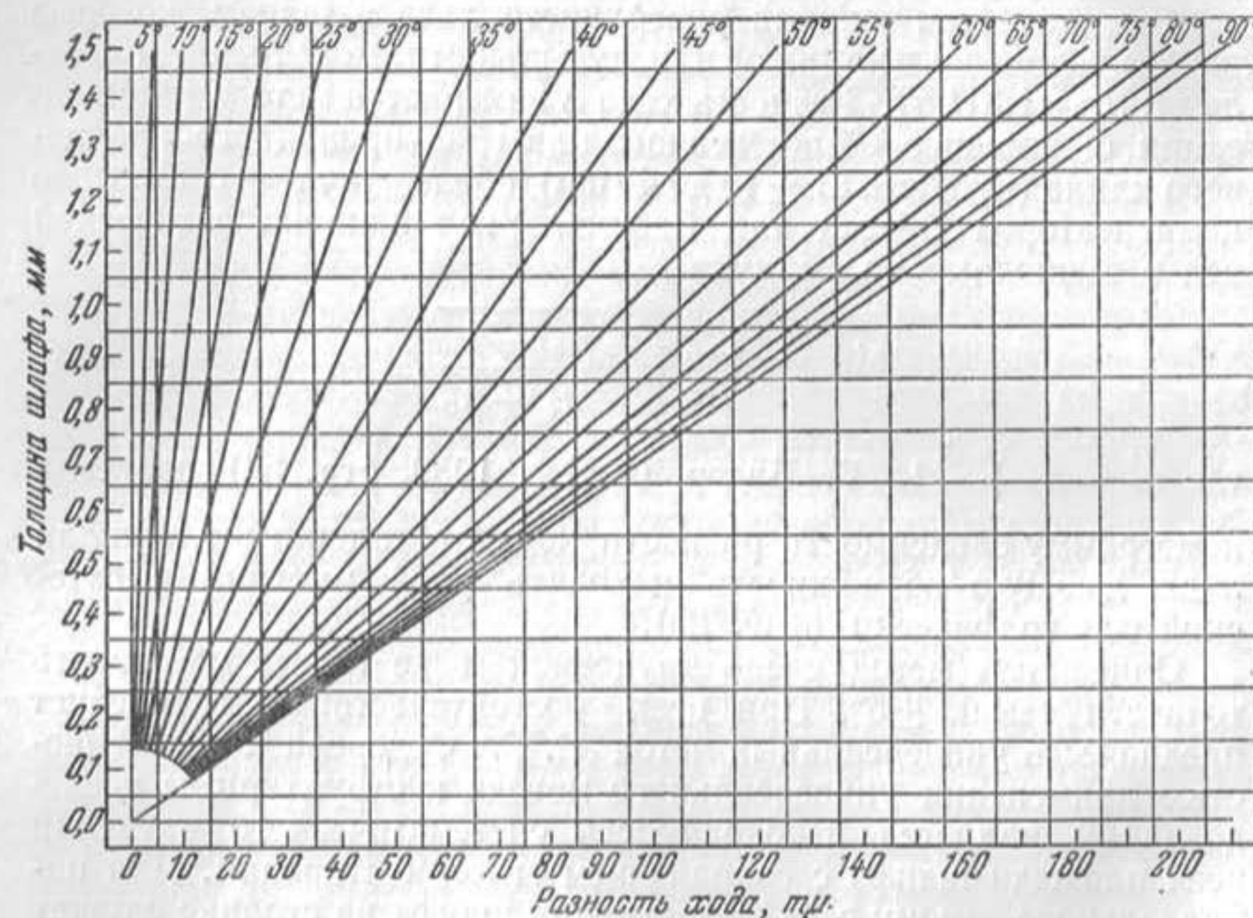
Фиг. 25. Зависимость разности хода обыкновенного и необыкновенного лучей от толщины шлифа льда.
