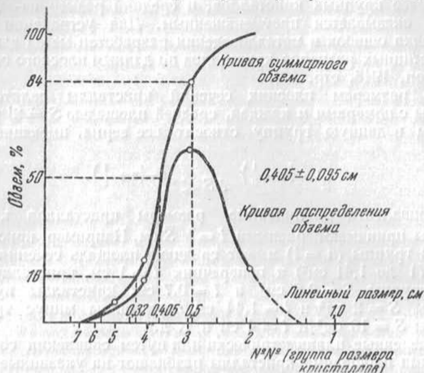
Фиг. 27. Кривые распределения общего объема породы между кристаллами разного линейного размера.
