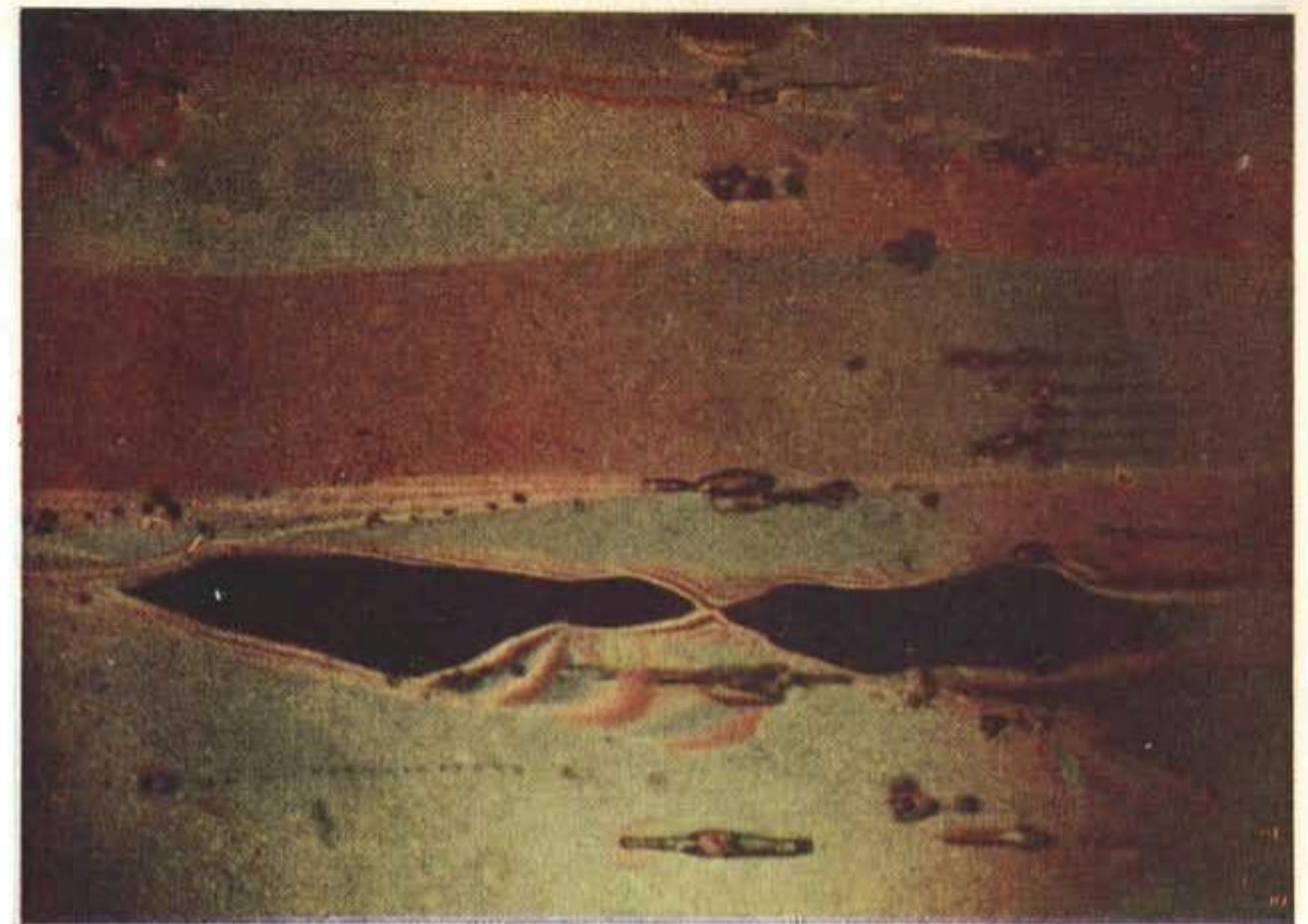
Фиг. 37. Призматически-зернистая структура конжеляционного льда (разрез в направлении роста) \times 6 . (Фото Б. А. Савельева)
