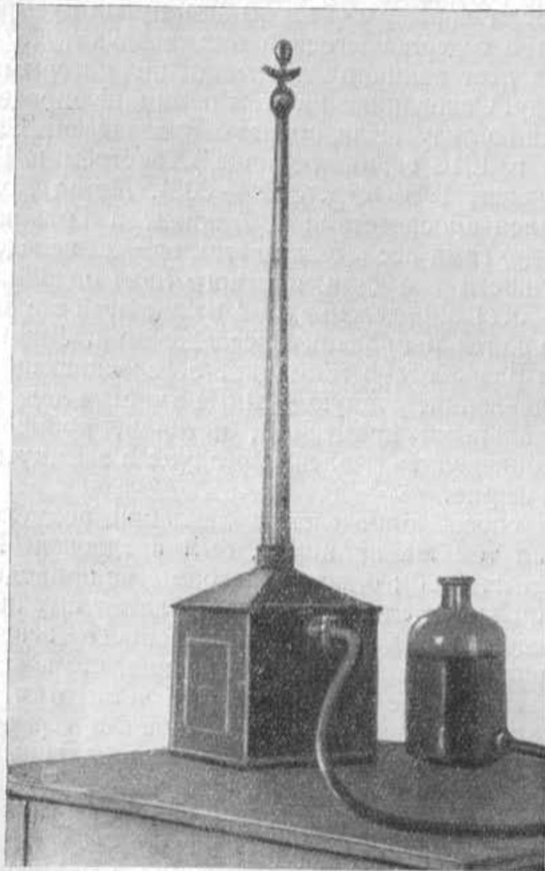
Фиг. 30а. Прибор для определения давления включенного во льду воздуха.
