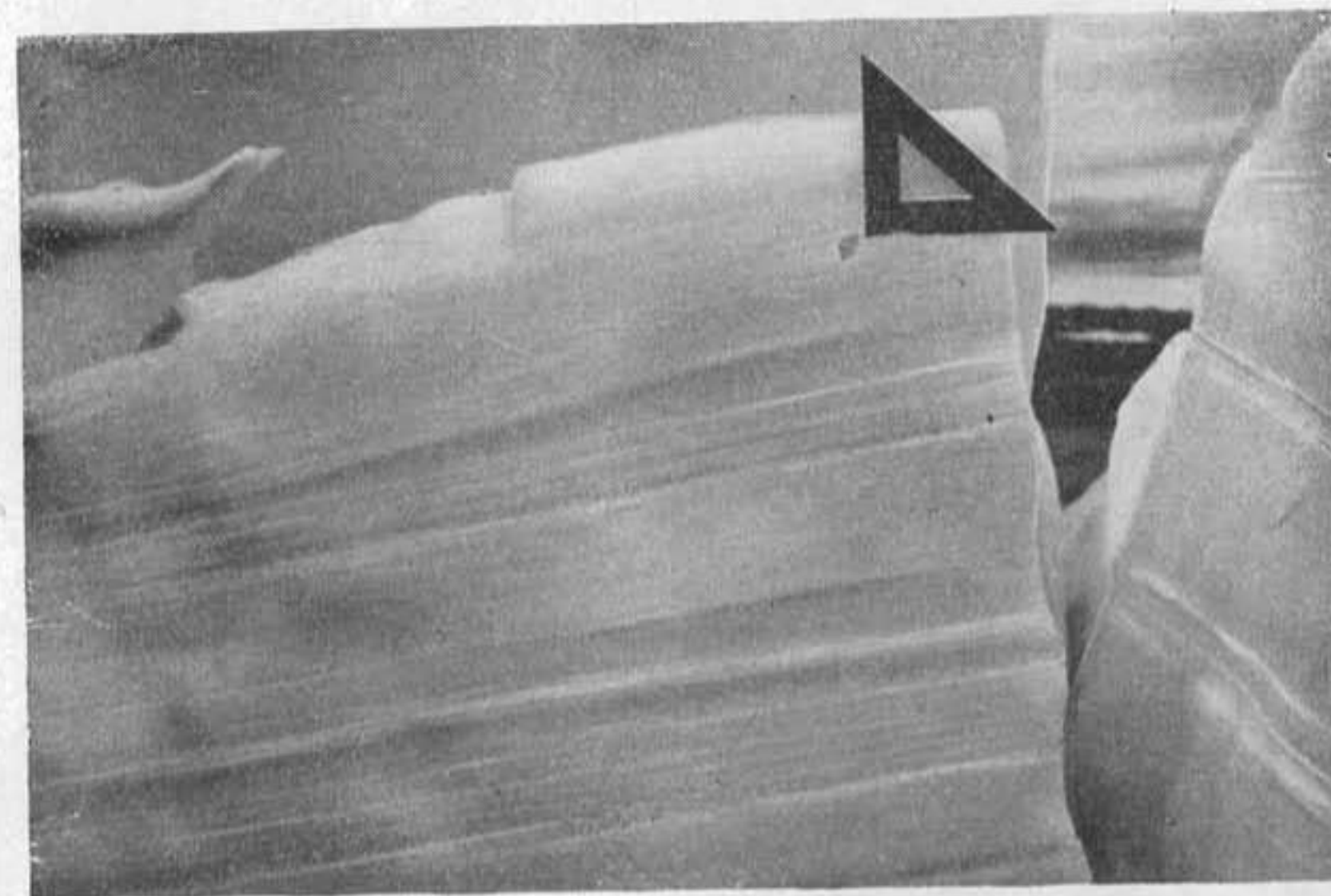
Фиг. 51. Слоистость натечного льда гидроэффузива.
