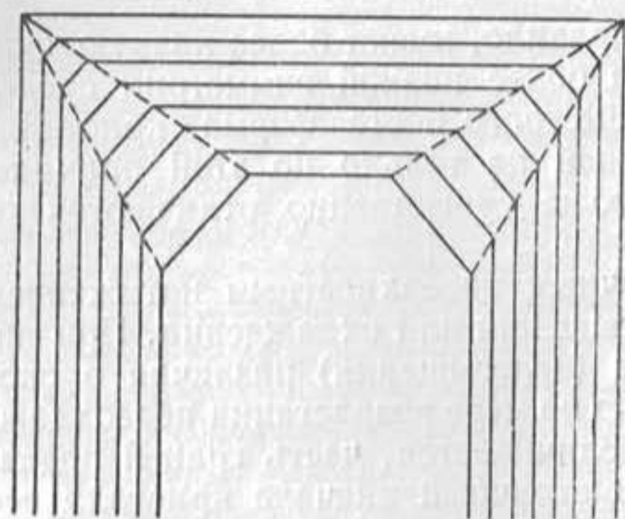
Фиг. 13. Исчезновение быстрее растущих граней кристалла.
