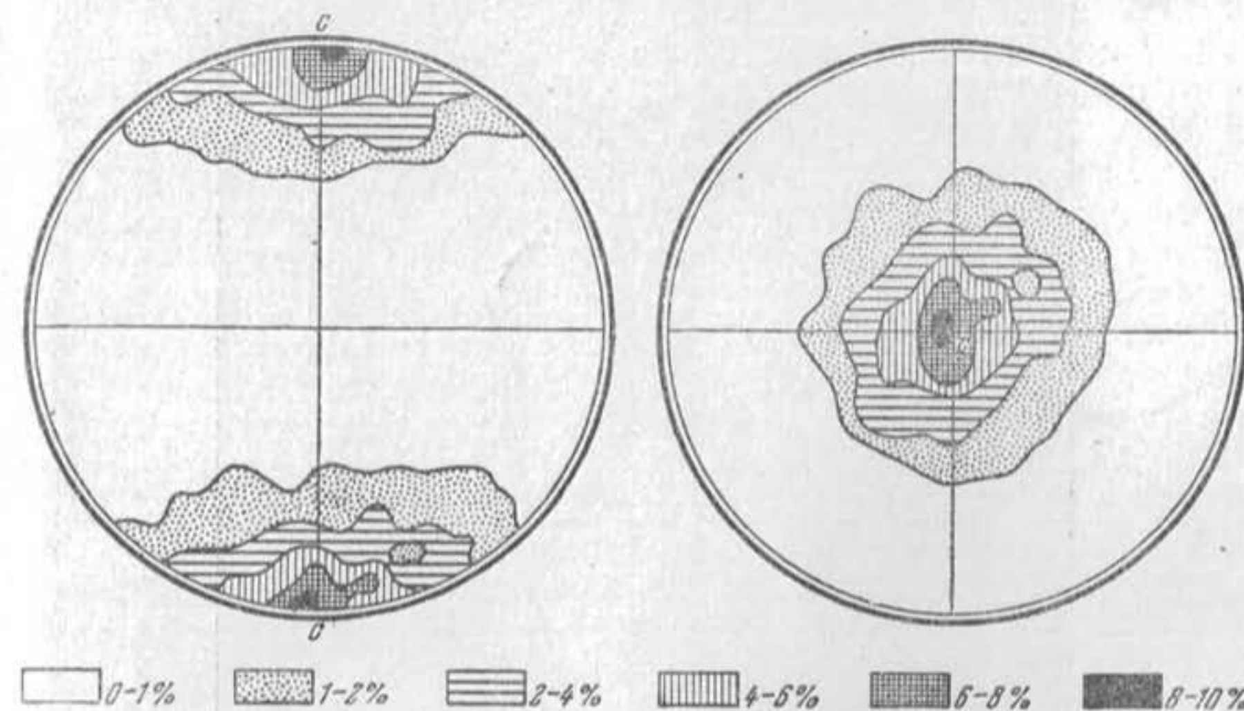
Фиг. 85. Стереограмма кристаллографической ориентировки инфильтрационно-конжеляционного льда (57 кристаллов).
