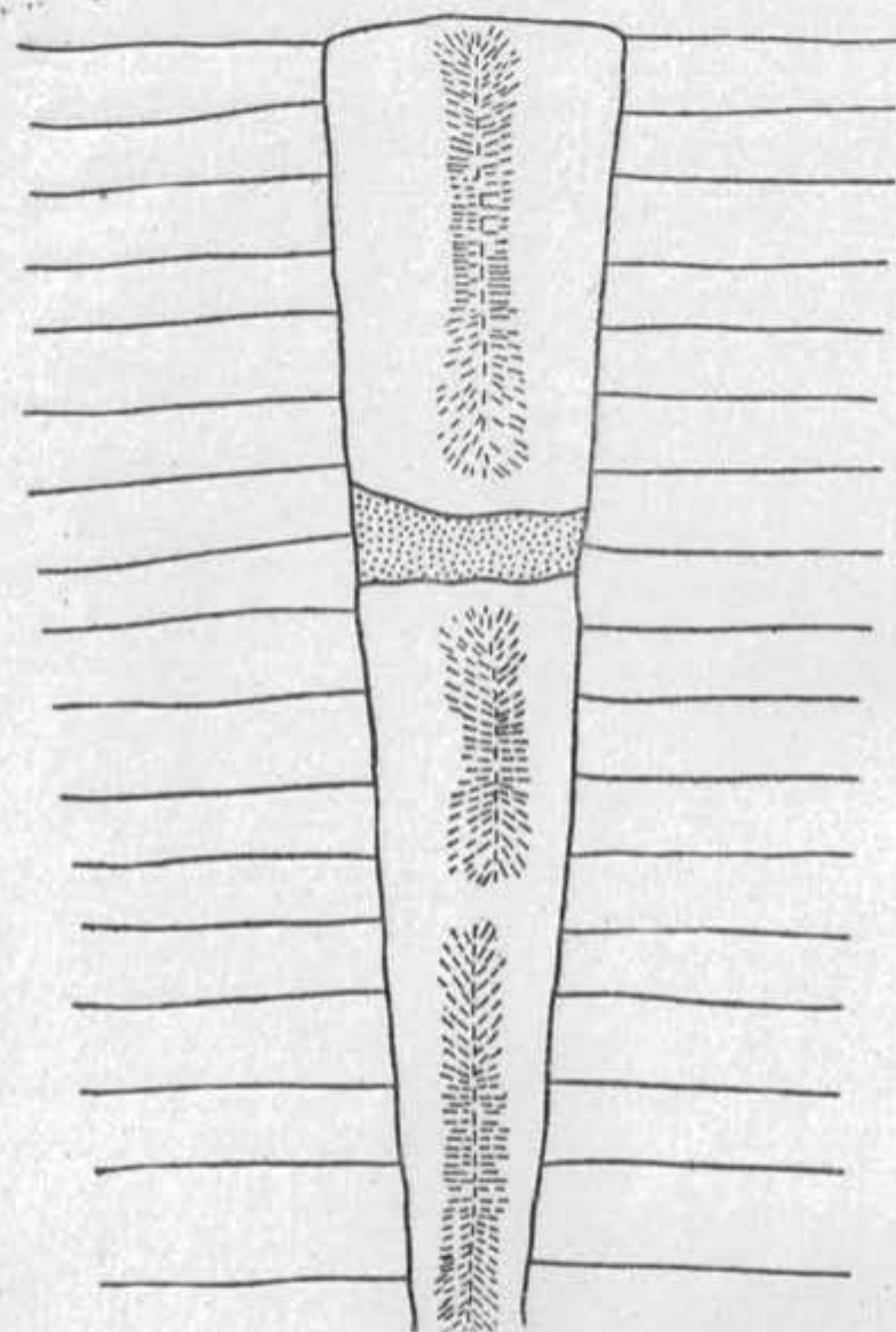
Фиг. 50. Схема строения трехэтажной ледяной жилы.
