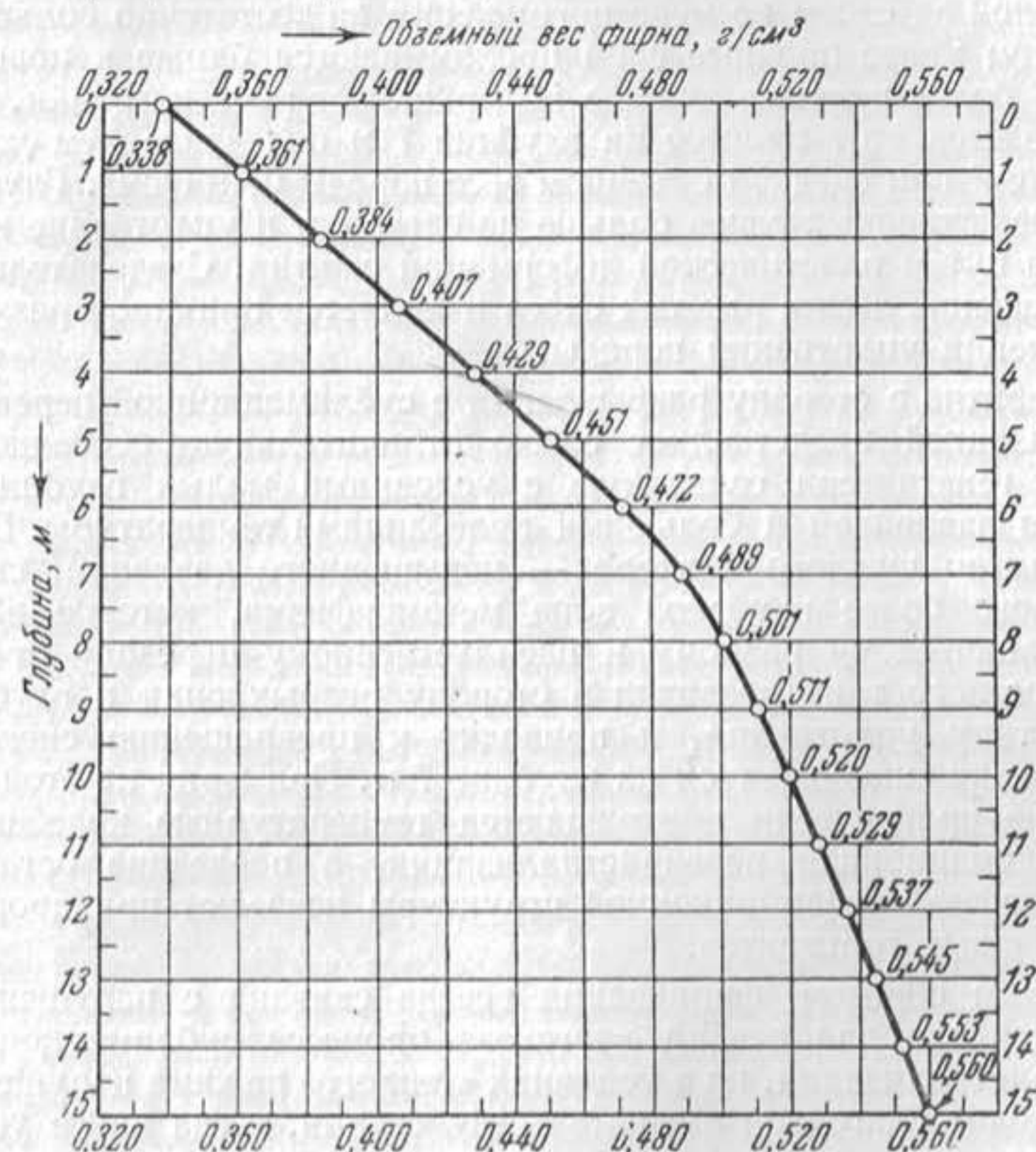
Фиг. 78. Кривая объемного веса снега и фирна по вертикальному профилю в центре Гренландии.
