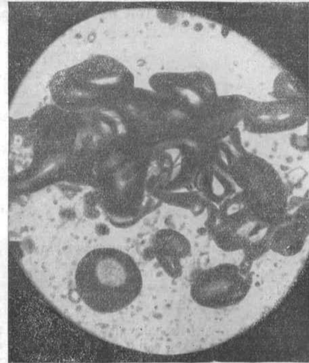
Фиг. 80. Форма пузырьков воздуха — остатков фирновых пор в инфильтрационно-рекристаллизационном льду. \times 15 .
