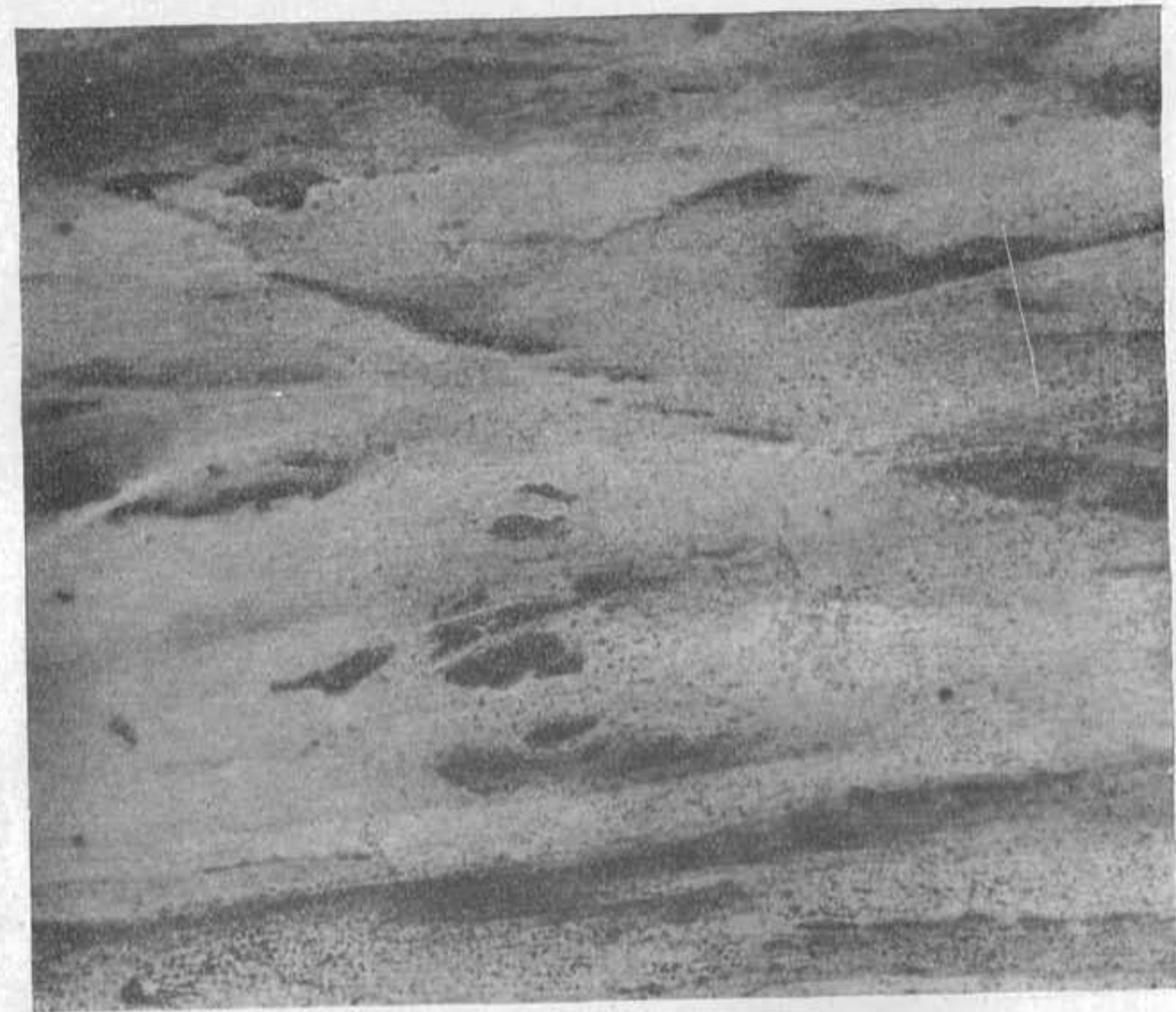
Фиг. 57. Слоистость повторно-жильного льда. Уменьш. в 1,8 раза (Фото Б. И. Втюрина)
