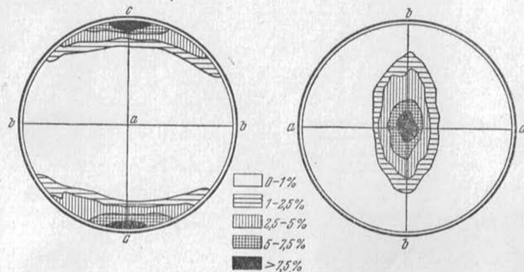
Фиг. 101. Стереогрaмма кристаллографической ориентировки льда, изображенного на фиг. 100
