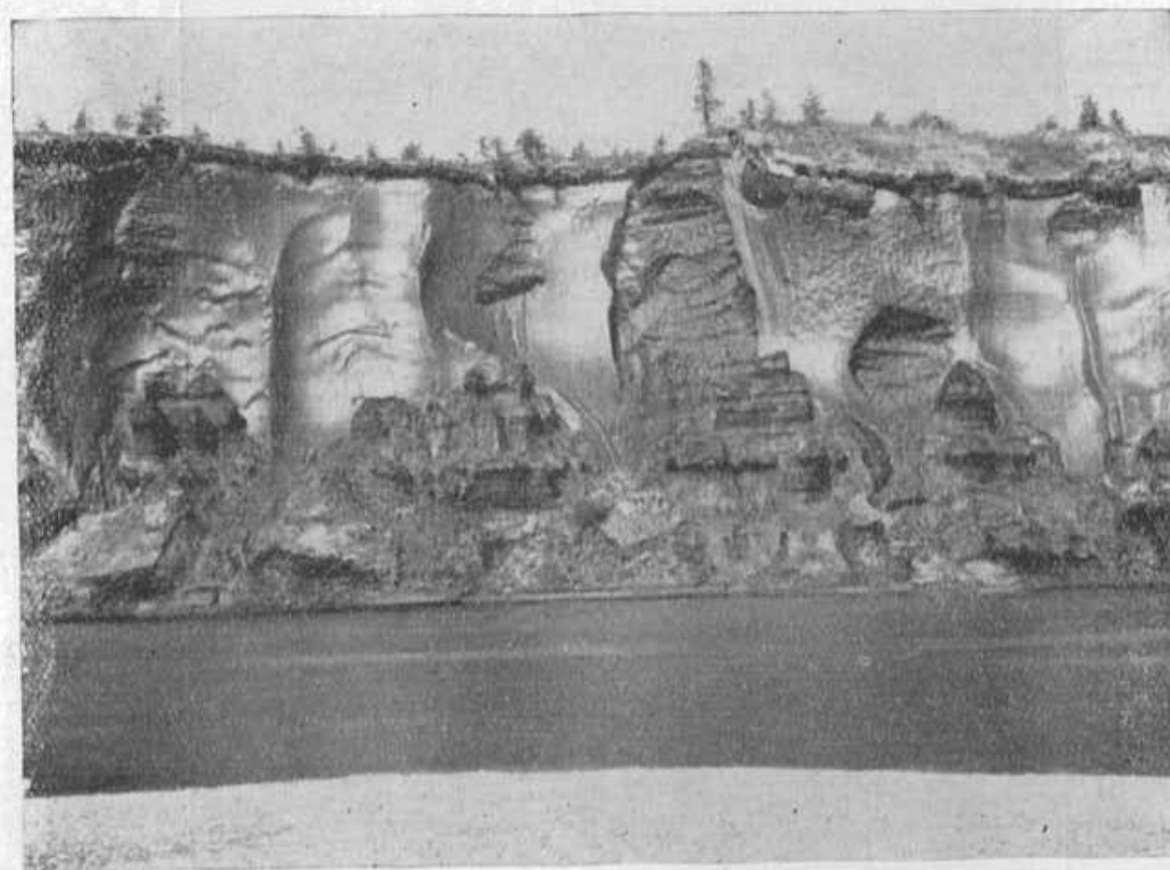
Фиг. 55. Формы выходов решетки сингенетических ледяных жил в том же обнажении, что и на фиг. 54. (Фото Е. М. Катасонова)
