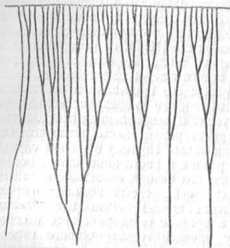
Фиг. 35. Схема структуры льда в зоне геометрического отбора.
