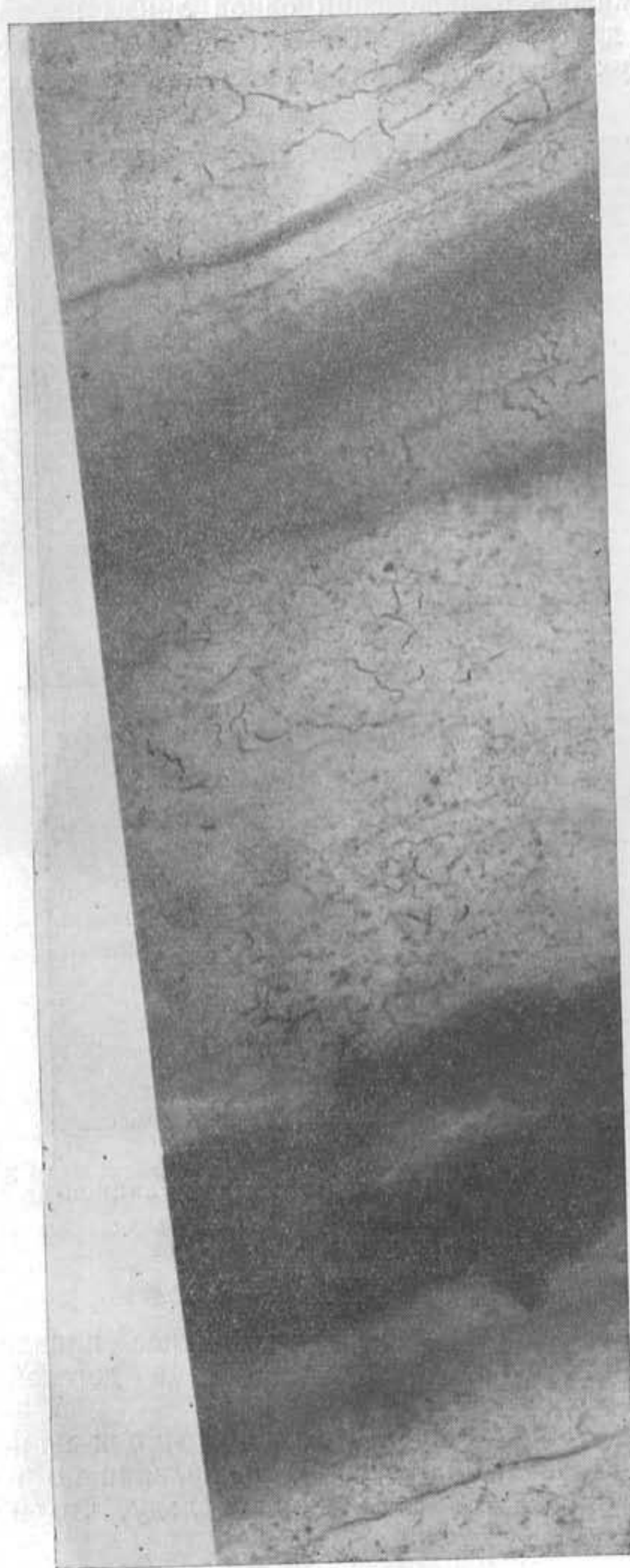
Фиг. 110. Сечение той же складки, что на фиг. 109, в плоскости ab . В одном крыле складки между моренными прослойками — конец режеляционной линзы, в другом крыле — небольшой валун. Уменьш. вдвое. (Фото Н. В. Черепанова)
