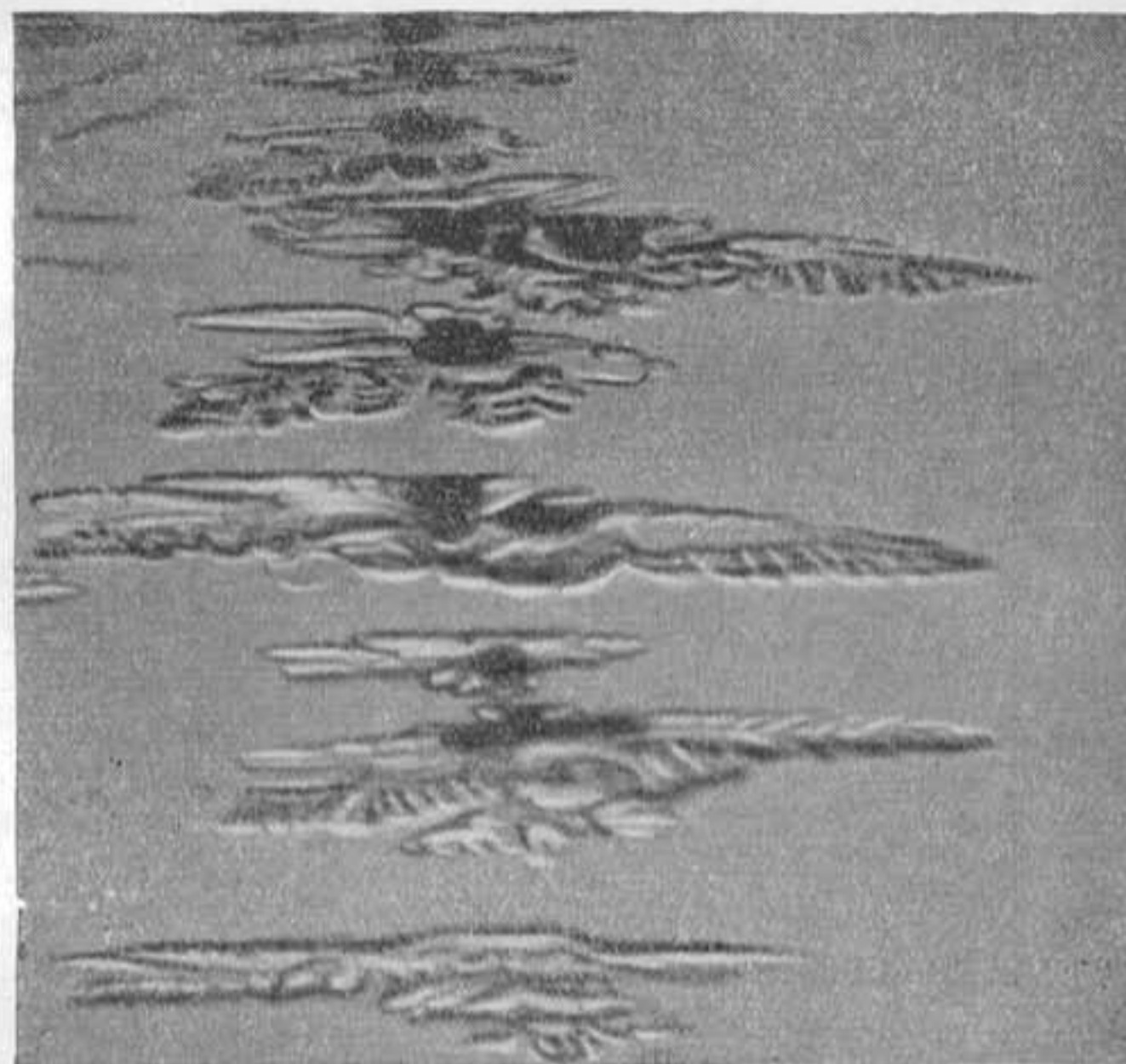
Фиг. 10. «Ледяные цветы» (вид сбоку). (Фото из Н. Schoentjes, 1905)
