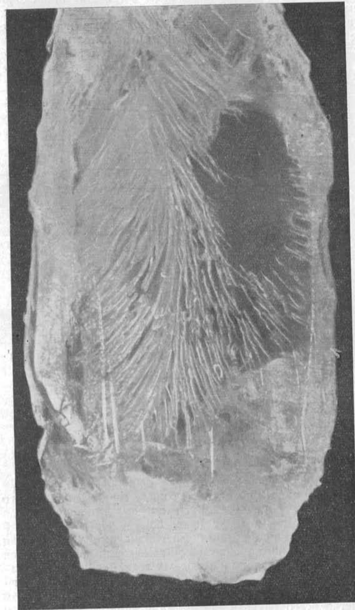
Фиг. 49. Веер трубчатых воздушных включений в жильном льду. Уменьш. в 4 раза. (Фото Н. В. Черепанова)
