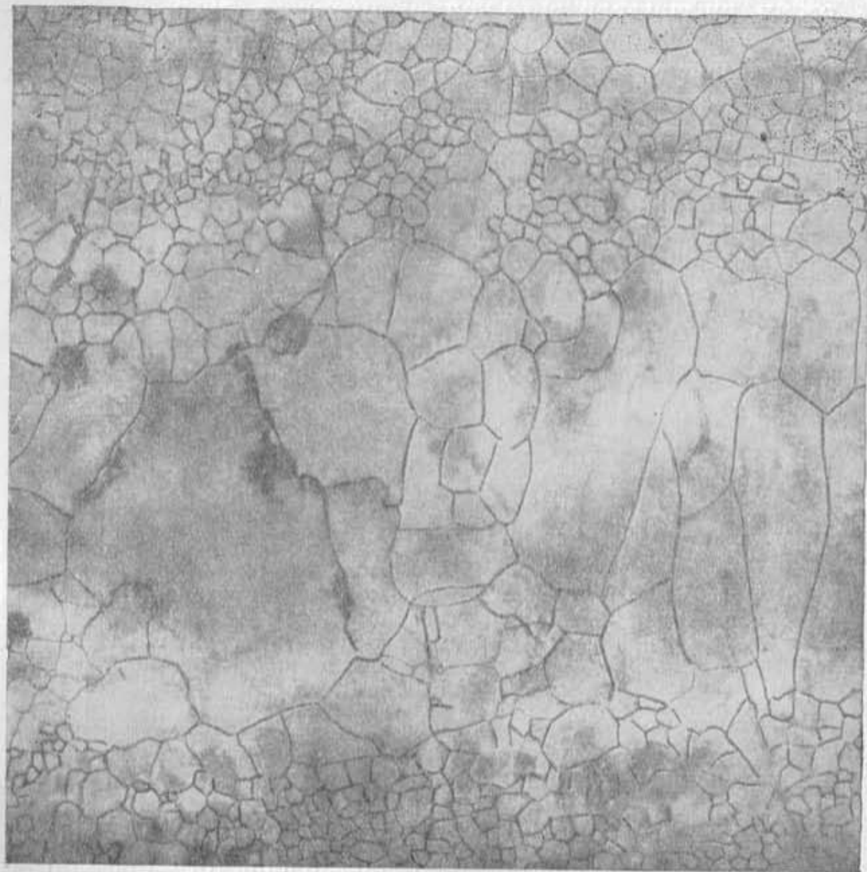
Фиг. 88. Гнезда инфильтрационно-конжеляционного льда среди инфильтрационного льда.
