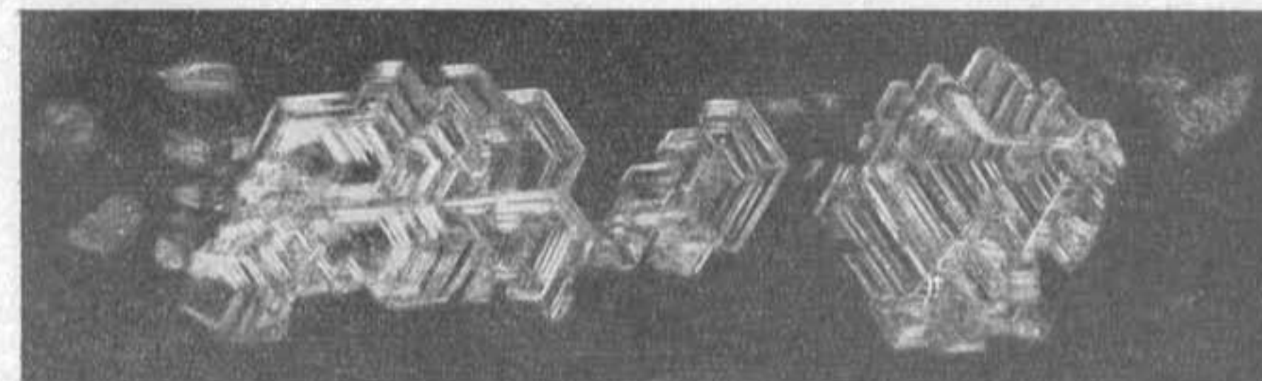
Фиг. 16. Сrostки пластинчатых кристаллов глубинной изморози из ледниковых трещин.
