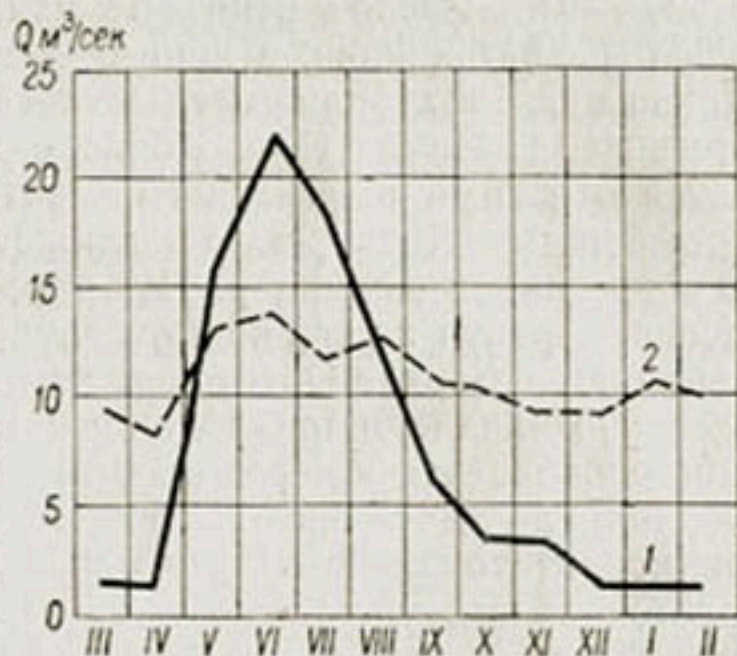
Рис. 158. Ход средних месячных расходов воды р. Кочкор в створах Верхней (1) и Нижней (2) станций.
