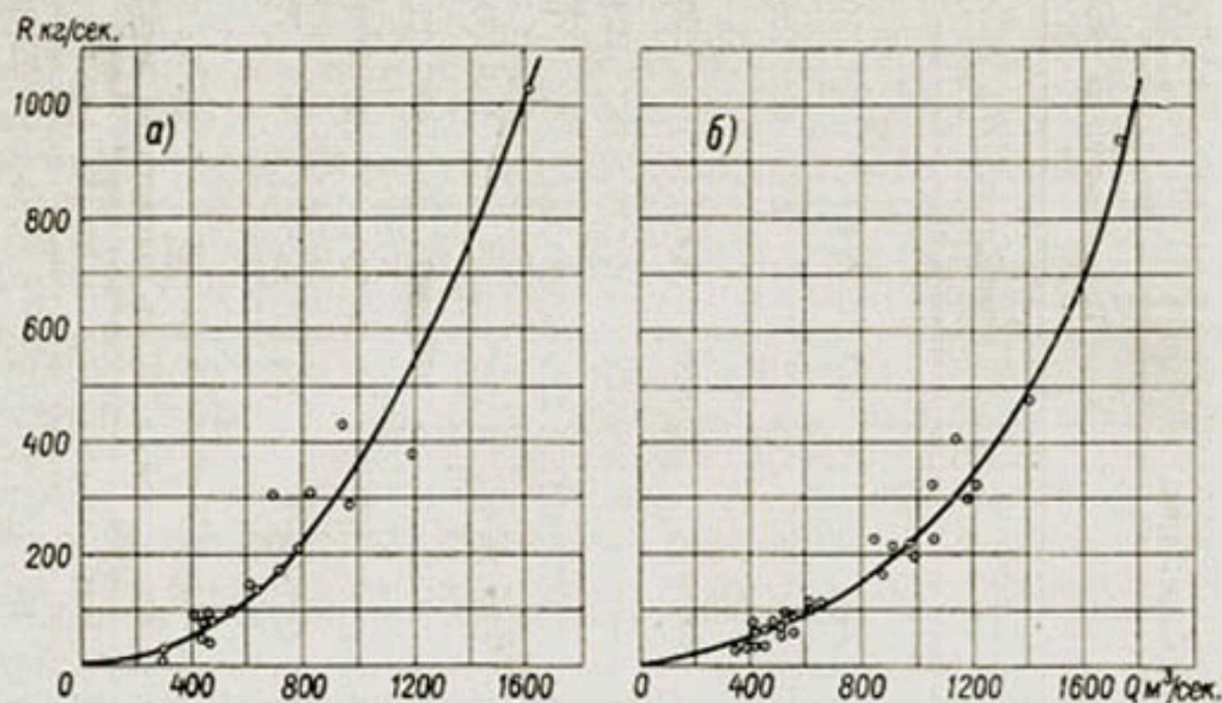
Рис. 148. Зависимость средних месячных расходов взвешенных наносов ( R ) от средних расходов воды ( Q ) Сыр-Дарьи у г. Беговат (ст. Запорожская). а — период подъема половодья, б — период максимальных расходов и спада половодья.
