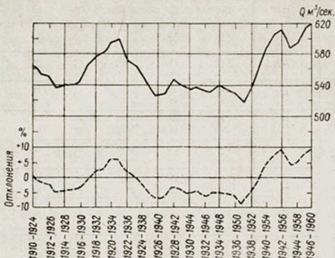
Рис. 146. Расходы Сыр-Дарьи у г. Беговат по скользящим 15-летиям и отклонения средних за 15-летия расходов воды в % от среднего за весь период наблюдений.
