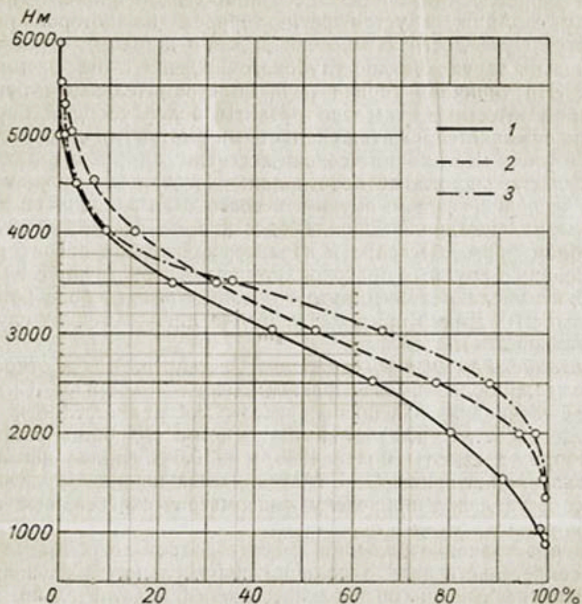
Рис. 130. Гипсометрические кривые бассейнов рек Зеравшан, Матча и Фандарья.
