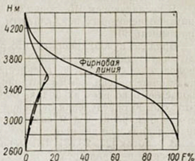
Рис. 15. Кривая распределения и гипсометрическая кривая площади оледенения в водосборе р. Сох (пунктирная прямая принята для расчетов стаивания от конца ледника к фирновой линии).
