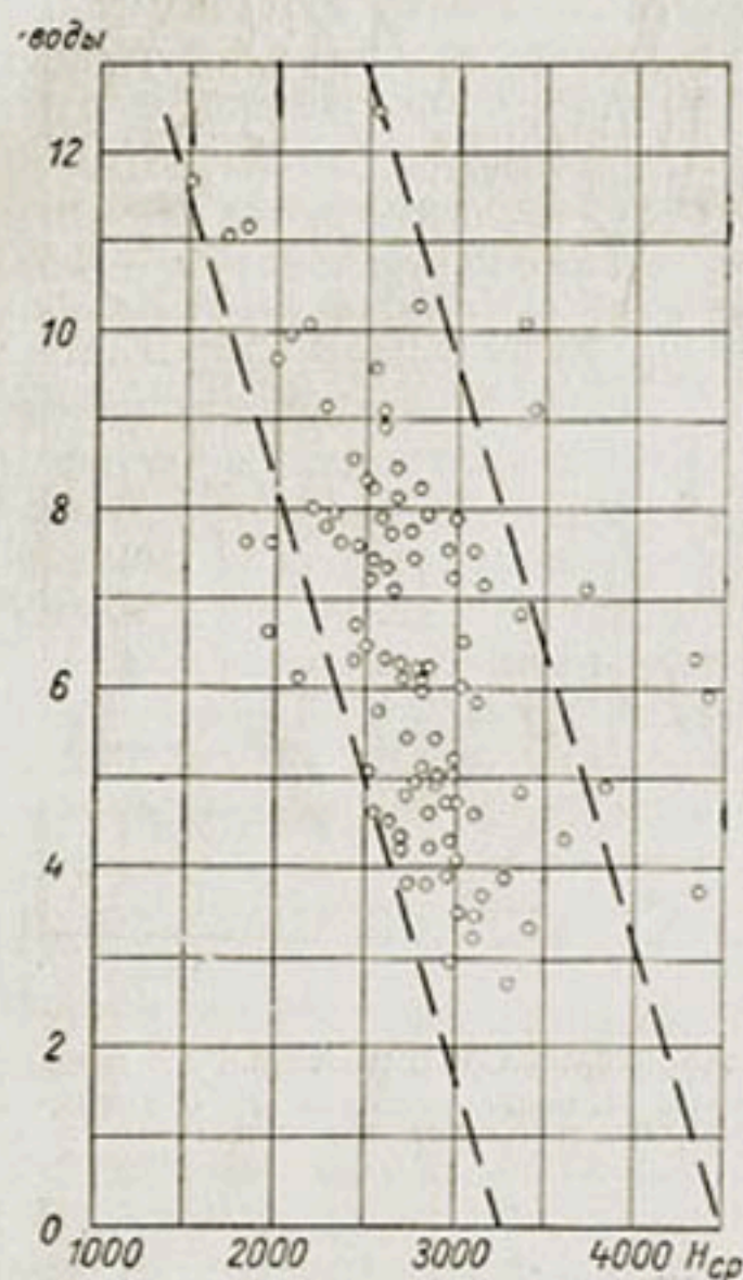
Рис. 89. Зависимость средней многолетней температуры воды от средней взвешенной высоты водосбора.
