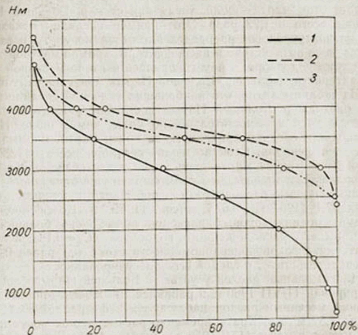
Рис. 134. Гипсометрические кривые водосборов.
