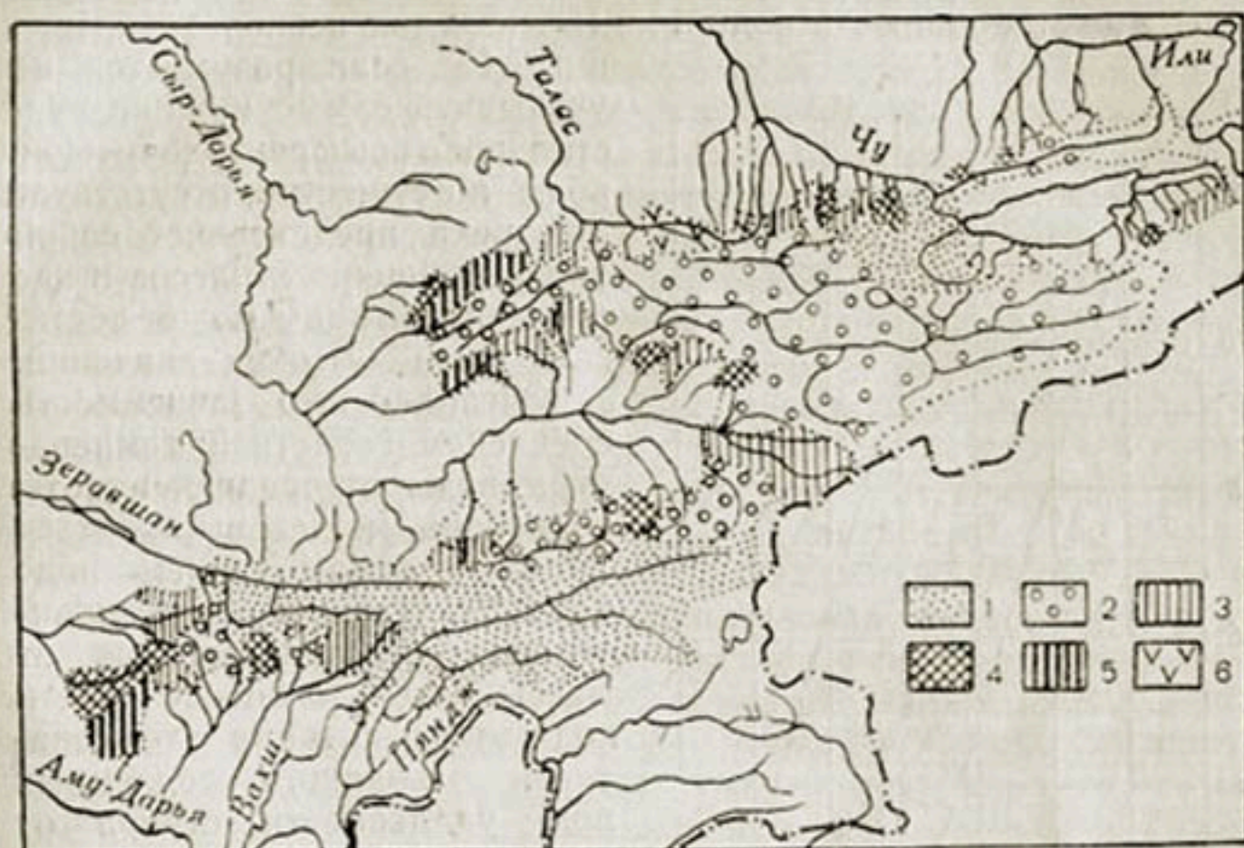
Рис. 88. Распределение коэффициентов вариации минимальных средних месячных расходов воды по территории Средней Азии.
