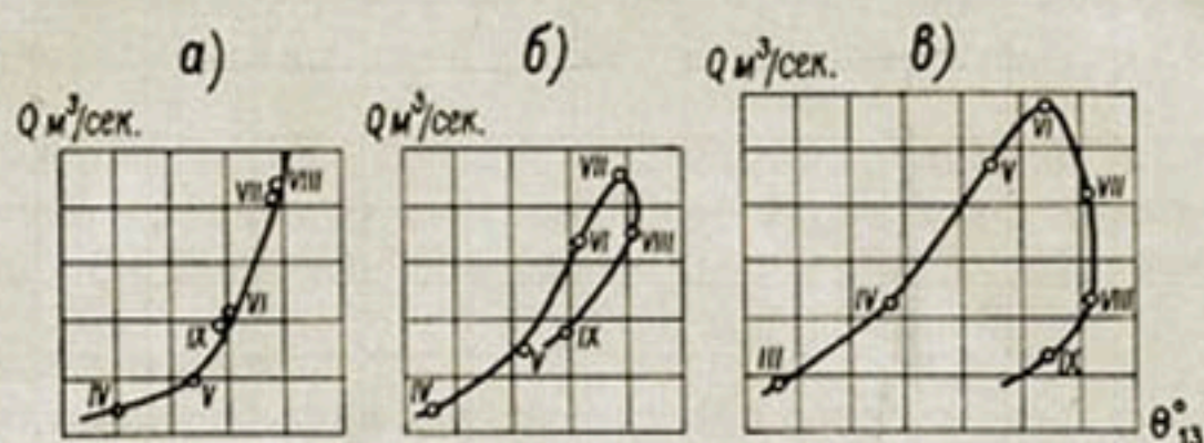
Рис. 34. Зависимость средних месячных расходов воды рек Исфара (а), Зеравшан (б), Чирчик (в) от средних месячных температур воздуха в 13 час.
