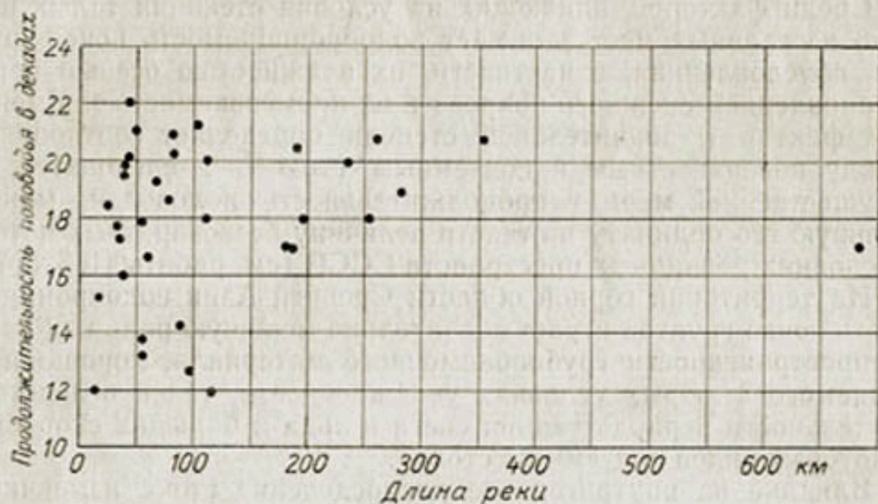
Рис. 63. Зависимость продолжительности половодья от длины реки.
