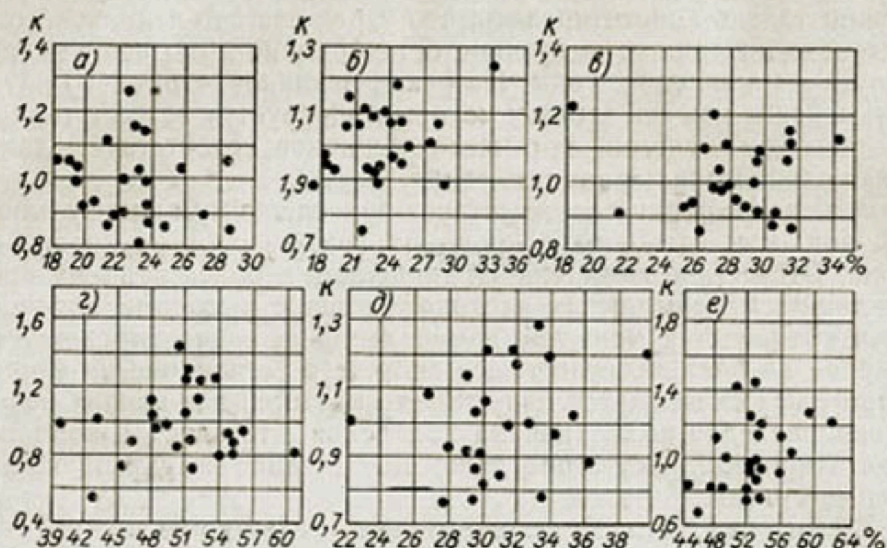
Рис. 64. Зависимость стока (в % годового стока) за период март—июнь от водности года (от модульного коэффициента средних годовых расходов k ).
