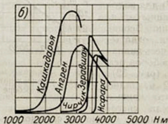
Рис. 52. Подобранные кривые тыла снеготаяния для водосборов рек Кашкадарья, Ангрен, Чирчик, Зеравшан и Исфара (а) и зависимость водности снежного покрова от высоты (б).
