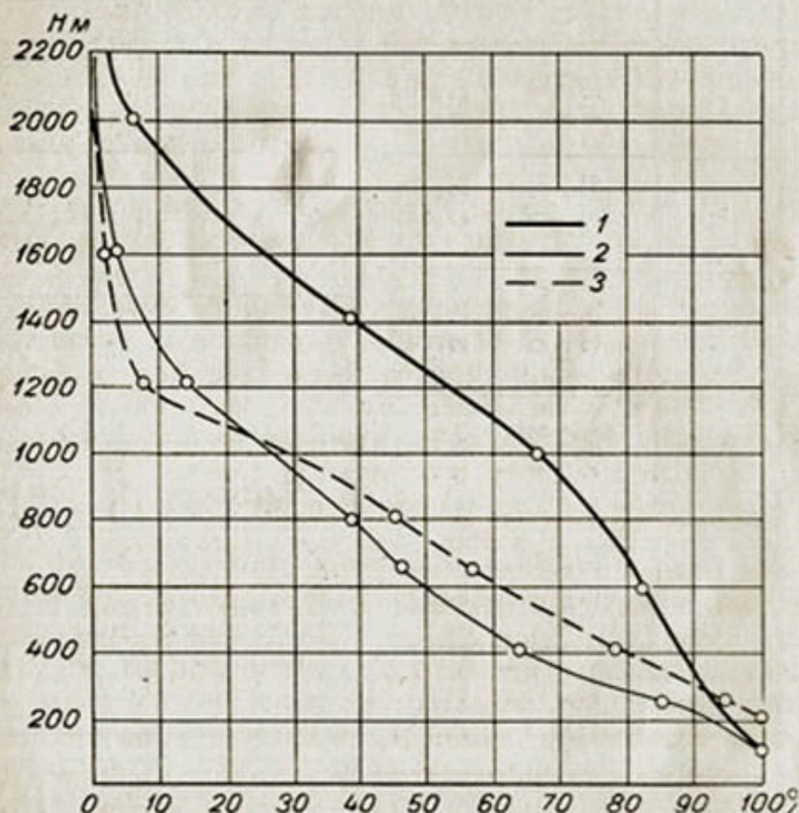
Рис. 101. Гипсометрические кривые водосборов рек Атрек (1), Сумбар (2) и Чандыр (3).
