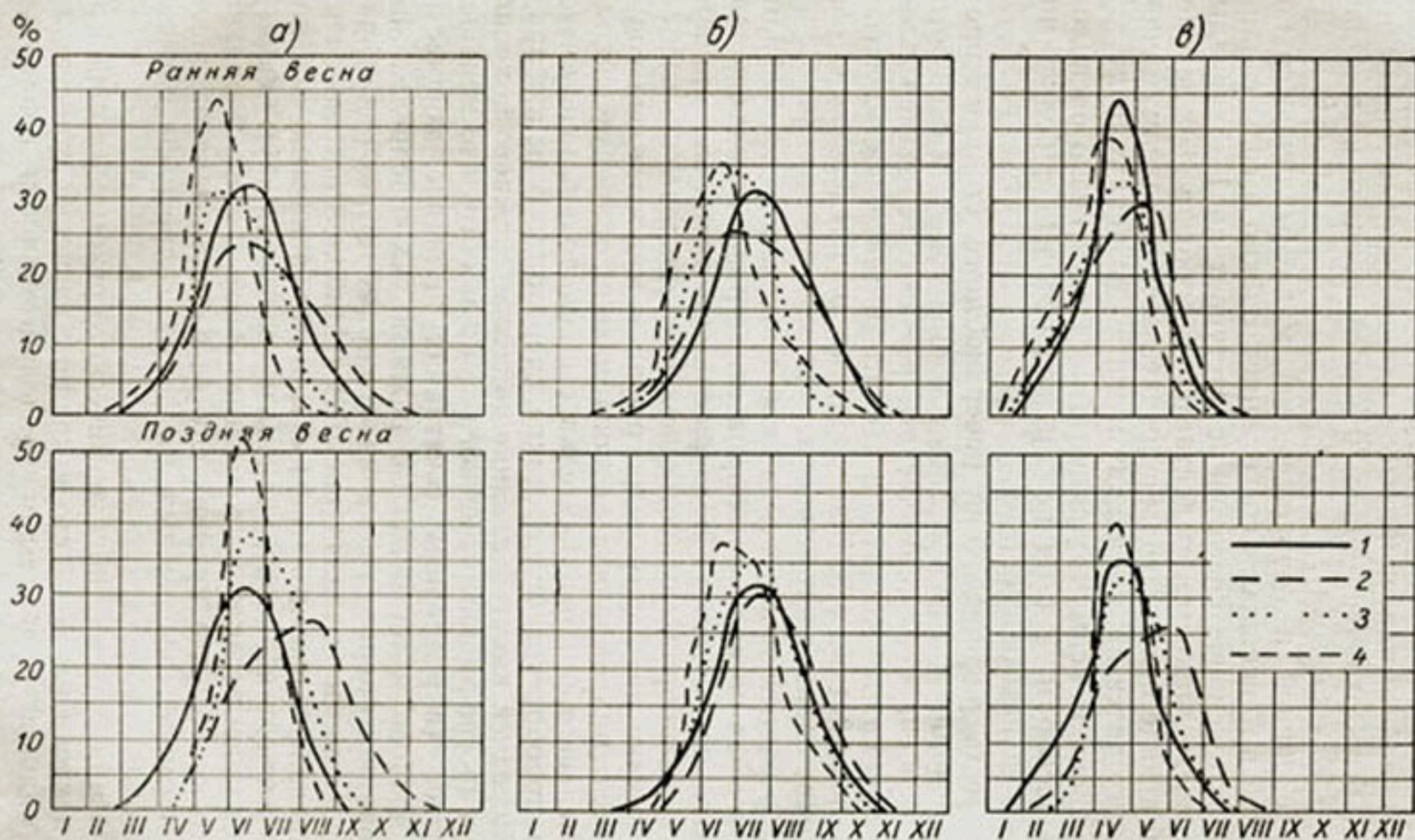
Рис. 62. Гидрографы талых вод рек при различном сочетании термического режима и водности снежного покрова.
