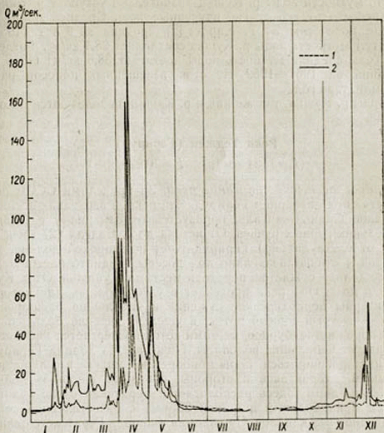
Рис. 106. Гидрографы р. Кашан у с. Кульджа (1) и р. Кушка в уроч. Палачная (2) за 1957 г.
