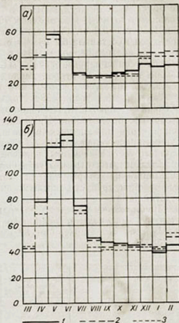
Рис. 105. Средние месячные расходы воды р. Мургаб в 1927-28 (а) и в 1934-35 гг. (б).
