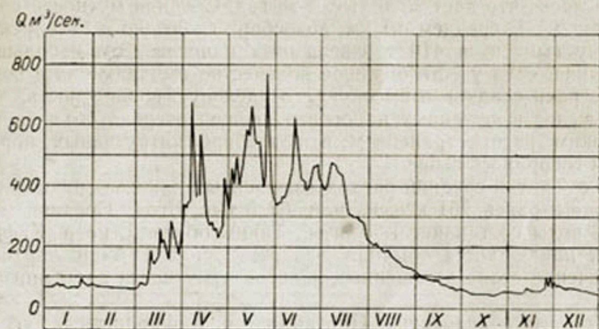
Рис. 129. Гидрограф р. Кафирниган у с. Айвадж за 1942 г.
