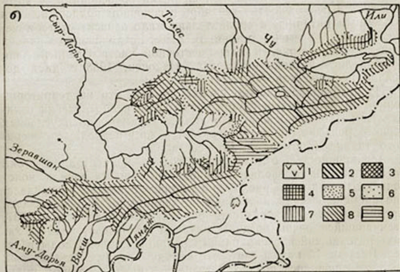
Рис. 69. Распределение концентрации стока (коэффициент a ) по территории Средней Азии.
