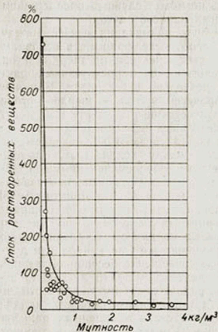
Рис. 95. Зависимость стока растворенных веществ (в % от стока взвешенных наносов) от мутности воды.
