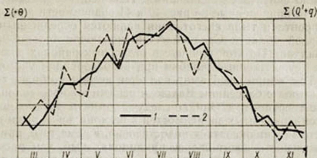
Рис. 42. Ход суммы средних декадных температур воздуха и прихода суммарной солнечной радиации за декаду в г. Ташкенте за 1949 г.
