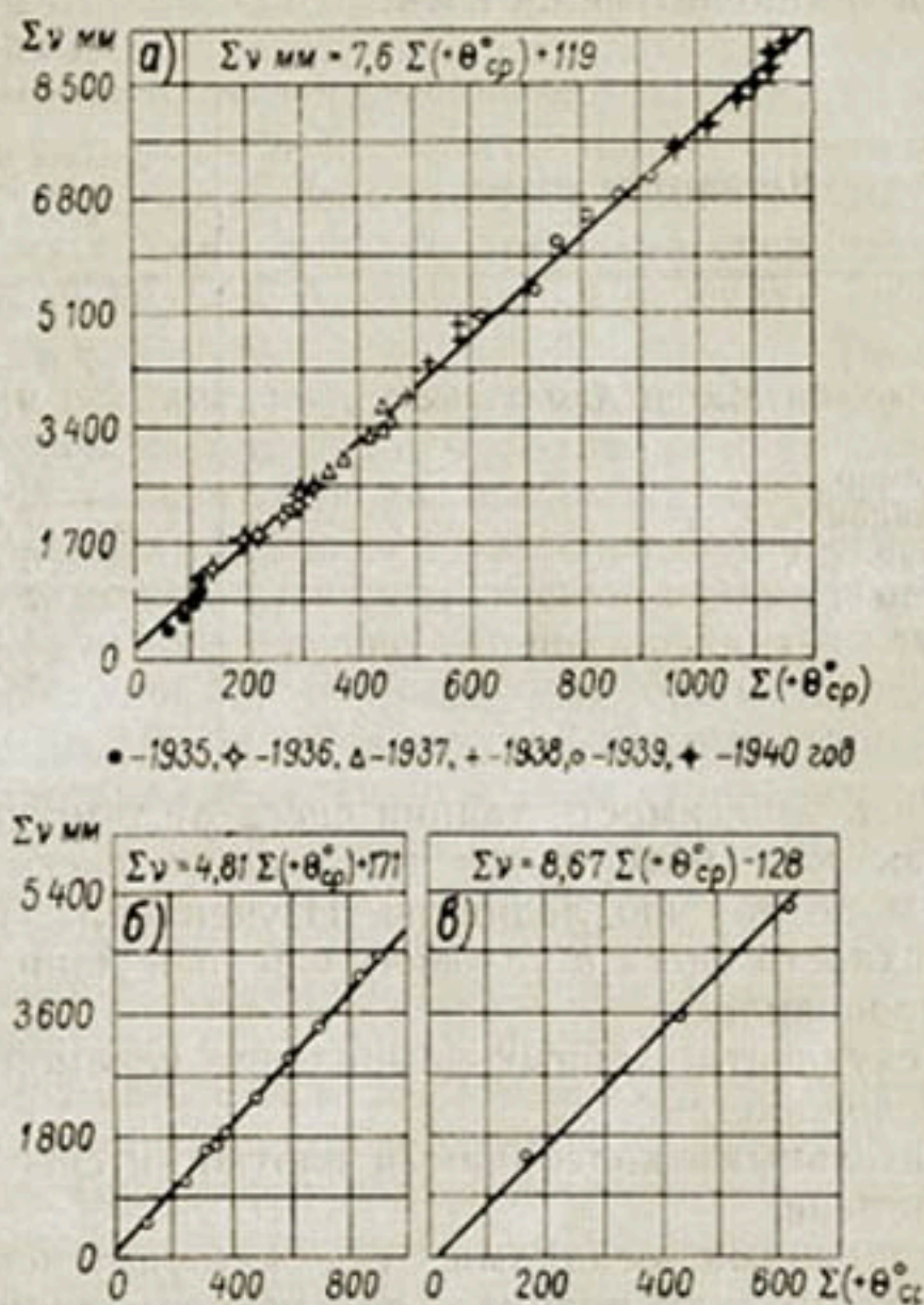
Рис. 44. Зависимость между стаиванием льда и суммами средних суточных температур воздуха на ледниках.
