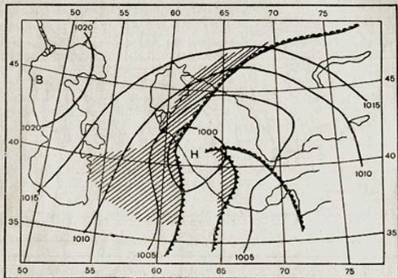
Рис. 5. Регенерация юго-западного циклона на арктическом фронте. синоптическая карта за 9 час. 9/II 1959 г.
