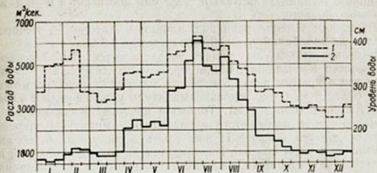
Рис. 127. Колебания средних декадных уровней (1) и расходов воды (2) Аму-Дарьи у с. Ташсака в 1934 г.
