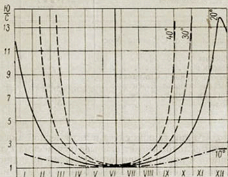
Рис. 48. Отношение прихода прямой солнечной радиации за день на южном склоне к приходу на северном склоне при крутизне склонов 10, 20, 30, 40°.
