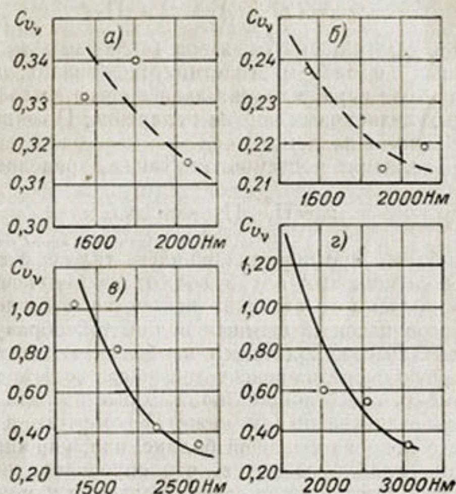
Рис. 27. Зависимость изменчивости водности снежного покрова ( C_{v_v} ) от высоты местности ( H ). а — р. Чаткал, б — Падшаата, в — р. Карадарья, г — Исфайрам.
