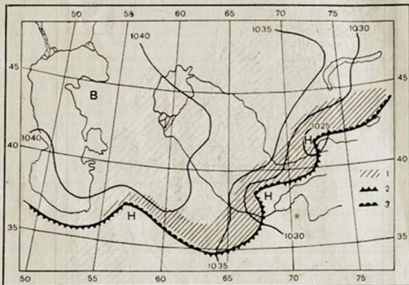
Рис. 3. Волновая деятельность на юго-востоке Средней Азии, синоптическая карта за 21 час 21/II 1954 г.
