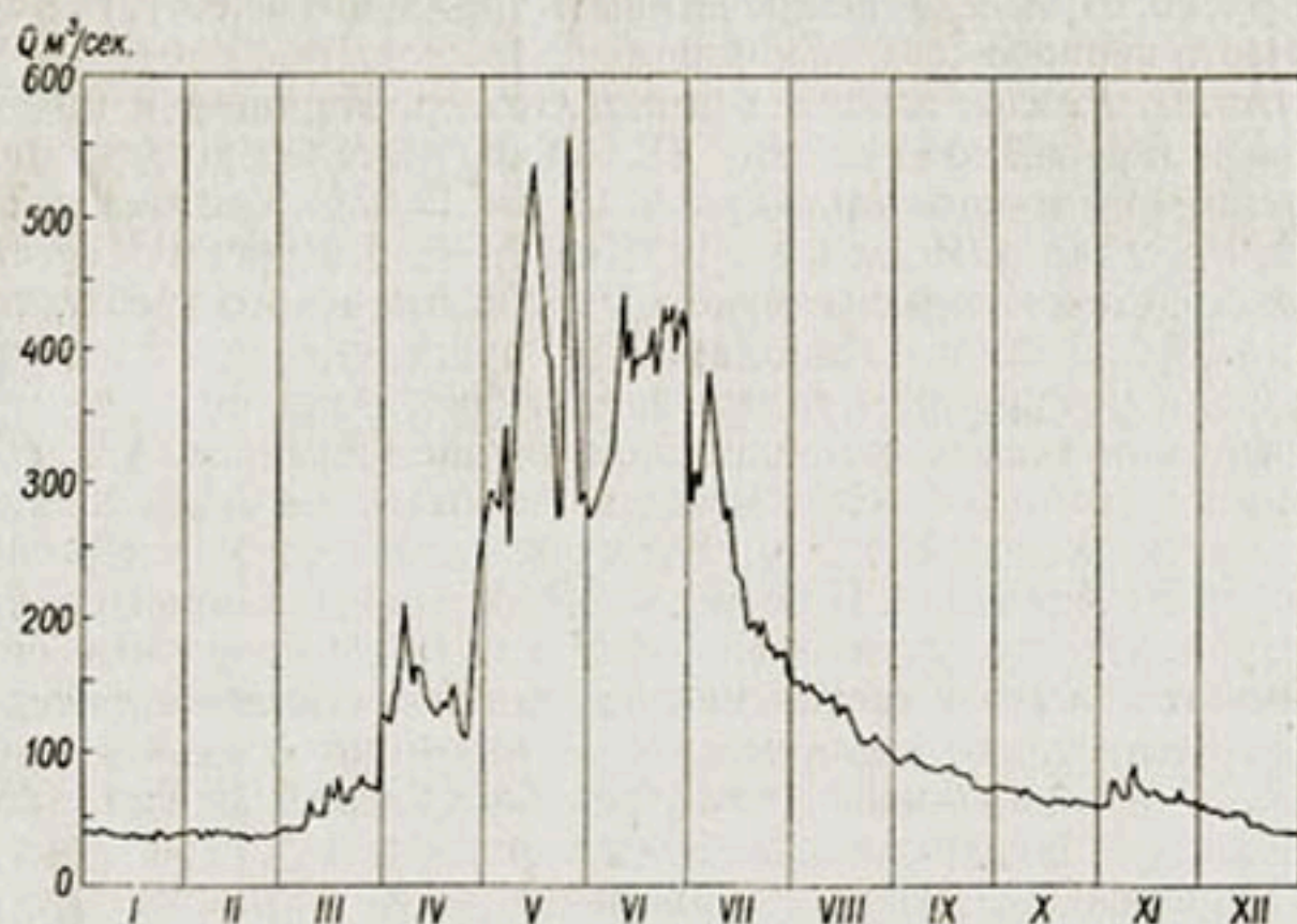
Рис. 142. Гидрограф р. Карадарья у с. Кампыррават за 1942 г.
