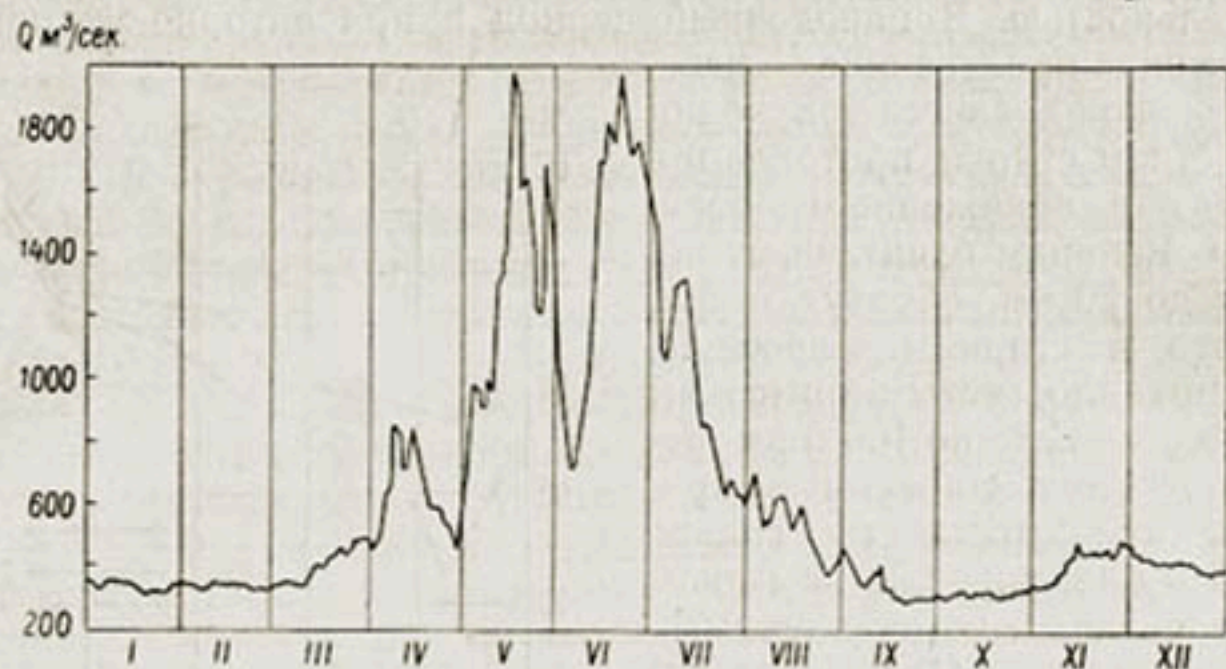
Рис. 145. Гидрограф Сыр-Дарьи у г. Беговат за 1942 г.
