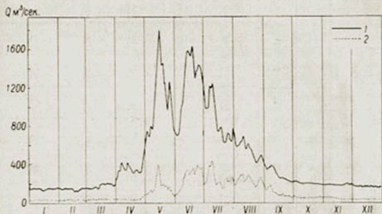
Рис. 136. Гидрографы р. Нарын за 1942 г. 1 — у г. Учкурган, 2 — у г. Нарын.
