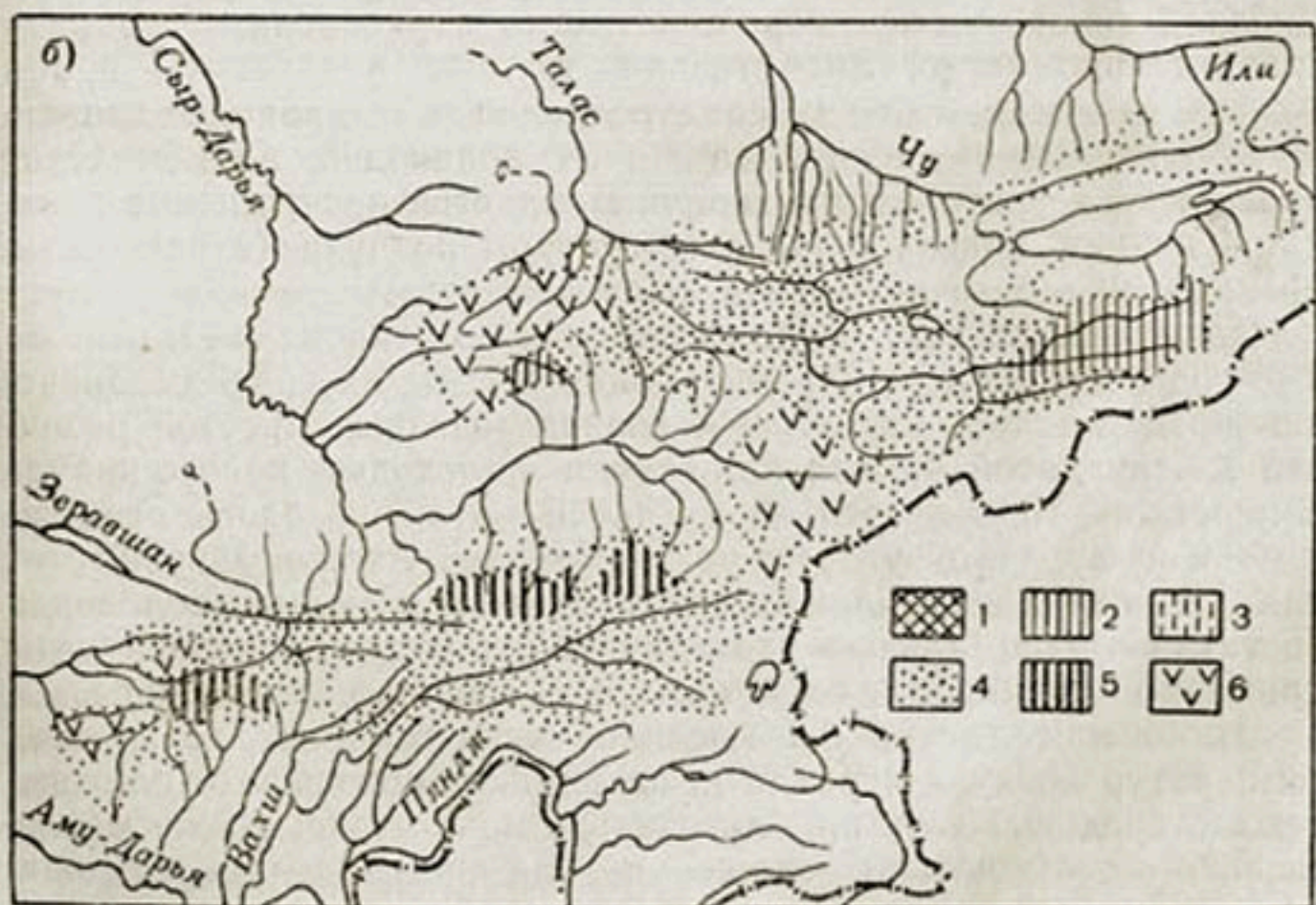
Рис. 70. Распределение времени начала половодья по территории Средней Азии.
