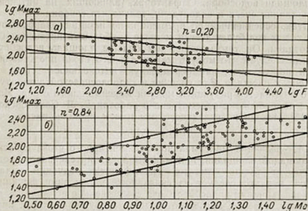
Рис. 73. Зависимость модулей максимального стока от площадей водосборов (а) и средних модулей стока (б).
