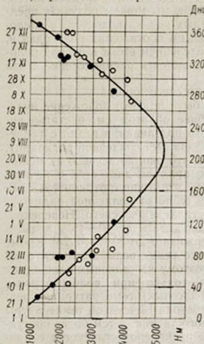
Рис. 40. Зависимость среднего времени перехода температур воздуха в 13 час. через 0^{\circ} (положения фронта снеготаяния) от высоты местности.
