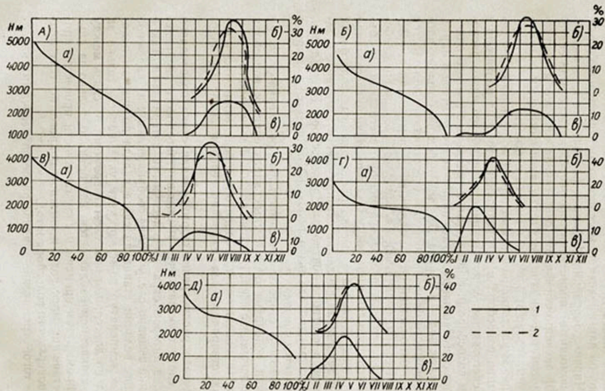
Рис. 53. Гипсометрические кривые (а), гидрографы талых вод (б) и площади возможного одновременного снеготаяния (в).
