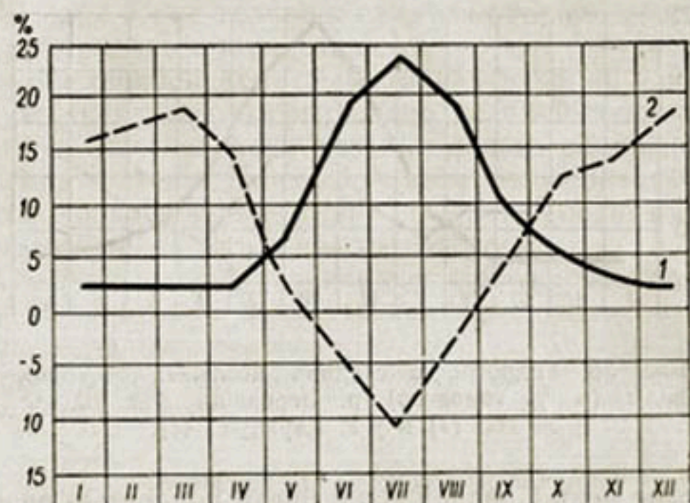
Рис. 37. Ход величин месячного стока (в % годового) р. Зеравшан при выходе из гор (1) и возвратных вод (2).
