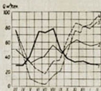
Рис. 161. Ход средних месячных расходов воды р. Чу в 1940-41 г. 1 — с. Джильарык, 2 — с. Чумыш, 3 — с. Ташуткул, 4 — с. Фурмановка.
