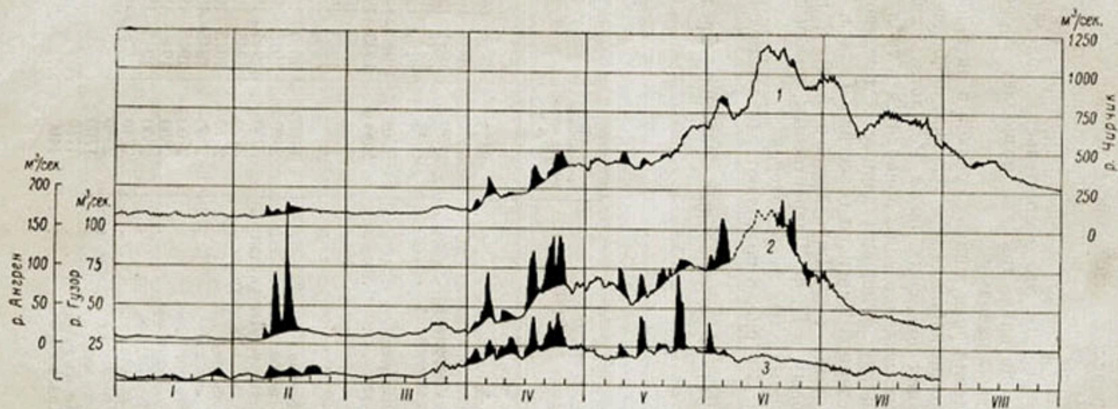
Рис. 8. Ход срочных расходов воды за 1933-34 г. с выделением дождевого питания.
