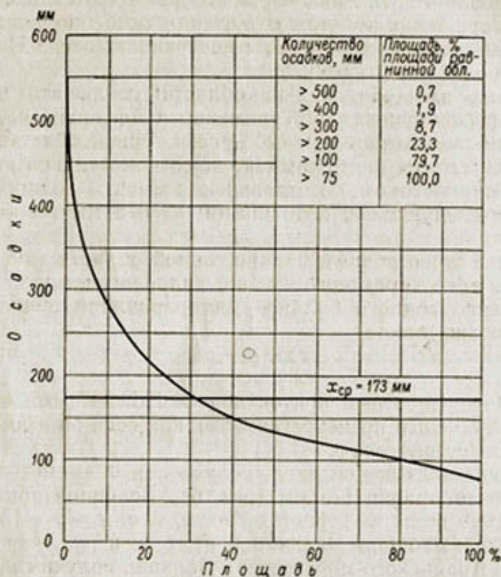
Рис. 6. Кривая обеспеченности годовых сумм осадков для равнинной области Средней Азии.
