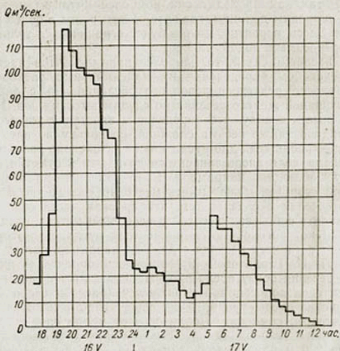
Рис. 78. Гидрограф селя на Каттасае у г. Уратюбе в мае 1939 г.
