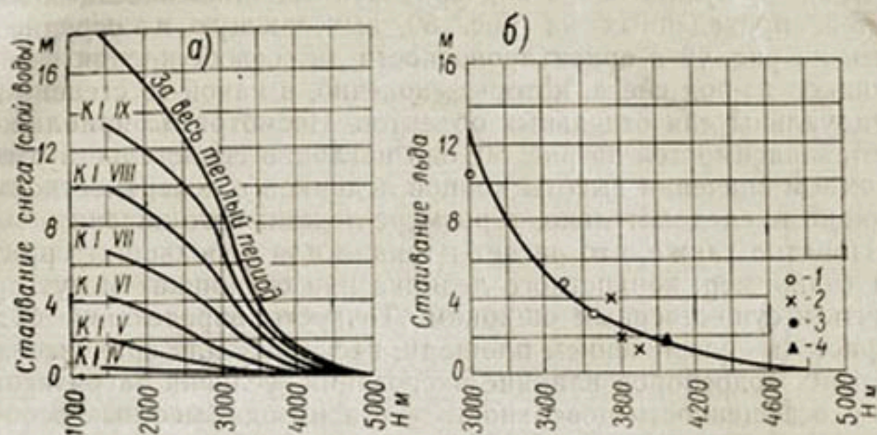
Рис. 50. Возможное стаивание снега в зависимости от времени и высоты местности (а) и стаивание льда за теплый период в зависимости от высоты (б).
