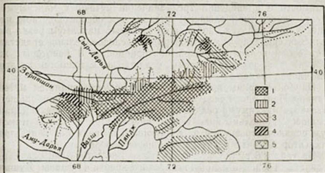
Рис. 75. Распределение коэффициентов вариации максимальных расходов воды по территории Средней Азии.
