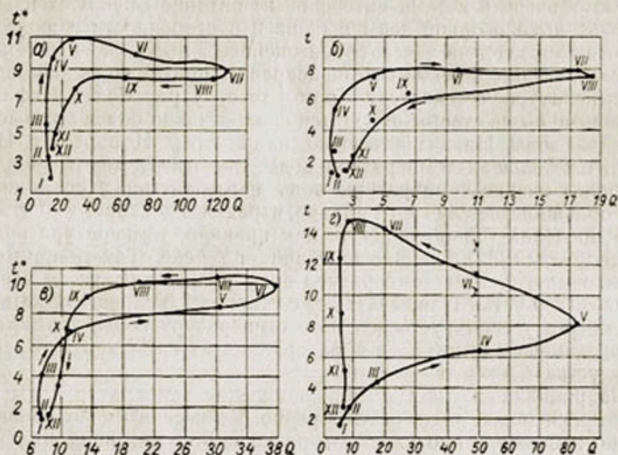
Рис. 90. Зависимость средних месячных температур воды от расхода воды.
