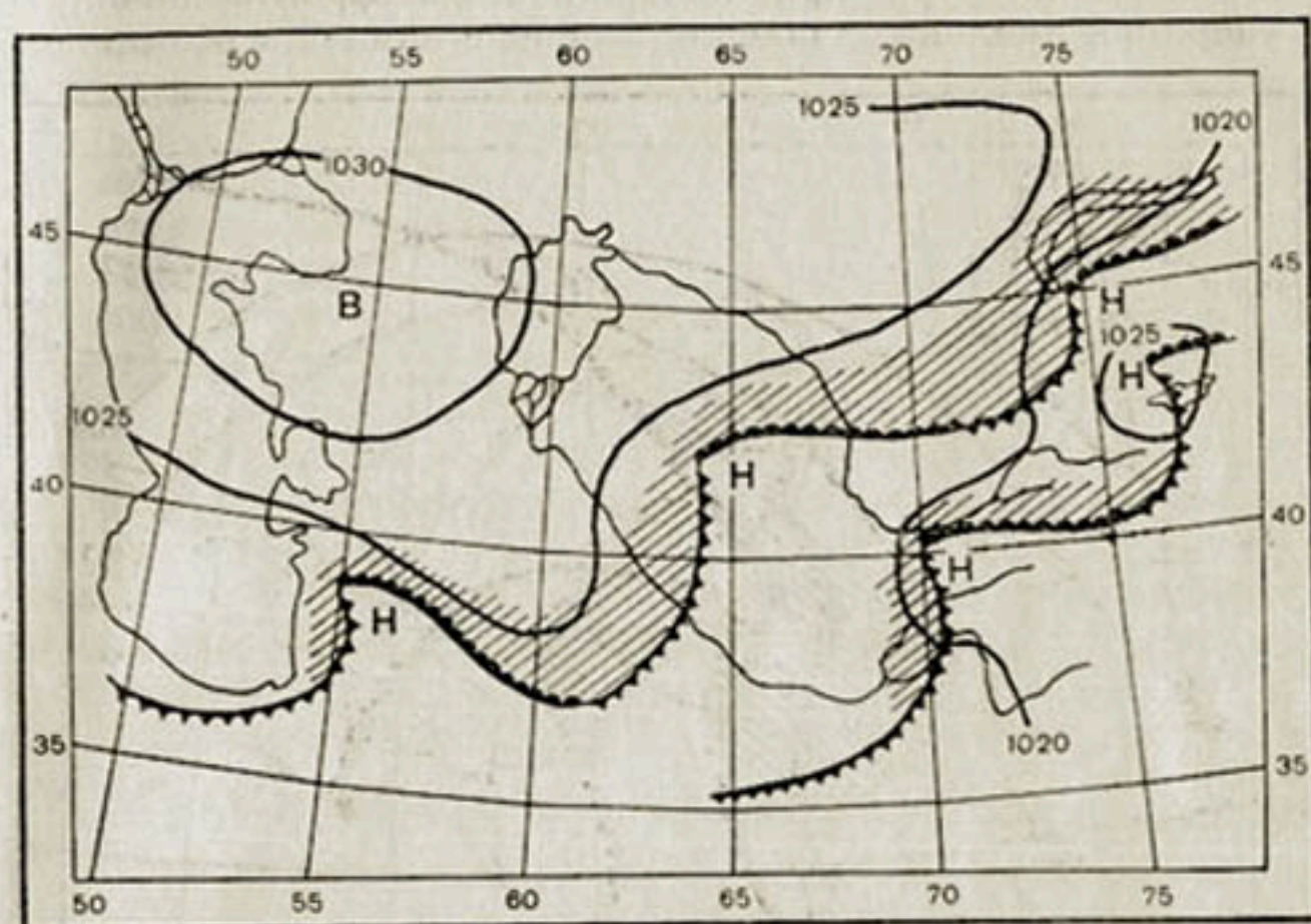
Рис. 4. Волновая деятельность на юго-востоке Средней Азии, синоптическая карта за 9 час. 24/1 1950 г.
