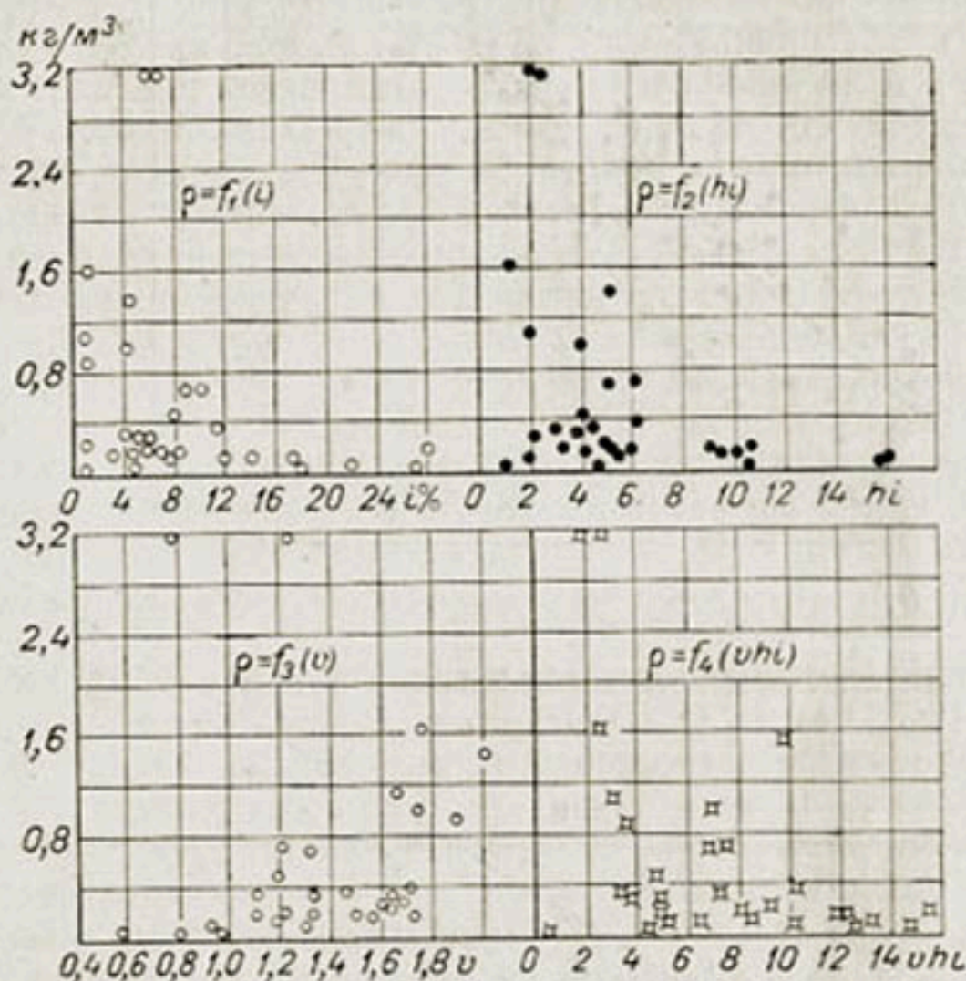
Рис. 93. Зависимость относительной мутности от гидравлических элементов русла.
