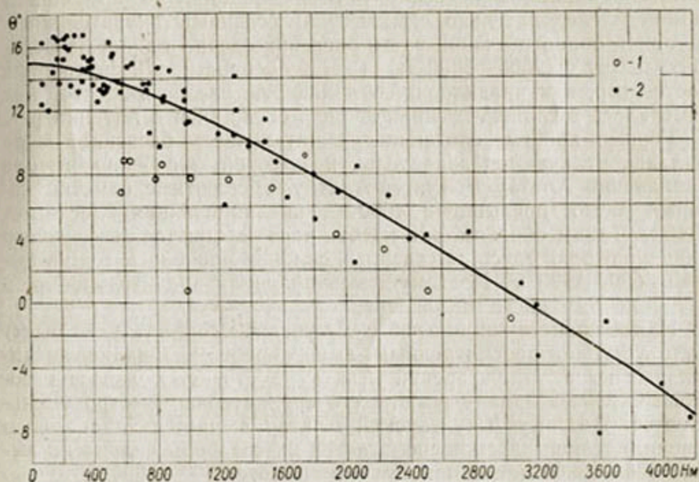
Рис. 163. Зависимость средних годовых температур воздуха \theta от высоты местности ( H ).
