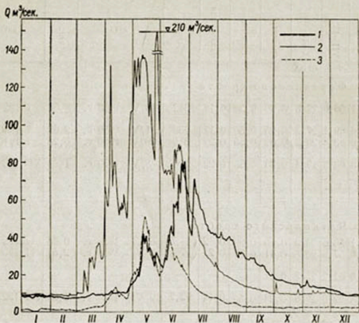
Рис. 150. Гидрографы типичных рек Ферганской котловины за 1942 г.
