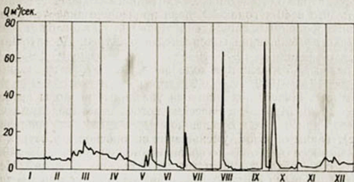
Рис. 102. Гидрограф р. Атрек у г. Кизыл-Атрек за 1942 г.
