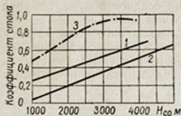
Рис. 12. Зависимость коэффициента стока от средней взвешенной высоты водосбора ( H_{ср} ).
