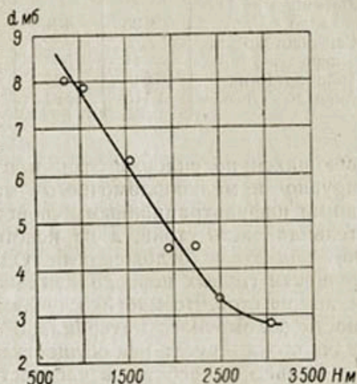
Рис. 20. Зависимость дефицита влажности ( d ) от высоты местности ( H ).
