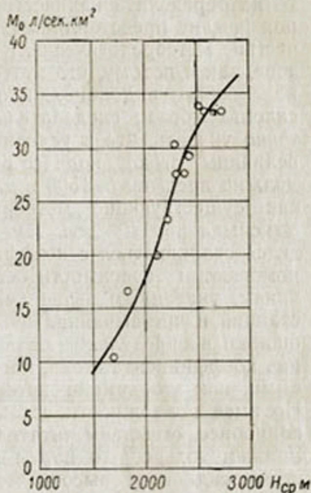
Рис. 19. Зависимость среднего многолетнего модуля стока ( M_0 ) от средней взвешенной высоты водосбора ( H_{\text{ср}} ) для рек южного склона Гиссарского хребта.
