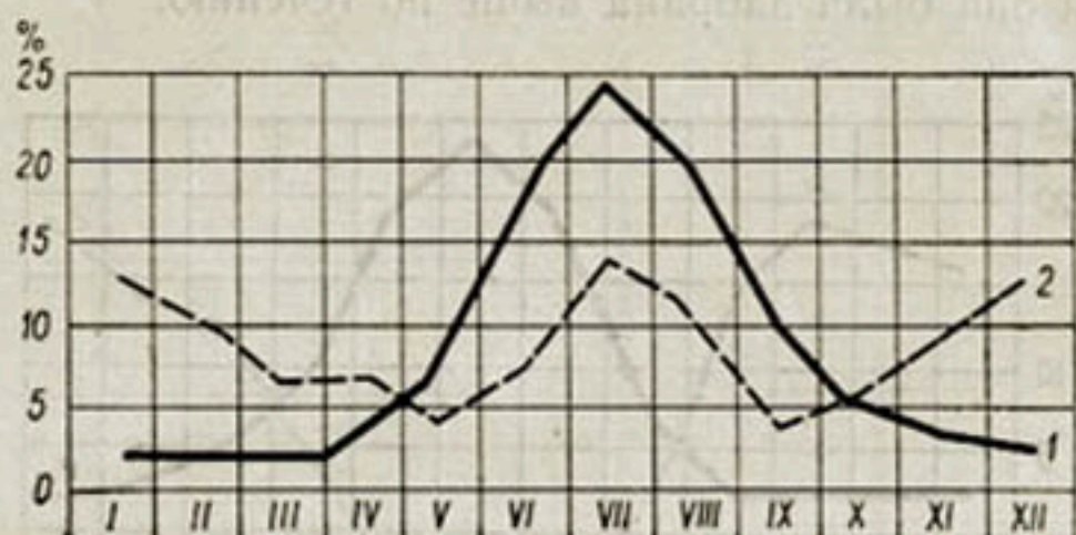
Рис. 38. Гидрографы средних месячных расходов воды (в % годового) р. Зеравшан при выходе из гор (1) и у г. Каракуль (2).
