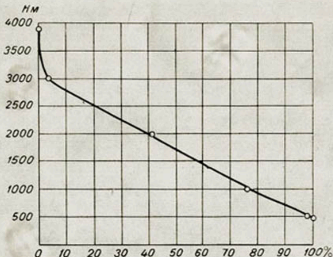
Рис. 104. Гипсометрическая кривая бассейна р. Мургаб у с. Сепп-Али (ст. Меручакская).
