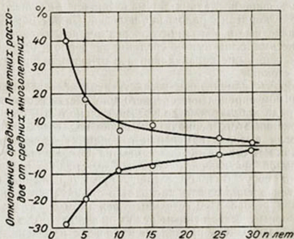
Рис. 26. Зависимость наибольших ошибок (%) в подсчете средних многолетних расходов воды от продолжительности наблюдений ( n лет).
