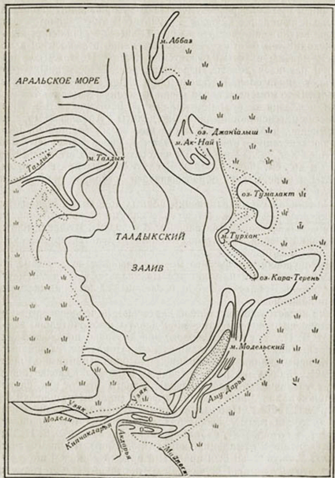
Рис. 122. Схема Талдыкского залива по состоянию на 1934 г.
