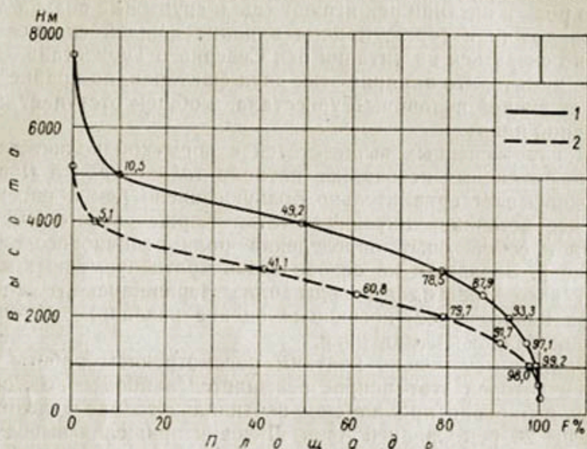
Рис. 7. Гипсометрические кривые водосборов Вахша и Пянджа (1), водосборов Нарына и Карадарьи (2).
