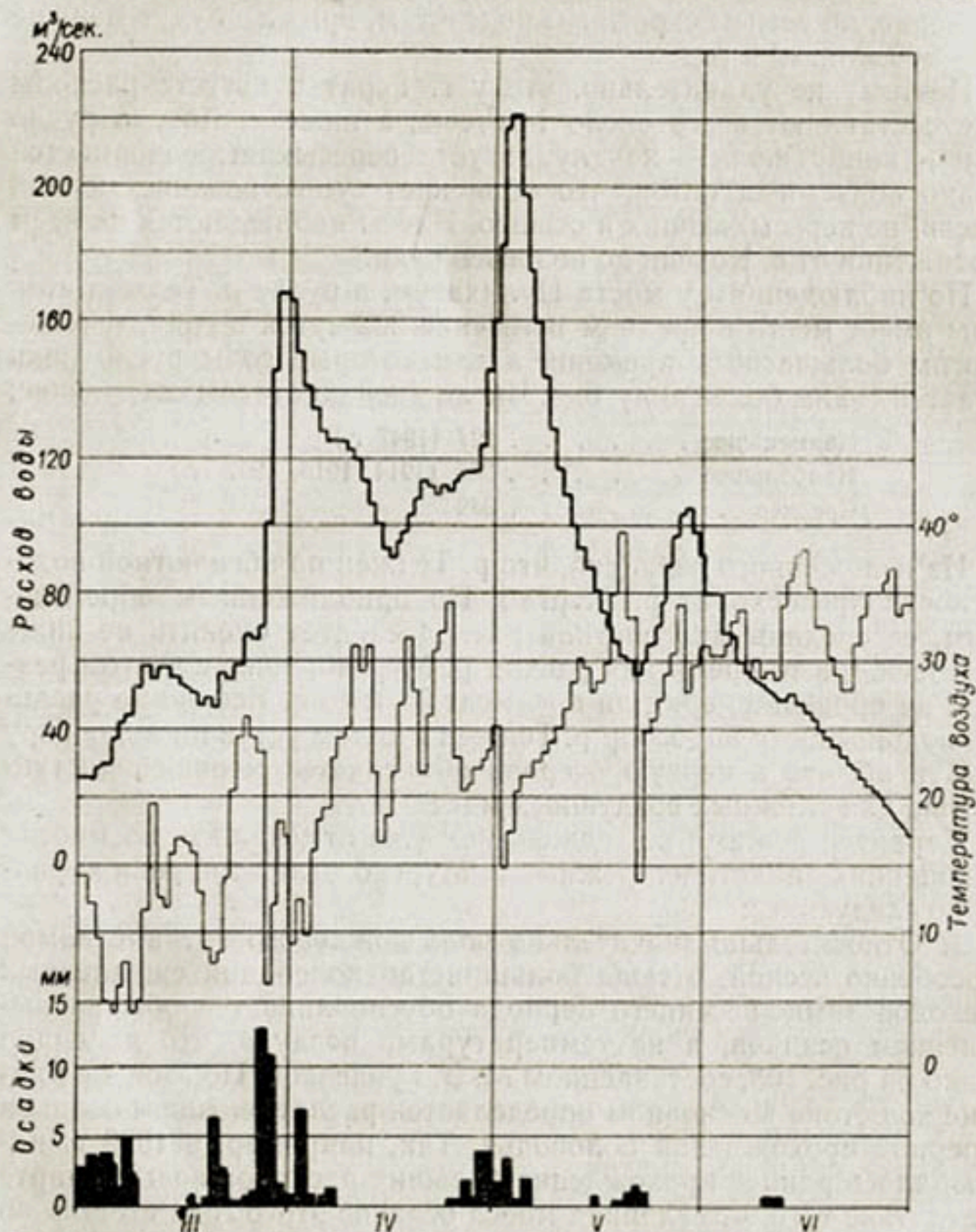
Рис. 108. Совмещенный ход температуры воздуха, атмосферных осадков и расходов воды р. Теджен у с. Пулихатум в 1932 г.
