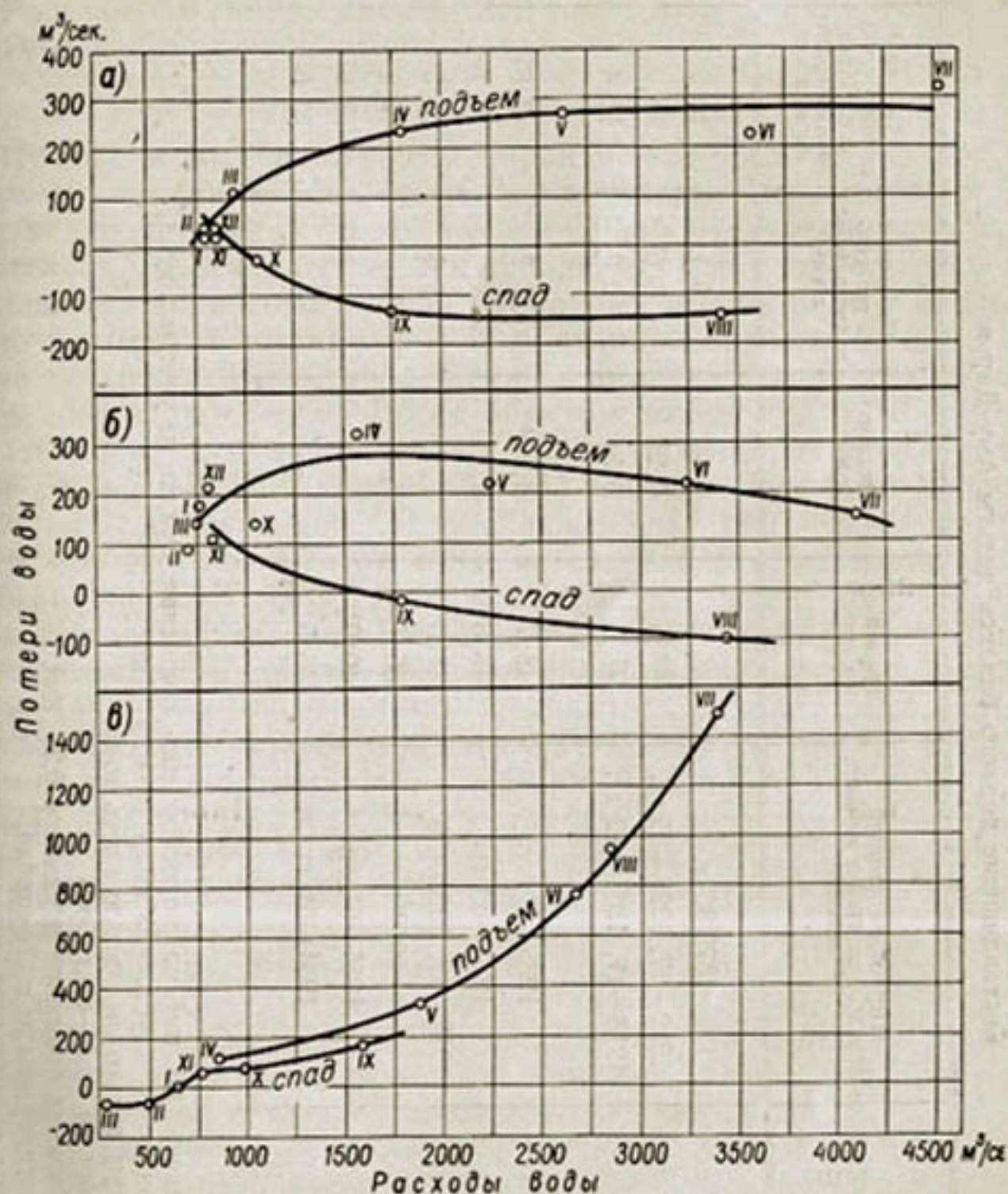
Рис. 126. Потери воды в русле и пойме Аму-Дарьи в зависимости от расходов воды в верхних створах участков.
