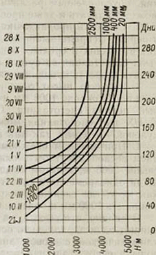
Рис. 41. Зависимость среднего времени схода снежного покрова (положения тыла снеготаяния) от его мощности (в слое воды) и высоты местности (H).
