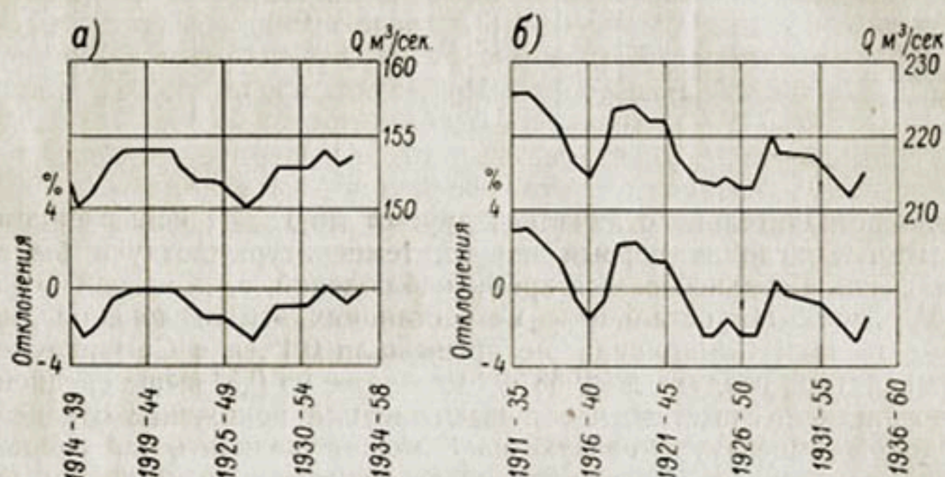
Рис. 25. Средние расходы воды по скользящим 25-летиям и отклонение их от среднего расхода за весь период наблюдений.
