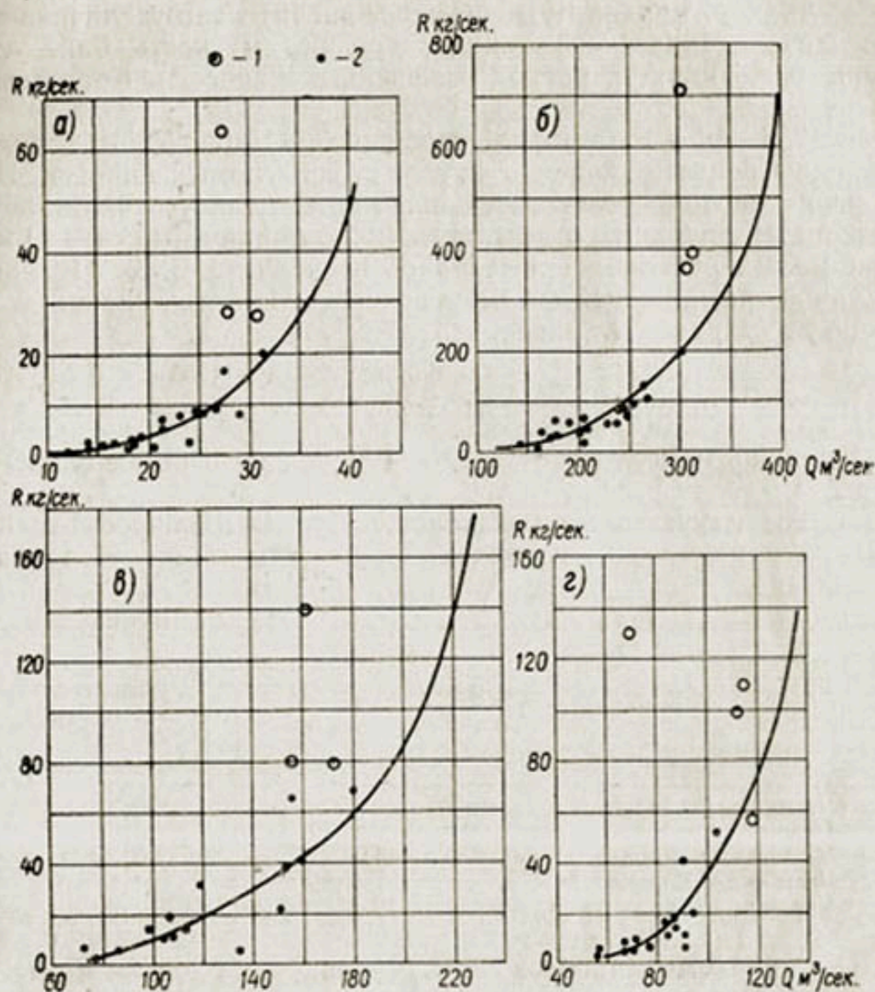
Рис. 156. Зависимость расходов взвешенных наносов от расходов воды.
