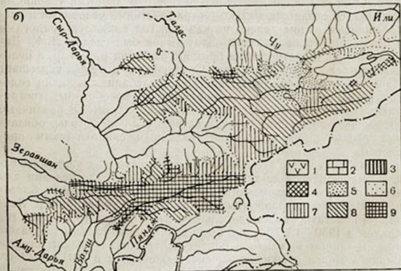
Рис. 30. Распределение водности по территории Средней Азии.
