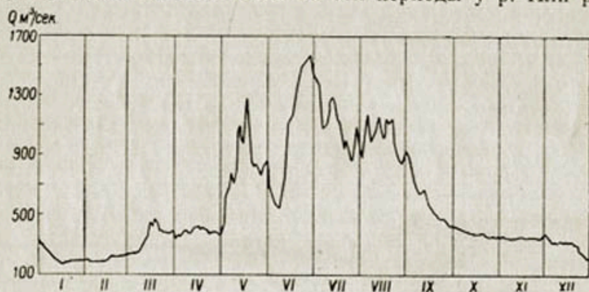
Рис. 165. Гидрограф р. Или у с. Илийское за 1942 г.
