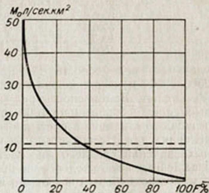
Рис. 23. Распределение (обеспеченность) средних модулей стока по территории горной области Средней Азии.
