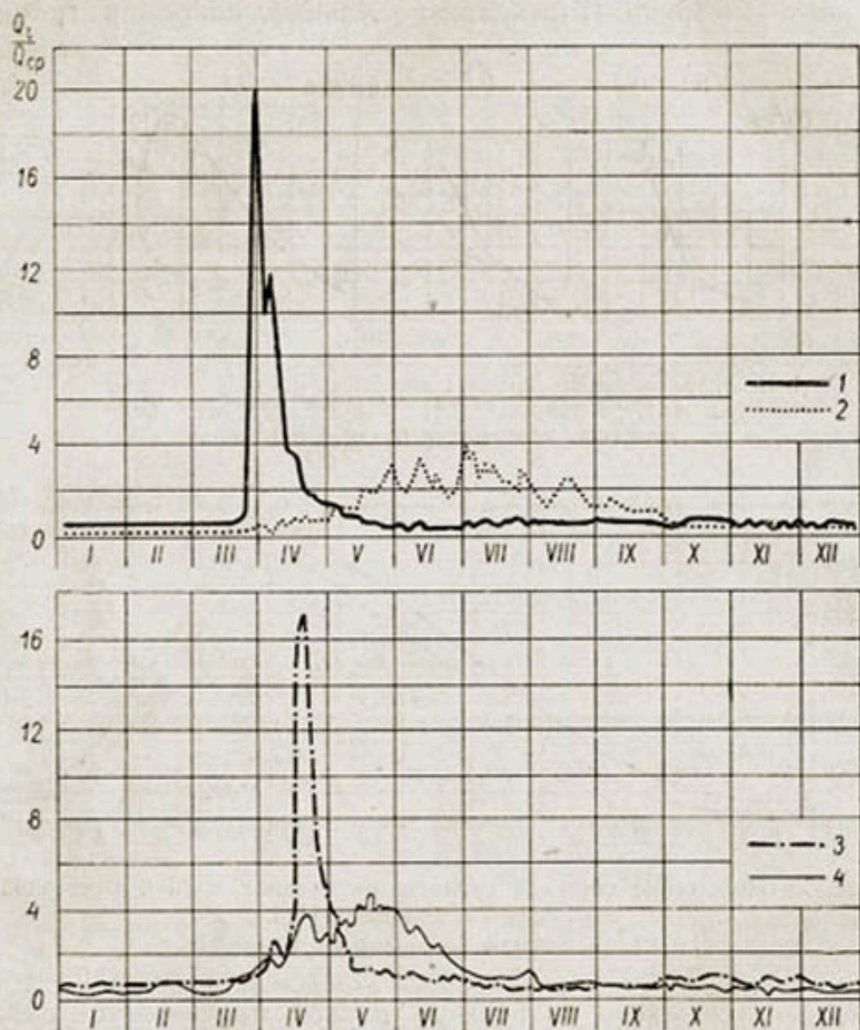
Рис. 36. Гидрографы рек Дон (1), Вахш (2), Волга (3) и Ангрен (4).
