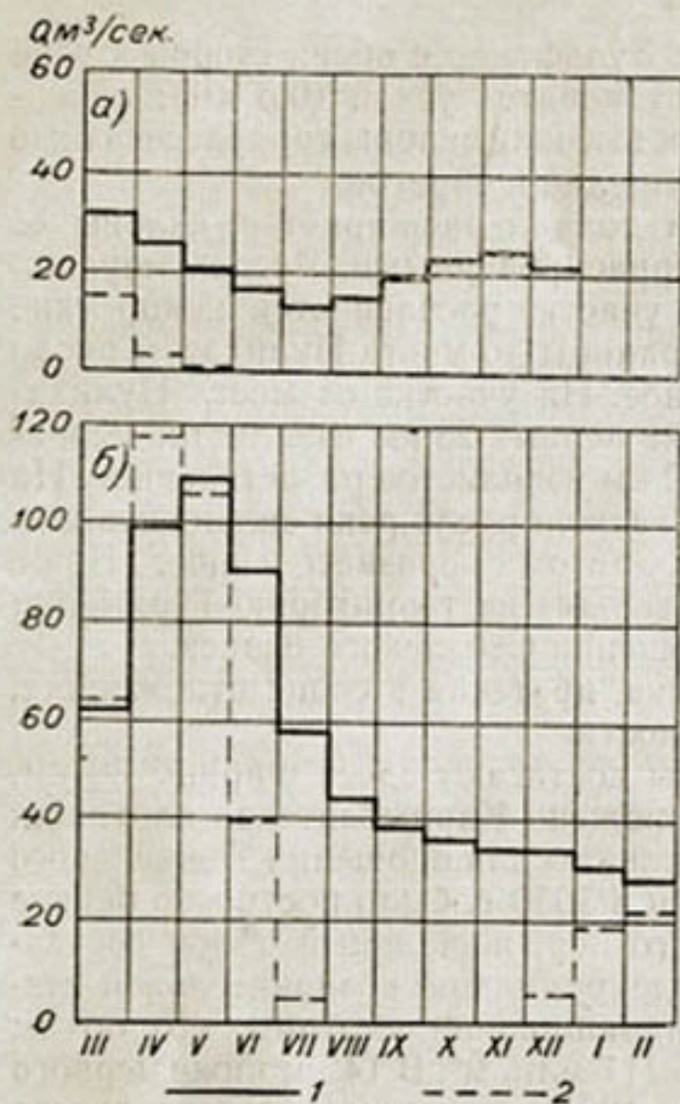
Рис. 107. Средние месячные расходы воды р. Теджен у с. Пулихатум (1) и р. Мургаб у с. Сеин-Али (2). а — 1917-18 г., б — 1932-33 г.
