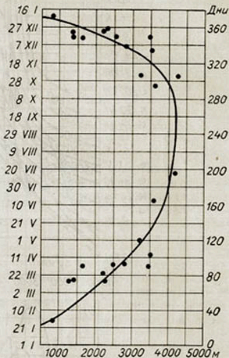
Рис. 51. Зависимость времени устойчивого схода и установления снежного покрова на водосборе Аму-Дарьи.
