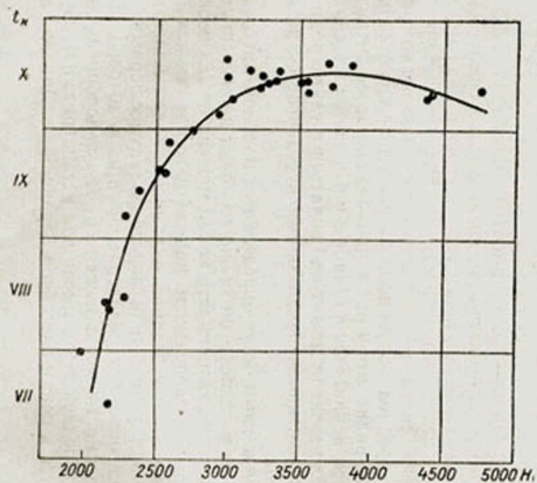
Рис. 82. Зависимость средних дат начала межени ( t_n ) от средних взвешенных высот водосборов ( H_{cp} ) для рек южного района Средней Азии (данные З. Мамбетовой).
