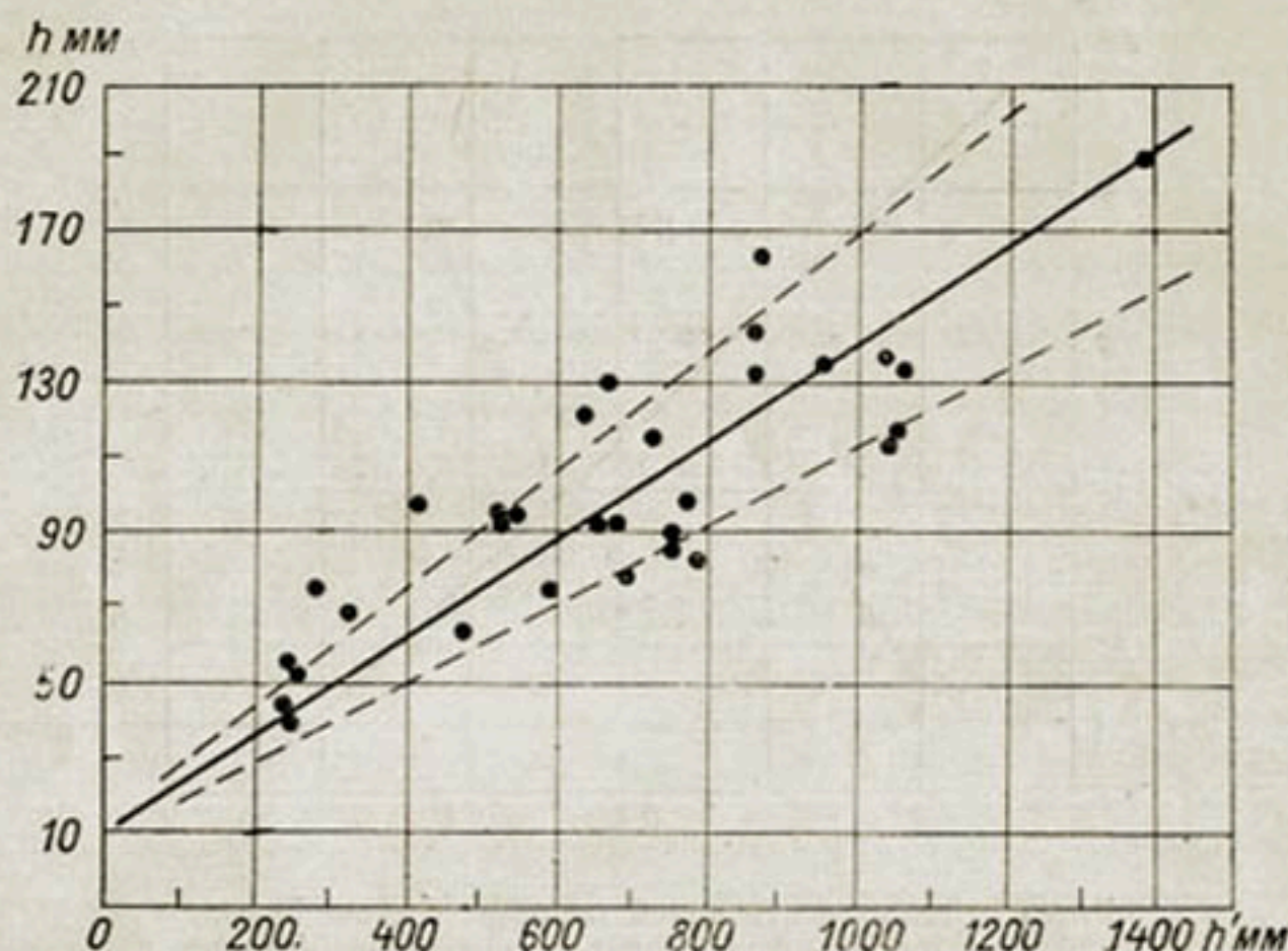
Рис. 85. Зависимость среднего многолетнего слоя межени стока ( h ) от годового ( h' ) для южного района Средней Азии.
