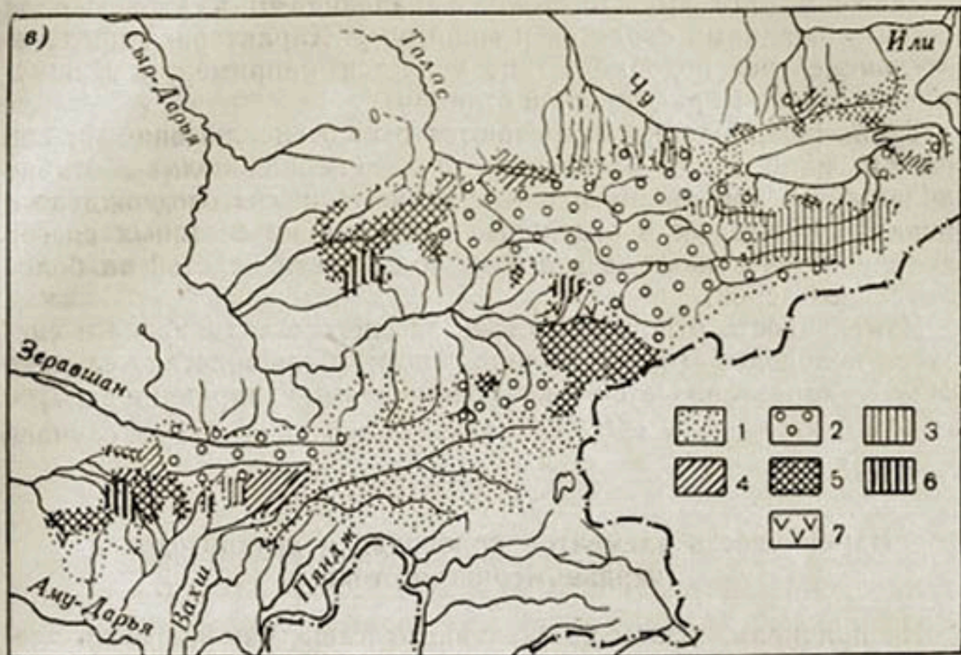
Рис. 67. Распределение коэффициентов вариации стока за фазово-однородные периоды.
