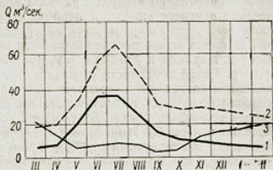
Рис. 157. Ход средних месячных расходов воды р. Талас.
