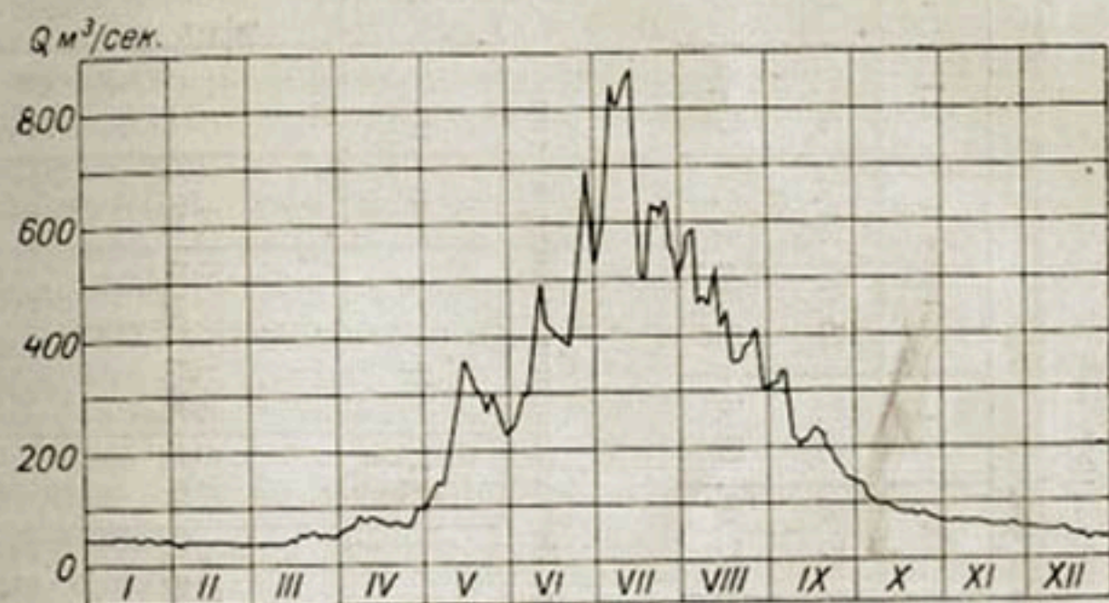
Рис. 131. Гидрограф р. Зеравшан у уроч. Дупули за 1942 г.
