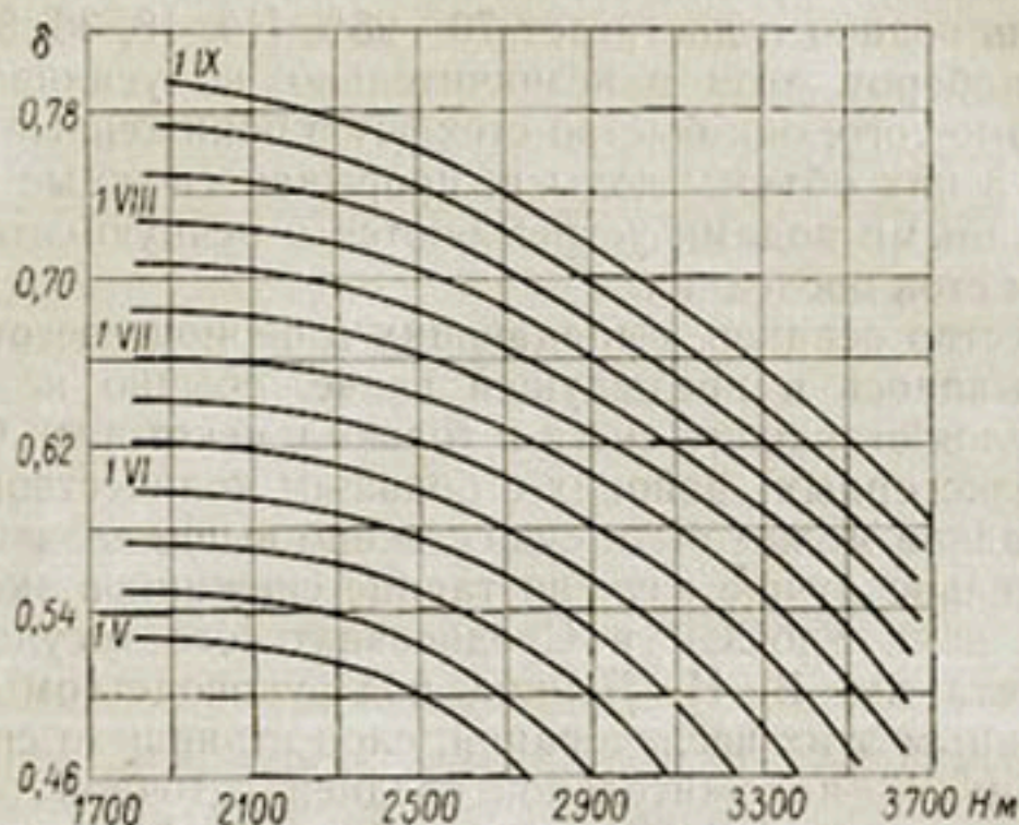
Рис. 45. Зависимость плотности снега ( \delta ) от высоты ( H ) и времени.
