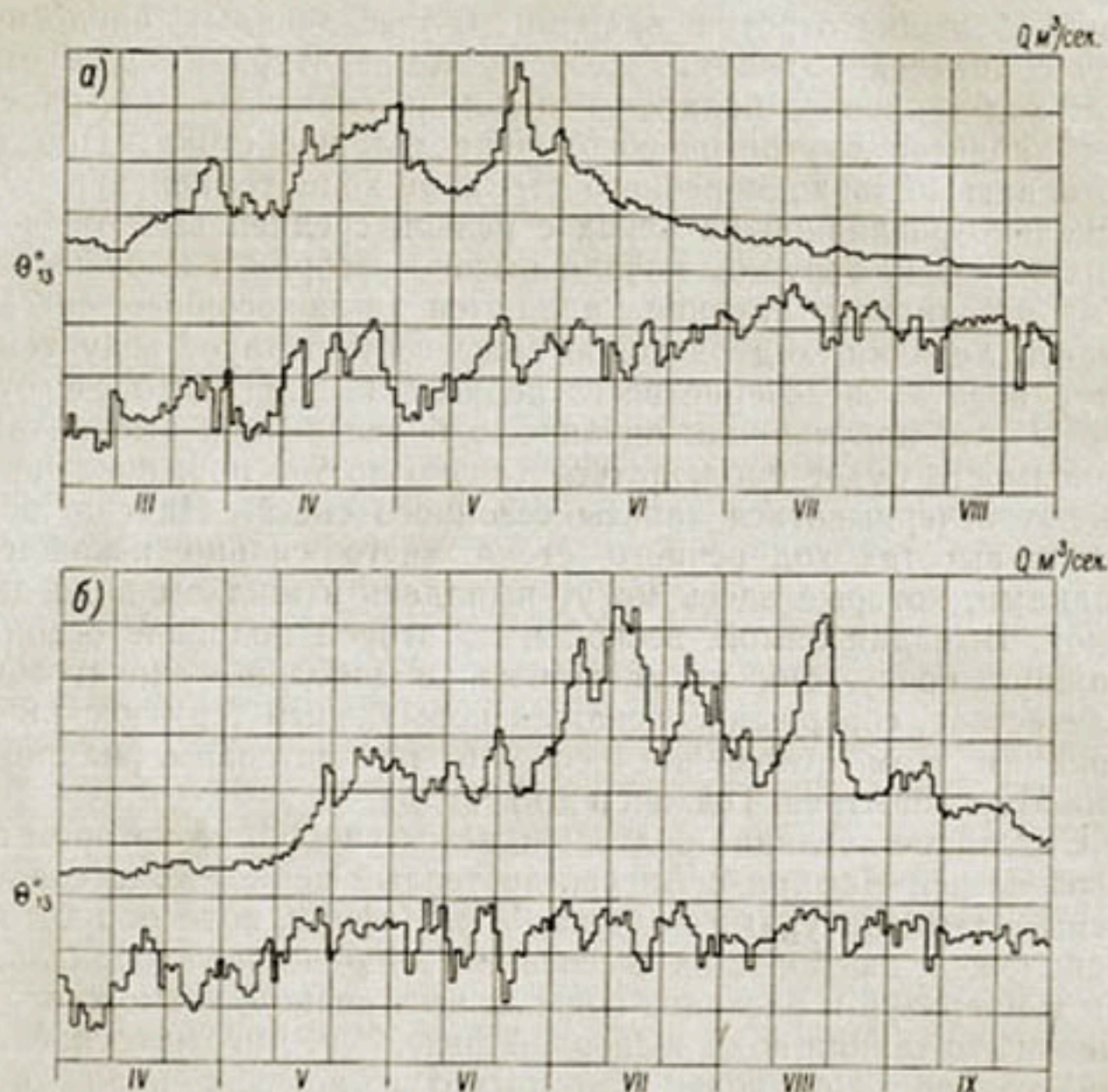
Рис. 33. Ход расходов воды ( Q ) и температур воздуха ( \theta_{13} ) за период интенсивного снеготаяния.
