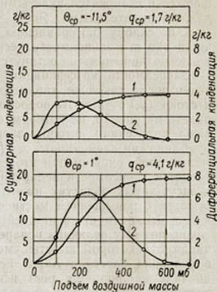
Рис. 17. Зависимость количества скопированной влаги от высоты подъема слоя атмосферы толщиной 500 мб.
