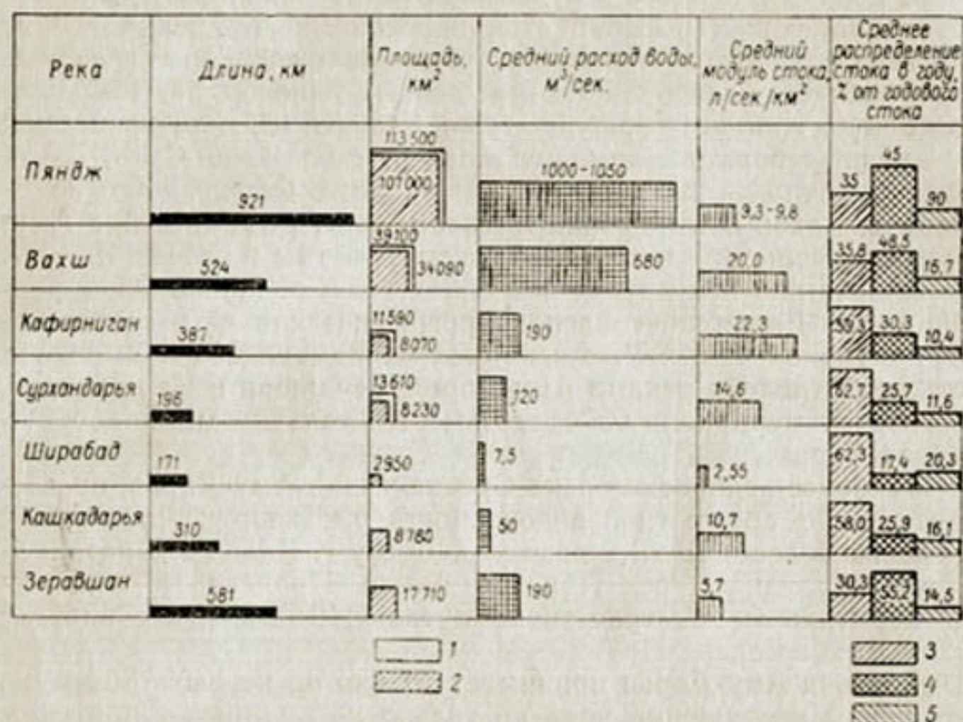
Рис. 111. Сравнительная диаграмма крупнейших рек бассейна Аму-Дарья. 1 — площадь бассейна, 2 — площадь водосбора, 3 — сток за март—июнь, 4 — сток за июль—сентябрь, 5 — сток за октябрь—февраль.
