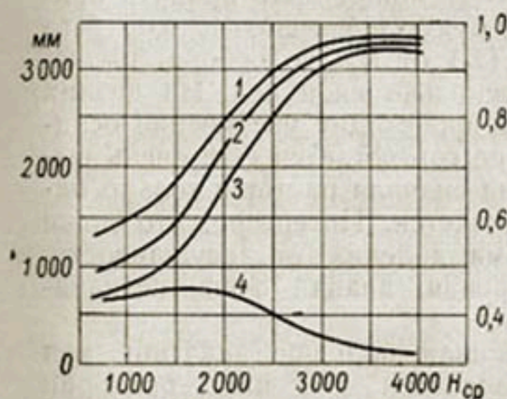
Рис. 16. Зависимость осадков (1), коэффициента стока (2), стока (3) и испарения (4) от высоты водосборов ( H_{cp} ) для рек бассейна Аара (по Шпильману).
