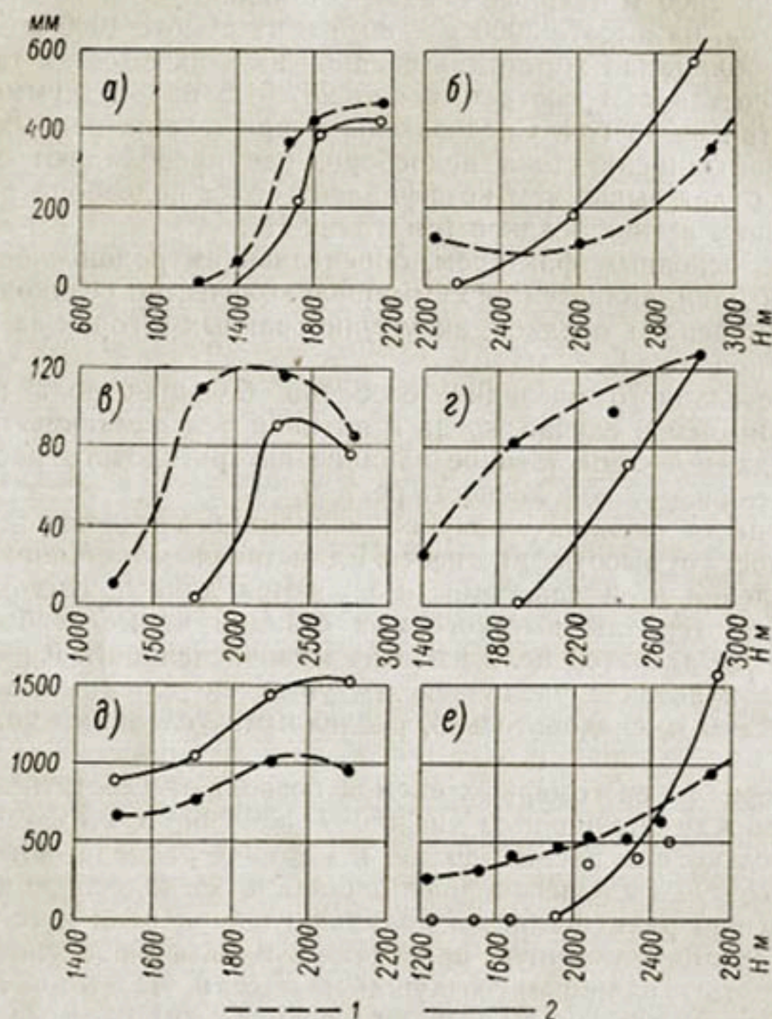
Рис. 18. Зависимость водности снежного покрова в 1942 г. от высоты местности.
