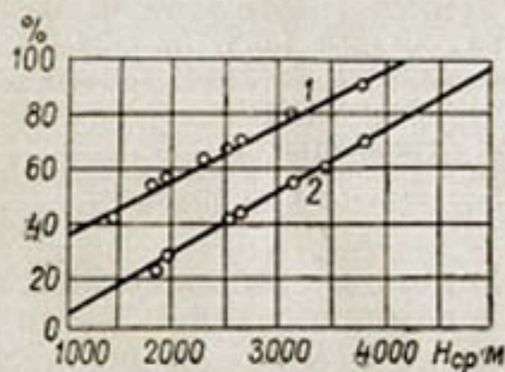
Рис. 11. Зависимость относительного количества твердых осадков (в % от общей величины осадков) от средней взвешенной высоты водосбора ( H_{cp} ).
