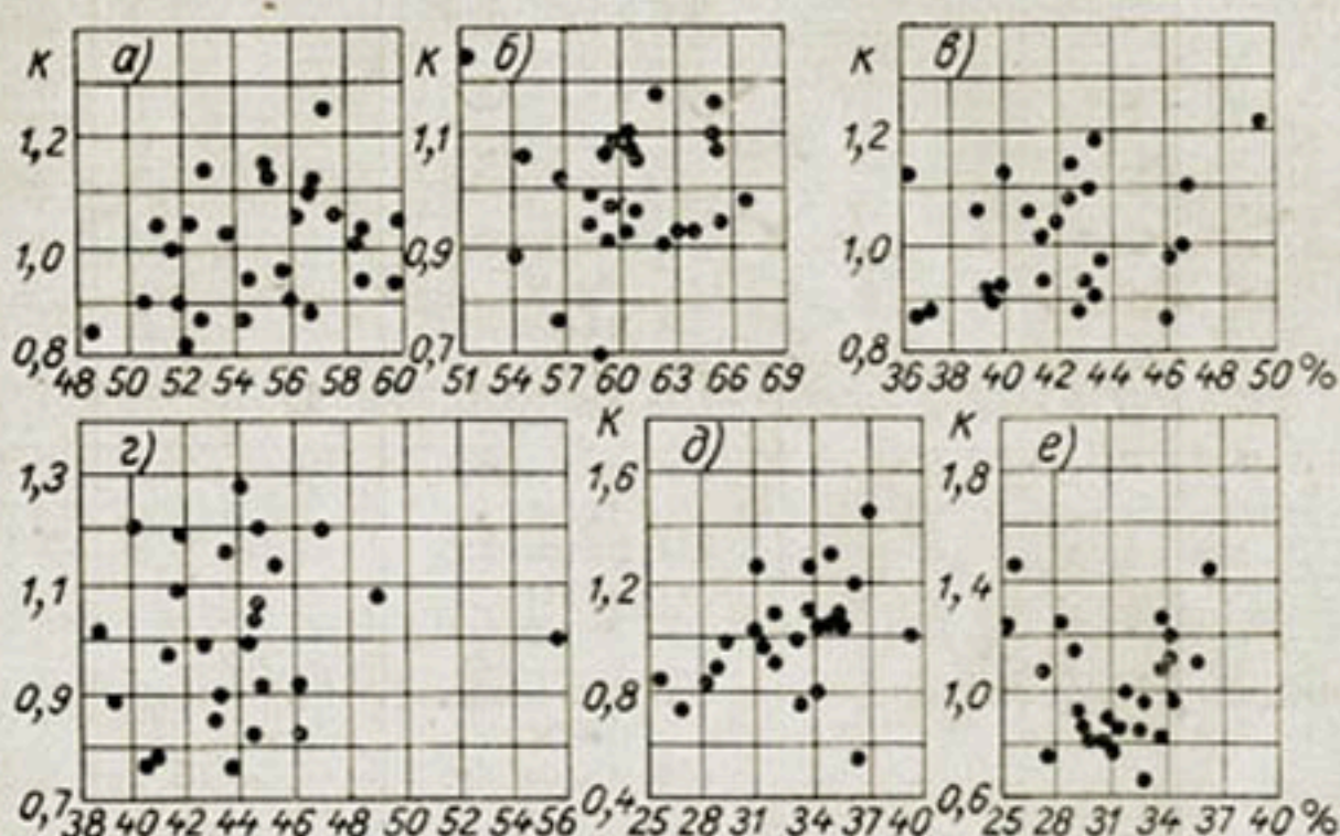
Рис. 65. Зависимость стока (в % годового стока) за период июль—сентябрь от водности года (от модульного коэффициента средних годовых расходов k ).
