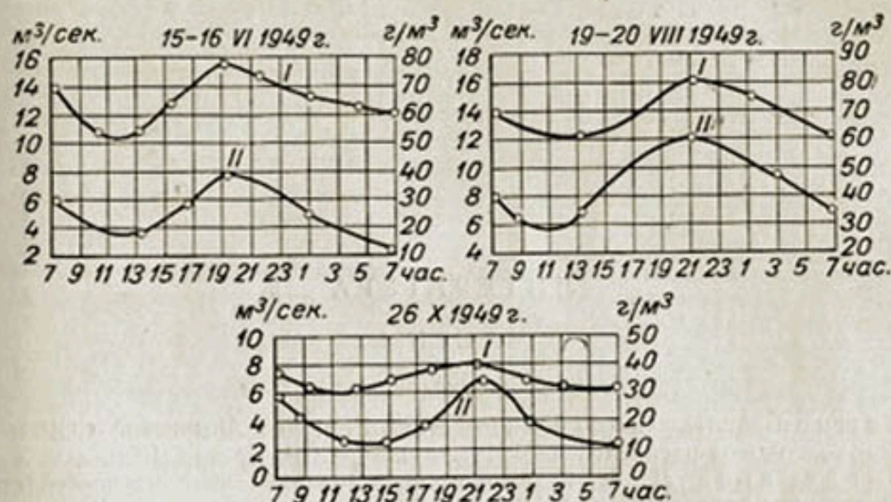
Рис. 98. Суточный ход расходов (м 3 /сек.) и мутности воды (г/м 3 ) на р. Большая Алмаатинка. I — расходы воды, II — мутность.
