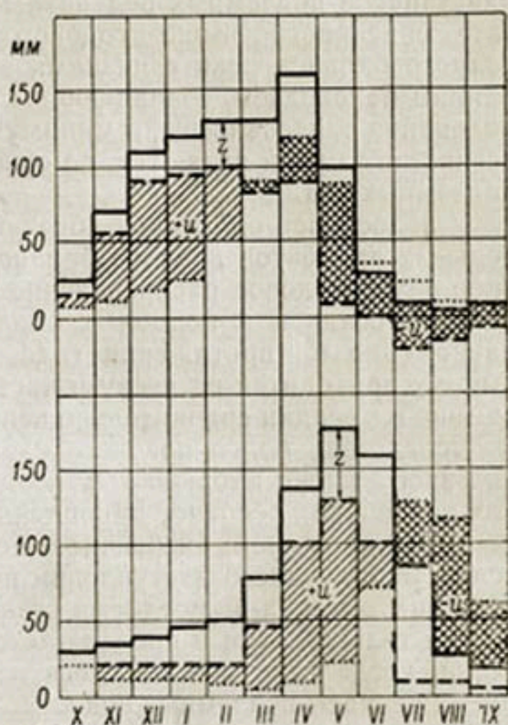
Рис. 32. Годовой ход элементов водного баланса водосборов рек Средней Азии.
