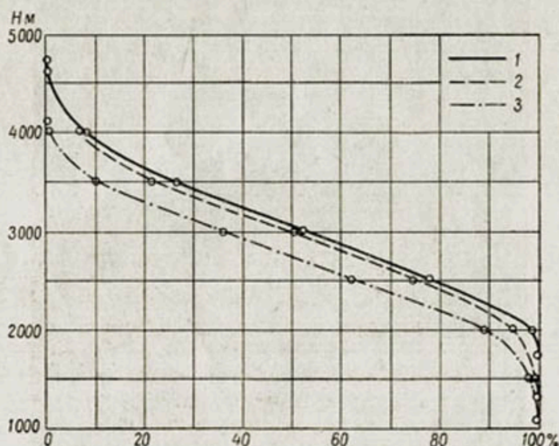
Рис. 138. Гипсометрические кривые водосборов крупнейших притоков р. Нарын.
