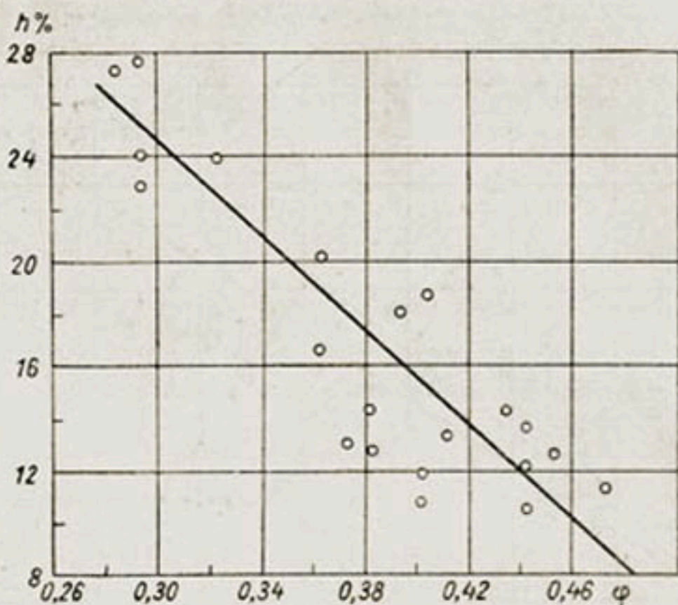
Рис. 84. Зависимость долей меженного стока в годовом ( h ) от коэффициента внутригодовой неравномерности стока ( \phi ) для южного района Средней Азии.
