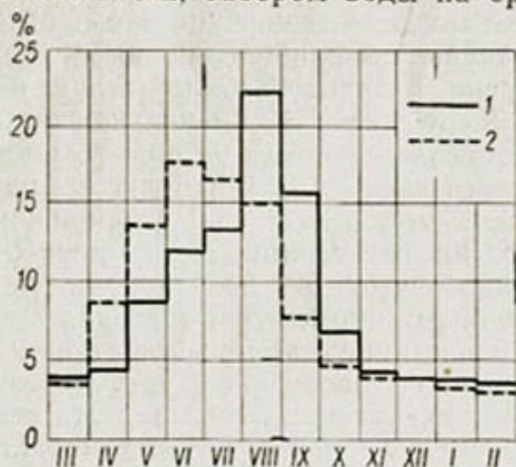
Рис. 125. Внутригодовое распределение стока Аму-Дарьи у г. Керки в % от годового. 1 — 1917-18 гг., 2 — 1928-29 гг.
