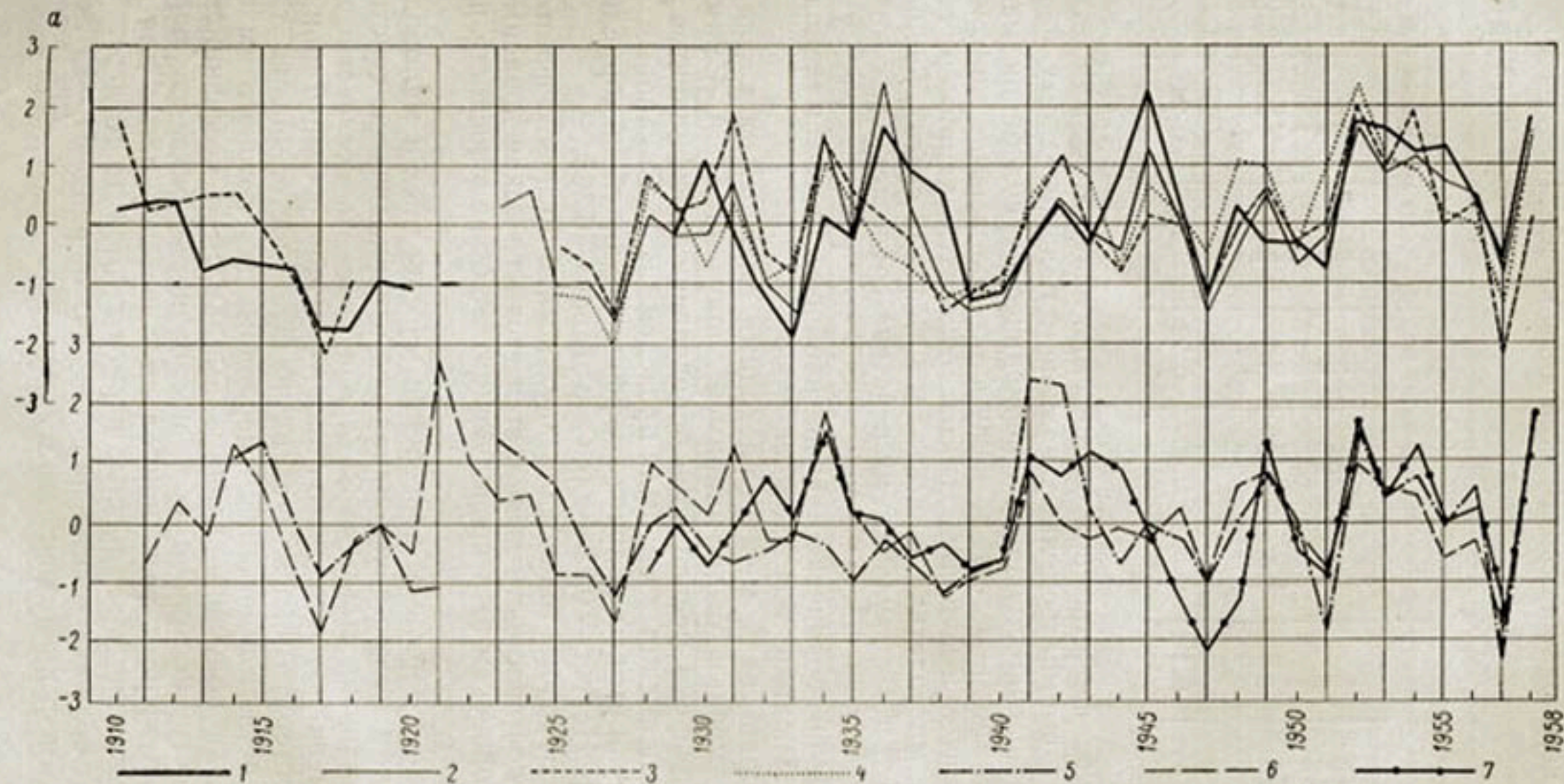
Рис. 29. Хронологическая последовательность лет различной водоносности.
