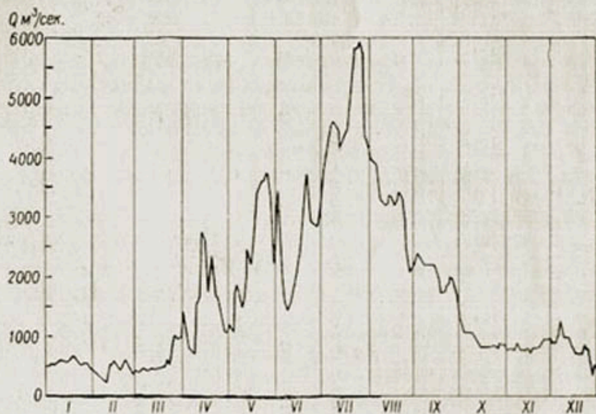
Рис. 124. Гидрограф Аму-Дарьи у г. Нукус за 1942 г.
