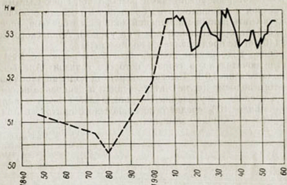
Рис. 24. Колебания средних годовых уровней Аральского моря.
