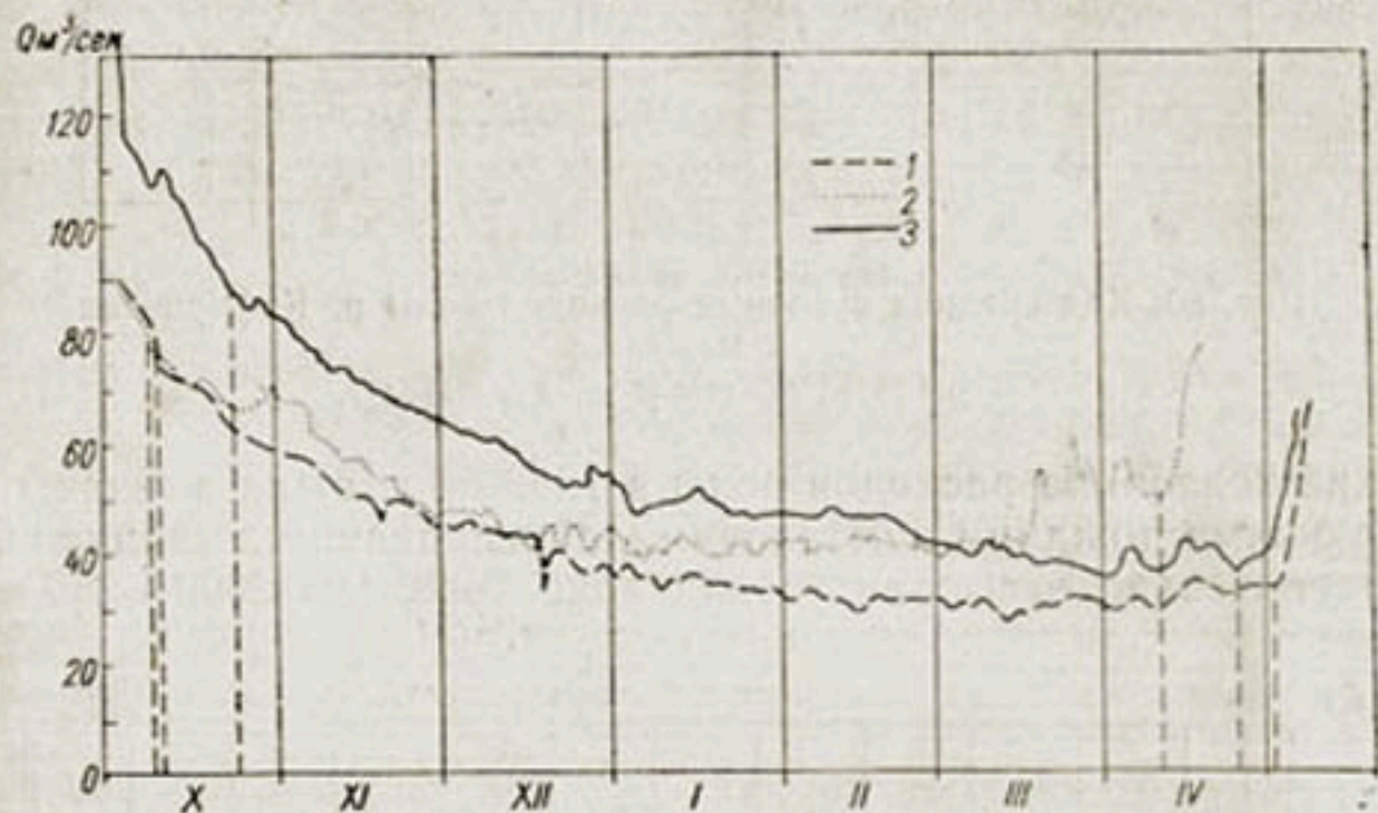
Рис. 79. Ход средних суточных расходов р. Зеравшан в межень. 1 — 1949-50 г., 2 — 1940-41 г., 3 — 1938-39 г.
