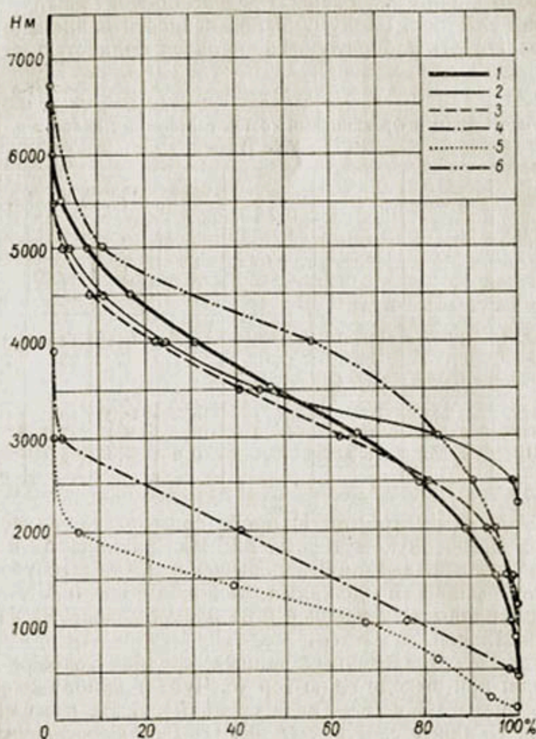
Рис. 112. Гипсометрические кривые водосборов рек.
