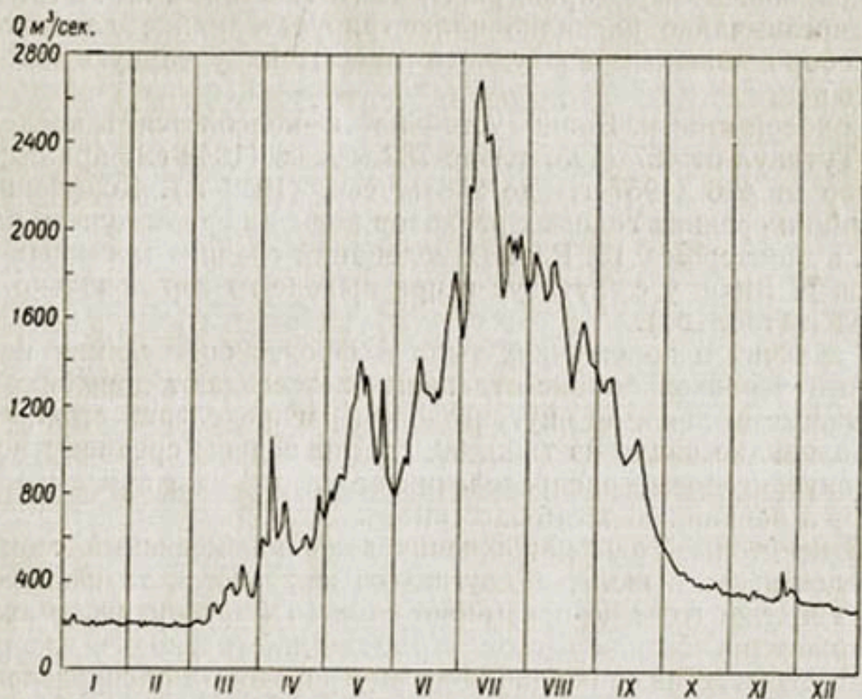
Рис. 115. Гидрограф р. Вахш у с. Туткаул за 1942 г.
