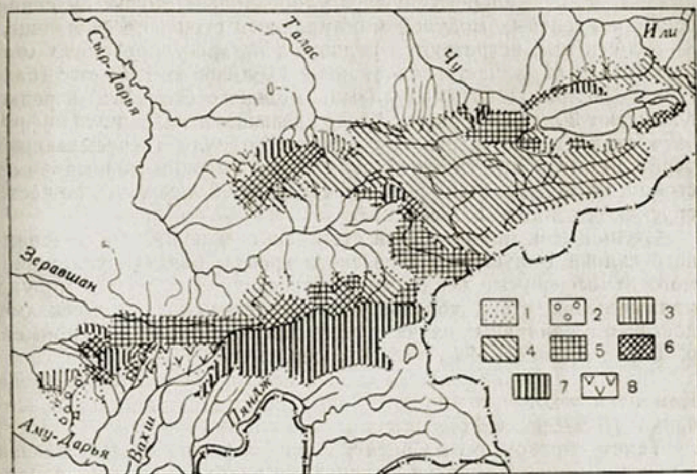
Рис. 87. Распределение минимальных средних месячных модулей стока по территории Средней Азии (л/сек. км 2 ).
