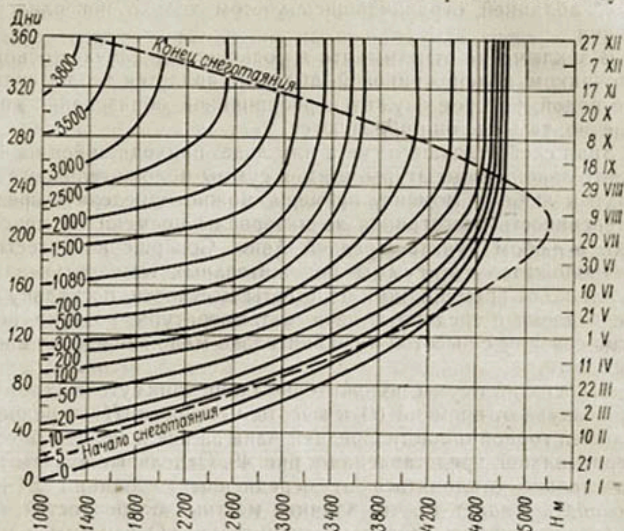
Рис. 49. Зависимость сумм положительных средних суточных температур воздуха от времени и высоты местности.
