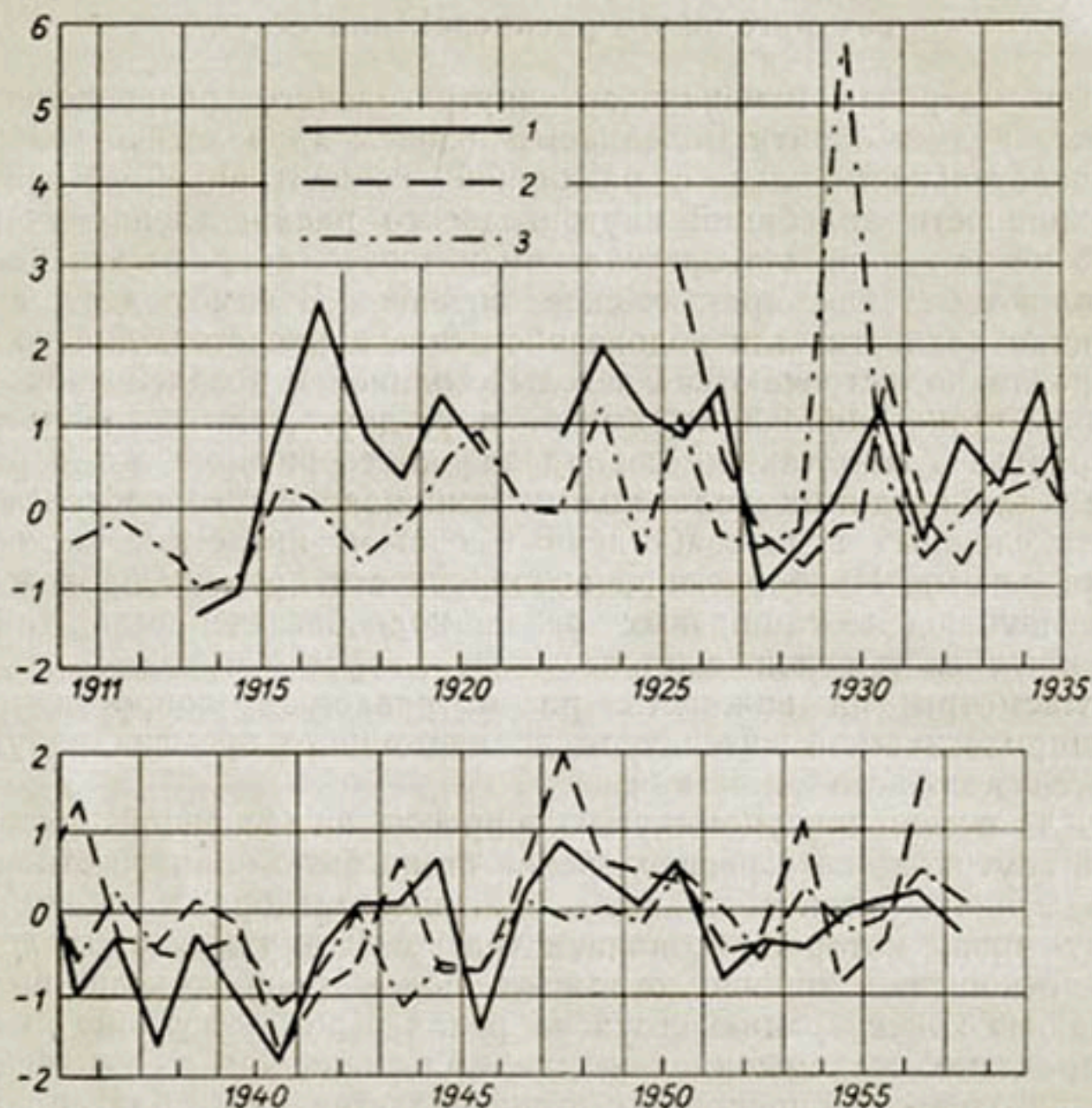
Рис. 68. Хронологическая последовательность лет с различной концентрацией стока на протяжении половодного периода.
