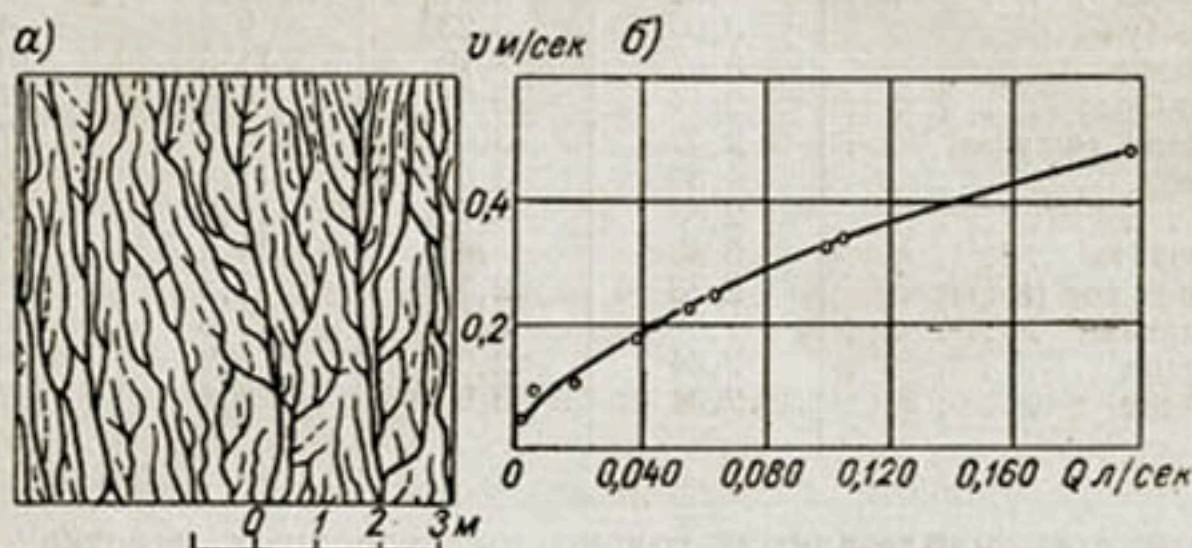
Рис. 76. Густота микроручейковой сети (а) и зависимость скоростей стекания (б) от величины расходов на эродированном склоне крутизной 32^\circ .
