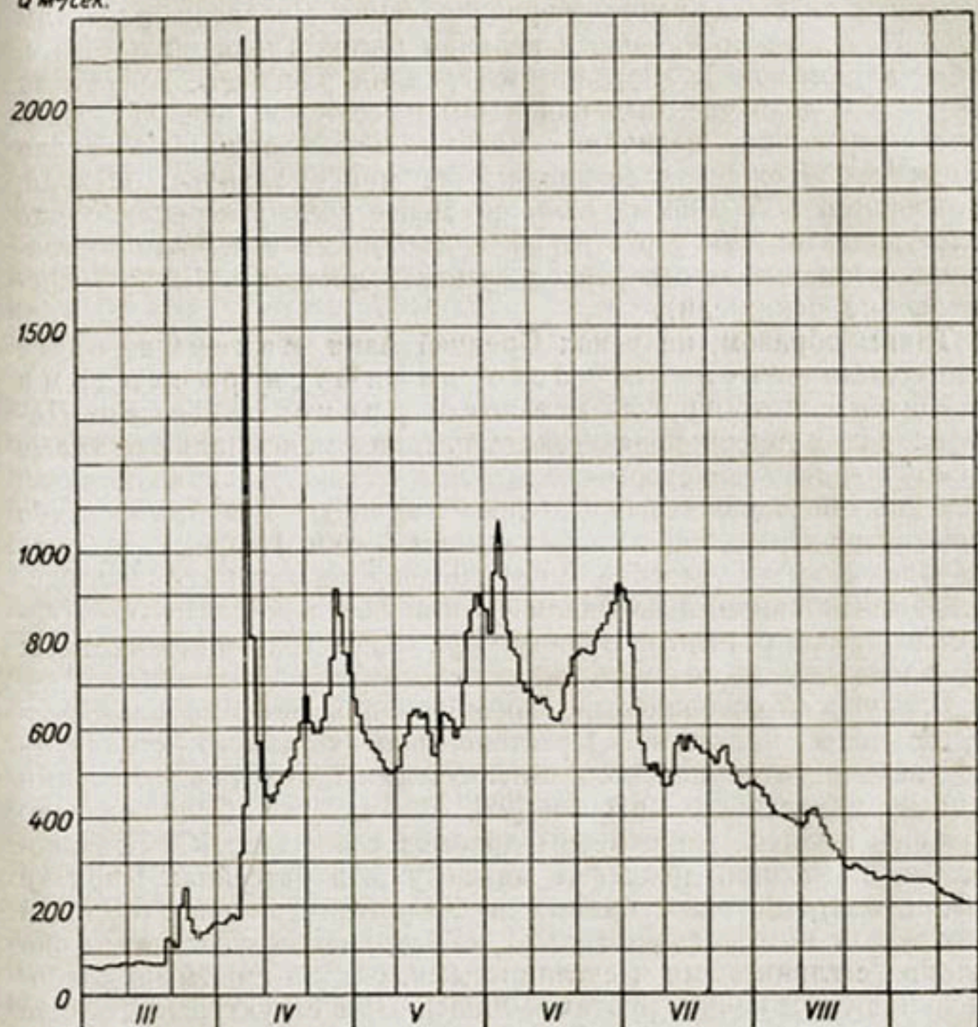
Рис. 72. Гидрограф половодья 1959 г. р. Чирчик — с. Ходжикент.
