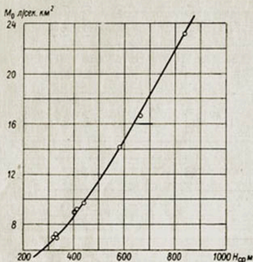
Рис. 22. Зависимость M_0 от H_{ср} для западного склона Урала (бассейн р. Камы).
