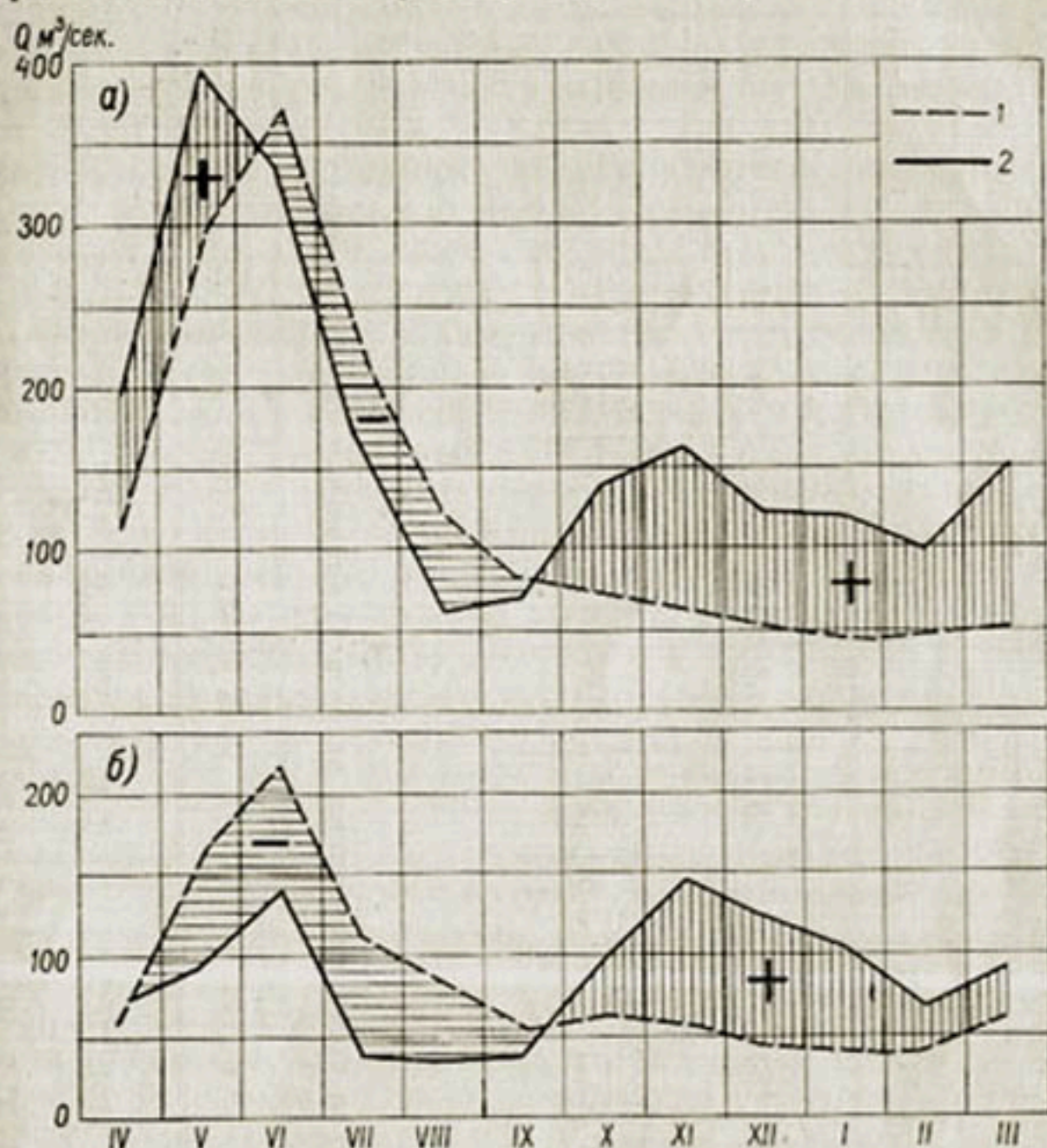
Рис. 143. Ход средних месячных расходов воды р. Карадарья в створах Кампырраватской (1) и Балыкчинской (2) станций.
