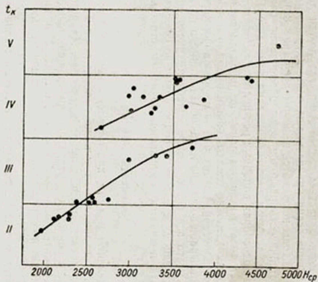
Рис. 83. Зависимость конца межени ( t_k ) от средних взвешенных высот водосборов ( H_{cp} ) для южного района Средней Азии.
