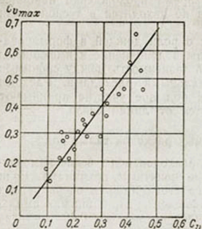
Рис. 74. Связь коэффициентов вариации максимальных и средних годовых расходов воды.
