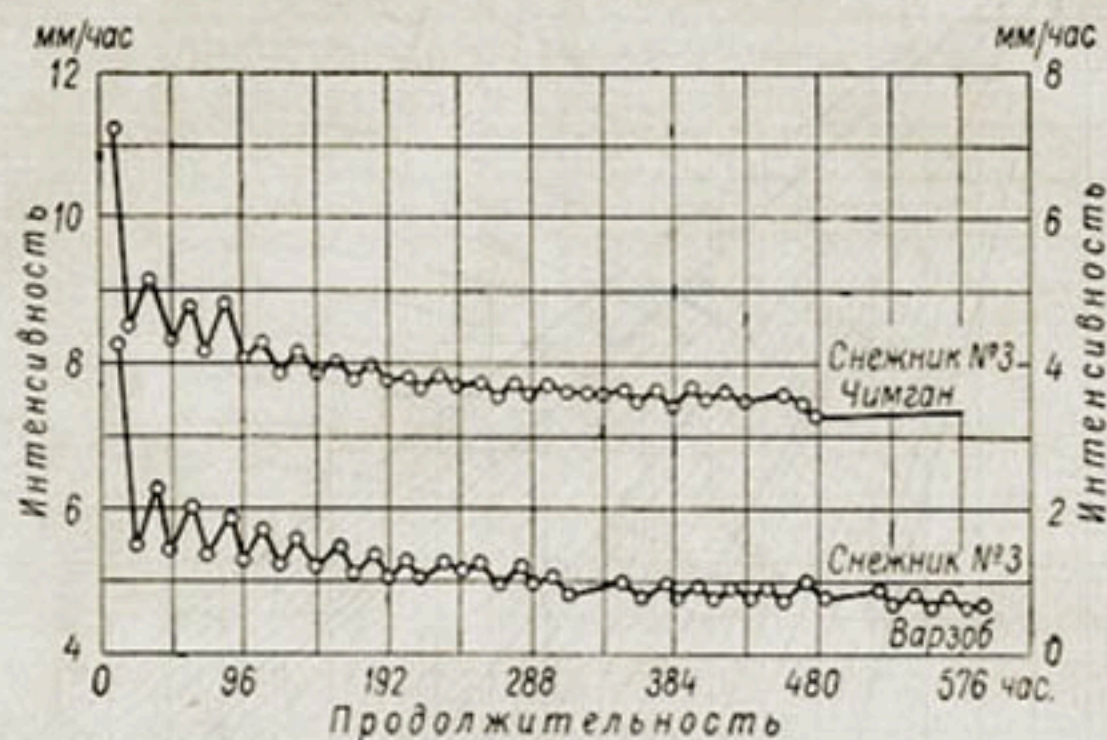
Рис. 47. Зависимость средней интенсивности снеготаяния (в слое воды) от его продолжительности.
