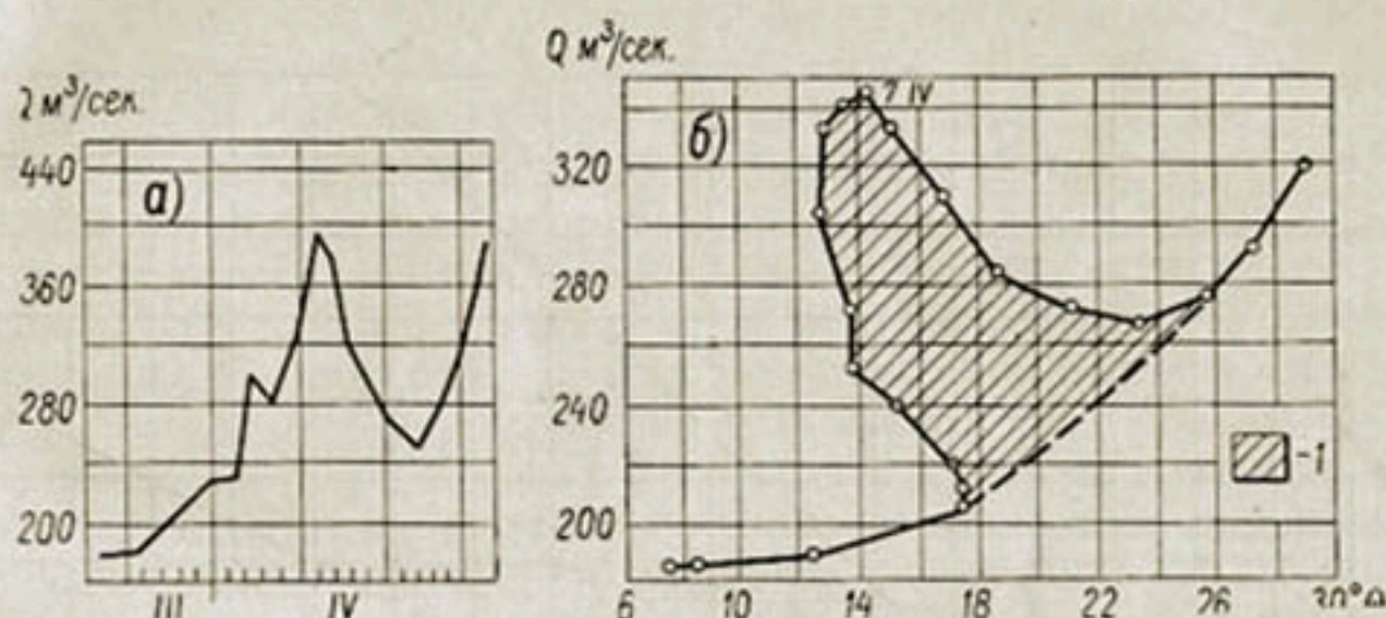
Рис. 13. Гидрограф средних суточных расходов р. Нарын — ст. Уч-кур-ган (а) и зависимость средних суточных расходов от температуры воздуха за 13 час. по ст. Андижан для скользящих пентад (б). Март—апрель 1936 г. I — дождевой сток.
