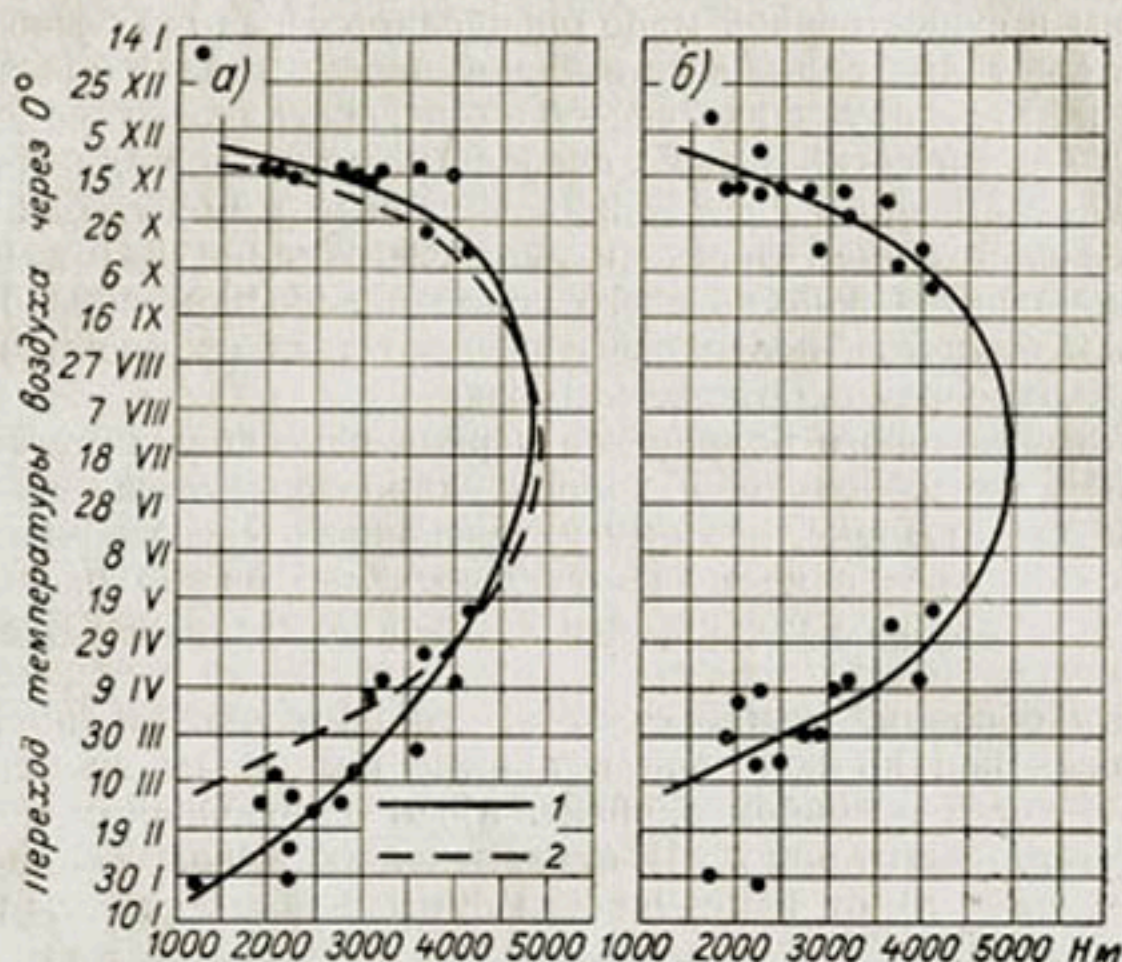
Рис. 59. Зависимость времени перехода 13-часовых температур воздуха через 0^{\circ} (положение фронта снеготаяния) от высоты местности.
