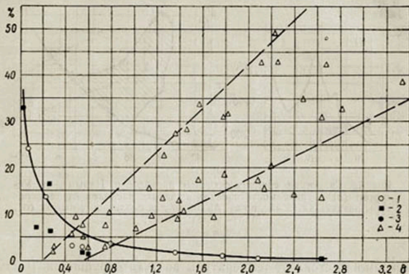
Рис. 14. Зависимость дождевого и ледникового питания (в % от годового) от коэффициента \delta .
