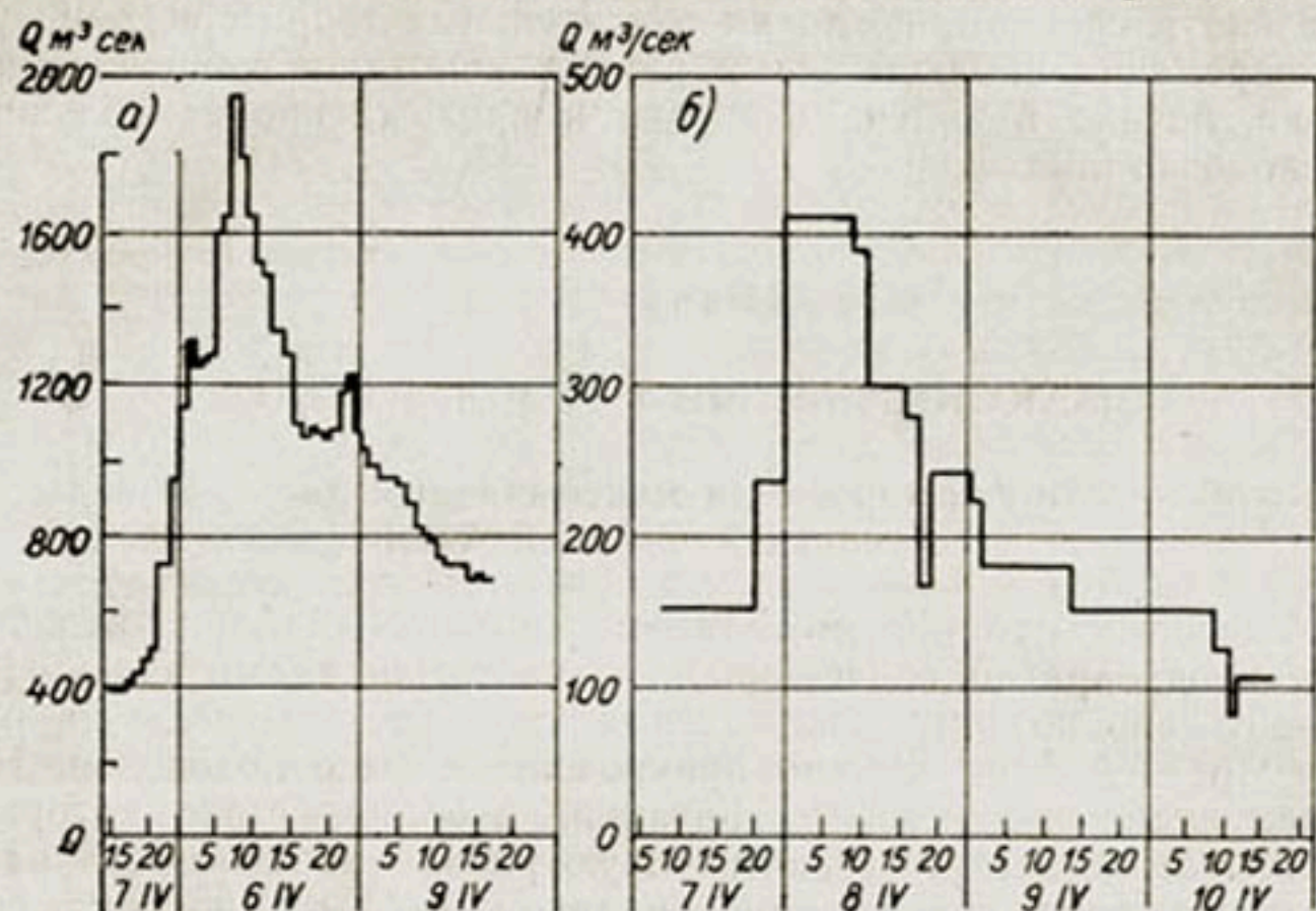
Рис. 71. Гидрографы паводков, прошедших в апреле 1959 г.
