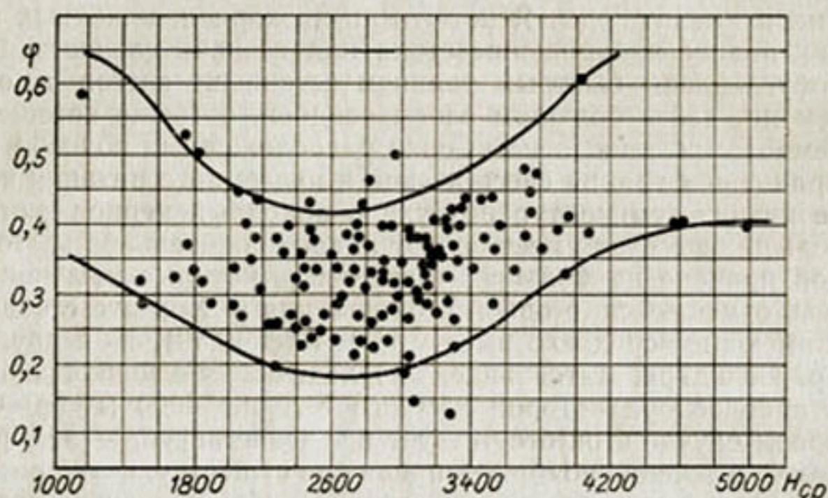
Рис. 57. Зависимость коэффициента внутригодовой неравномерности стока ( \varphi ) от средней взвешенной высоты водосбора.
