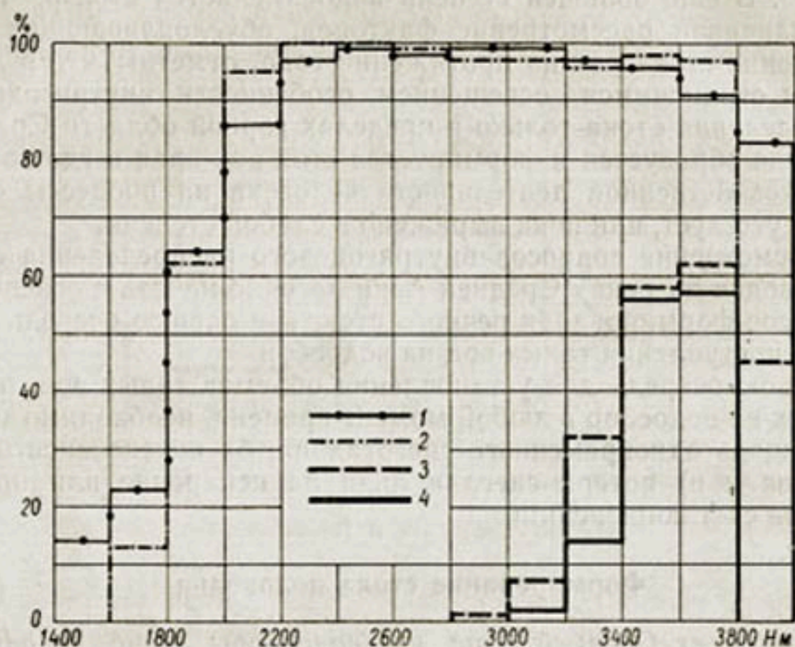
Рис. 39. Заснеженность водосборов (в % площади) по отдельным высотным зонам.
