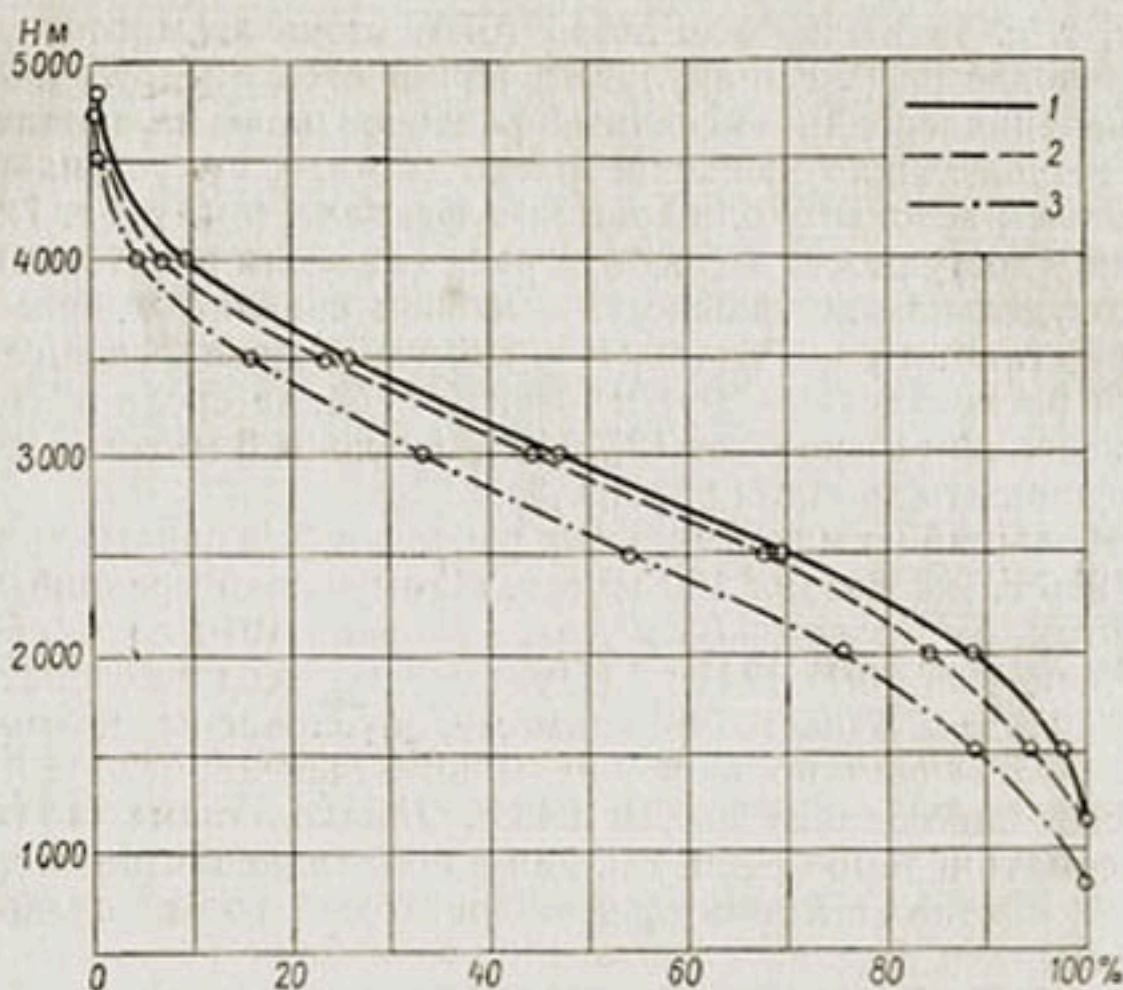
Рис. 141. Гипсометрические кривые водосборов р. Карадарья и ее составляющих.
