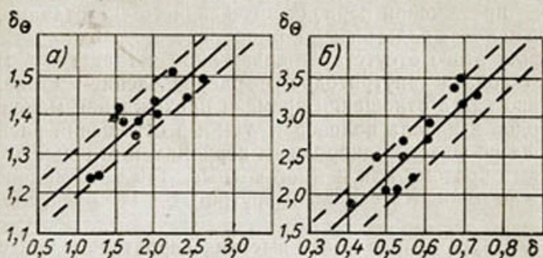
Рис. 66. Зависимость отношения стока за период июль—сентябрь к стоку за период март—июнь \delta от отношения средних температур воздуха за эти же периоды \delta_\theta .
