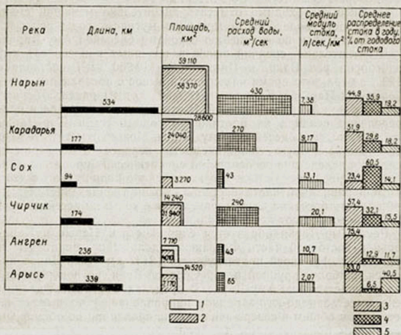
Рис. 133. Сравнительная диаграмма крупнейших рек бассейна Сыр-Дарьи. 1 — площадь бассейна, 2 — площадь водосбора, 3 — сток за март—июнь, 4 — сток за июль—сентябрь, 5 — сток за октябрь—февраль.
