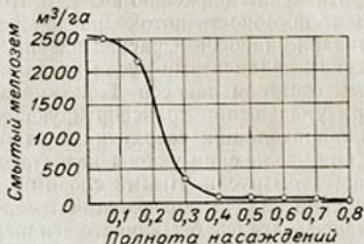
Рис. 92. Зависимость смыва грунта от полноты насаждения арчи.
