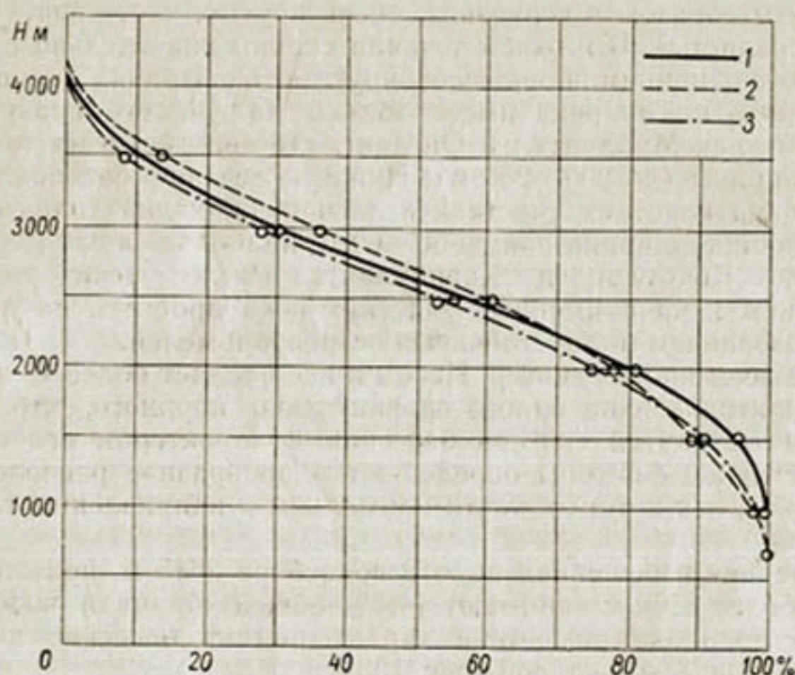
Рис. 153. Гипсометрические кривые водосборов рек Чаткал (1), Пскем (2) и Чирчик (3).
