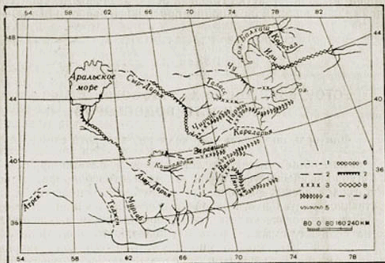
Рис. 91. Схема распределения ледовых образований по длине основных рек Средней Азии.
