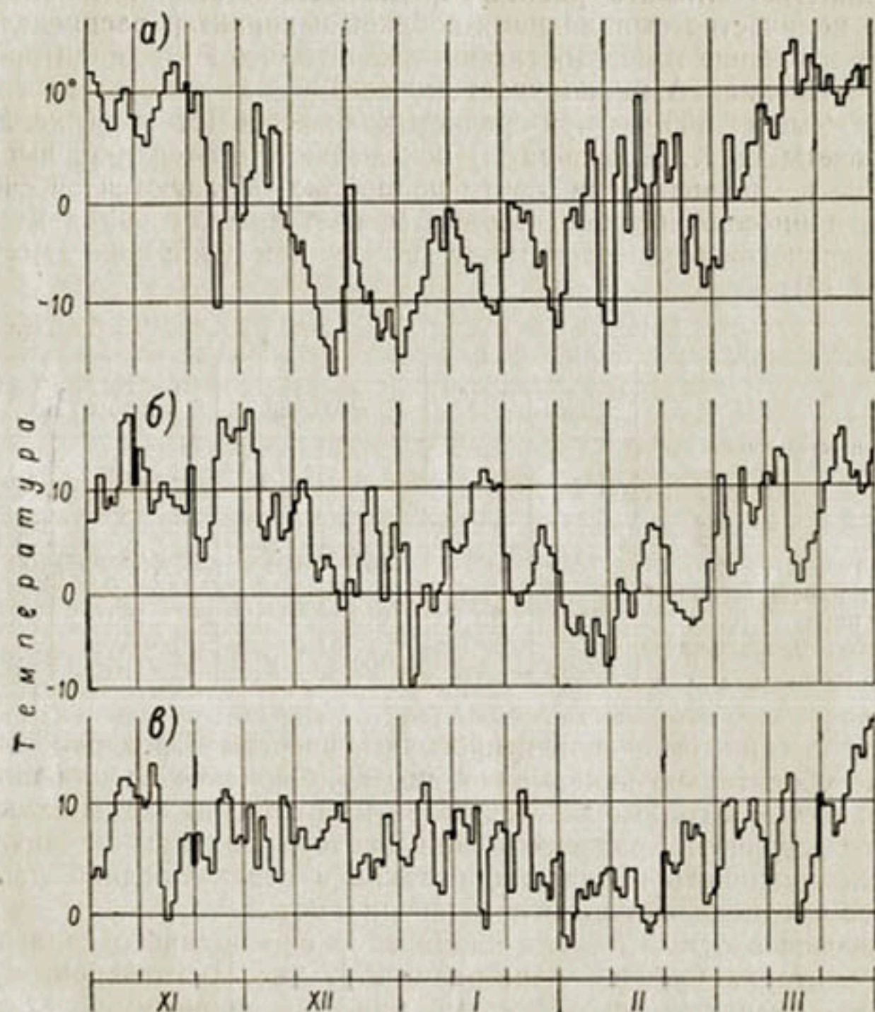
Рис. 1. Ход средних суточных температур воздуха зимой. а — 1929-30 г. (суровая зима), б — 1915-16 г. (средняя), в — 1913-14 г. (мягкая).
