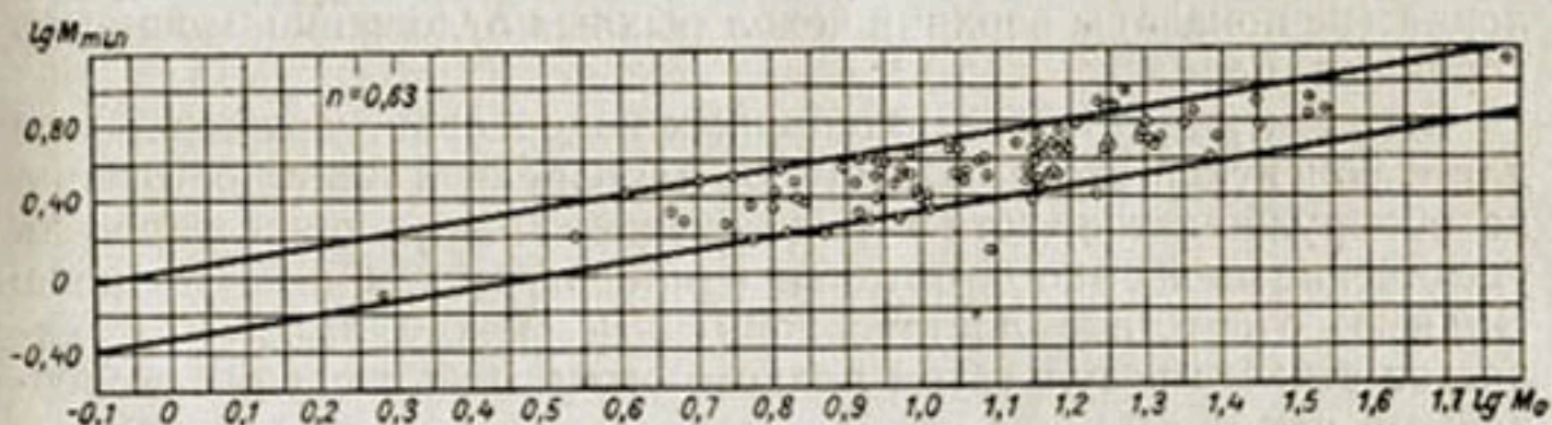
Рис. 86. Зависимость минимальных средних месячных модулей стока ( M_{min} ) от средних многолетних модулей ( M_0 ).
