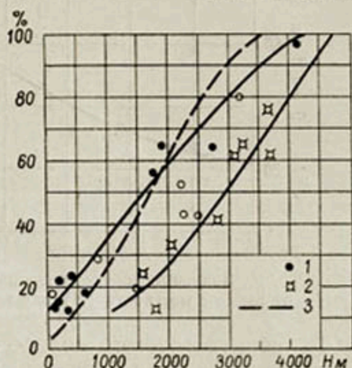
Рис. 9. Зависимость относительного количества осадков (в % от общей величины осадков) от высоты местности ( H ).
