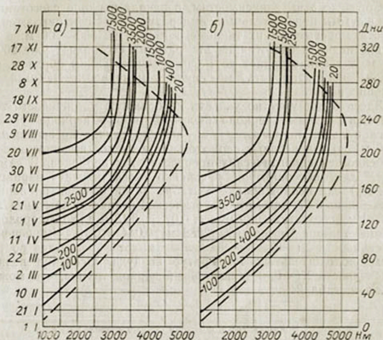
Рис. 60. Зависимость времени схода снежного покрова (положение тыла снеготаяния) от времени и высоты местности для крайних лет.
