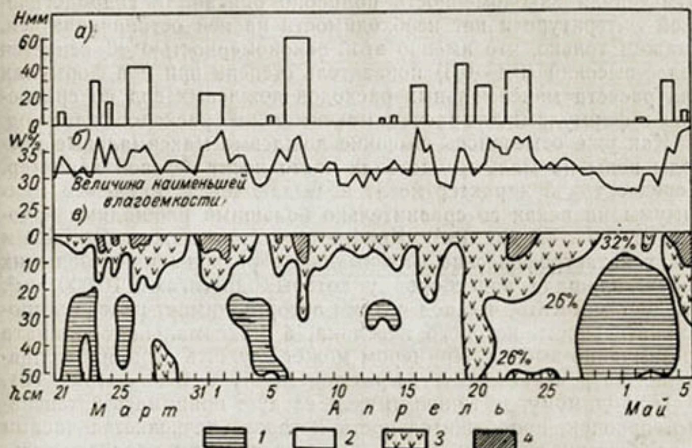
Рис. 77. Изменения влажности почвы за весенний период 1958 г. (р. Тарагайсай, южный склон хребта Каратепе).
