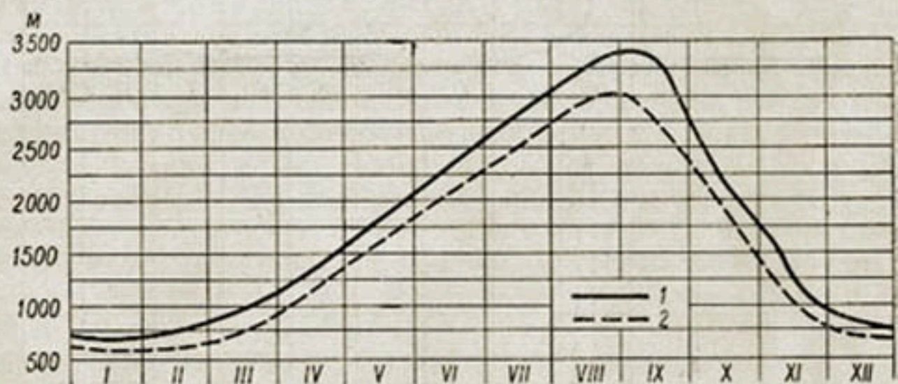
Рис. 35. Положение снеговой границы на склонах южной и северной экспозиций в долине р. Инн.
