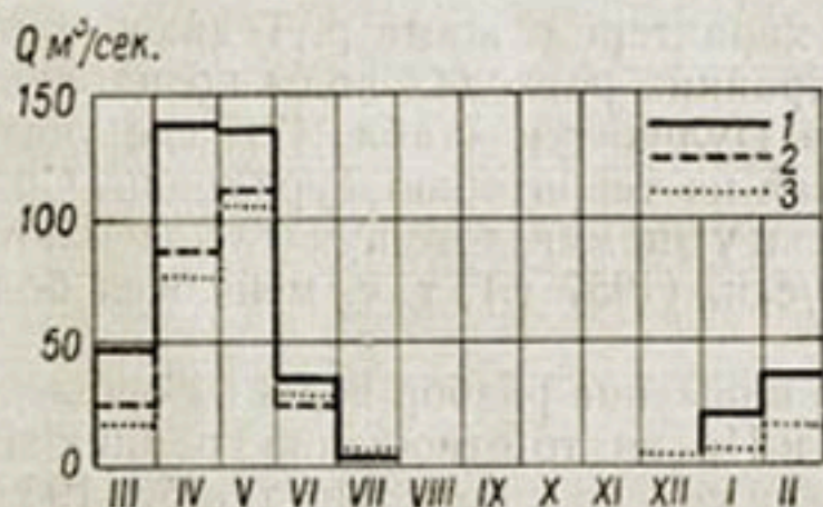
Рис. 109. Средние месячные расходы воды р. Теджен в 1930-31 г.
