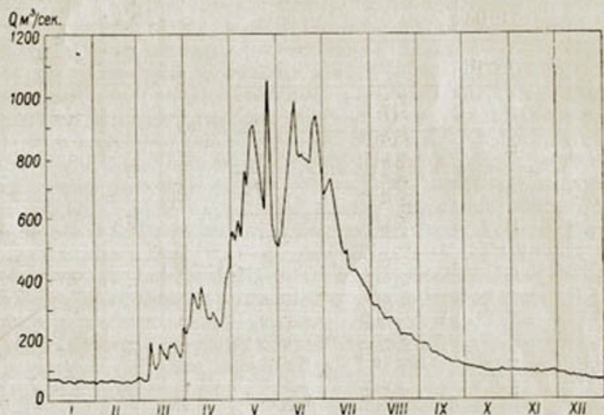
Рис. 155. Гидрограф р. Чирчик у г. Ходжикента за 1942 г.
