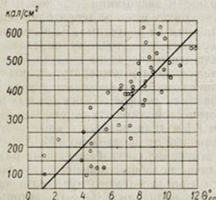
Рис. 43. Зависимость между приходом тепла и средними суточными температурами воздуха ( \theta ).
