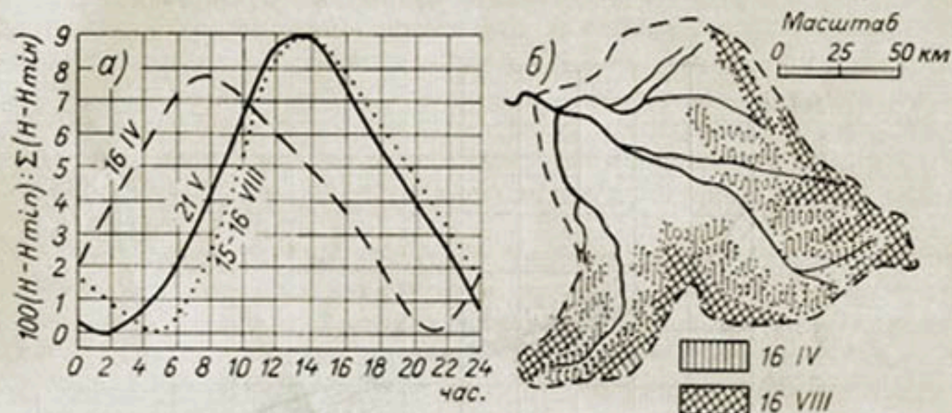
Рис. 54. Суточный ход уровней воды (а) Карадарьи в 1941 г. и схема водосбора с площадями возможного одновременного снеготаяния на 16/IV и на 16/VIII (б).
