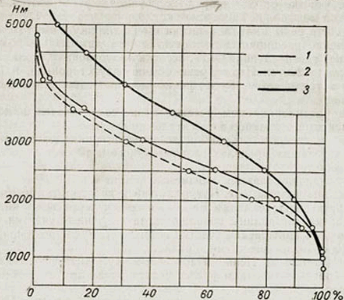
Рис. 128. Гипсометрические кривые водосборов рек Кафирниган, Варзоб и Вахш.
