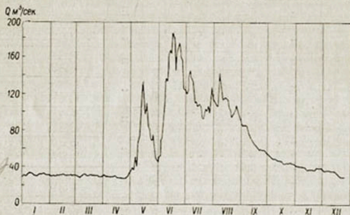
Рис. 160. Гидрограф р. Чу при выходе из гор за 1942 г.
