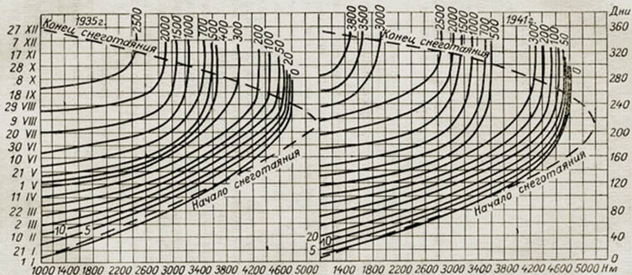
Рис. 61. Зависимость сумм положительных средних суточных температур от времени и высоты местности для характерных лет.
