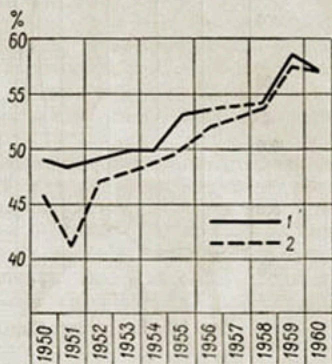
Рис. 144. Расходы воды протока Караузьяк в % от расходов воды Сыр-Дарьи.
