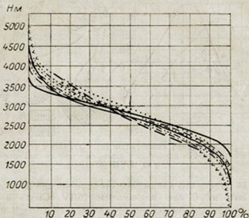
Рис. 55. Гипсометрические кривые водосборов некоторых рек Средней Азии для интервалов средневзвешенных высот 2700—2800 м.
