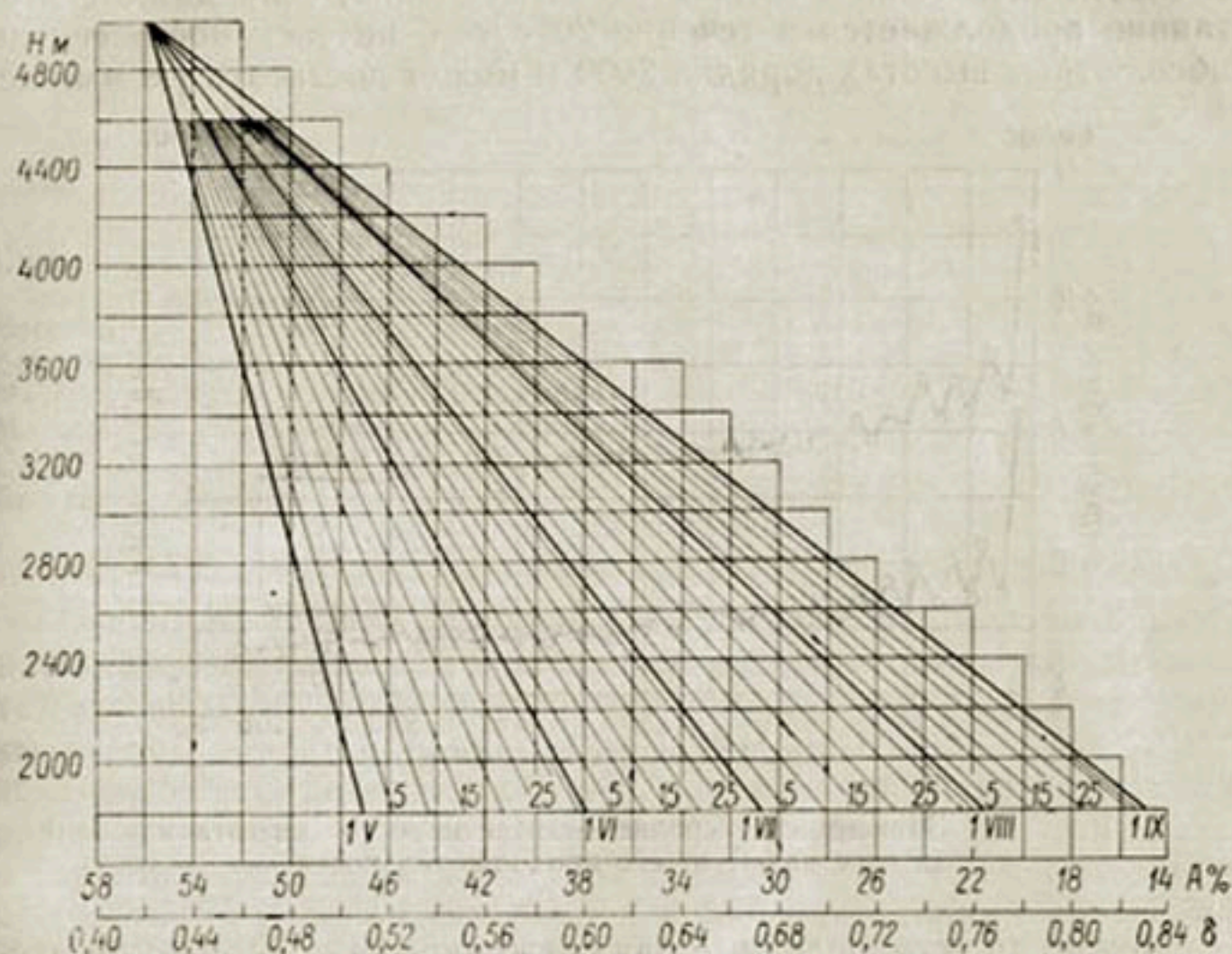
Рис. 46. Номограмма для расчета альбедо и плотности снежников в период таяния.
