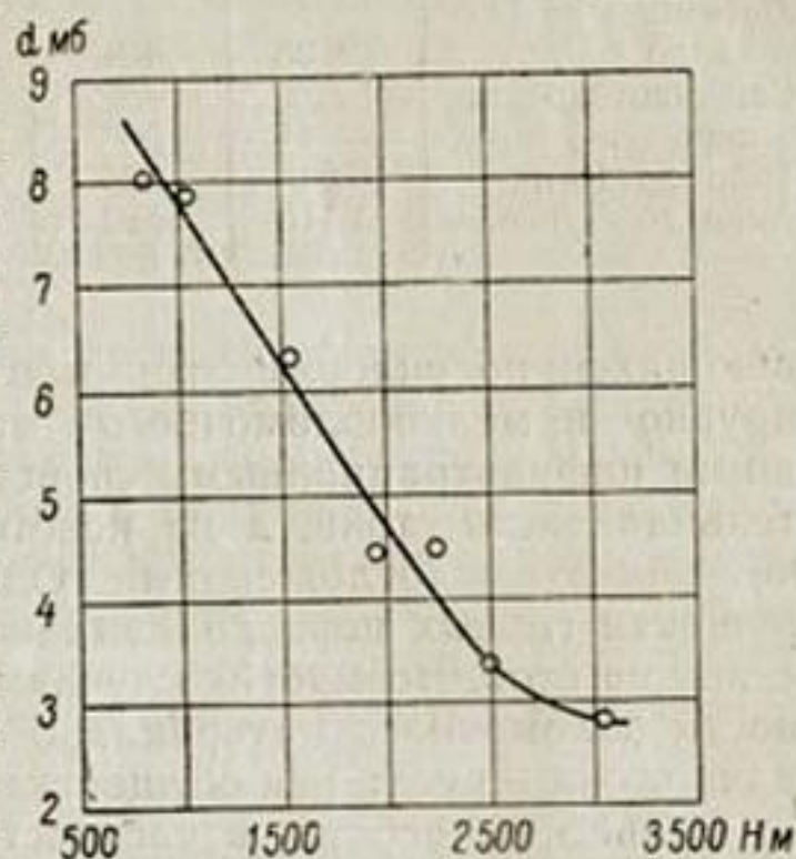
Рис. 20. Зависимость дефицита влажности ( d ) от высоты местности ( H ).
