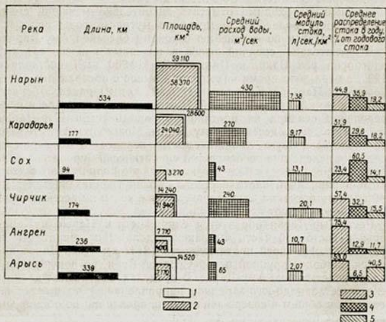
Рис. 133. Сравнительная диаграмма крупнейших рек бассейна Сыр-Дарьи. 1 — площадь бассейна, 2 — площадь подосбора, 3 — сток за март—июнь, 4 — сток за июль—сентябрь, 5 — сток за октябрь—февраль.
