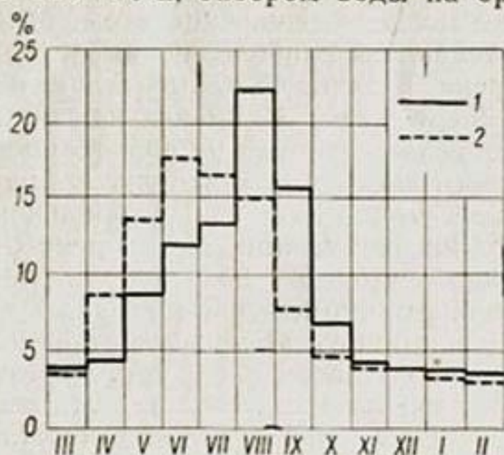
Рис. 125. Внутригодовое распределение стока Аму-Дарьи у г. Керки в % от годового.
