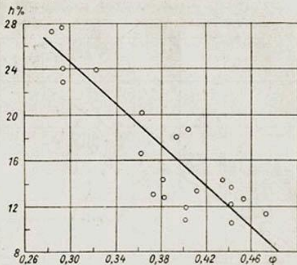
Рис. 84. Зависимость долей межennого стока в годовом ( h ) от коэффициента внутригодовой неравномерности стока ( \phi ) для южного района Средней Азии.
