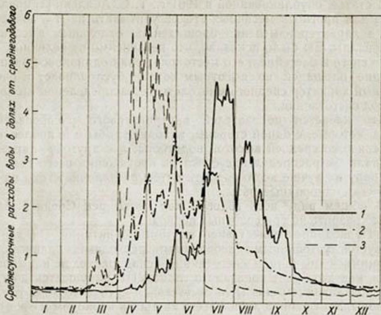
Рис. 56. Гидрографы рек за 1956 г.
