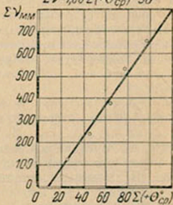
Рис. 32. Зависимость между стаиванием льда и суммами средних суточных положительных температур воздуха на леднике № 4 в бассейне р. М. Алматинки, на ледниках Имат, Казантемир и Кок-Майнак.
