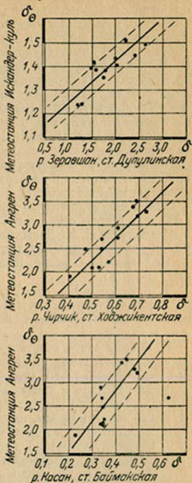
Рис. 54. Зависимость отношения стока за период июль—сентябрь к стоку за период март—июнь от отношения средних температур воздуха за эти же периоды по бассейнам рек Зеравшан, Чирчик и Каса.
