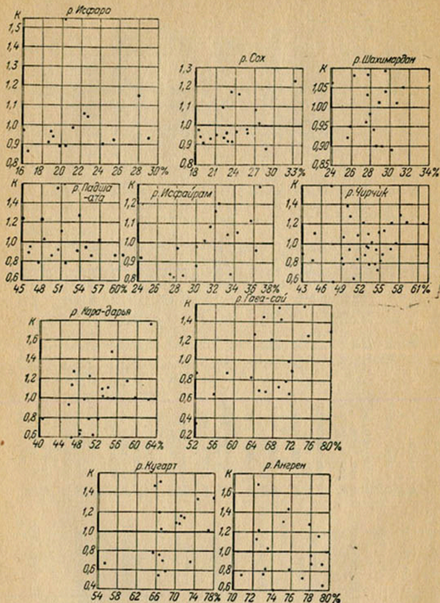
Рис. 52. Зависимость стока за период март—июль от водоносности года (модульного коэффициента (K) средних годовых расходов).
