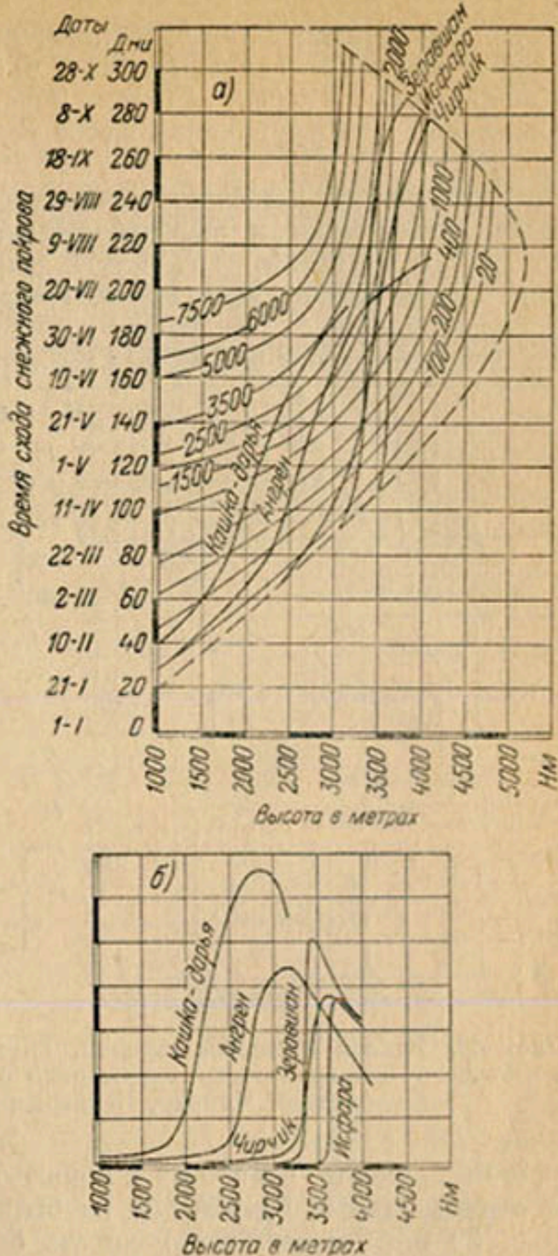
Рис. 39. Подобренные кривые тыла снеготаяния для водосборов рек Кашка-дарья, Ангрен, Чирчик, Зеравшан и Исфара (а) и зависимость влажности снежного покрова от высоты в водосборах тех же рек (б).
