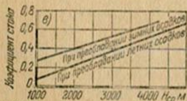
в) Зависимость коэффициентов стока от средней взвешенной высоты водосбора
