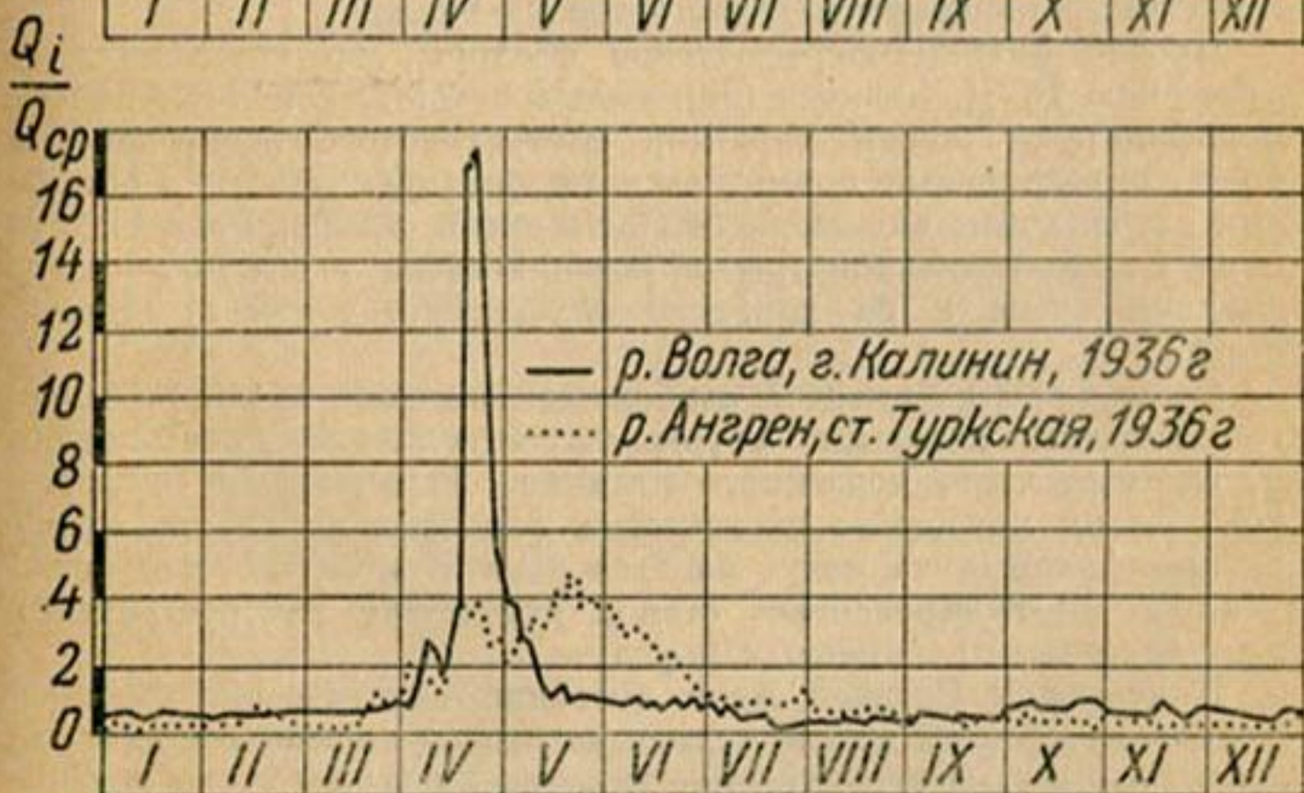
Рис. 23 и 24. Гидрографы рек Дон, Вахш, Волга и Ангрен.
