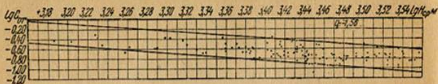
Рис. 16. Зависимость коэффициентов вариации ( C_v ) от средней взвешенной высоты водосбора ( H_{ср} ).
