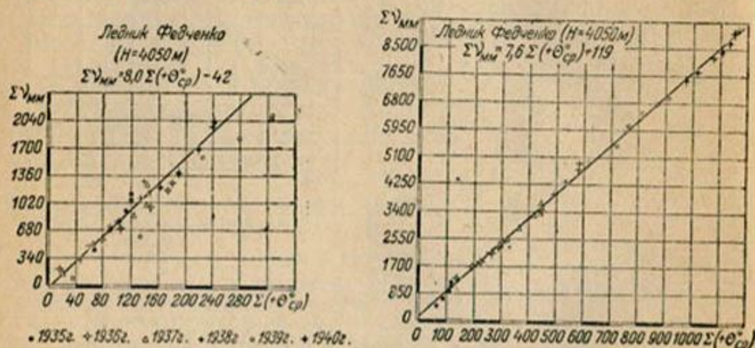
Рис. 31. Зависимость между стаиванием льда и суммами средних суточных положительных температур воздуха на леднике Федченко.
