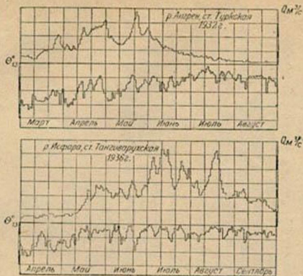
Рис. 21. Ход расходов воды и температур воздуха за период интенсивного снеготаяния в водосборах р. Ангрен (ст. Туркская) за 1932 г. и р. Исфара (ст. Тангиварухская) за 1936 г.
