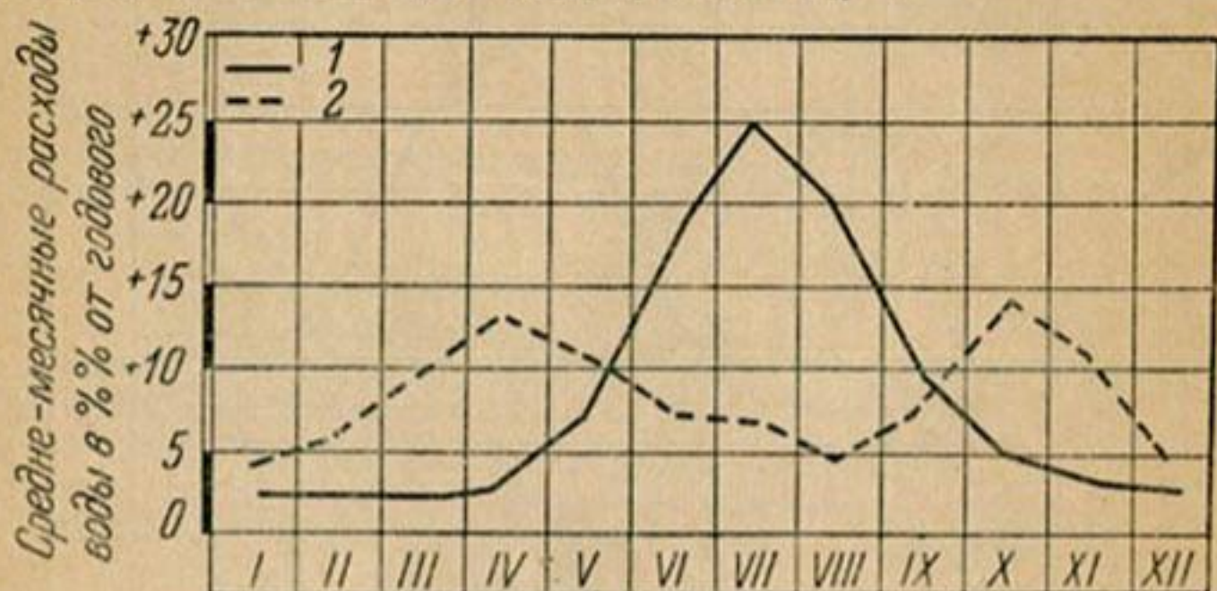
Рис. 26. Гидрографы р. Зеравшан при выходе из гор и близ устья.
