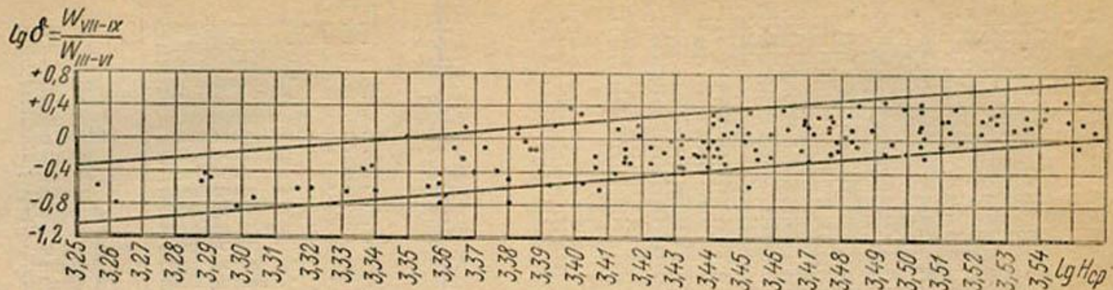
Рис. 43. Зависимость отношения стока за периоды июль—сентябрь и март—июнь ( \delta ) от средних высот водосборов ( H_{cp} ).
