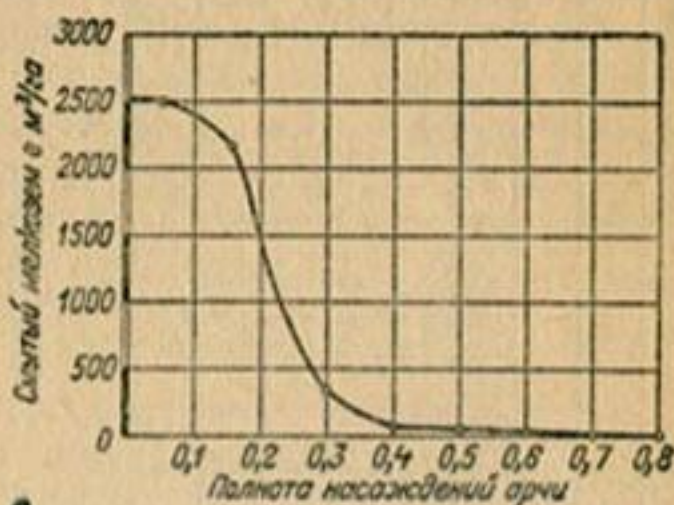
Рис. 66. Зависимость смыва от полноты насаждения арчи.
