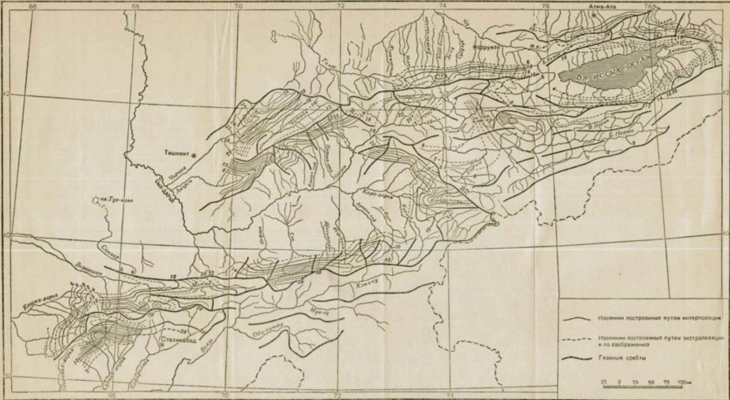
Рис. 62. Схема изотерм коэффициента A_{1\%} в формуле M_{max} = \frac{11}{T_{0,20}} для горной области Средней Азии.
