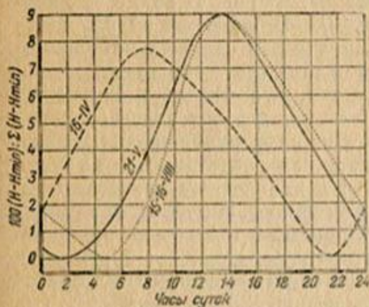
Рис. 41. Суточный ход уровней воды Кара-дарьи в 1941 г.
