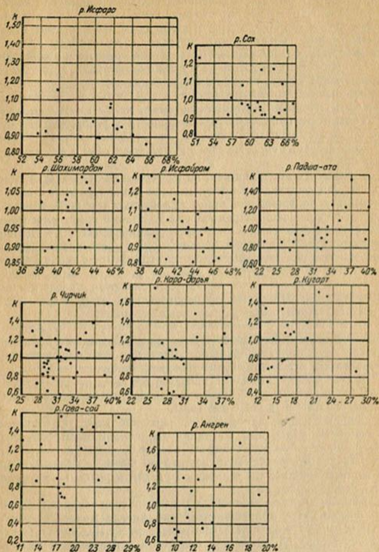
Рис. 53. Зависимость стока за период июль—сентябрь от водоносности года (модульного коэффициента ( K ) средних годовых расходов).
