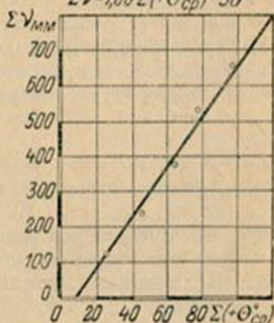
Рис. 32. Зависимость между стаиванием льда и суммами средних суточных положительных температур воздуха на леднике № 4 в бассейне р. М. Алматинка, на ледниках Имат, Казантемир и Кок-Майнок.
