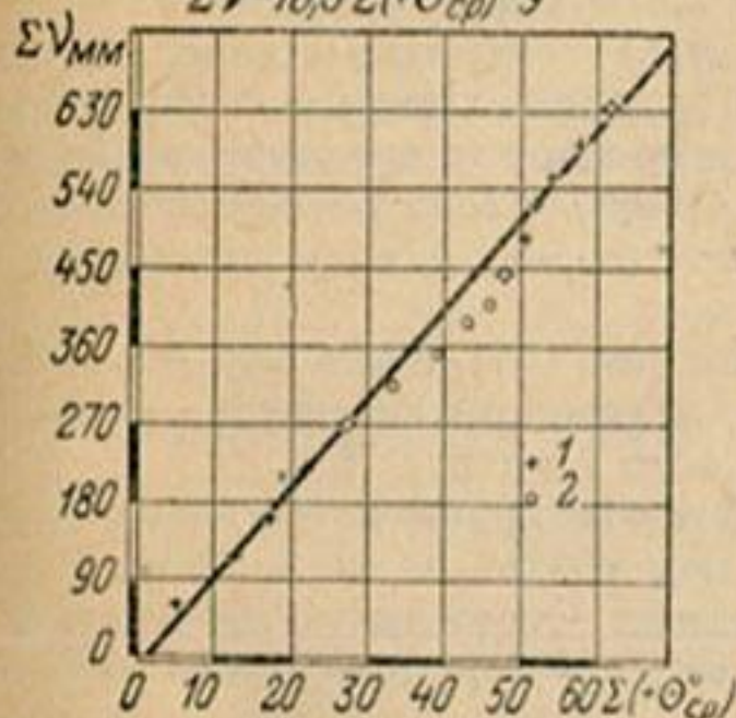
Рис. 32. Зависимость между стаиванием льда и суммами средних суточных положительных температур воздуха на леднике № 4 в бассейне р. М. Алматинка, на ледниках Имат, Казантемир и Кок-Майнок.
