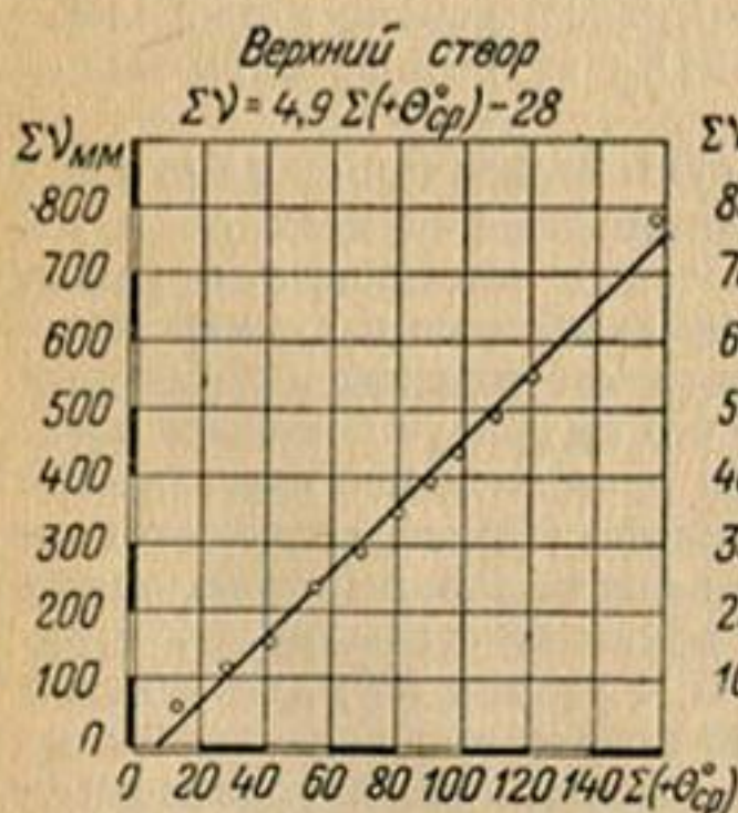
Рис. 35. Зависимость между стаиванием снега и суммами средних суточных температур воздуха на снежнике северного склона Большого Чимгана (верхний и нижний створы).
