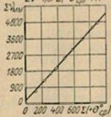
Рис. 33. Зависимость между стаиванием льда и суммами средних суточных положительных температур воздуха на ледниках Караугом, Башкара и Алладин.
