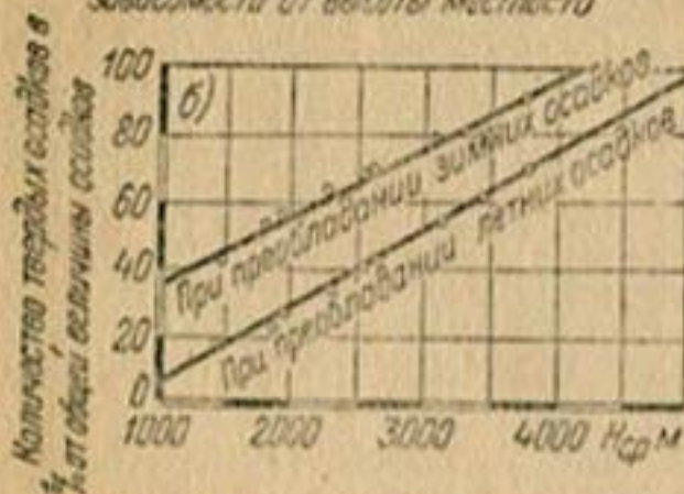
б) Зависимость относительного количества твердых осадков от средней взвешенной высоты водосбора
