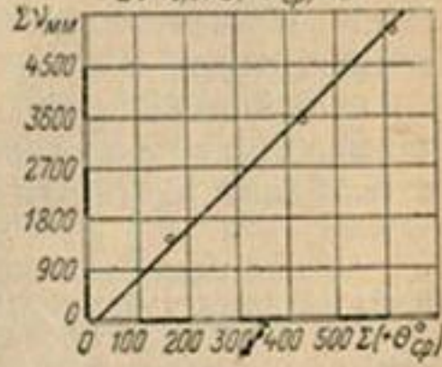
Рис. 33. Зависимость между стаиванием льда и суммами средних суточных положительных температур воздуха на ледниках Караугом, Башкара и Алладин.
