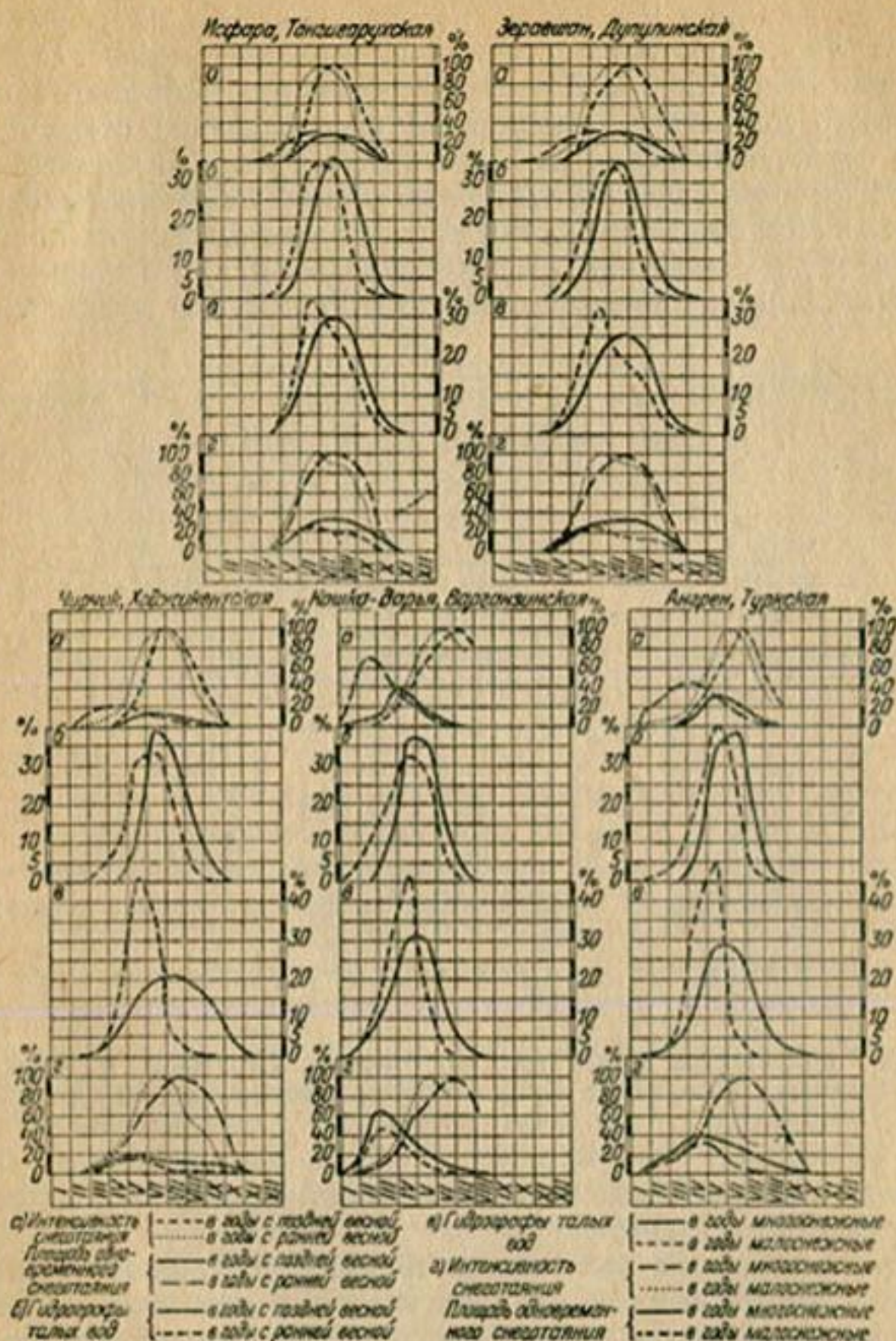
Рис. 49. Интенсивность снеготаяния, гидрографы талых вод и площади возможного одновременного снеготаяния при различной водности снежного покрова и различном термическом режиме в водосборах рек Исфара, Зеравшан, Чирчик, Ангрен, и Кашка-дарья.
