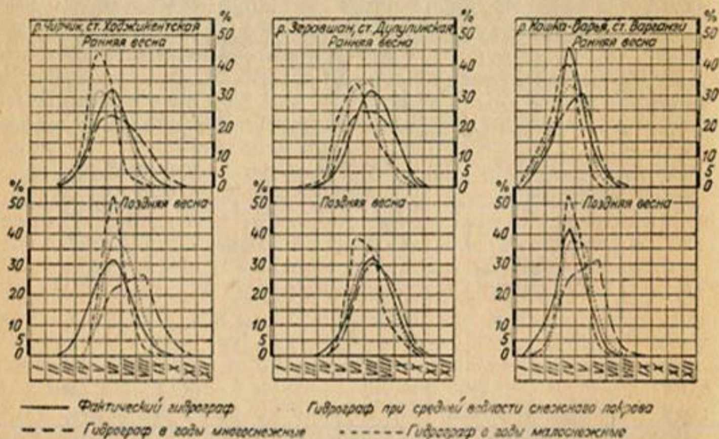
Рис. 50. Гидрографы талых вод рр. Чирчик, Зеравшан и Кашка-дарья при различных сочетаниях термического режима и водности снежного покрова.
