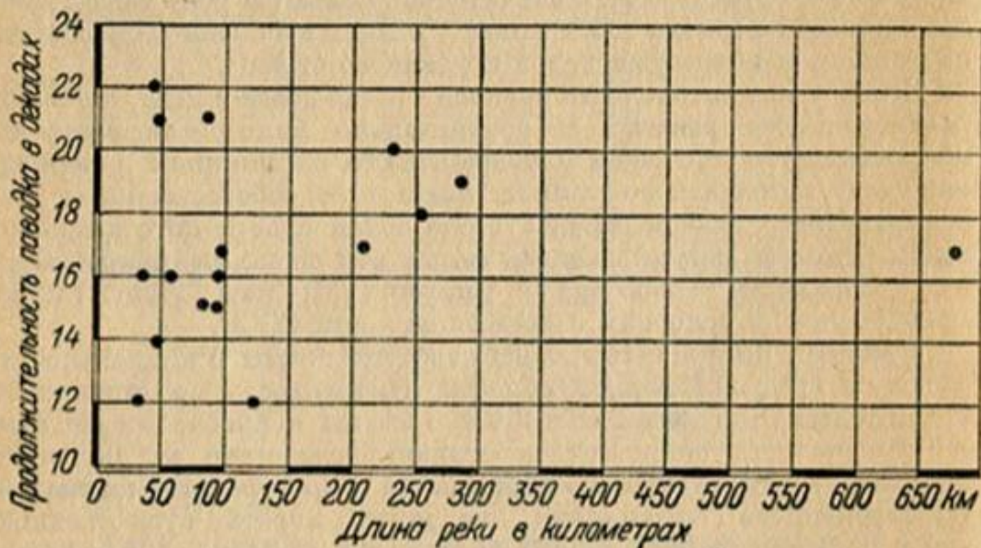
Рис. 51. Зависимость продолжительности паводка от длины реки.
