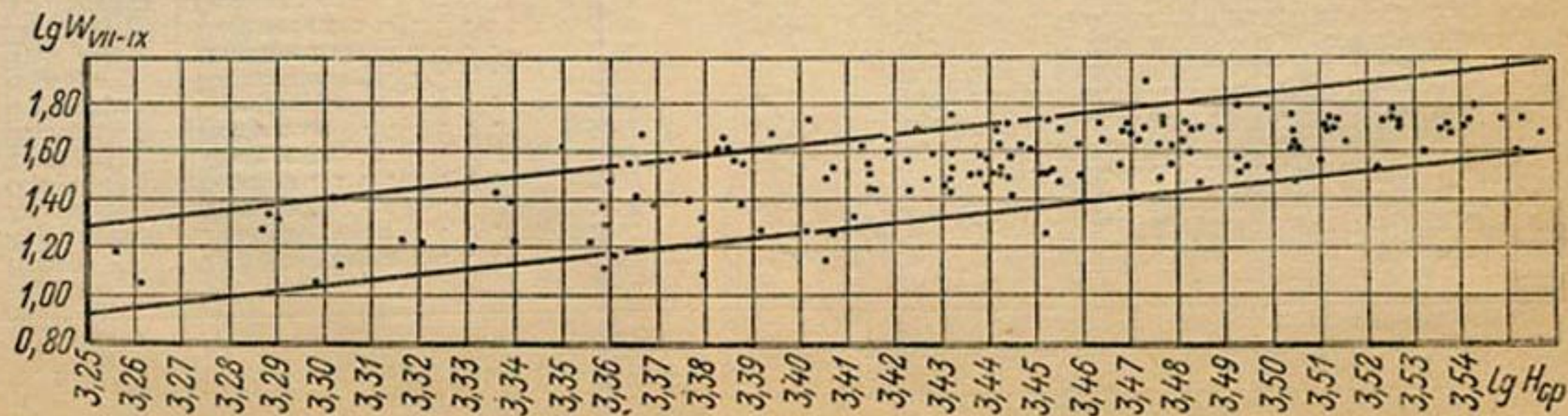
Рис. 44. Зависимость стока за период июль—сентябрь ( W_{VII-IX} ) от средних высот водосборов ( H_{cp} ).
