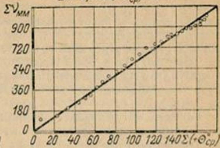
г) Ледник Кок-Майнок около Фирна (H=3170м) \Sigma V = 7,00 \Sigma(+\theta_{\text{ср}}^{\circ}) - 50
