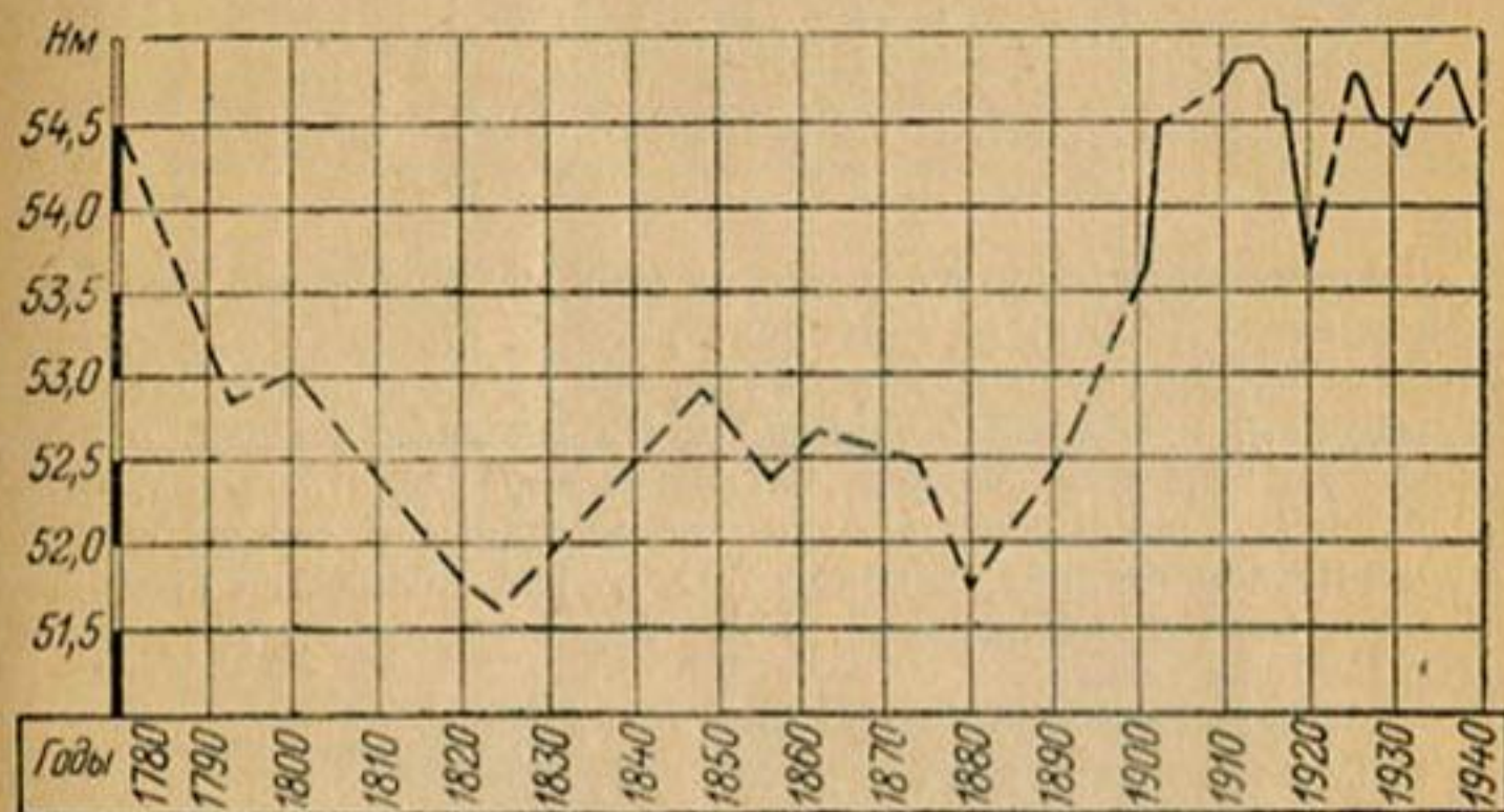
Рис. 14. Колебание средних годовых уровней Аральского моря.
