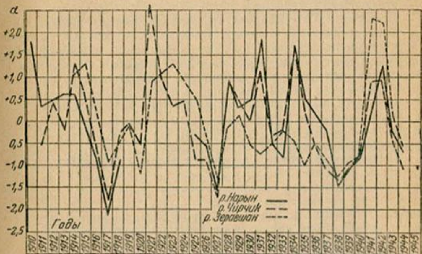
Рис. 18. Хронологическая последовательность лет различной водоносности у рек Нарын, Зеравшан и Чирчик.
