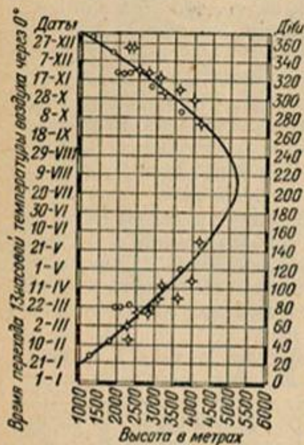
Рис. 27. Зависимость среднего времени перехода температур воздуха в 13 часов через 0° (положения фронта снеготаяния) от высоты местности.
