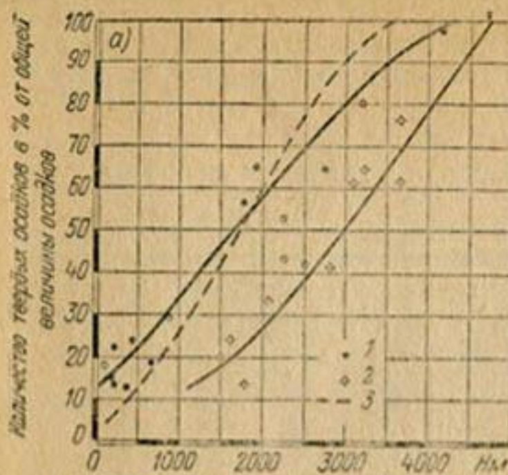
а) Относительное количество твердых осадков в зависимости от высоты местности
