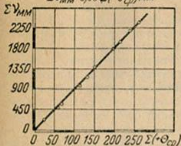
в) Ледник Казантемир 24/VIII-7/IX 1933г. \Sigma V = 10,3 \Sigma(+\theta_{\text{ср}}^{\circ}) - 9
