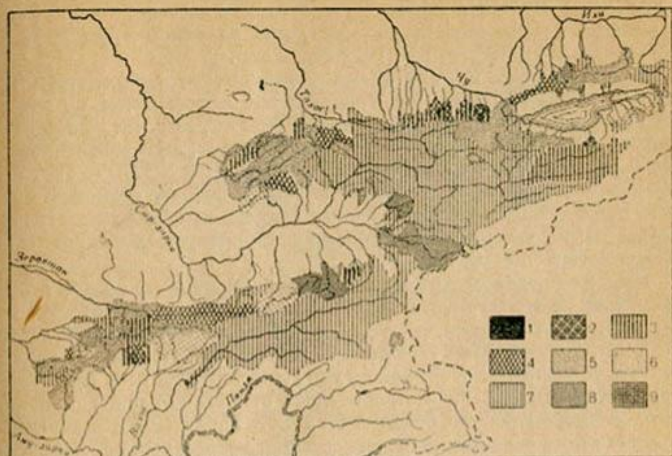
Рис. 19 1-7 . Распределение водоносности по территории Средней Азии.
