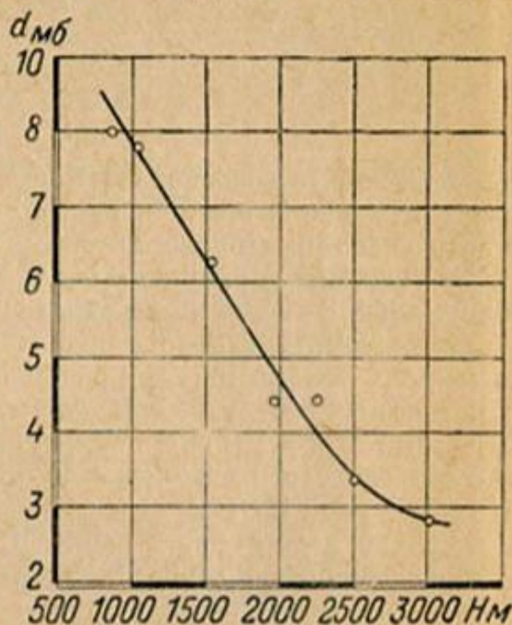
Рис. 11. Зависимость дефицита влажности от высоты местности.
