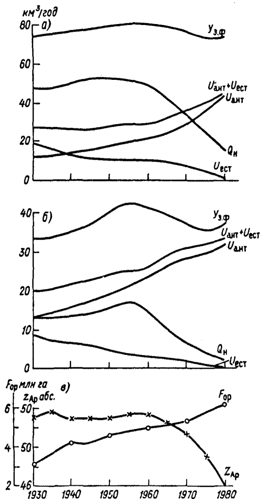
Рис. 7. Динамика значений водных ресурсов в зоне формирования Y_{з.ф.} , стока в замыкающем створе Q_n , естественных U_{ест} и антропогенных U_{ант} потерь стока для р. Амударья — Чатлы (а) и р. Сырдарья — Казалинск (б), уровней Аральского моря и суммарных площадей в его бассейне (в).
