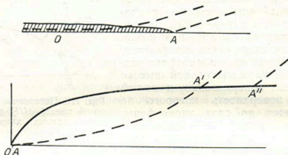
Рис. 113. Зарождение и возможное развитие ледникового покрова при низкой хионосфере.
