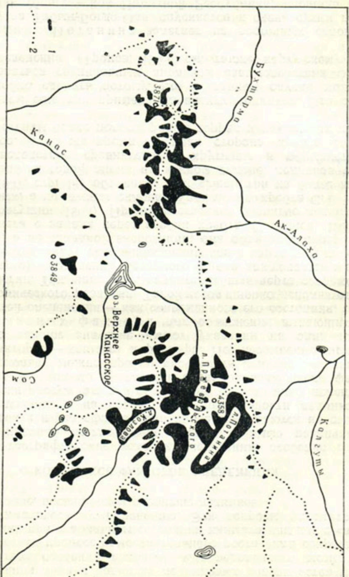
Рис. 12. Схема дельников восточной части Южно-Алтайского хребта (по Б. В. Тронову и М. В. Тронову) и горного узла Табын-Богдо-Ола (по В. В. Сапожникову).
