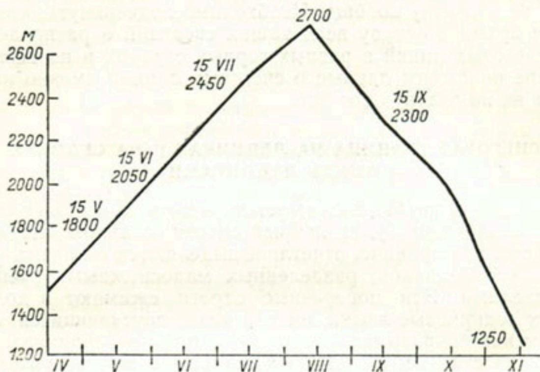
Рис. 14. Сезонное изменение высоты снеговой линии для области Зоннблика (по Мареку).
