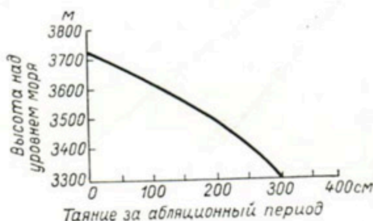
Рис. 57. Связь стаивания льда на поверхности Туюксуйских ледников с высотой места (по Н. Н. Пальгову).
