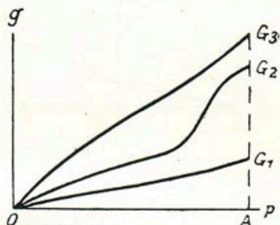
Рис. 102. Простые ледниковые кривые.
