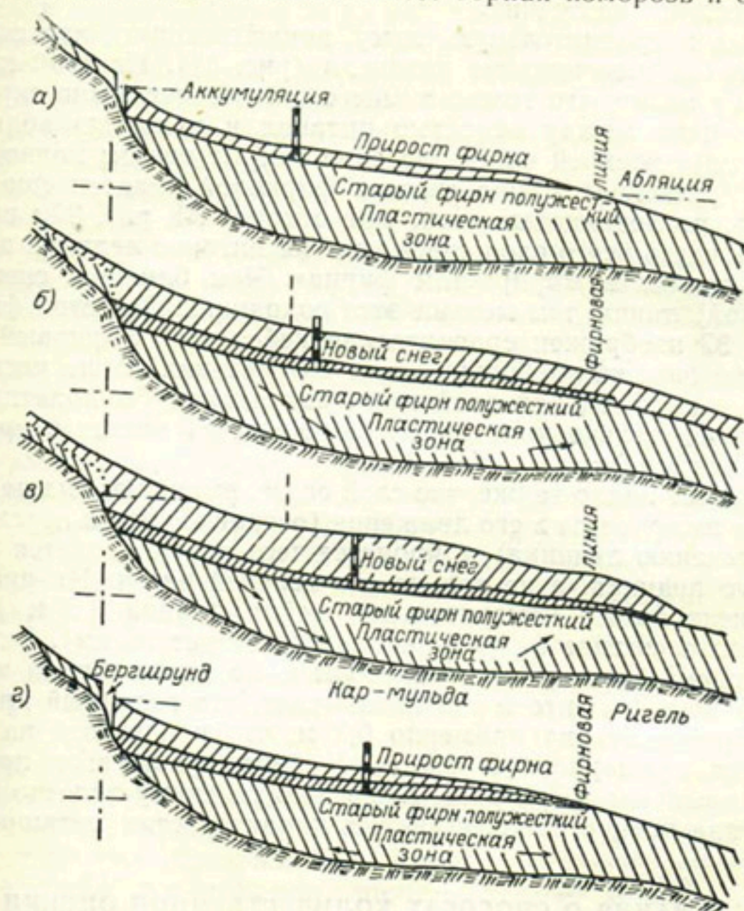
Рис. 37. Ход развития фирнового слоя (по Р. Штрейф-Беккеру). а — 15 сентября 1950 г., б — март 1951 г., в — июнь 1951 г., г — 15 сентября 1951 г.
