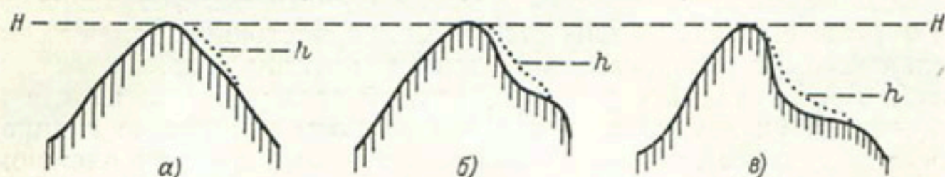
Рис. 22. Соотношение между границей оледенения ( H ) и высотой снеговой линии на ледниках ( h ).
