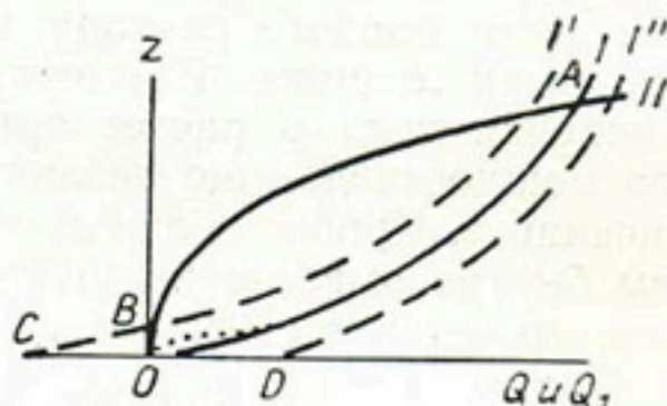
Рис. 93. Общий вид кривых накопления ( I, I', I'' ) и истечения ( II ).
