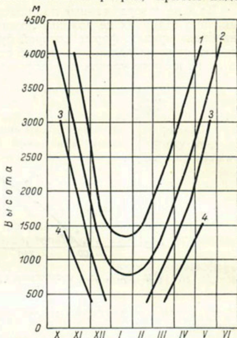
Рис. 27. Изменение с высотой дат образования и разрушения устойчивого снежного покрова (по О. М. Челпановой).
