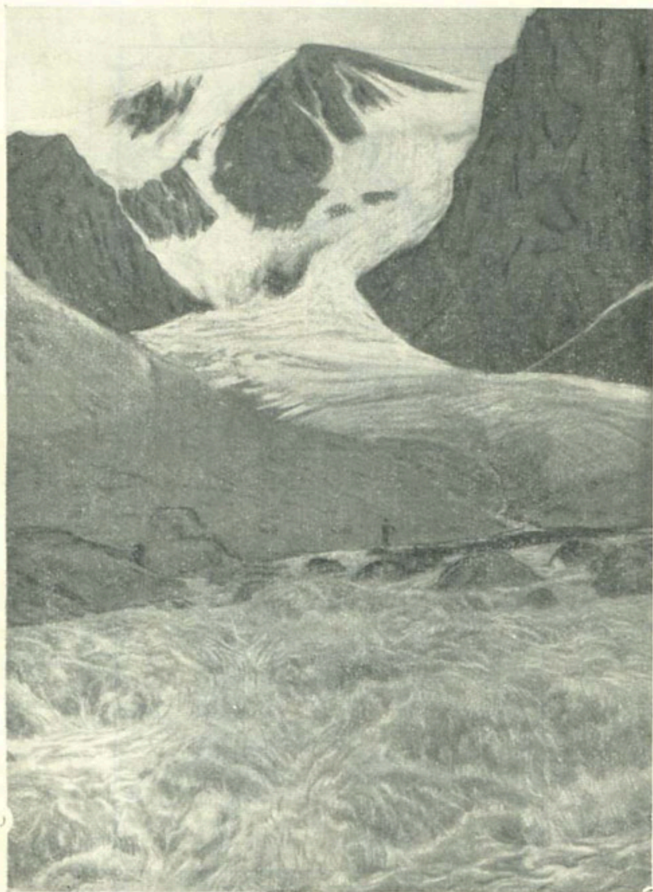
Рис. 42. Исток реки с ледниковым питанием.
