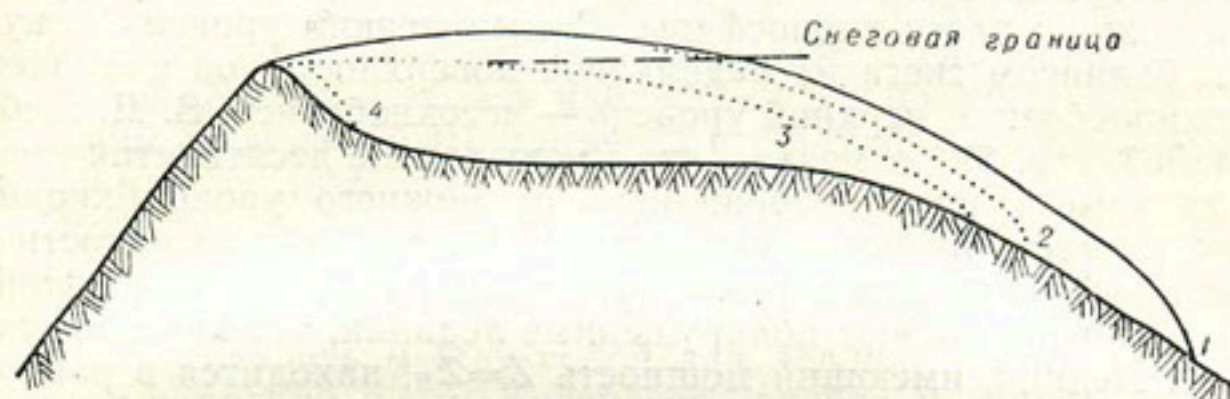
Рис. 98. Схема, иллюстрирующая значение инерции сохранения ледников, залегающих на плоских ступенях и водоразделах.
