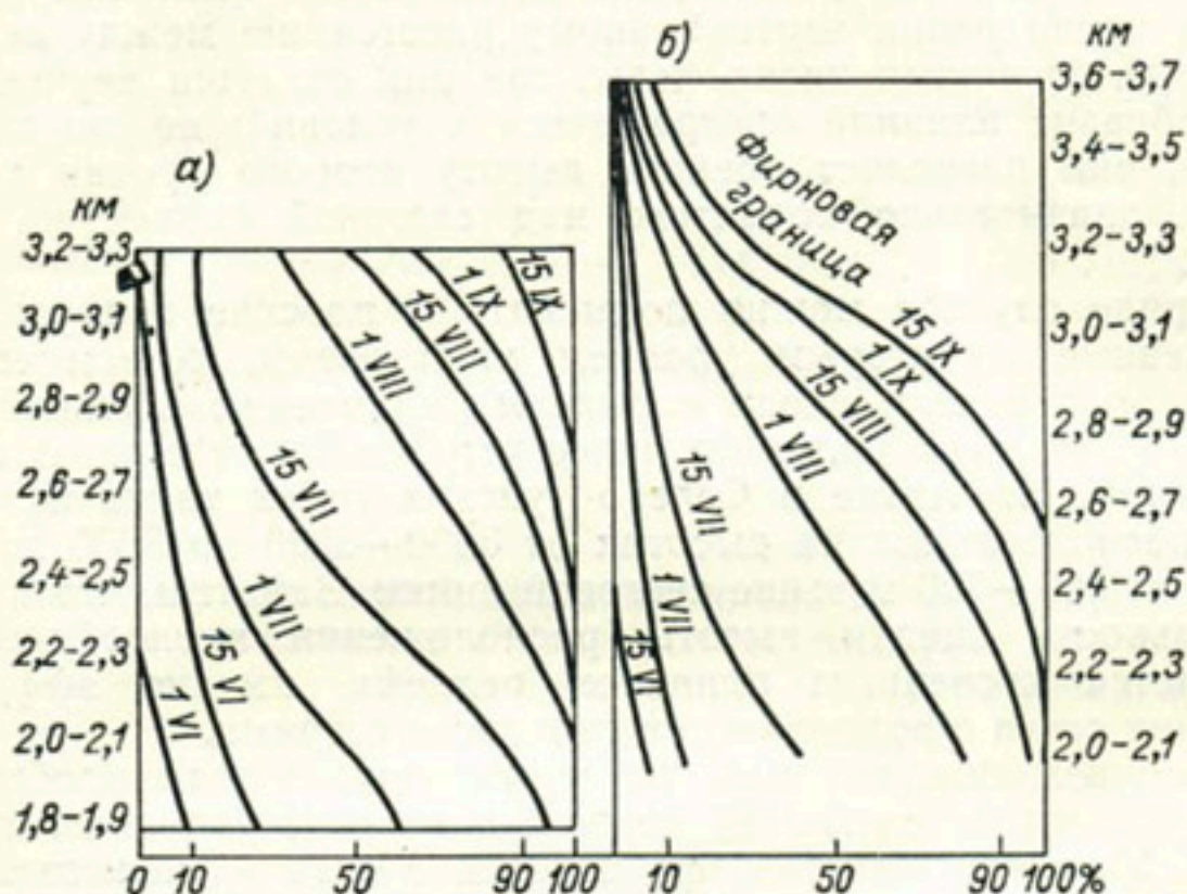
Рис. 26. Степень обнажения поверхностей (%) в области ледника Пастерце (по Г. Фриделю). 1935 г. а — склон без ледника, б — ледниковая поверхность.
