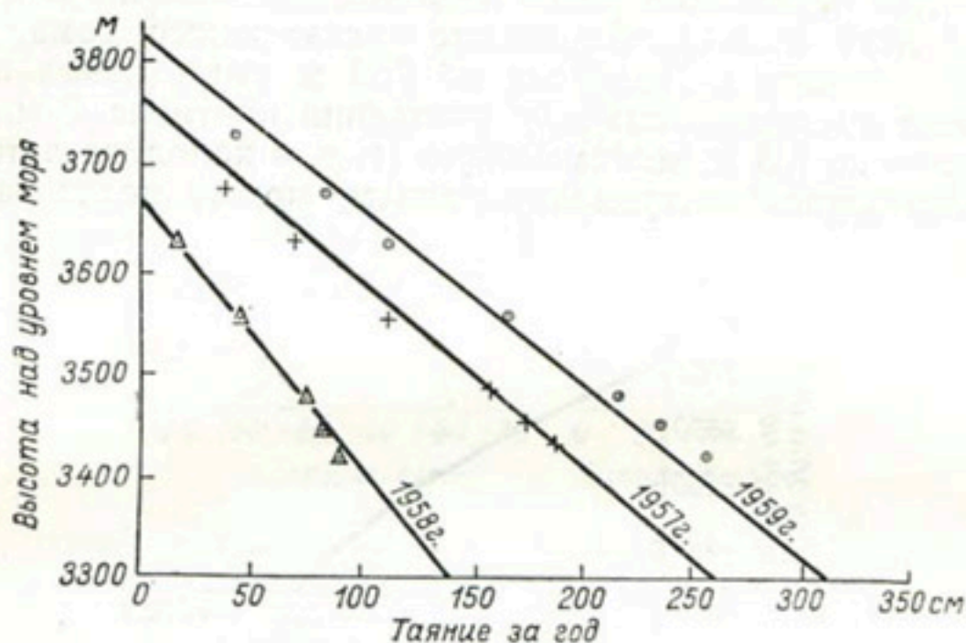
Рис. 58. Среднее суммарное стаяние льда на поверхности Туюксуйских ледников в разные годы на различной высоте (по Е. М. Калмыкиной).
