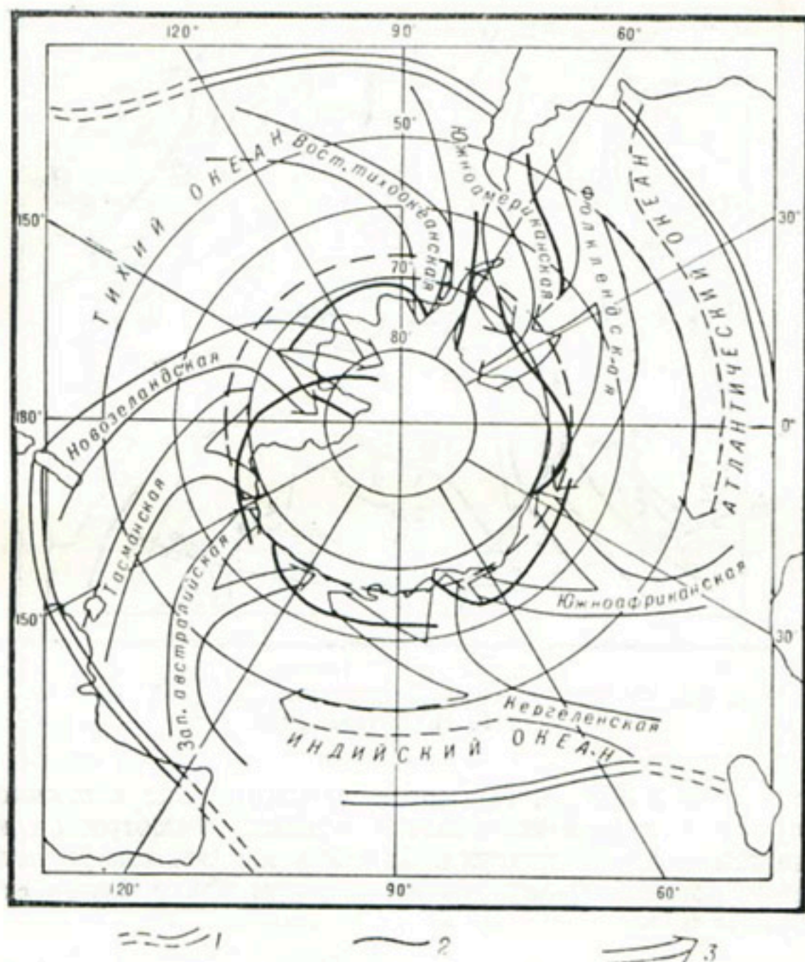
Рис. 53. Траектории циклонов над океаном и положение главных фронтов зимой (по П. Д. Астапенко).
