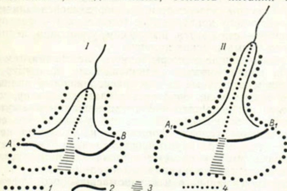
Рис. 11. Неподпруженный (I) и подпруженный (II) ледники.
