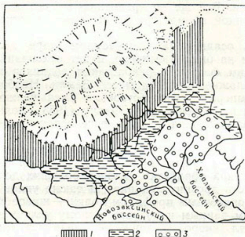
Рис. 87. Схематическая карта растительного покрова Русской равнины в эпоху валдайского оледенения (по В. П. Гричук, 1952).
