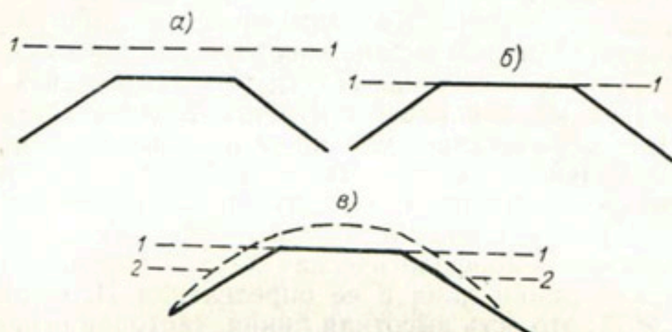
Рис. 13. Схема образования снеговой линии.
