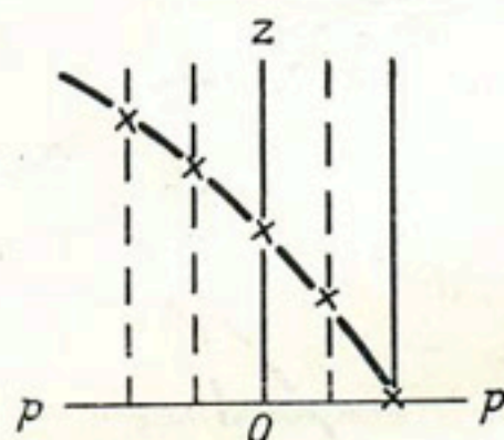
Рис. 106. Простая балансовая кривая в случае изменения климата.
