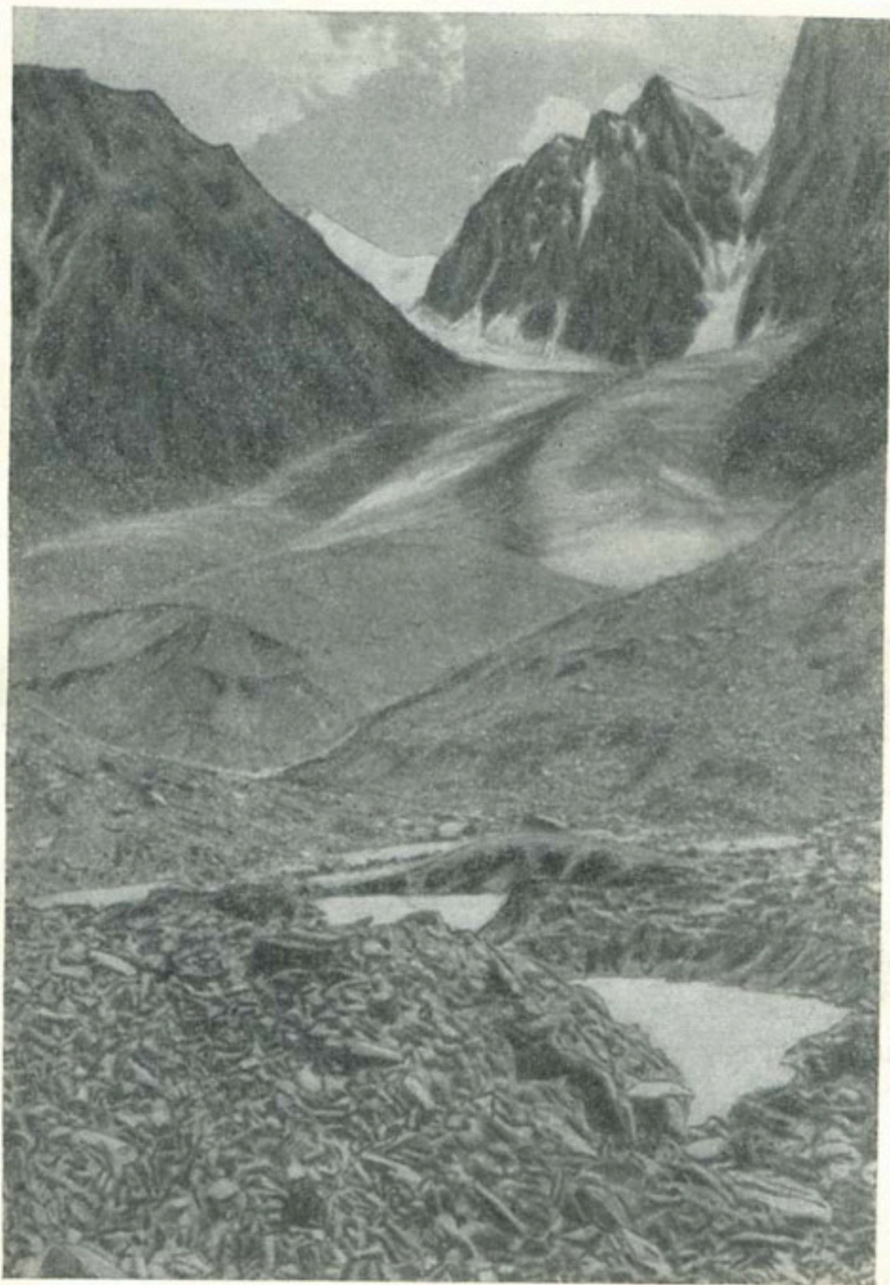
Рис. 81. Конец ледника, загруженный мореной.
