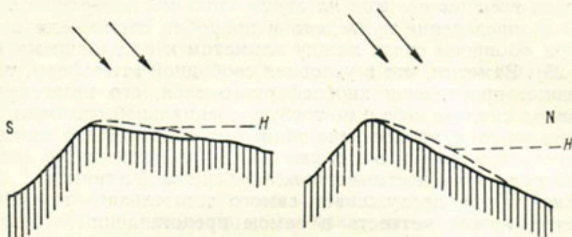
Рис. 19. Снижение снеговой линии на северном склоне большой крутизны.
