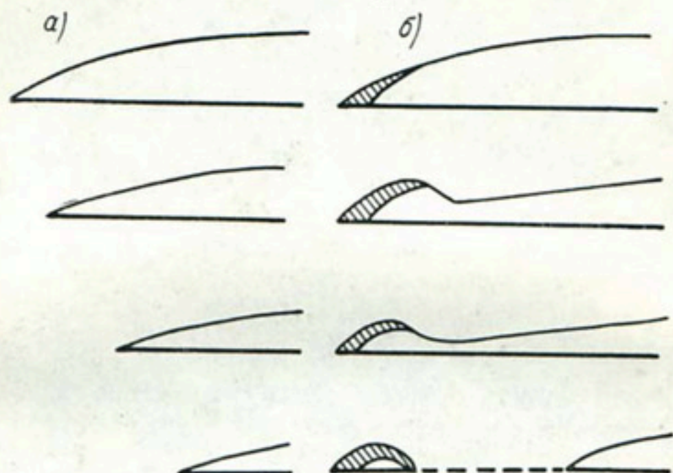
Рис. 63. Скачок в линейном сокращении ледника, конец которого консервируется мореной. а — сокращение незагрязненного ледника, б — возникновение изолированной глыбы мертвого льда.
