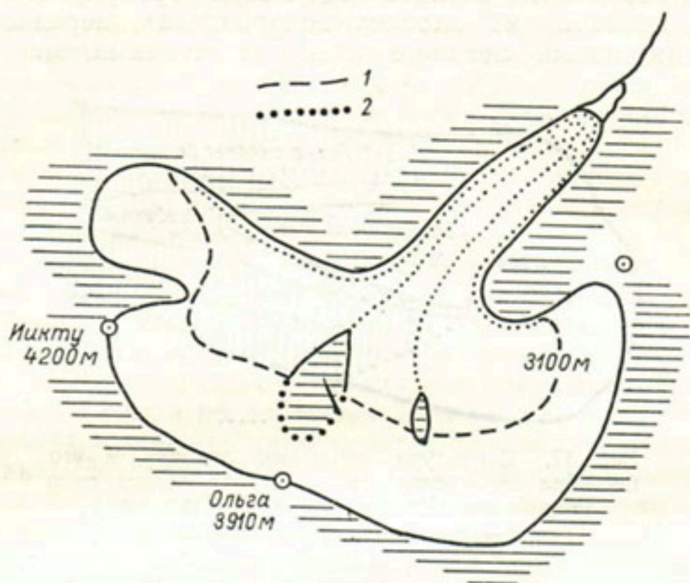
Рис. 16. Схема Талдуринского ледника (по В. В. Сапожникову).
