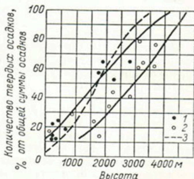
Рис. 2. Схема зависимости относительного количества твердых осадков от высоты местности.
