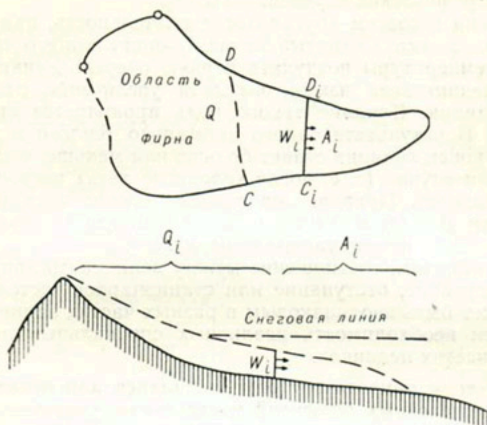
Рис. 83. Общие условия стационарности ледника для произвольно взятого поперечного профиля ( Q_i = W_i = A_i ).
