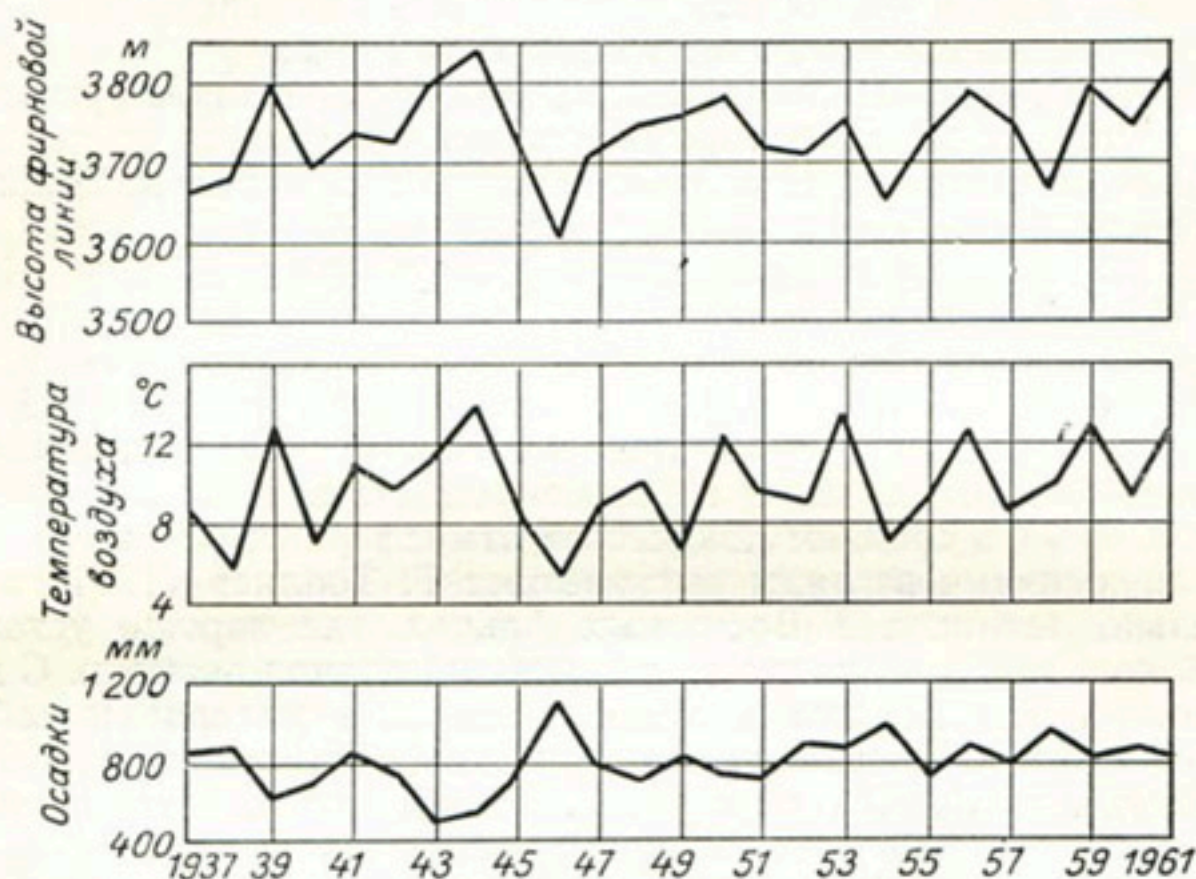
Рис. 82. Ход основных метеорологических элементов и высоты фирновой линии на Центральном Туяксийском леднике (по Н. Н. Пальгову).
