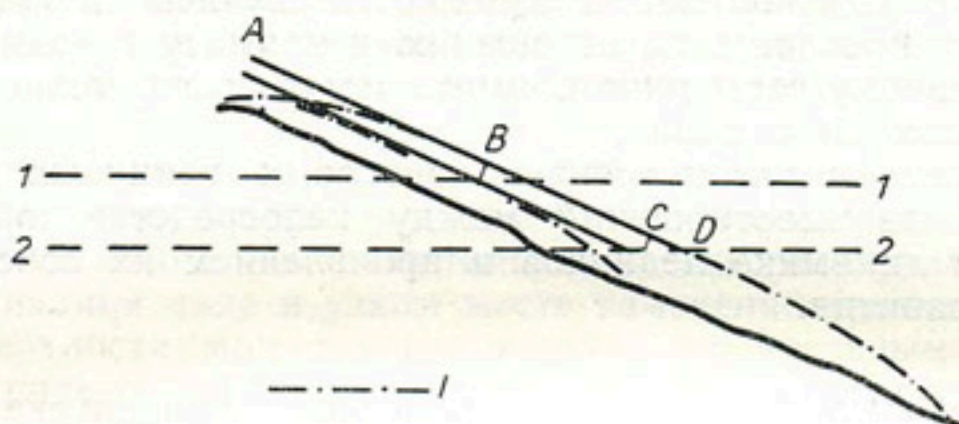
Рис. 89. Изменение размеров ледника простейшего вида при понижении снеговой линии от уровня 1—1 к уровню 2—2.
