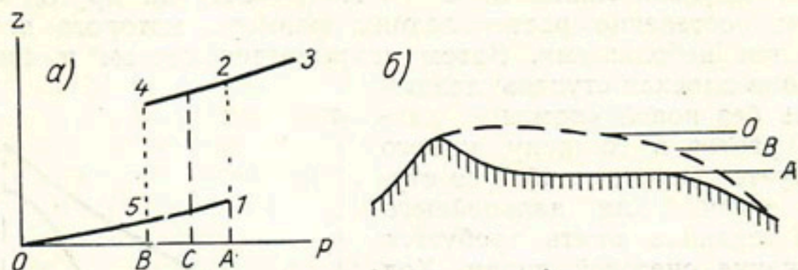
Рис. 103. Сложная ледниковая кривая.
