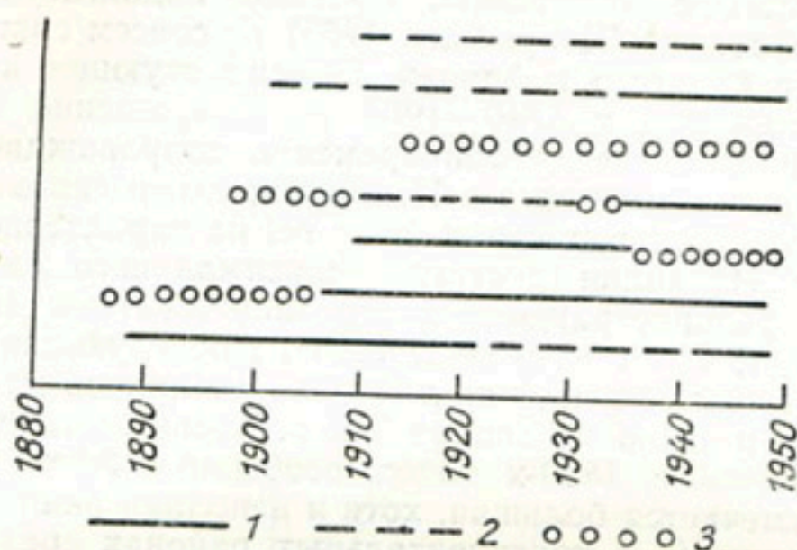
Рис. 76. Характер колебаний некоторых ледников в западной части гор Чугач (Аляска) (по С. В. Калеснику).
