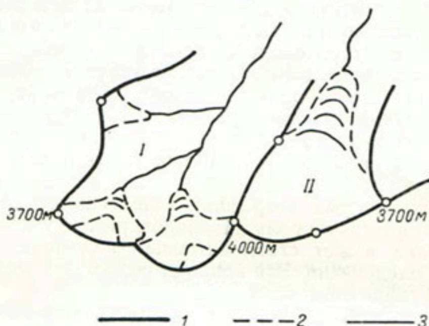
Рис. 9. Схема, иллюстрирующая принцип соответствия. Образование нескольких малых ледников в «слишком большом» бассейне (I) и одного крупного ледника в бассейне меньших размеров (II).
