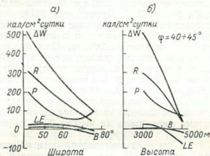
Рис. 64. Изменения с широтой места (а) и высотой (б) составляющих теплового баланса ледников северного полушария (по М. К. Гавриловой).
