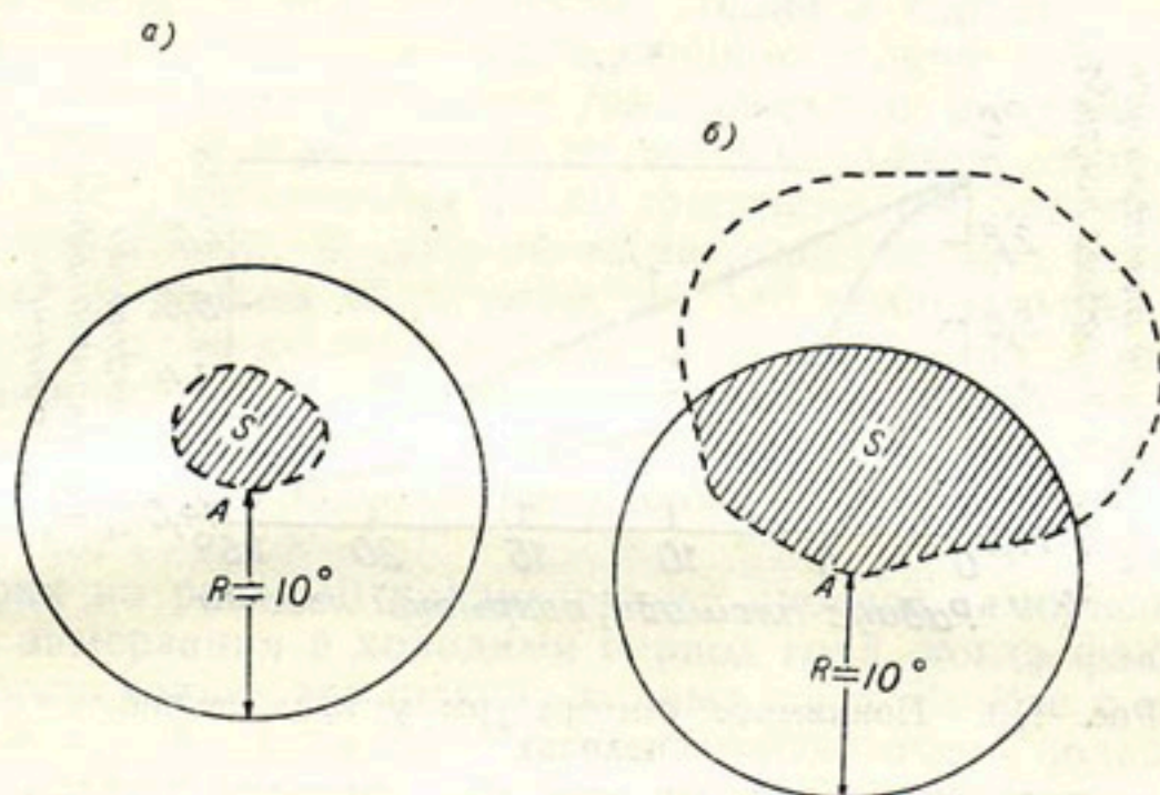
Рис. 109. Схема, поясняющая расчет охлаждающего влияния ледникового покрова (по К. Бруксу).
