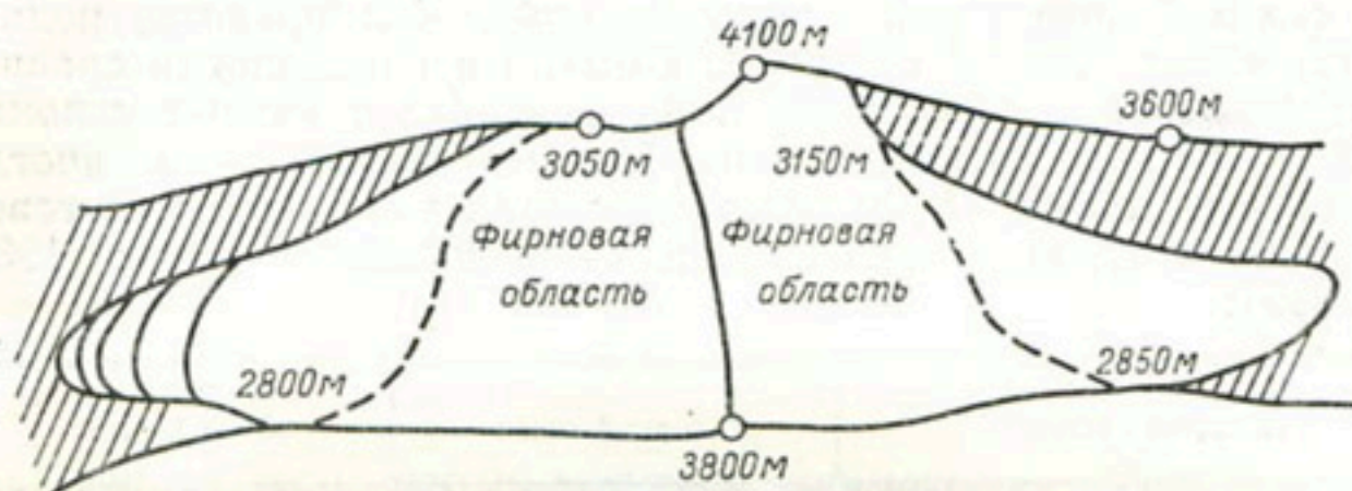
Рис. 30. Схема расположения снеговой линии на ледниках, имеющих западную и восточную экспозицию.
