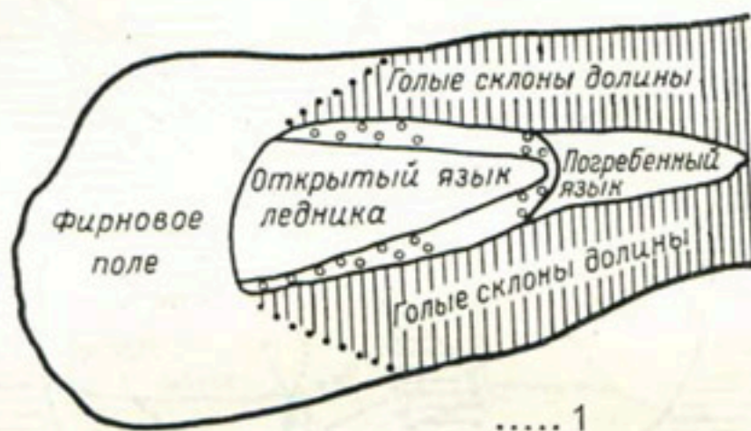
Рис. 17. Структура типичного ледника и его бассейна в центральном районе оледенения Заилийского Алатау (по Н. Н. Пальгову).
