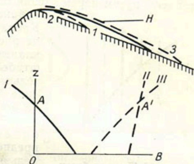
Рис. 105. Построение балансовых кривых простой формы. I — общая, II — приходная, III — расходная.
