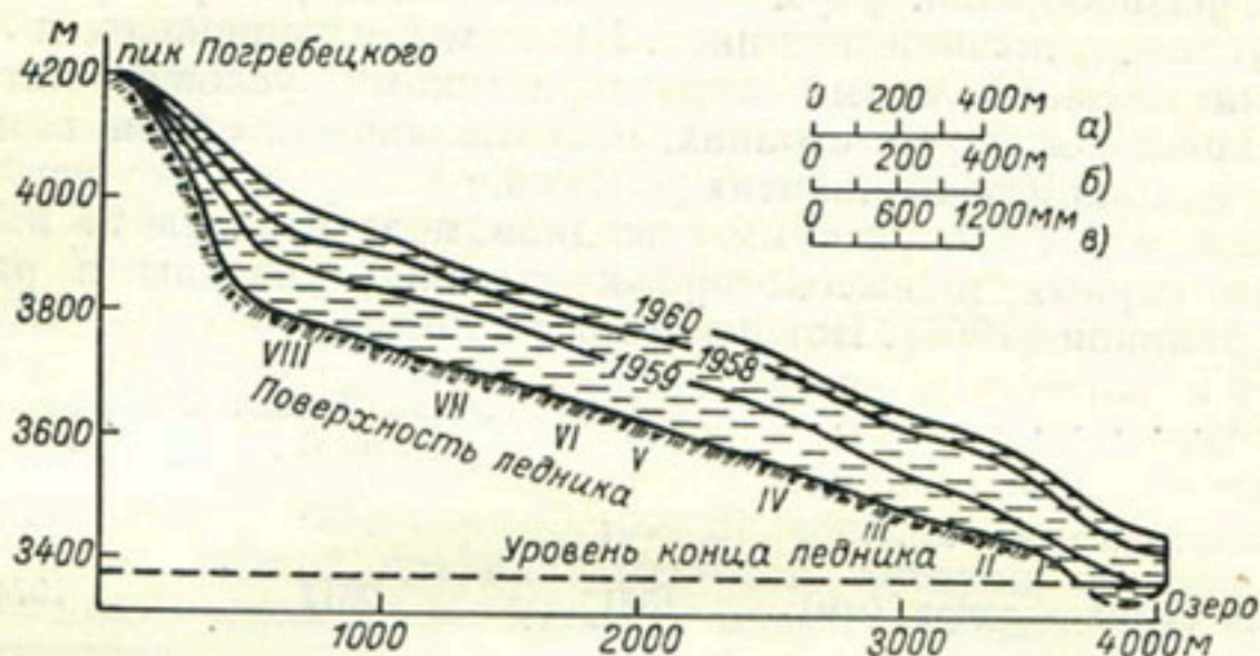
Рис. 46. Распределение запасов воды в снежном покрове на Центральном Тууксуйском леднике (по П. А. Судакову и Е. Н. Вилесову).
