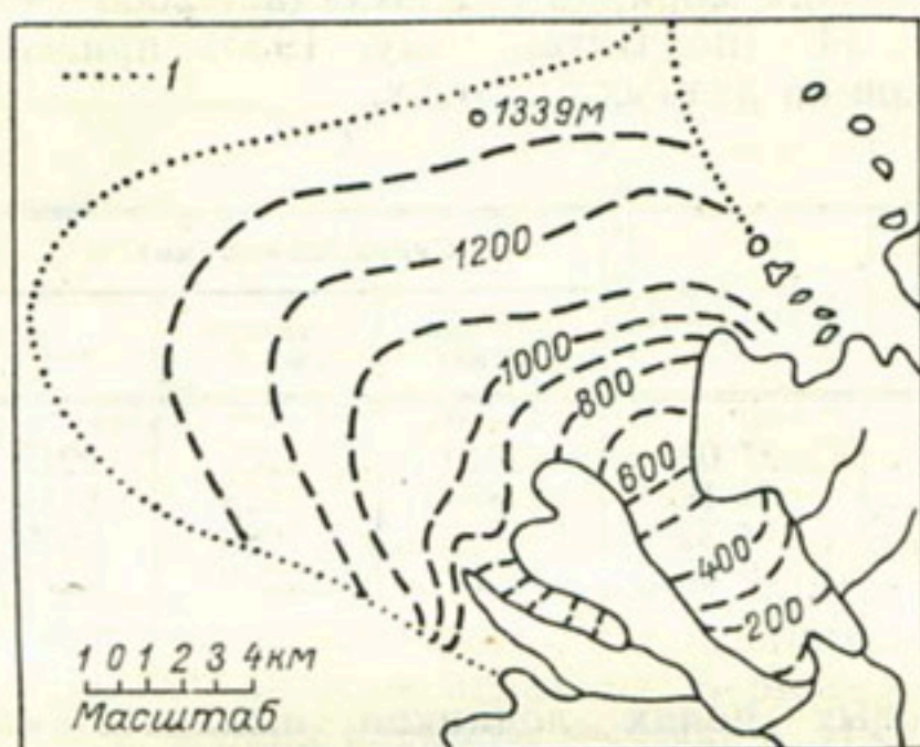
Рис. 47. Ледник Хоффельсйокуль в 1937 г. (по Г. Альману).
