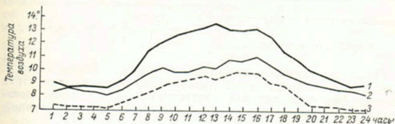
Рис. 1. Суточный ход температуры воздуха над ледником и над камнями (по Г. П. Дубинскому). 1 — над камнями, 2, 3 — над ледником.
