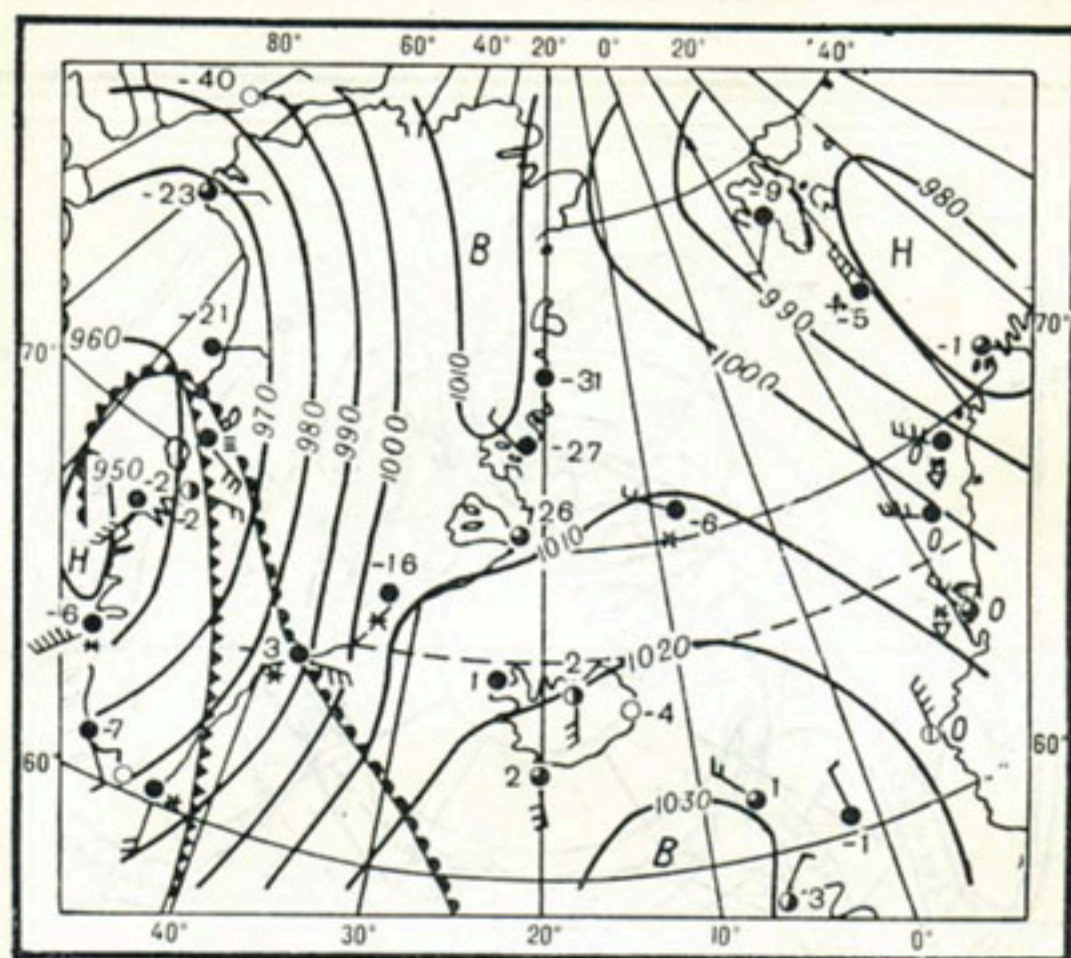
Рис. 52. Циклоническая деятельность над Гренландией (по Г. Н. Витвицкому).
