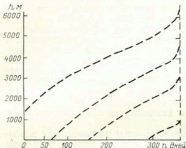
Рис. 29. Семейство кривых зависимостей n от h .
