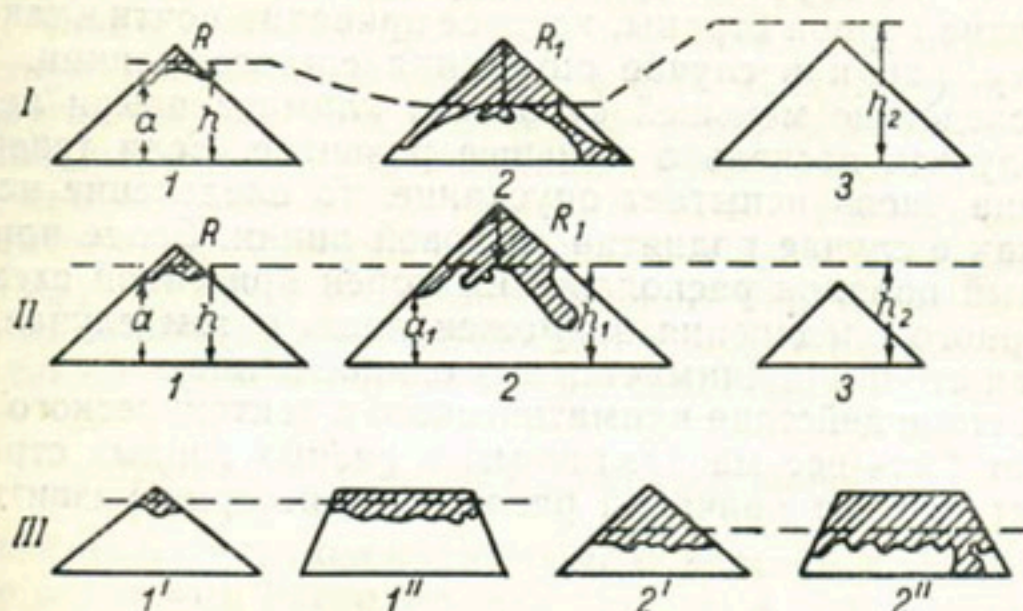
Рис. 5. Роль общеклиматического, тектонического и геоморфологического факторов в развитии оледенения (по К. К. Маркову).
