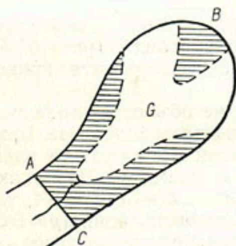
Рис. 104. Ледник и ледниковый бассейн.
