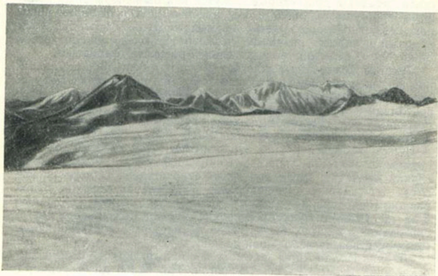
Рис. 10. Ледник, залегающий в широком плоском бассейне.
