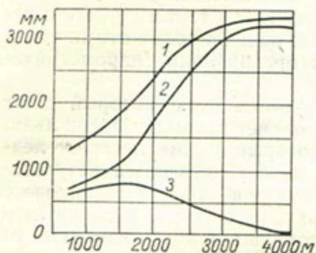
Рис. 39. Зависимость осадков, стока и испарения (ось ординат) от высоты водосбора (ось абсцисс) рек бассейна Ааре [по В. Шпильману из книги В. Л. Шульца (1963)]. 1 — осадки, 2 — сток, 3 — испарение.
