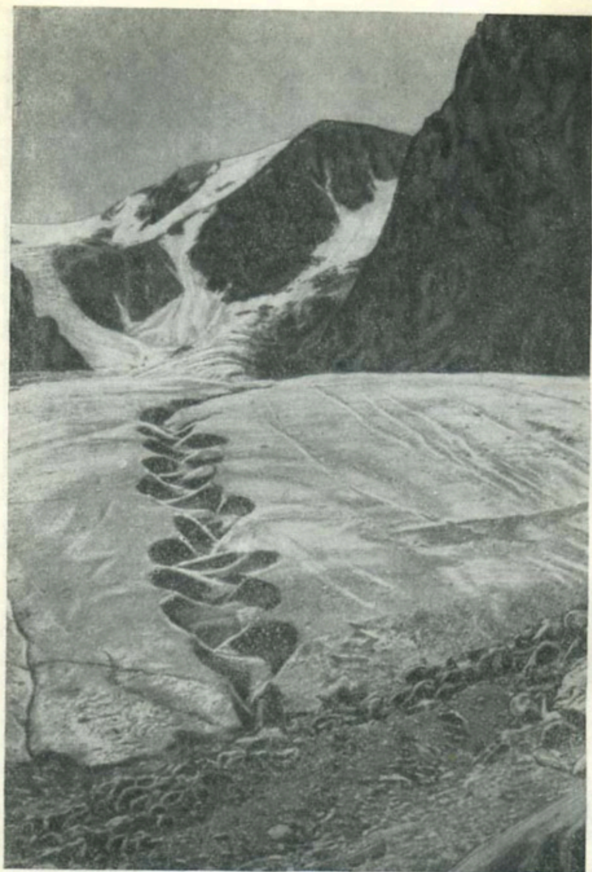
Рис. 80. Открытый конец отступающего ледника.
