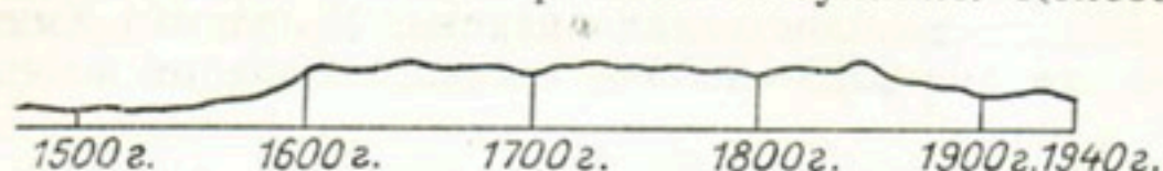
Рис. 73. Схема колебания ледников в Альпах (по Е. Дригальскому и Ф. Махачеку).
