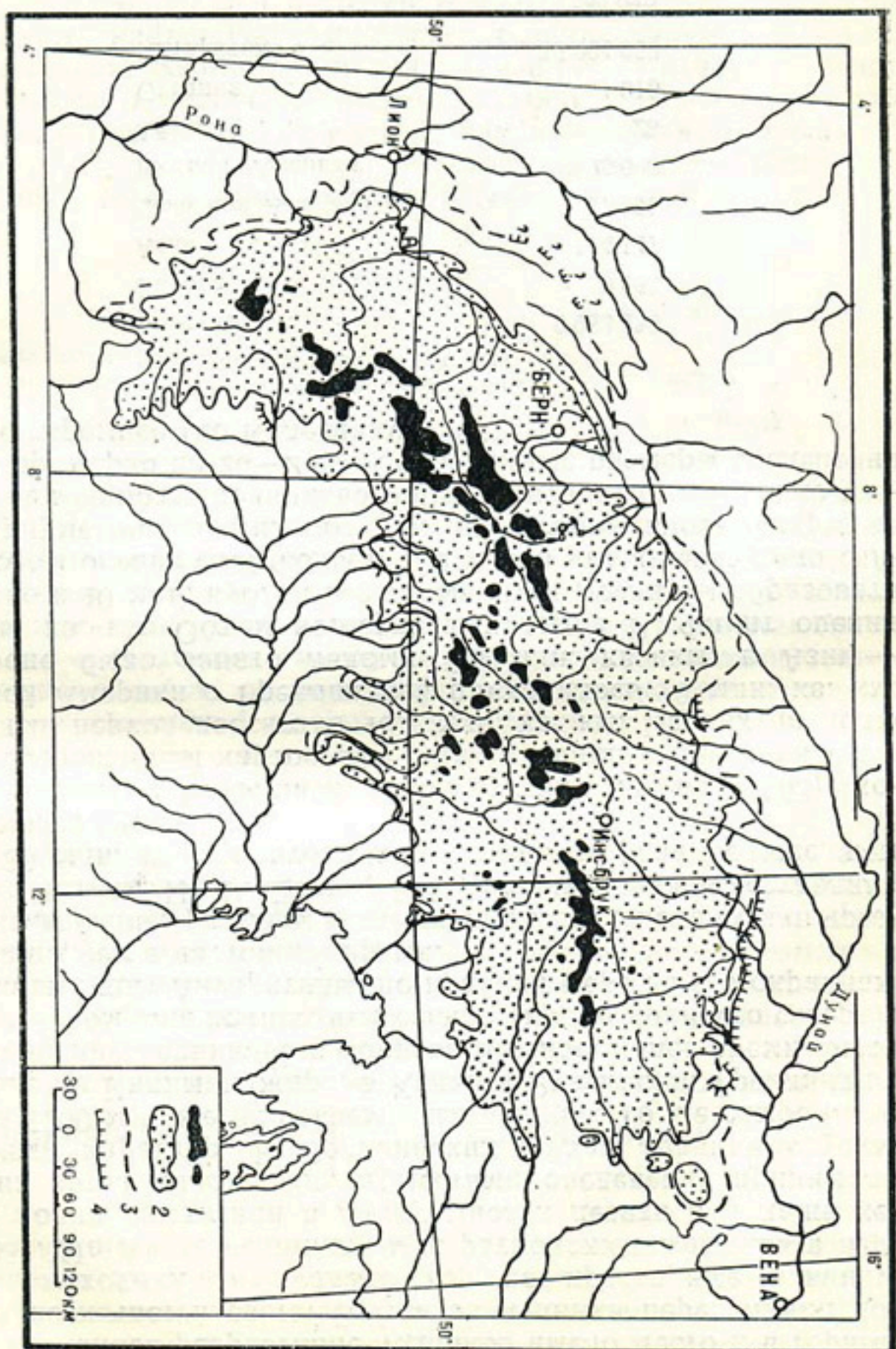
Рис. 85. Плейстоценовое оледенение Альп (по И. С. Жукину).
