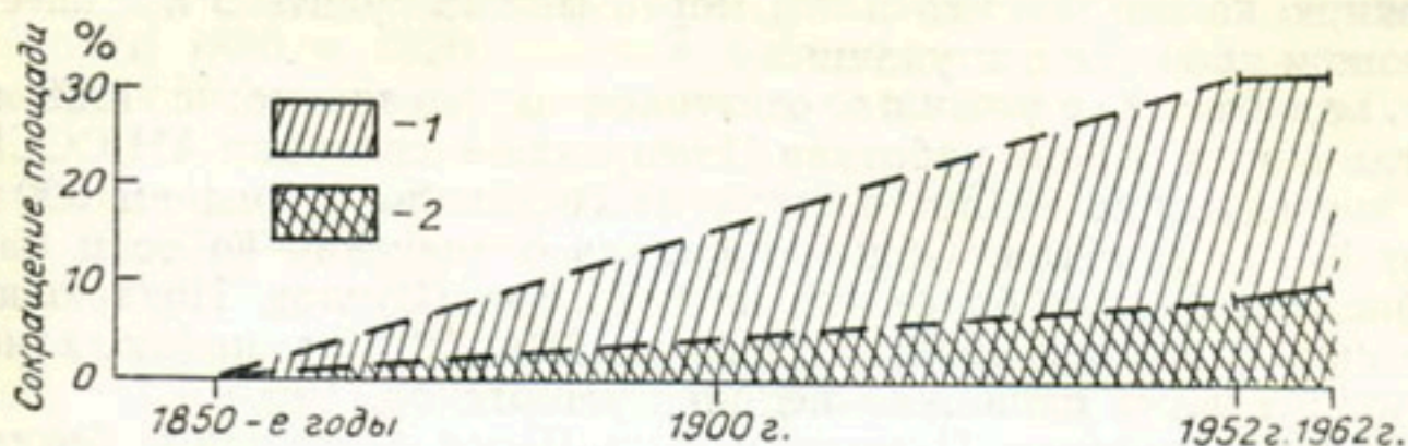
Рис. 71. Темпы сокращения разнотипных ледников на Алтае (по П. А. Окишеву). 1 — малые формы оледенения, 2 — долинные ледники.
