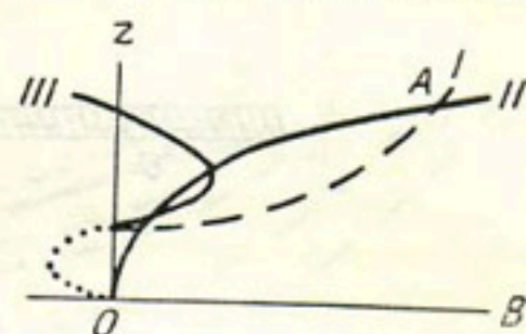
Рис. 112. Построение балансовой кривой (III) при помощи кривых накопления (I) и растекания (II).
