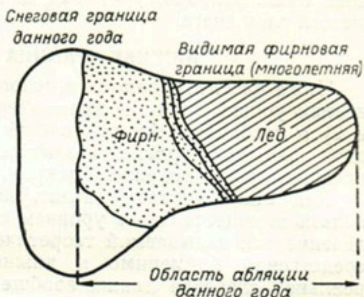
Рис. 18. Снеговая граница и фирновая линия (по Л. С. Троицкому).
