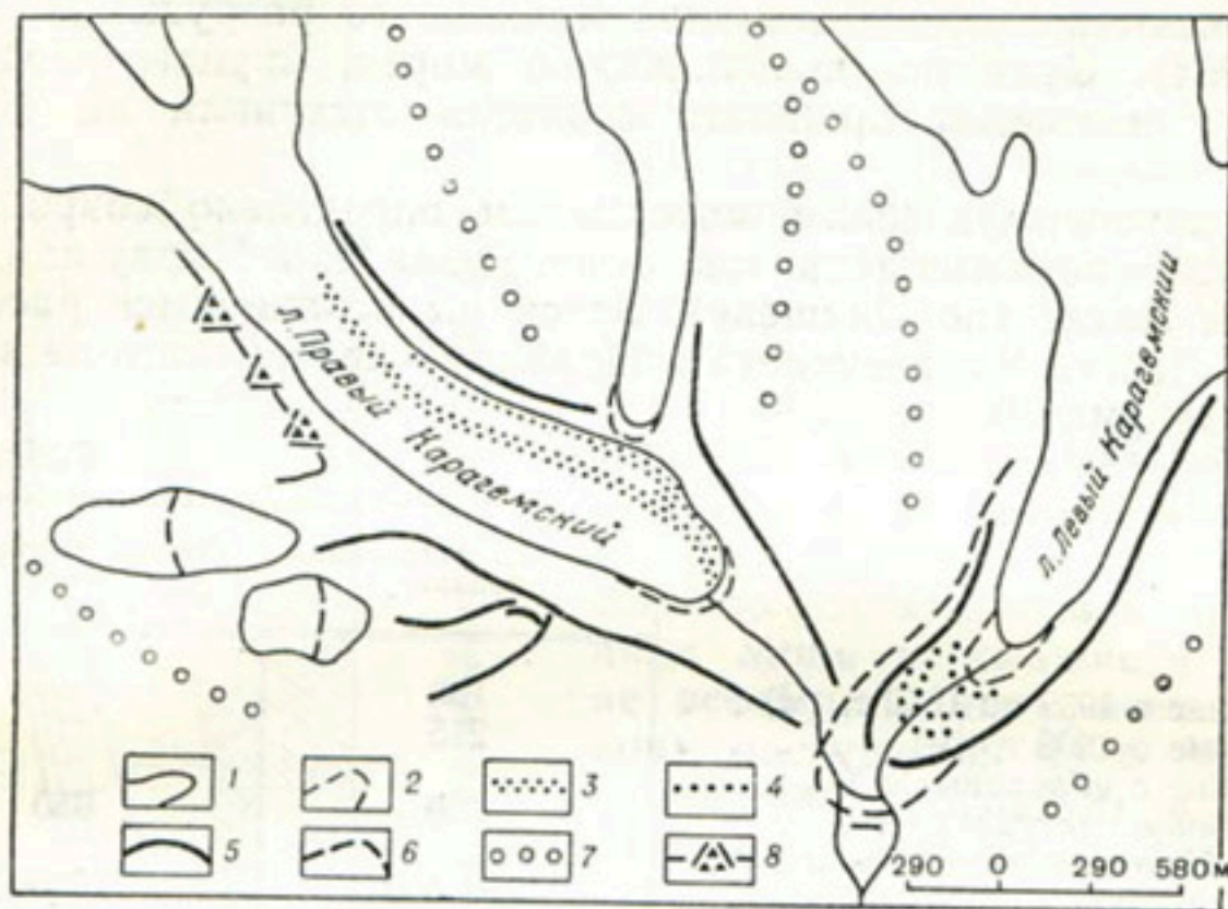
Рис. 70. Схема отступления Левого Карагемского и Правого Карагемского ледников (по П. А. Окишеву).
