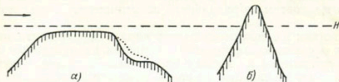
Рис. 23. Нарушение нормальной границы оледенения ( H ) под влиянием особенностей рельефа.
