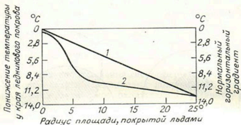
Рис. 110. Понижение температуры у края ледникового покрова.
