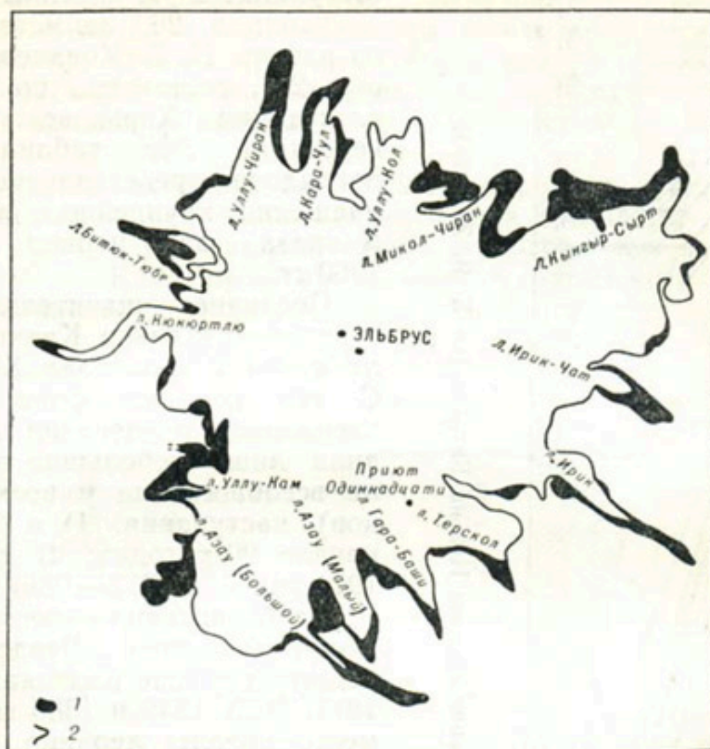
Рис. 68. Оледенение Эльбруса в 1887 и 1957 гг. (по Г. К. Тушинскому).
