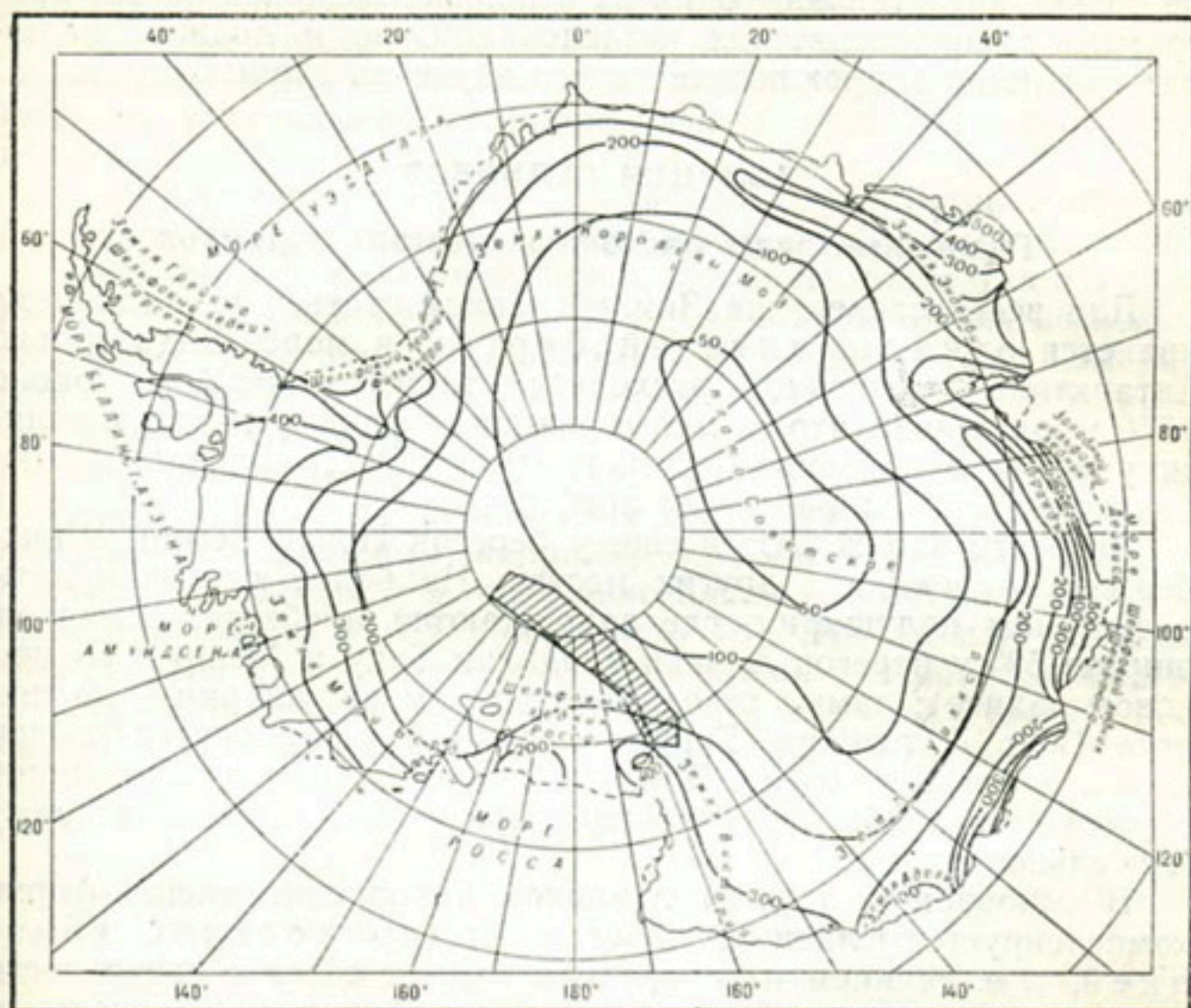
Рис. 55. Карта интенсивности питания ледникового покрова (мм слоя воды) Антарктиды (по В. М. Котлякову).
