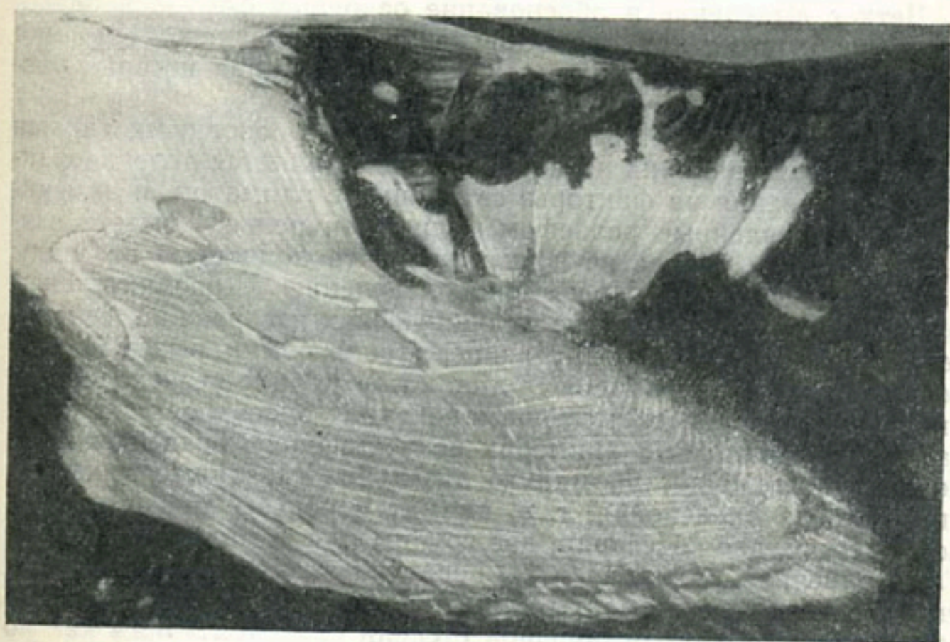
Рис. 4. Навеянный ледник под невысоким плоским водоразделом в Восточном Саяне. Фото Г. М. Томилова.
