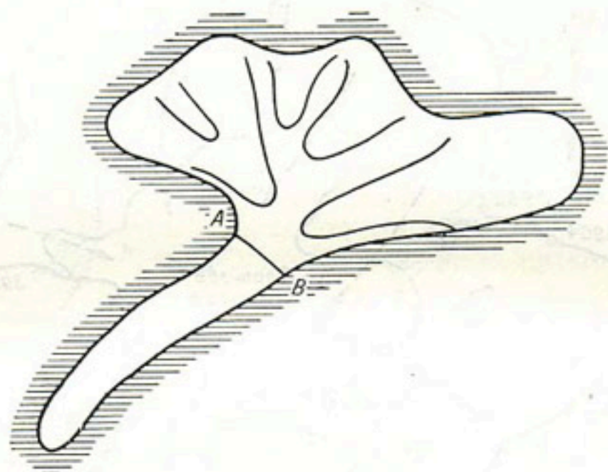
Рис. 92. Бассейн и профиль подпруживания ледника.
