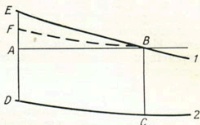
Рис. 84. Схема, поясняющая приток льда сверху к поперечному профилю ледника.
