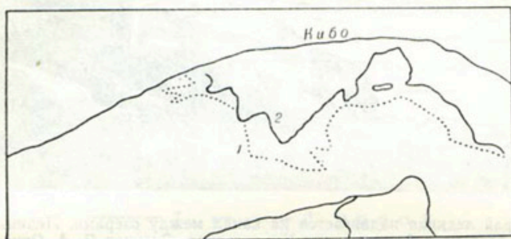
Рис. 79. Вид на вершину Кибо с западо-северо-запада (по Ф. Егеру).
