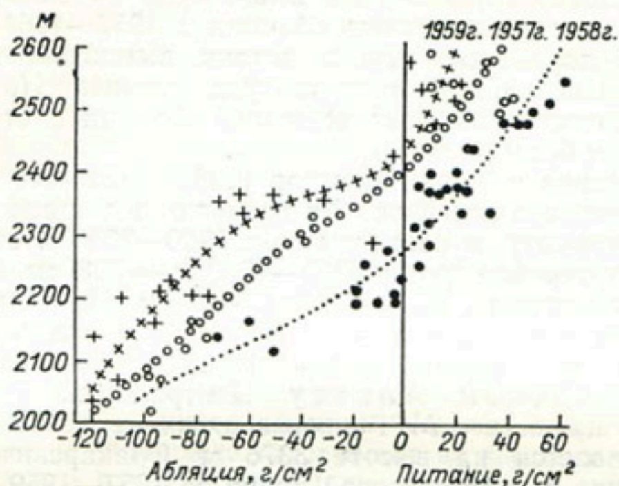
Рис. 56. Кривые питания и абляции на леднике № 31 в 1957—1959 гг. (по М. М. Корейша).
