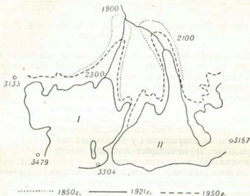
Рис. 75. Ледники Ваксекеес (I) и Горнкеес (II) в Циллертальских Альпах (по Г. Кинцлю).
