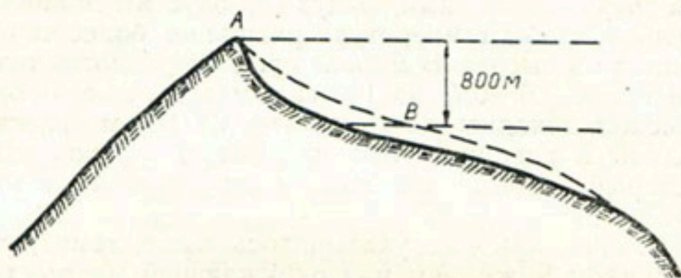
Рис. 8. Соотношение между опусканием снеговой линии ниже гребня хребта (800 м) и встречным поднятием поверхности ледника (200 м).
