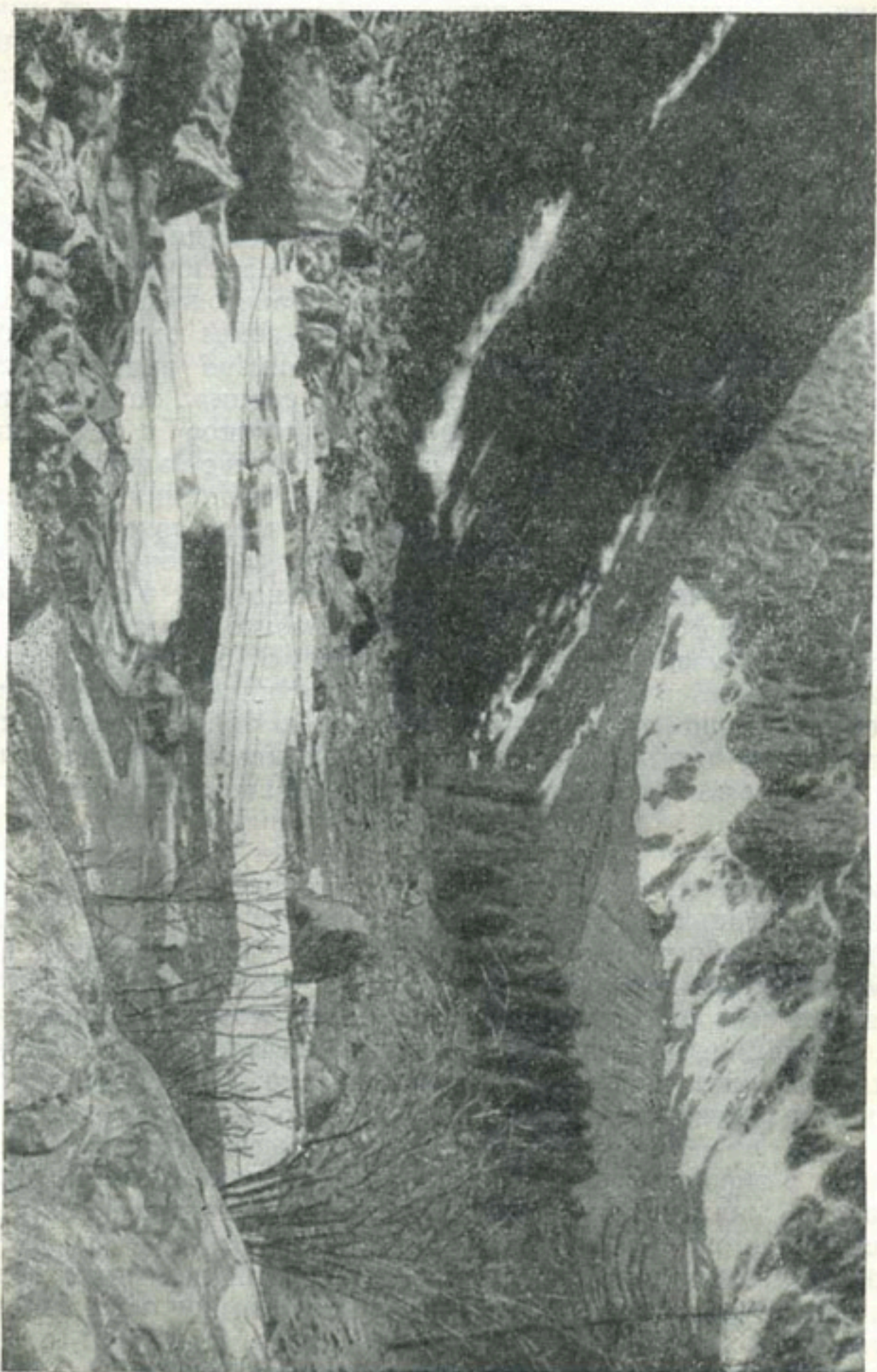
Рис. 65. Наледь близ ледника Малый Актру на Алтае. фото Н. И. Иванова.
