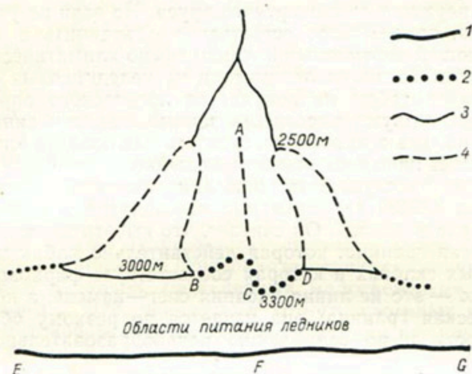
Рис. 15. Снеговая линия первого и второго рода.
