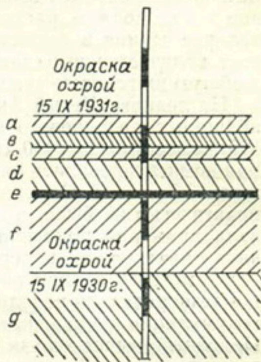
Рис. 38. Разрез поверхностных слоев в фирновой области (2700 м) на леднике Клариденфирн (по Р. Штрейф-Беккеру).
