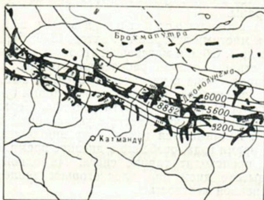
Рис. 33. Снеговая граница в Гималаях (по Г. Виссману).
