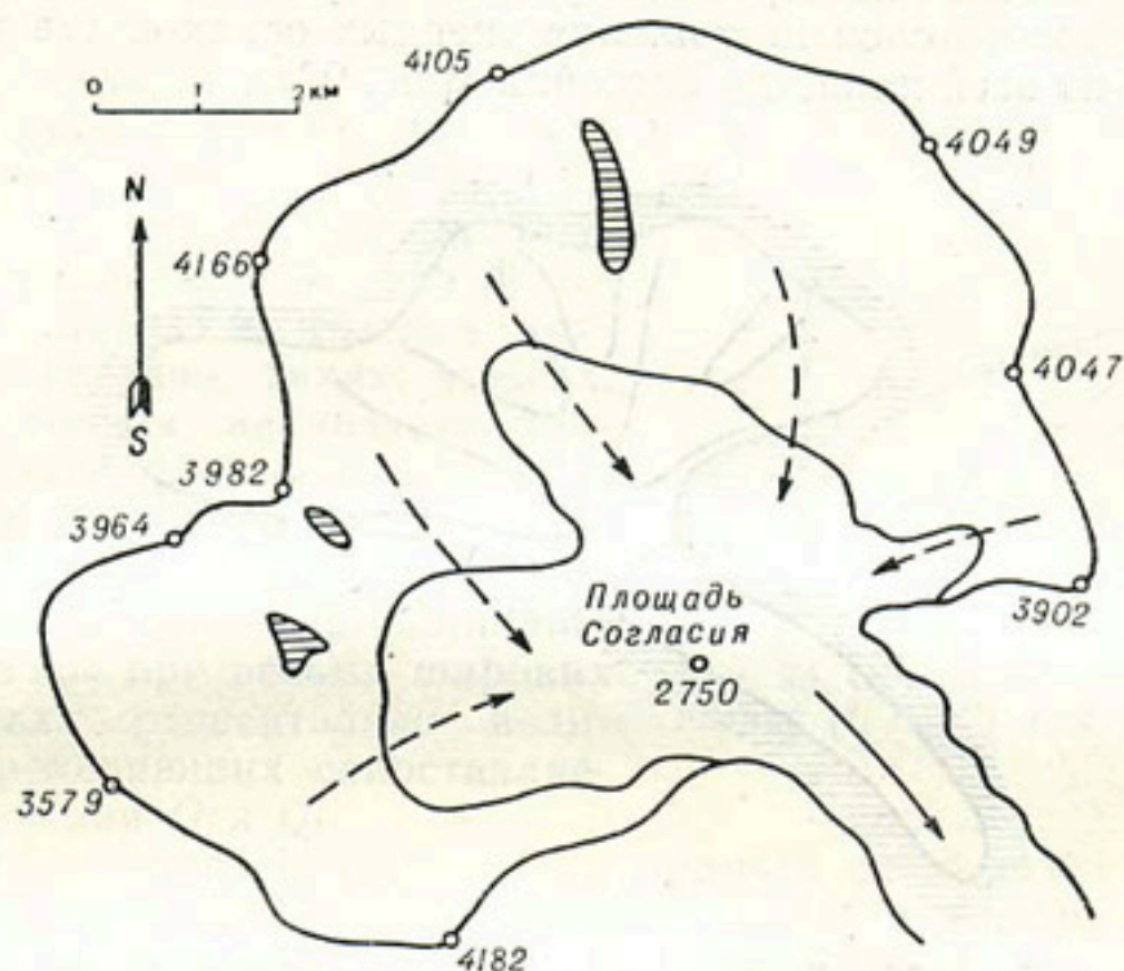
Рис. 91. Фирновая область Алецкого ледника (по Р. Штрейф-Беккеру).
