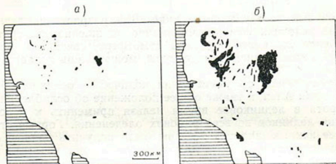
Рис. 88. Современные озера (а) и озера ледниковой плювиальной эпохи (б) в Большом бассейне США (по Мейнцеру и Флинту).
