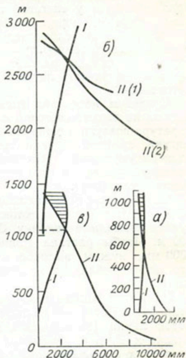
Рис. 67. Кривые аккумуляции (I) и абляции (II) для случаев большей или меньшей энергии оледенения (по П. А. Шумскому).
