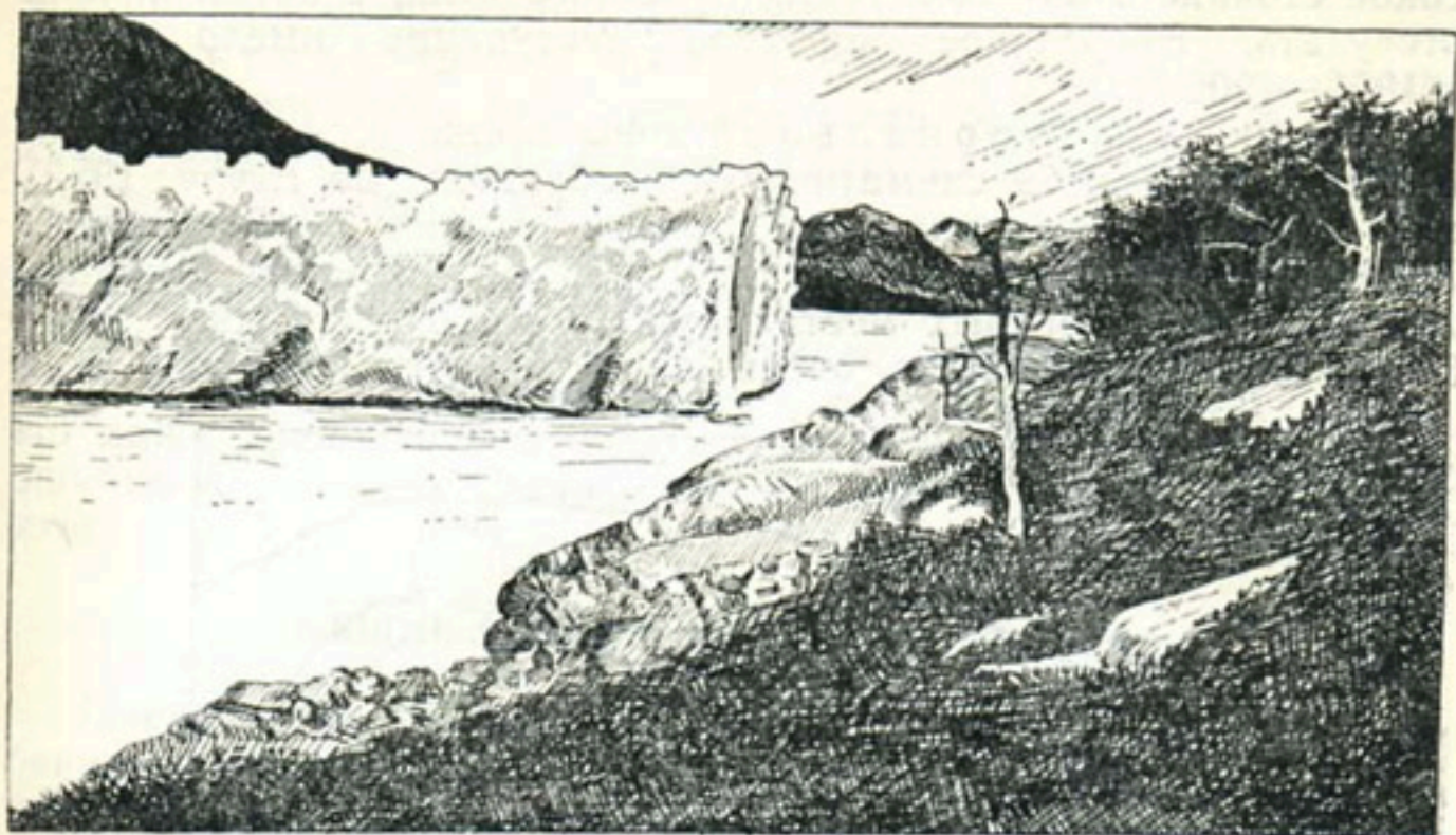
Рис. 77. Край ледника надвигается на канал между озерами. Ледник Вентискверо-Морено в Аргентинских Кордильерах. Рисунок П. А. Окишева.
