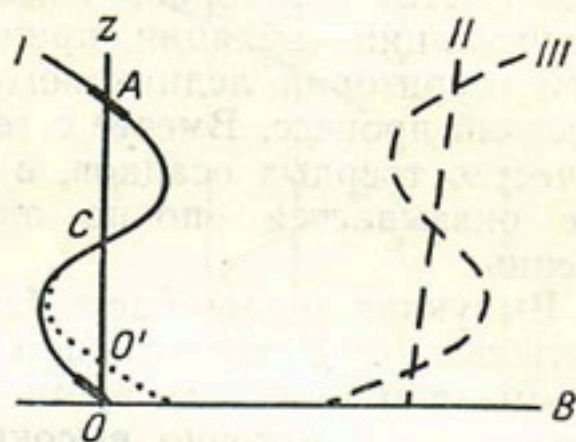
Рис. 107. Балансовые кривые сложной формы.
