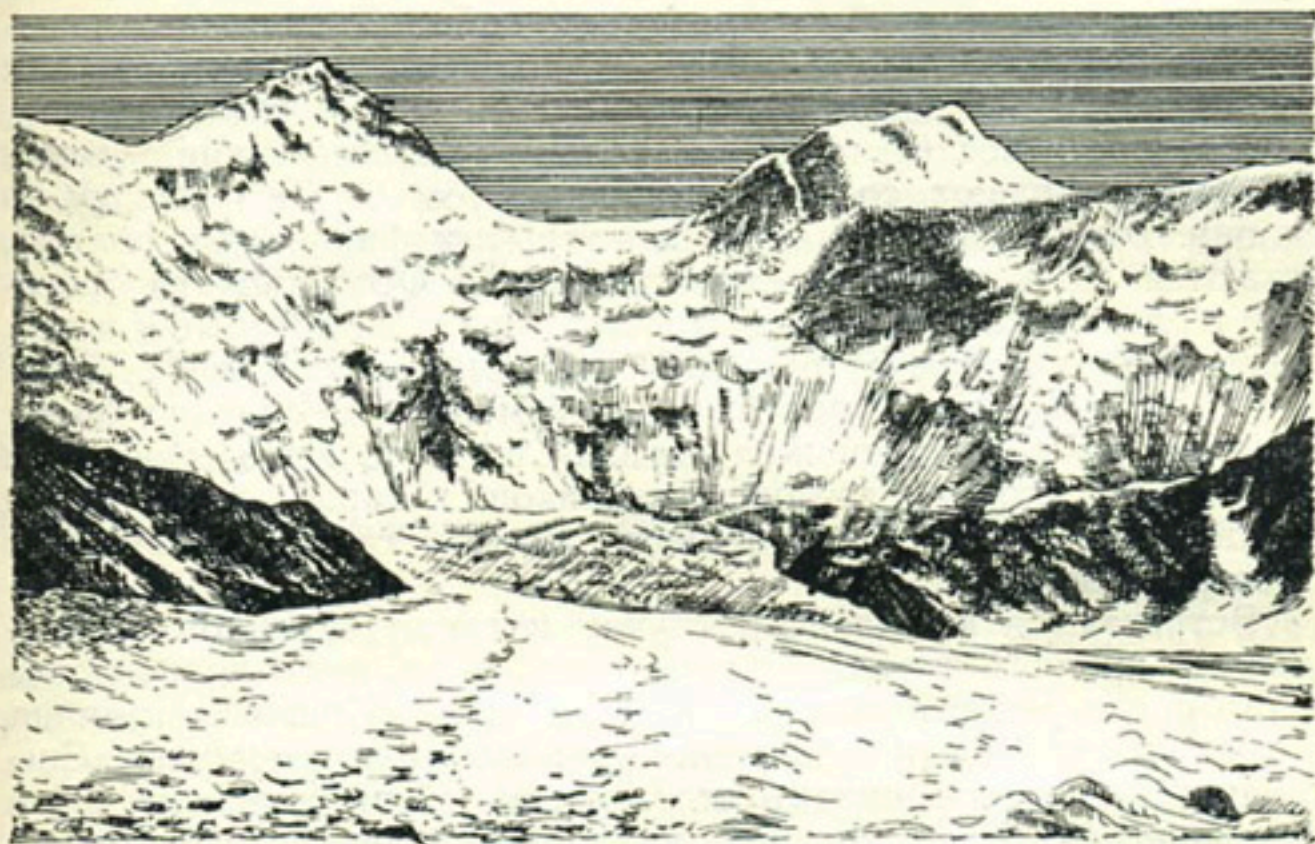
Рис. 45. Северная стена Белухи на Алтае. Рисунок П. А. Окишева.
