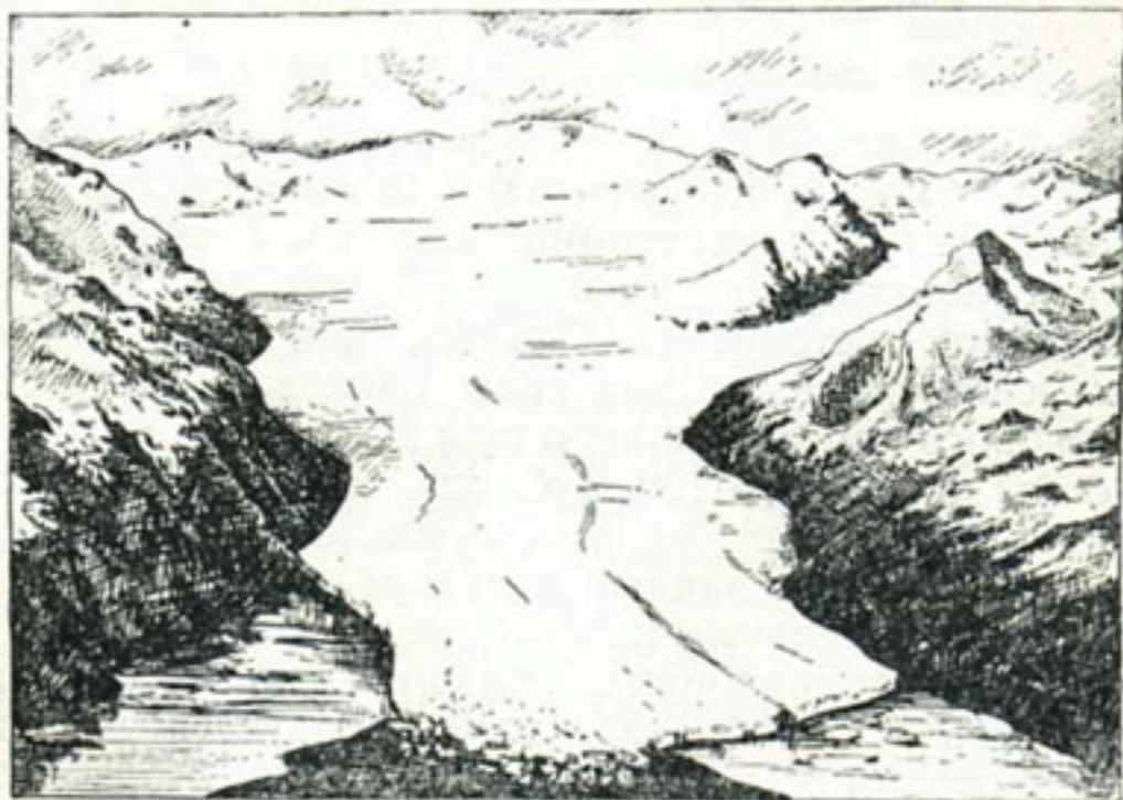
Рис. 78. Наступающий ледник перегородил канал между двумя озерами. Ледник Вентискверо-Морено в Аргентинских Кордильерах. Рисунок П. А. Окишева.
