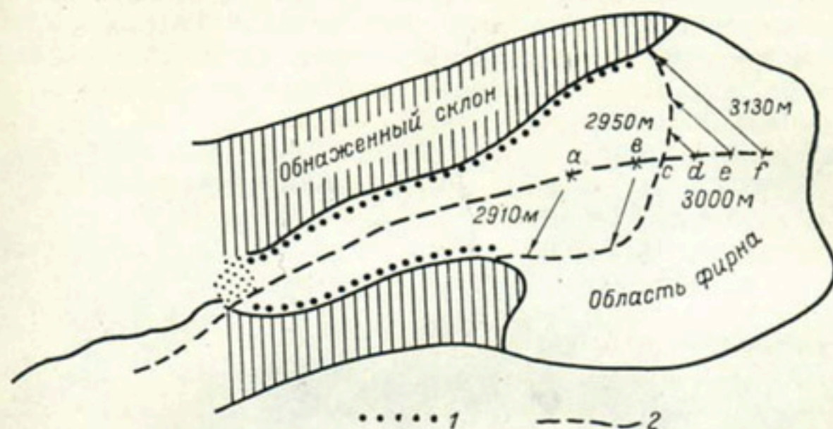
Рис. 24. Схема маршрутного определения высоты снеговой линии.
