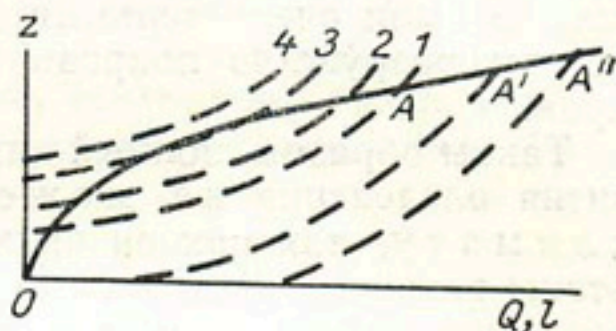
Рис. 114. Изображение цикла развития оледенения при помощи перемещения кривой накопления.
