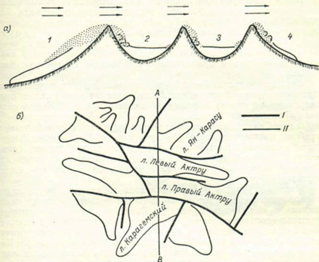
Рис. 44. Распределение аккумуляции снега на наветренных и подветренных склонах гребней в горном узле Биш-Иирду на Алтае.
