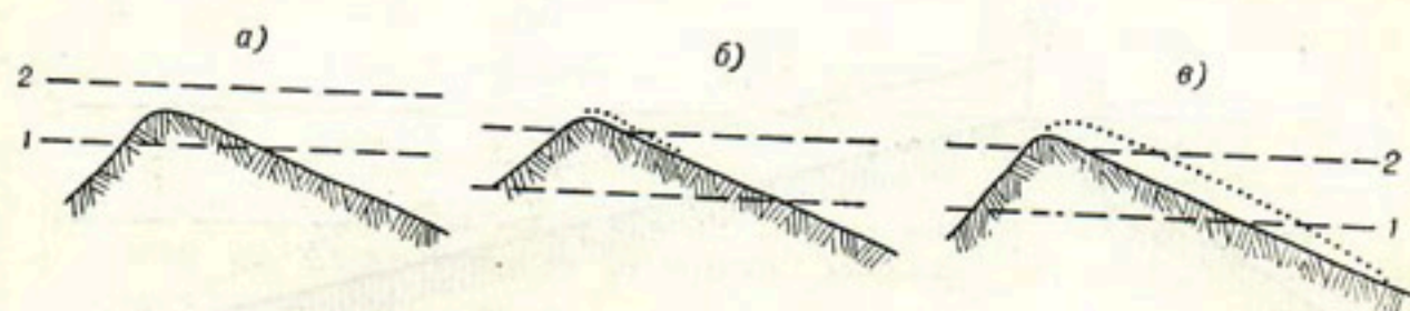
Рис. 95. Схема зарождения ледника. 1—1 и 2—2 — первый и второй уровни хионосферы соответственно.
