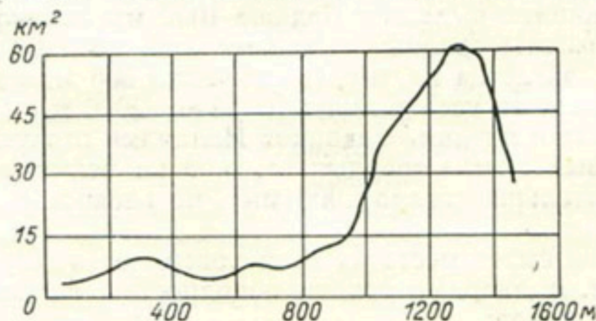
Рис. 48. Кривая распределения площади ледника Хоффельсйокуль по высотным поясам (по Г. Альману).
