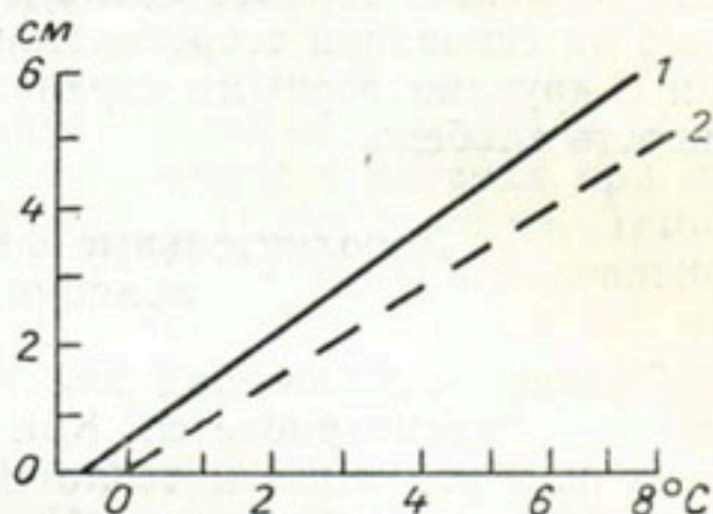
Рис. 66. Среднее суточное стаивание льда (1) и снега (2) с поверхности Туяксуйских ледников в связи со средней суточной температурой воздуха. По данным 1937—1942 гг. (по Н. Н. Пальгову).
