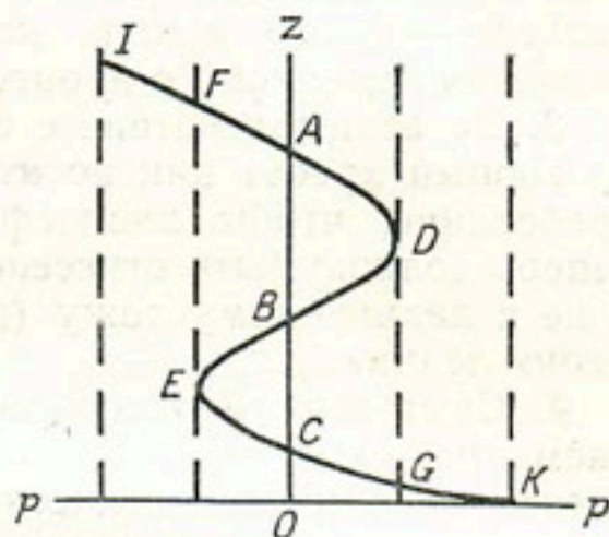
Рис. 108. Построение сложной балансовой кривой в случае изменения климата.
