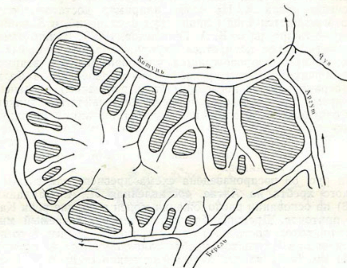
Рис. 86. Схема Катунского ледника в период максимальной фазы последнего оледенения (по Л. А. Варданянцу).
