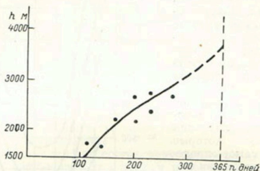
Рис. 28. Схема построения кривой зависимости n от h .
