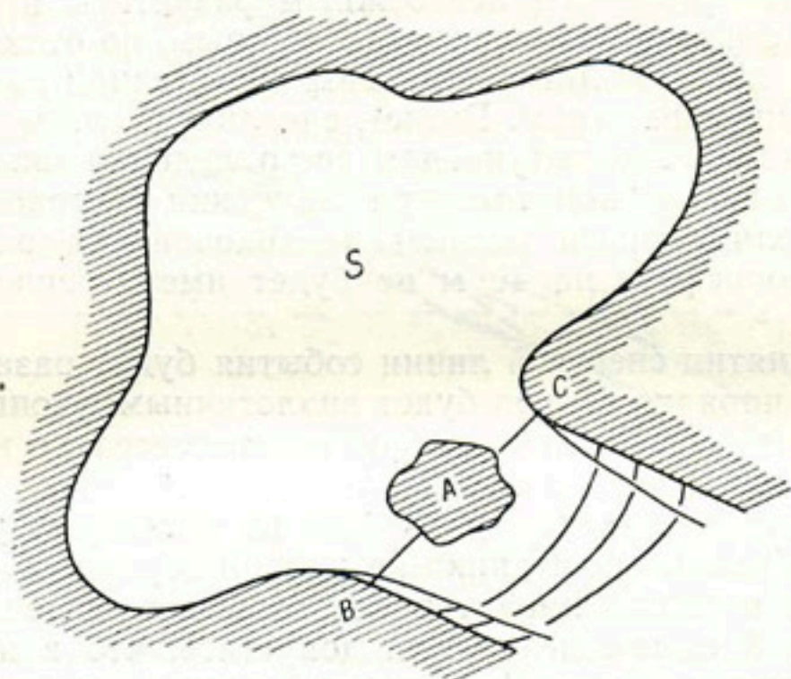
Рис. 90. Один из видов подпруживания ледника.
