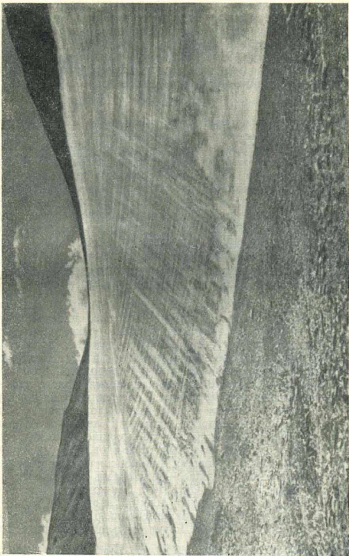
Рис. 101. Присклоновый ледник, устойчивый благодаря залеганию на уровне снеговой границы.
