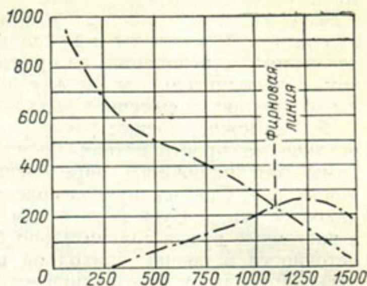
Рис. 49. Средние значения суммарной аккумуляции и абляции на леднике Хоффельсйокуль за период 1935—1938 гг. (по Г. Альману).
