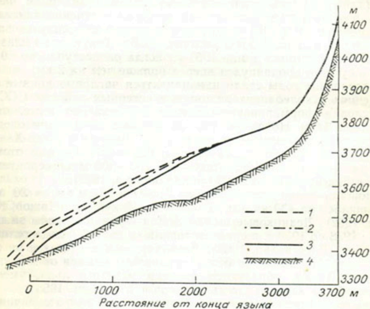
Рис. 72. Продольный разрез и уровень поверхности Центрального Туюксуйского ледника (по К. Г. Макаревичу). 1 — уровень поверхности в 1923 г., 2 — в 1937 г., 3 — в 1957 г., 4 — ложе ледника.
