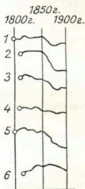
Рис. 74. Колебания некоторых ледников в Альпах (по Маурери).
