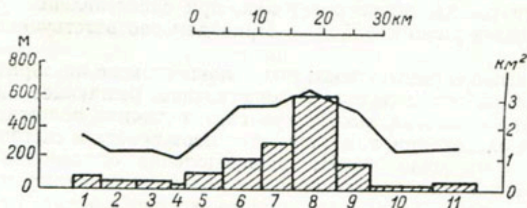
Рис. 6. Диаграмма распределения оледенения вдоль Южно-Алтайского хребта.
