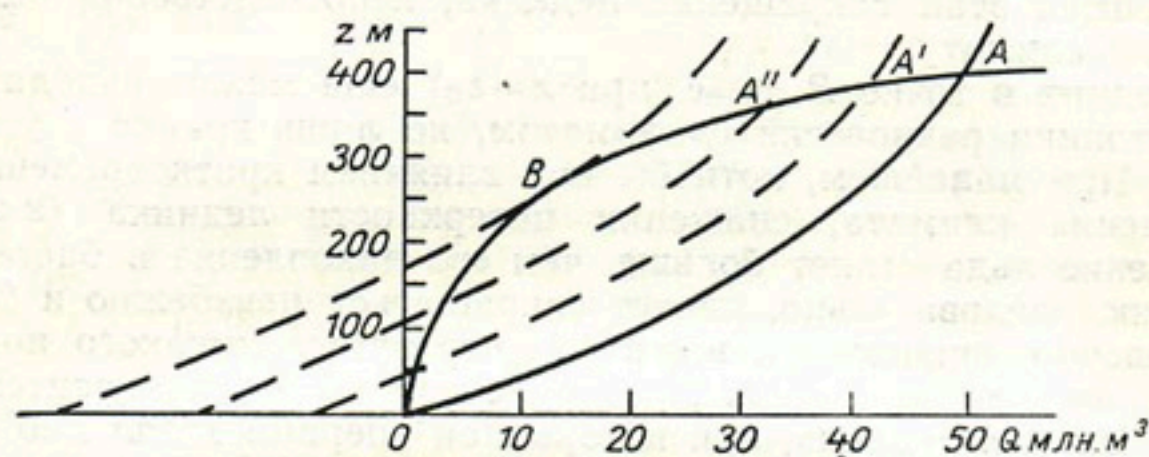
Рис. 94. Механизм разрушения подпруженного ледника при поднятии снеговой линии до критического уровня.
