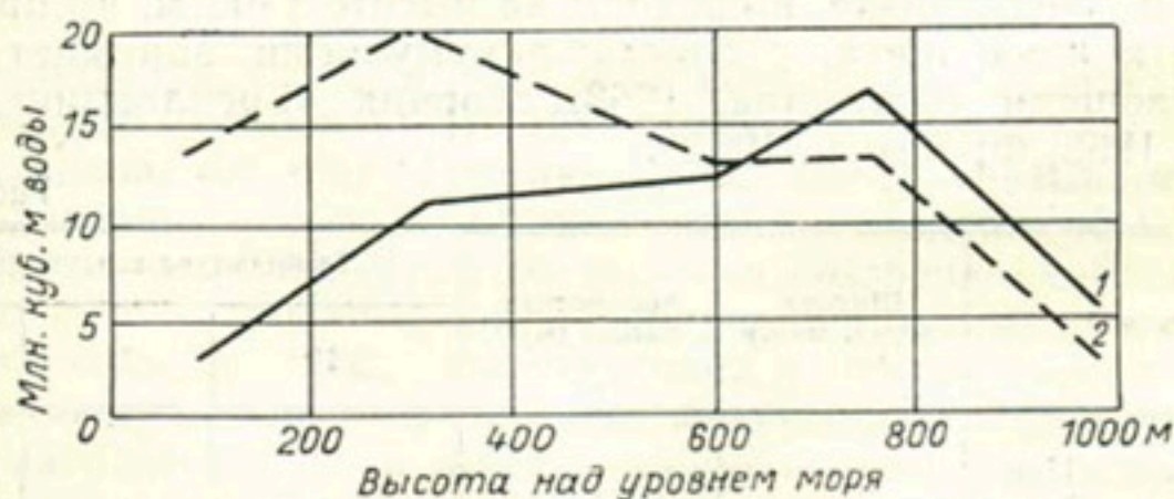
Рис. 50. Балансовая диаграмма ледника 14-го июля на Шпицбергене за 1933-34 «бюджетный» год (по Г. Альману).
