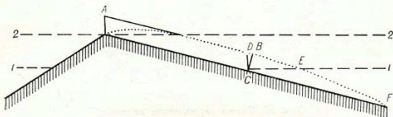
Рис. 96. Схема зарождения ледника и образования снеговой линии после касания гребня вторым уровнем хионосферы.
