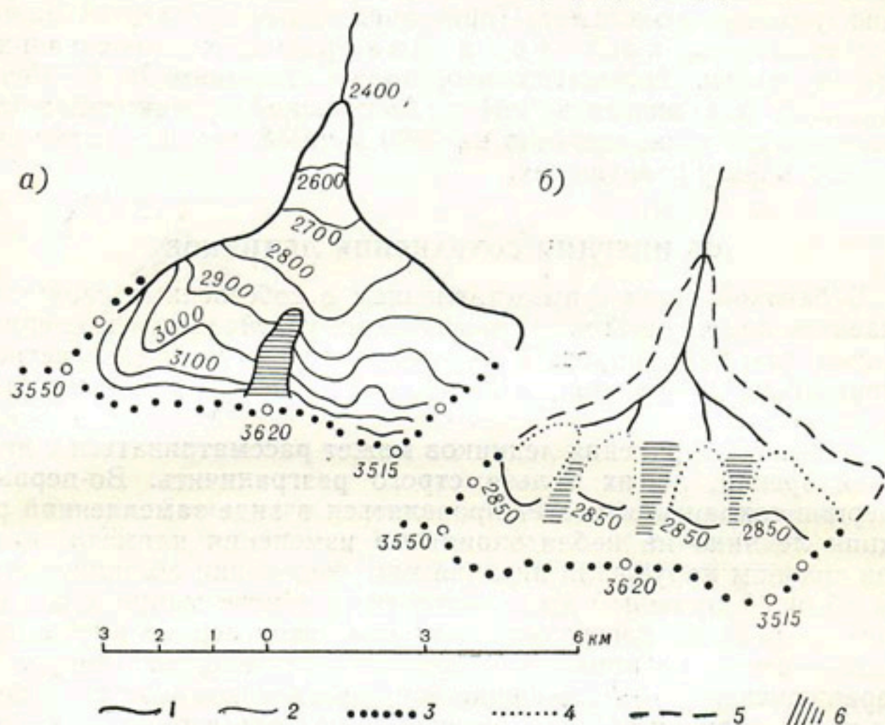
Рис. 97. Схематический план Алахинского ледника.
