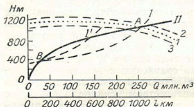
Рис. III. Кривые накопления ( I и I' ) и растекания ( II ).
