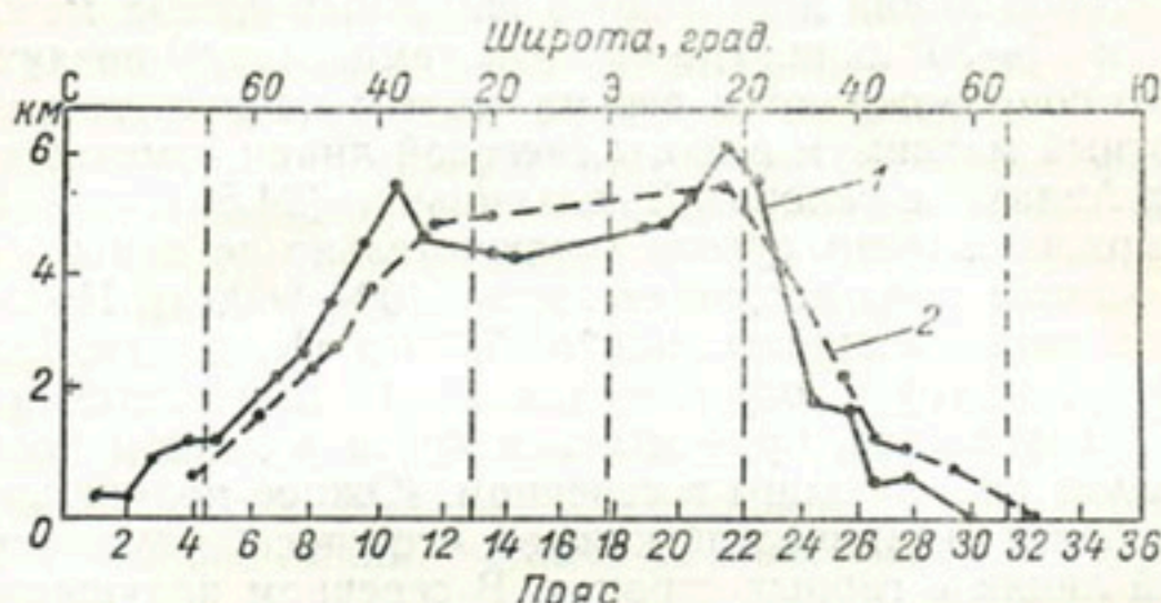
Рис. 35. Схематическое распределение высоты снеговой линии по широтным поясам Земли (1) и по параллелям (2) (по С. В. Калеснику).
