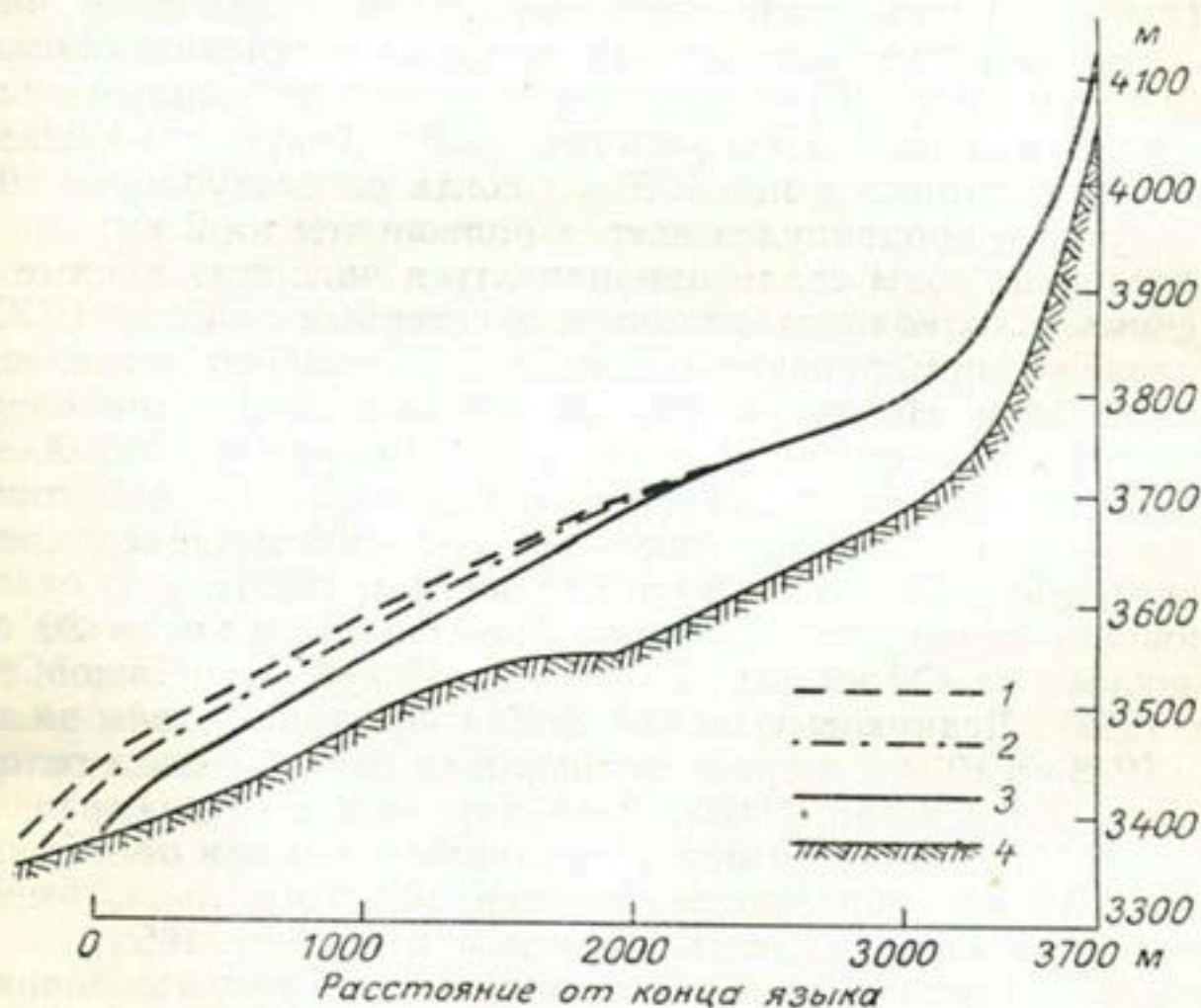
Рис. 72. Продольный разрез и уровень поверхности Центрального Туюксуйского ледника (по К. Г. Макаревичу). 1 — уровень поверхности в 1923 г., 2 — в 1937 г., 3 — в 1957 г., 4 — ложе ледника.
