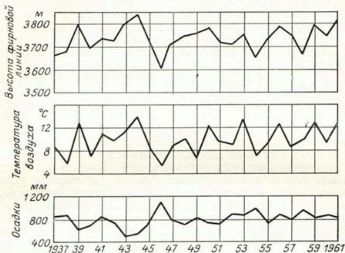
Рис. 82. Ход основных метеорологических элементов и высоты фирновой линии на Центральном Туяксайском леднике (по Н. Н. Пальгову).
