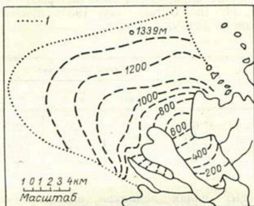
Рис. 47. Ледник Хоффельсйокуль в 1937 г. (по Г. Альману). 1 — граница ледника.
