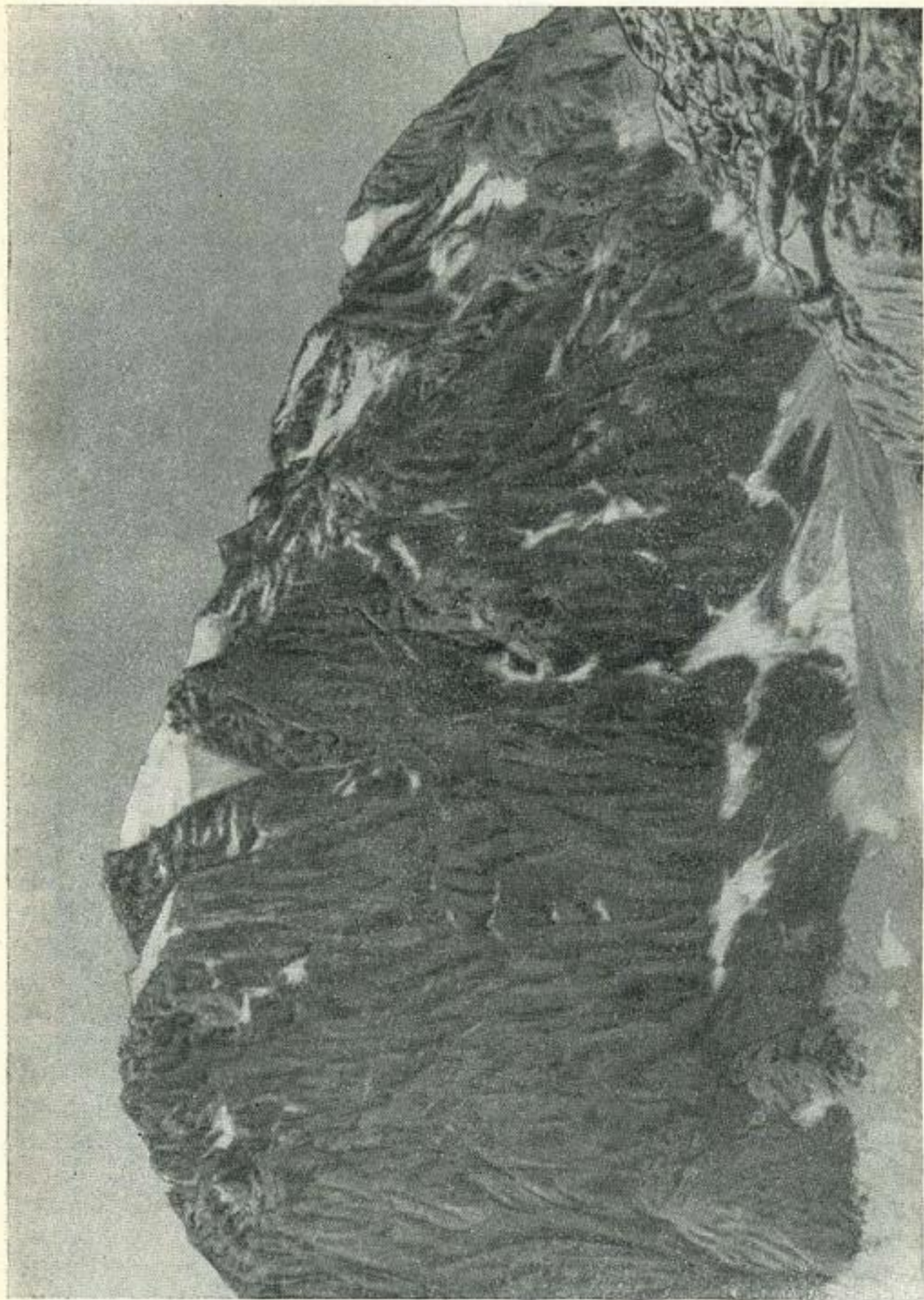
Рис. 100. Высоко расположенный малый ледник, сбрасывающий вниз избыток фирна.
