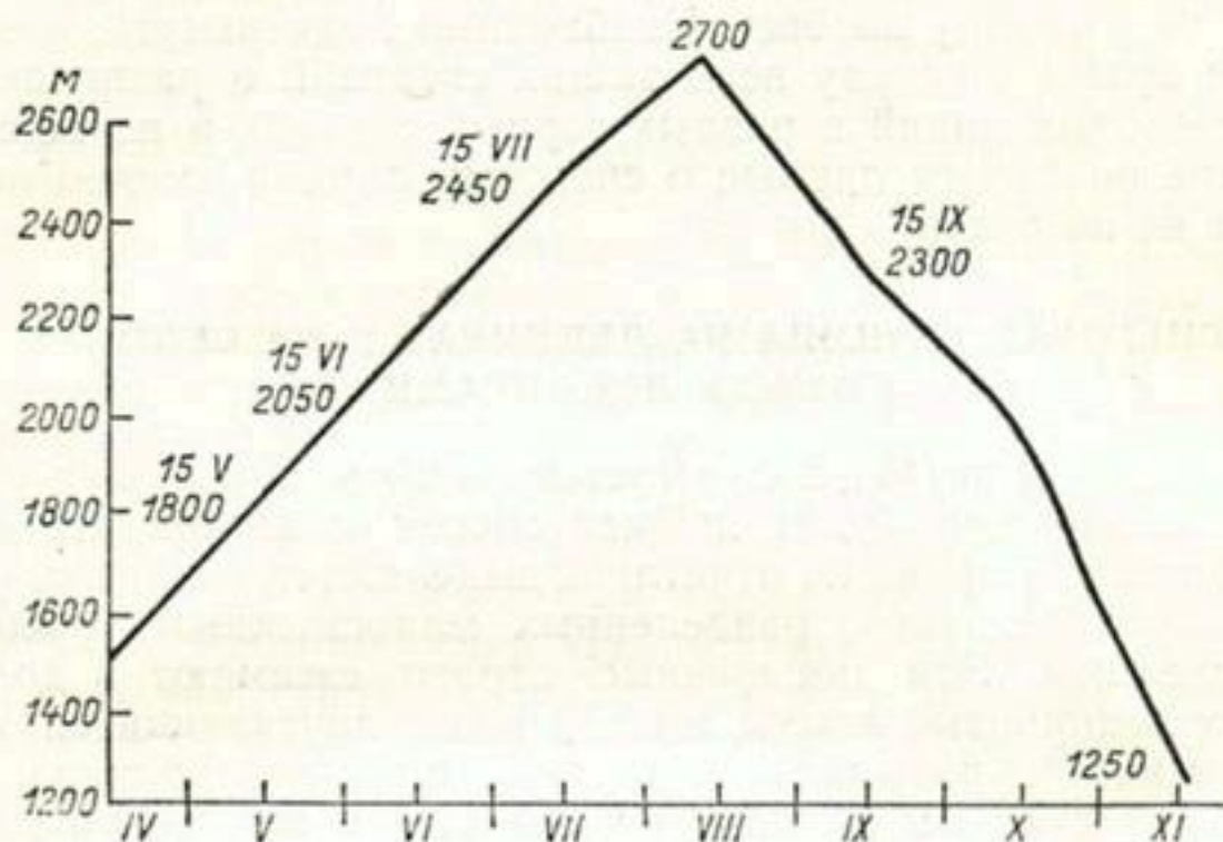
Рис. 14. Сезонное изменение высоты снеговой линии для области Зонблика (по Мареку).
