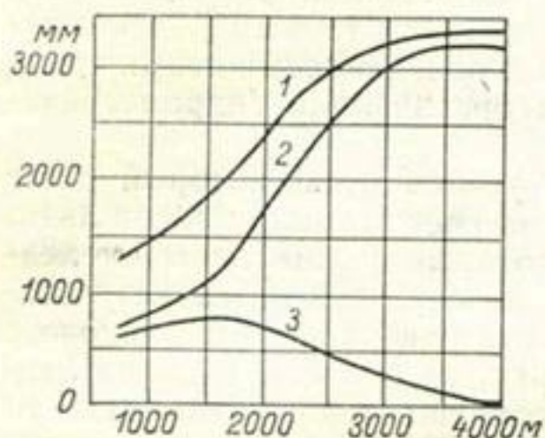
Рис. 39. Зависимость осадков, стока и испарения (ось ординат) от высоты водосбора (ось абсцисс) рек бассейна Ааре [по В. Шпильману из книги В. Л. Шульца (1963)].
