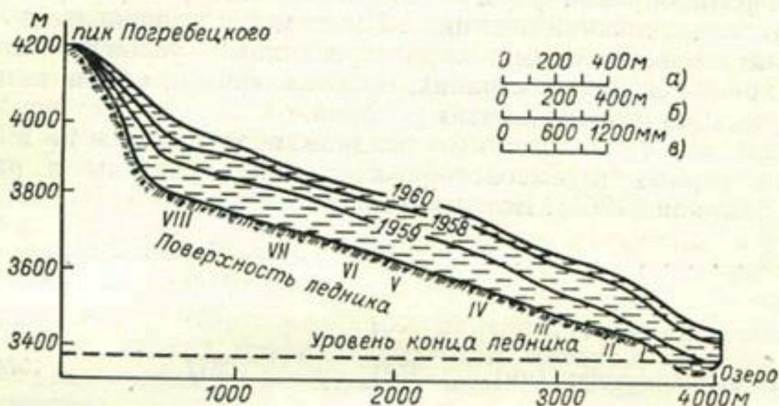
Рис. 46. Распределение запасов воды в снежном покрове на Центральном Туюксуйском леднике (по П. А. Судакову и Е. Н. Вилесову).
