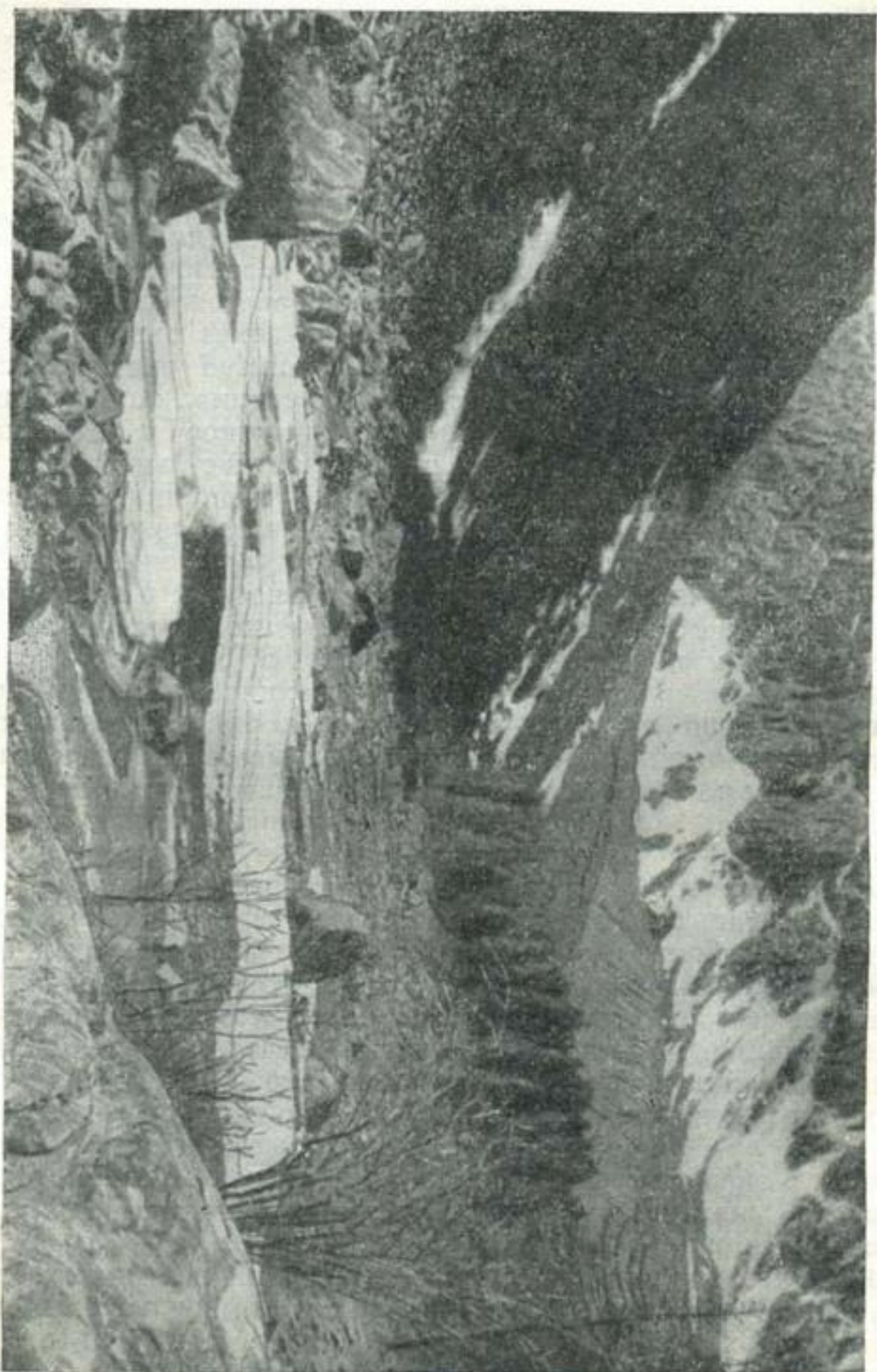
Рис. 65. Нагель близ ледника Малый Актуру на Алтае, фото Н. И. Иванова.
