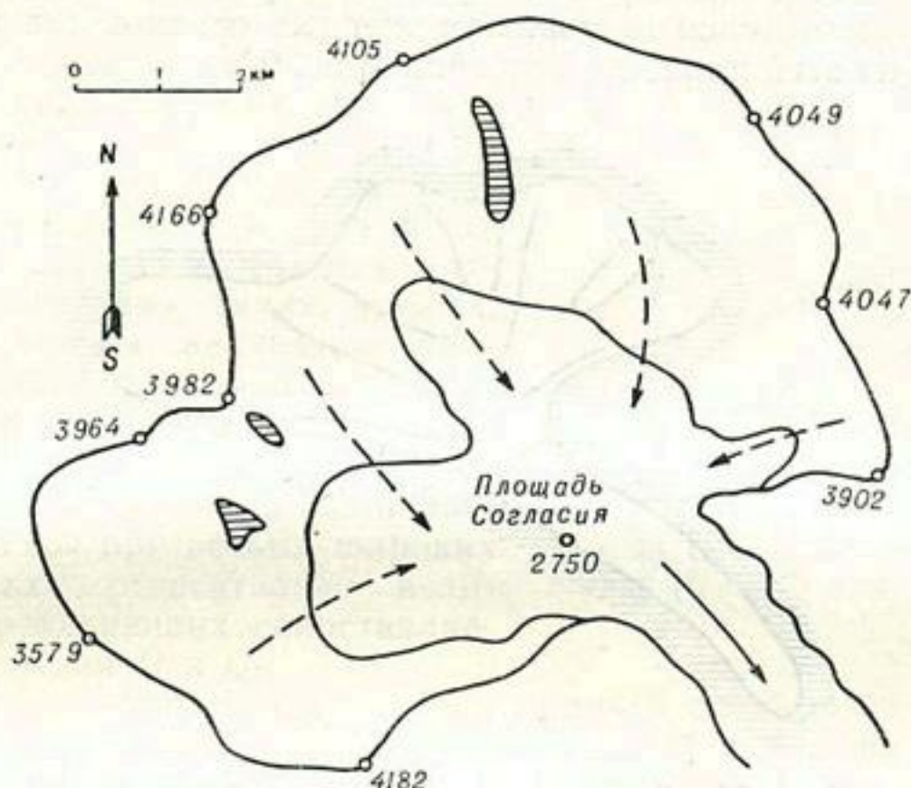
Рис. 91. Фирновая область Алевского ледника (по Р. Штрейф-Беккеру).
