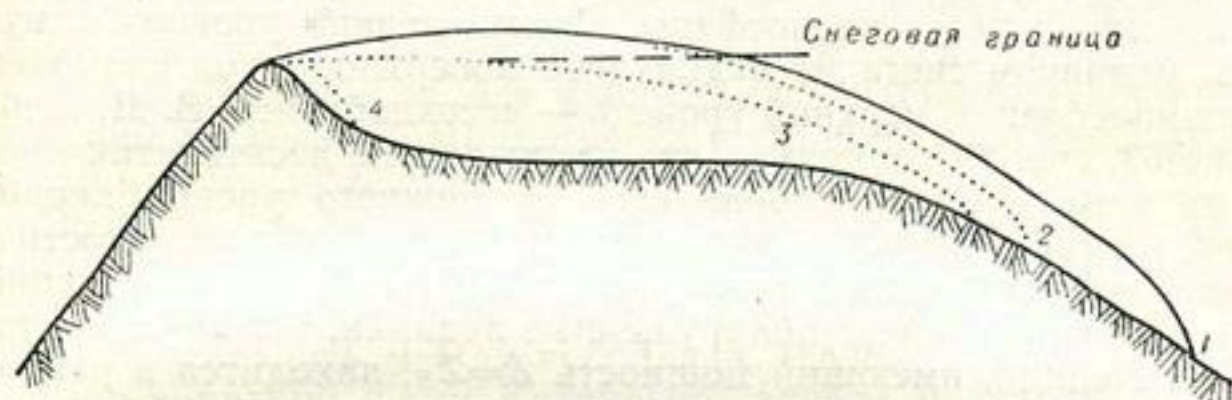
Рис. 98. Схема, иллюстрирующая значение инерции сохранения ледников, залегающих на плоских ступенях и водоразделах.
