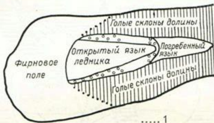
Рис. 17. Структура типичного ледника и его бассейна в центральном районе оледенения Заилийского Алатау (по Н. Н. Пальгову). 1 — снеговая линия второго рода.
