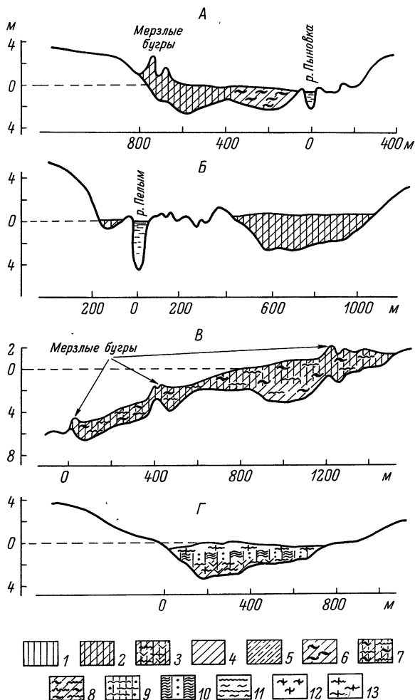
Рис. 1. Геоморфологические условия залегания болот на междуречье Лозьвы и Пельмы.
