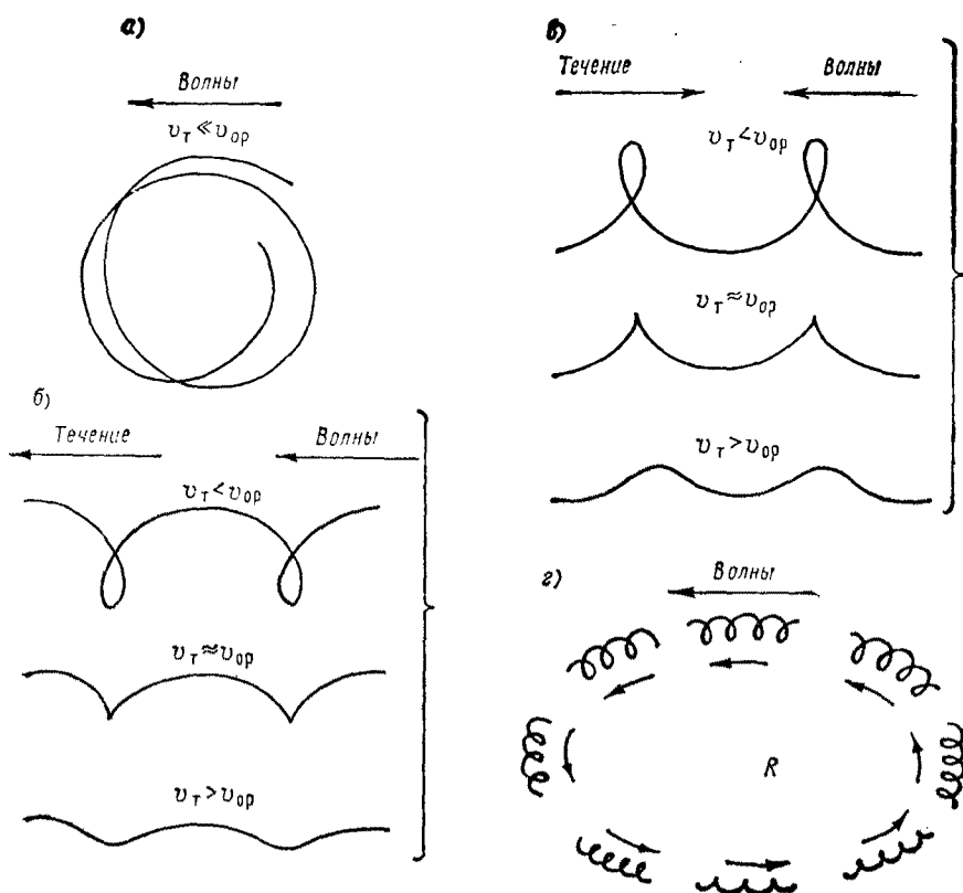
Рис. 2.3. Основные виды траектории частиц жидкости при различных направлениях и соотношениях скорости течения ( v_T ) и скорости орбитального движения ( v_{ор} ).
