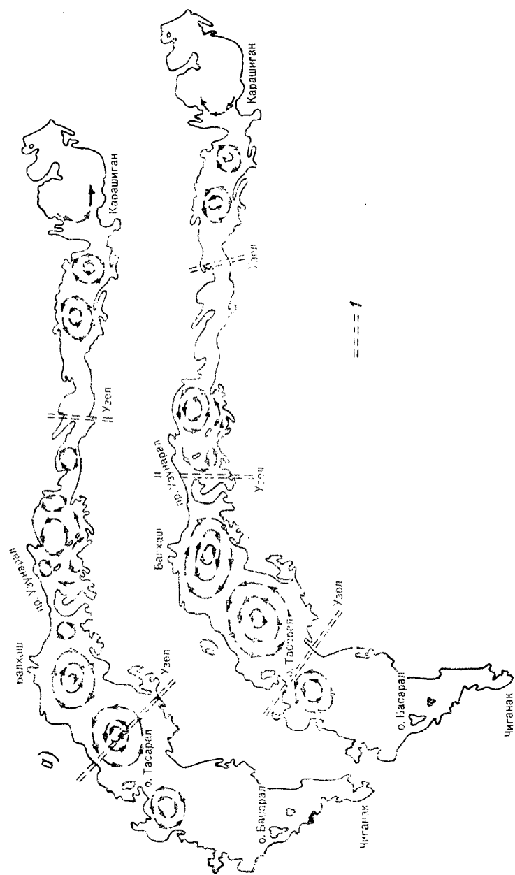
Рис. 2.12. Схемы дискретных крупномасштабных вихрей в оз. Балхаш, сформированные двухузловой (а) и трехузловой (б) сейсмами при однородной плотности воды. I — узловые створы сейш.
