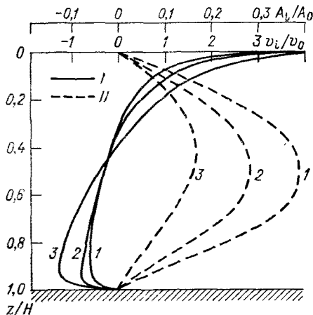
Рис. 4.13. Изменение распределения скорости ветрового течения по вертикали ( v ) при различных законах распределения коэффициентов турбулентной вязкости ( lf ) и температуры воды (по Б. Г. Вагнеру и В. В. Симону).
