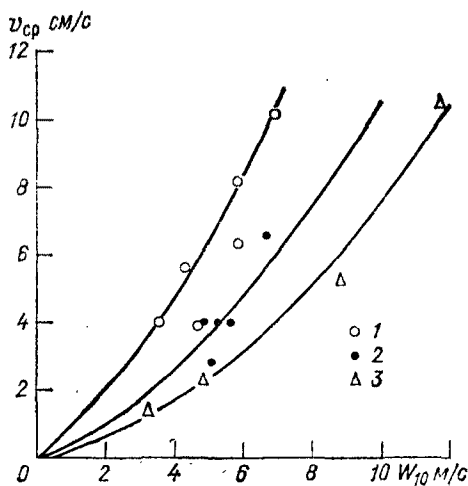
Рис. 6.6. Зависимости средней на вертикали скорости одноподвижного по глубине ветрового течения от скорости ветра при разных глубинах.
