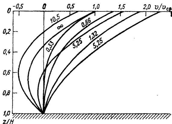
Рис. 4.1. Изменение распределения относительных значений скорости и направления развивающегося ветрового течения в мелководном водоеме [9].
