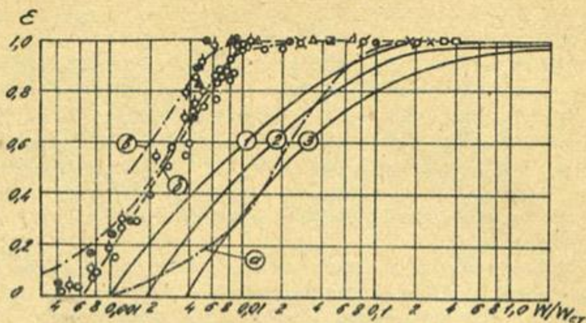
Рис. 3.8. Графики зависимости степени осветления от отношения объема водохранилища W к среднегодовому стоку воды W_{cr} . Кривые Брюне: 1 — крупные наносы; 2 — средние наносы; 3 — мелкие наносы.
