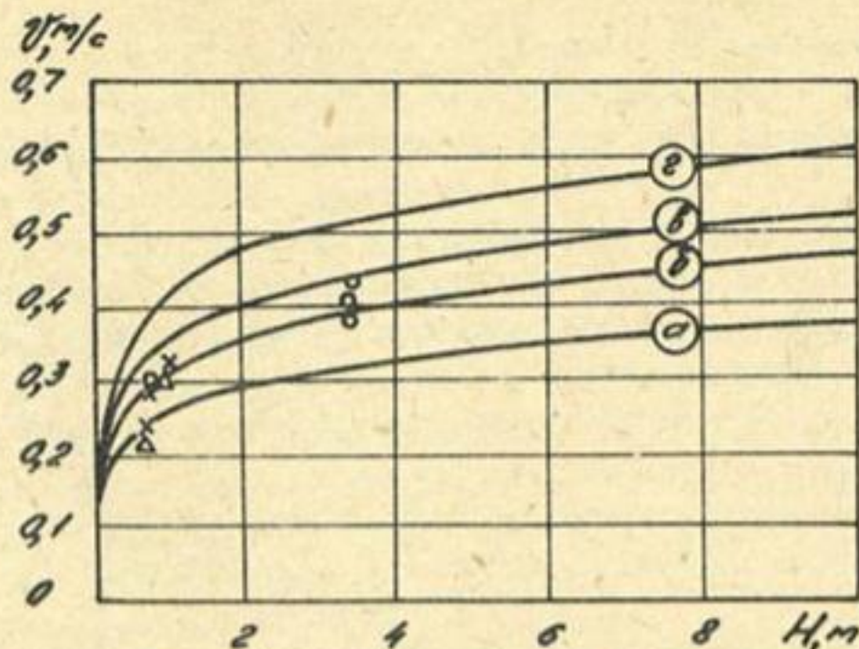
Рис. II.6. График сопоставления расчетной неразмывающей скорости с данными натурных исследований САНИИРИ на каналах: X – Кызылкумский, 1978 г.; \Delta – Шават, 1979 г.; O – Кызылкумский 1979 г.
