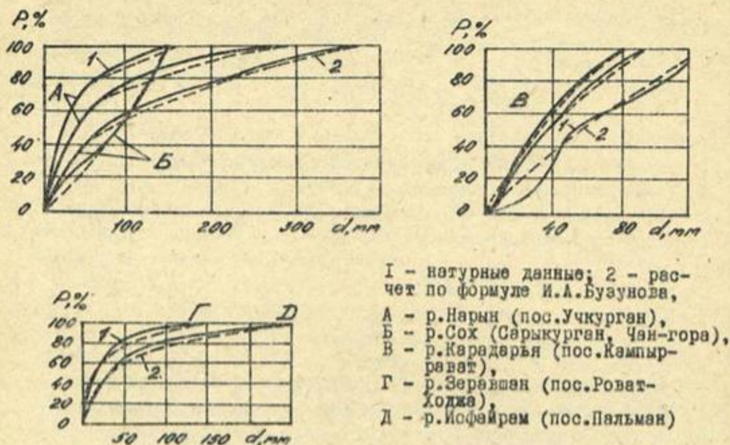
Рис. 4.1. Кривые суммарного фракционного состава влекомых наносов и донных отложений для рек Средней Азии горно-предгорной зоны
