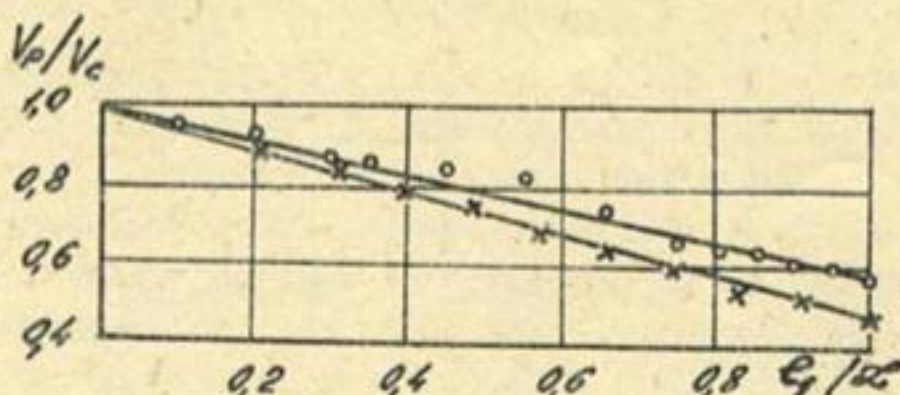
Рис. 5.4. График зависимости V_p/V_c от относительной длины подпора в верхнем бьефе Сарыжурганского гидроузла: x — 1950 г.; o — 1954 г.
