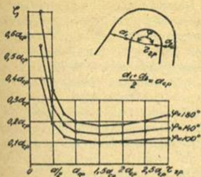
Рис. 9.3. Зависимость гидравлического сопротивления от радиуса гребня и угла поворота \zeta = f(\varphi_{cp}, \varphi)
