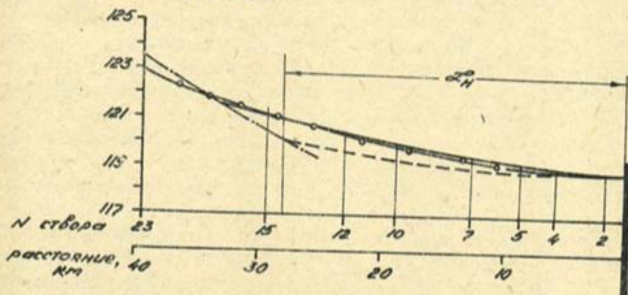
Рис. 5.5. Кривые подпора в верхнем бьефе Фархадского гидроузла: — о — натура на 15.07.1950 г. Q = 710 \text{ м}^3/\text{с} ; — по расчету на 1952 г. для расчетного расхода Q_n = 988 \text{ м}^3/\text{с} ; — по расчету на начало работы гидроузла; — бытовой уровень воды при расходе 990 \text{ м}^3/\text{с}
