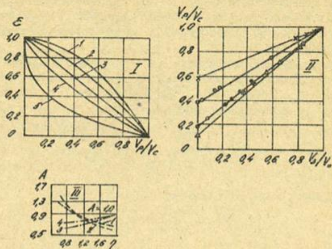
Рис. 4.3. Графики зависимостей \varepsilon = f(V_p/V_c) (I), V_p/V_c = f(V_3/V_0) (II) по расчету и натурным данным: A = f(\eta) (III) I - при значениях \eta : 1-2; 2-1,4; 3-1,0; 4-0,778; 5-1/3. II - бьефы: x - Кампырватский, o - Сарыкурганский; • - Верхнезеравшанский, Δ - Газалкентский. III - расчет по формулам: --- (4.22), —·— (4.33), 1,3 - a = 0,2 ; 2,4 - a = 0,4
