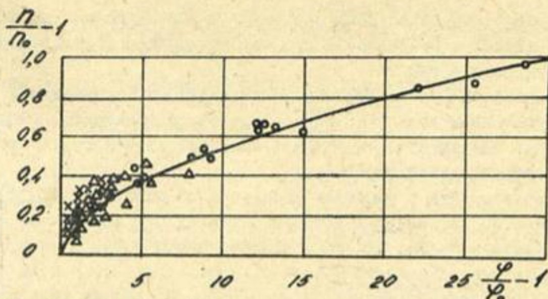
Рис. II.4. График n = f(\varphi) по данным гидрологических ежегодников для гравелисто-галечниковых русл рек: \circ - р. Пскем; \bullet - р. Нарын; \Delta - р. Чаткал; \times - р. Асса; \circ - р. Чу; — — расчет по предлагаемой формуле
