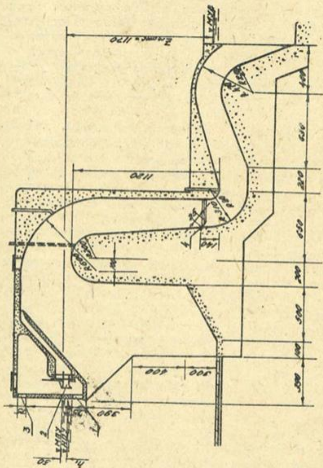
Рис. 9.13. Сифонный водосброс на 1150 м 3 /с при n = 12 трубах, B_{тр} = 4,00 м, \alpha_{тр} = 2,30 м, Q_{мин.} = 5,0 м 3 /с запроектирован ВСО Совхозодоканалпроект.
