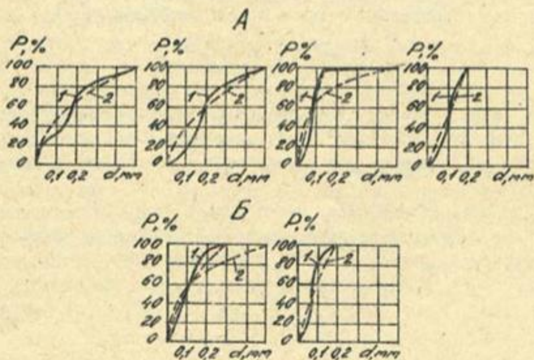
Рис. 4.2. Кривые фракционного состава донных отложений р. Амударьи по расчету и фактическим данным: 1 — натурные данные; 2 — расчет по формуле И.А.Бузунова. Створы: А — Керки; Б — Тяньмунь
