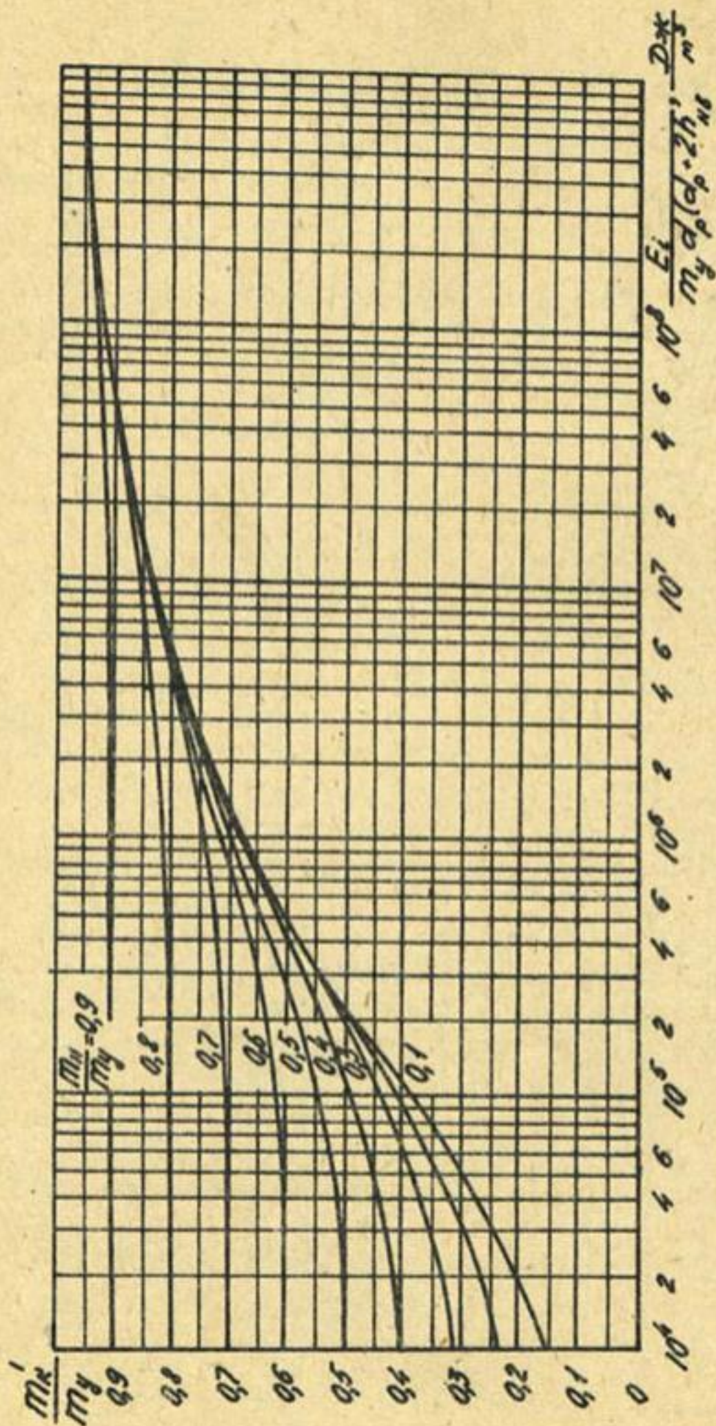
Рис. 6.16. График для определения коэффициента откоса m'_k из связных грунтов
