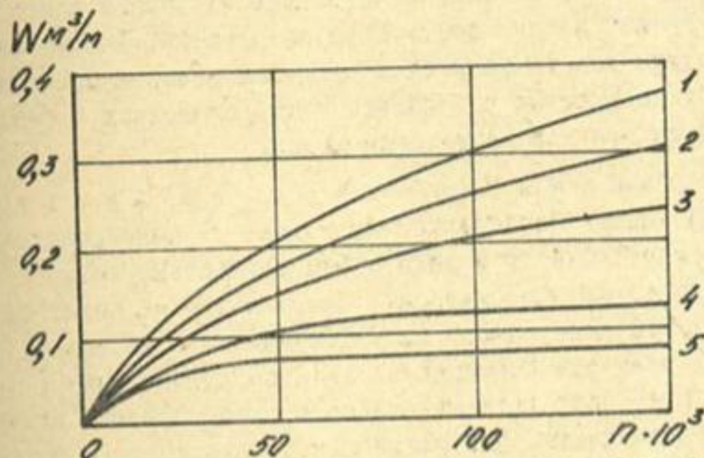
Рис. 7.2. График изменения объема размыва откоса по опытным данным в зависимости от длины подводной бермы и количества ударов волн:
