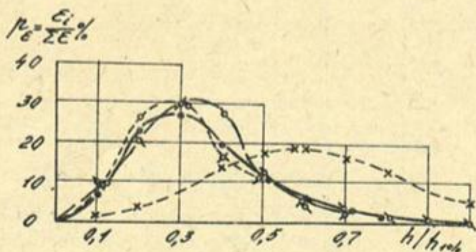
Рис. 6.5. Зависимость энергии волн от высоты волны с учетом кривых распределения высот волн и скоростей ветра для водохранилищ: ● - Ташкентского; □ - Чардаринского; ○ - Бугуньского; × - без учета кривой распределение ветра
