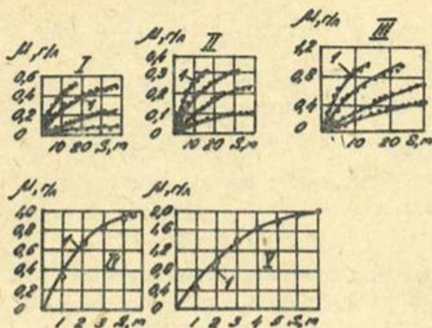
Рис. 12.2. Графики изменения удельного содержания наносов по длине размываемого русла:
