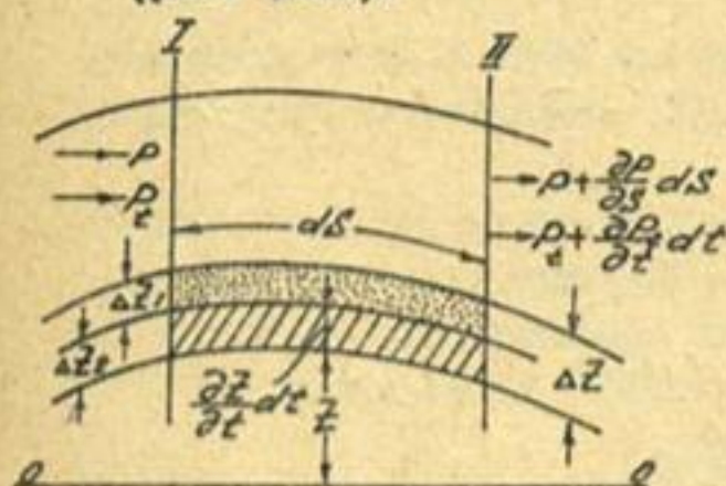
Рис. 12.3. Расчетная схема размыва русла в нижнем бьефе низконапорных гидроузлов.
