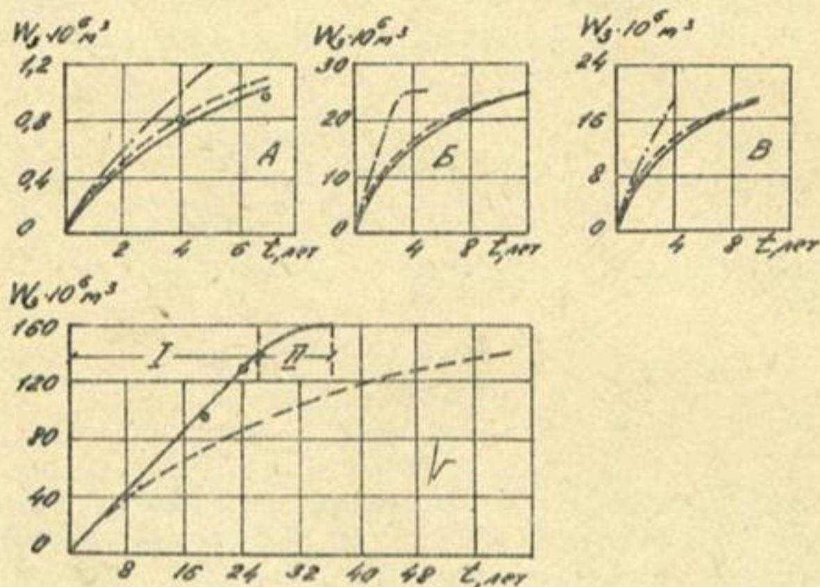
Рис. 3.4. Объемы заиления по расчету и натурным данным для верхних бьефов: А - Бозсуйский; Б - Уч-курганский; В - Султанбентский (вторая стадия); Г - Ташкепринский; О - натурные данные; — по расчету предлагаемым методом; --- по методу В.С.Лапшенкова; —·— по методу И.А.Шнеера; I - I стадия заиления; II - II стадия заиления
