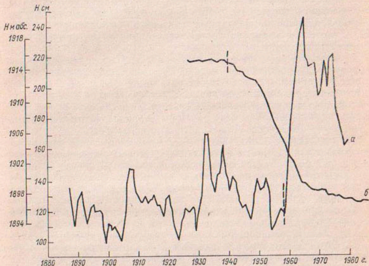
Рис. 6.3. Хронологические графики колебаний уровня озер, подверженных антропогенному влиянию. а — оз. Байкал; б — оз. Севан.
