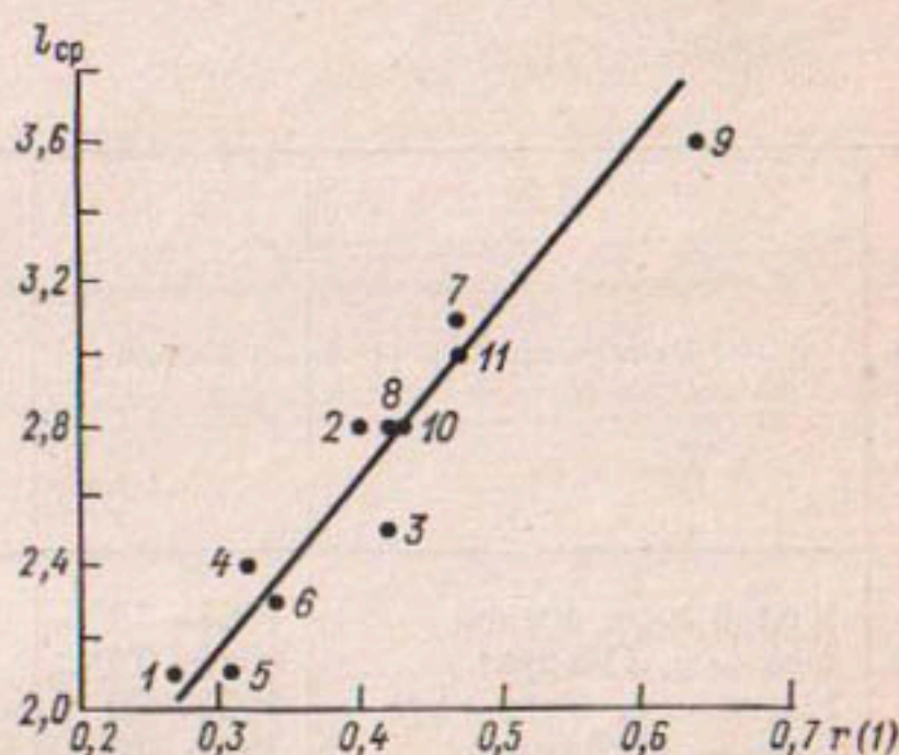
Рис. 5.9. Зависимость средней продолжительности группировок лет различной водности ( l_{\text{ср}} ) от коэффициента корреляции между стоком смежных лет r(1) в рядах подземного стока.
