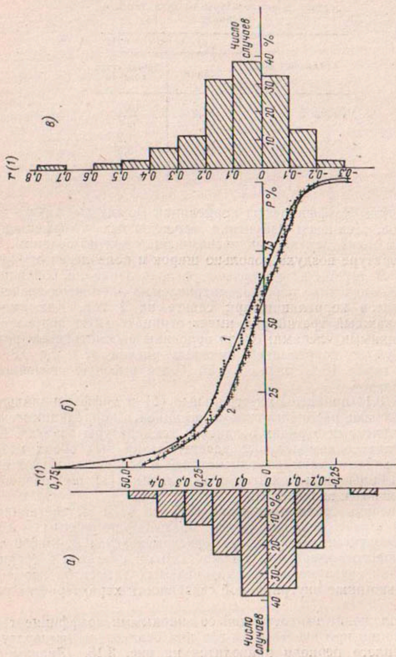
Рис. 3.14. Дифференциальные (а, в) кривые распределения и кривые распределения r(1) (б) в рядах температуры и осадков. 1) r(1) для осадков, 2) r(1) для температуры воздуха.
