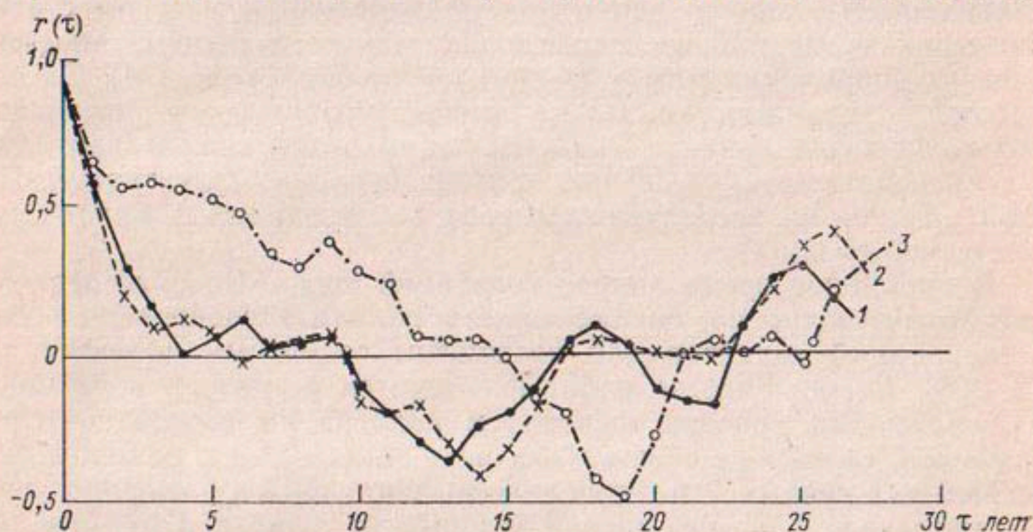
Рис. 6.6. Автокорреляционные функции среднегодовых значений уровня озера Селигер.
