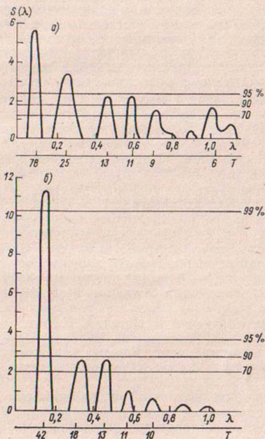
Рис. 6.7. Спектральные плотности уровня озера Байкала (а) и Б. Чаны (б).
