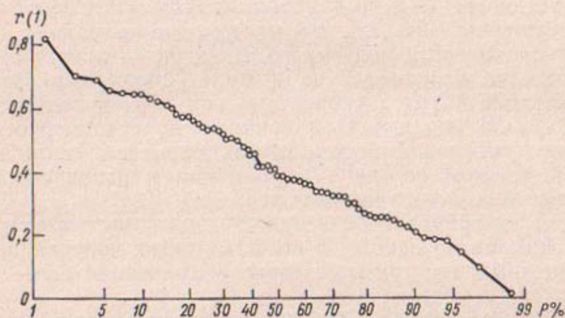
Рис. 5.2. Эмпирическая кривая обеспеченности коэффициентов корреляции между стоком смежных лет r(1) для всей совокупности рядов подземного стока.
