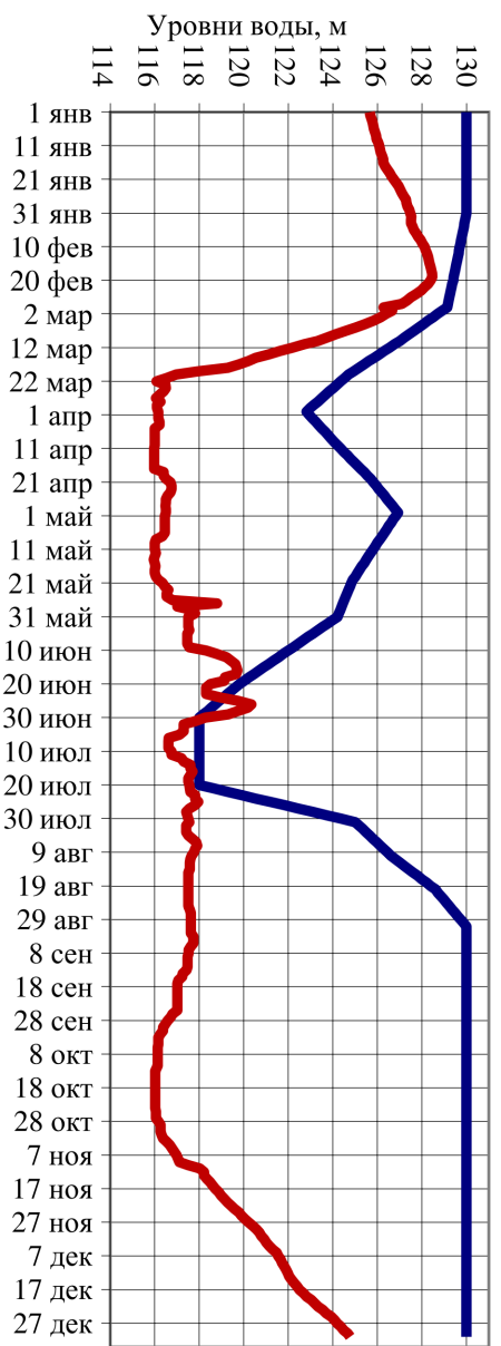
Рис. 3.1 Сравнение работы Руслового водохранилища по фактическим и рекомендуемым вариантам режимов для различных по водности годов:
