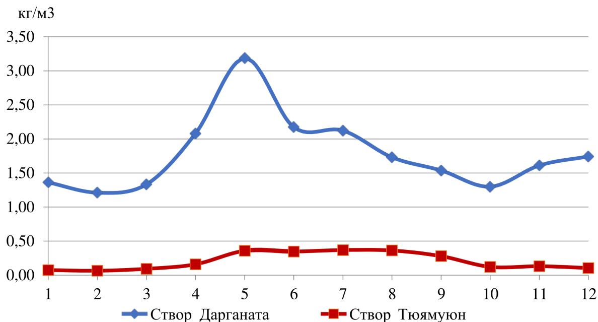
Рисунок 1.4 Среднемесячные мутности воды
