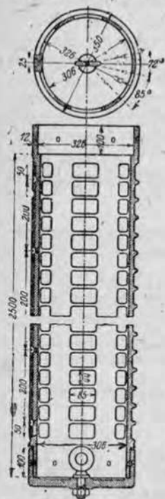
Рис. 220. Чугунный фильтр (по А. Тиму).
