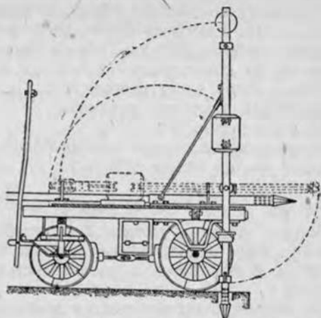
Рис. 210. Оборудование для устройства абиссинских колодцев, помещенное на особой тележке (по Донна).
