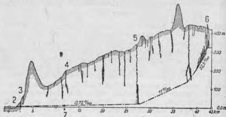
Рис. 157. Продольный разрез подземного течения реки Тимаво между гротом Сен-Кауц-иан и Дуино (по Бегану).
