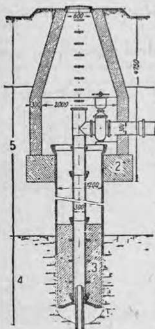
Рис. 251. Предохранение артезианского колодца Карани от притока воды.
