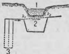
Рис. 289. Устройство подъемного трубопровода в виде дюкера.
