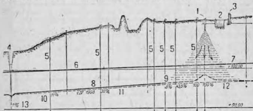
Рис. 320. Сооружение для образования грунтовой воды в городе Франкфурте-на-Майне (по Шельгге).
