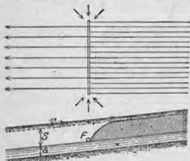
Рис. 123. Схематическое изображение режима горизонтального колодца.
