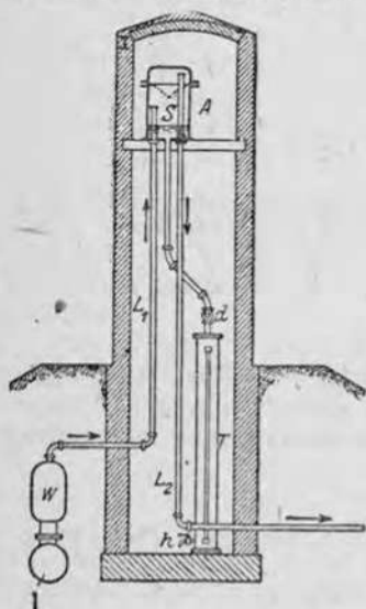
Рис. 291. Вентиляционная башня каптака грунтовой воды в городе Праге.
