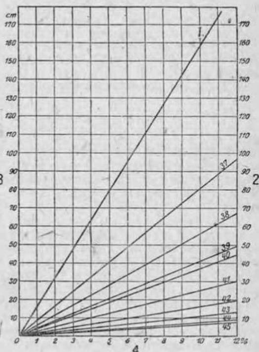
Рис. 126. Водопроницаемость просеянных песков (по Кинг-Людюк).
