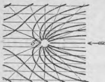
Рис. 117. Графическое изображение водных струй в районе действия колодца (по Баудину).
