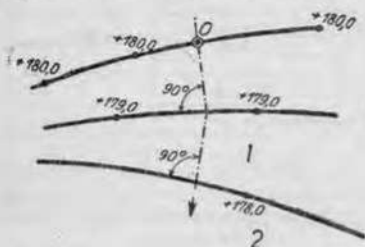
Рис. 73. Нанесение на план в горизонталях одинаковых уровней грунтовой воды (+180+179+178).
