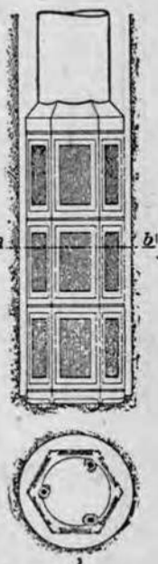
Рис. 271. Фильтр со стеклянными пластинами (по Путзейсу).
