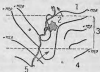
Рис. 80. Изменение взаимоотношений между поверхностной водой и грунтовой (по А. Тимму).
