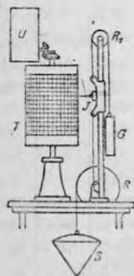
Рис. 49. Самопишущий футиток (по Будау).
