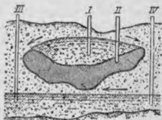
Рис. 67. Образование ложного зеркала воды в слабопроницаемом пласте, залегающем на пласте глин.
