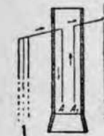
Рис. 293. Правильное соединение подъемного и всасывающего трубопровода.
