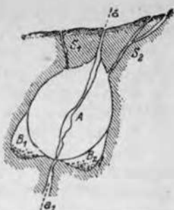
Рис. 147. Схематическое изображение образования вследствие коррозии и эрозии подземной пустоты.
