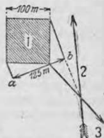
Рис. 140. Четырехугольный каптаж водопровода города Люттиха (по Дегинне).
