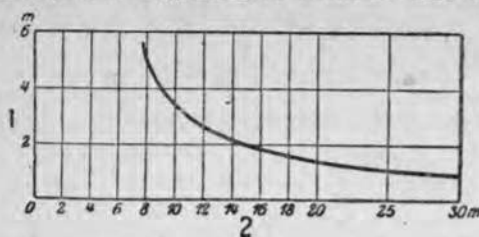
Рис. 138. Диаграмма зависимости между депрессией и мощностью водоносного пласта (по Кирпильеу).
