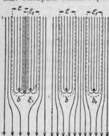
Рис. 122. Два смежных колодца, взаимно отбирающие друг у друга воду (слева), и два таких же колодца, между которыми протекает некаптированная вода (справа).
