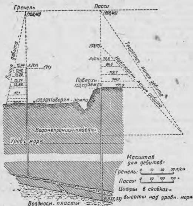
Рис. 134. Линии дебита артезианских колодцев в Гренеле и Пасси (по Дююи).
