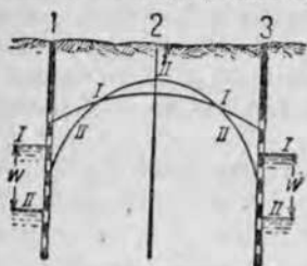
Рис. 308. Сопроительство в каптаже.
