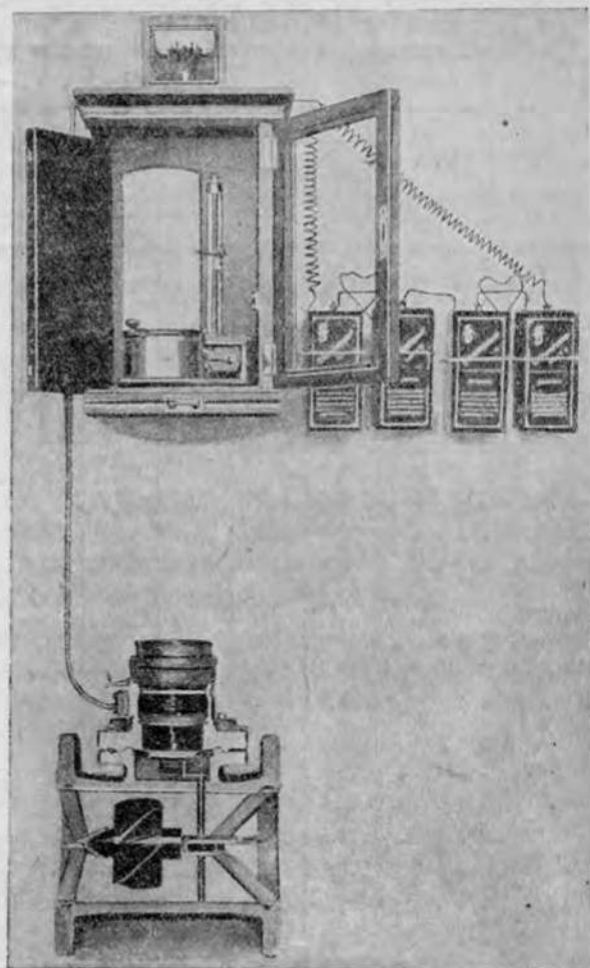
Рис. 50. Водомер Вольтмана с саморегистрирующим аппаратом (по Сименсу и Гальске).
