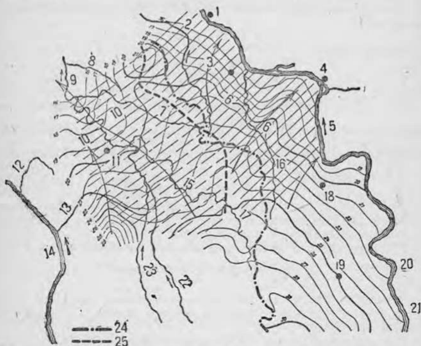
Рис. 95. План в гидроизоглипах между Рейном и Маасом и направление поверхностного и подземного водоразделов (зеркало воды от декабря 1908 г. до октября 1909 г.).
