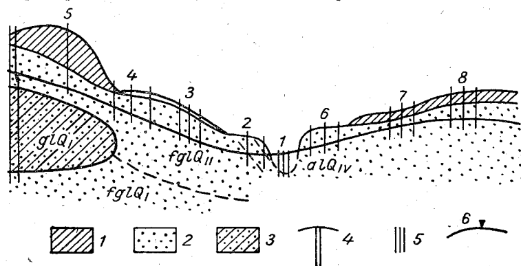
Рис. 19. Створ наблюдательных скважин по поперечнику к реке. 1 — суглинки, 2 — пески, 3 — линза суглинков с гравием, 4 — скважина в зоне местного напора, 5 — тройник скважин для расчета элементарных расходов подземного потока, 6 — уровень грунтовых вод.
