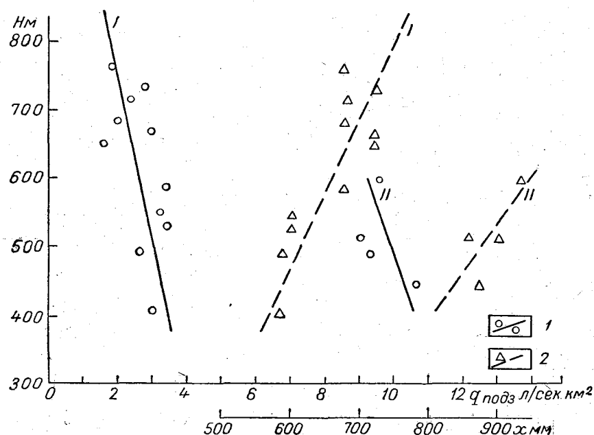
Рис. 54. Зависимость подземного стока в реки западного склона Урала от осадков и средней высоты водосбора.
