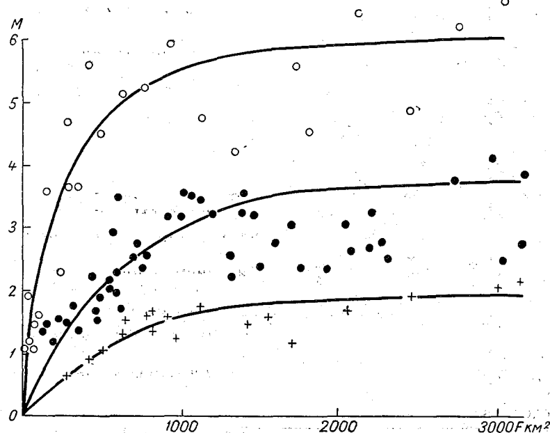
Рис. 41. Зависимость модуля минимального 30-дневного летнего стока от площади бассейна при равномерном возрастании интенсивности питания по длине реки.
