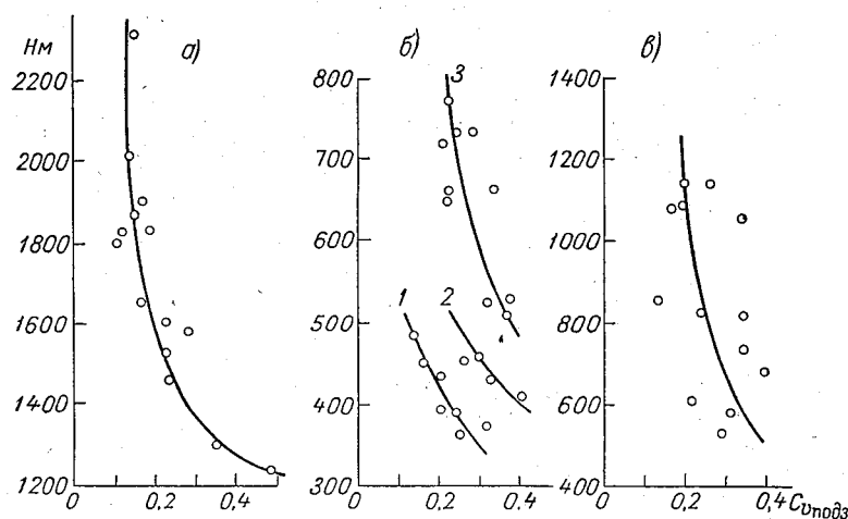
Рис. 65. Зависимость коэффициента вариации подземного стока в реки от средней высоты водосбора H для горных районов ЕТС.
