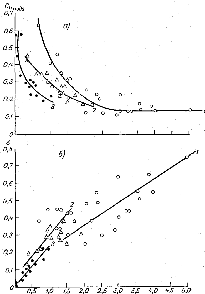
Рис. 63. Зависимость коэффициента вариации C_{v \text{ подз}} и среднеквадрата \sigma от расхода q_{\text{подз}} для равнинных районов, а — для
