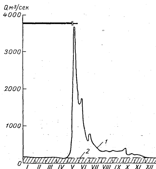
Рис. 35. Схема расчленения гидрографа болотной реки по устойчивой меже. 1 — поверхностный сток, 2 — подземный сток.
