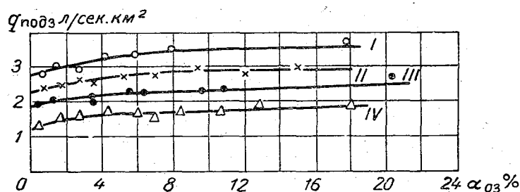
Рис. 32. Связь среднегодовых модулей подземного стока в реку q_{подз} и коэффициентов озерности бассейнов \alpha_{оз} .
