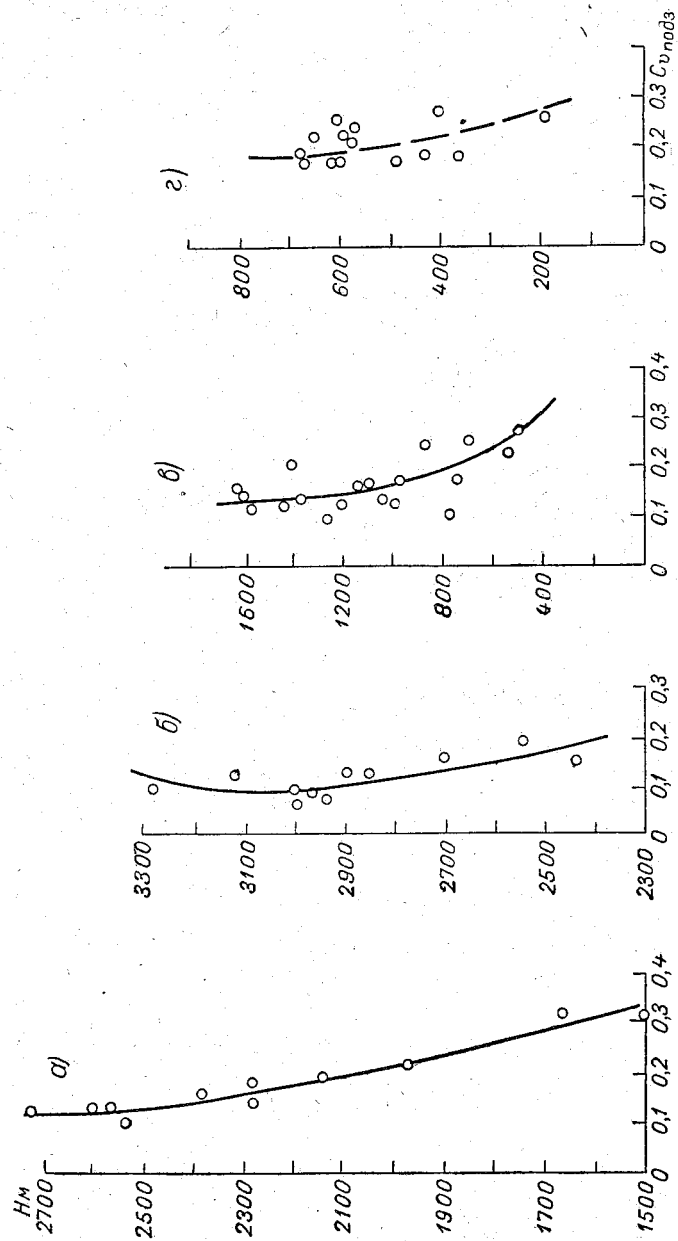
Рис. 68. Зависимость коэффициента вариации подземного стока в реки от средней высоты водосбора для горных районов Азиатской территории СССР. а — южный склон Гиссарского хребта, б — Киргизский хребет, в — западный склон хребта Сихотэ-Алинь, г — восточный склон хребта Сихотэ-Алинь.
