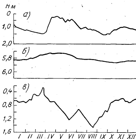
Рис. 5. Изменение уровня грунтовых вод в различных природных зонах.
