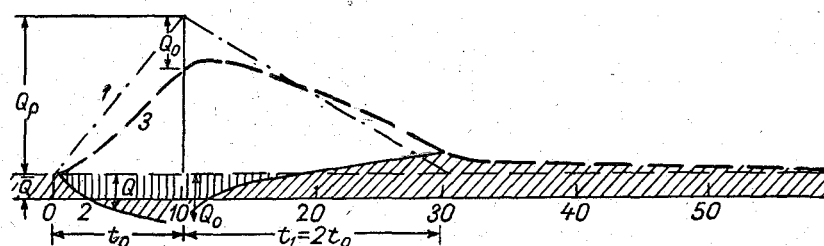
Рис. 36. График поступления воды в берега реки и обратно при прохождении паводка (по С. Ф. Аверьянову). Приняты условия: Q_0=2Q ; Q_p=6Q .
