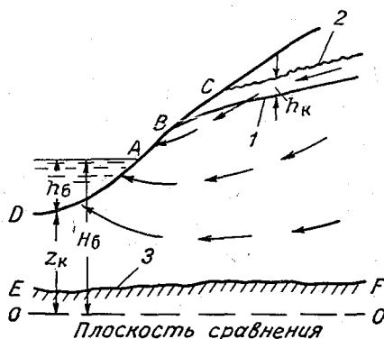
Рис. 7. Элементарная схема дренирования водоносного пласта рекой.
