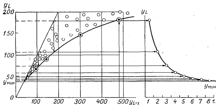
Рис. 2. Схема построения «кривой истощения» по нижней огибающей, по М. И. Гуревичу.
