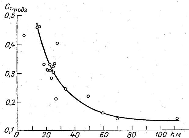
Рис. 66. Зависимость коэффициента вариаций подземного стока от глубины эрозионного вреза рек ( h м) для поля четвертичных отложений в западной части Русской плиты.
