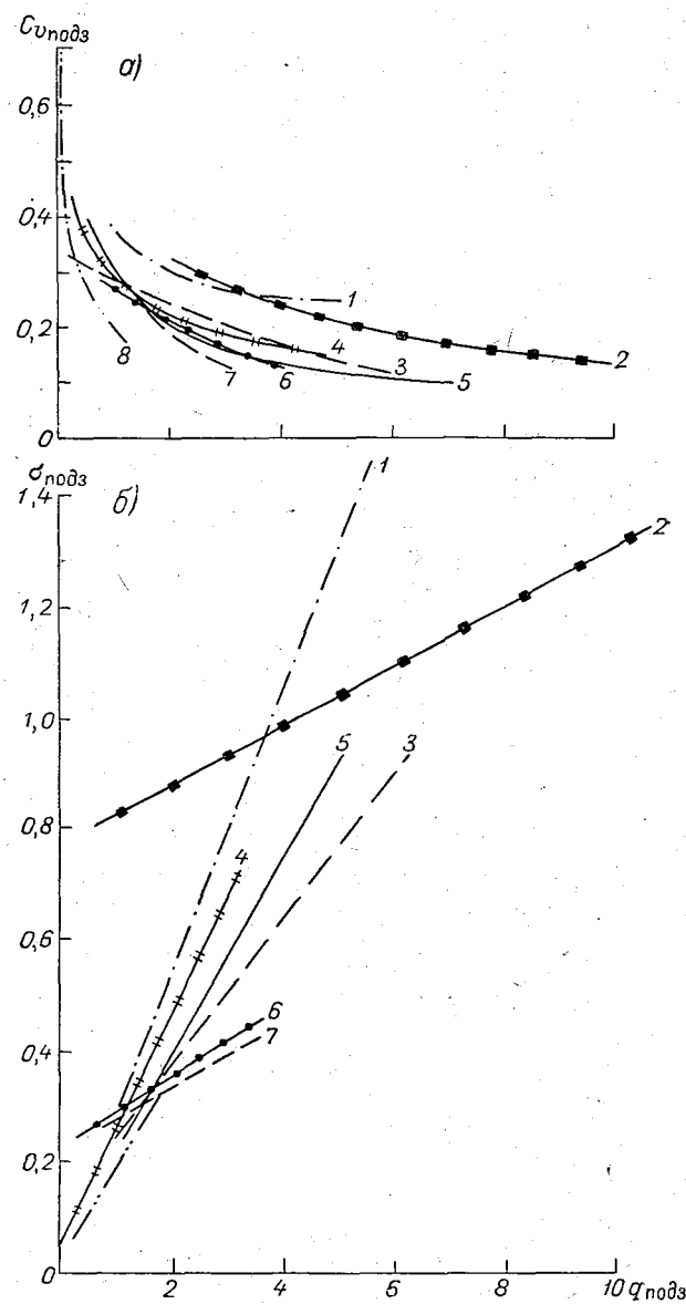
Рис. 69. Совмещенный график зависимостей коэффициентов вариации Cv_{\text{подз}} от модуля подземного стока q_{\text{подз}} (а) и среднего квадратичного отклонения \delta_{\text{подз}} (б) от модуля подземного стока для различных районов Азиатской территории СССР.
