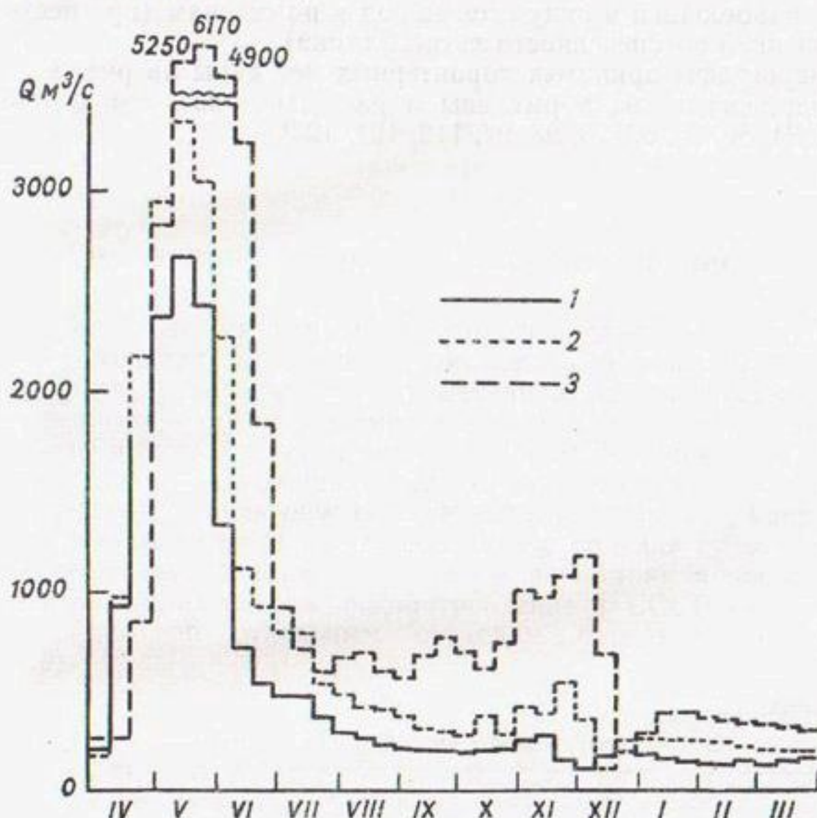
Рис. 3. Характерные гидрографы.
