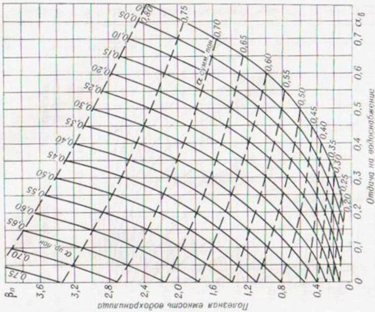
Рис. 70. Номограмма для расчета водохранилищ, работающих на водоснабжение и ирригацию при C_{\text{вр}}=0.7 (ориентировочная).
