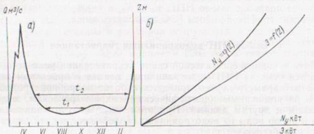
Рис. 90. Зависимость установленной мощности N_y и средней годовой энерговыработки ГЭС E от отметки НПГ водохранилища Z .
