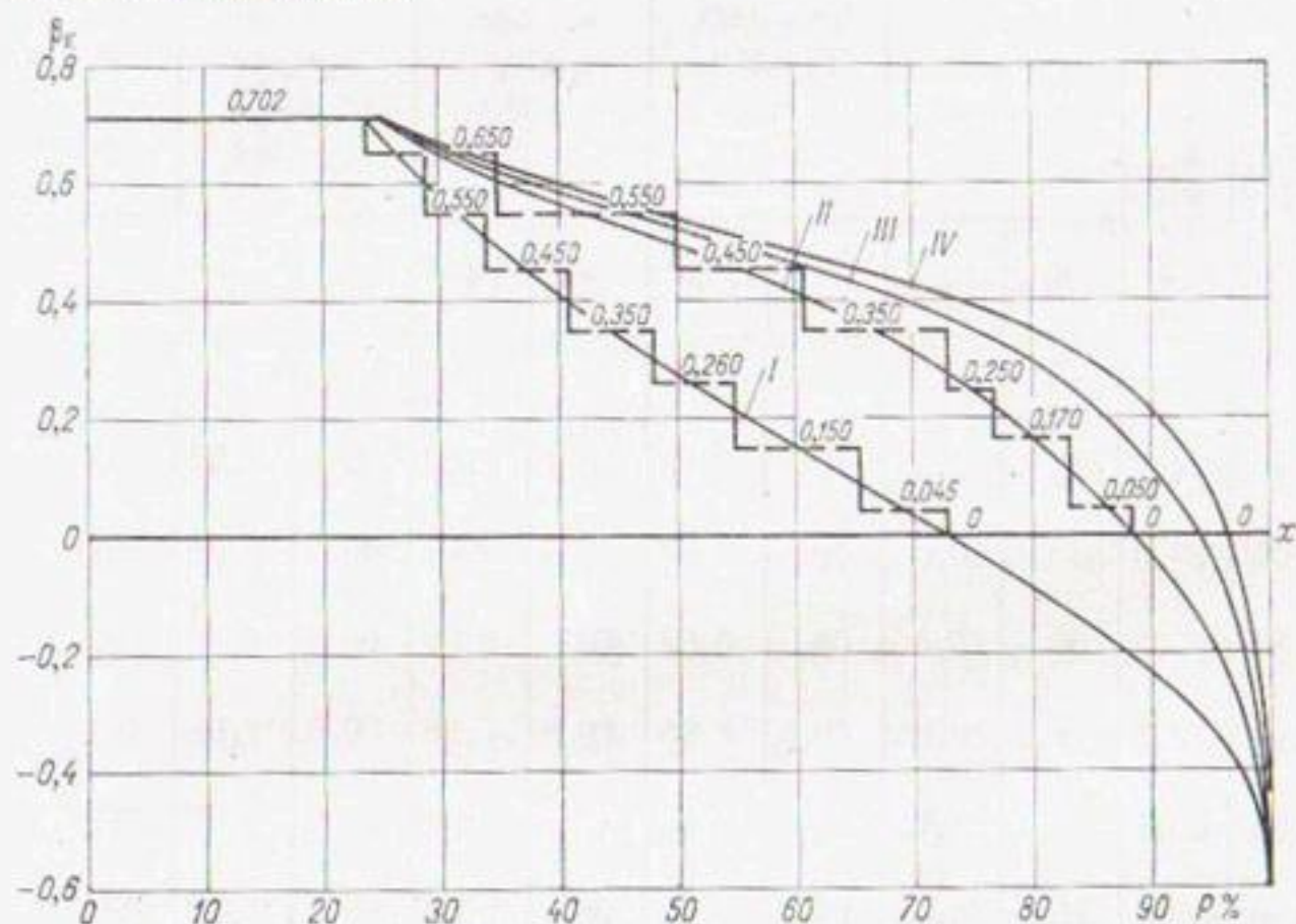
Рис. 49. Кривые обеспеченности наполнений водохранилища к концу года (к началу весны) из расчета по году в целом при \alpha=0,62 , \beta_{\text{н}}=0,702 , C_{\text{вг}}=0,55 , C_{\text{з}}=2C_{\text{вг}} , m=0,40 .
