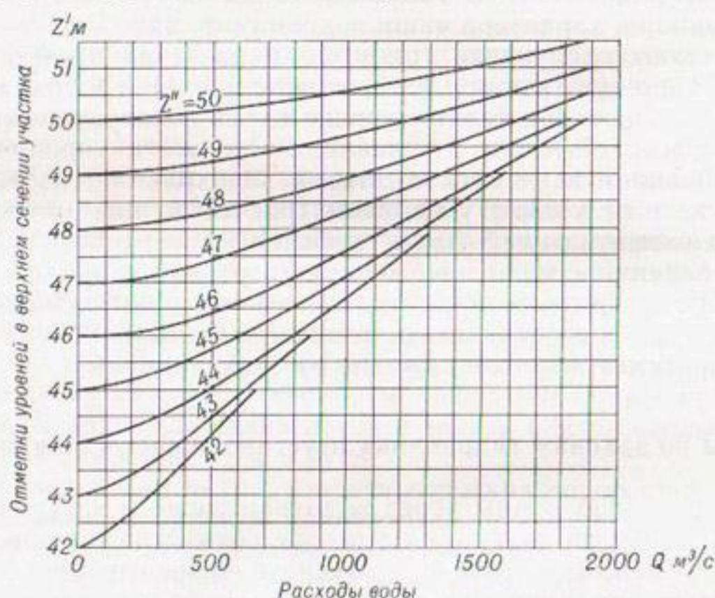
Рис. 115. Зависимость Q = \varphi(Z', Z'') .
