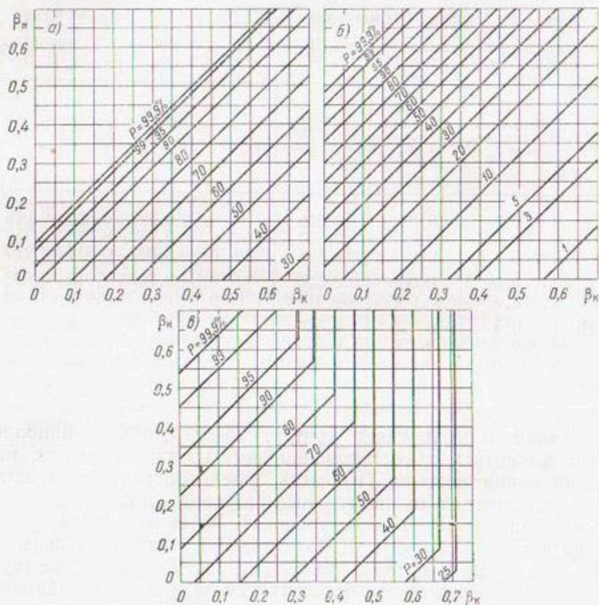
Рис. 47. Номограмма \beta_k = \varphi(\beta_v, P) раздельно по фазам стока (а и б) и по году в целом (в).
