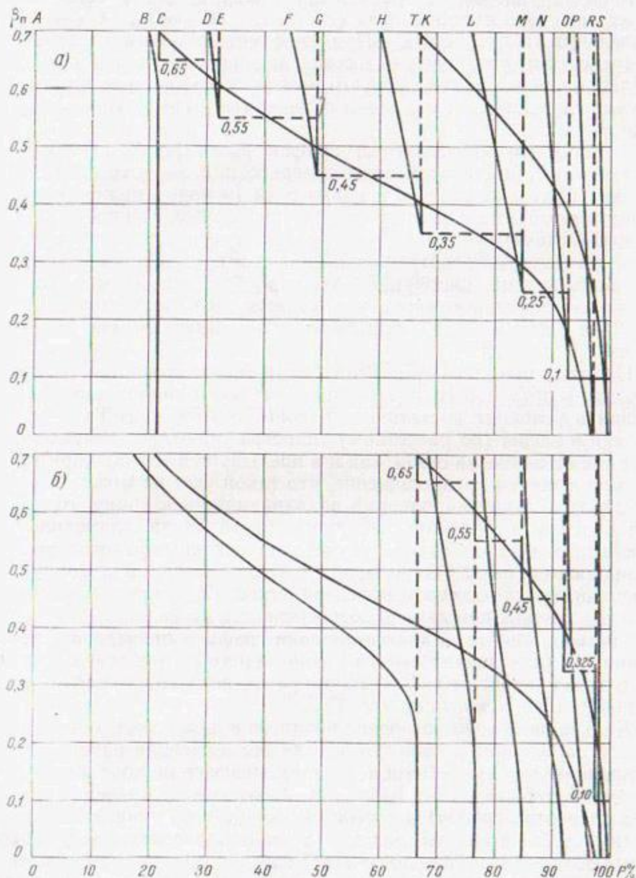
Рис. 48. Построение кривых обеспеченности наполнений водохранилища при разбивке годового стока на две фазы.
