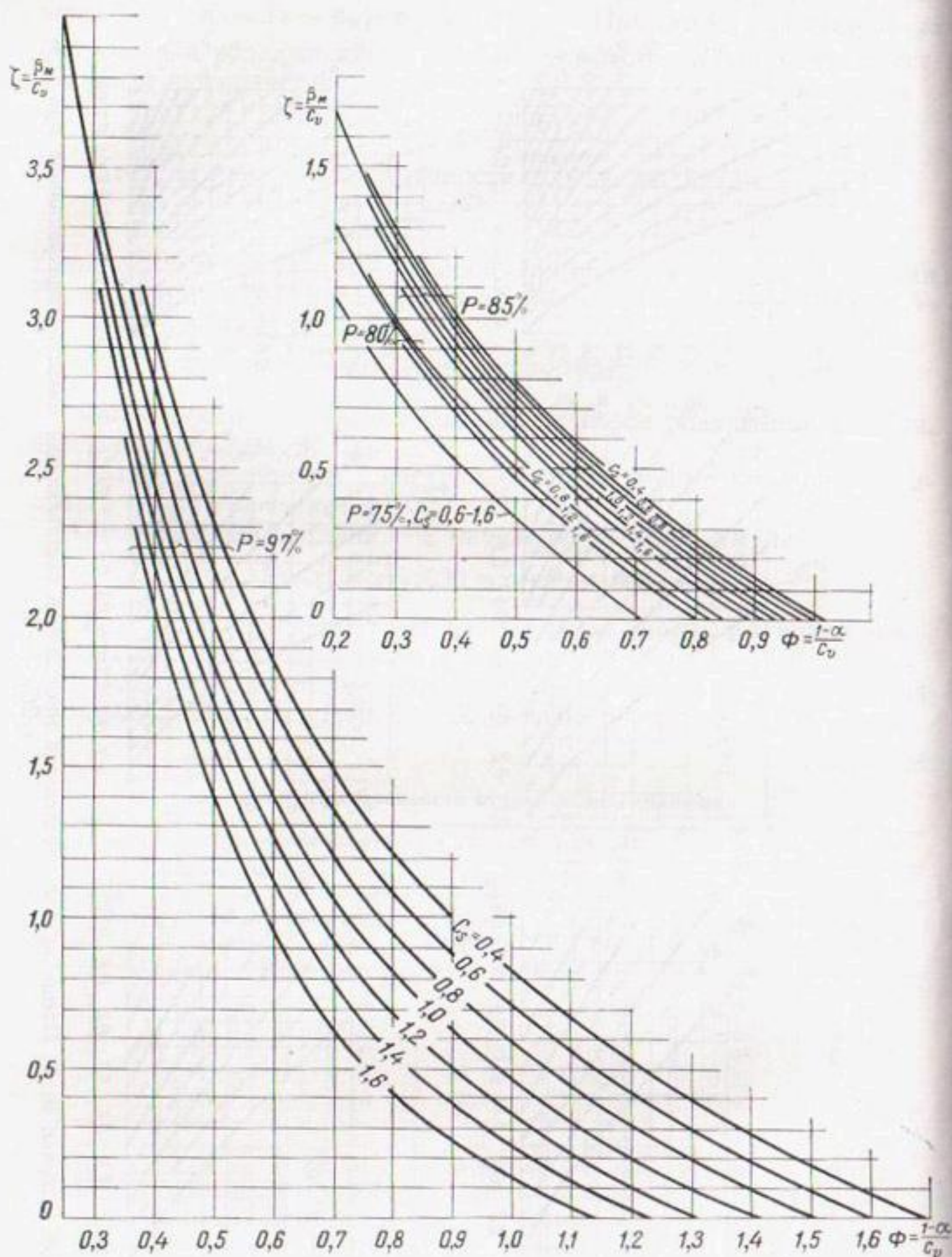
Рис. 39. Графики Н. М. Милославского для определения многолетней составляющей емкости водохранилища при C_s \leq 2C_v , r=0 и P , равных 75, 80, 85, 97%.
