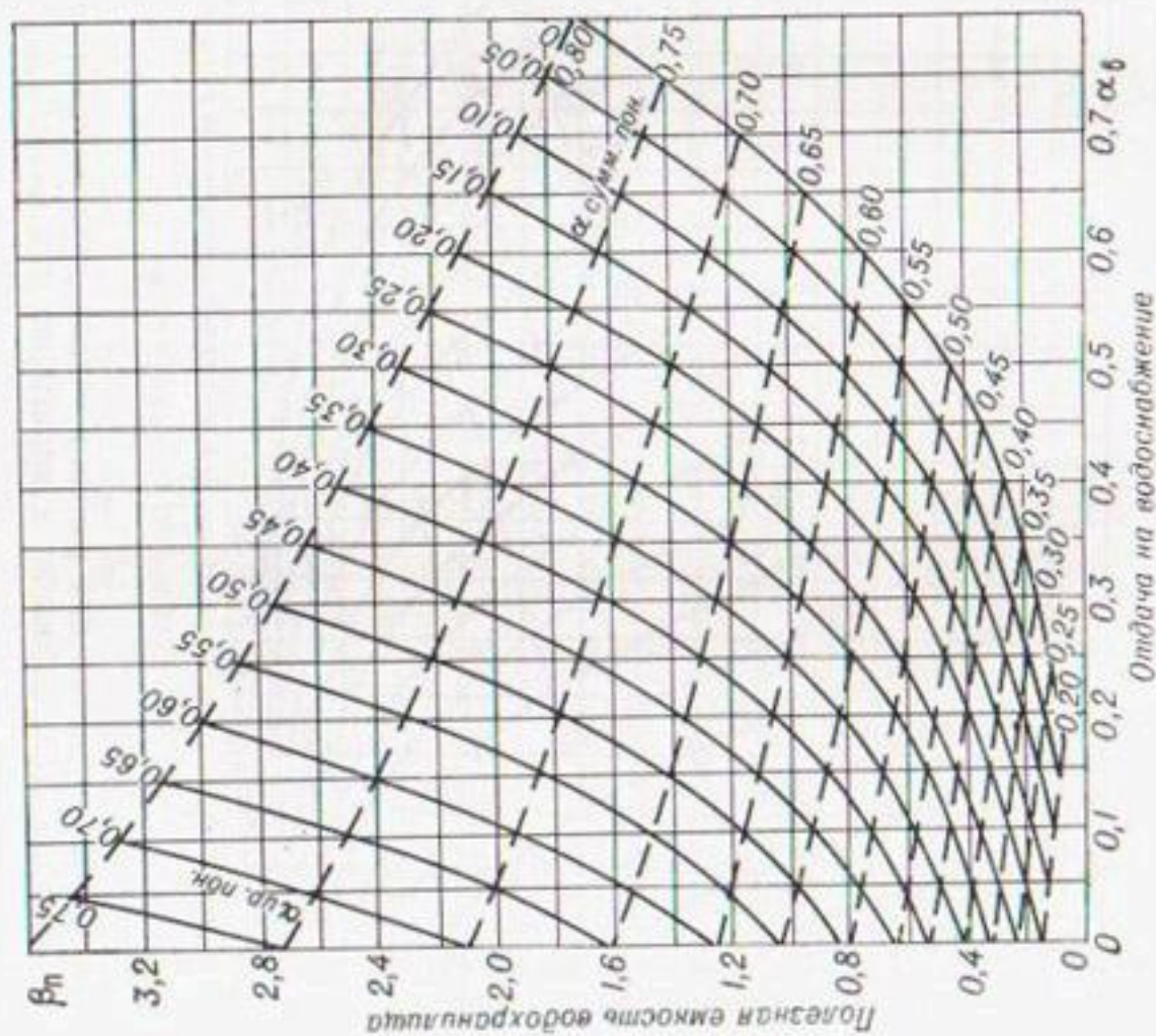
Рис. 69. Номограмма для расчета водохранилищ, работающих на водоснабжение и ирригацию при C_{\text{вр}}=0.6 .
