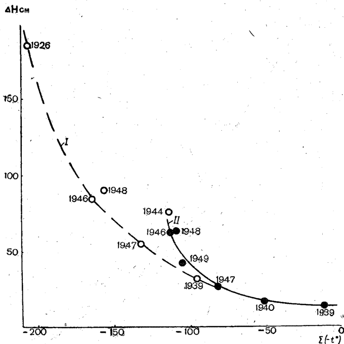
Рис. 14. Связь сумм отрицательных среднесуточных температур воздуха предледоставного периода с повышениями уровней от их минимума на „птичке“ до ледостава (годы наблюдений указаны на точках связи).
