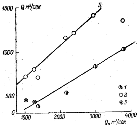
Рис. 15. Зависимости Q_{\min} и Q_{\text{вост}} от устойчивых расходов открытого русла ( Q_0 ). Р. Кама, с. Тарловка.
