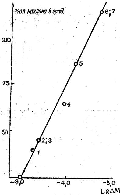
Рис. 11. Зависимость углов наклона кривых \Sigma(t^\circ) = f(M_{\text{пр}}) от величины приращения модулей стока на 1 км длины реки (номера при точках соответствуют порядку расположения вододельных постов в табл. 7).
