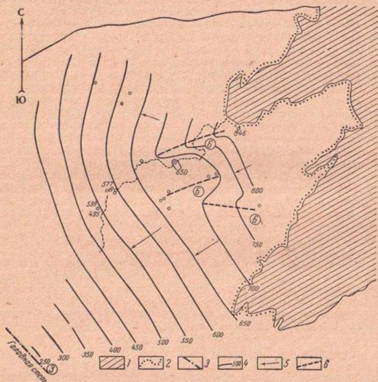
Рис. 30. Схема естественного потока подземных вод сеноманского водоносного горизонта Приташкентского артезианского бассейна. Составил В. А. Вaleyшo
