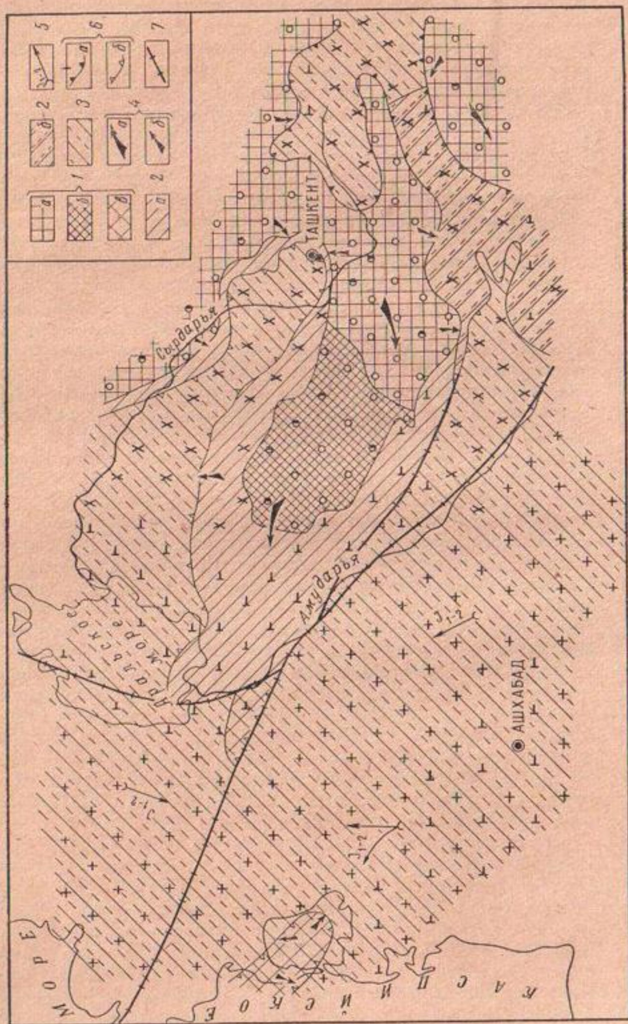
Рис. 5. Палеогеологическая схема раннего мела (неоком) области и фильтрации. Зоны формирования: 1 — пресных (до 1 з 4) трещинно-карстовых и трещинных вод в пределах выходов складчатого фундамента палеозой: а — в глубоких расчлененных восточных горах; б — в глубоких горах; в — в слабосклонных равнинах; г — в слабосклонных равнинах; д — в слабосклонных равнинах; е — в слабосклонных равнинах; ж — в слабосклонных равнинах; з — в слабосклонных равнинах; и — в слабосклонных равнинах; к — в слабосклонных равнинах; л — в слабосклонных равнинах; м — в слабосклонных равнинах; н — в слабосклонных равнинах; о — в слабосклонных равнинах; п — в слабосклонных равнинах; р — в слабосклонных равнинах; с — в слабосклонных равнинах; т — в слабосклонных равнинах; у — в слабосклонных равнинах; ф — в слабосклонных равнинах; х — в слабосклонных равнинах; ц — в слабосклонных равнинах; ч — в слабосклонных равнинах; ш — в слабосклонных равнинах; щ — в слабосклонных равнинах; ъ — в слабосклонных равнинах; ы — в слабосклонных равнинах; ь — в слабосклонных равнинах; э — в слабосклонных равнинах; ю — в слабосклонных равнинах; я — в слабосклонных равнинах.
