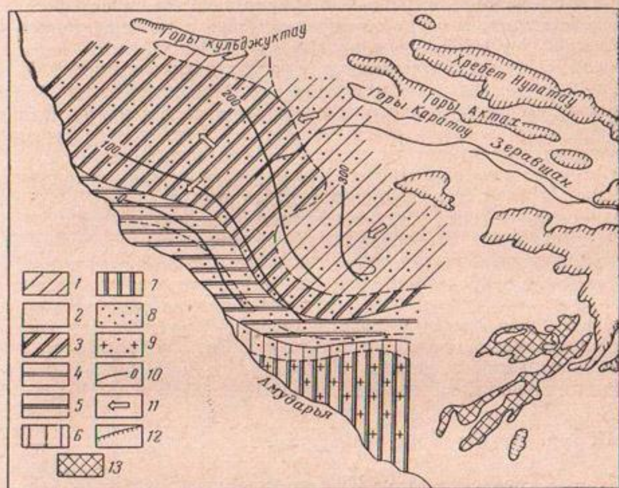
Рис. 23. Схематическая карта гидрогеохимических зон и гидродинамических условий сеноманских отложений (X пронизанный горизонт) Бухаро-Каршинского артезианского бассейна. Составил Л. Е. Михайлов
