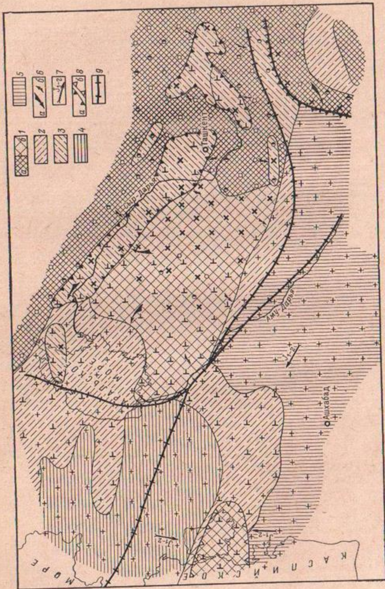
Рис. 4. Палеогеологическая схема поздней юры
