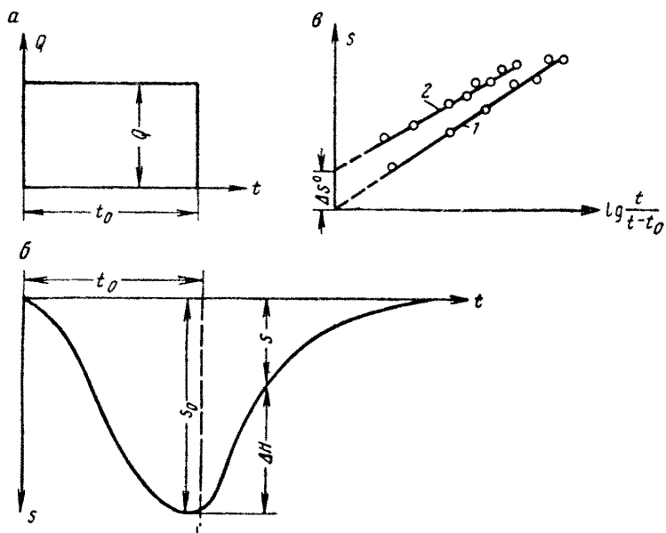
Рис. 25. Восстановления уровня после остановки откачки.
