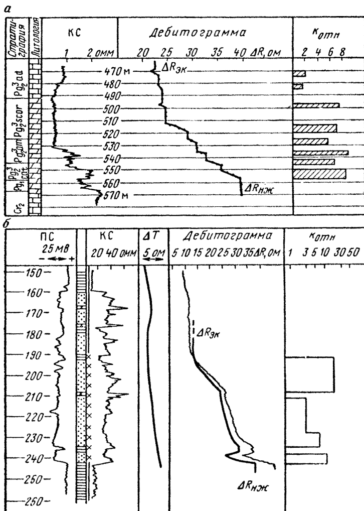
Рис. 62. Расходомерия с использованием термдебитомера. а — по методике дискретных замеров; б — по методике непрерывных измерений
