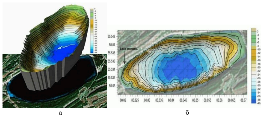
Рис. 1. Схема оз. Инголь с отметками глубин (изобатами)
