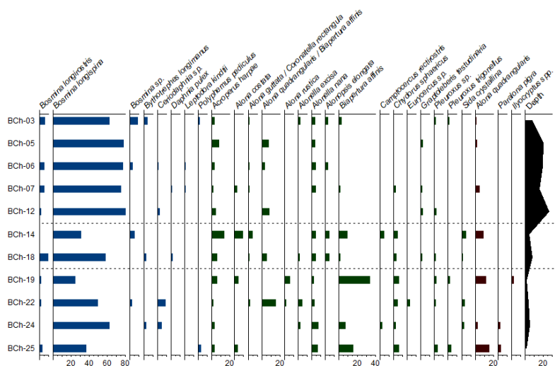
Рис. 2. Относительное обилие таксонов Cladocera в %: синим цветом обозначены пелагические таксоны, зеленым – литоральные, коричневым – бентосные
