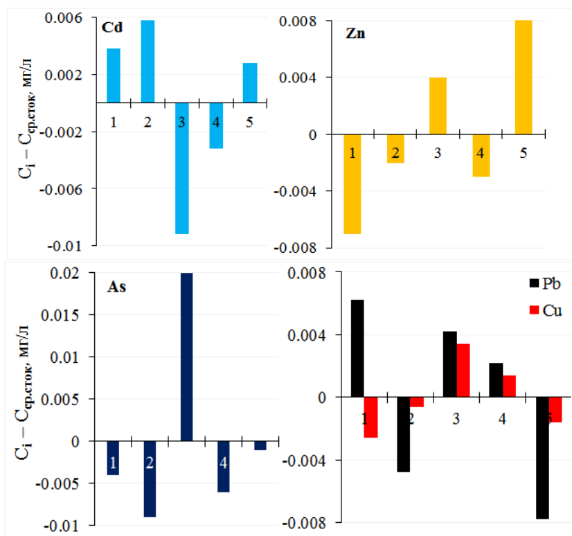
Рис. 3. Динамика изменения концентрации вдоль русла реки Сырдарья и значений концентраций Cd, Zn, As, Pb, Cu и Cг в соответствующих точках отбора проб воды
