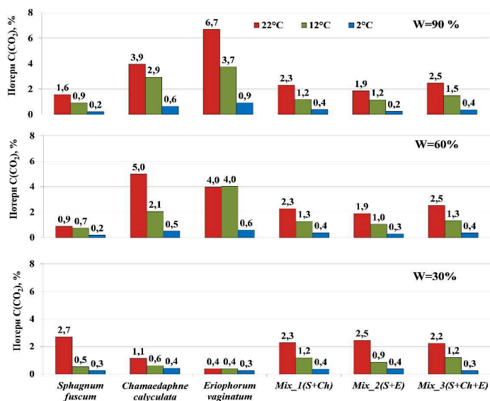
Рис. 2. Суммарные потери C(CO_2) за 30 дней из различных видов растительного опада при температурах (2, 12, 22 °C) и разных уровнях влажности (30, 60 и 90 % их полной влагоемкости), % от исходного количества С в образце
