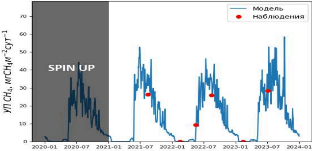
Рис. Годовой ход УП метана по данным наблюдений и моделирования для Куйбышевского водохранилища
