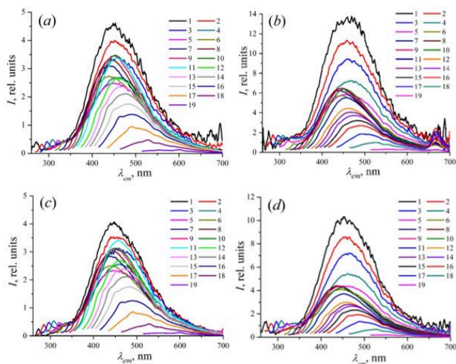
Рис. 2. Спектры флуоресценции РОВ в оз. Трехцветное – горизонты 0 м (а) и 2 м (б); и в оз. Елового – горизонты 0 м (с) и 3 м (д). Кривые с 1 по 16 соответствуют \lambda_{\text{ex}} 250–400 нм с шагом 10 нм, 17 – 420 нм, 18 – 450 нм, 19 – 500 нм
