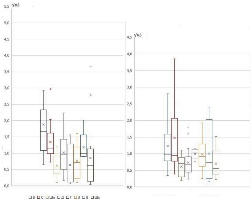
Рис. 2. Биомасса фитопланктона в июне (слева) и августе-сентябре (справа) в различных районах акватории Ладожского озера в 2020-2023 гг.
