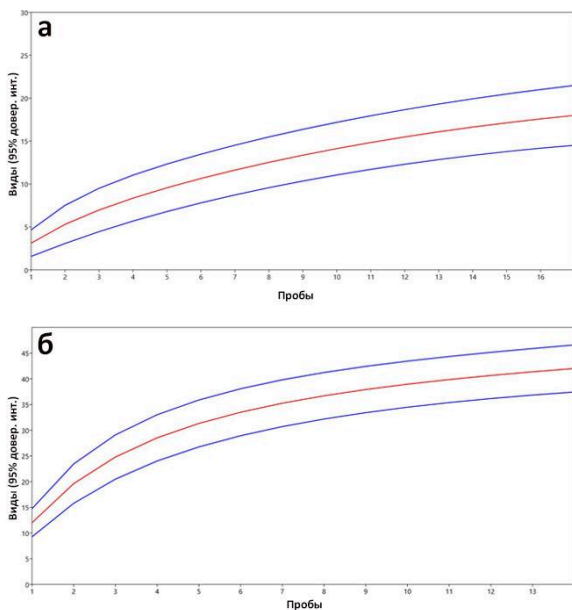
Рис. 2. Кривые накопления видов: а – для района высокогорья (окрестности озера Бунисяк); б – для района низкоргорья (исток реки Муксун). Синие линии – 95% доверительные интервалы
