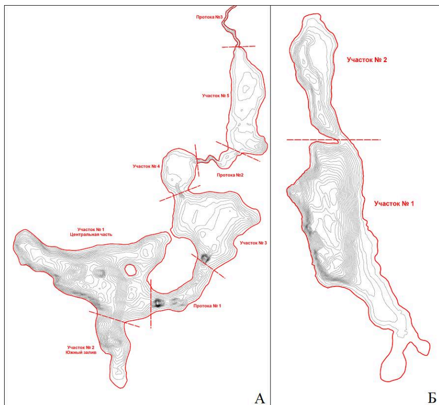
Рис. Планы озер по результатам батиметрической съемки 2016 г. А – Ковалевское; Б – Архирейское
