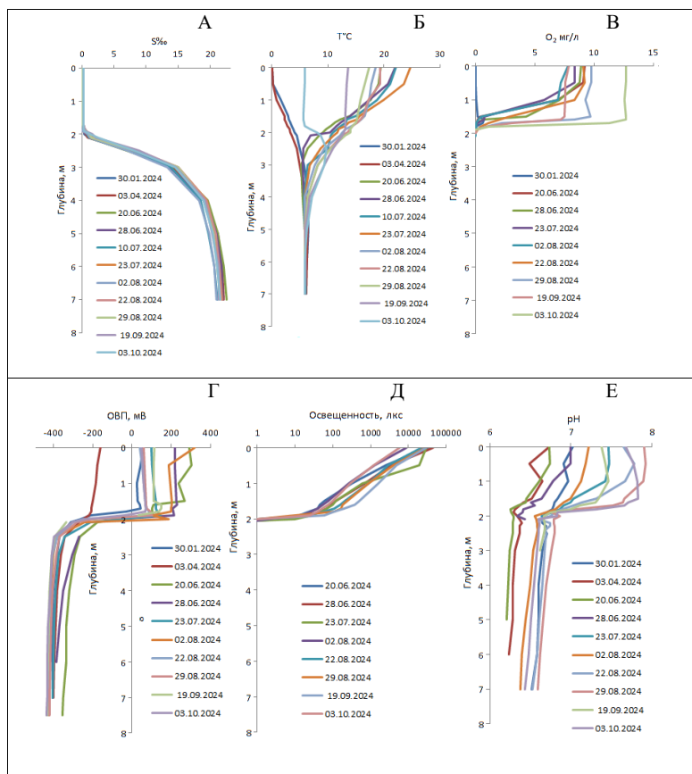
Рис. 1. Профили гидрологических параметров в оз. Трехцветное в разные месяцы 2024 года по данным 11 сезонных съемок: А – соленость (‰), Б – температура (°C), В – концентрация растворенного в воде кислорода (мг/л), Г – окислительно-восстановительный потенциал (мВ), Д – освещенность под водой (лк), Е – Ph
