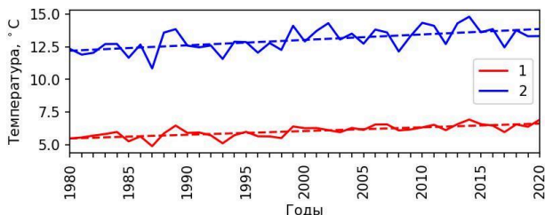
Рис. 1. Межгодовая изменчивость среднегодовой, осредненной по всему объему озера (1), и средней за вегетативный период (май-октябрь), осреднённой по фотическому слою (2), температуры воды по результатам моделирования
