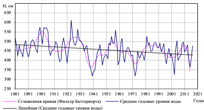
Рис. 3. Хронологический график хода уровней воды Ладожского озера
