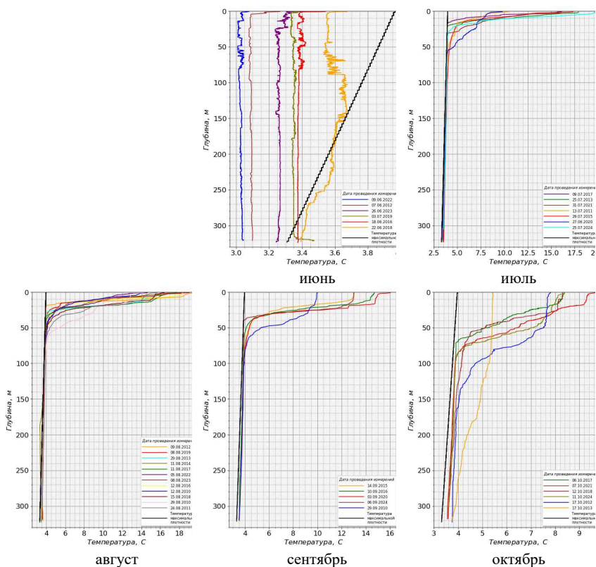
Рис. 2. Вертикальные профили температуры по измерениям за 2010-2024 гг. на станции р031
