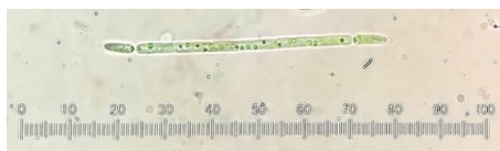
Рис. 2. Микрофотографии Raphidiopsis raciborskii из оз. Лунское (цена деления линейки на фотографиях – 1 мкм)
