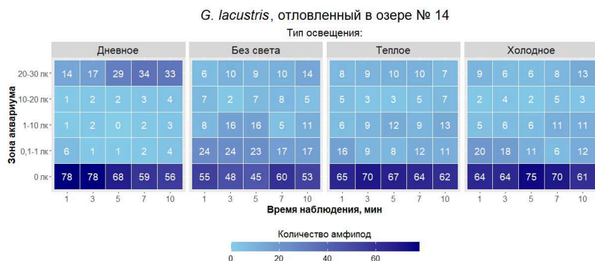
Рис. 1. Распределение суммарного количества особей G. lacustris , отловленных в озере № 14, в зависимости от уровня освещенности и времени наблюдения при различных типах освещения
