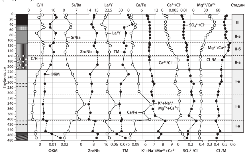
Рис. 3. Геохимические индикаторы условий осадконакопления. ФКМ – фосфор-кальциевый модуль ( P_2O_5/CaO ), ТМ – титановый модуль ( TiO_2/Al_2O_3 ), М – минерализация. I–III стадии эволюции озера (см. в тексте). Жирными линиями показаны участки донных отложений с резкой сменой распределения геохимических маркеров (отделяющие основные этапы развития озера) и подстилающие породы
