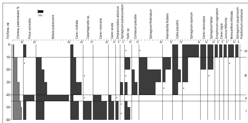
Рис. 2. Сквжина 8. Стратиграфия торфяной залежи, угленосный прослой (40-45 см)
