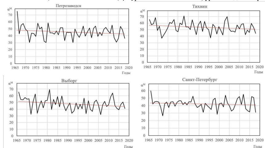
Рис. 1. Хронологические графики индексов Де-Мартона
