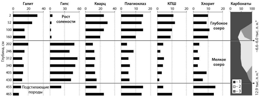
Рис. 2. Вертикальные профили распределения минеральных компонентов (%) в донных отложениях: 1 – кальцит, 2 – низко-Са-магнезит, 3 – арагонит. * – калиброванные даты (по Rudaya et al., 2020). Жирными линиями показаны участок донных отложений с резкой сменой распределения минеральных компонентов и подстилающие породы
