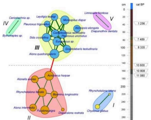
Рис. 2. Граф положительно ассоциированных видов Cladocera. Размер маркера узлов логарифмически пропорционален встречаемости вида в колонке, толщина ребра пропорциональна силе связи между видами. Положение видов относительно шкалы глубин условное
