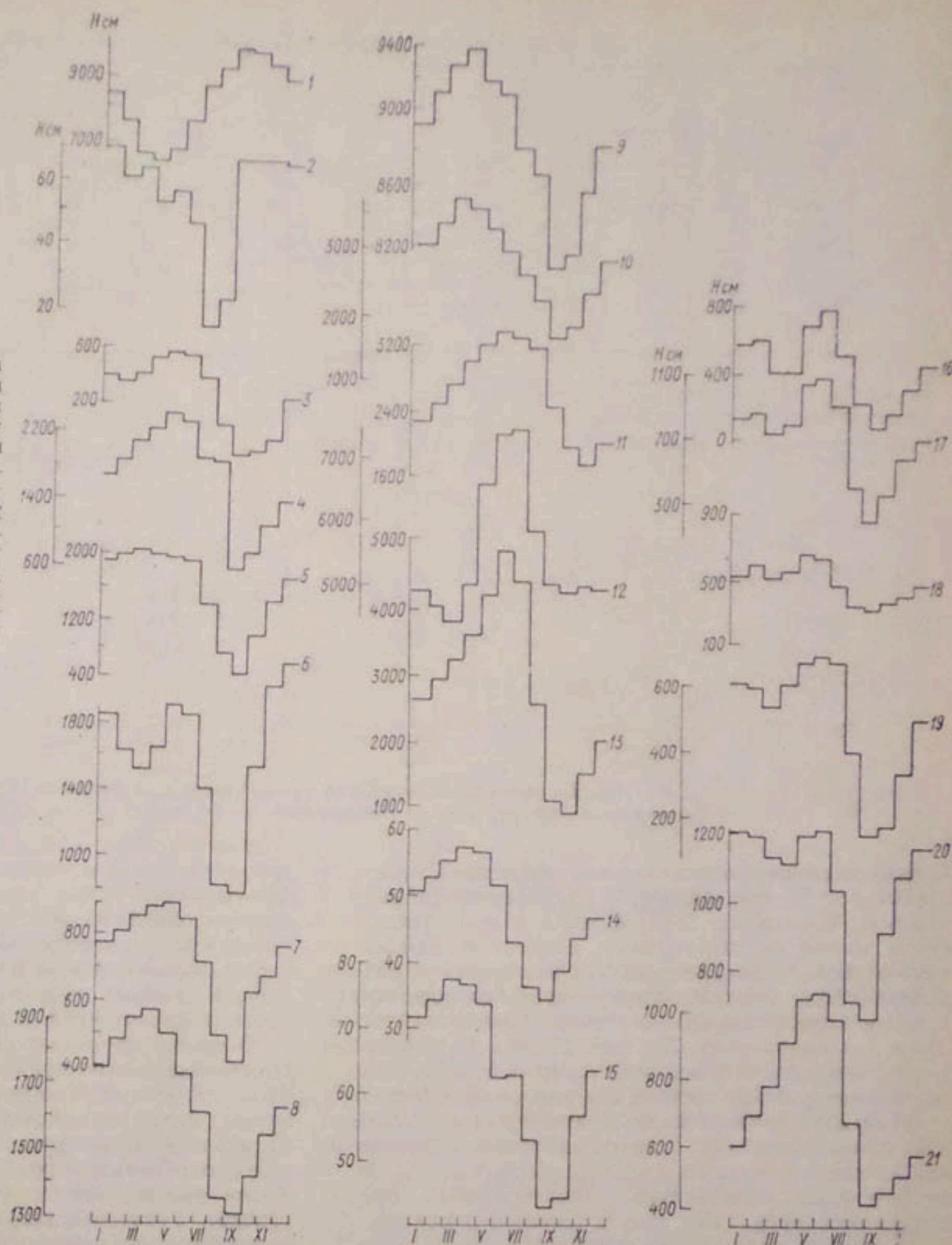
Рис. 3.1. Внутригодовой ход уровня воды водохранилищ (Н) бассейнов рек Амударьи (1—6), Сырдарьи (7—13), Чу и Талас (14, 15) и Туркмении (16—21). Водохранилище: 1 — Нурекское, 2 — Головной ГЭС, 3 — Учкызылское, 4 — Чимкуртанское, 5 — Каттакуртанское, 6 — Куюмаларское, 7 — Кайраккумское, 8 — Чардаринское, 9 — Найманское, 10 — Папанское, 11 — Тунбугузское, 12 — Чарвакское, 13 — Уртатокайское, 14 — Ортатокайское, 15 — Кировское, 16 — Ташкепринское, 17 — Сары-Ямское, 18 — Колхозбеатское, 19 — Илолганское, 20 — Хауз-Ханское, 21 — Тедженское II.
