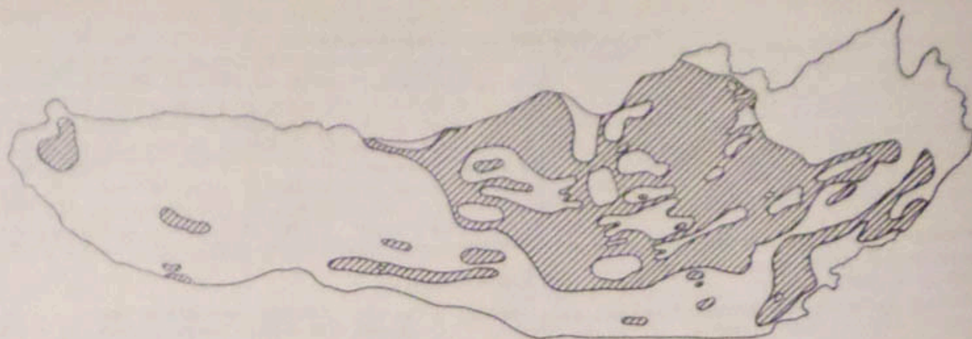
Рис. 9.3. Схема просядок грунта Кайраккумского водохранилища. Штриховкой выделена зона просядок.
