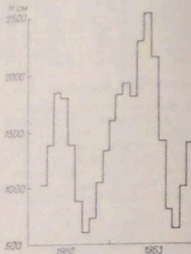
Рис. 3.5. График наполнения Чимкурганского водохранилища.
