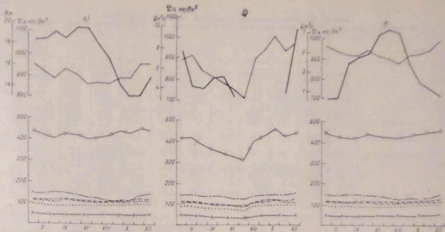
Рис. 10.4. Средневзвешенное содержание ионов и минерализация воды Учкызылского водохранилища (а), канала Заг (б) и нижнего бьефа водохранилища (в). Усл. обозначения см. на рис. 10.3.
