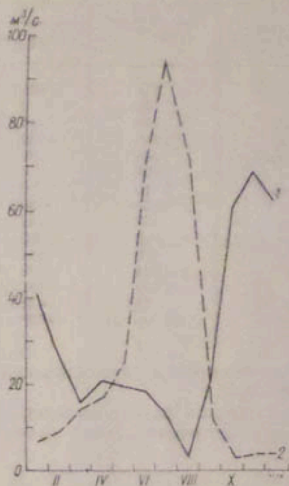
Рис. 11.4. Внутригодовое перераспределение стока. Каттакурганское водохранилище. 1 — приток, 2 — отток.
