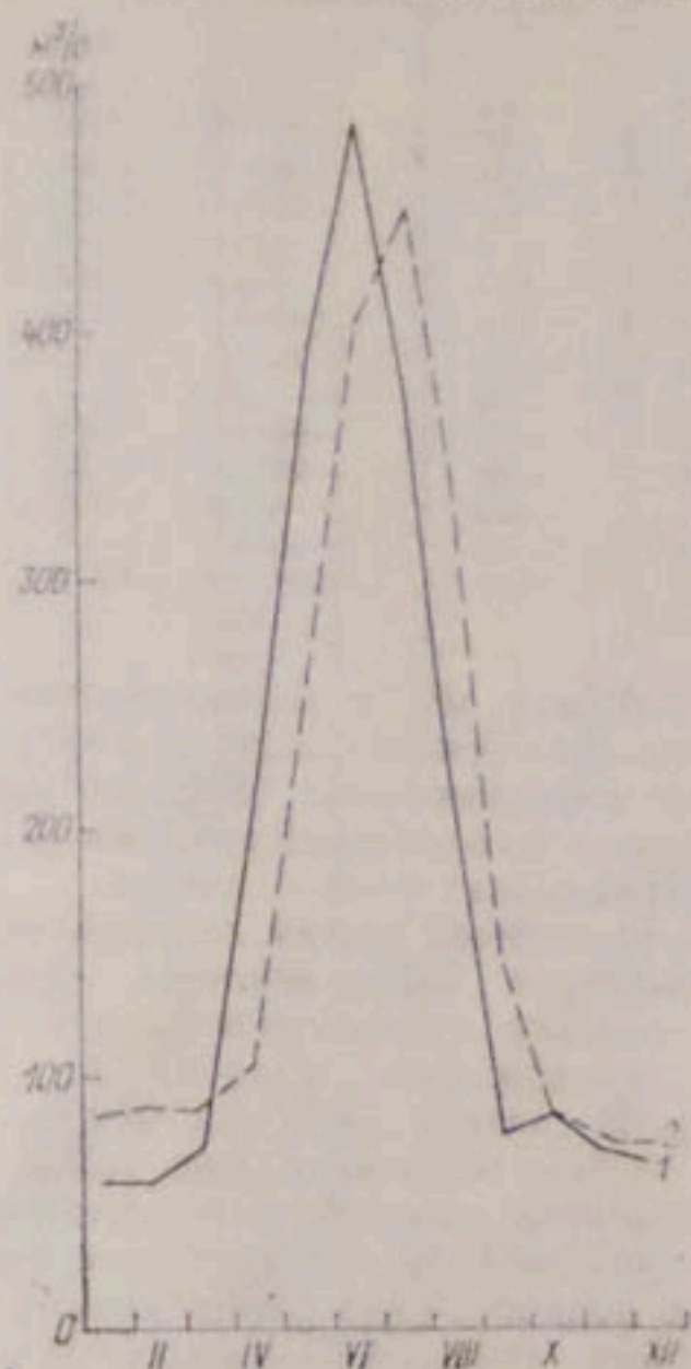
Рис. 11.3. Внутригодовое перераспределение стока. Чарвакское водохранилище. 1 — приток, 2 — отток.
