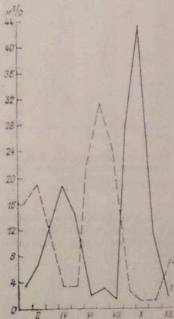
Рис. 11.5. Внутригодовое перераспределение стока. Куюмазарское водохранилище. 1 — приток, 2 — отток.
