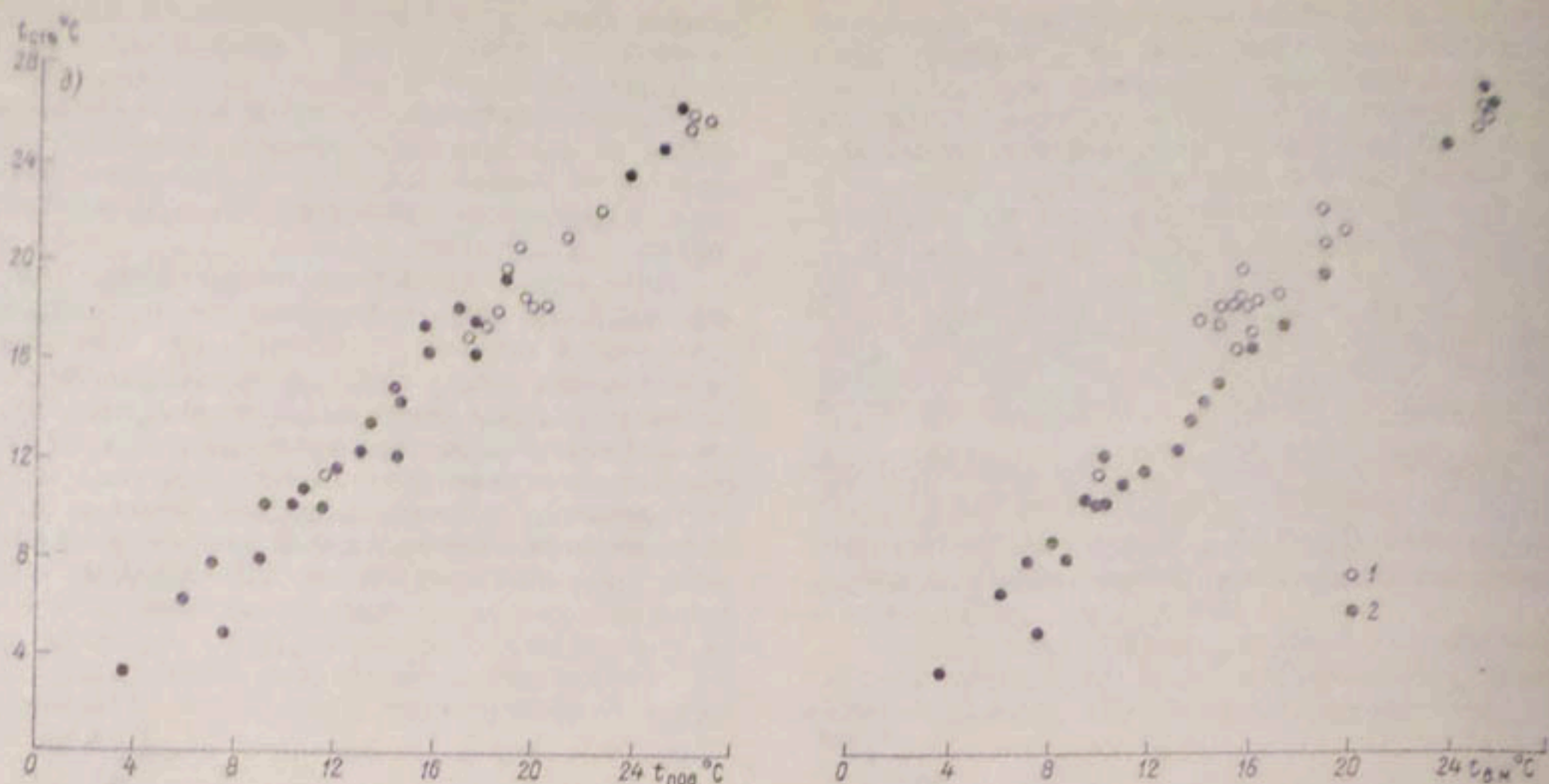
Рис. 5.7. Зависимости температуры поверхности воды (1) ( t_{\text{поверх}} ) и водной (2) ( t_{\text{в}} ) в водохранилищах: а — Чимкурганское, б — Каттакурганское, в — Куюмазарское.
