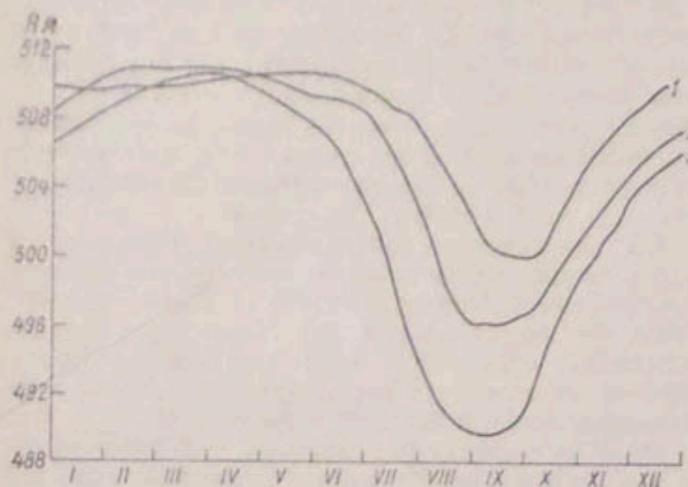
Рис. 3.9. Ход уровня Каттакурганского водохранилища за характерные годы. Годы: 1 — многоводный, 2 — средний, 3 — маловодный.
