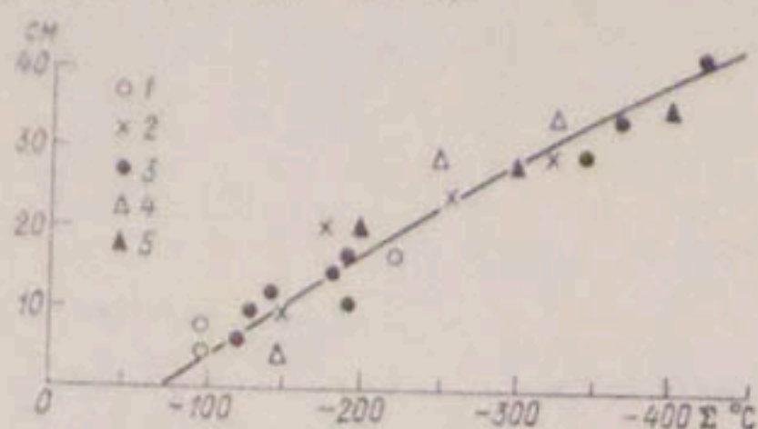
Рис. 6.7. Зависимости толщины льда (см) от сумм отрицательных температур воздуха для водохранилищ Средней Азии. Водохранилища: 1—Каттакурганское, 2—Чардаринское, 3—Туймукское, 4—Бугуньское, 5—оз. Балхаш.
