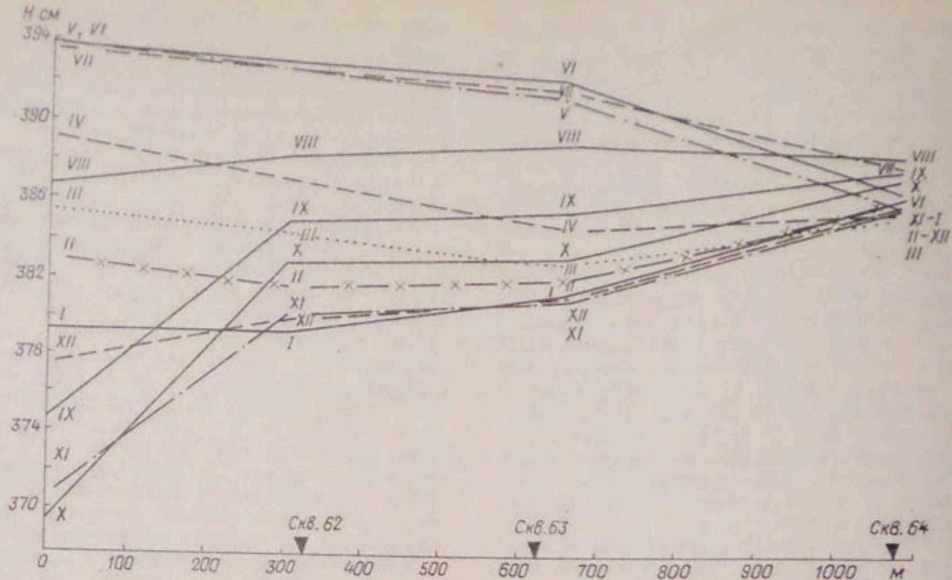
Рис. 4.4. Внутригодовой ход уровня воды в водохранилище и скважинах гидрологического разреза левого берега Туябугузского водохранилища. I—XII — месяцы.
