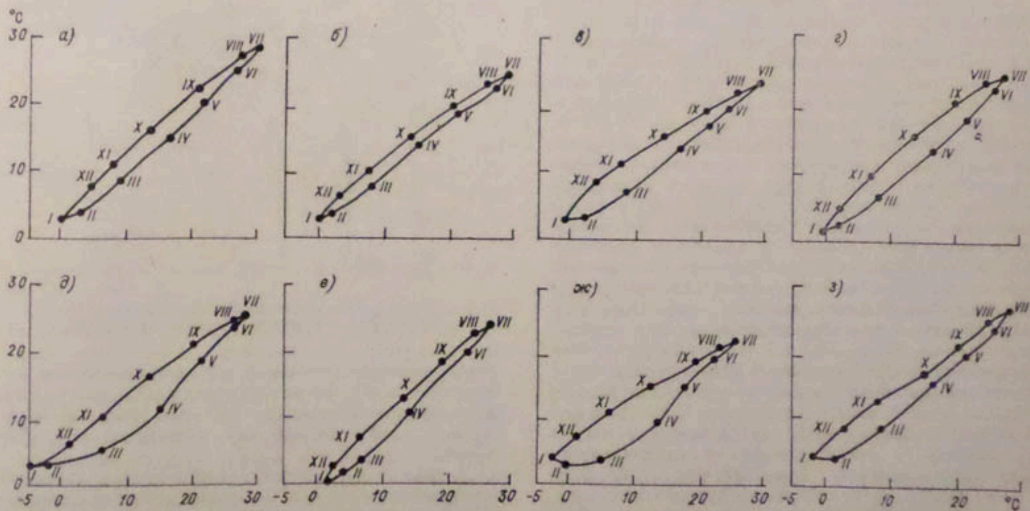
Рис. 5.4. Зависимости температуры поверхности воды (вертикальная шкала) от температуры воздуха (горизонтальная шкала). Водохранилище: а — Каттакурганское, б — Каттакурганское, в — Кукмазарское, г — Кайраккумское, д — Чардаринское, е — Уртатокайское, ж — Чарвакское, з — Туябугузское.
