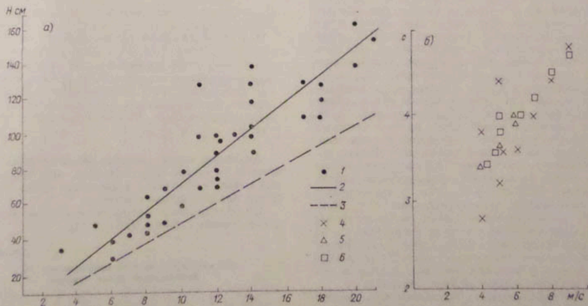
Рис. 7.7. Зависимость высоты волн (см) (а) и ее периода (с) (б) от скорости ветра (м/с) для Каттакурганского водохранилища.
