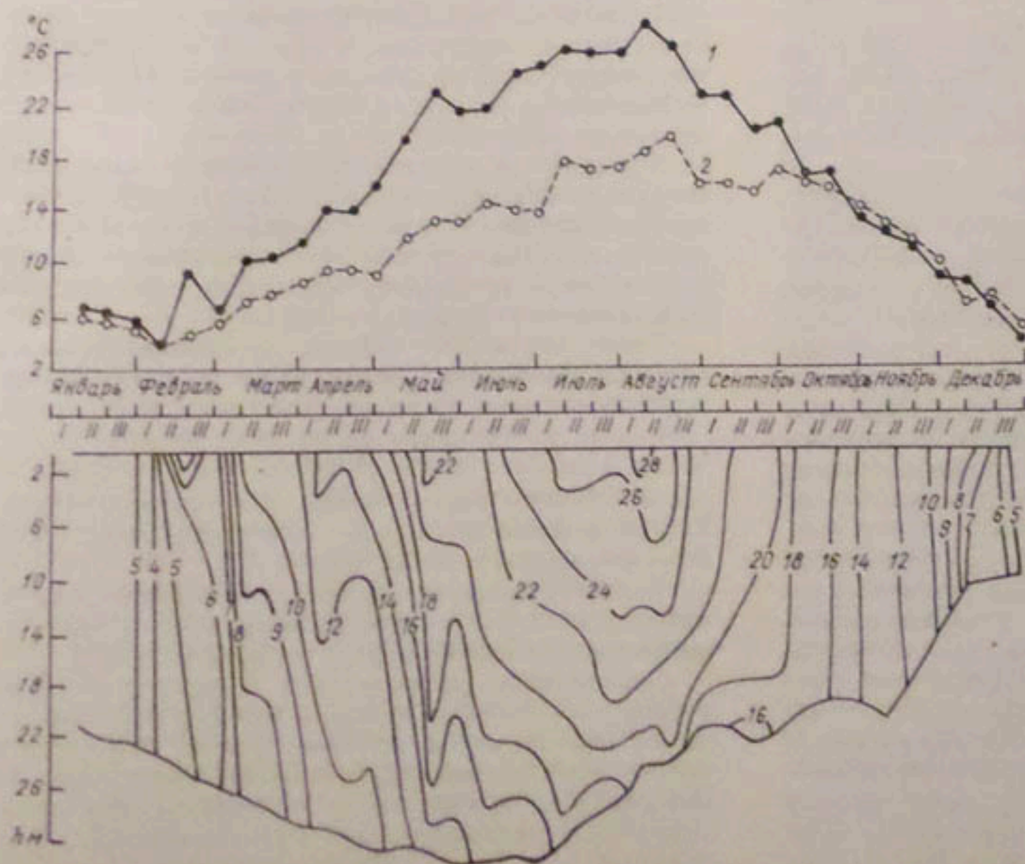
Рис. 5.12. Термоизоплеты на рейдовой вертикали Туябугузского водохрани- ща. 1 — поверхность, 2 — дно.
