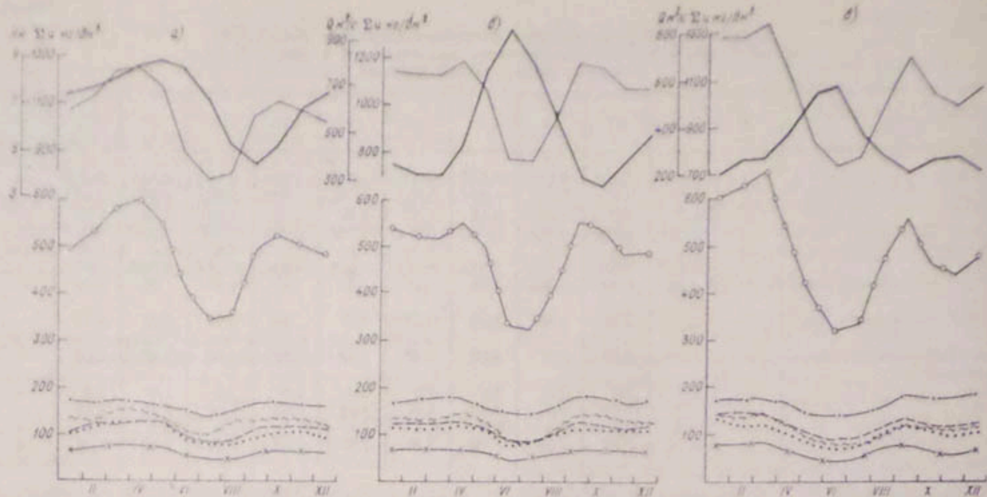
Рис. 10.8. Средневзвешенное содержание ионов и минерализация воды Кайраккумского водохранилища (а), р. Сырдарьи у поста Кызылкишлак (б), р. Сырдарьи у поста Чильмахрам (в). Усл. обозначения см. на рис. 10.3.
