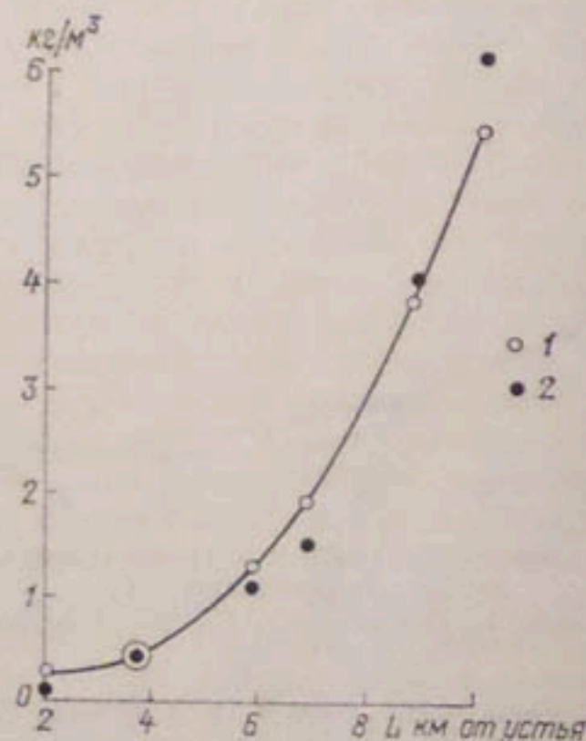
Рис. 9.8. Изменение мутности ( \text{кг/м}^3 ) по длине реки ( L ) в оголившейся зоне Чимкурганского водохранилища по съемке 1981 г.
