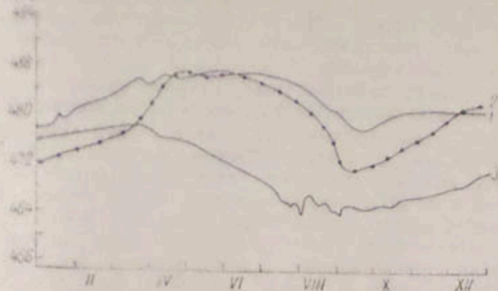
Рис. 3.6. Ход уровня воды Чимкурганского водохранилища за характерные годы.
