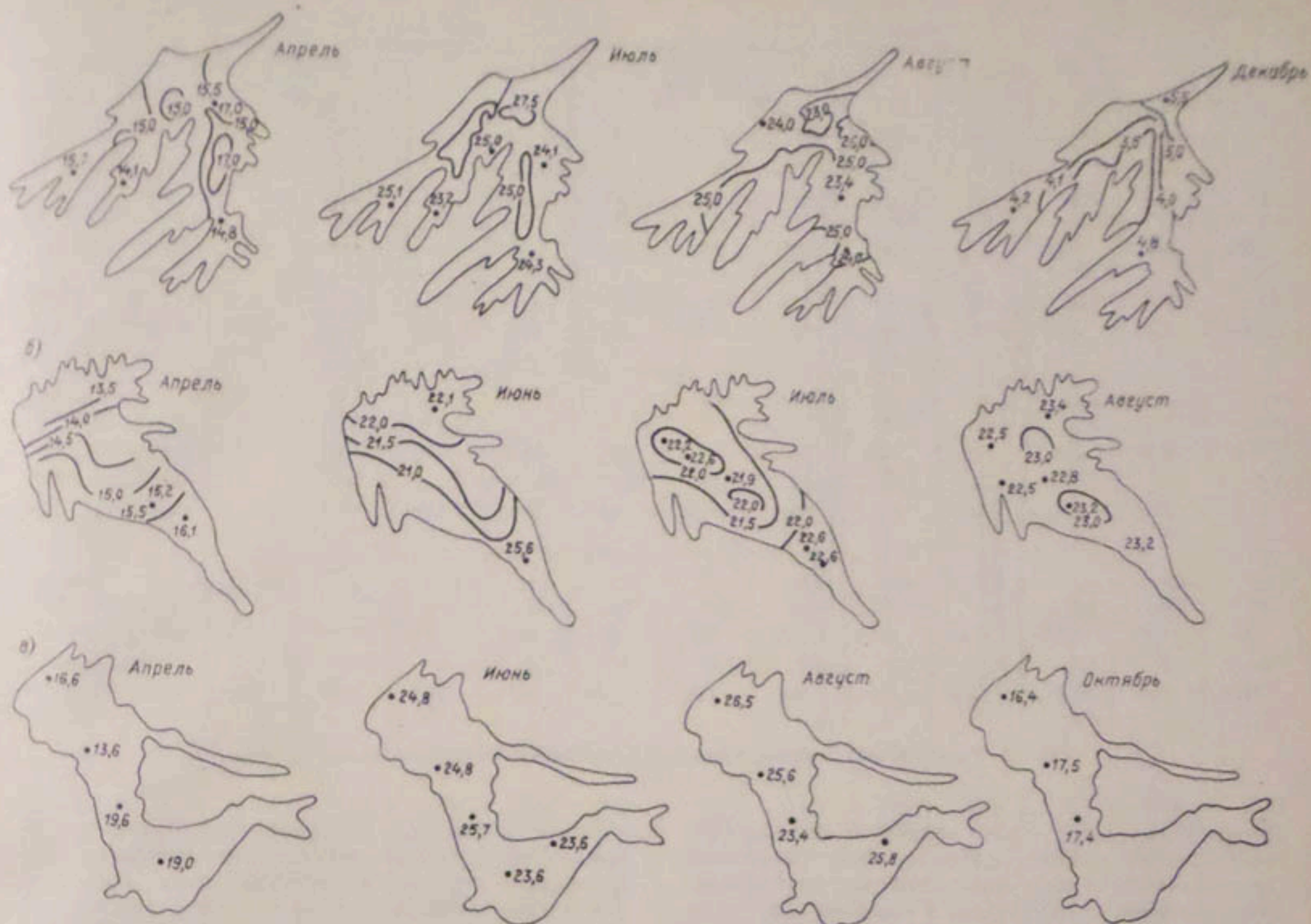
Рис. 5.3. Изменение температуры воды ( ^{\circ}\text{C} ) по сезонам года на поверхности водохранилищ. Водохранилище: а — Каттакурганское, б — Уртатокайское, в — Туябугузское.
