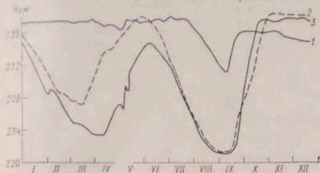
Рис. 3.12. Ход уровня воды Куюмазарского водохранилища за характерные годы.
