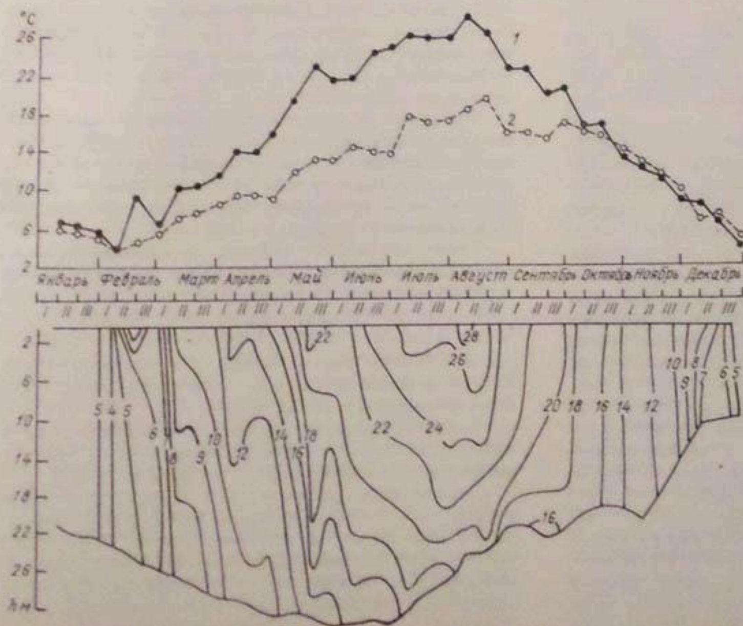
Рис. 5.12. Термоизоплеты на рейдовой вертикали Тузбугузского водохрани- ща. 1 — поверхность, 2 — дно.
