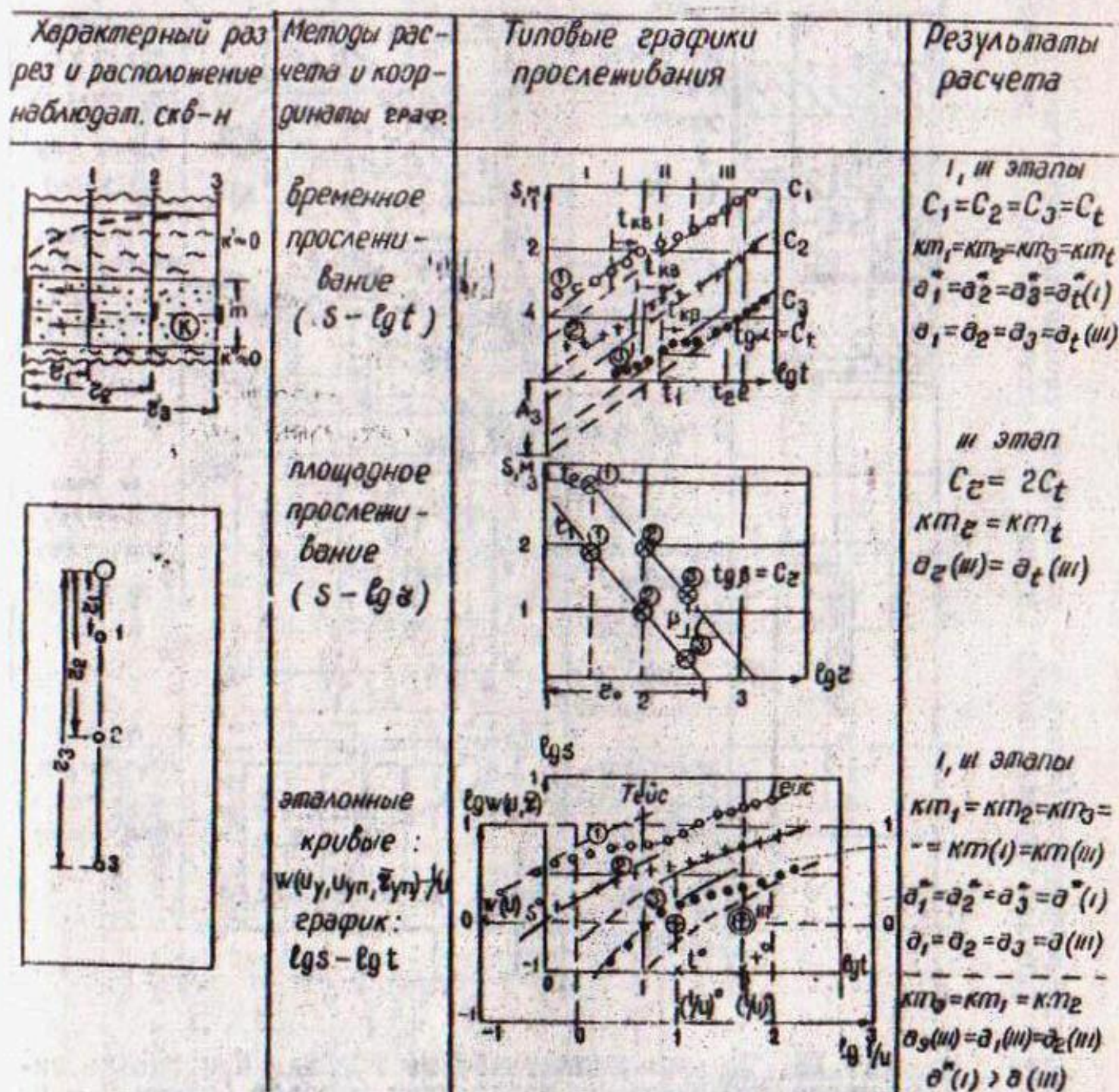
Рис. 17. Типовые аналитические графики при оценке параметров рациональным комплексом методов (схема 16 - потенциально-напорный водоносный пласт).
