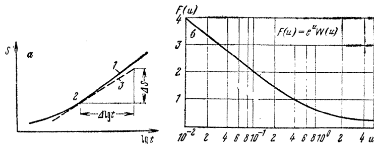
Рис. 28. Обработка графиков временного прослеживания по способу В. Т. Чоу:
