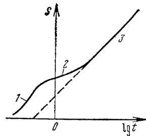
Рис. 39. Индикаторный график откачки из скважины, вскрывающей слоистый пласт (1, 2, 3 — характерные участки графика)
