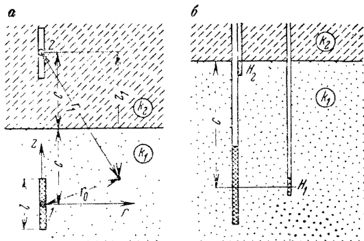
Рис. 65. Несовершенная скважина вблизи границы областей (слоев) различной проницаемости:
