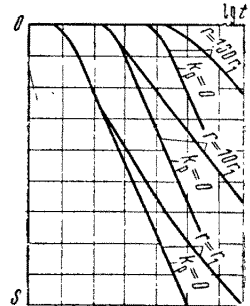
Рис. 31. Характерные индикаторные графики откачки при наличии подтока из слабопроницаемого слоя
