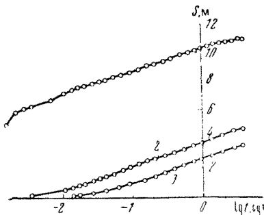
Рис. 74. Индикаторные графики откачки по центральной (1) и наблюдательным (2; 3) скважинам (схема куста дана на рис. 40, а)
