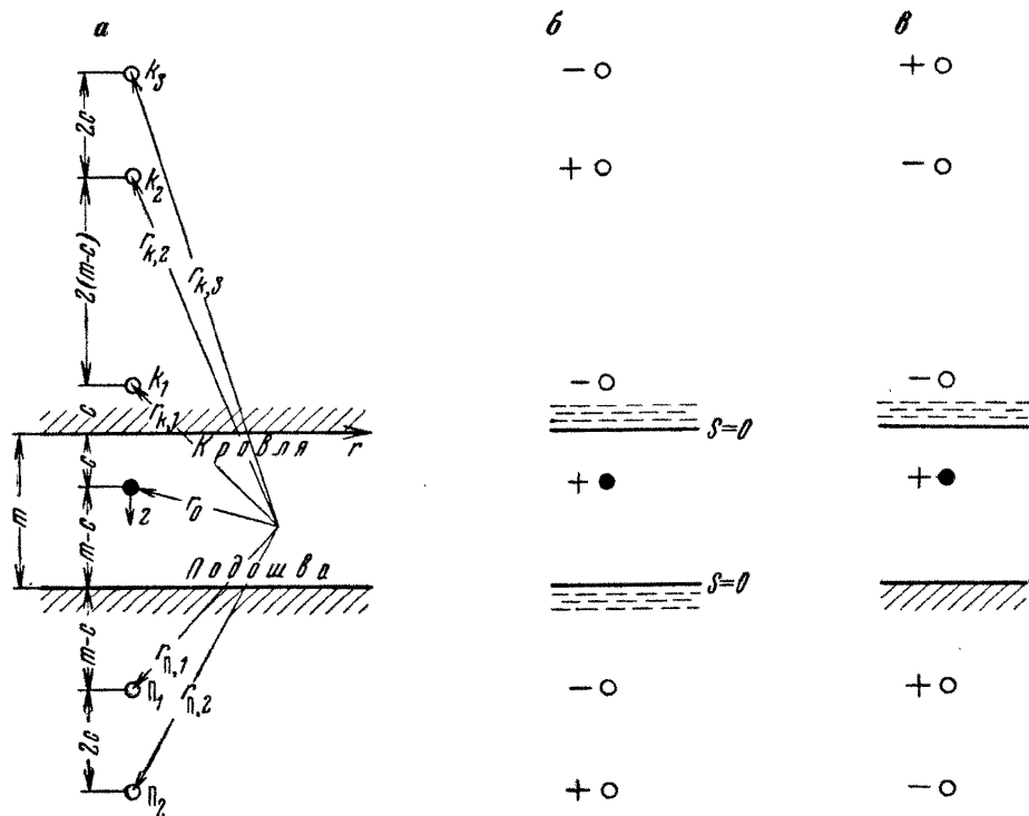
Рис. 60. Построение отраженных точечных источников-стоков в однородном пласте ограниченной мощности (а, б и в) при различных условиях на подошве и кровле пласта
