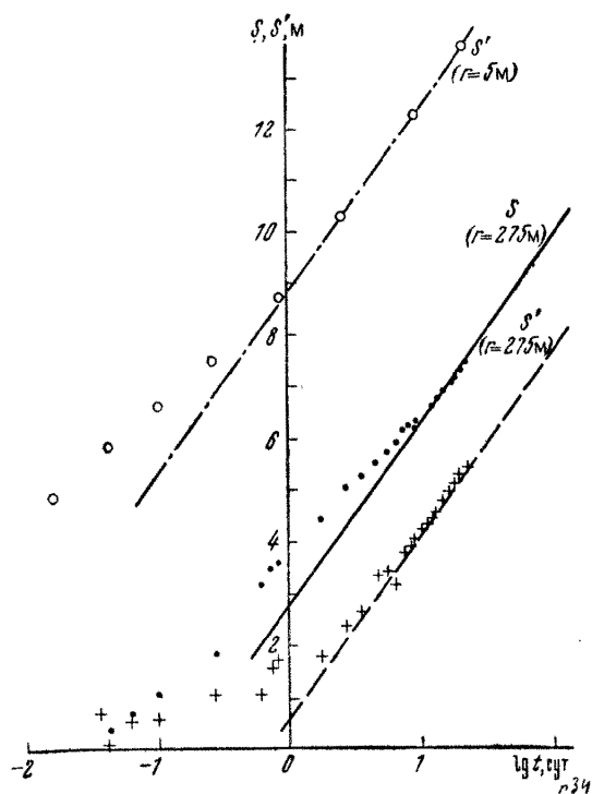
Рис. 34. Индикаторные графики откачки из напорного пласта.
