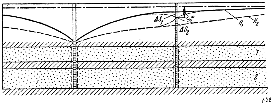
Рис. 22. Схема двухпластовой системы: 1 и 2 — верхний и нижний пласты
