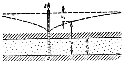
Рис. 9. Схема однородного напорного пласта
