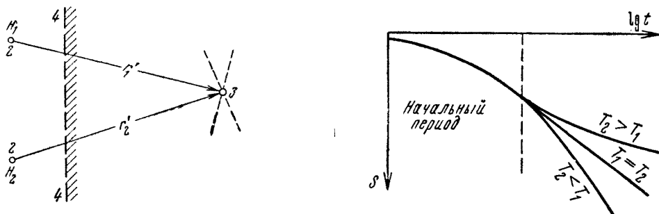
Рис. 44. Построение непроницаемой границы по данным временного прослеживания:
