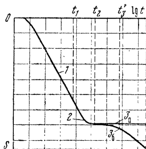
Рис. 30. Типовые индикаторные графики откачки при наличии перетекания
