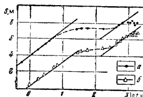
Рис. 43. Индикаторные графики откачки из пласта закарстованных известняков (по А. Ф. Потемкиной):
