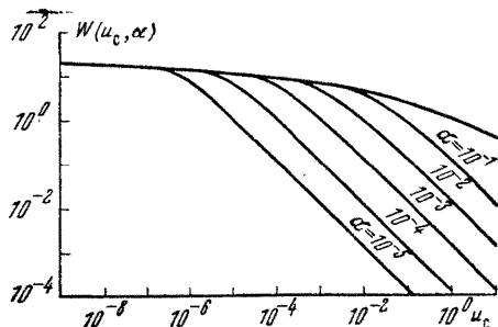
Рис. 69. График функции W(u_c, \alpha)
