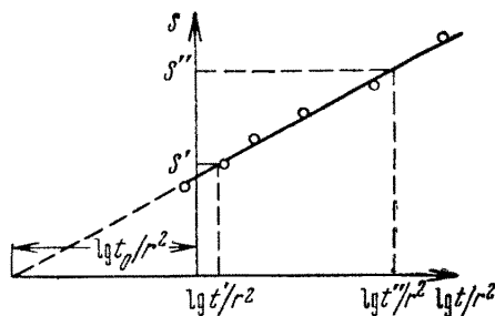
Рис. 27. Полулогарифмический график прослеживания уровня для обработки по способу прямой Джейкоба
