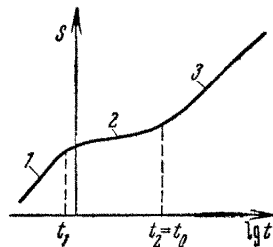
Рис. 42. Типовой индикаторный график откачки из пласта пород с двойной емкостью (1, 2, 3 — характерные участки графика)
