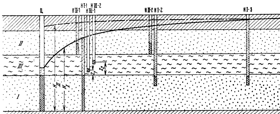
Рис. 38. Схема опытного куста при опробовании взаимодействующих пластов:
