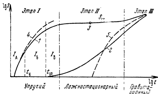
Рис. 49. Кривые понижения уровня при откачке в двухслойном пласте:
