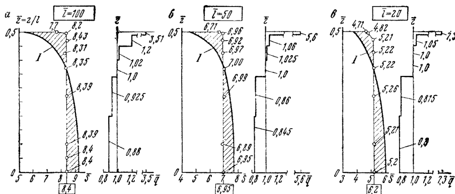
Рис. 56. Эпюры безразмерных понижений \bar{S} = 4\pi k l S_c / Q и безразмерных удельных притоков \bar{q} = q_l / Q по длине скважины: а — при l/r_c = 100 ; б — при l/r_c = 50 ; в — при l/r_c = 20
