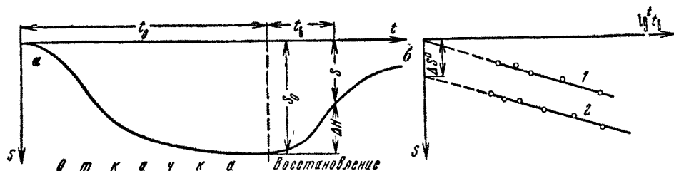
Рис. 29. Графики восстановления уровня после откачки:
