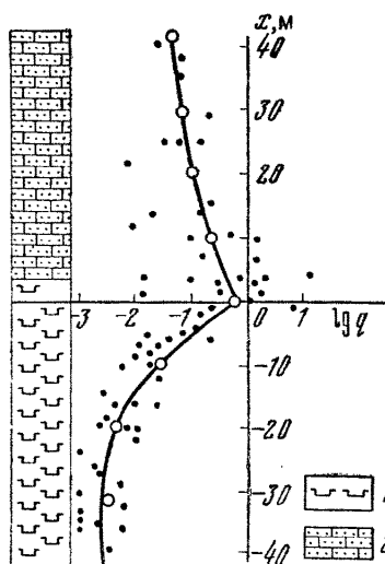
Рис. 4. Распределение логарифмов удельных поглощений q ( \text{м}^2/\text{сут} ) в траппах (1) и вмещающих породах (2) вблизи их контакта (по С. Н. Чернышеву)
