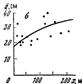
Рис. 5. Изменение средних расстояний ( \bar{x} ) между соседними трещинами по мере удаления ( x ) от тектонического разрыва (по М. В. Рацу): а — в гранитах; б — в песчаниках
