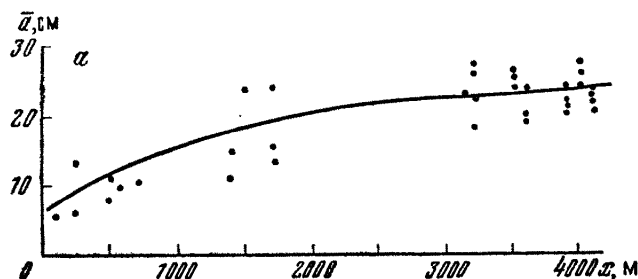
Рис. 5. Изменение средних расстояний ( \bar{x} ) между соседними трещинами по мере удаления ( x ) от тектонического разрыва (по М. В. Рацу): а — в гранитах; б — в песчаниках
