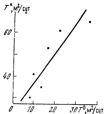
Рис. 76. Сопоставление значений проводимости, полученных по одиночным ( T^o ) и кустовым ( T^k ) откачкам
