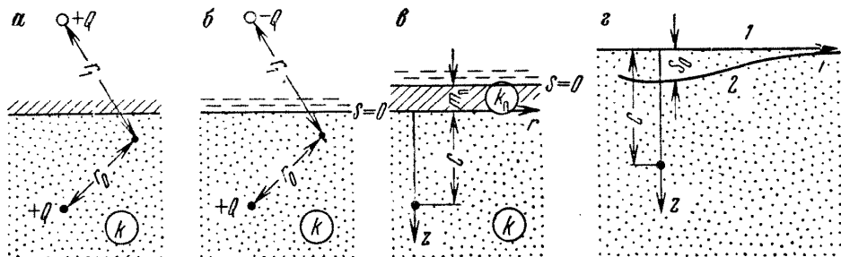
Рис. 59. Схема расположения источников-стоков:
