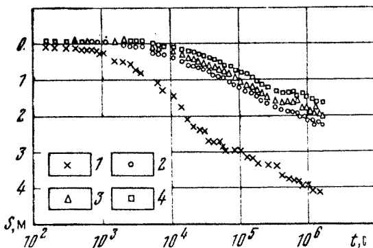
Рис. 37. Графики понижения напоров по пьезометрам основного пласта (1) и в толще слабопроницаемых пород при z = 0,5 м (2), z = 1,46 м (3) и z = 2,56 м (4)
