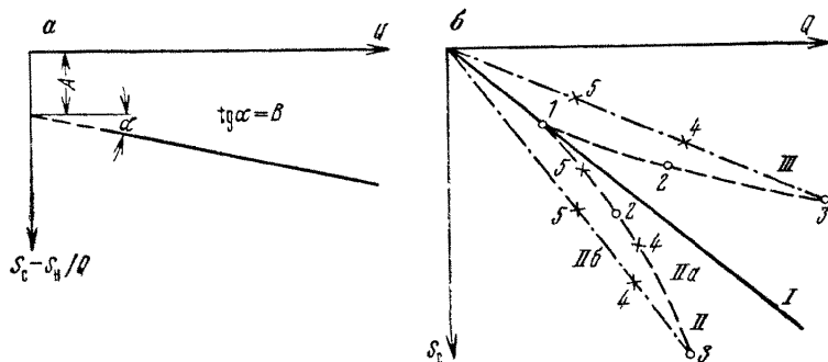
Рис. 68. Индикаторные графики зависимости понижения в скважине от расхода опробования:
