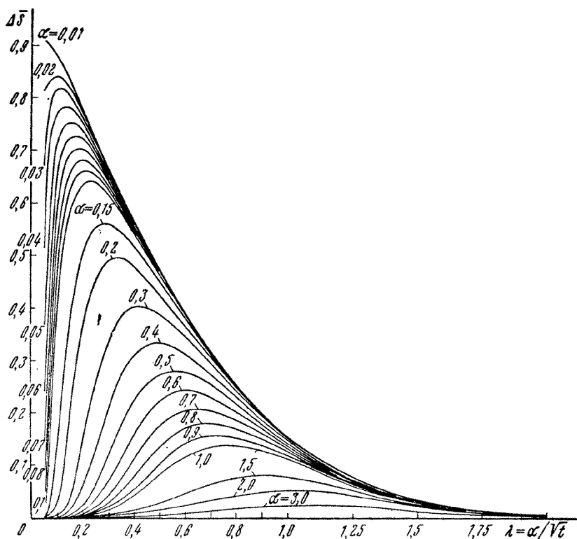
Рис. 73. График для относительной разницы уровней за счет инерционности пьезометра при откачке из несовершенной скважины в неограниченном пласте (по данным расчетов Г. С. Туманской)
