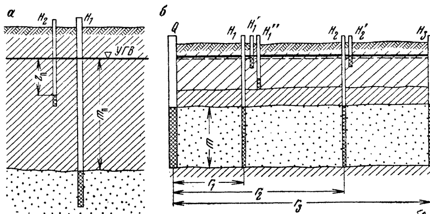
Рис. 50. Расположение наблюдательных скважин при откачке в двухслойном пласте:
