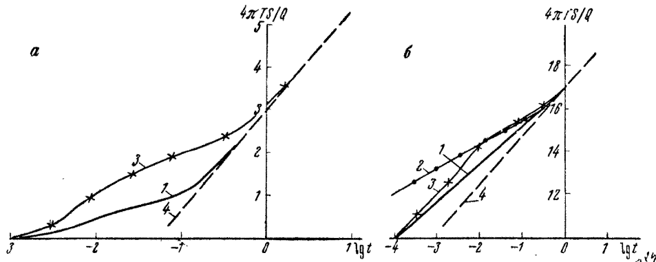
Рис. 24. Расчетные графики приведенного понижения для пласта гетерогенных пород:
