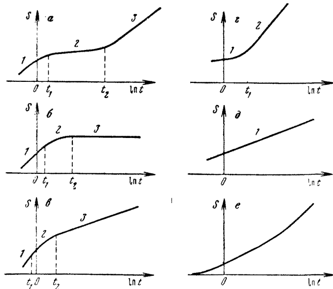
Рис. 48. Типовые формы временных графиков прослеживания для кустовых откачек
