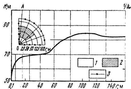
Рис. 19. Аномальная форма депрессионной кривой (планово-неоднородный пласт):
