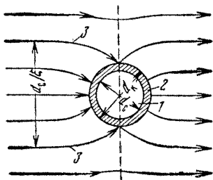
Рис. 72. Поток вблизи наблюдательной скважины при наличии прискважинной зоны:
