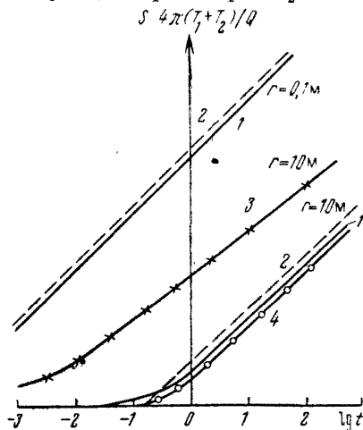
Рис. 23. Расчетные графики приведенных понижений для двухпластовой системы:
