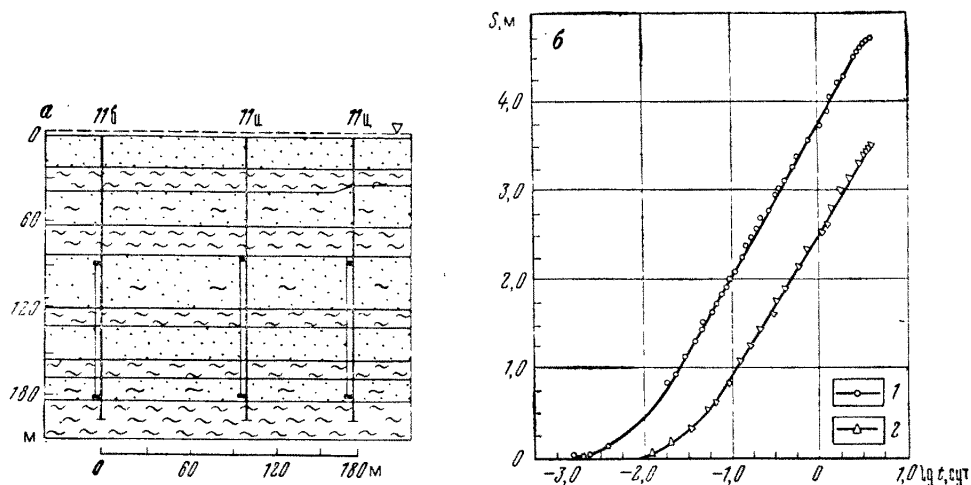
Рис. 40. Схема и индикаторные графики откачки из слоистого пласта (по В. В. Антонову): а — схема расположения скважин; б — индикаторные графики для наблюдательных скважин: (1 — для 11а, 2 — для 11б)
