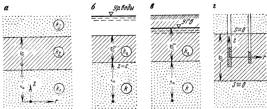
Рис. 66. Несовершенные скважины вблизи или внутри слабопроницаемых слоев:
