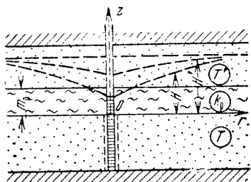
Рис. 10. Схема взаимодействия пластов
