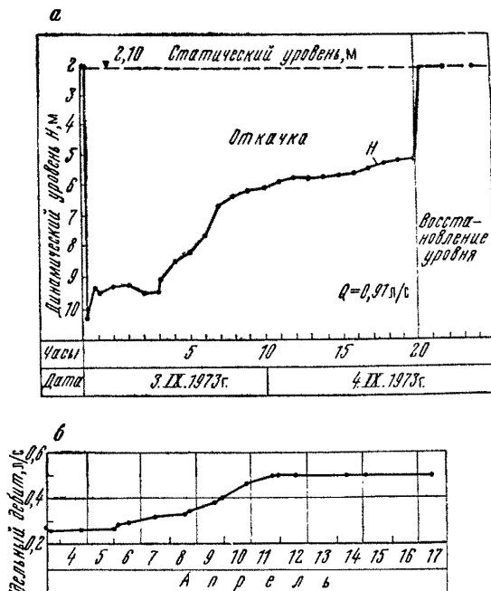
Рис. 67. Примеры откачек с переменным во времени удельным дебитом:
