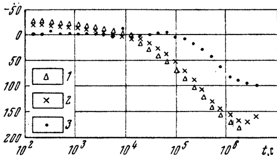
Рис. 36. Графики понижения напоров в слабопроницаемом слое:
