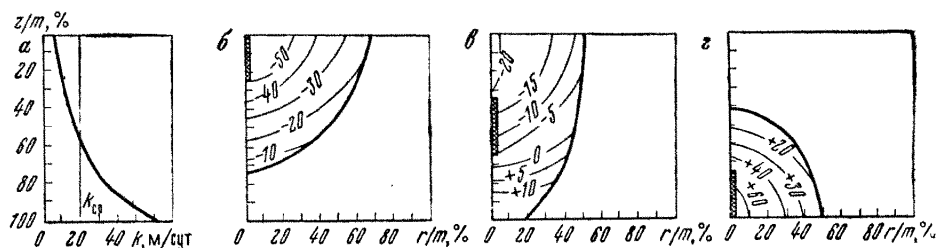
Рис. 62. Результаты моделирования откачки из несовершенной скважины в профильно-неоднородном пласте:
