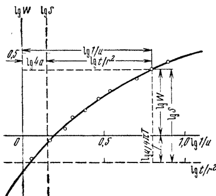
Рис. 26. Совмещение опытных точек для прослеживания уровня с эталонной кривой (кружочками показаны опытные точки, а сплошной линией — эталонная кривая)
