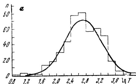
Рис. 7. Гистограммы распределения логарифмов водопроницаемости пород (м 2 /сут): а — мячковско-подольский водоносный горизонт Московского артезианского бассейна; б — московско-днепровские флювиогляциальные отложения
