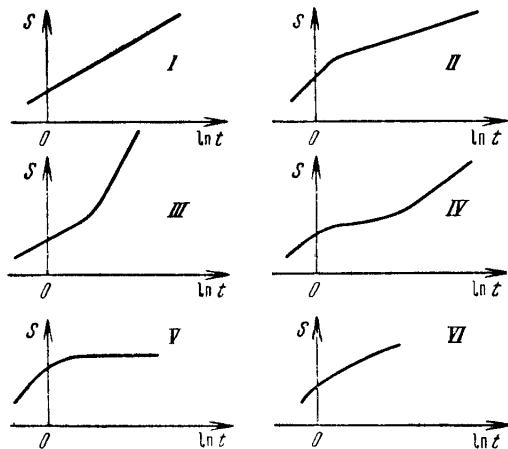
Рис. 70. Характерные графики временного прослеживания уровня в центральной скважине
