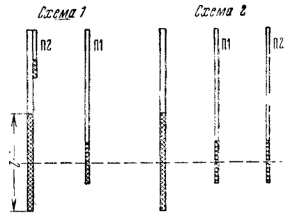
Рис. 64. Схемы расположения наблюдательных скважин при откачке из не совершенной скважины в анизотропном пласте
