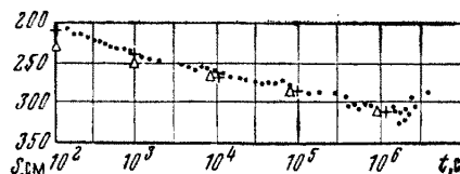
Рис. 35. График понижения напоров в основном пласте:
