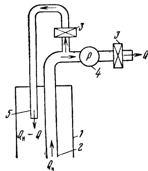
Рис. 15. Схема откачки с обратным сбросом:
