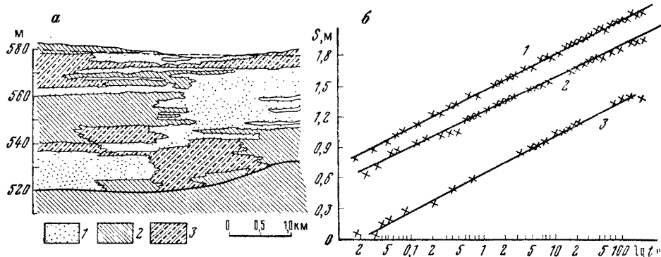
Рис. 41. Пример откачки из слоистого пласта (по В. А. Манукяну): а — схематический геологический разрез (1 — пески, 2 — глины, 3 — суглинки); б — индикаторные графики наблюдательных скважин: r_1 = 1,6 \text{ м} (1), r_2 = 10 \text{ м} (2) и r_3 = 92 \text{ м} (3)
