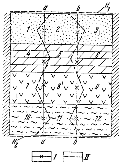
Рис. 81. Схема разбивки расчетной модели по Ш. Ньюману [24]:
