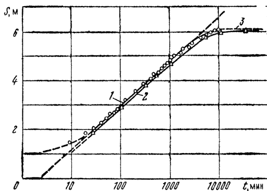
Рис. 33. Индикаторные графики откачки из напорного пласта при наличии перетекания:
