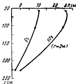
Рис. 32. График изменения напора ( \Delta H ) в пределах глинистого пласта на начальном этапе откачки ( z — расстояние от контакта пласта с водоносным горизонтом)
