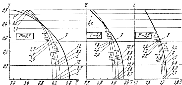
Рис. 57. Эпюры безразмерных понижений \bar{S} = 4\pi k l S_c / Q при действии неограниченного скважины в неограниченном пласте:
