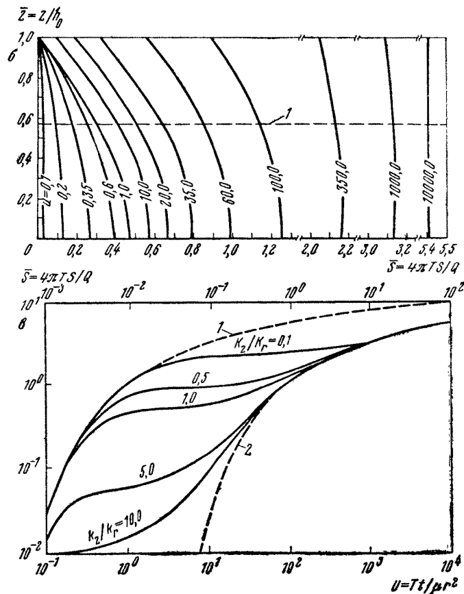
Рис. 52. Графики относительных понижений в безнапорном потоке (по Ш. Ньюману [22]):
