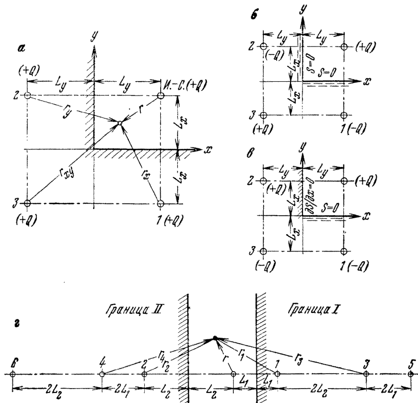
Рис. 13. Схема отражений источника-стока в угловом (а, б, в) и в полосовом пласте (г)
