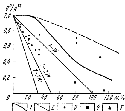
Рис. 79. Зависимость отношения Q^n/Q^{cp} от коэффициента вариации гидрогеологических параметров по области фильтрации:
