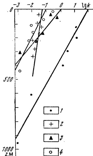
Рис. 6. Изменение коэффициента фильтрации k (м/сут) по глубине в трещиноватых породах (по Н. А. Ярцеву):
