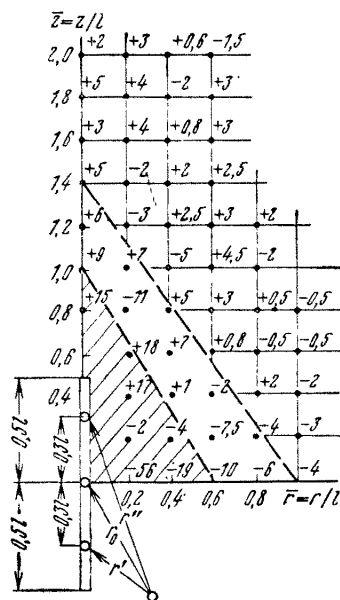
Рис. 58. Распределение относительной разницы понижений \delta_{\text{тл}}\% для линейного и точечного стоков (цифрами показаны значения \delta_{\text{тл}} в точках, косой штриховкой покрыта область с \delta_{\text{тл}} > 10\% , а квадратной сеткой с \delta_{\text{тл}} < 5\% , кружком показана точка, в которой определяется расчетное расстояние r^0 до точечного стока
