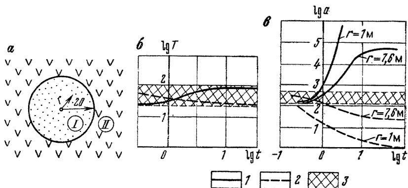
Рис. 46. График изменения расчетных параметров плано-неоднородного пласта, определенных временным прослеживанием:
