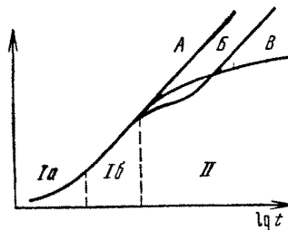
Рис. 25. Типовые кривые прослеживания уровней в неограниченных напорных пластах:
