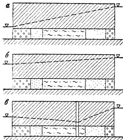
Рис. 82. Схемы моделей плано-неоднородной области фильтрации:
