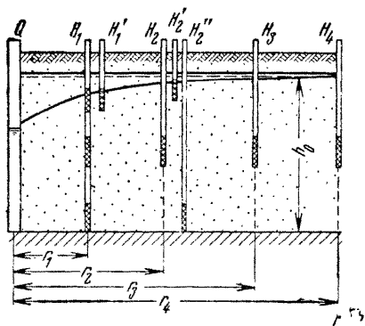
Рис. 53. Рекомендуемая схема расположения наблюдательных скважин в относительно однородном безнапорном потоке
