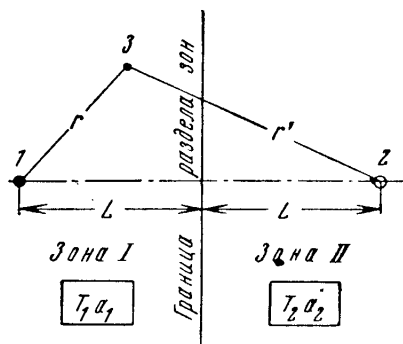
Рис. 18. План расположения скважины у прямолинейной границы зон с различными параметрами (1 и 2 — действующая и отраженная скважины; 3 — расчетная точка)
