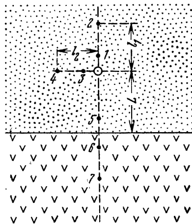
Рис. 47. Схема опытного куста при откачке вблизи границы фильтрационной неоднородности (1—7 — наблюдательные скважины)
