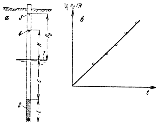
Рис. 71. Схема экспресс-налива в несовершенную скважину:
