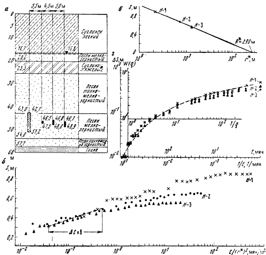
Рис. 63. Данные для примера расчета откачки из несовершенной скважины:
