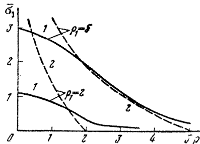
Рис. 20. Графики приведенных давлений: 1 — расчетных; 2 — фактических
