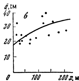
Рис. 5. Изменение средних расстояний ( \bar{x} ) между соседними трещинами по мере удаления ( x ) от тектонического разрыва (по М. В. Рапу): а — в гранитах; б — в песчаниках
