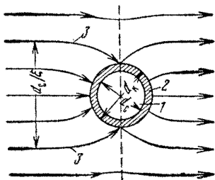
Рис. 72. Поток вблизи наблюдательной скважины при наличии прискважинной зоны:
