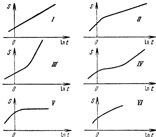
Рис. 70. Характерные графики временного прослеживания уровня в центральной скважине
