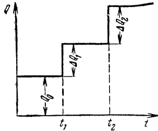
Рис. 12. График переменного расхода источника-стока
