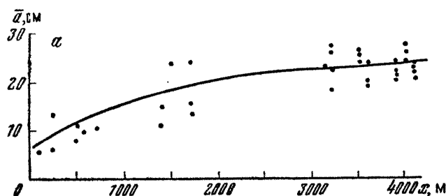
Рис. 5. Изменение средних расстояний ( \bar{x} ) между соседними трещинами по мере удаления ( x ) от тектонического разрыва (по М. В. Рапу): а — в гранитах; б — в песчаниках
