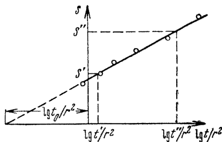
Рис. 27. Полулогарифмический график прослеживания уровня для обработки по способу прямой Джеккоба
