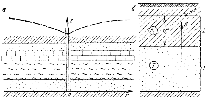
Рис. 11. Схемы слоистых пластов:
