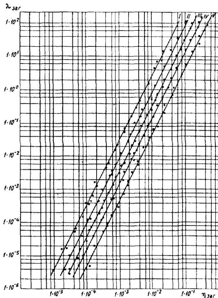
Рис. 3.9. График связи \lambda_{\text{заг}} = f(\eta_{\text{заг}}) .
