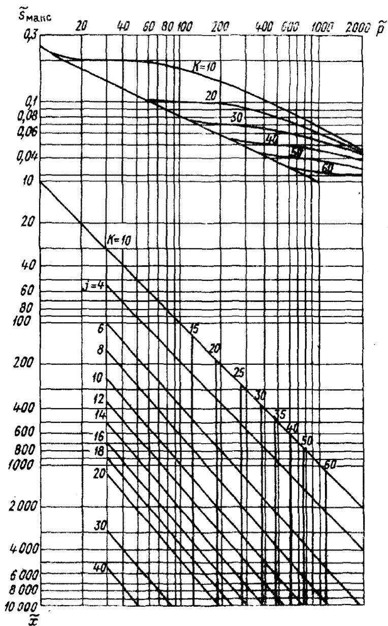
Рис. 4.10. Номограмма \tilde{s}_{\max} = f(j, K, \tilde{x}) .
