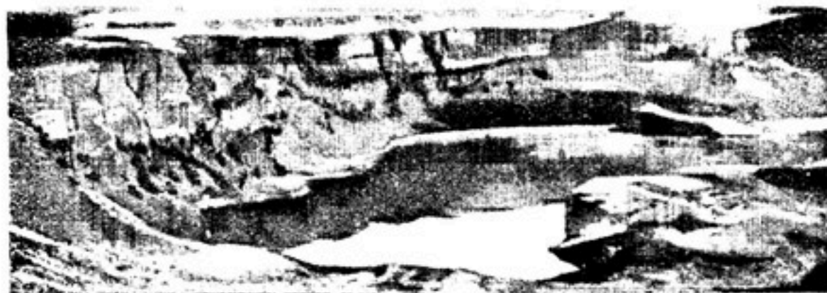
Рис. 71. Базальт Колумбийского плато, обнаруживающий слоистость. Место бывших водопадов реки Колумбии в Гран Кула, 120 м высоты. (По фотогр. А. Т. Швенезена.)
