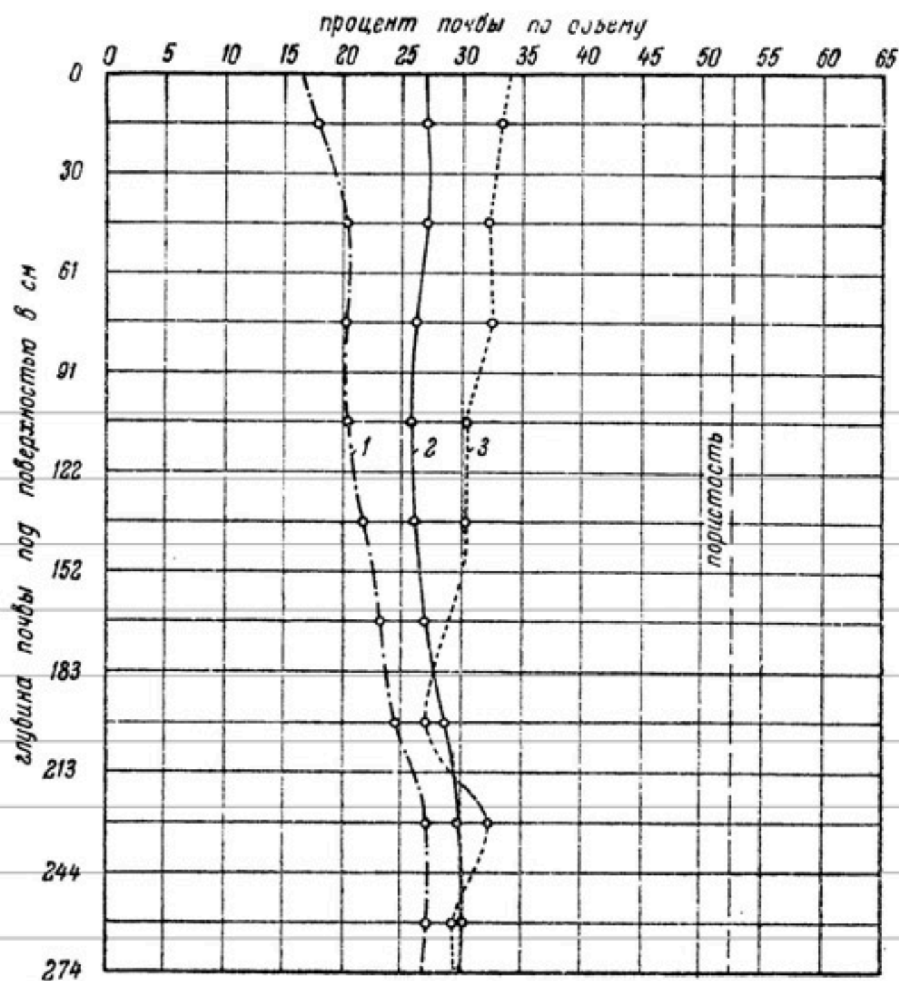
Рис. 22. Диаграмма водоудерживающей способности и водоотдачи в сiltовой суглинистой почве (по О. В. Израэльсену). Каждая кривая содержания воды построена на основании среднего из результатов, полученных из 87 буровых.
