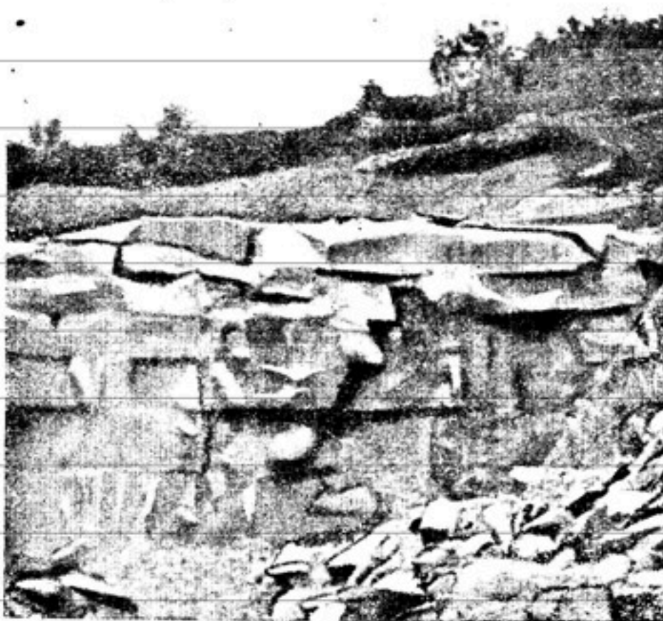
Рис. 43. Плотный слоистый известняк с плоскостями отдельности, по которым просачивается вода. (По фотогр. С. Р. Кэппса.)
