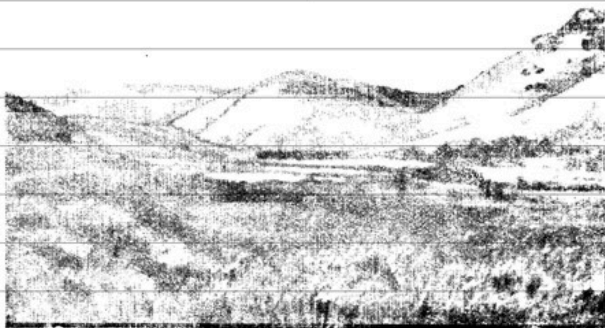
Рис. 116б. Внутренняя часть хребта Тоуаве, Невада. Этот район менее расчленен, так как его еще не захватил эрозионный цикл, обусловленный поднятием хребта. (По фотогр. О. Э. Мейнцера.)
