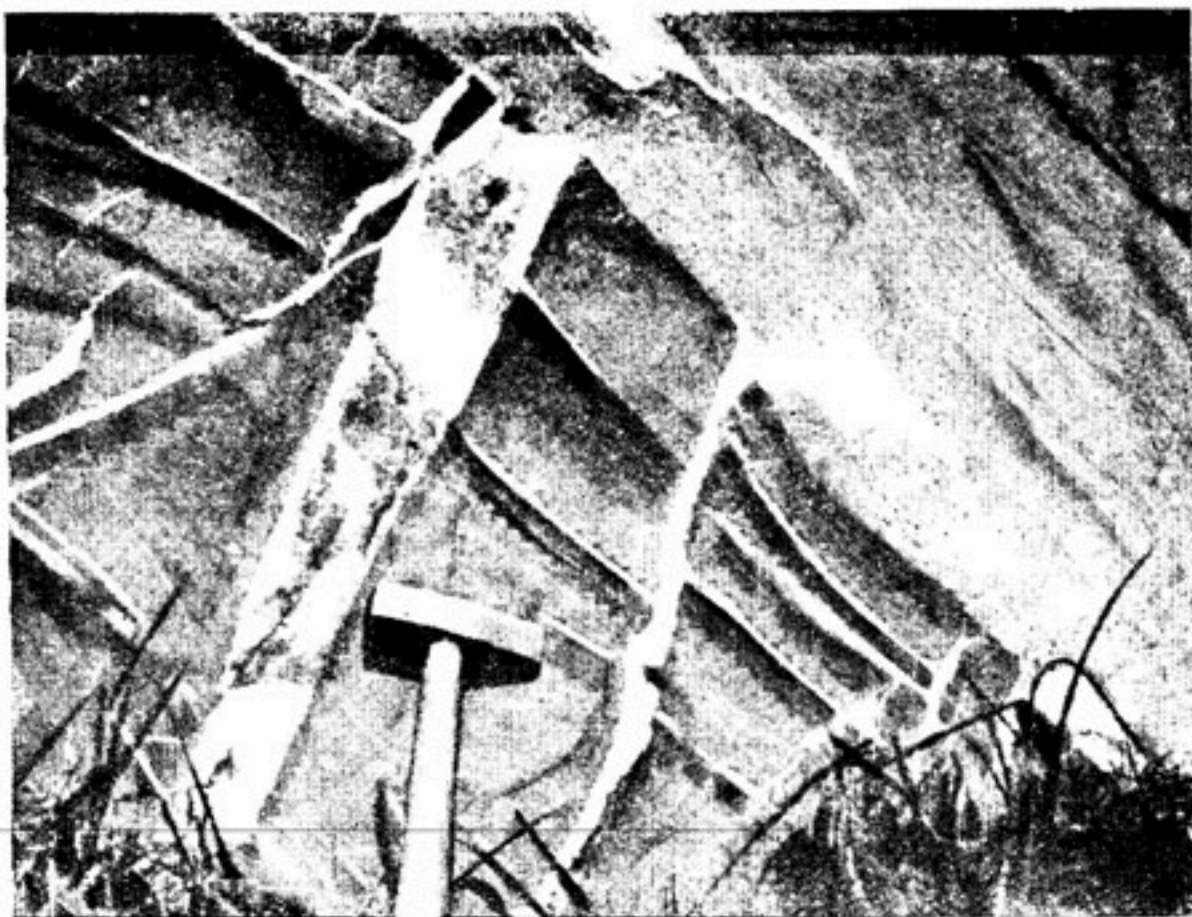
Рис. 120. Небольшие дайки и пластовые жилы в кристаллическом сланце. (По фотогр. Э. Хоув.)
