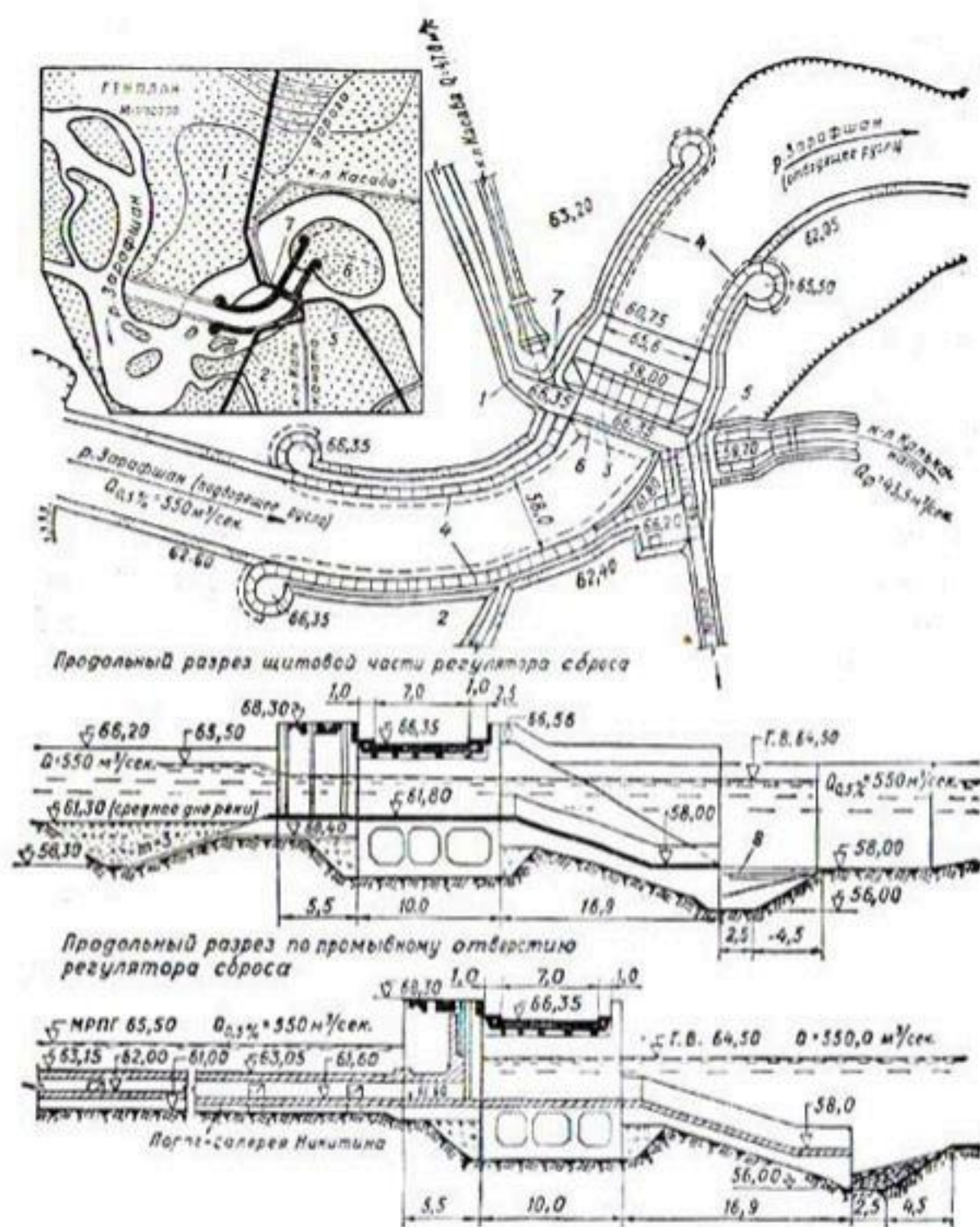
Рис. 5. План Кармининского гидроузла:
