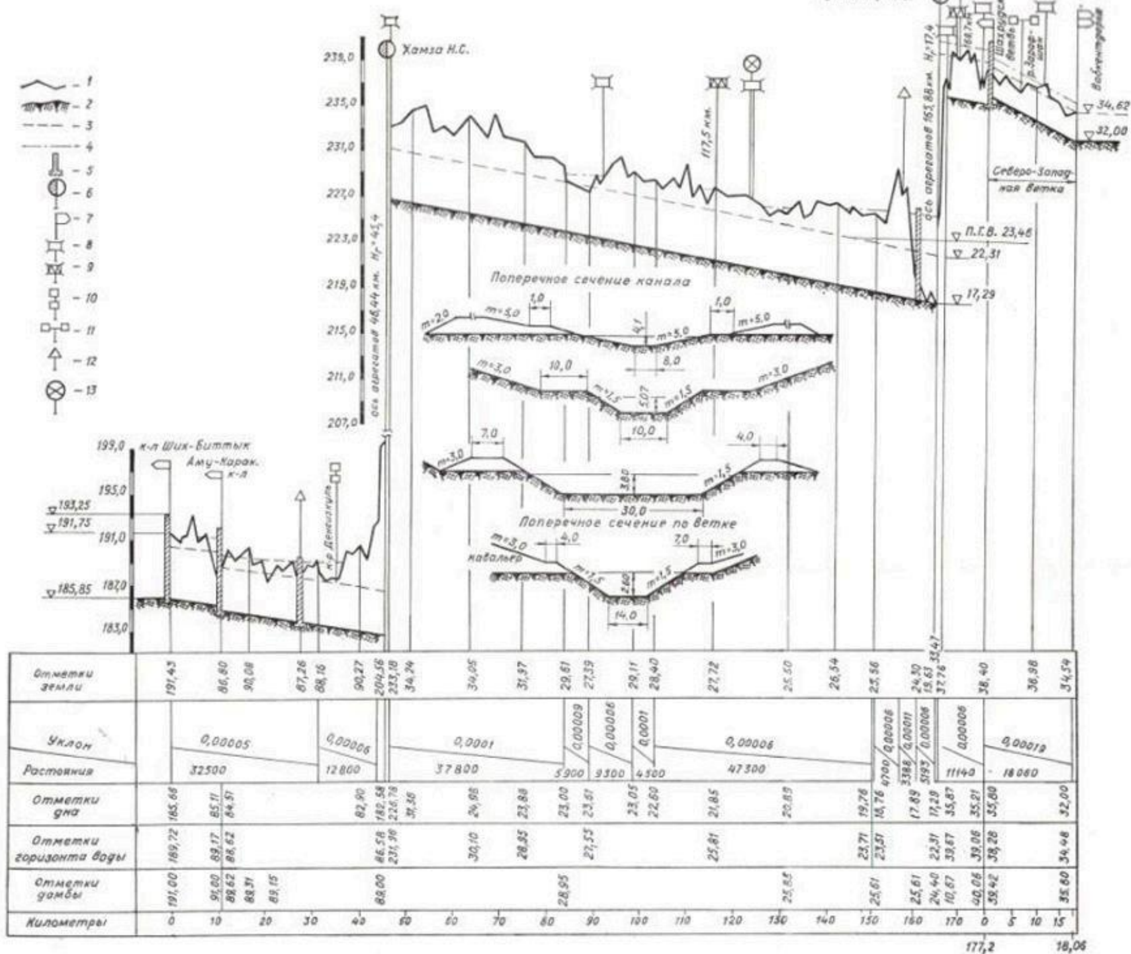
Рис. 13. Продольный профиль Амударьинского канала, первая очередь.
