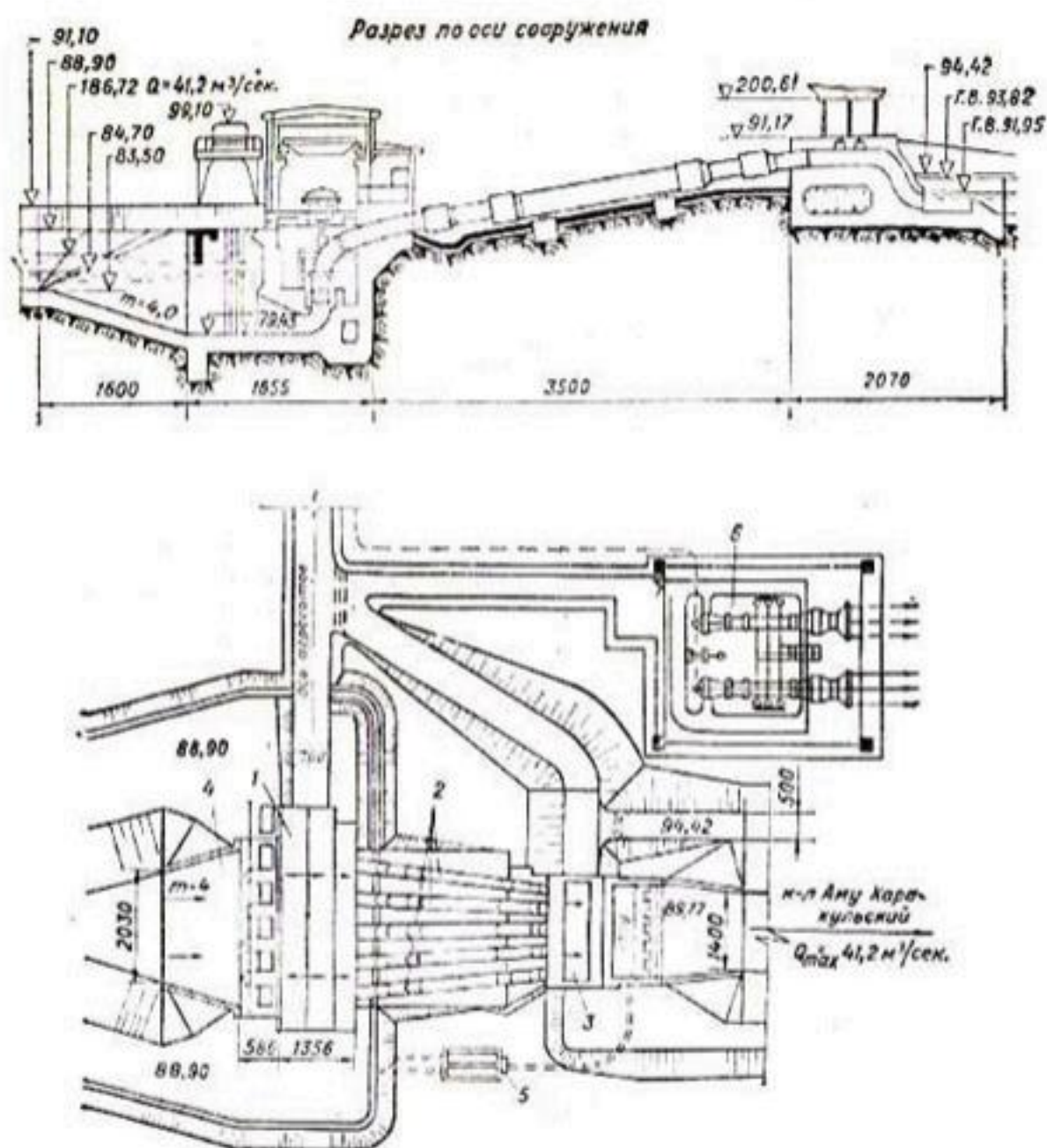
Рис. 14. Алатская насосная станция:
