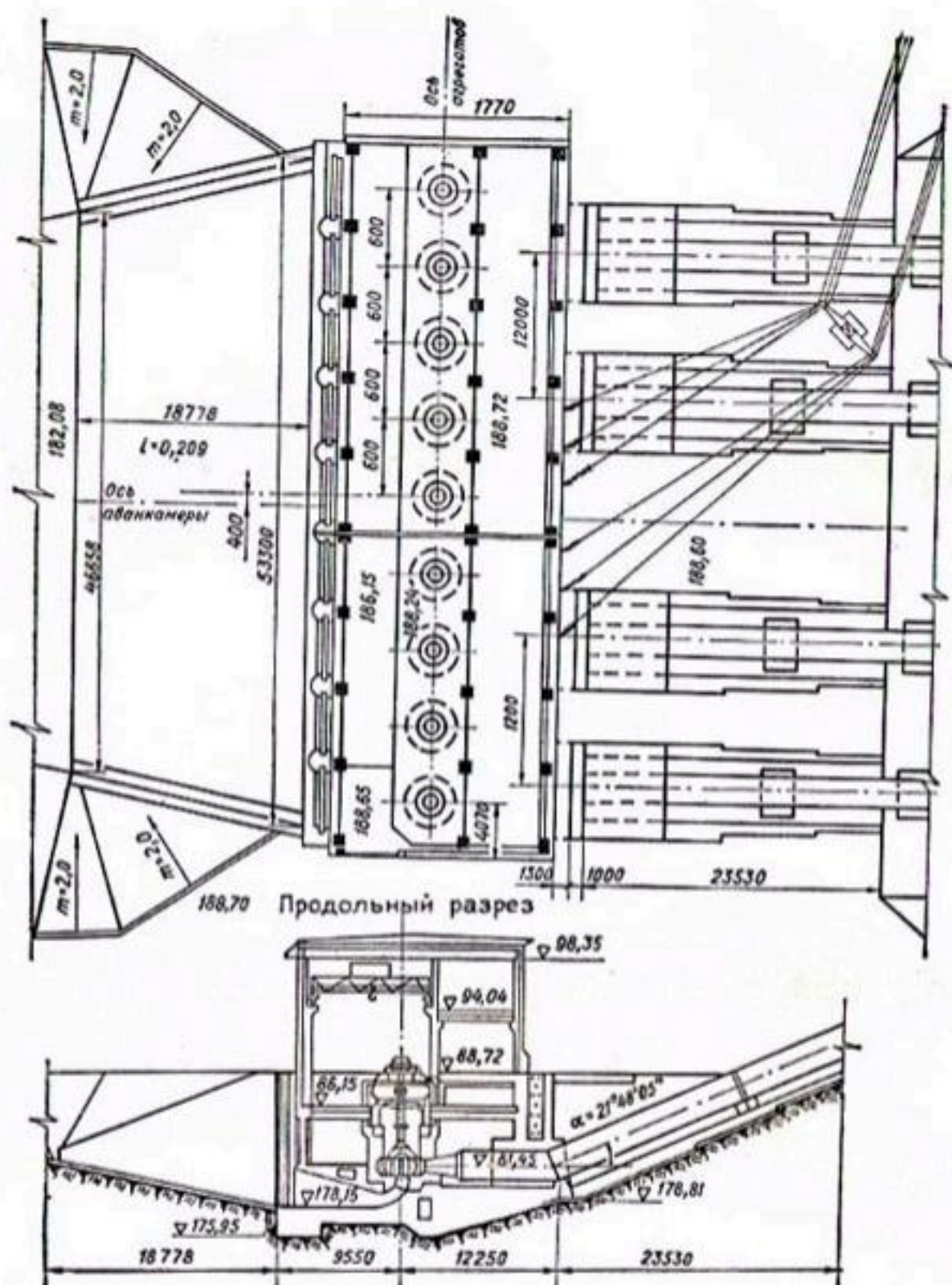
Рис. 20. Насосная станция Хамза-1.
