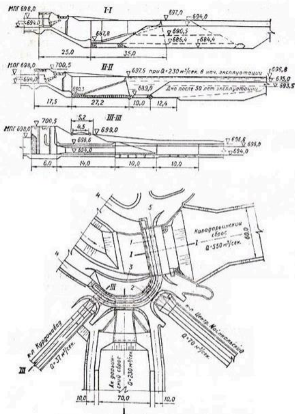
Рис. 3. Аккарадарьинский гидроузел:
