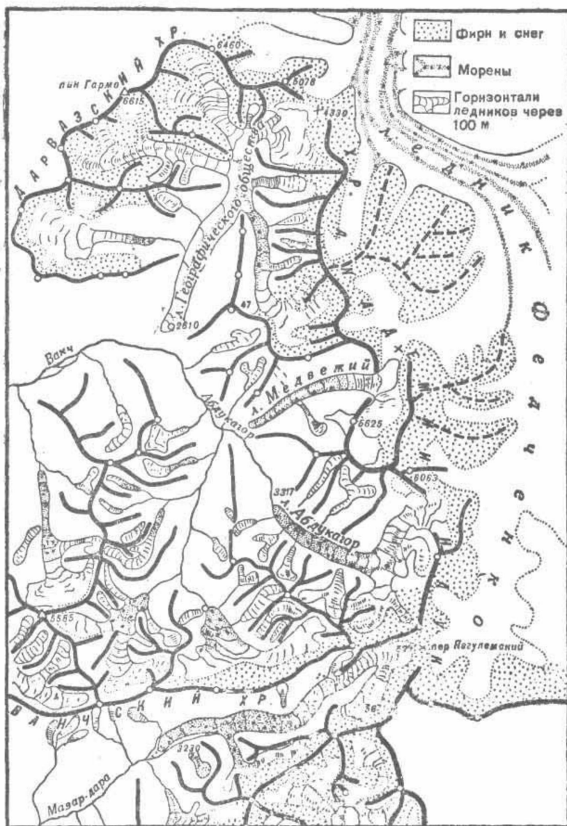
Схема оледенения истоков рек Ванч и Язгулем (по схеме Р. Д. Забирова, участника гляциологической экспедиции профессора И С Щукина 1947--1948 годов).
