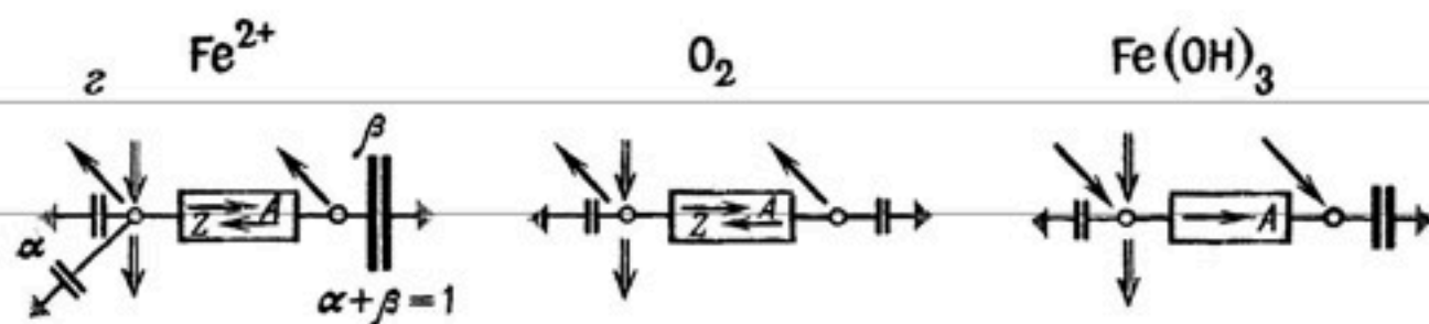
Рис. 15. Многоступенчатая цепь наглядных моделей миграции железа \text{Fe}^{2+} , кислорода \text{O}_2 и гидроокиси железа в грунтовых водах.
