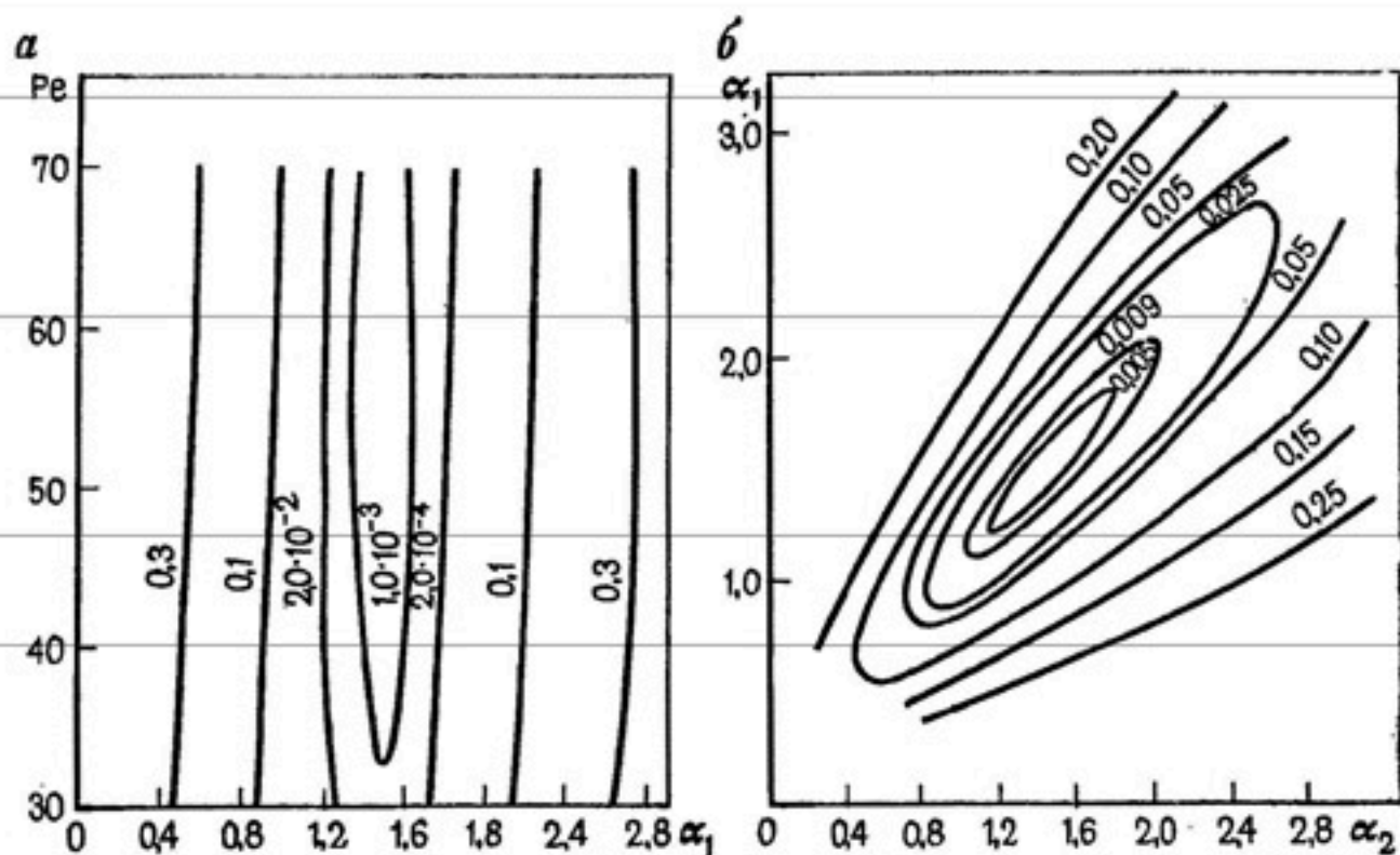
Рис. 41. Графики функции качества F_k при изменении параметров \text{Re} , \alpha_1 и \alpha_2 . a - \alpha_1 = 1.5 , \xi = 1.0 , \tau = 1.4 \cdot 10^{-4} \text{ c}^{-1} ; b - \text{Re} = 50 , \xi = 1.0 , \tau = 1.4 \cdot 10^{-4} \text{ c}^{-1}
