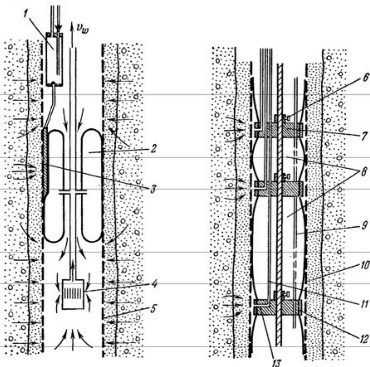
Рис. 49. Специальный пакер.
