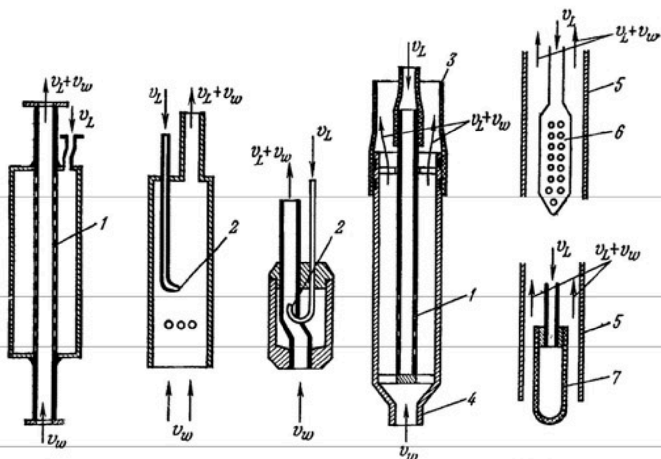
Рис. 59. Примеры устройства эрлифтов (эжекторных насосов) [78].
