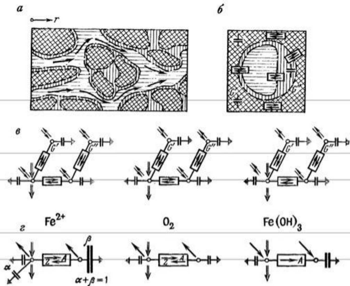
Рис. 15. Многоступенчатая цепь наглядных моделей миграции железа \text{Fe}^{2+} , кислорода \text{O}_2 и гидроокиси железа в грунтовых водах.
