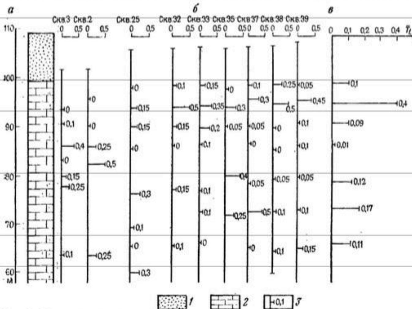
Рис. 8. Выделение проницаемых зон в карбонатных породах по данным расходометрии скважин (материалы А. Л. Петрова).
