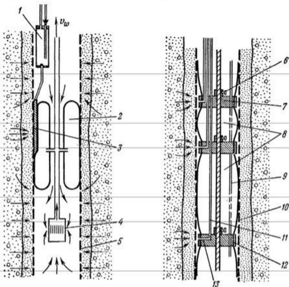
Рис. 49. Специальный пакер.
