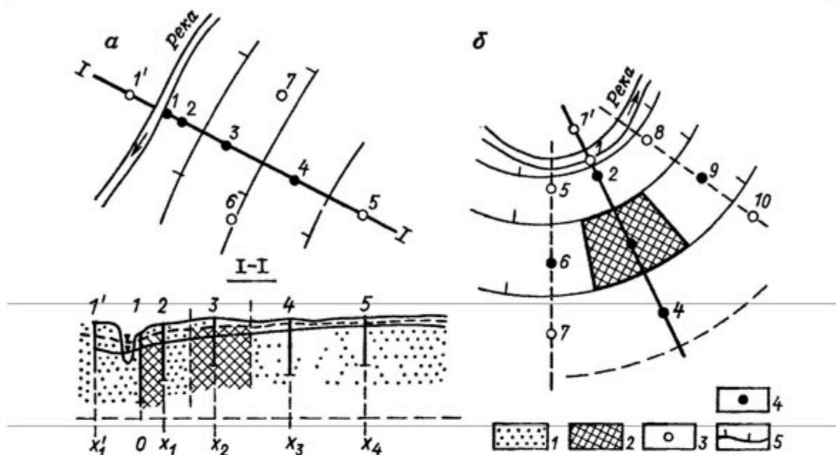
Рис. 31. Схемы расположения наблюдательных скважин в створах по потоку при одномерном в плане (а) и двухмерном (б) движении вод:
