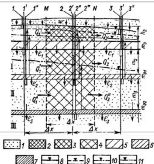
Рис. 4. Схема многослойной толщи водоносных пород:
