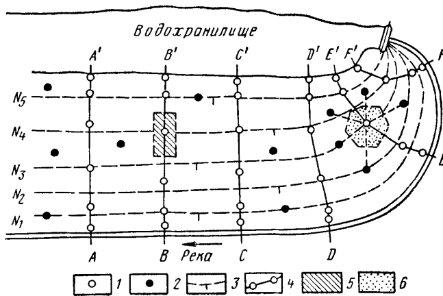
Рис. 3. Расположение наблюдательных скважин на междуречье. 1 — наблюдательная скважина в створе; 2 — то же, вне створа; 3 — гидроизогипсы; 4 — створ наблюдательных скважин; 5 — расчетный элемент одномерного потока; 6 — то же, для двухмерного в плане потока
