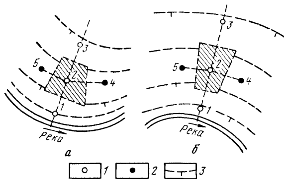
Рис. 4. Расположение наблюдательных скважин около излучин реки (заштрихованы элементы потока).
