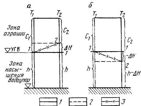
Рис. 57. Схема обозначений запасов влаги в почвенно-грунтовой призме на моменты времени T_1 и T_2 .
