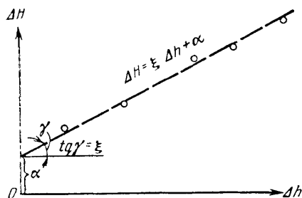
Рис. 20. График связи напоров напорных вод с уровнем грунтовых вод
