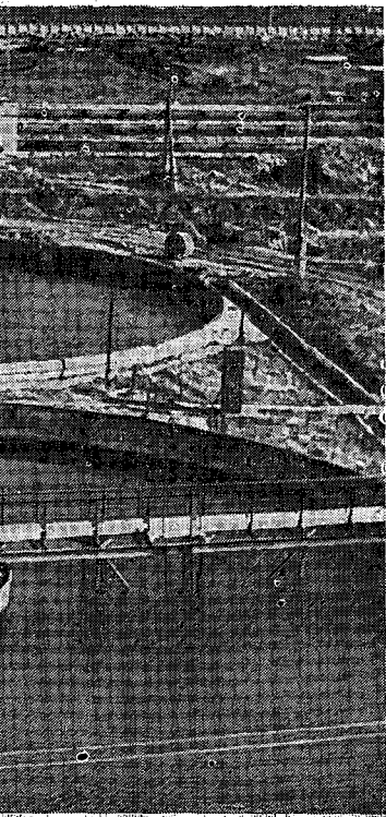
Рис. 3. Очистные соору- жения Рязанского нефте- перерабатывающего заво- да. На переднем плане — отстойник.
