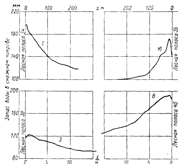
Рис. 24. Убыль среднего по маршруту запаса воды в снеге в зависимости от его длины (расстояния \frac{B}{2} + x от середины лесной полосы по направлению
