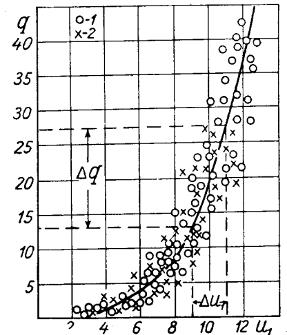
Рис. 13. Зависимость общей интенсивности переноса снега от скорости ветра по данным метелемерных наблюдений (Комаров, 1954а). 1 — на открытой площадке, 2 — за преградами.
