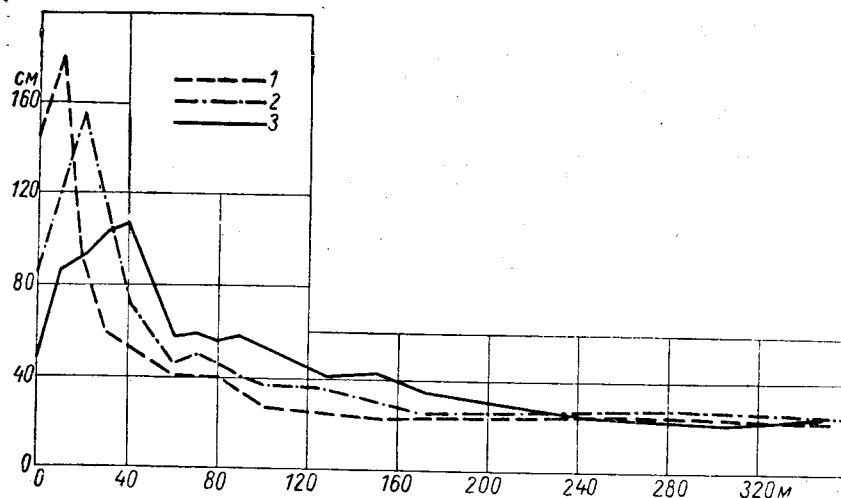
Рис. 18. Высота снега (см) на различных расстояниях от лесных полос (м) в зависимости от их конструкции (Никитин и Минин, 1949). Лесная полоса: 1 — плотная, 2 — ажурная, 3 — продузаемая.
