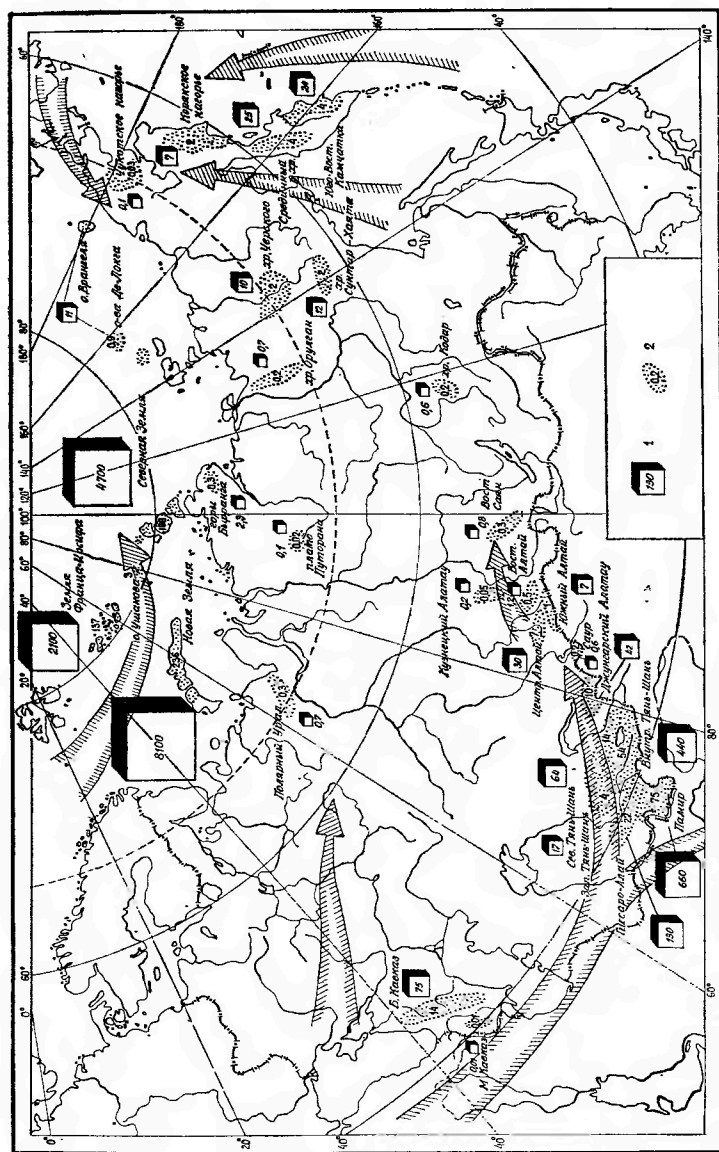
Рис. 16. Распределение площадей и массы льда по ледниковым системам и их связь с циркуляцией атмосферы.
