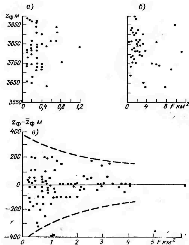
Рис. 4. Отсутствие связи высоты границы питания на ледниках z_{\phi} с их площадью F .
