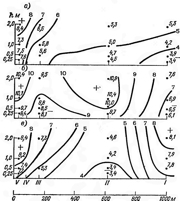
Рис. 1. Вертикальный разрез температуры воздуха (°C) в приледном слое по поперечнику через Марухский ледник.
