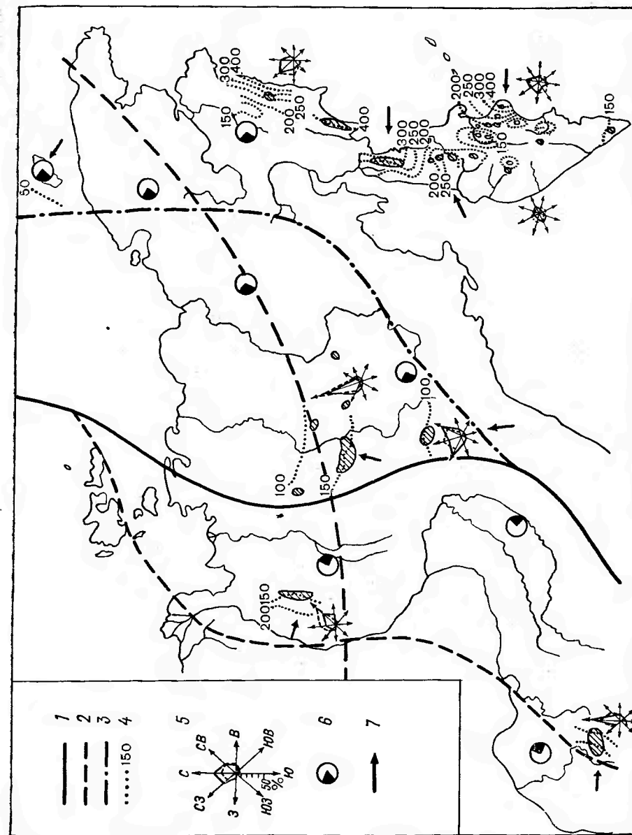
Рис. 32. Преобладающие направления поступления влаги в ледниковые системы Северо-Востока СССР. 1 — граница преобладающей тихоокеанской влаги; 2 — граница преобладающей атлантической влаги; 3 — граница преобладающей тихоокеанской влаги; 4 — граница преобладающей атлантической влаги; 5 — граница преобладающей тихоокеанской влаги; 6 — граница преобладающей атлантической влаги; 7 — граница преобладающей тихоокеанской влаги. Цифры — количество осадков, мм/год. Стрелки — направление преобладающих ветров.
