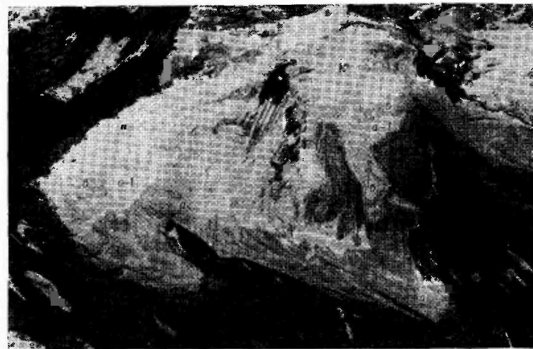
Рис. 8. Склоновый ледник № 904 (площадь 0,8 км 2 ) в бассейне р. Шах-дара на восточном макросклоне Ишкашимского хребта (Памир), 12 августа 1973 г. Фото О. В. Роттаевой.
