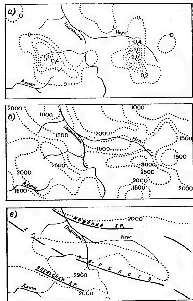
Рис. 12. Климатический и орографический факторы оледенения хребта Черского.
