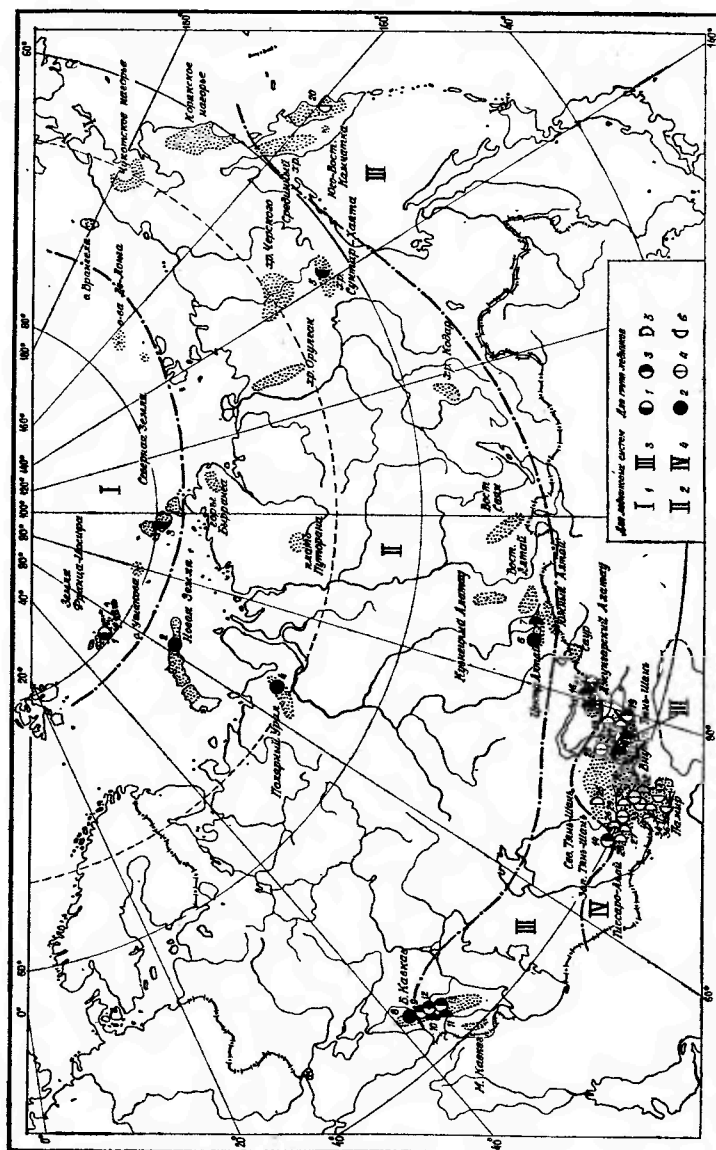
Рис. 41. Типы структуры теплового баланса поверхности ледников в ледниковых системах.
