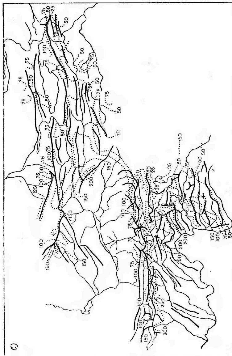
Рис. 35. Поля аккумуляции (г/см 2 ) (а) и твердых осадков (см) (б) на высоте границы питания ледников в ледниковых системах Средней Азии.
