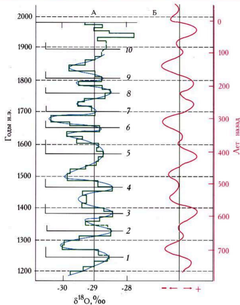
Рис. 3.36. Циклические изменения палеотемператур северо-западной Гренландии за последние 800 лет по изотопно-кислородным исследованиям ледяного керна со станции Кемп-Сенчури
