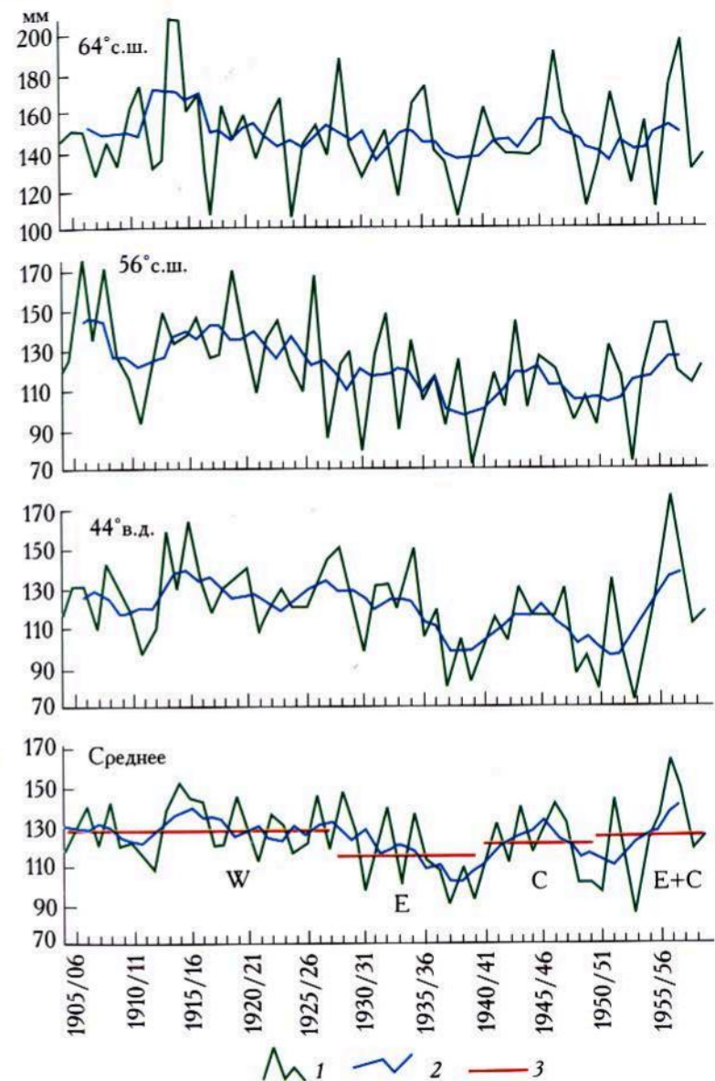
Рис. 1.23. Изменение снегозапасов от года к году по трем профилям на Русской равнине и в целом на всей ее территории 1 – ежегодные данные, 2 – осредненные за 5 лет, 3 – среднее снегонакопление за отдельные эпохи господствующей формы циркуляции атмосферы
