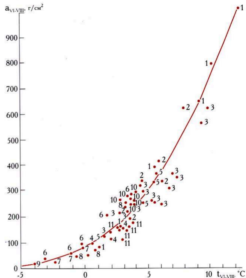
Рис. 2.29. Зависимость среднего за летний период таяния a_{VI-VIII} от средней летней температуры t_{VI-VIII} По А.Н. Кренке и В.Г. Ходакову (1966)
