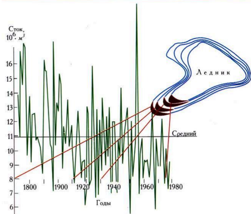
Рис. 3.46. Изменение ледникового стока в связи с деградацией ледника Джанкуат Зачернены конечные морены
