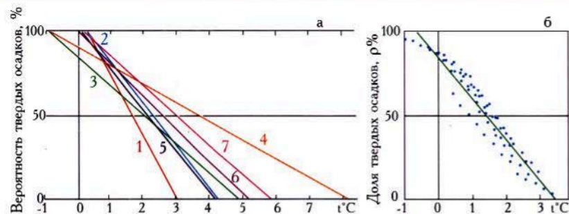
Рис. 3.20. Связь выпадающих осадков с температурой воздуха а – вероятность выпадения твердых осадков при данной температуре t : 1 – Непальские Гималаи, 4958 м над ур. моря; 2 – гора Богда в Восточном Тянь-Шане, 3640 м; 3 – Западный Тянь-Шань, 1780 м; 4 – Западный Тянь-Шань, 3670 м; 5–7 – Япония (внутренняя равнина, побережья Тихого океана и Японского моря). б – доля твердых осадков в общем количестве осадков \rho при данной средней температуре воздуха t за полмесяца
