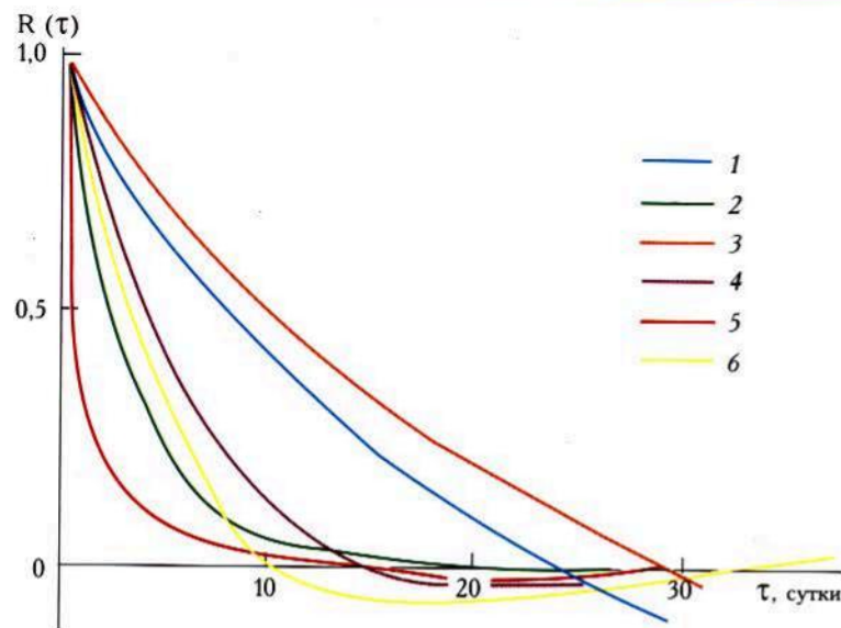
Рис. 3.45. Нормированные автокорреляционные функции параметров внешнего массоэнергообмена ледника Джанкуат на Центральном Кавказе 1 – баланс коротковолновой радиации, 2 – температура воздуха, 3 – таяние в опорной точке, 4 – таяние языка ледника, 5 – таяние всего ледника, 6 – сток воды с горно-ледникового бассейна, степень оледенения которого равна 48%
