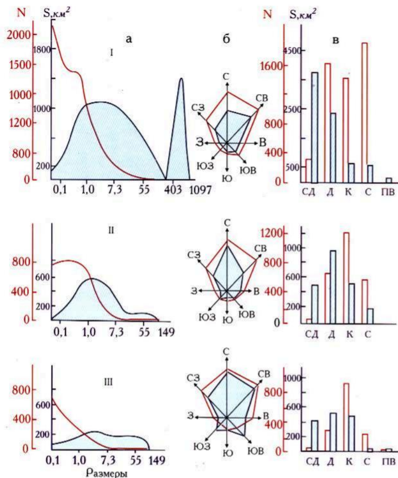
Рис. 2.37. Распределение количества N (красная линия) и площади S , км 2 (синяя линия с голубой заливкой) ледников по размерам и градациям в логарифмической (натуральные логарифмы) шкале (а), по экспозициям (б) и по группам морфологических типов (в) на Памире (I), Гиссаро-Алае (II) и Кавказе (III)
