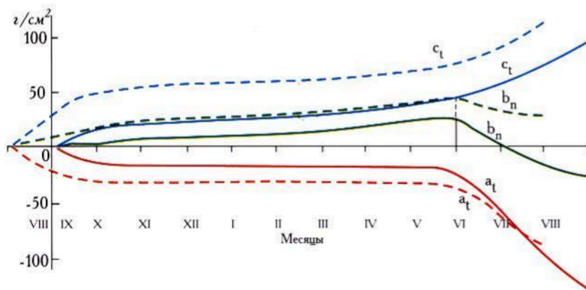
Рис. 3.21. Годовой ход аккумуляции c_t , абляции a_t и баланса массы b_n для ледника с летним максимумом абляции Штрих-пунктирные линии – при понижении средней годовой температуры на 0,5°
