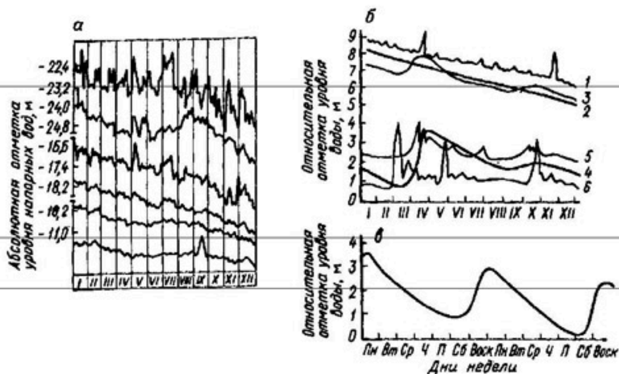
Рис. 4. Графики гидродинамического режима подземных вод в районе водозаборов. а — по мере удаления от центра водозабора (сверху вниз); б — внутригодовой режим уровней в различных условиях; в — режим уровней в течение недели. 1 — 6 — типы режимов подземных вод, характерные для: 1 — артезианских бассейнов платформенного типа, замкнутых котловин и изолированных переуглубленных долин; 2 — то же, и для линз пресных вод с отсутствием питания; 3 — артезианских бассейнов платформ и межгорных впадин с перетеканием из грунтовых вод или привлечением вод из областей питания, подоцерных надмерзлотных таликов, замкнутых структур трещинно-карстовых вод, линз пресных вод с наличием сезонного питания, ледниковых отложений; 4 — речных долин второго и третьего типов, месторождений трещинно-карстовых вод с наличием регулирующей емкости; 5 — речных долин первого типа; 6 — месторождений трещинно-карстовых вод при отсутствии регулирующей емкости
