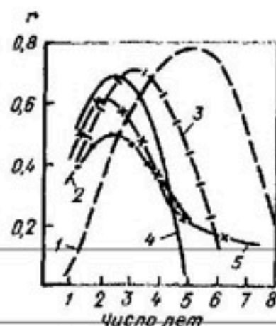
Рис. 13. Графики зависимости тесноты связи ( r ) среднегодовых уровней грунтовых вод от количества суммируемых атмосферных осадков (2–5) или резности осадков и испарения (1) за ряд лет.
