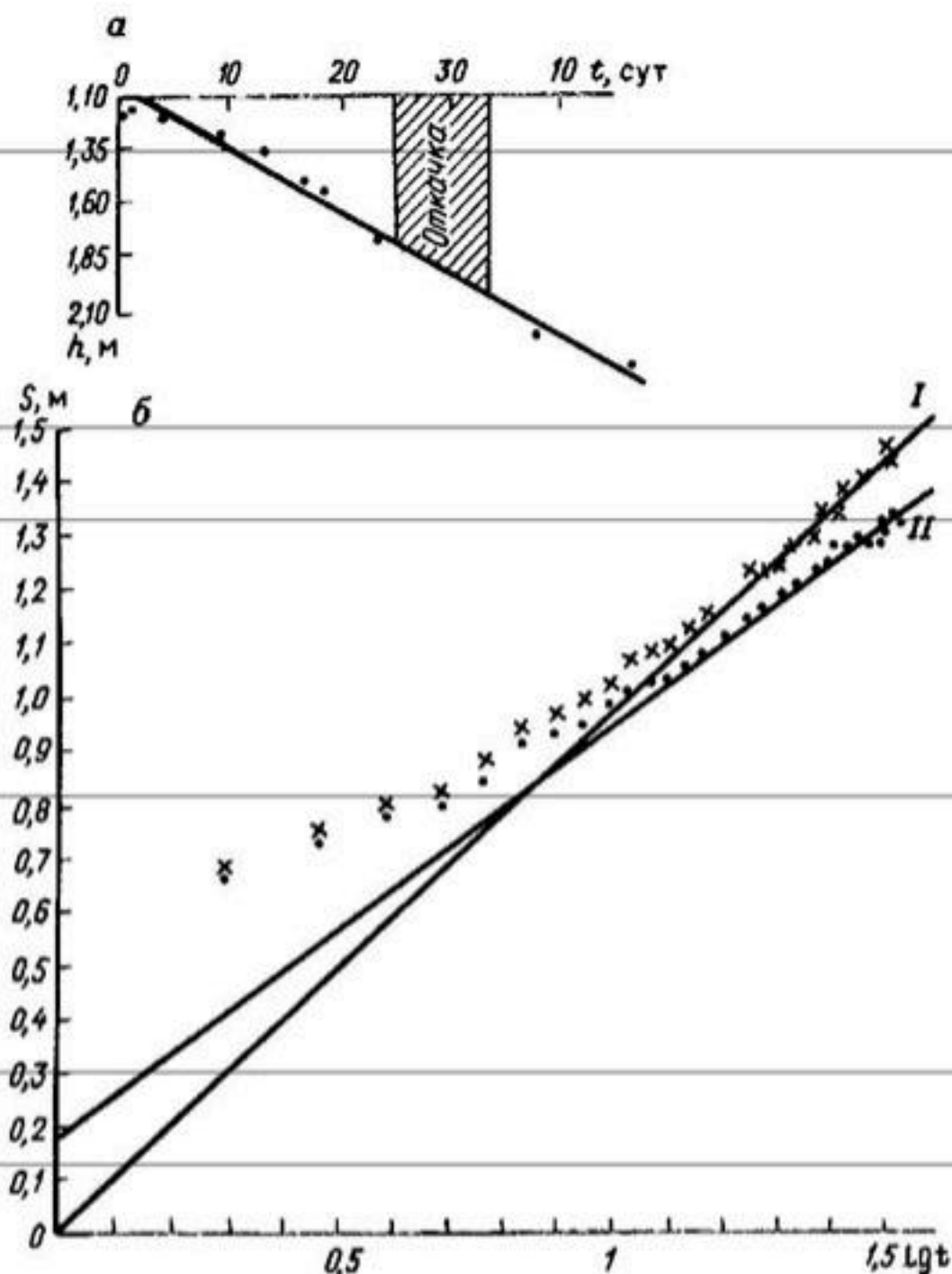
Рис. 15. Оценка влияния снижения уровня грунтовых вод ( h ) на величину понижения ( S ) в процессе откачки (по материалам ПГО "Востоквзгеология").
