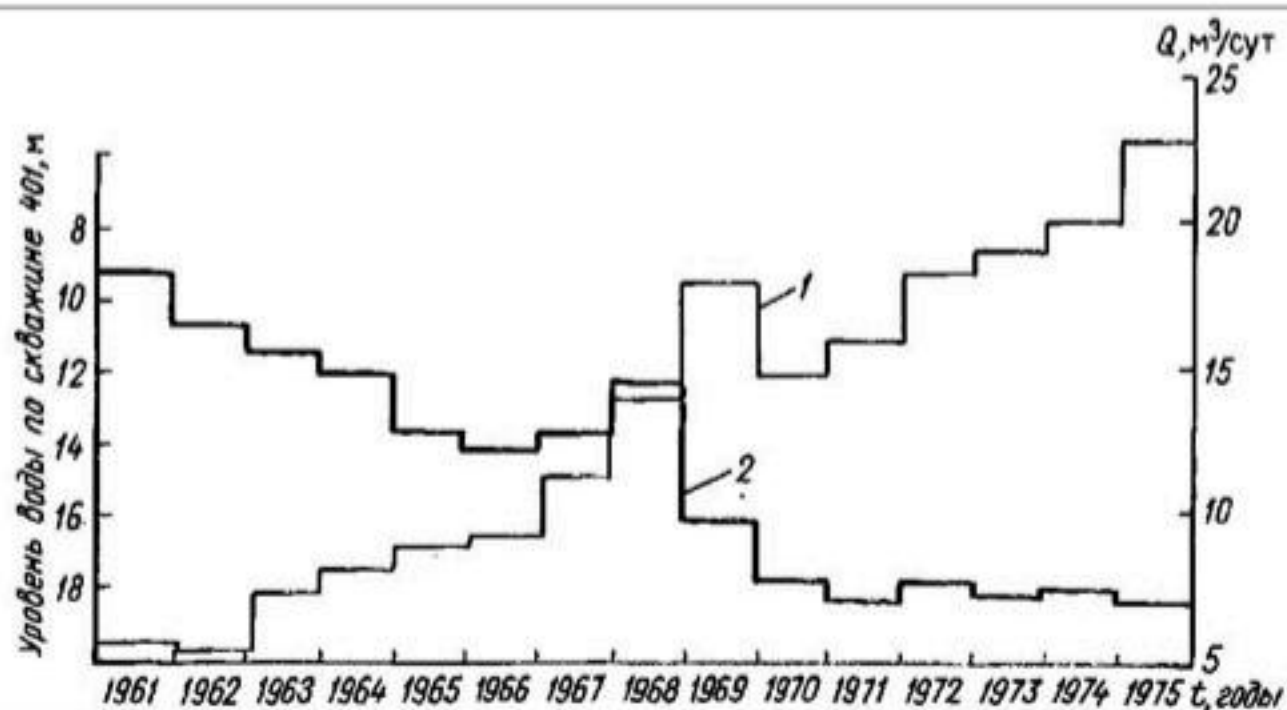
Рис. 30. График водоотбора (1) и понижения уровней подземных вод во времени (2) для одного из водозаборов Эстонии
