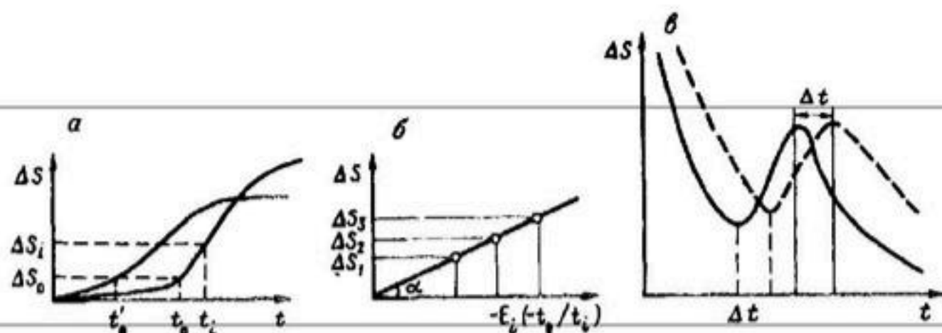
Рис. 27. Схемы определения коэффициента пьезопроводности по "времени добывания".
