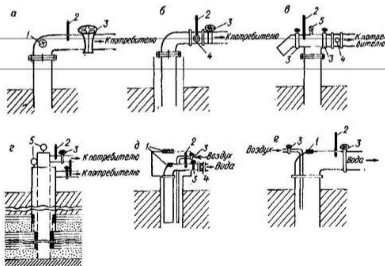
Рис. 10. Схемы оборудования эксплуатационных скважин для наблюдений за режимом подземных вод.
