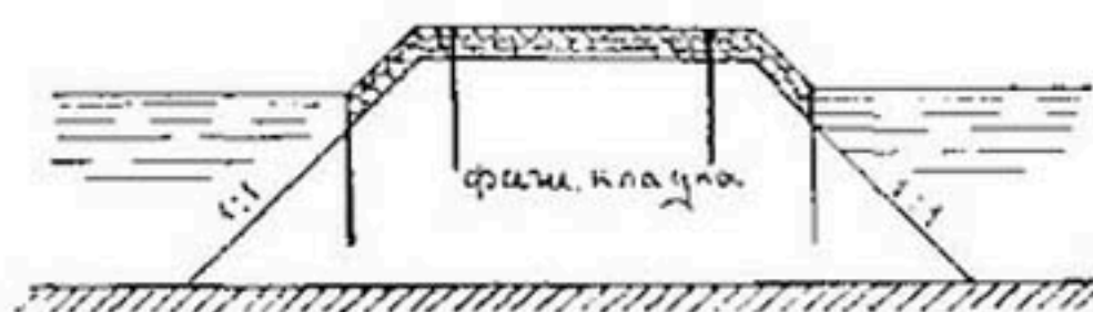
Рис. 170. Укрепление гребня полузапруд на р. Западной Двине.
