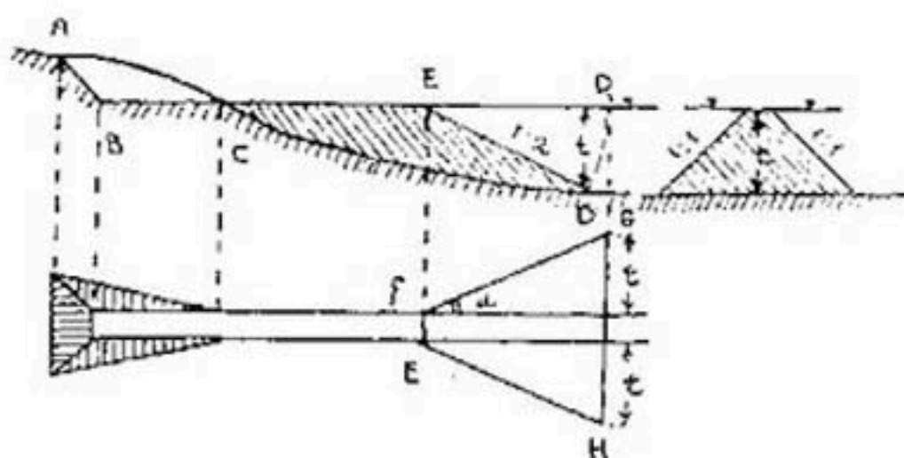
Рис. 109. Всерная кладка фашин для образования подводной части дамбы.
