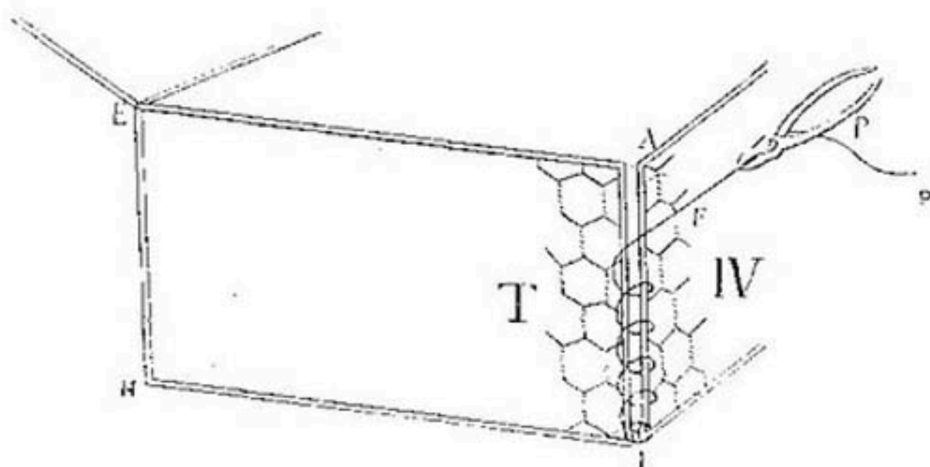
Рис. 85. Скрепление проволокой (p) ребер габбионного ящика. Стягивание проволоки производится клещами (P).
