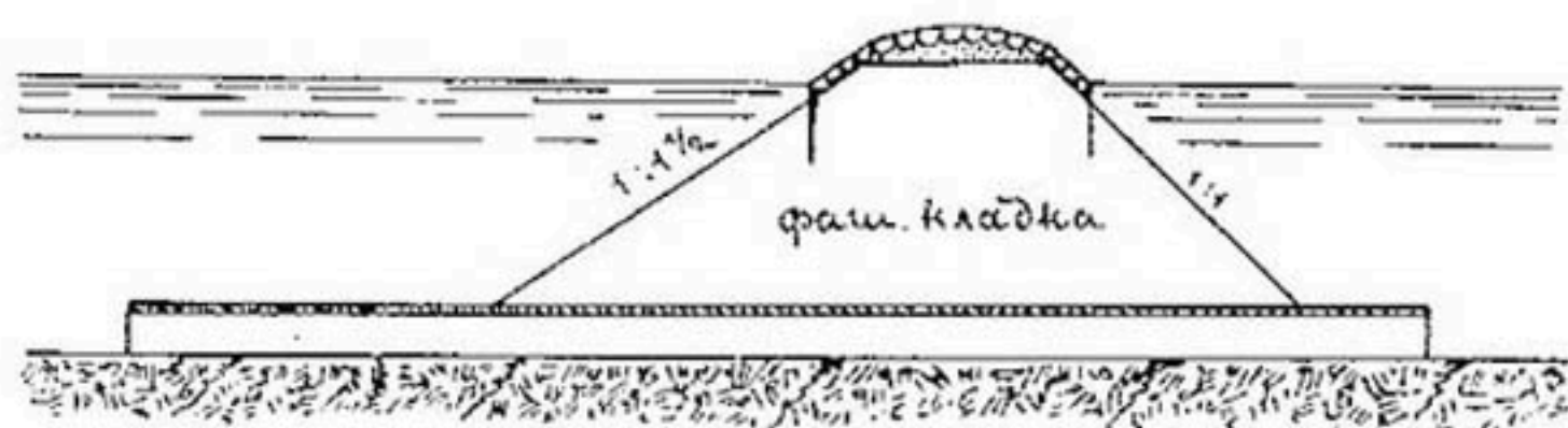
Рис. 202. Запруда из фашинной кладки на фашинном тюфяке.
