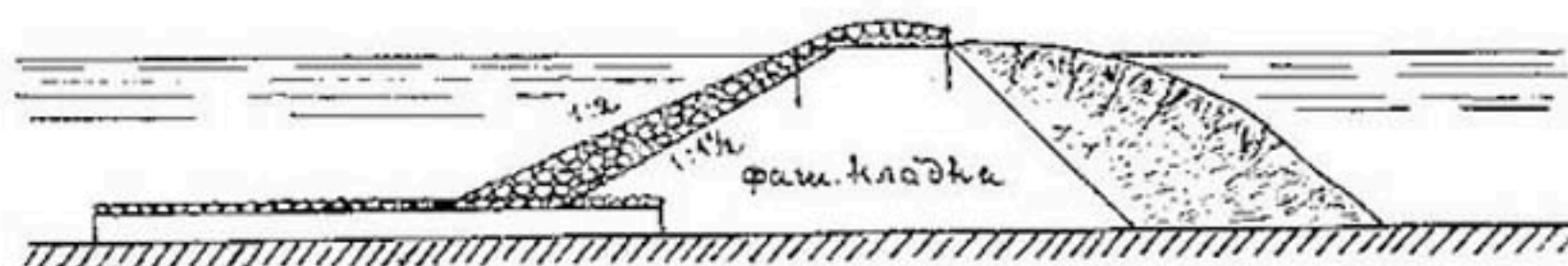
Рис. 179. Тип продольной дамбы на р. Западной Двине.
