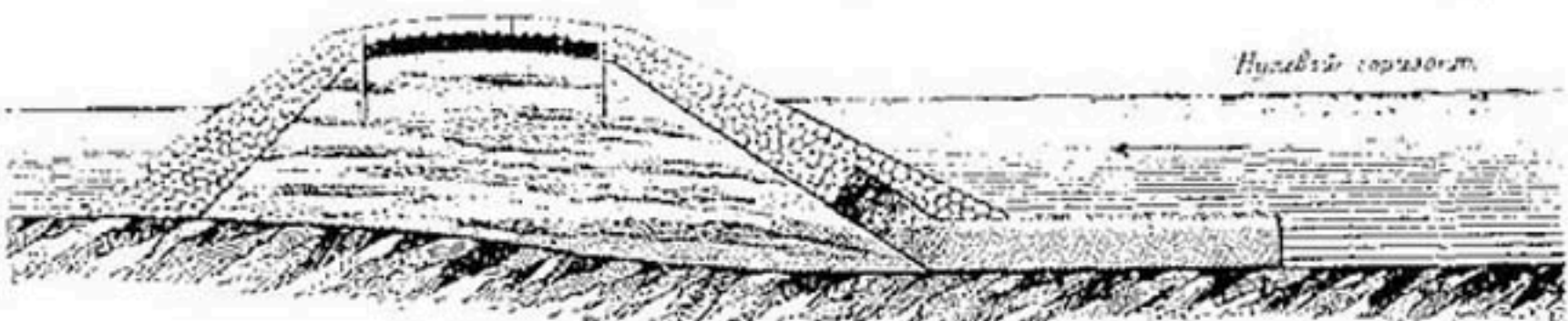
Рис. 182. Продольная дамба с укрепленными каменной заброской откосами по обоим сторонам.
