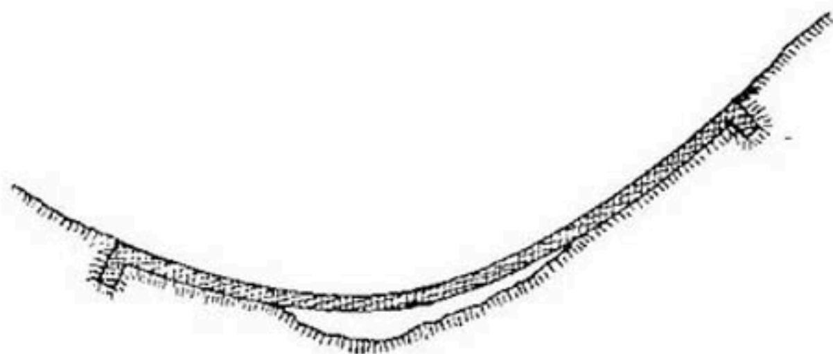
Рис. 124. Корни берегового укрепления.
