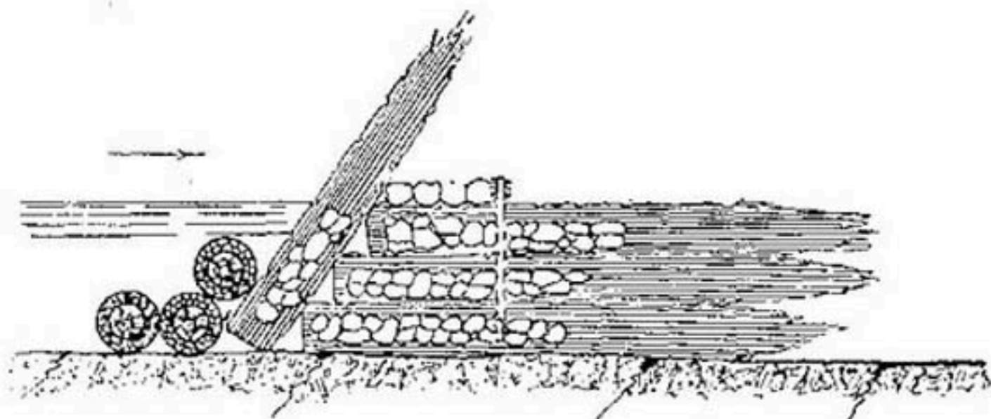
Рис. 223. Фашинные бун-илоудержатели на р. Дунае.
