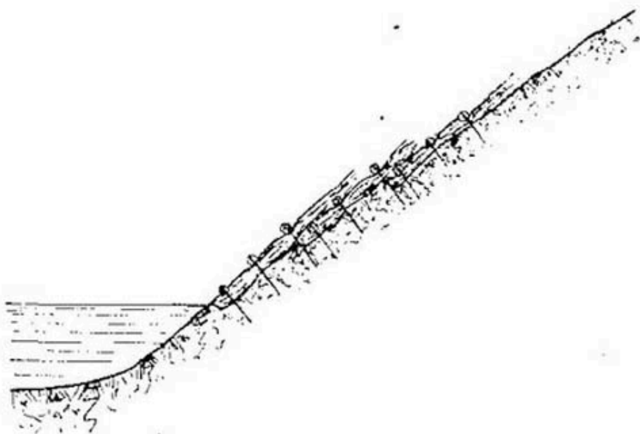
Рис. 155. Поперечная хворостяная выстилка в несколько рядов.
