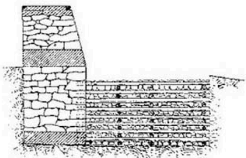
Рис. 257. Ряжевый водобойный пол запруды.
