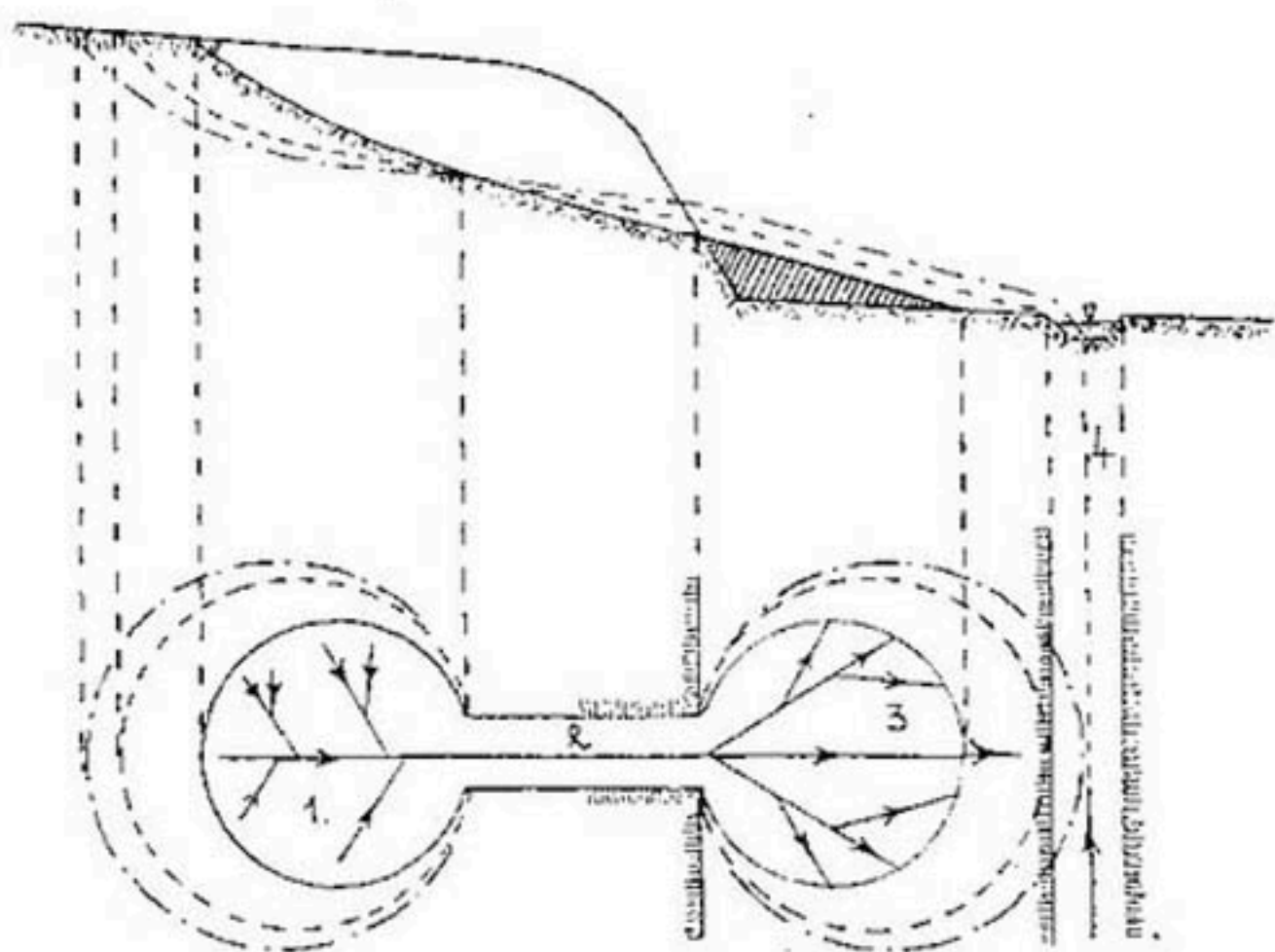
Рис. 245. Схема частей горного потока: 1) сборный бассейн, 2) канал, 3) высышка.
