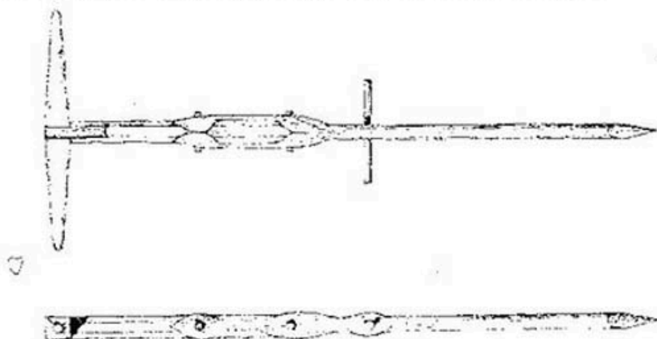
Рис. 241. Сверло для делания лунок при посадке черенков пияка.
