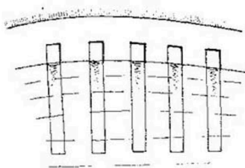
Рис. 140. Ленточное укрепление берега фашинными тюфяками.
