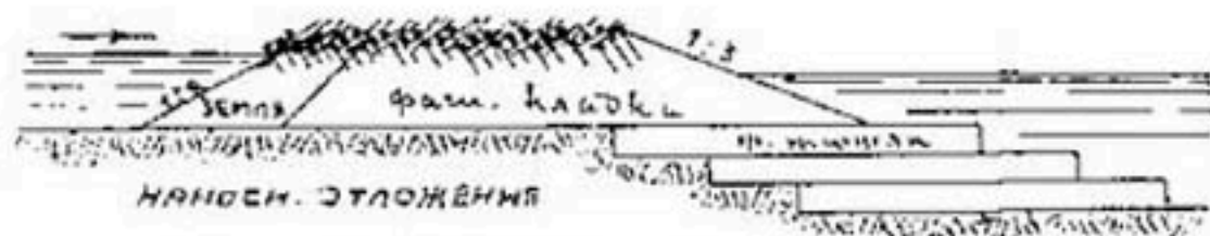
Рис. 208. Постепенное устройство запруды.
