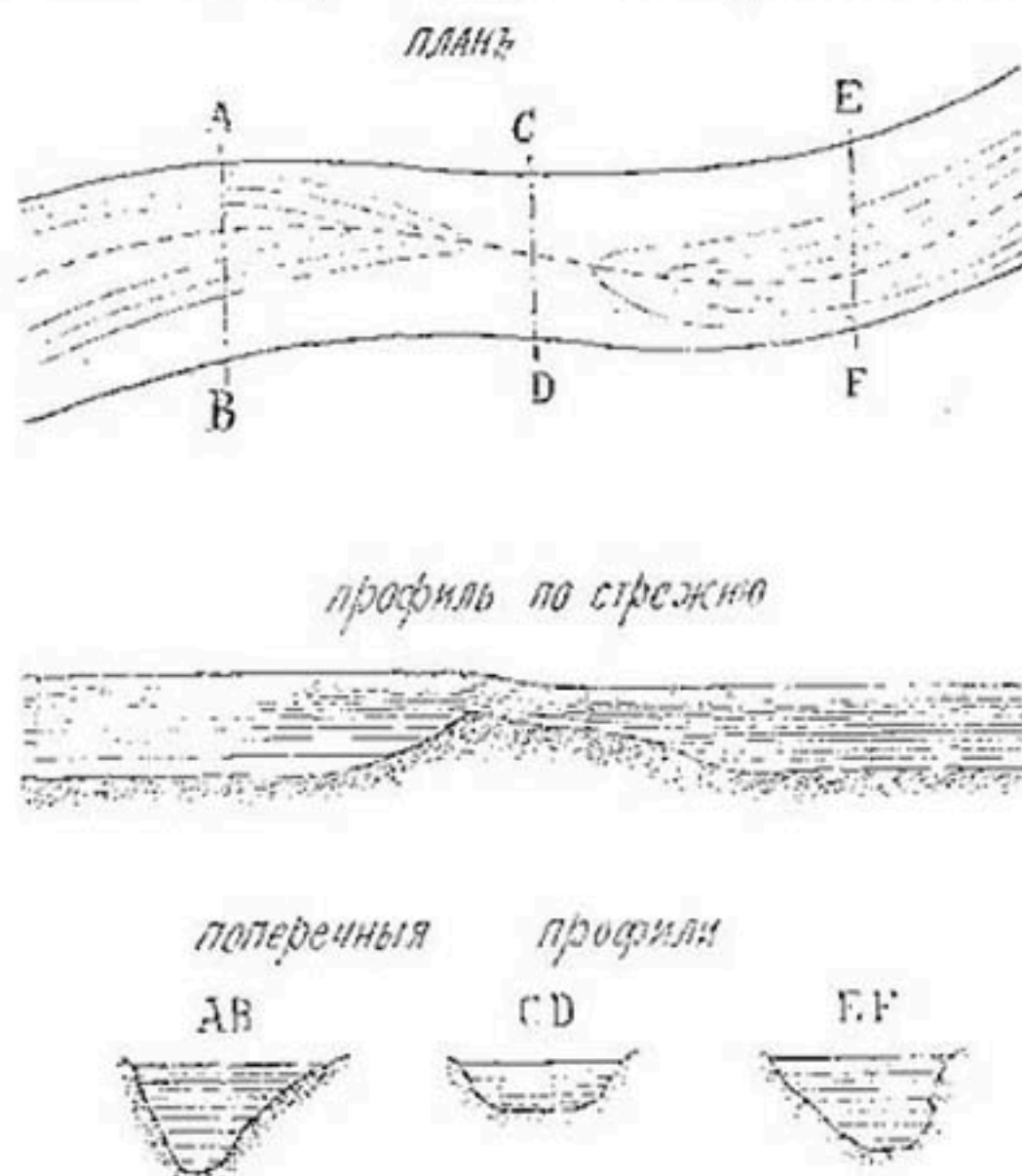
Рис. 54-56. Тип 2-й — (хороший перекат).
