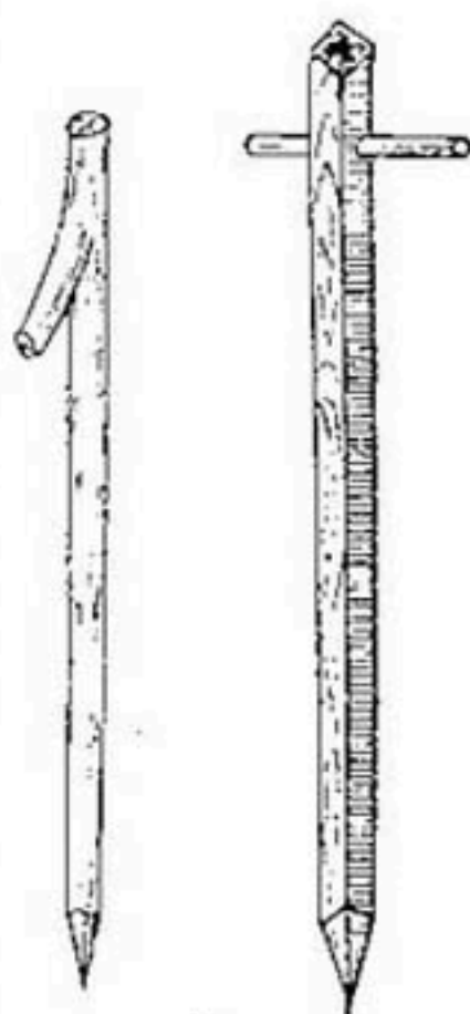
Рис. 95. Колья для закрепления фашины и прутяных канатов в фашиной кладке.
