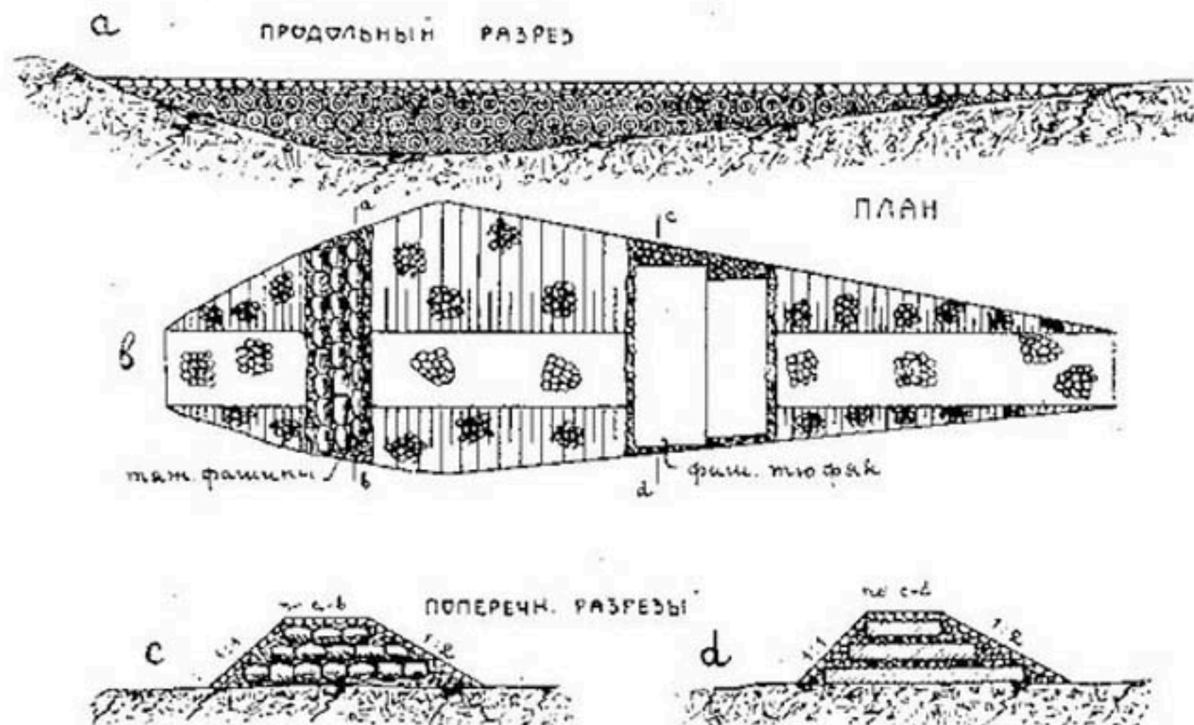
Рис. 198. Донный порог, устроенный из fascии.
