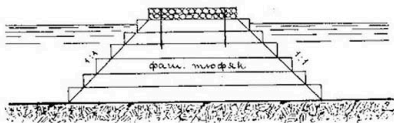
Рис. 203. Запруда из нескольких слоев фашинных тюфяков.
