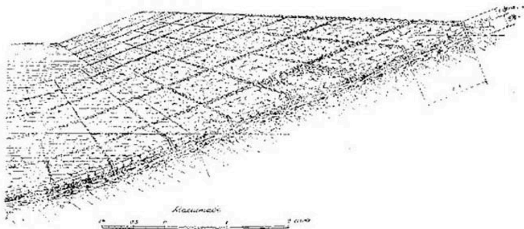
Рис. 160. Плетневые клетки, сделанные на хворостяном туюфке, покрывающем надводную часть откоса берега.
