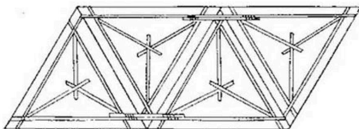
Рис. 191. Сопряжение между собой трехугожных сипаев.
