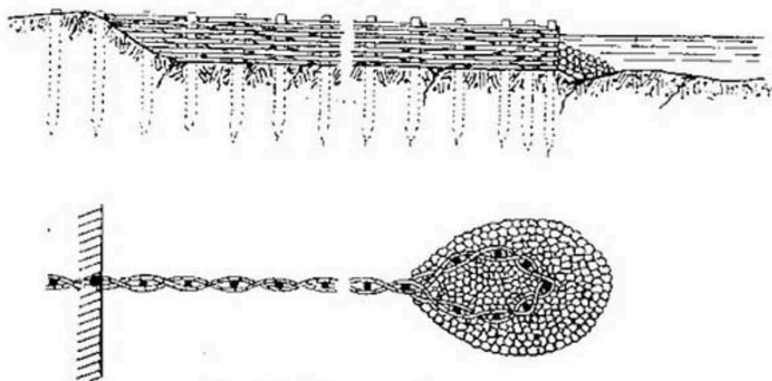
Рис. 216. Плетневой илоудержатель.
