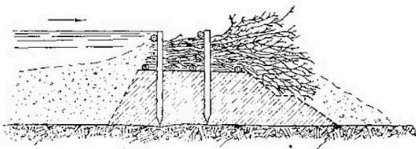
Рис. 224. Фашинные траверсы-илоудержатели на р. Инне.
