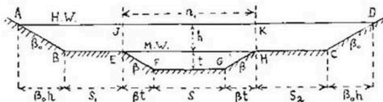
Рис. 41. Двухъярусное русло.
