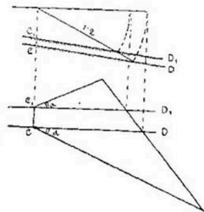
Рис. 110. Форма слоев фашинной всерной кладки при крутом уклоне дна.
