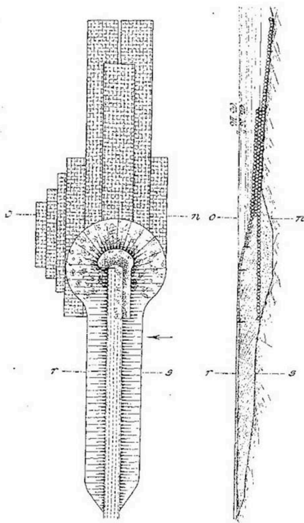
Рис. 197. Донная полузапруда на р. Эльбе, состоящая из тяжелых фашин и прибитая к голове полузапруды.
