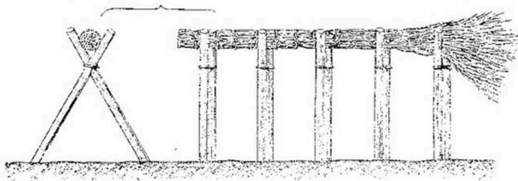
Рис. 90. Вязка фашин.
