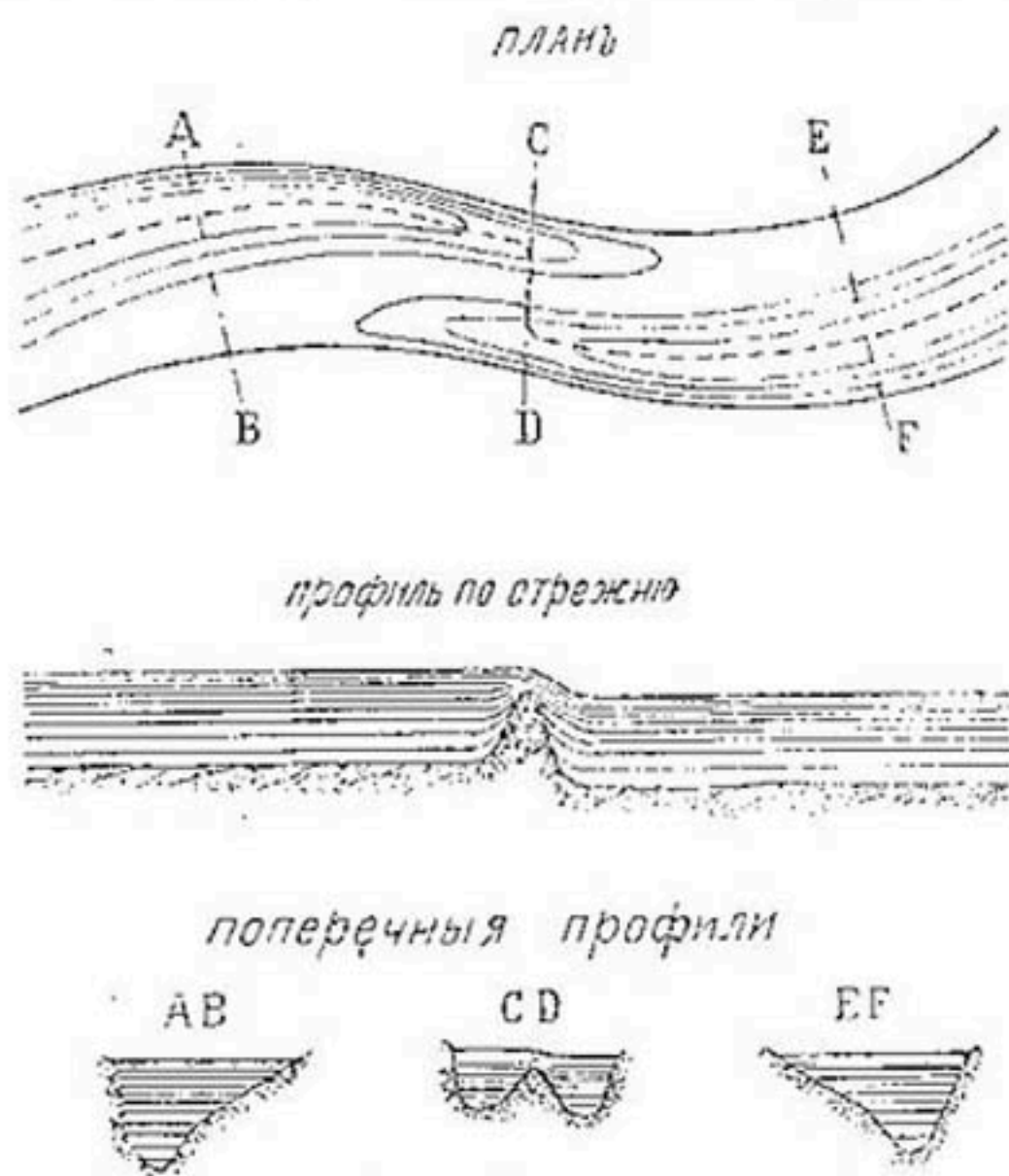
Рис. 54-а. Тип 1-й—(плохой перекат).
