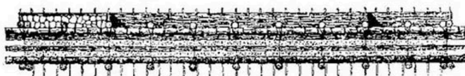
Рис. 105-б. Связанный хворостяной тюфяк.
