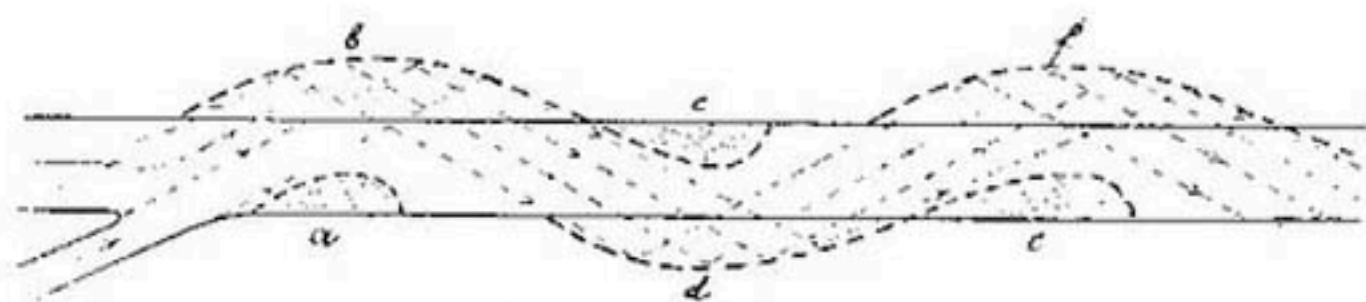
Рис. 17. Извилины реки.
