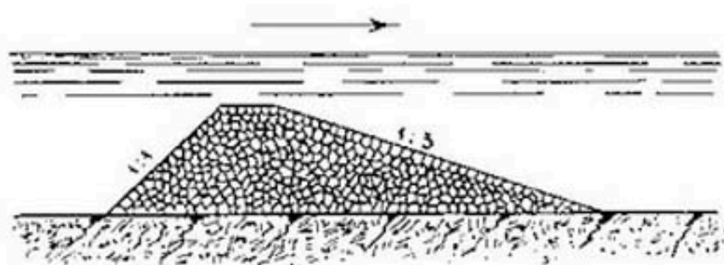
Рис. 199. Донный порог, построенный из каменной наброски.
