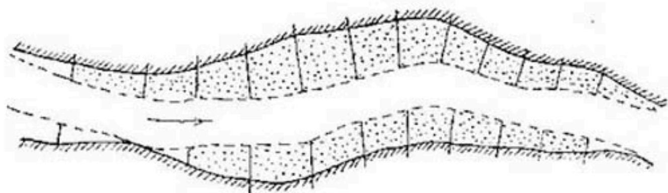
Рис. 47. Выправление русла полузапрудами.
