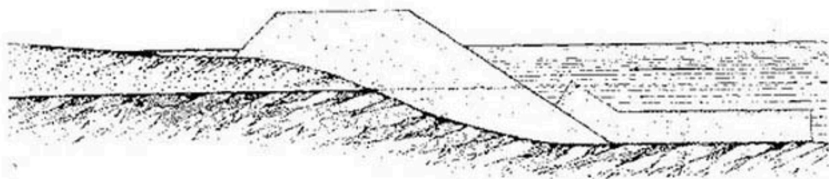
Рис. 184. Продольная дамба, расположенная вблизи берега.
