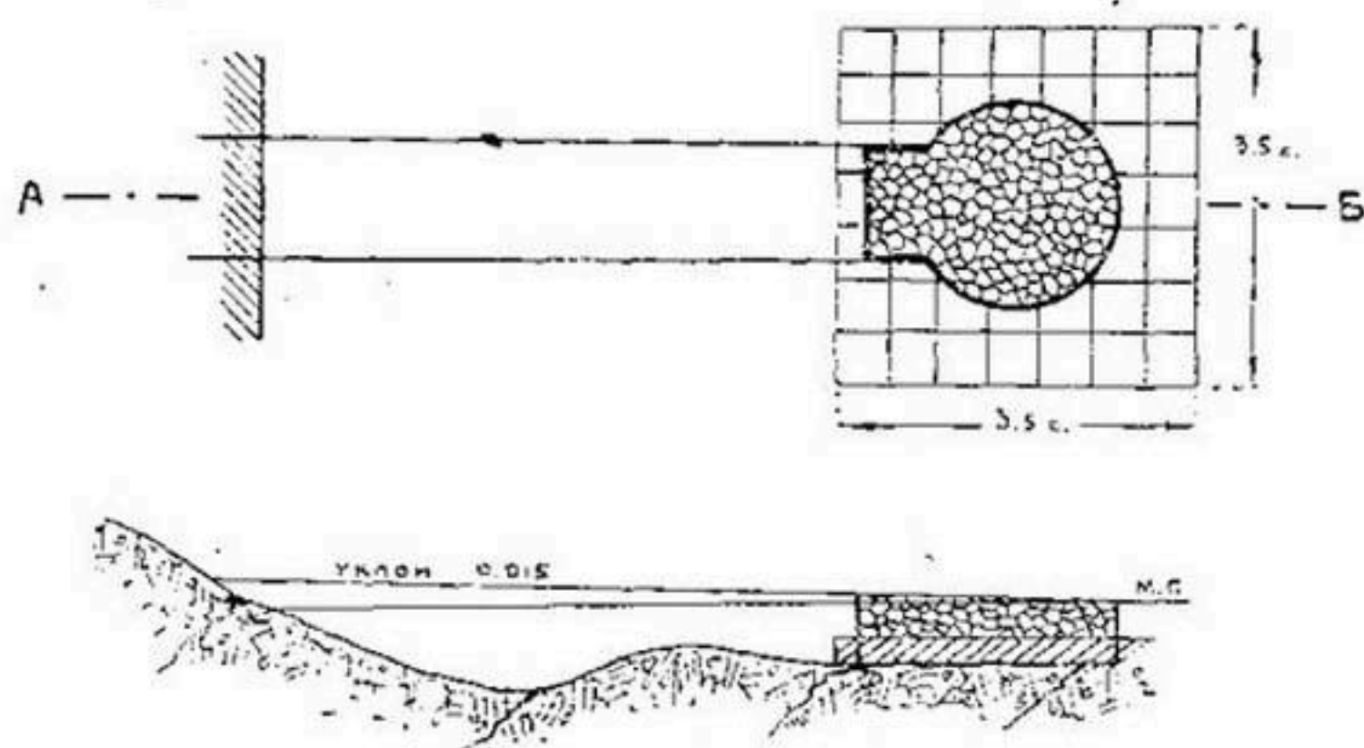
Рис. 219. Плетневые полузапруды на р. Днепре. Усиление головной части помощью фашиновых тюфяков
