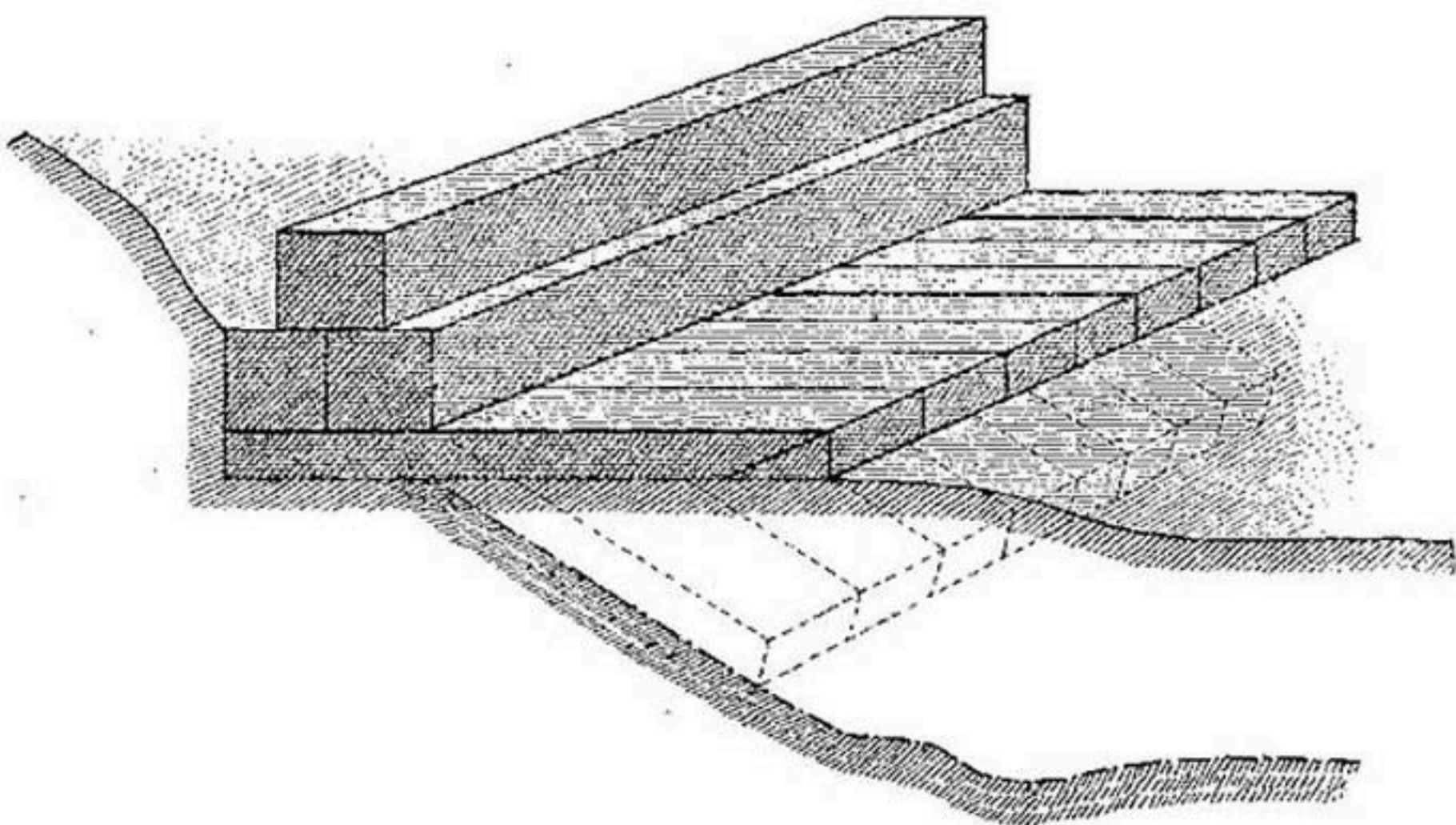
Рис. 134. Кладка из габионов в берегоукрепительных сооружениях.
