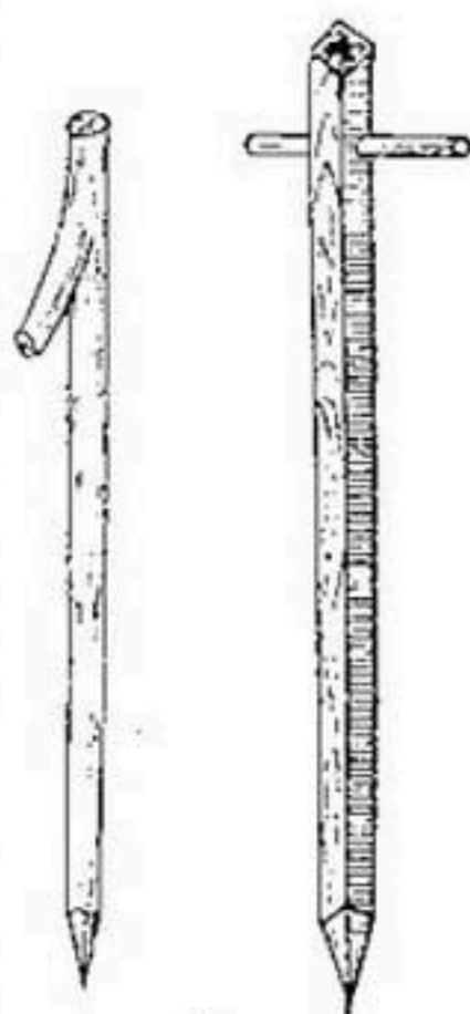
Рис. 95. Колья для закрепления фашин и прутяных канатов в фашиновой кладке.
