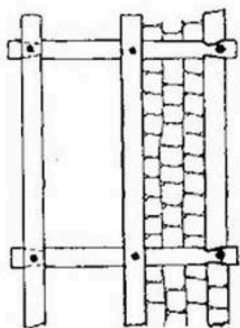
Рис. 270. Укрепление откосов русла на конической высыпке.
