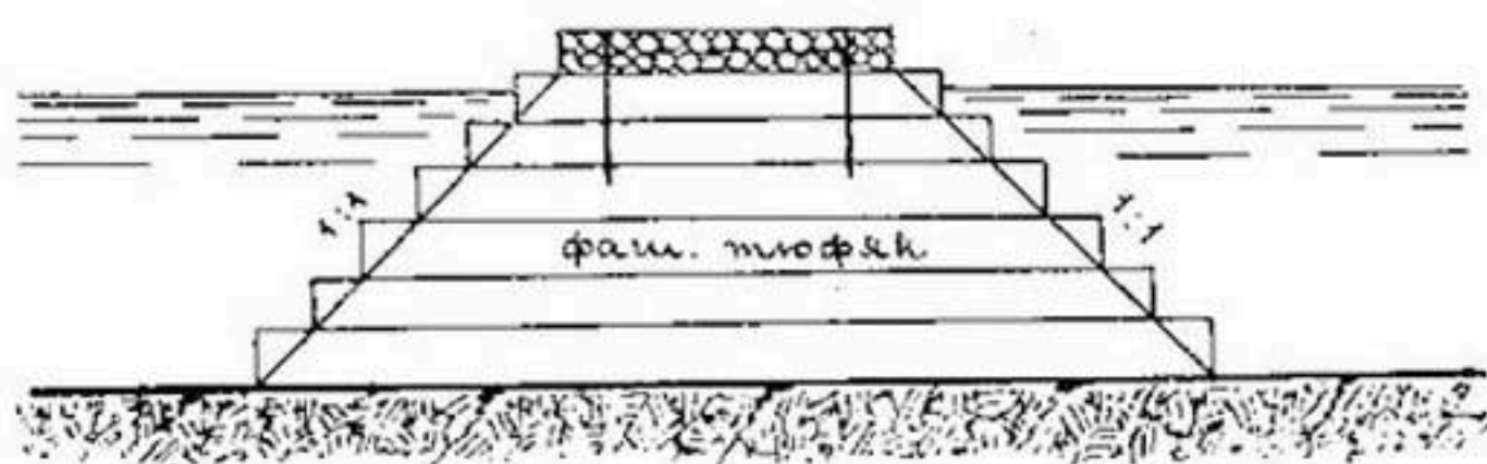
Рис. 203. Запруда из нескольких слоев фашинных туюфов.
