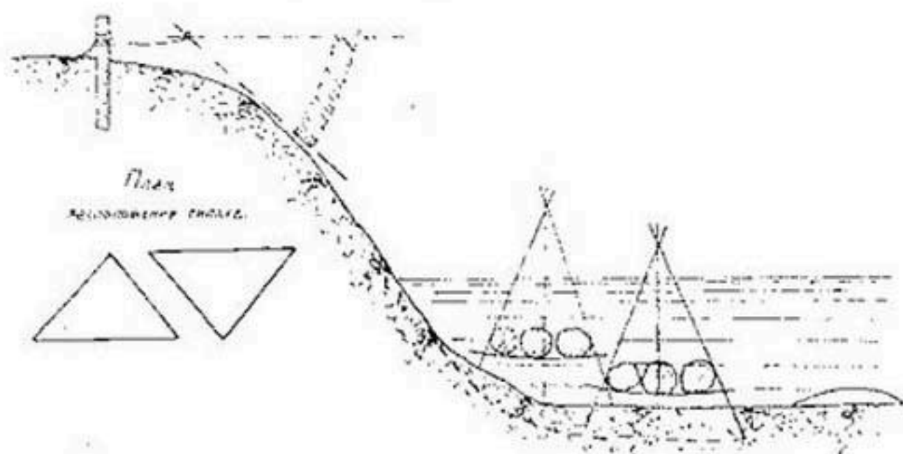
Рис. 149. Сипайное укрепление берега. Установка сипаев.
