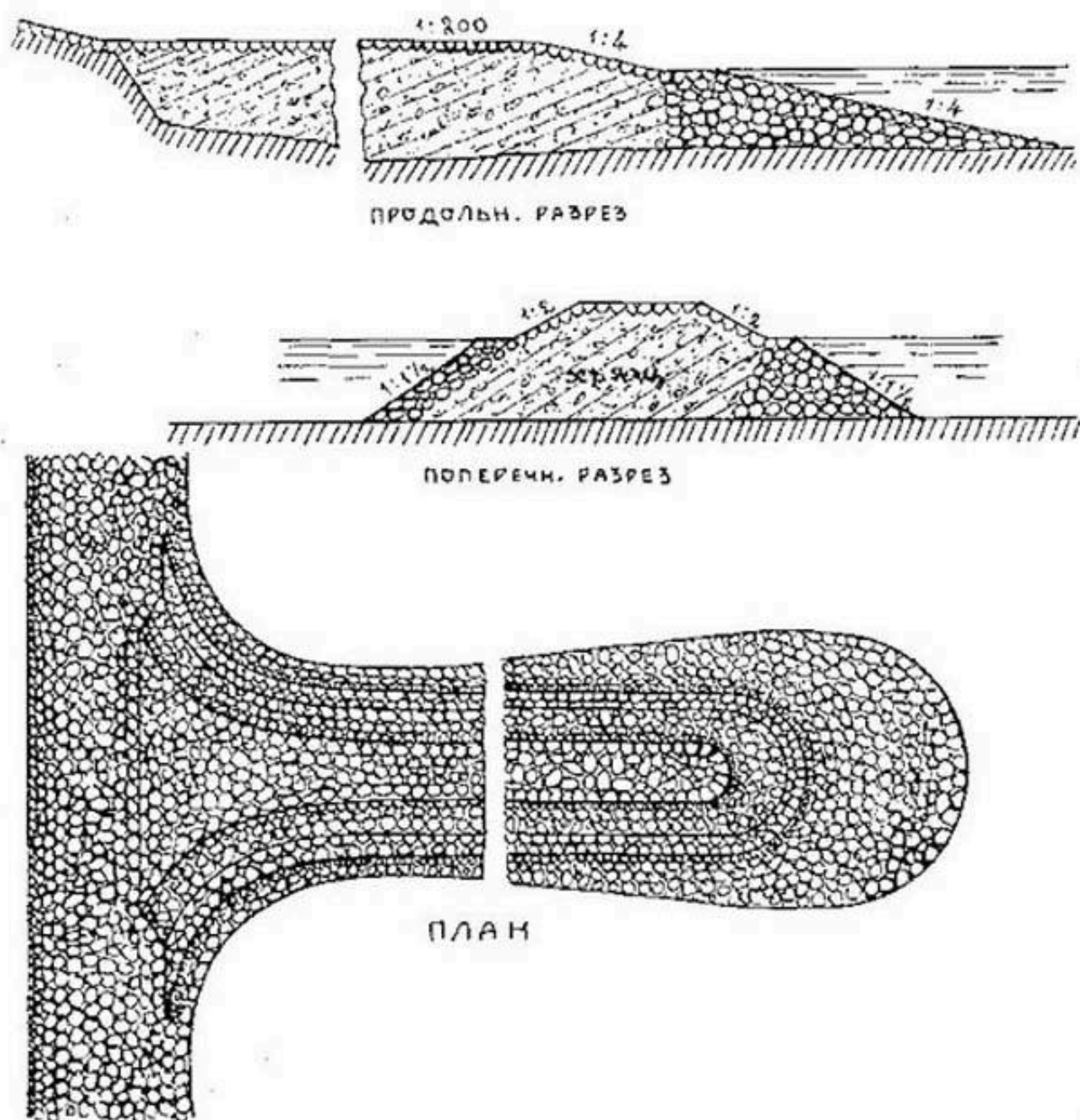
Рис. 172. Конструкция каменной полузапруды на р. Рейне.
