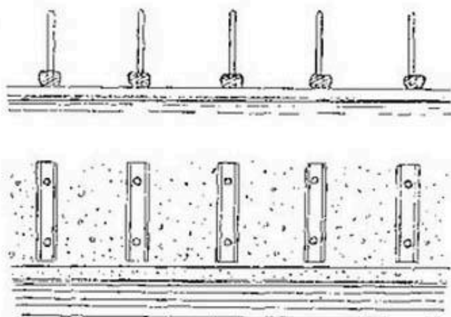
Рис. 99. Установка станков для изготовления тяжелой фашины.
