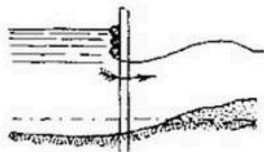
Рис. 225. Неподвижный щит системы Вольфа.
