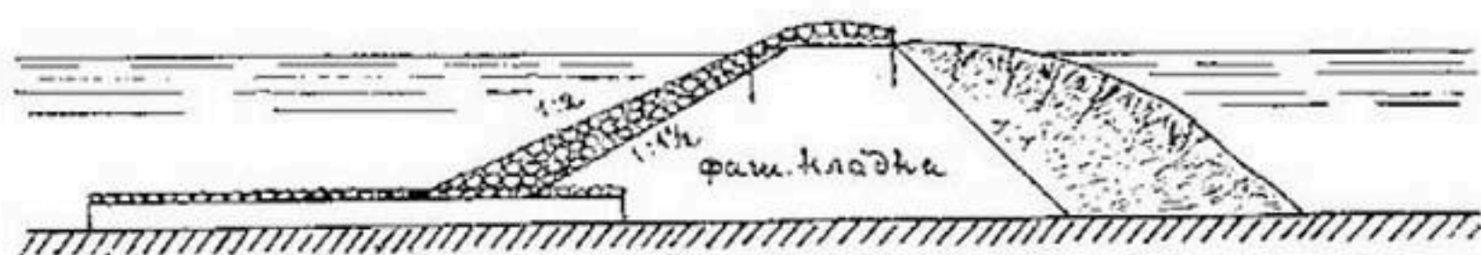
Рис. 179. Тип продольной дамбы на р. Западной Двине.
