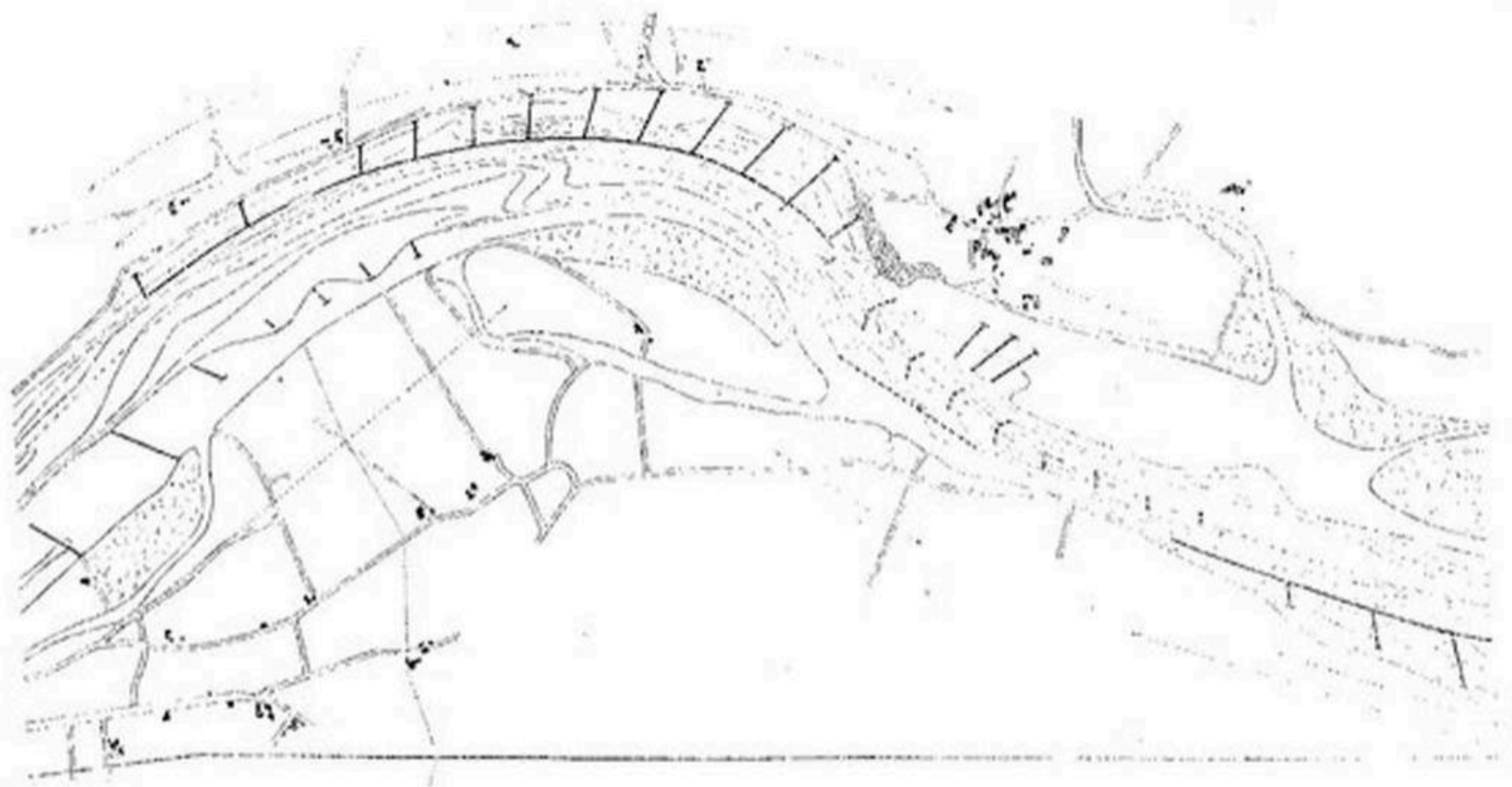
Рис. 55. Регуляционные сооружения на Свент-Албанском перекате р. Роны (течение слева направо по рисунку).
