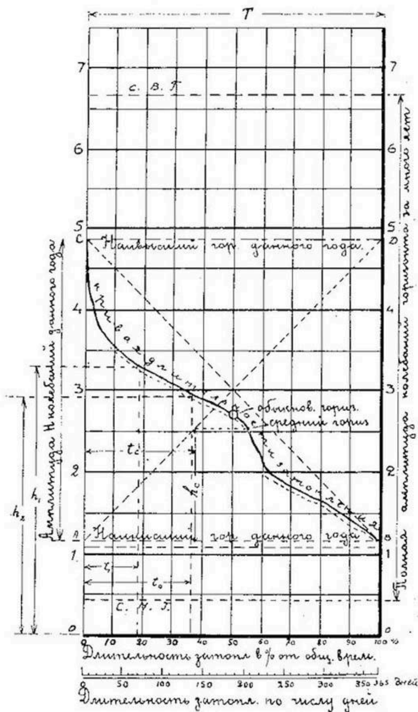
Рис. 4. График длительности покрытия (затопления) горизонтов.
