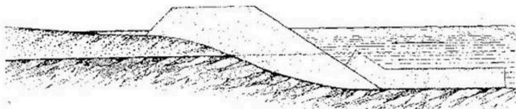
Рис. 184. Продольная дамба, расположенная вблизи берега.
