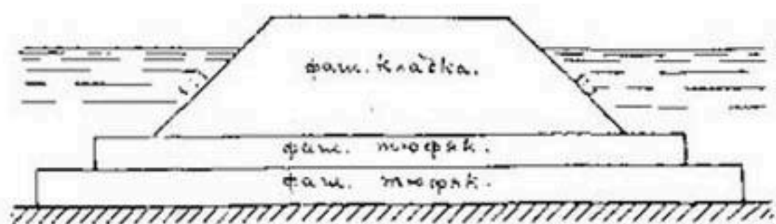
Рис. 167. Тюфячное основание полузапруды.
