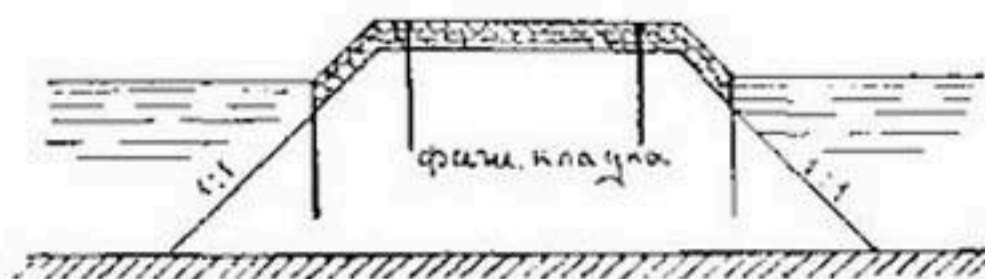
Рис. 170. Укрепление гребня полузапруд на р. Западной Двине.
