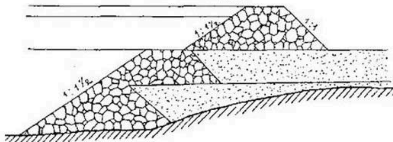
Рис. 187. Продольная дамба, построенная в виде призм из каменной наброски.
