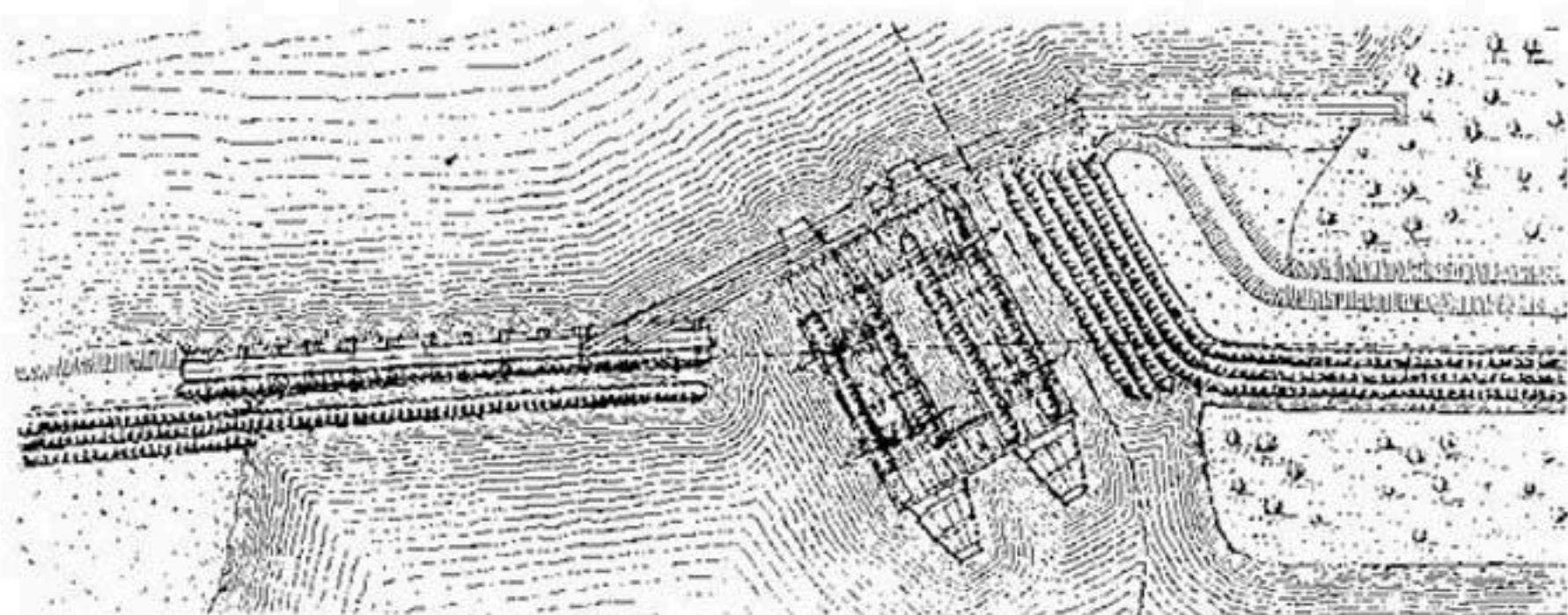
Рис. 213. Замкнутие отверстия во входе в старое русло помощью погружки тяжелых фашин с плавучих подмостей.
