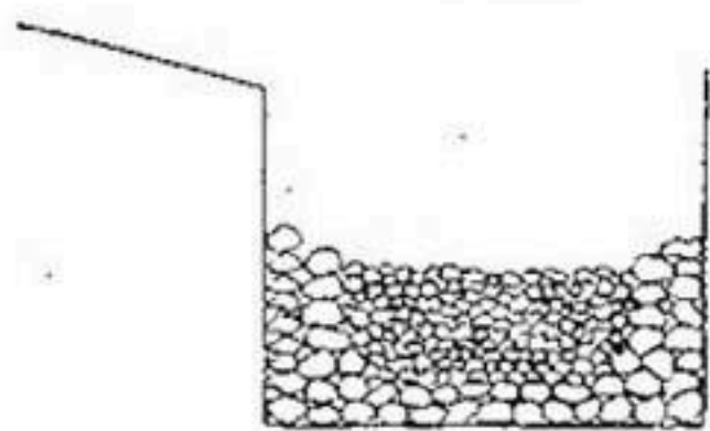
Рис. 88. Заполнение габиона мелким камнем.
