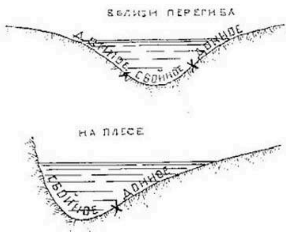
Рис. 57. Расположение сбойного и донного (расходящегося) течения.
