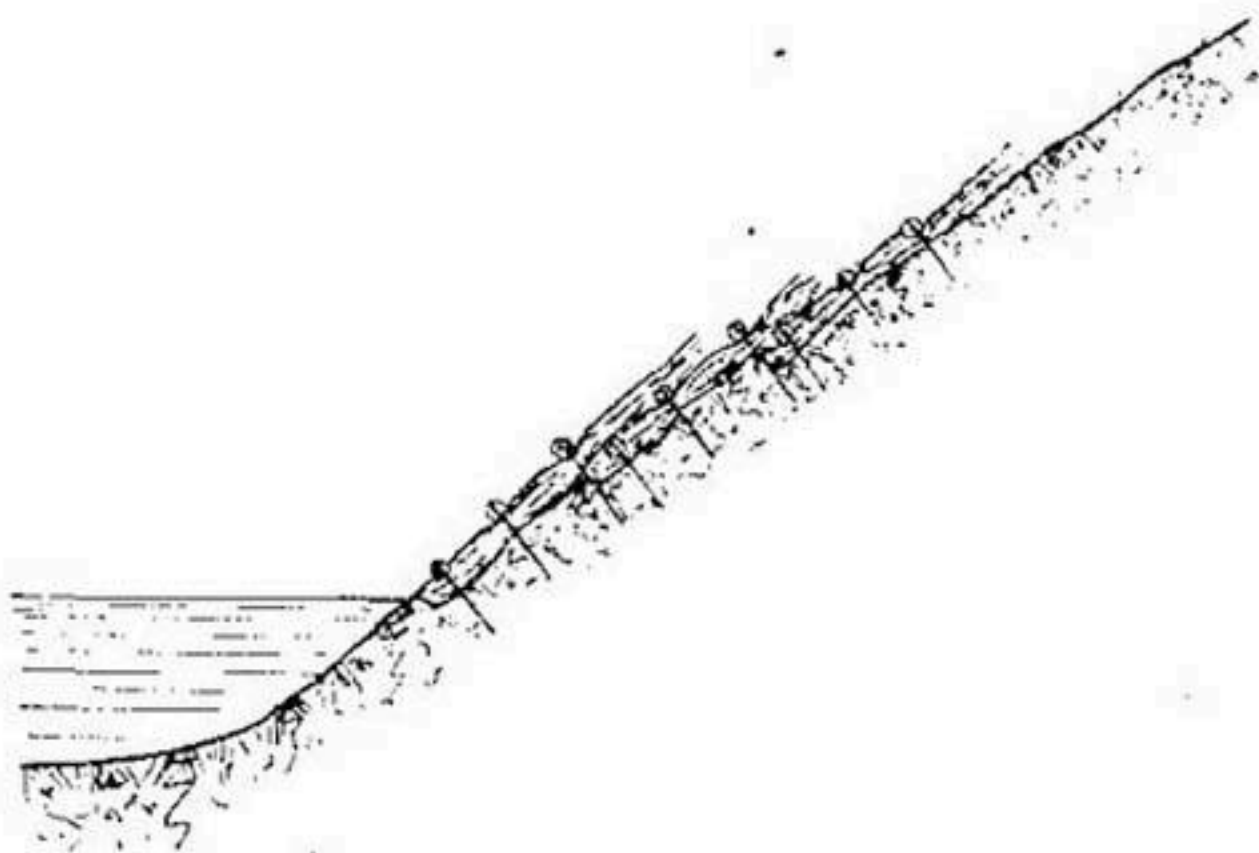
Рис. 155. Поперечная хвостяная выстилка в несколько рядов.
