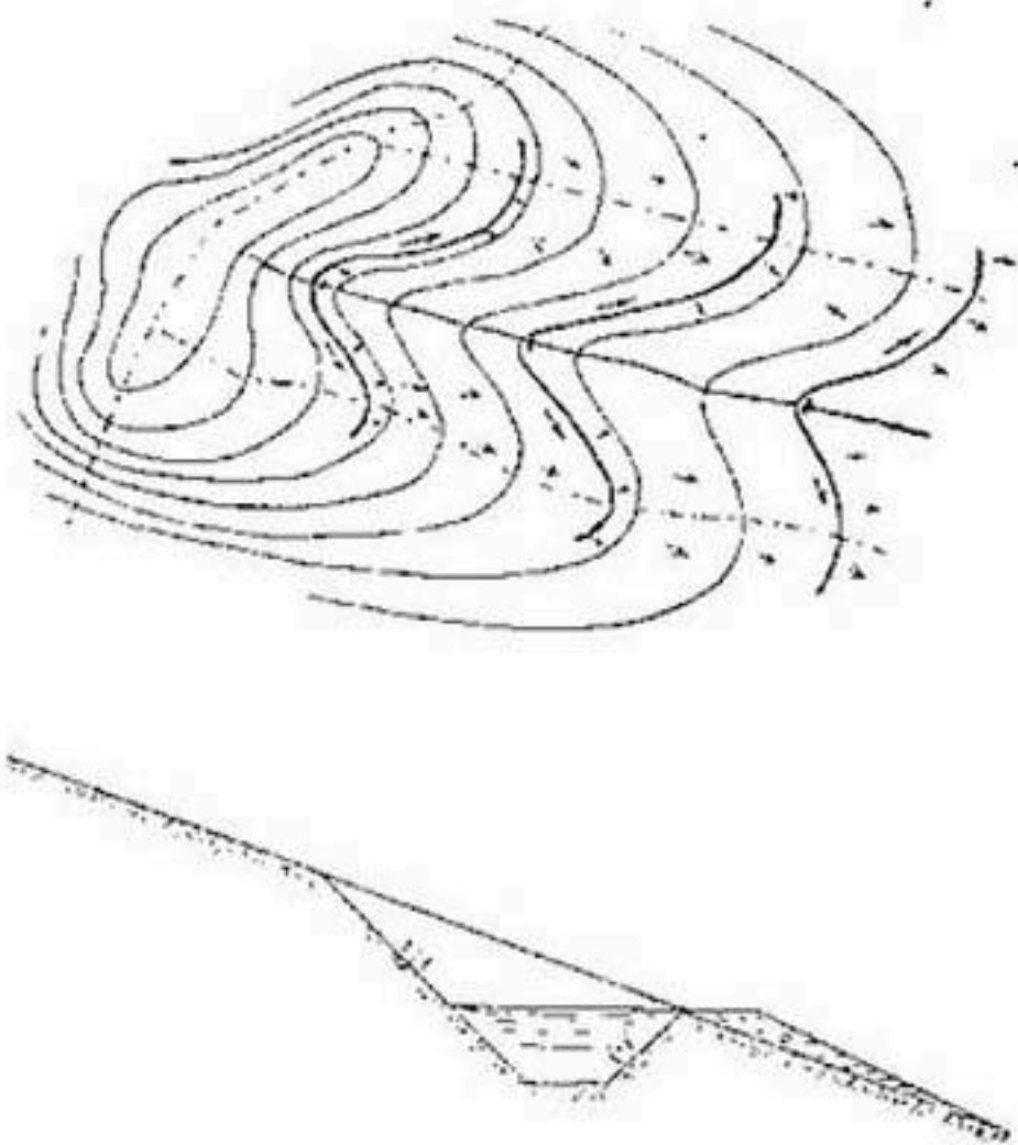
Рис. 246. Ярусные канавы.
