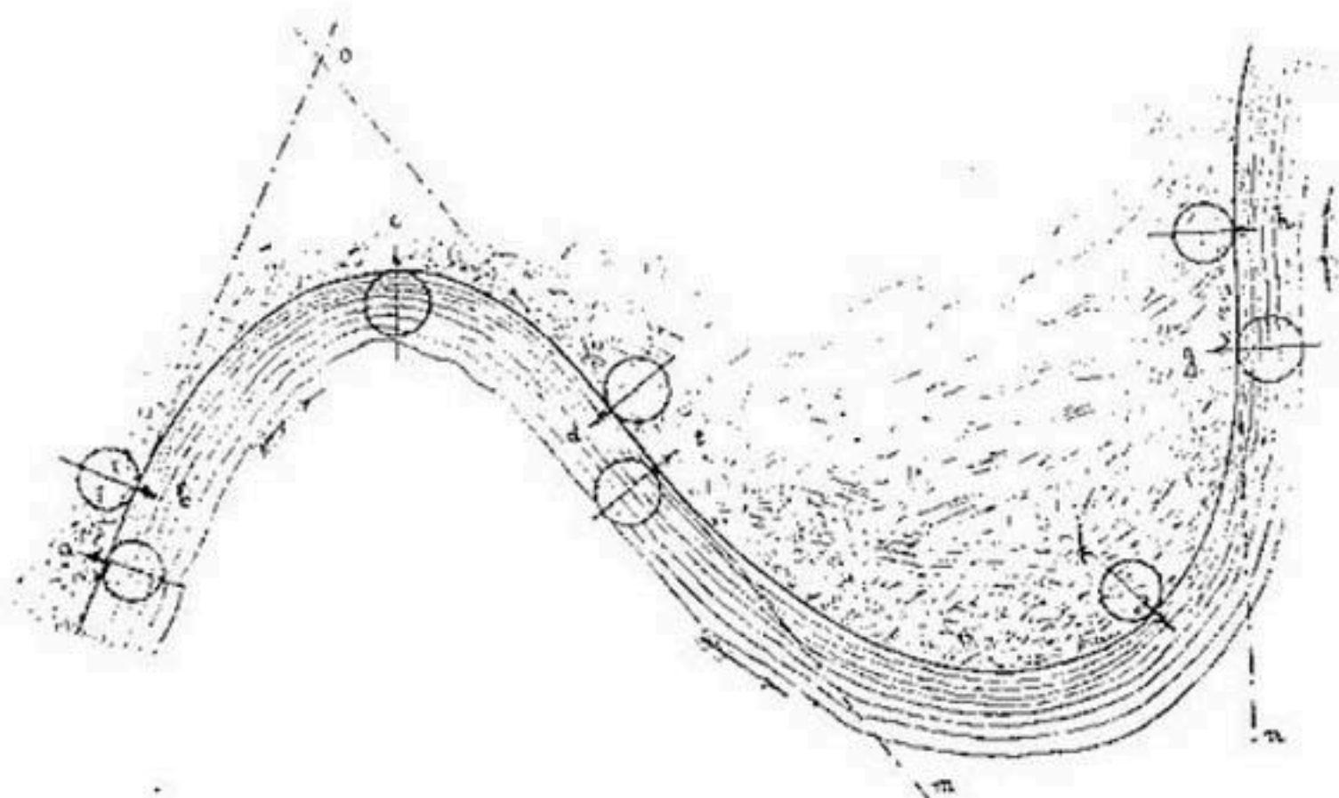
Рис. 121. Начертание линии берега по изгибу упругой линейки.
