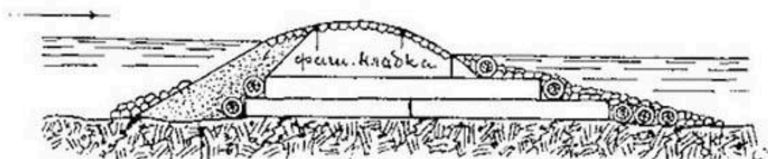
Рис. 205. Укрепление откосов запруды тяжелыми фашинами.
