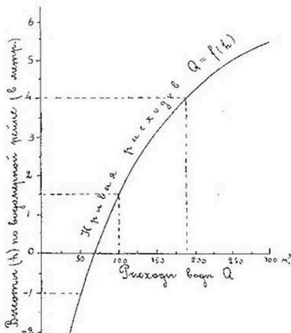
Рис. 10. Кривая зависимости расхода воды от высоты уровня.
