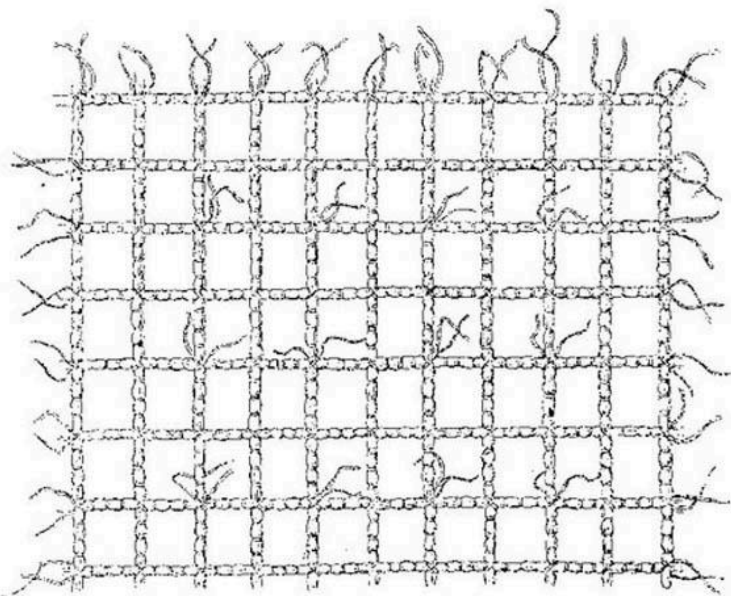
Рис. 103. Нижняя сетка прутяных канатов, служащая для скрепления тюфяка.
