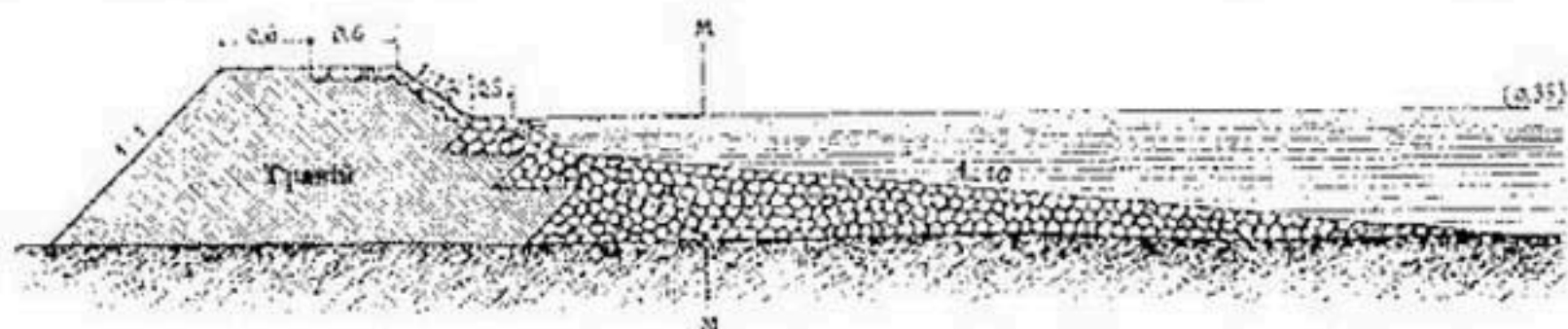
Рис. 194. Каменная донная полузапруда, примкнутая к продольной дамбе.
