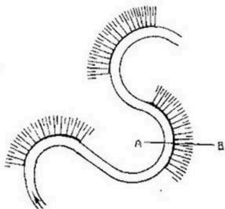
Рис. 251-а. Укрепление откосов ложбины потока (план).
