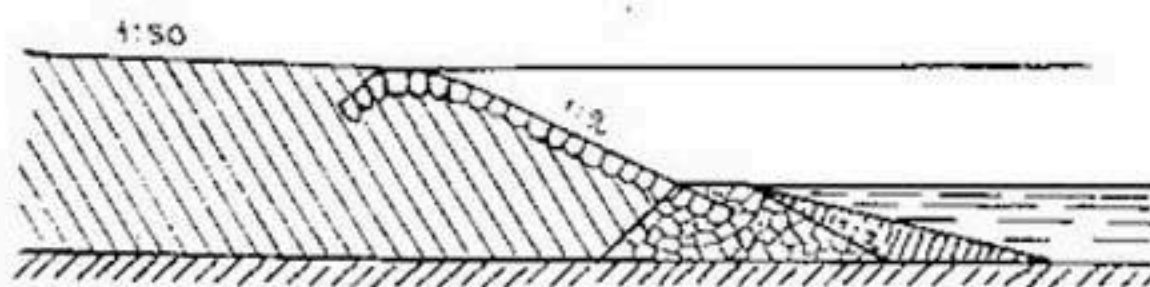
Рис. 190. Каменная продольная дамба в виде береговой опояски.
