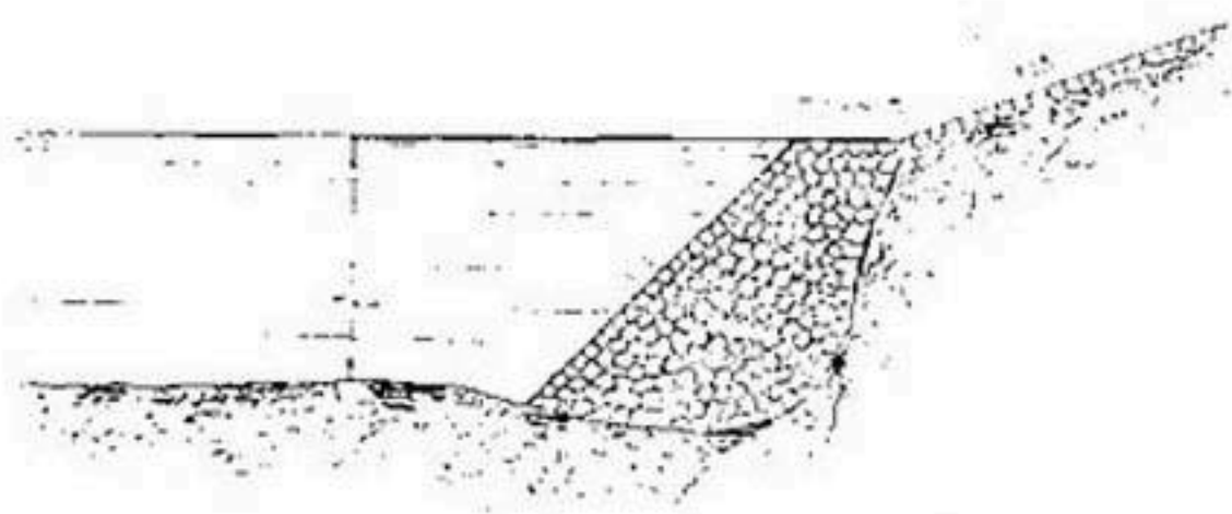
Рис. 128. Укрепление берега призмой каменной наброски.
