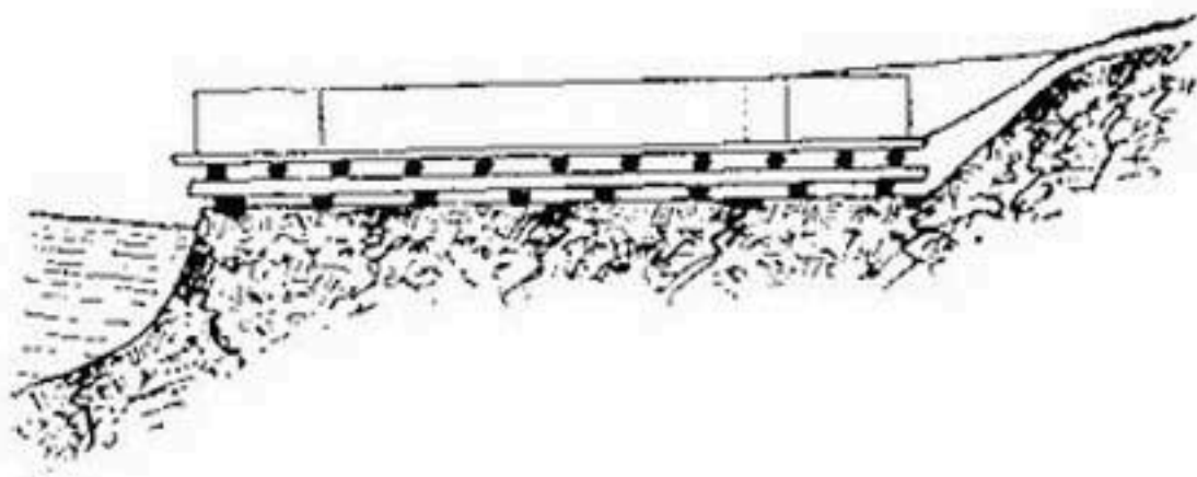
Рис. 106. Подмости для вязки тюфяка на берегу.
