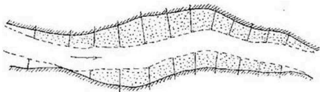
Рис. 47. Выправление русла полузапрудками.
