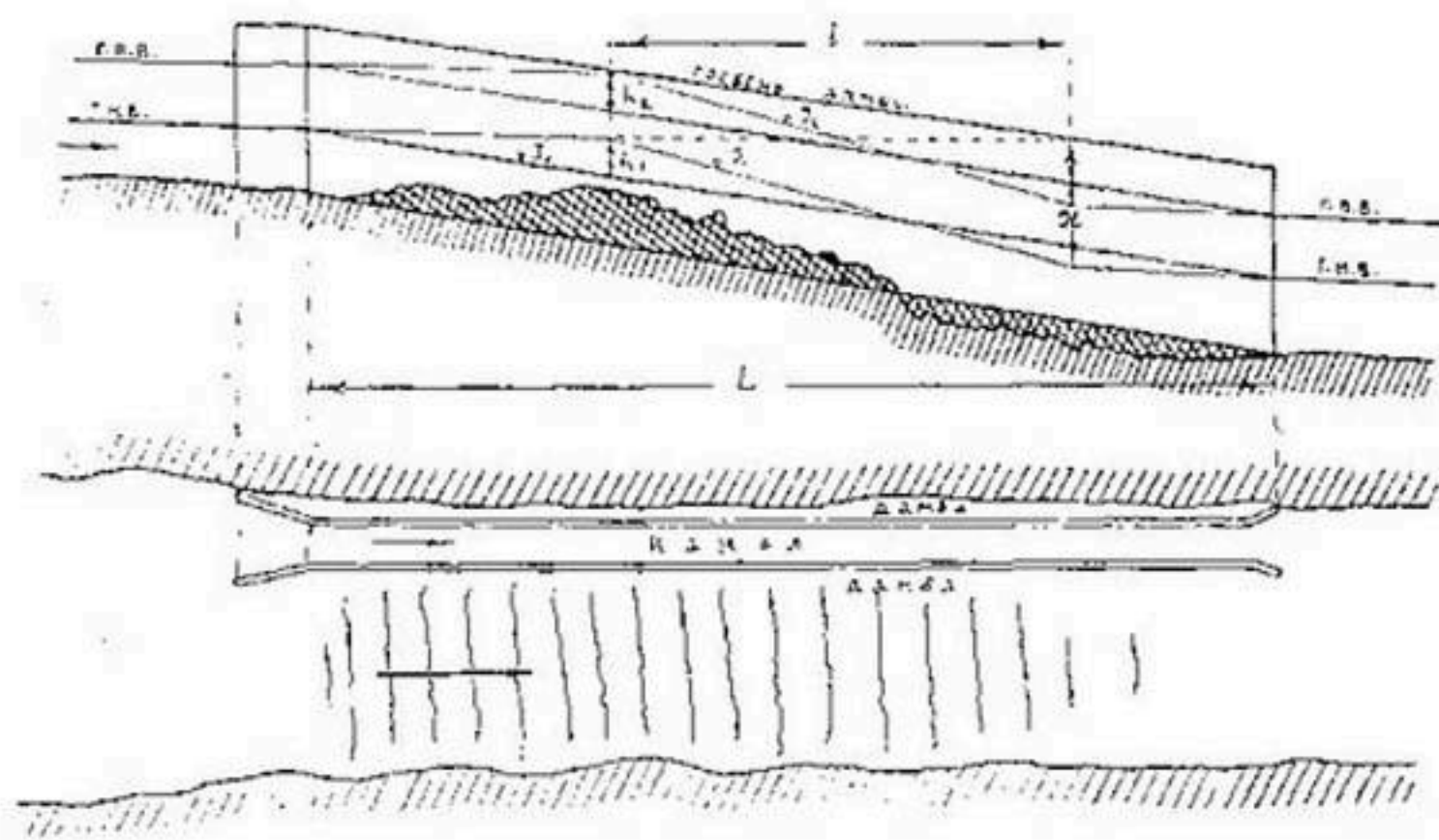
Рис. 74. План и продольный профиль канала, огражденного дамбами.
