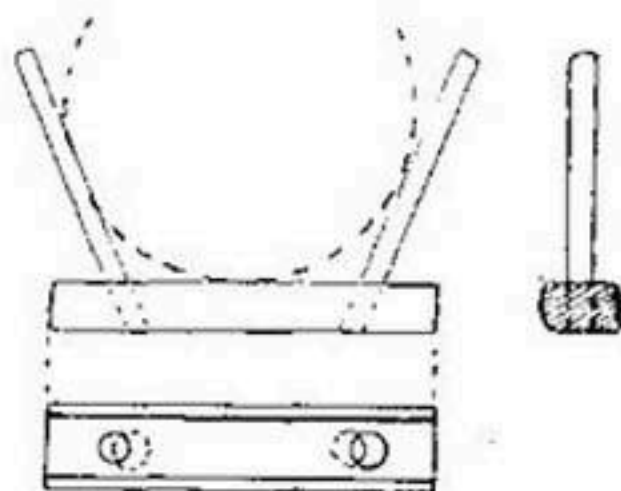
Рис. 98. Конструкции станка для изготовления тяжелой фашины.
