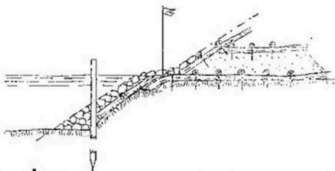
Рис. 230. Закрепление результатов действия щитов Вольфа.
