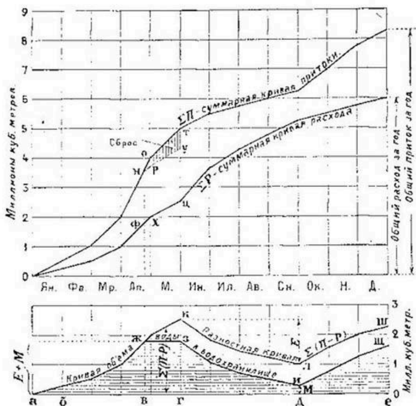
Рис. 275. Графический способ определения необходимой величины полезного объема воды по имеющимся диаграммам приточности и расходования воды.
