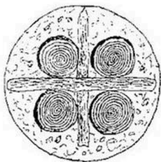
Рис. 248. Жердяные дрены (разрез).
