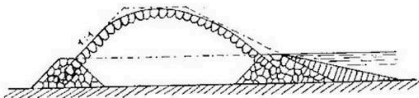
Рис. 188. Продольная дамба, ядро которой сделано из гравия.
