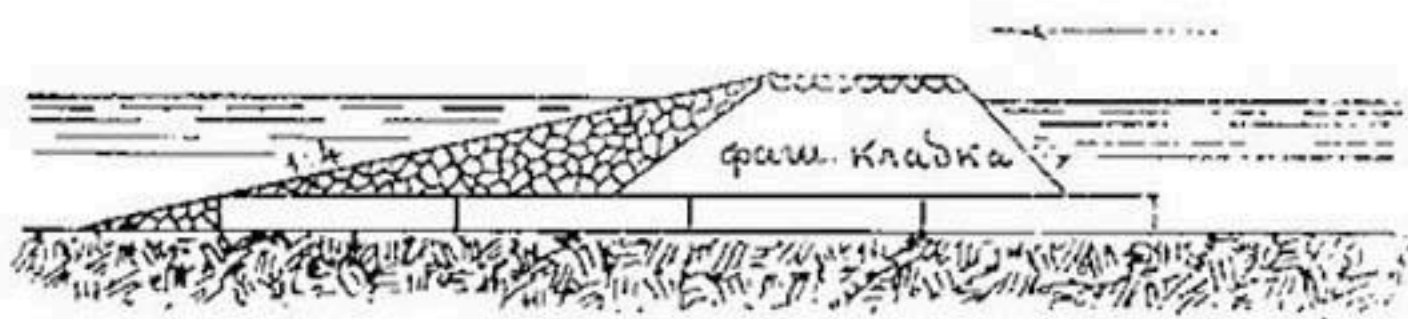
Рис. 204. Укрепление низового откоса запруды каменной наброской.
