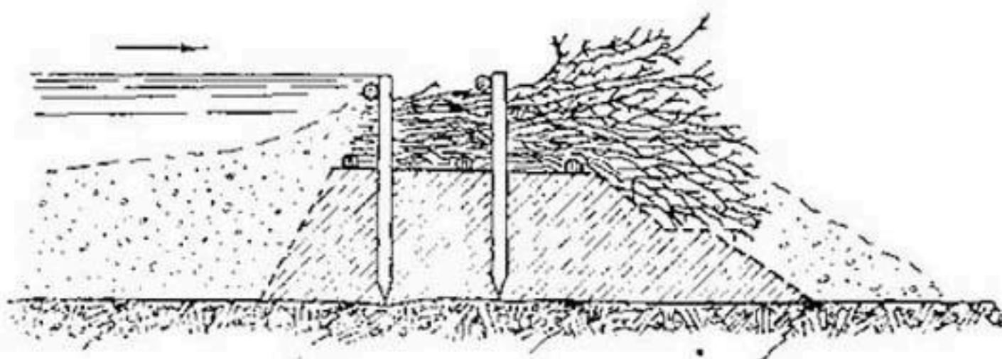
Рис. 224. Фашиновые траверсы-илоудержатели на р. Инне.
