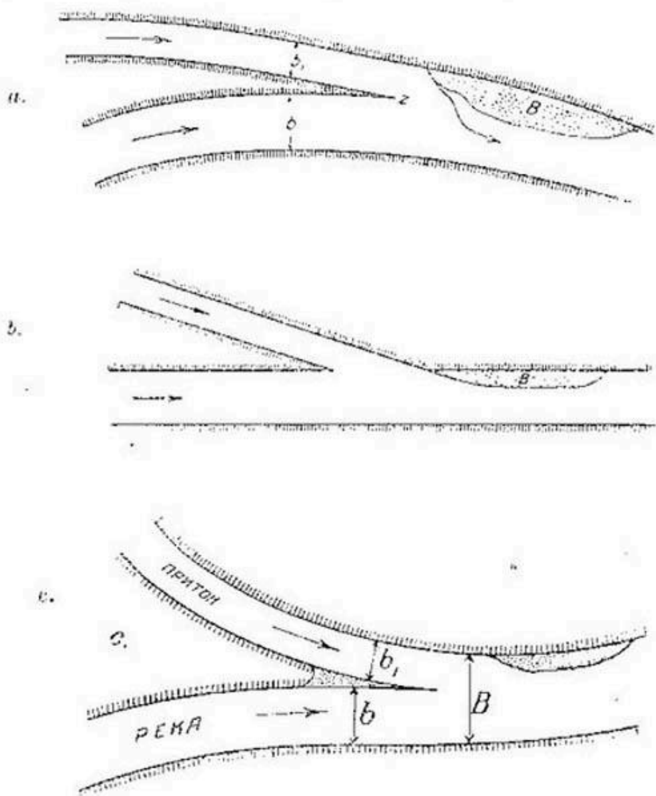
Рис. 70-а, б, с. Типичные формы сопряжения русла реки и притока.
