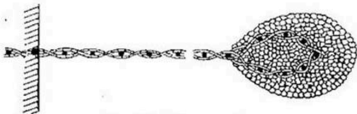
Рис. 216. Плетневой илоудержатель.
