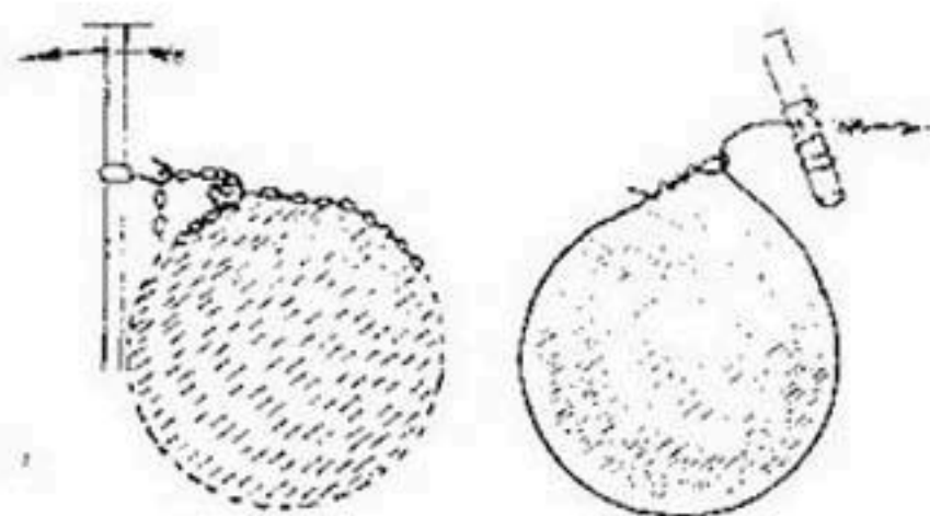
Рис. 97. Затяжка тяжелой фашины проволокой.
