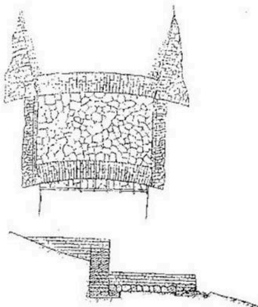
Рис. 256. Конструкция водобойного пола запруды с передовым порогом.
