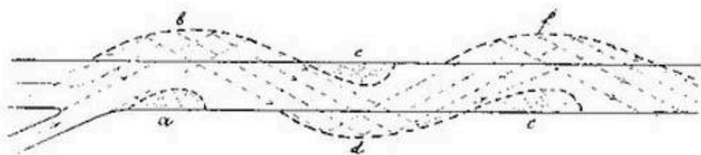
Рис. 17. Извилины реки.
