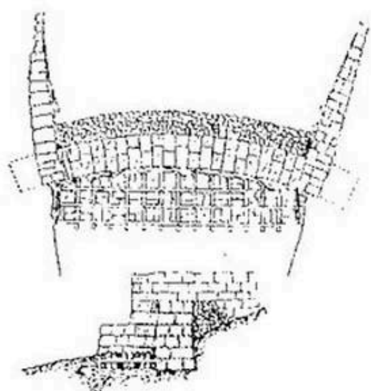
Рис. 254. Водобойный пол каменного порога, сделанный из выстилки крупного камня в жердяной клет.
