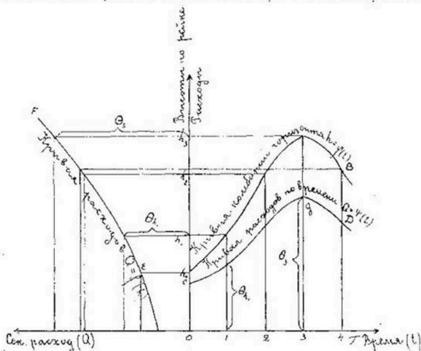
Рис. 13. Совмещенный график колебаний уровня и расхода воды.
