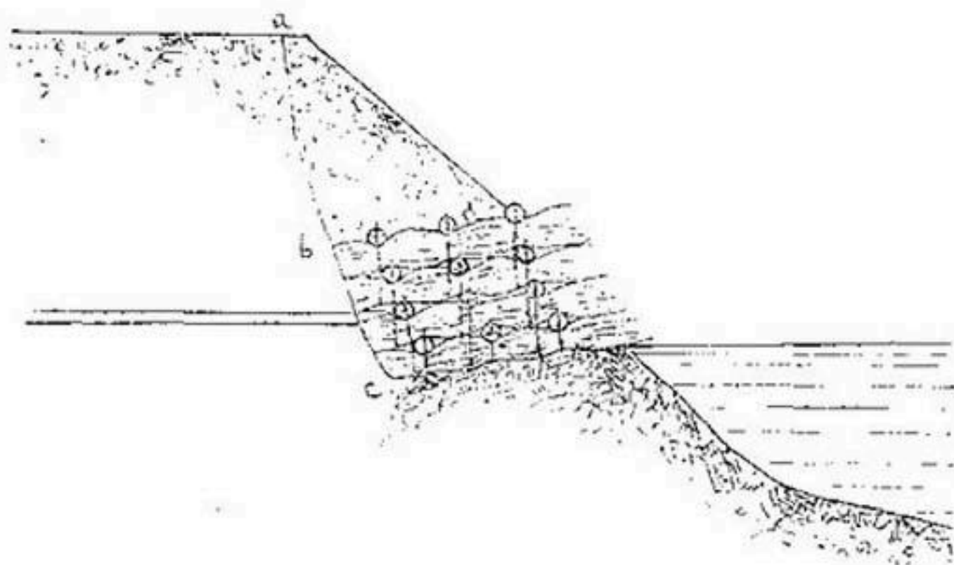
Рис. 157. Хворостяная кладка в стенку.
