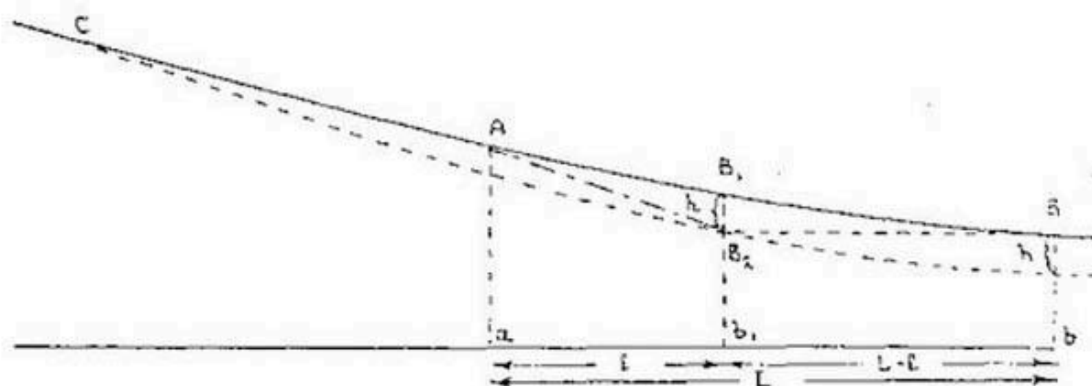
Рис. 63. Влияние прокопа на поверхность воды в случаях размываемого грунта.
