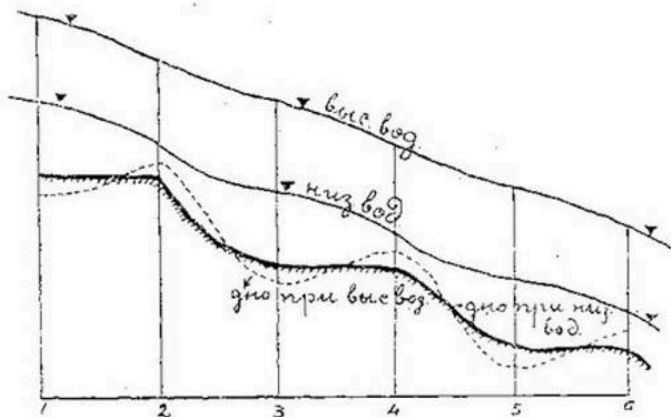
Рис. 24-б. Продольный профиль реки по стрежню.
