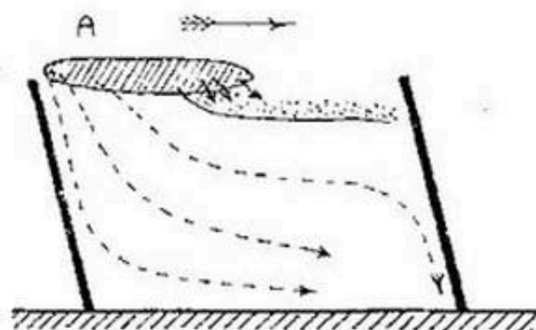
Рис. 166. Развитие вымоин и наносов при высокой воде.
