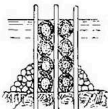
Рис. 221. Буна-плоудержатель, построенная из длинных фашин.
