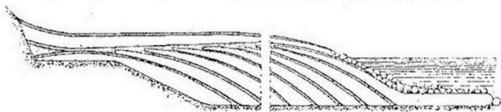
Рис. 115. Разрез сооружения из веерной фашиновой кладки в готовом виде.
