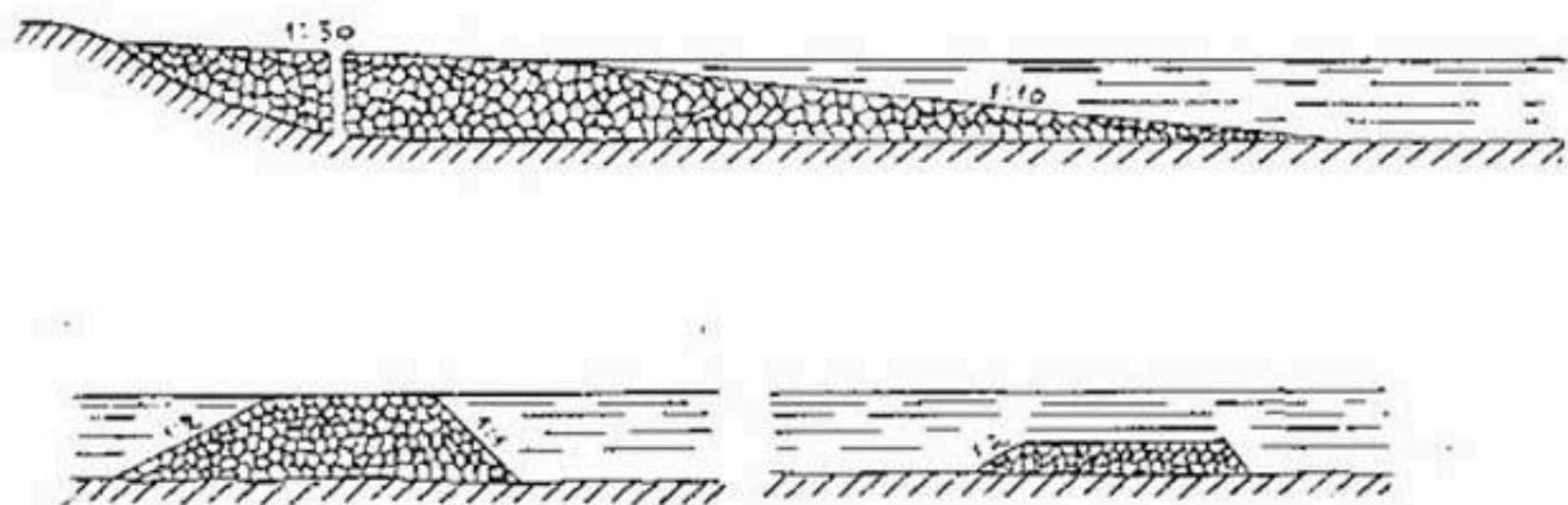
Рис. 193. Донная полузапруда, выведенная от берега.
