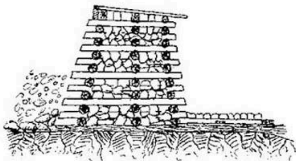
Рис. 264-б. Поперечный разрез.
