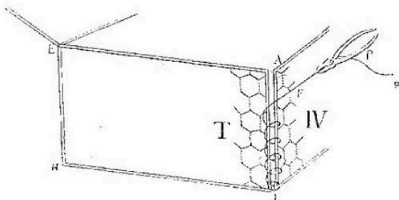
Рис. 85. Скрепление проволокой (p) ребер габионного ящика. Стягивание проволоки производится клещами (P).
