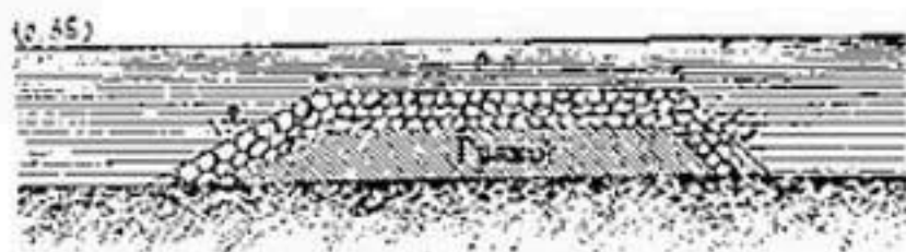
Рис. 195. Поперечный разрез донной полузапруды.
