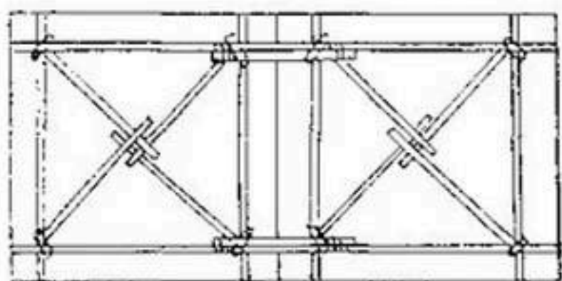
Рис. 192. Соприжение между собой четырехугольных сипаев.
