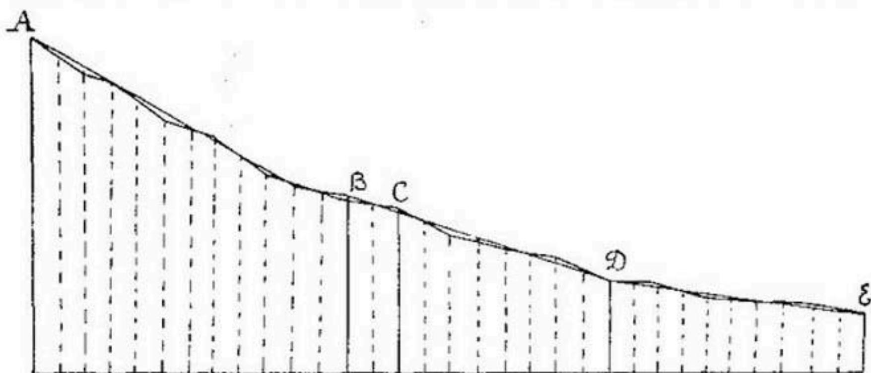
Рис. 7. Продольный профиль поверхности воды реки.
