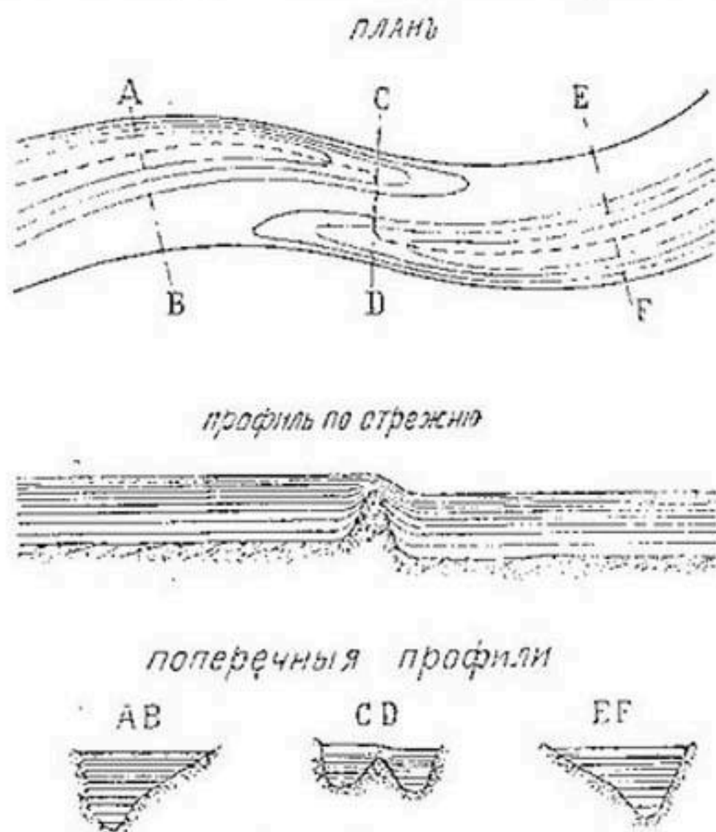
Рис. 54-а. Тип 1-й—(плохой перекаат).
