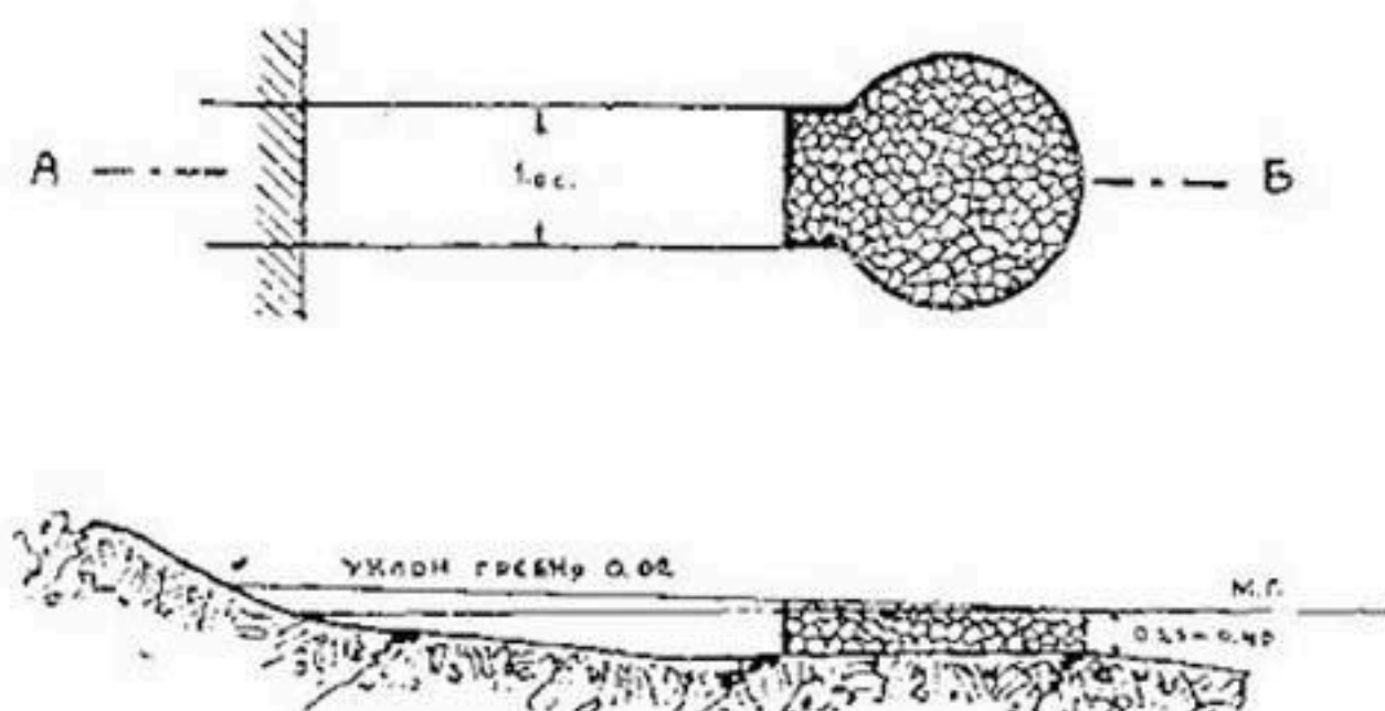
Рис. 218. Плетневые полузапруды на р. Днепре. Устройство головной части.
