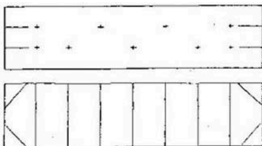
Рис. 87. Связи габионного ящика.
