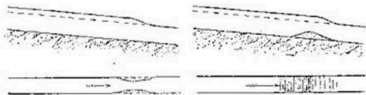
Рис. 295. Подпор, вызванный обмелением дна или сужением русла.
