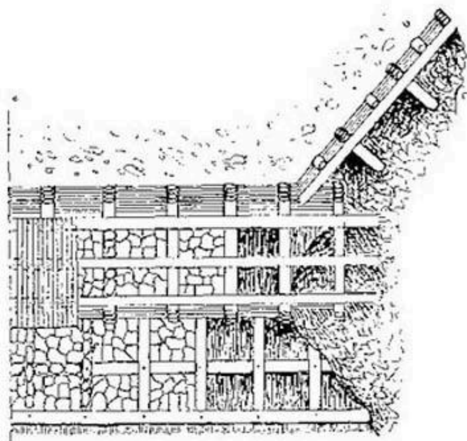
Рис. 264-а. План.
