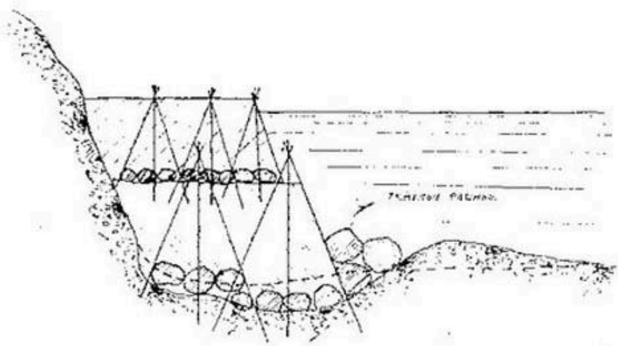
Рис. 150. Укрепление берега сипаями в два яруса.
