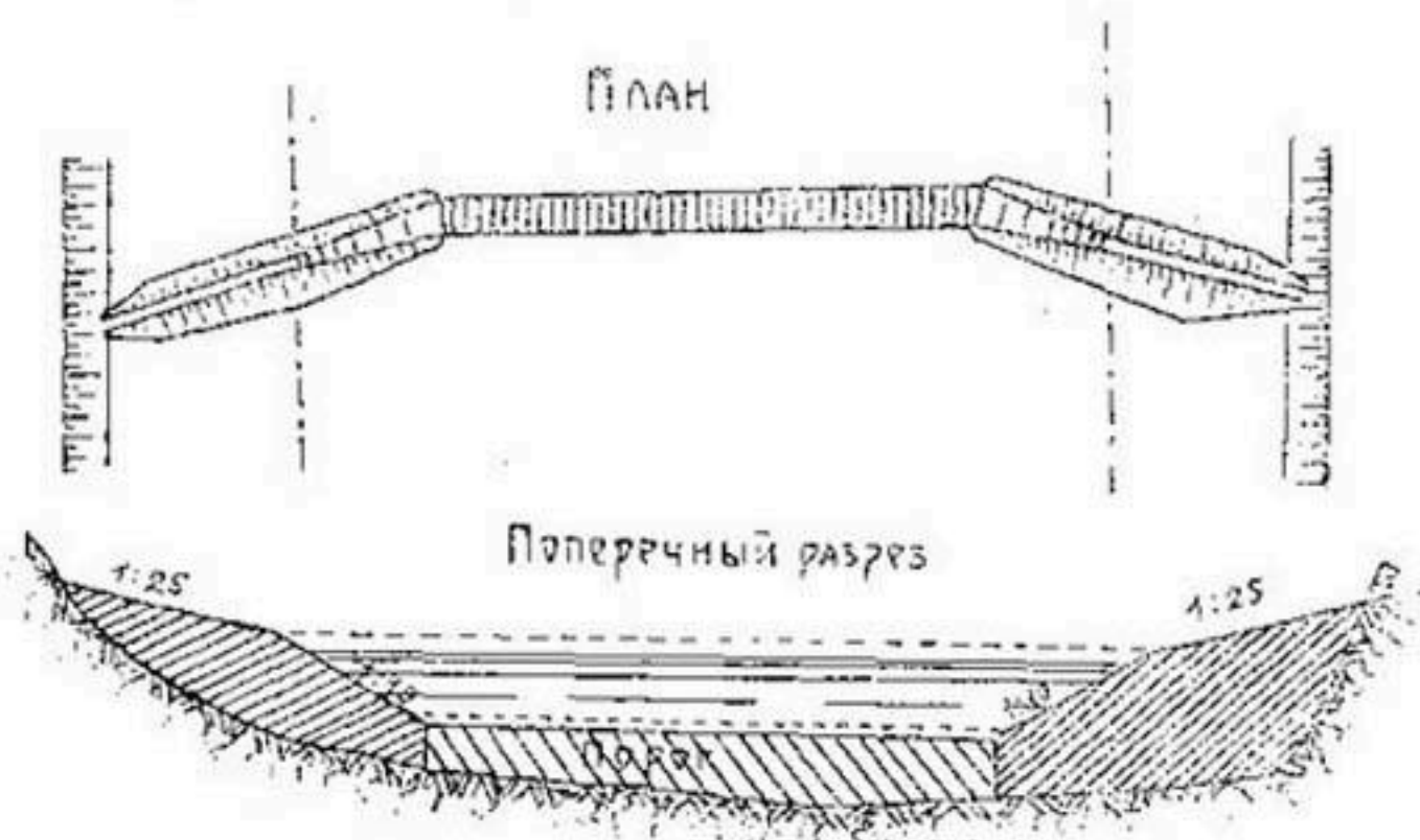
Рис. 53. Донная запруда (порог), сопряженная по концам с донными полузапрудами
