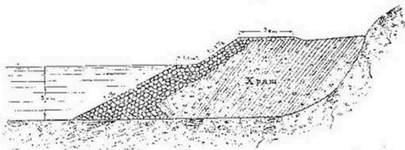
Рис. 131. Укрепление берега каменной наброской с ядром из хряща.
