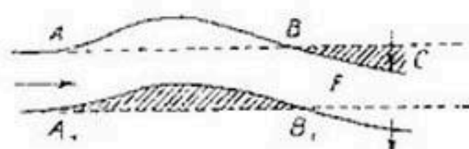
Рис. 32. Образование наносов около выпуклого берега.
