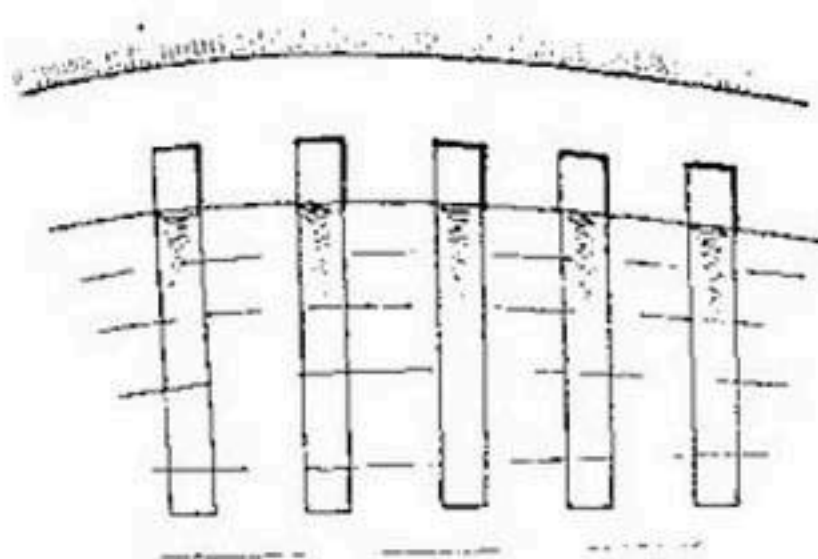
Рис. 140. Ленточное укрепление берега фашинными тюфяками.
