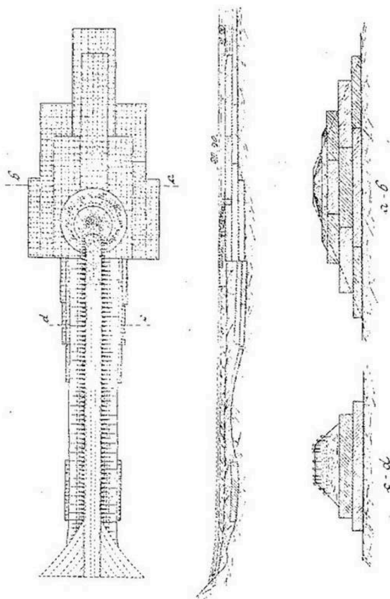
Рис. 198. Донная полузапруда из фашиных тюфяков, приквнутая к голове полузапруды на р. Одере).
