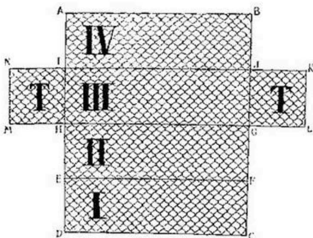
Рис. 84. Развернутый габионный ящик.
