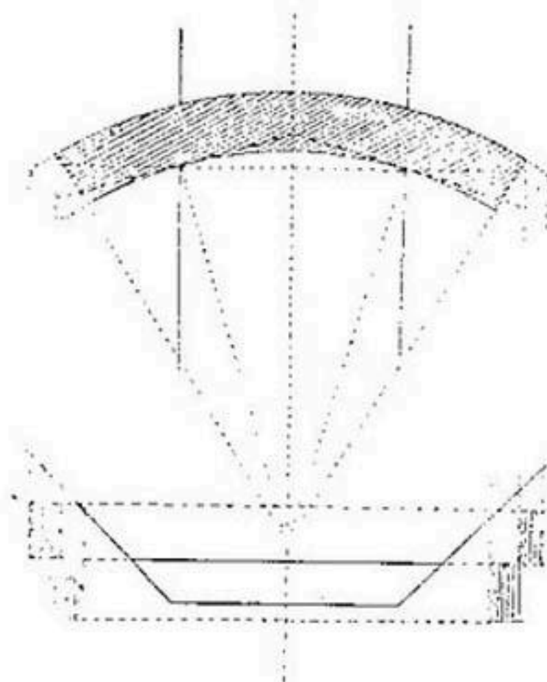
Рис. 253. Заделка в откос скалы пят каждого слоя каменной кладки сводчатого порога.
