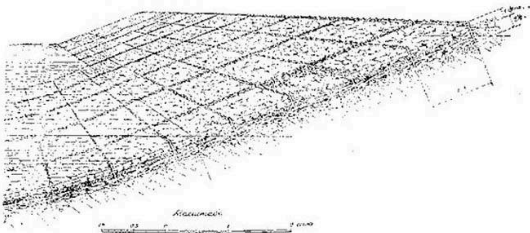
Рис. 160. Плетневые клетки, сделанные на хвостяном тюфяке, покрывающем надводную часть откоса берега.
