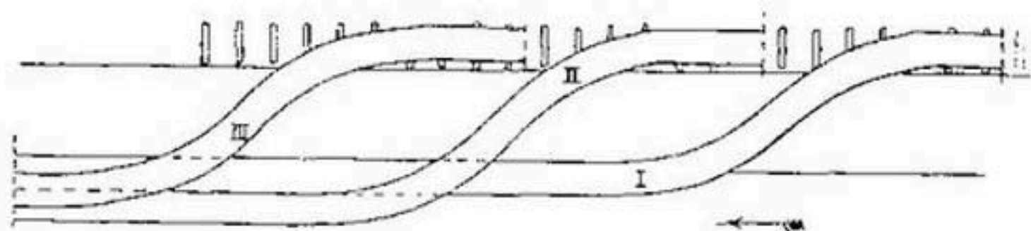
Рис. 102. Вязка и спуск трех тяжелых длинных фашин.
