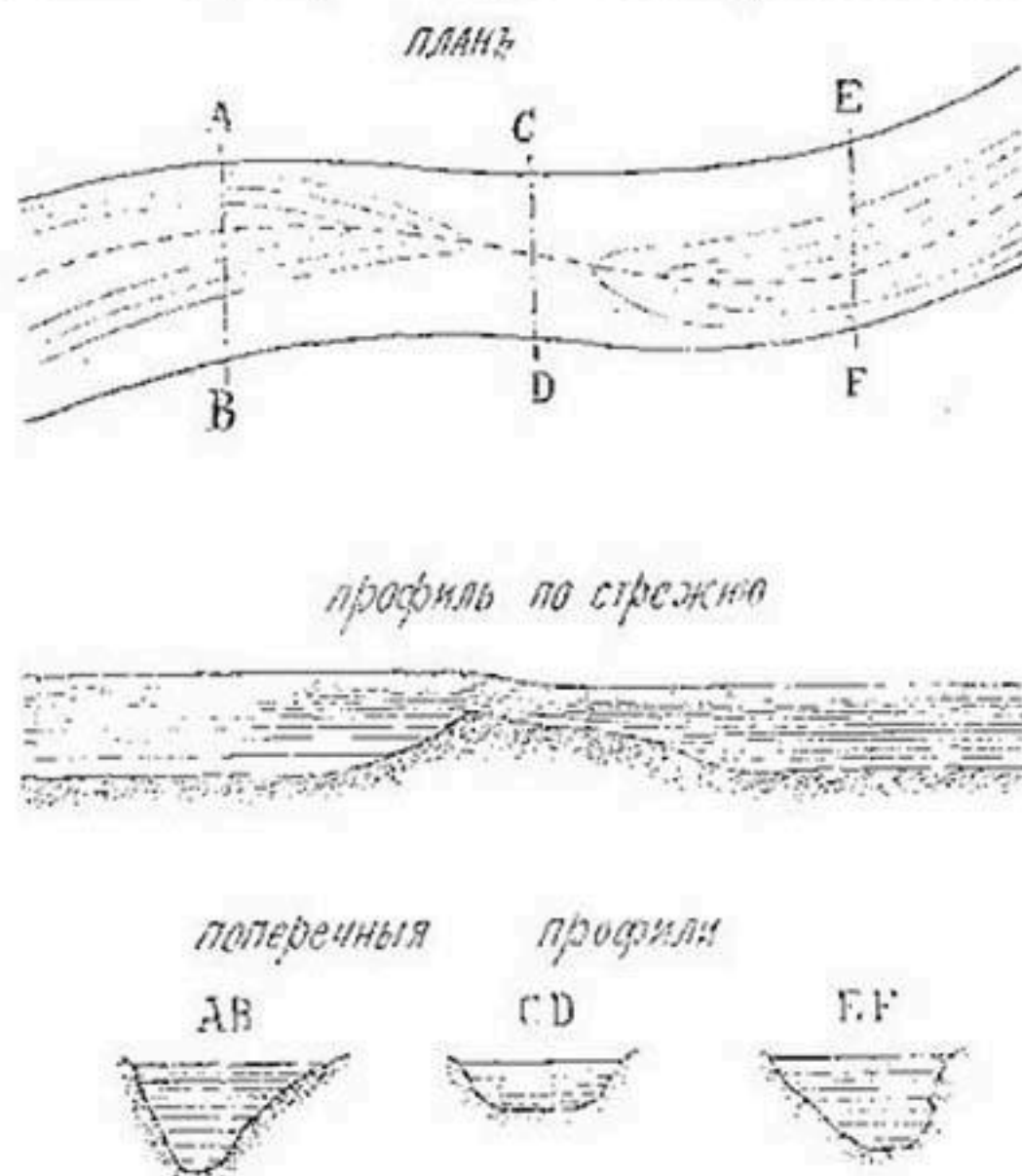
Рис. 54-56. Тип 2-й — (хороший перекаат).
