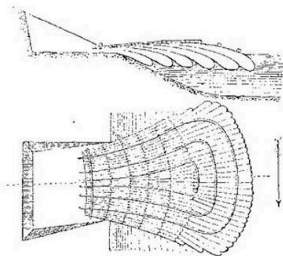
Рис. 113-а и б. Расположение слоев в разрезе и в плане.
