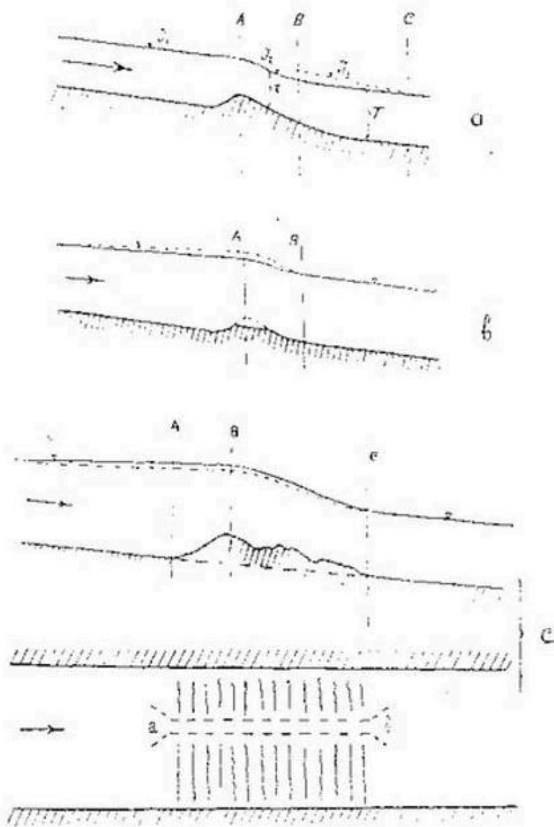
Рис. 73-а, б, с. Регулирование порожистых частей реки.
