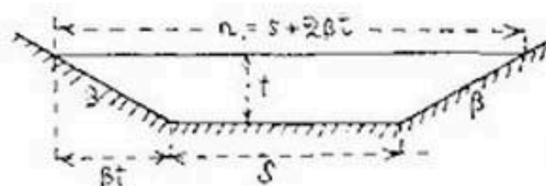
Рис. 40. Трапециoidalное русло.
