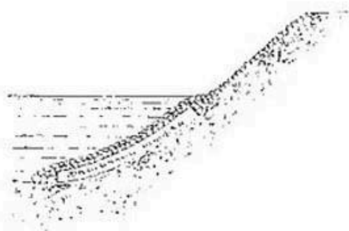
Рис. 136. Укрепление берега фашинным тюфяком.
