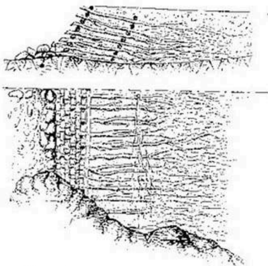
Рис. 261. Запруда из кладки древесных ветвей.
