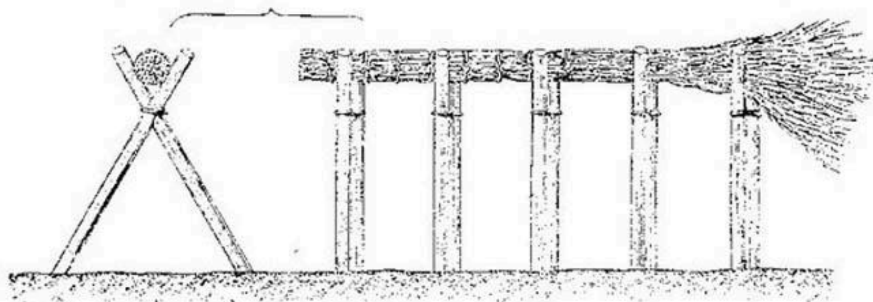
Рис. 90. Вязка фашин.
