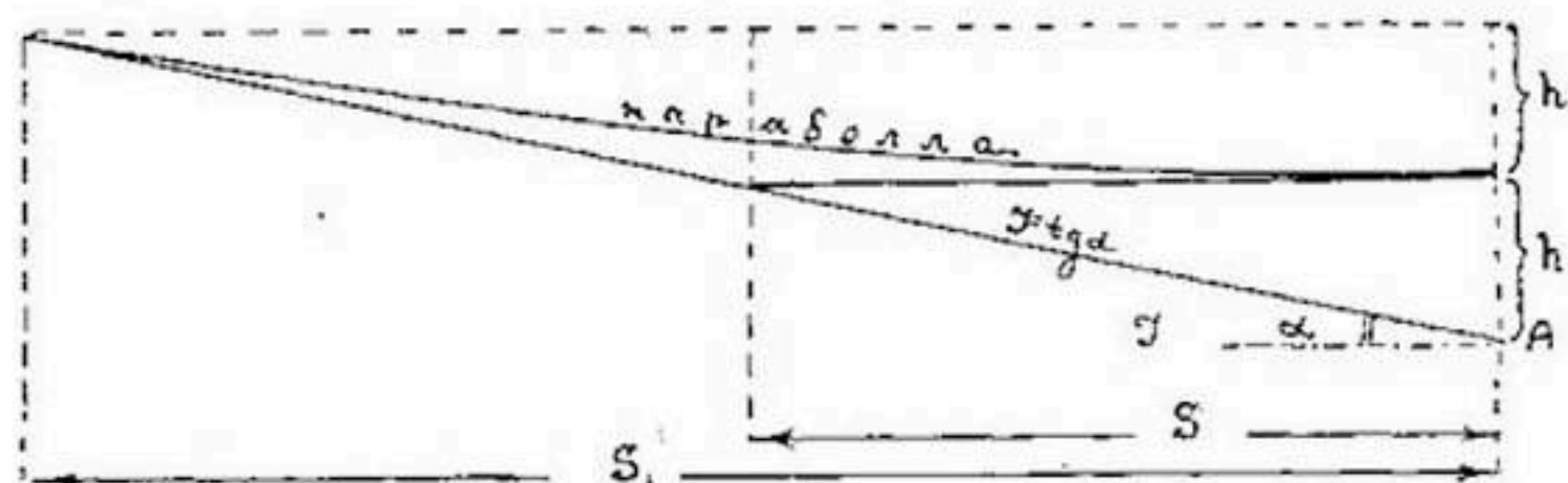
Рис. 62. Кривая подпертого уровня воды.
