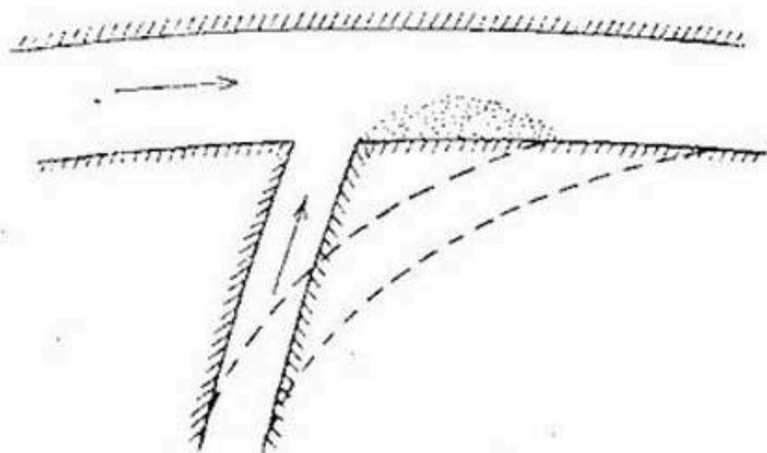
Рис. 69. Регулирование устья притока в местах, где приток впадает в реку под тупым углом.
