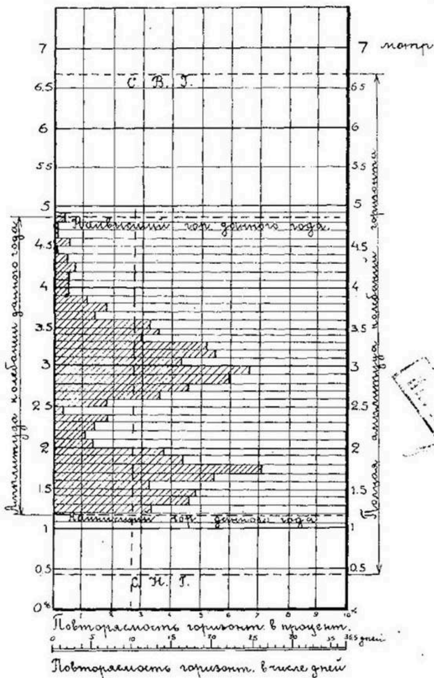
Рис. 3. График частоты повторяемости горизонтов.
