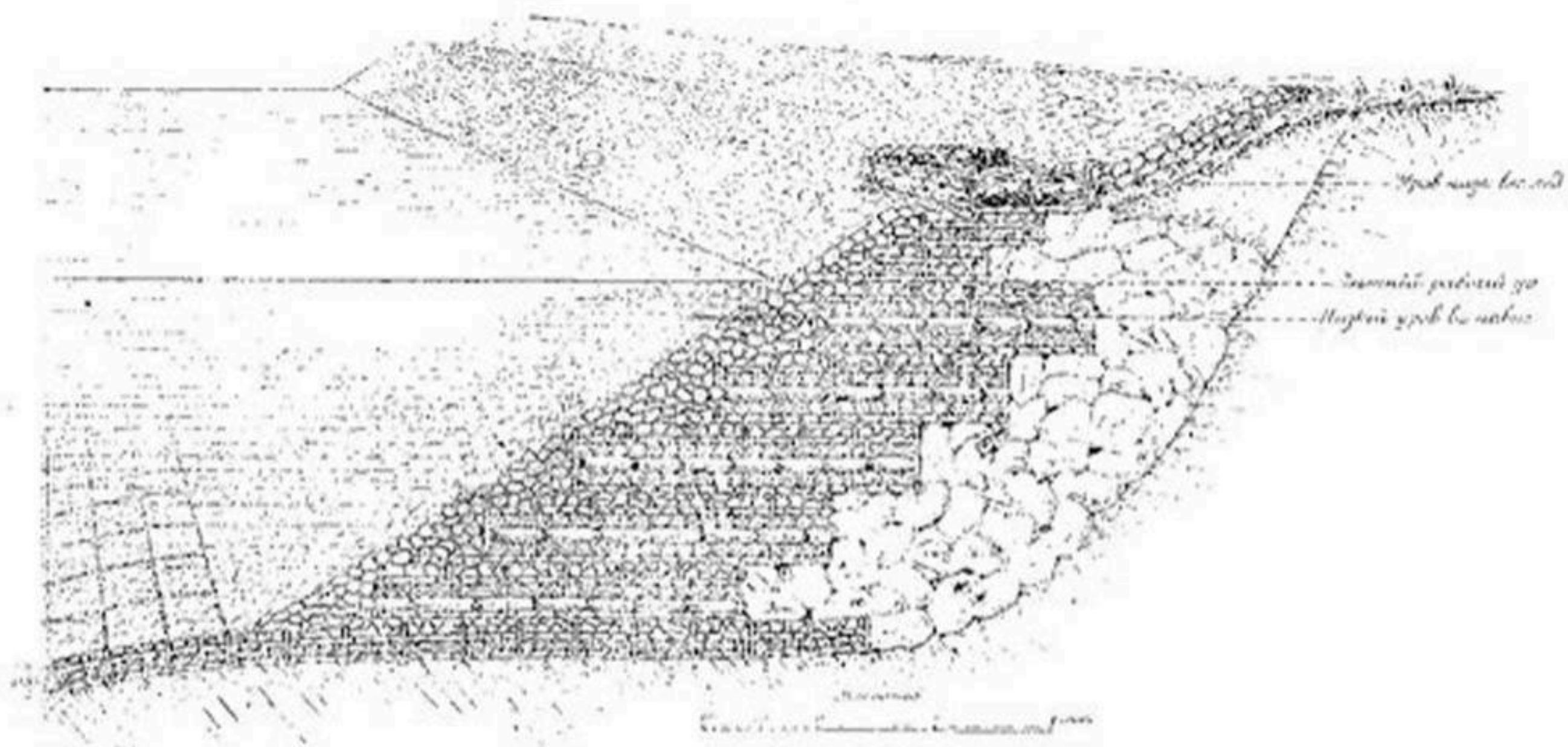
Рис. 148. Укремление берега, в виде оплеса, из кланки фантовых тюфяков на р. Волге.
