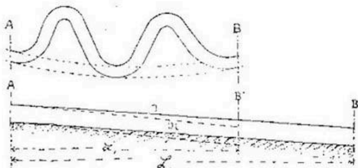
Рис. 296. Влияние спрямления русла на величину уклона.
