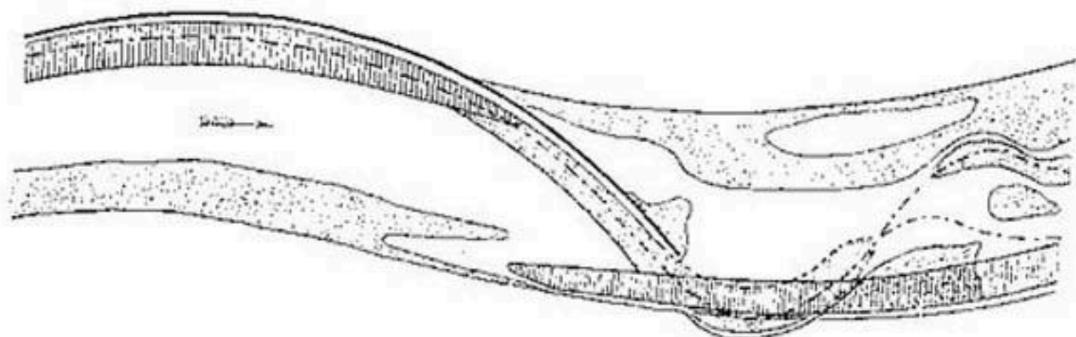
Рис. 58. Теоретически желательное расположение на перекате струенаправляющей дамбы для поддержания сбойного течения.
