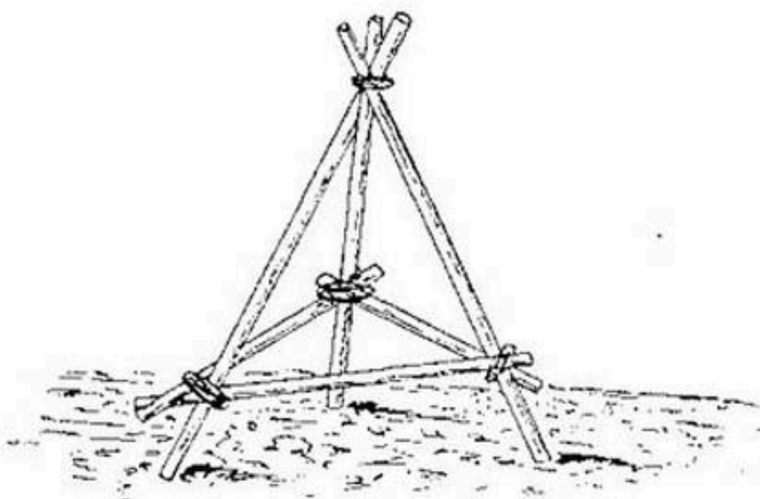
Рис. 117-а. Трехножный сипай.
