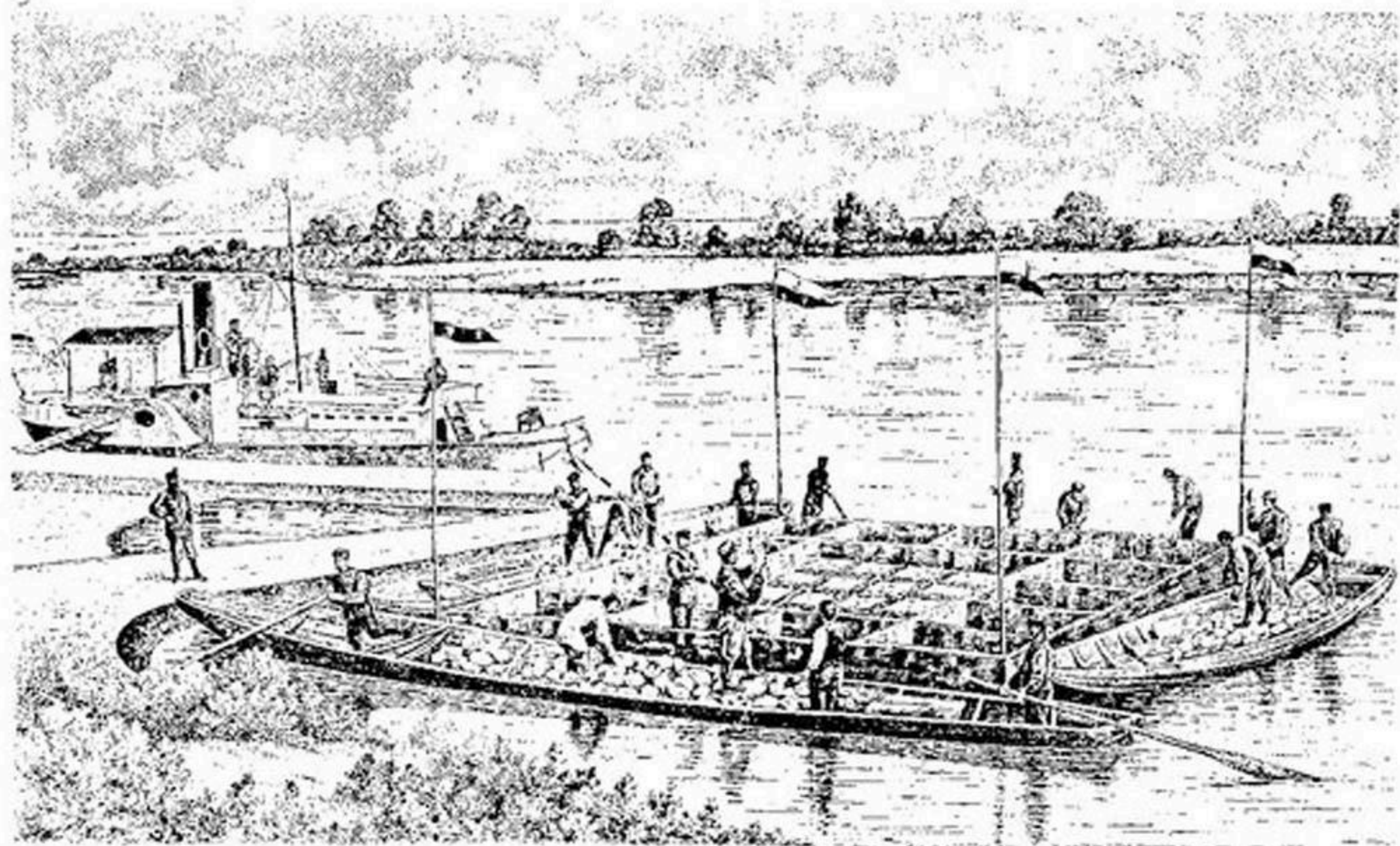
Рис. 105. Погружка тѣла на дно.
