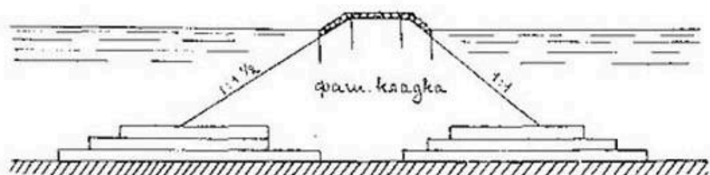
Рис. 178. Тип продольной дамбы на р. Западной Двине.
