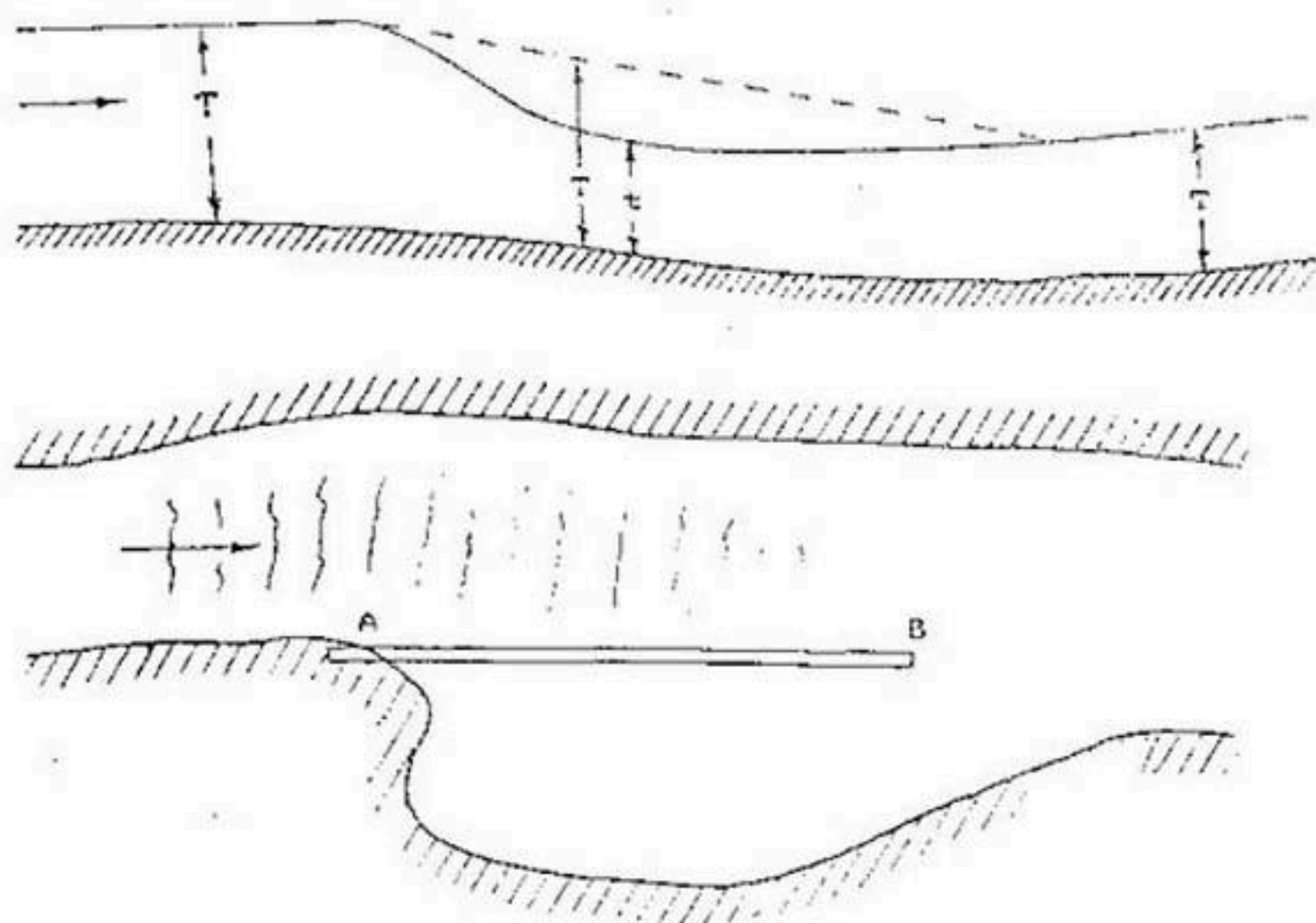
Рис. 77. Порожистый участок реки с внезапным расширением русла.
