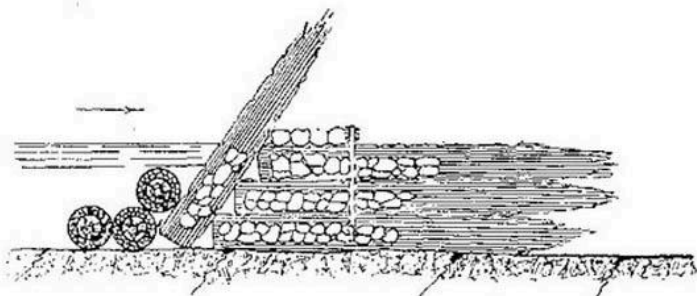
Рис. 223. Фашиновые бунны-илоудержатели на р. Дунае.
