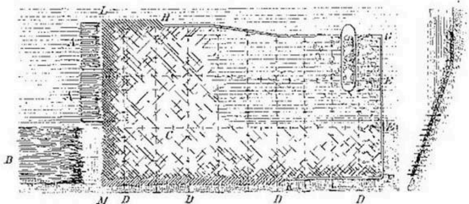
Рис. 141. Укрепление берега реки Миссиссиппи хворостяными покрывалами.
