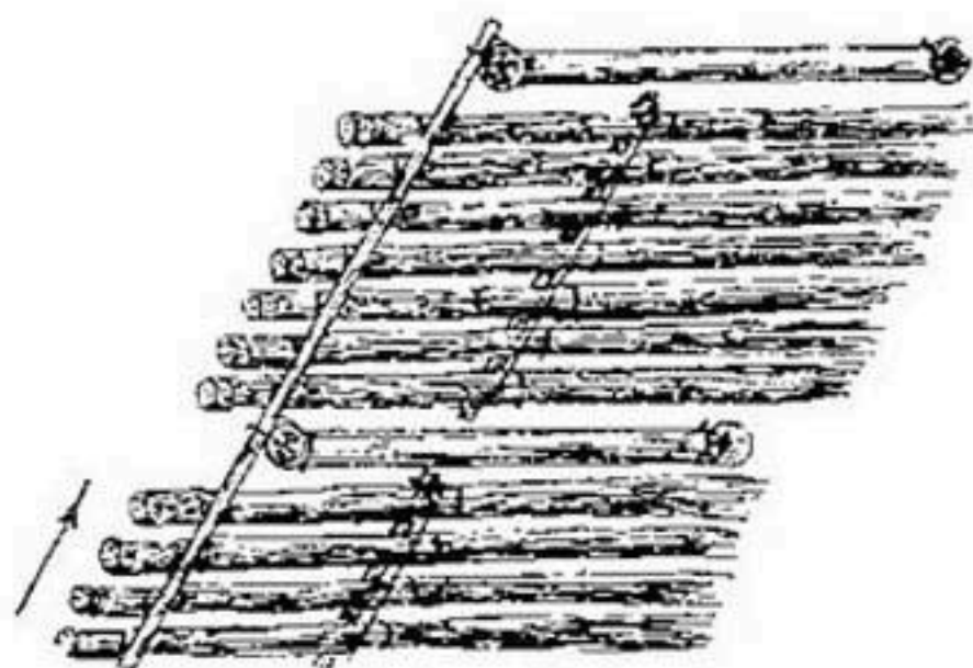
Рис. 227. Подвижной щит Вольфа. Тип щита для быстрого течения.
