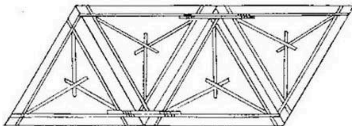
Рис. 191. Сопряжение между собой трехножных сипаев.
