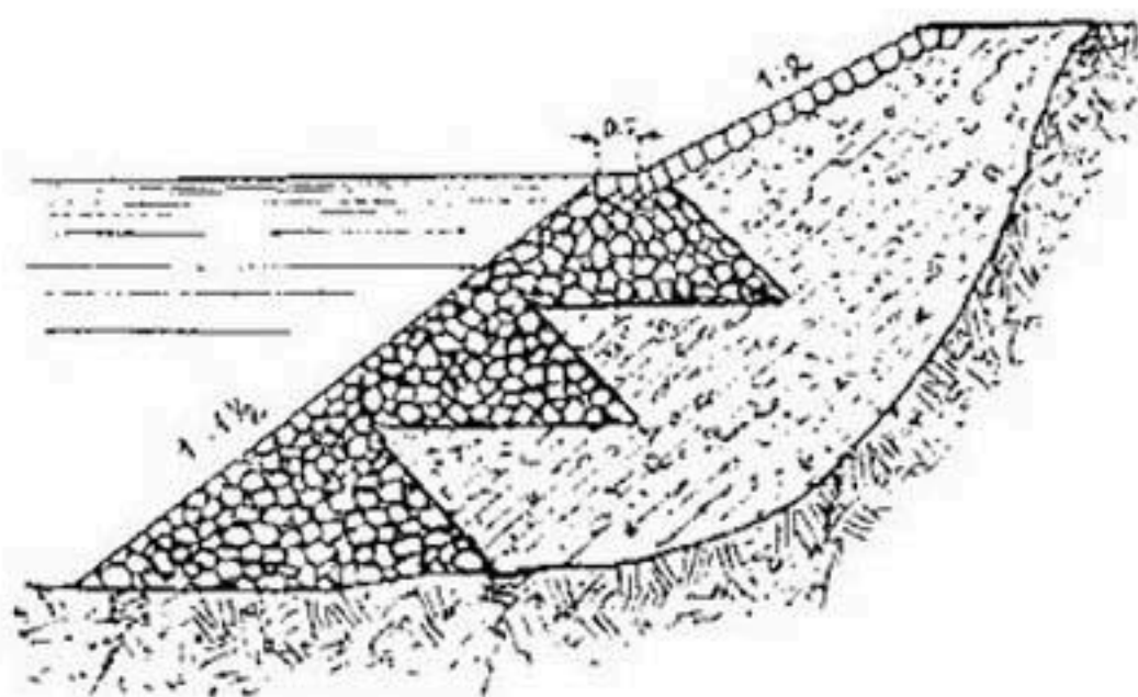
Рис. 132. Укрепление берега призмами каменной наброски с заполнением ядра хрищем.
