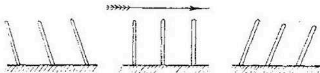
Рис. 162. Типы расположения полузапруд.
