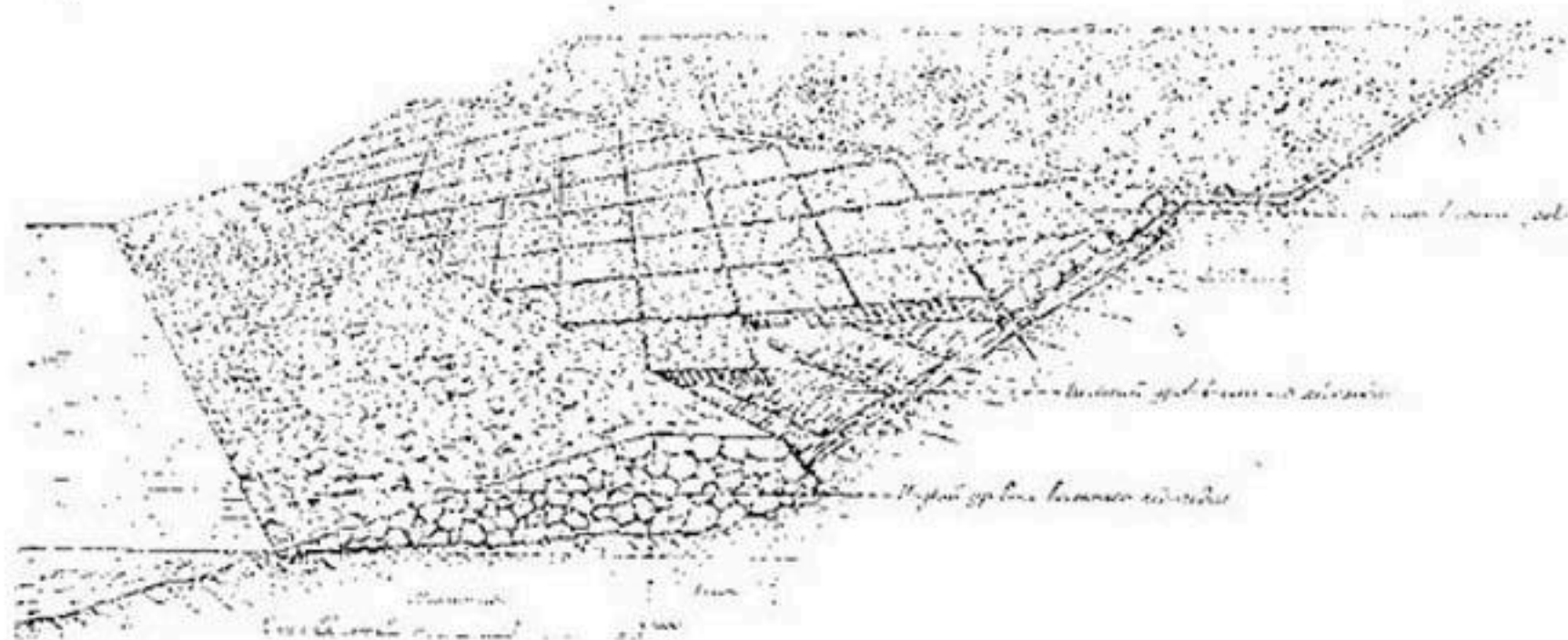
Рис. 161. Укрепление берега плетневыми клетками с хвостяной подстилкой.
