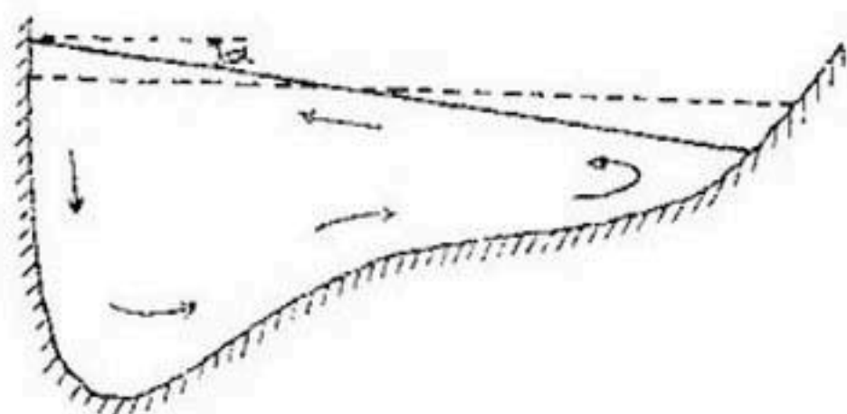
Рис. 29. Поперечные движения частиц воды в извилине реки.
