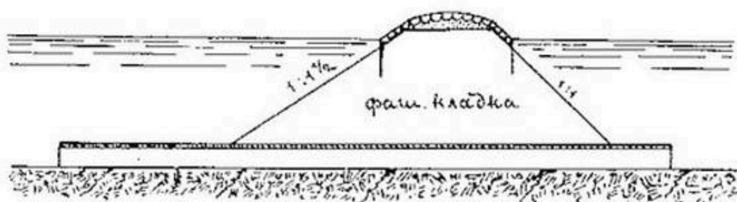
Рис. 202. Запруда из фашинной кладки на фашинном туюфе.
