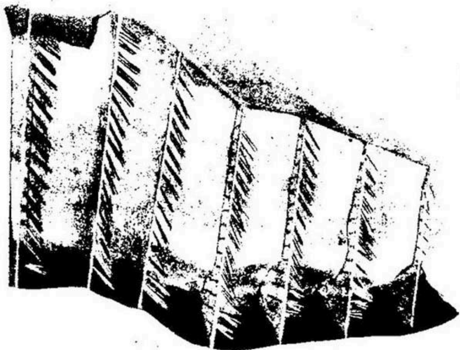
Рис. 56. Струи речного потока. Рисунок изображает фотографический снимок с находящейся в музее Института Инженеров Путей Сообщения модели участка реки Днепра на одном из его перекатов. В виде игол на модели изображены направления струй и их скорости, измеренные помощью особого прибора („Струенмерителя“).
