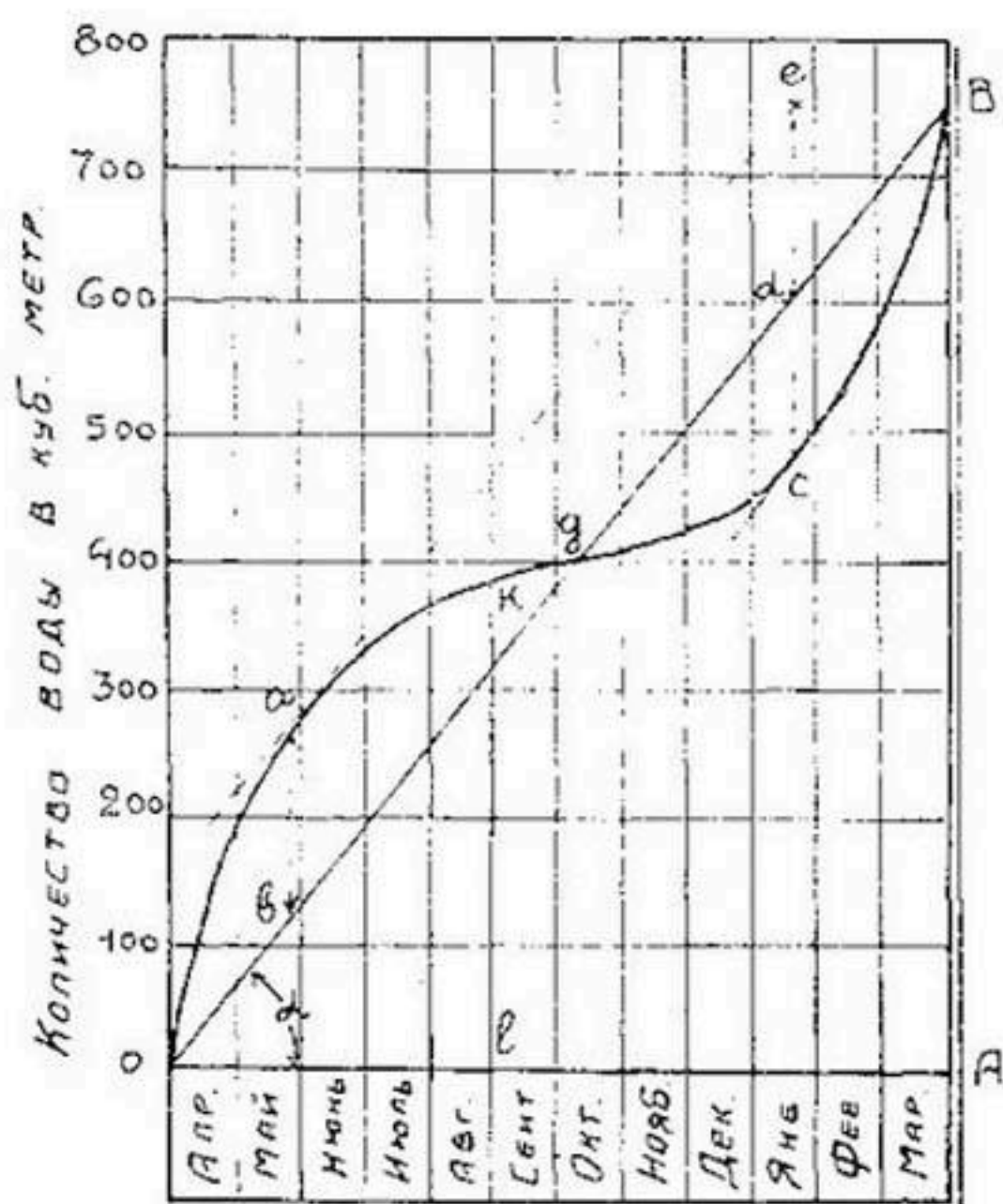
Рис. 16. Интегральная кривая расхода.
