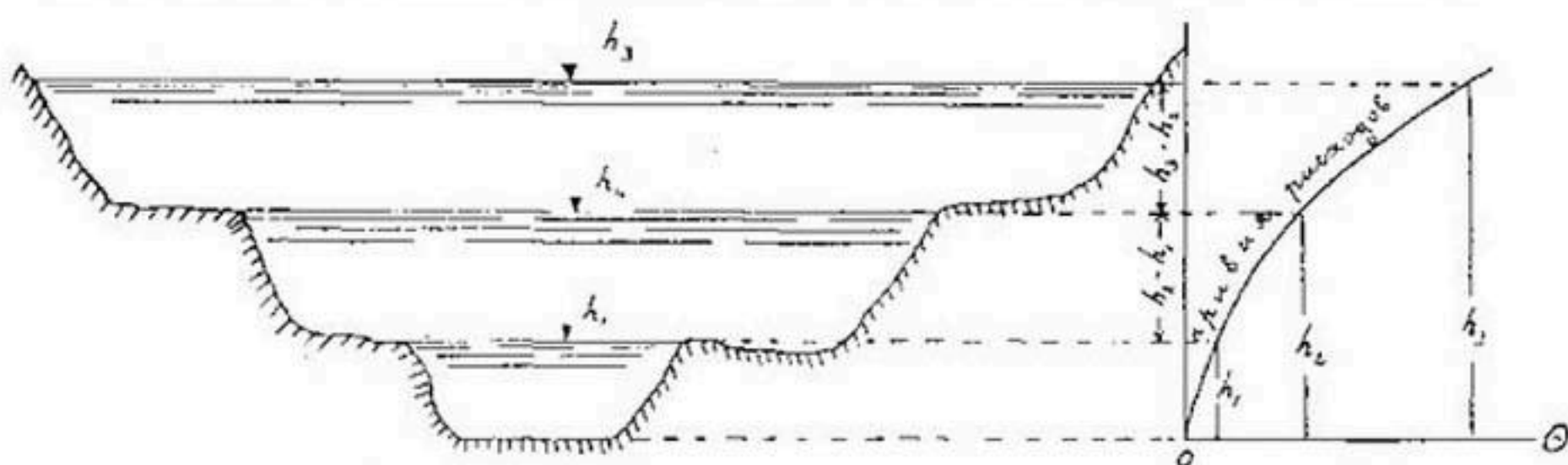
Рис. 12. Кривая расхода воды при многоярусном русле.
