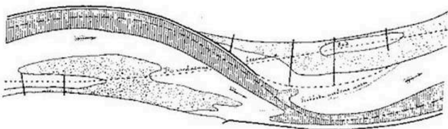
Рис. 59. Практически осуществимое расположение струенаправляющей дамбы на перекате.
