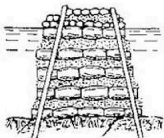
Рис. 220. Буна-плоудержатель, построенная из коротких фашин.
