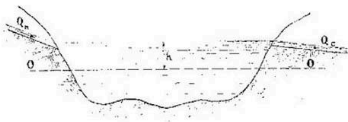
Рис. 281. Схема вертикального разреза озера.
