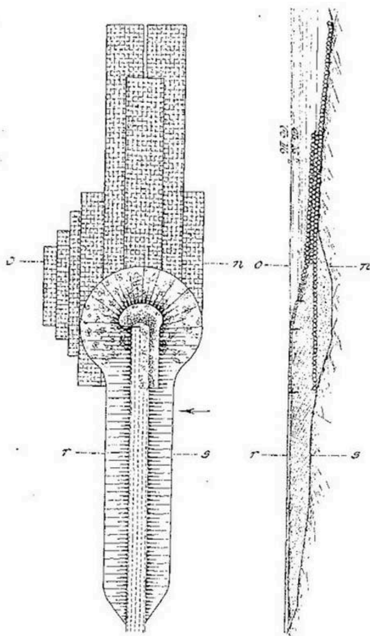
Рис. 197. Донная полузапруда на р. Эльбе, составленная из тяжелых фашин и прихвнутая к голове полузапруды.
