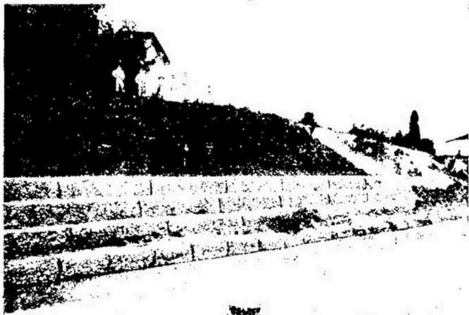
Рис. 133. Береговое укрепление, построенное из кладки габионов.
