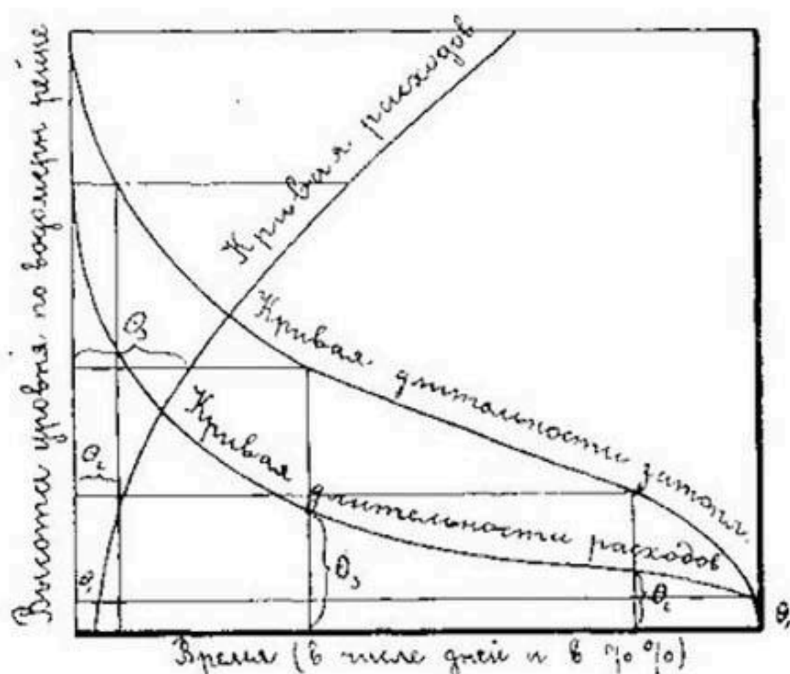
Рис. 14. График длительности расходов воды.
