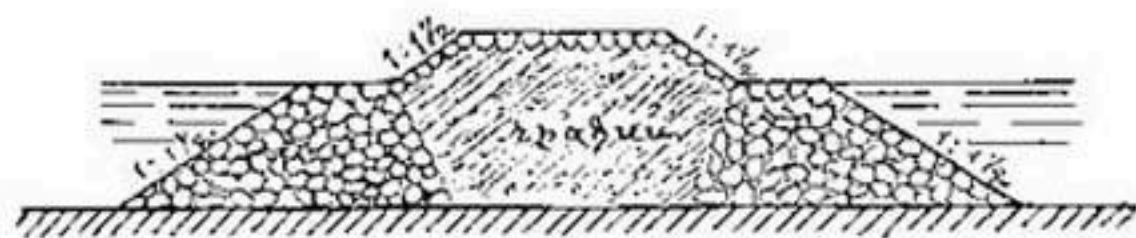
Рис. 174. Разрез головной части полузапруды из каменной наброски с ядром из гравия.
