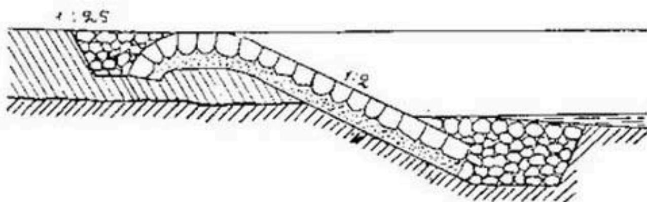
Рис. 189. Каменная продольная дамба в виде береговой опояски.
