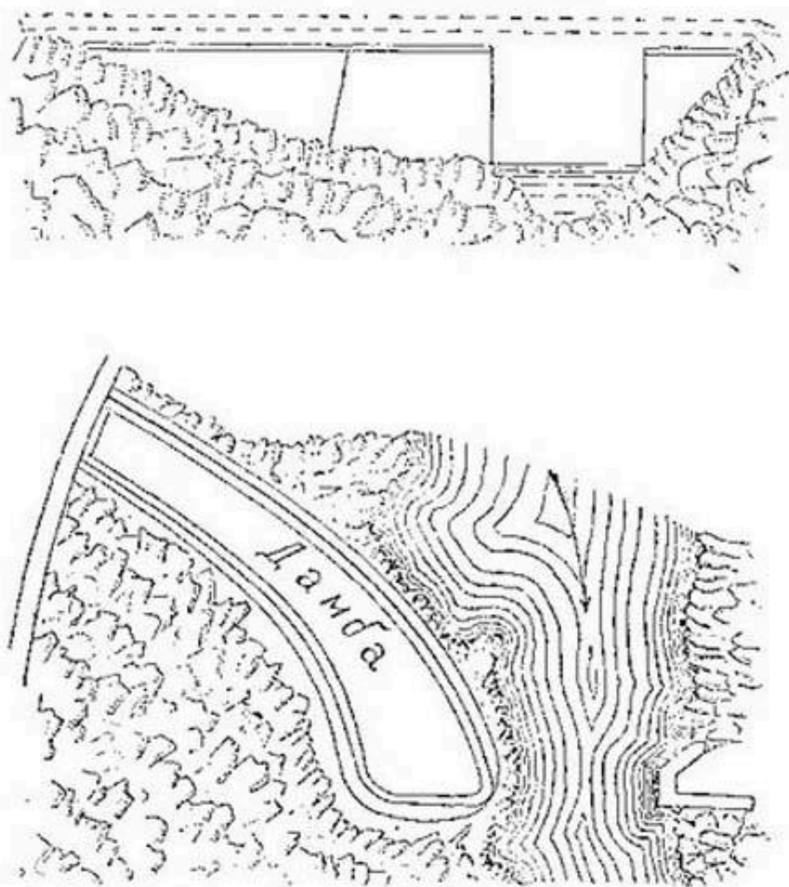
Рис. 294. Сужение тальвега полузапрудой.
