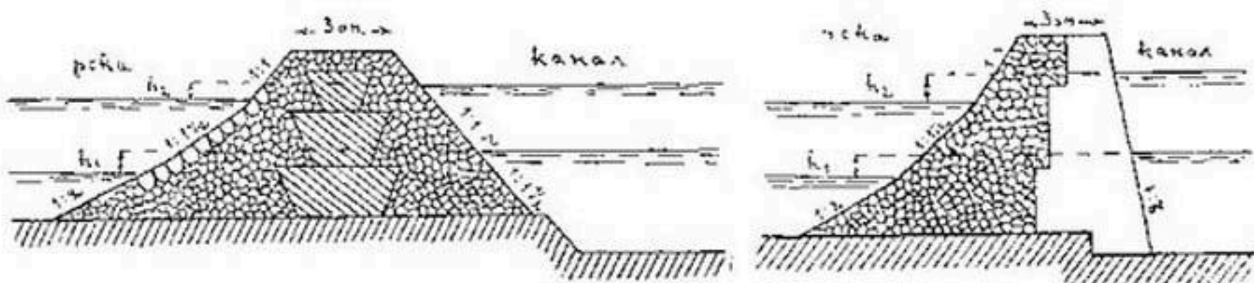
Рис. 75 и 76. Типы каменных дамб канала.
