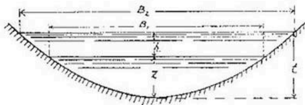
Рис. 11. Параболическое русло.
