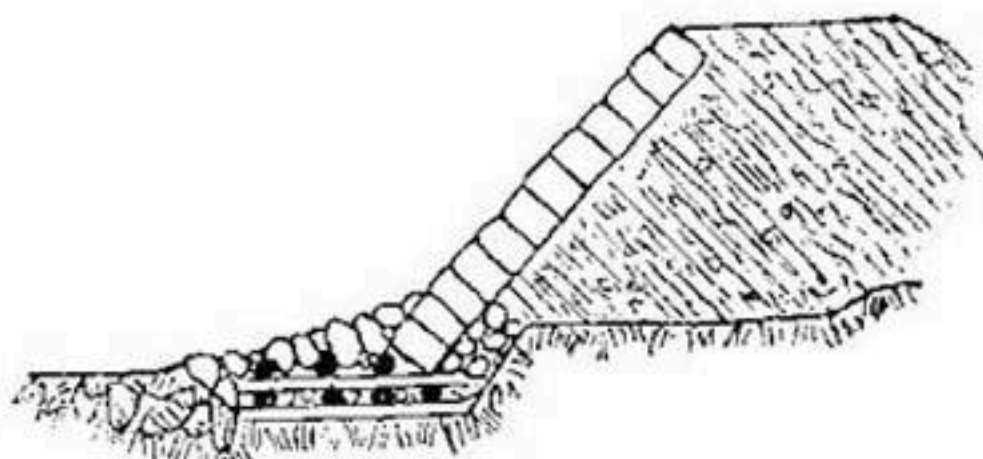
Рис. 271. Укрепление откосов русла на конической высыпке.
