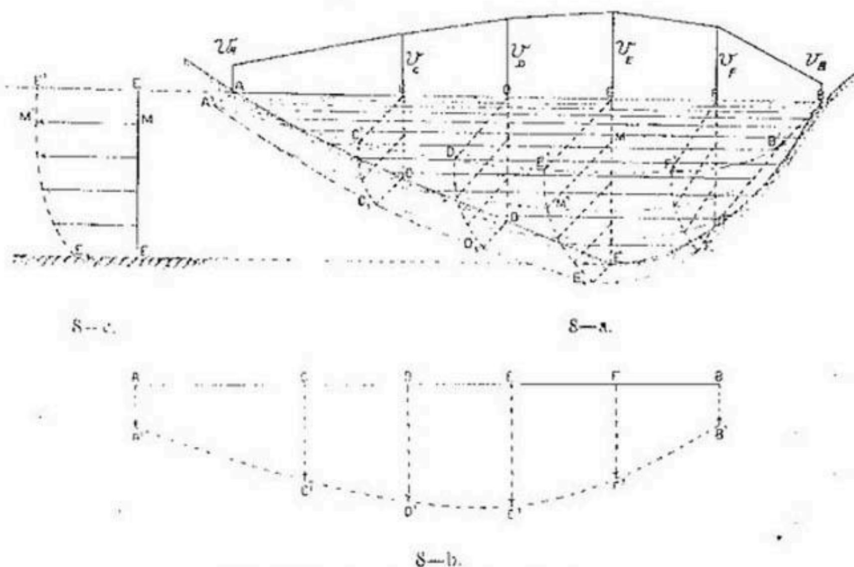
Рис. 8. Живое сечение и скорости течения.
