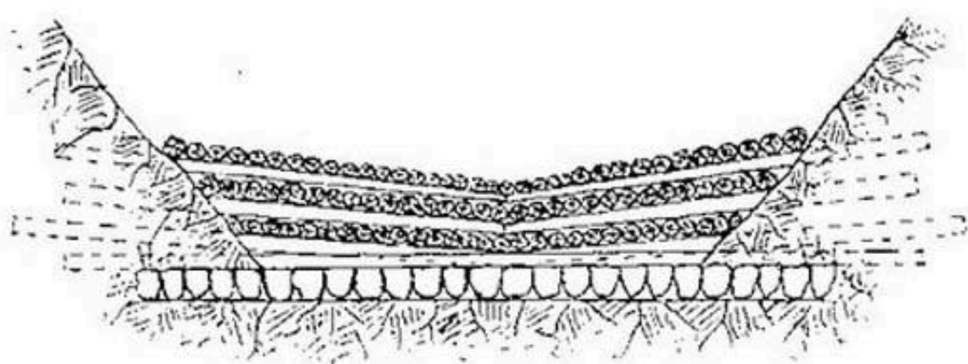
Рис. 263-б. Поперечный разрез.
