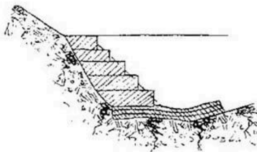
Рис. 146. Укрепление берега тюфячной кладкой.
