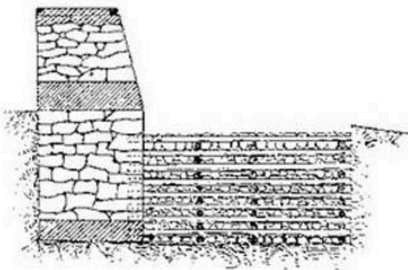
Рис. 257. Ряжевый водобойный пол запруды.
