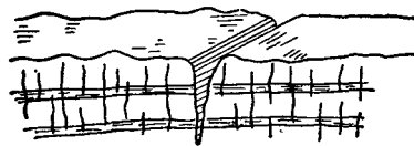
Рис. 35. Пересечение горизонтальной слоистости вертикальной полосчатостью
