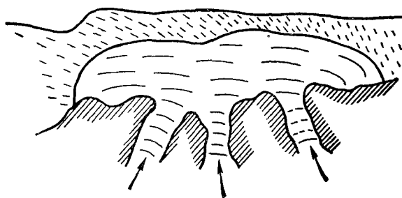
Рис. 121. Предгорный ледник (план)
