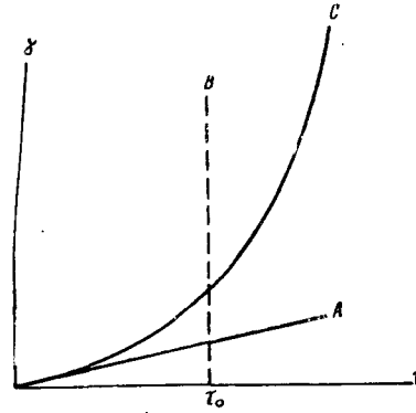
Рис. 14. Зависимость между скоростью деформации (скоростью течения) и напряжением сдвига:
