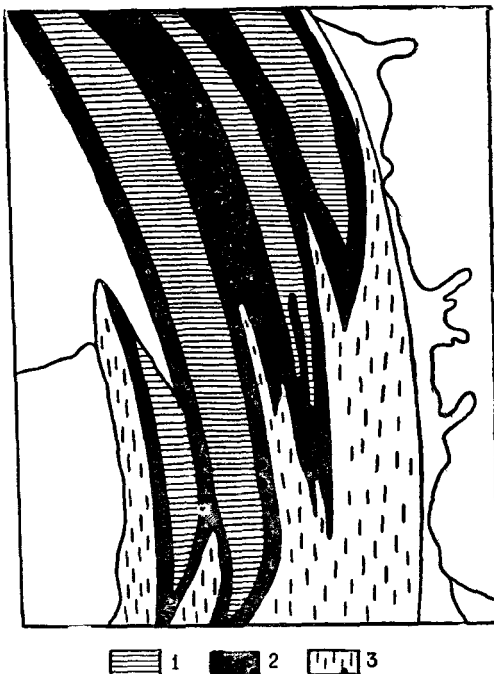
Рис. 36. Распределение масс льда на одном из участков языка Большого Алезского ледника (по Ф. Варески):
