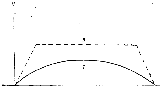
Рис. 58. Кривые распределения скоростей на леднике в поперечном створе при правильном (I) и глыбовом (II) движении
