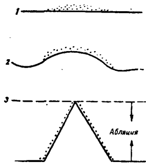
Рис. 96. Образование «грязевого конуса» на поверхности ледника (по Р. Штрейф-Беккеру)
