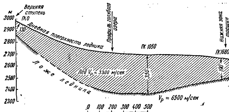
Рис. 42. Сейсмический разрез ледника Большой Актру (Алтай) по осевому профилю (по Г. С. Кравцову и А. Г. Терентьевой)
