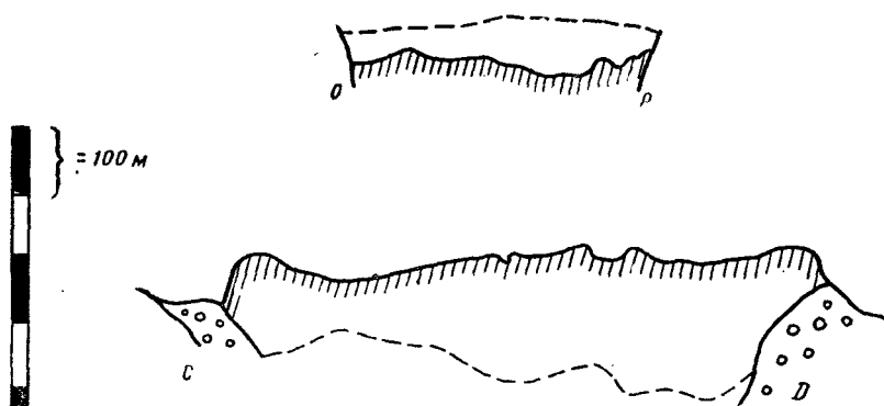
Рис. 109. Поперечные профили поверхности ледника Малдров в 1952 и 1957 гг. (по О. Посту). Положение профилей показано на рис. 108
