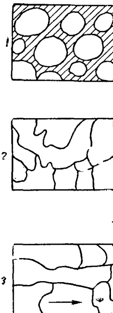
Рис. 6. Развитие ледниковых зерен:
