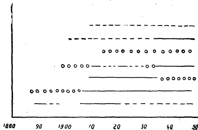
Рис. 106. Характер колебаний некоторых ледников в западной части гор Чугач (Аляска).
