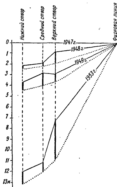
Рис. 41. Эпюра понижения (сплошная линия) и стаивания (точечная линия) поверхности ледника Сатпаева (по Н. Н. Пальгову)
