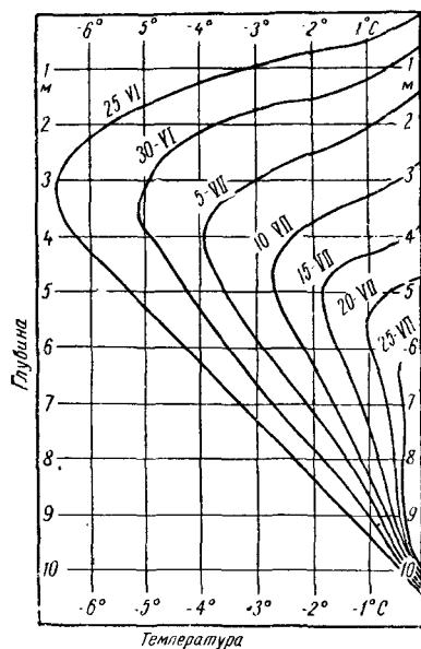
Рис. 46. Вертикальное распределение температуры фирна по пятидневкам (с 25 июня по 25 июля) на плато Изаксена (по Г. Свердрупу)
