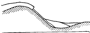
Рис. 116. Возрожденный ледник (продольный профиль)
