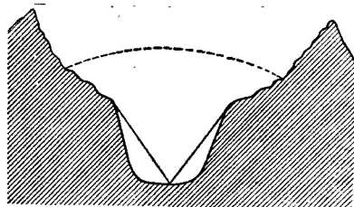
Рис. 136. Трог, возникший из V-образной долины.
