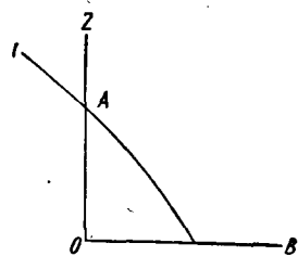
Рис. 110. Построение балансовых кривых простой формы (по М. В. Тронову)
