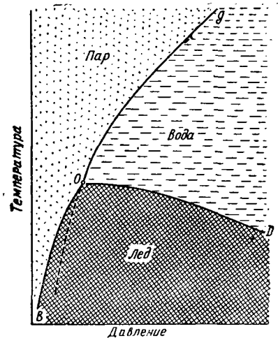
Рис. 1. Фазовая диаграмма воды (пунктиром — кривая равновесия пара и переохлажденной воды)
