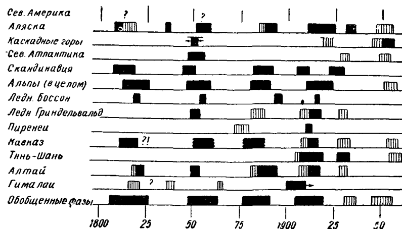
Рис. 107. Колебания ледников за 1800—1950 гг. (по А. В. Шнитникову).
