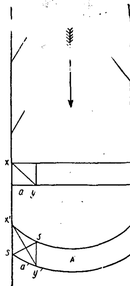
Рис. 64. Схема образования боковых трещин на леднике
