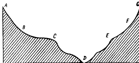
Рис. 137. Переломы в поперечном профиле ледниковой долины
