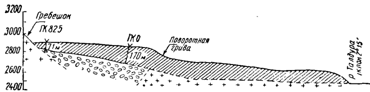
Рис. 43. Сейсмический разрез Большого Талдуринского ледника (Алтай) по азимуту 32° (по Г. С. Кравцову и А. Г. Терентьевой)
