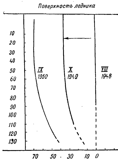
Рис. 53. Распределение скоростей движения льда в Юнгфрауфирне по вертикали (по М. Перутцу).
