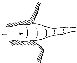
Рис. 125. Плавающий ледяной язык (план)
