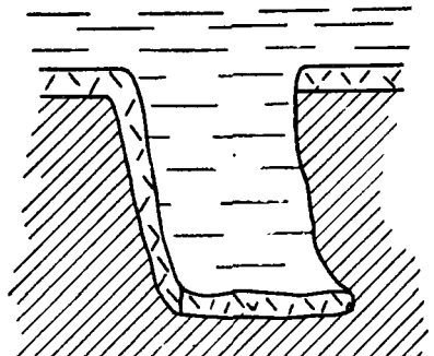
Рис. 115. Висячий, или крутобокий, ледник (вид спереди)
