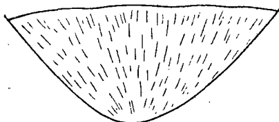
Рис. 31. Расположение полосчатости внутри ледника (по Краммеру)
