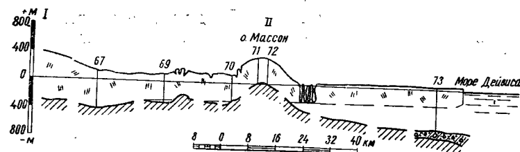
Рис. 127. Разрез шельфового ледника Шеклтон с «ледяным возвышением» («ледяным куполом») на острове Массон
