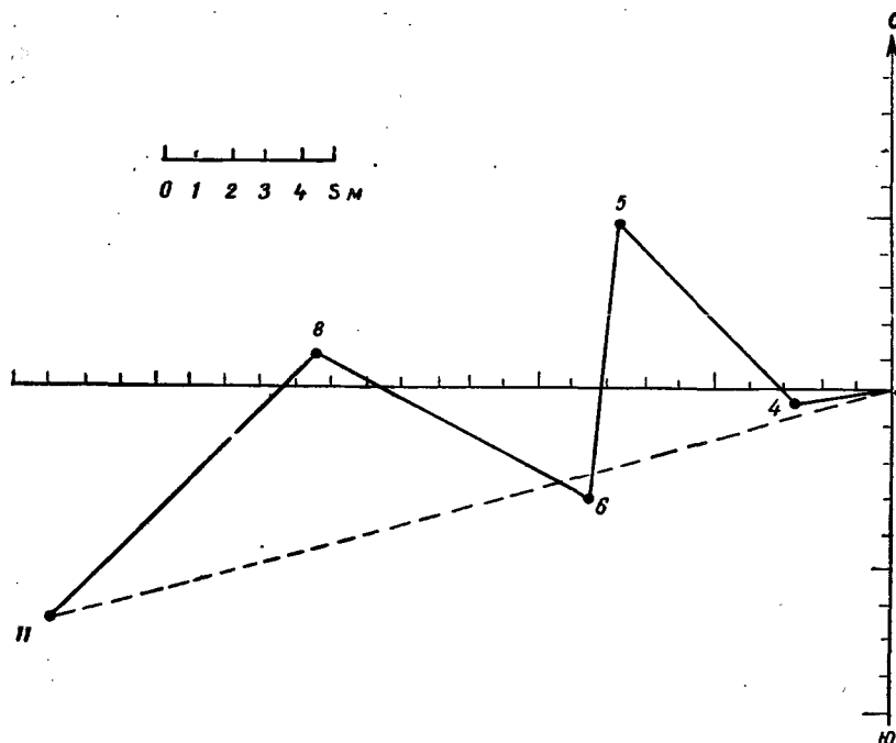
Рис. 57. Горизонтальное перемещение одной из точек на поверхности ледника Эке (Гренландия) с 3 по 11 сентября 1948 г. (по А. Бауэру). Цифры означают даты (3=3/IX и т. д.). Пунктирная линия — геометрическая сумма перемещения за время с 3 по 11 сентября
