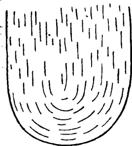
Рис. 32. Проекция полосчатой структуры на поверхность ледника вблизи его конца (по Краммеру)
