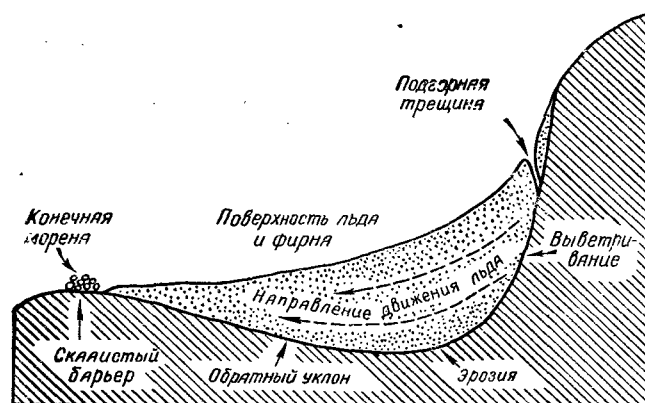
Рис. 135. Продольный разрез кара и карового ледника (по Р. Грэсвеллу)
