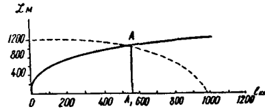
Рис. 103. Кривая равновесия и (пунктиром) возможный профиль ледника (по М. В. Тронову)
