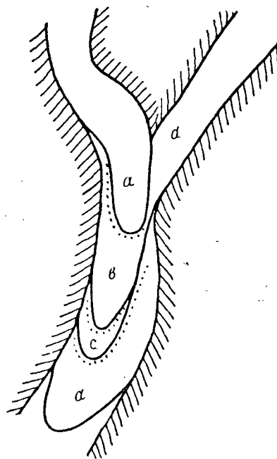
Рис. 89. Схема многоярусного ледника (по Ф. Виссеру)
