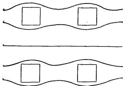
Рис. 68. Линии течения льда на ледниковом ложе вокруг препятствий (по Вэртману)
