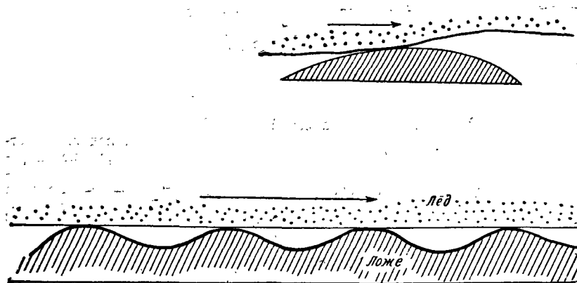
Рис. 69. Ледник при быстром скольжении по своему ложу опирается только на вершины неровностей ложа (по Л. Ллибутри).
