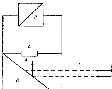
Рис. 21. Схема простейшего поляризационного прибора для изучения строения льда:
