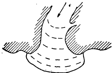
Рис. 118. Ширококонецный ледник (план)
