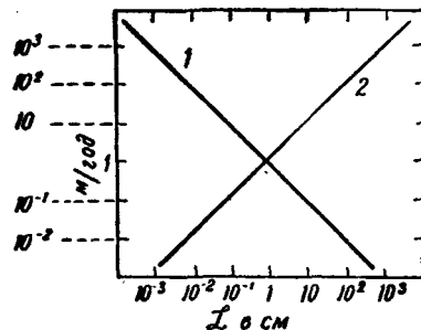
Рис. 67. Зависимость между логарифмами скорости скольжения ледника и логарифмами размеров неровностей ледникового ложа (по Вэртману):
