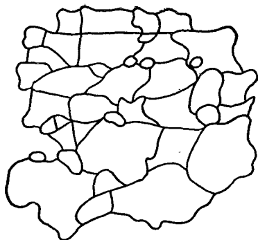
Рис. 20. Зернистая структура ледникового льда
