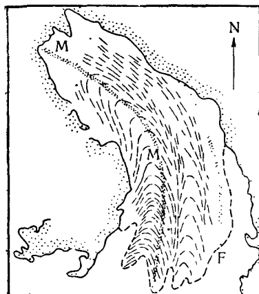
Рис. 26. Рисунок полосчатости на поверхности ледника Блю (США) (по В. Кэмбу):
