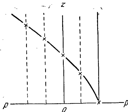
Рис. 112. Простая балансовая кривая в случае изменения климата (по М. В. Тронову)
