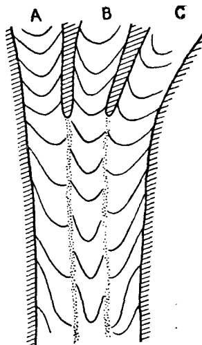
Рис. 27. Системы огив на сложном леднике
