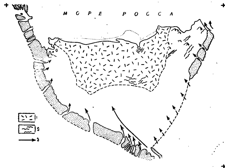
Рис. 126. Шельфовый ледник Росса. Стрелками показано направление стока выводных и долинных ледников в море Росса;
