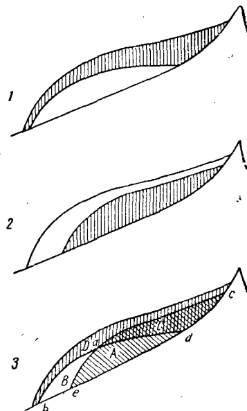
Рис. 47. Распределение температур в гипотетическом леднике (по Ф. Форелю)
