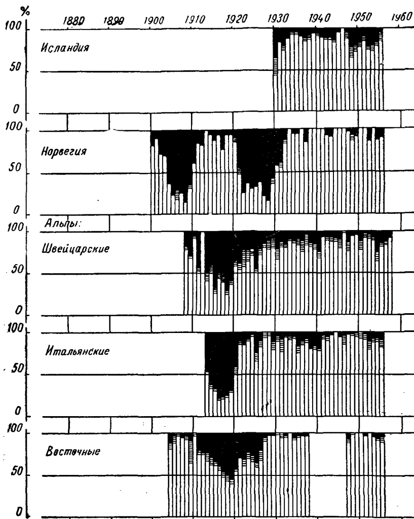
Рис. 105. Колебания ледников некоторых районов Европы в XX веке (по А. В. Шнитникову).
