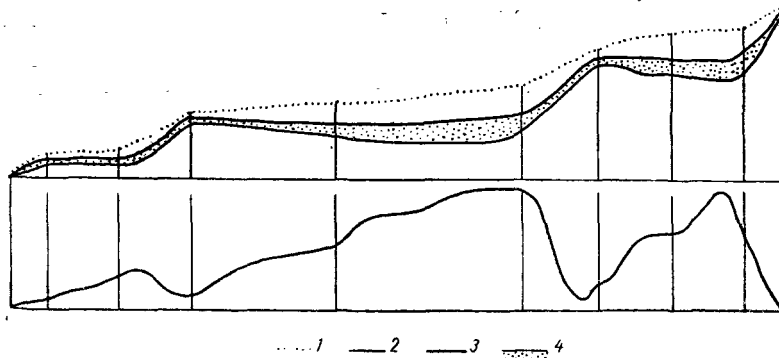
Рис. 138. Распределение интенсивности ледниковой эрозии по продольному профилю долины (по Э. Мартону):
