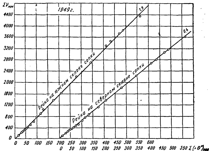
Рис. 92. Зависимость таяния снежников от суммы положительных температур воздуха (по В. Л. Шульцу)
