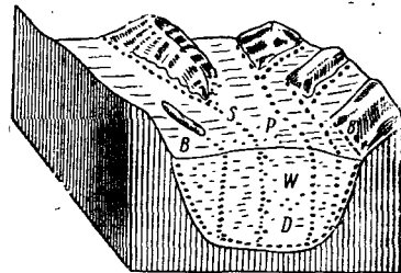
Рис. 129. Расположение различных морен на поперечном профиле долинного ледника вблизи его конца (по Кунскому):
