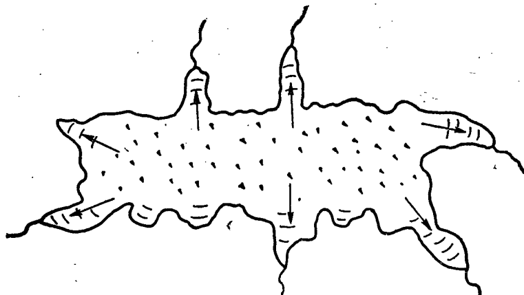
Рис. 119. Ледник плато (план)
