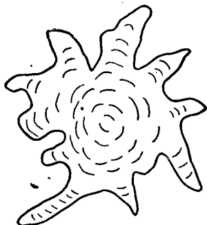
Рис. 114. Ледники вулканических конусов (план)
