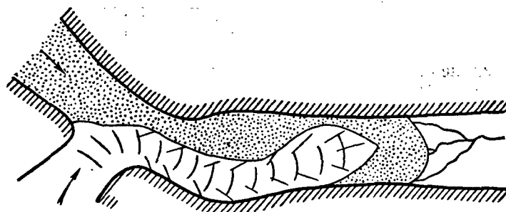
Рис. 86. Схема двухъярусного ледника (по Ф. Виссеру)
