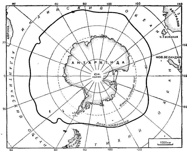
Рис. 142. Среднее положение антарктической конвергенции
