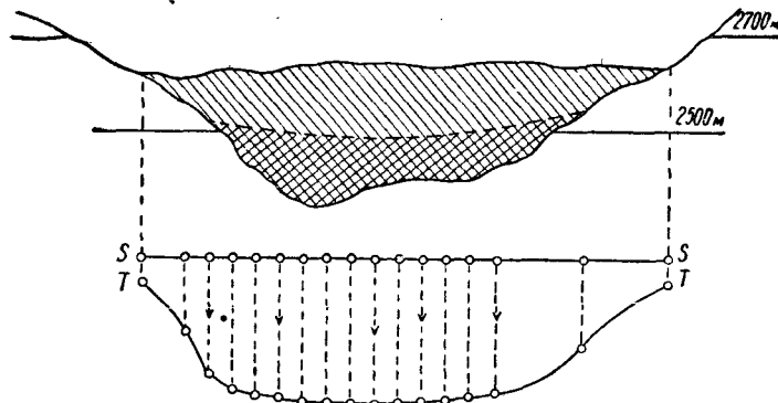
Рис. 50. Поперечный профиль долинного ледника и кривая распределения скорости на его поверхности (по Г. Гессу)
