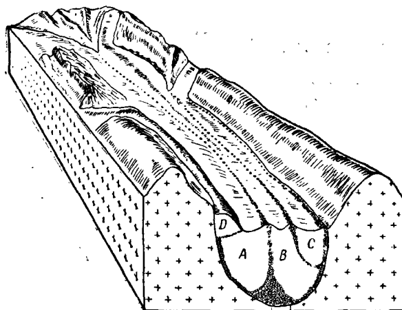
Рис. 91. Формы слияния ледников (по Р. Шарпу):
