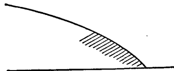
Рис. 33. Полосчатость на конце ледника (в продольном профиле)
