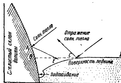
Рис. 93. Таяние ледника под действием теплового излучения склонов:
