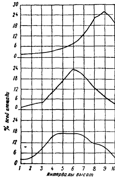
Рис. 128. Кривые нормального распределения площади ледника по высоте: в ледниковом куполе (наверху), в долинном леднике (типа Ронского ледника) (в середине) и в каровом леднике (внизу)
