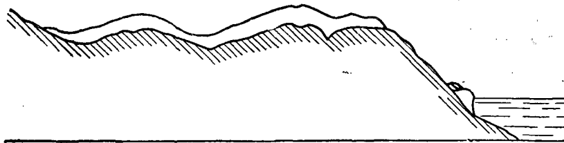
Рис. 120. Нагорные льды (профиль)
