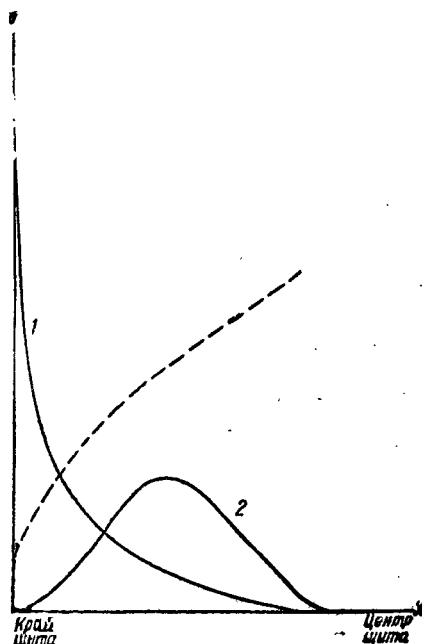
Рис. 85. Теоретические кривые изменения скорости движения поверхности ледникового щита при различных очертаниях этой поверхности (по С. Вялову):
