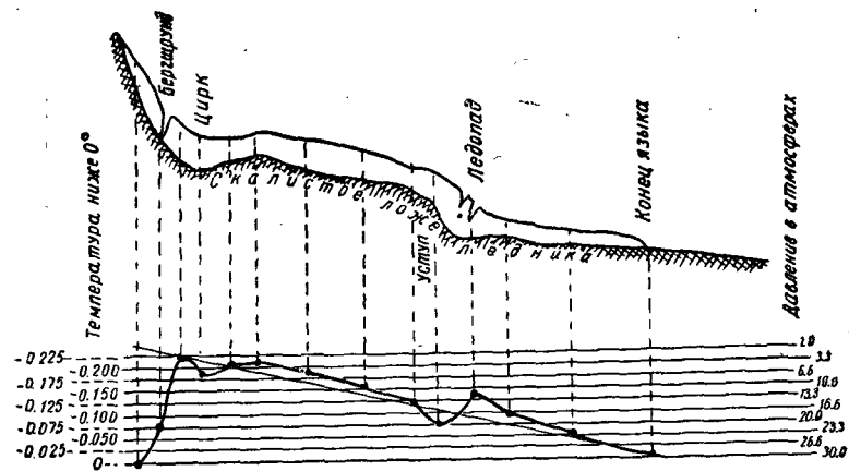
Рис. 141. Совмещенные кривые температуры льда (прямая линия) и местных, обусловленных давлением (мощностью льда) температур плавления льда (извилистая линия) (по Фишеру)
