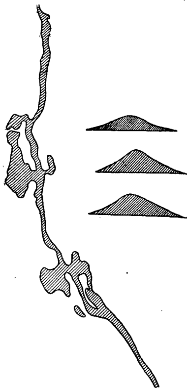
Рис. 132. Оз (слева — в плане; справа — поперечные профили)
