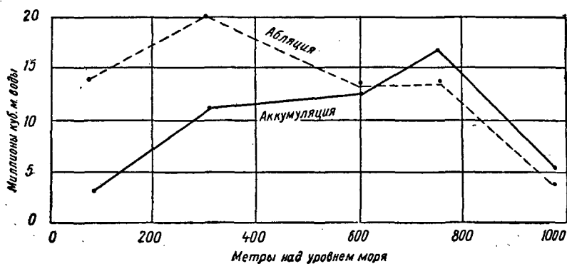
Рис. 15. Балансовая диаграмма ледника Четырнадцатого Июля на Шпицбергене за 1933/34 «бюджетный» год (по Альманну)
