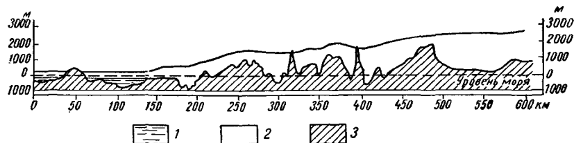
Рис. 143. Профиль ледникового щита в районе ст. Модхейм:
