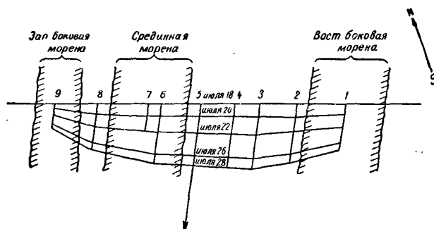
Рис. 51. Диаграмма скоростей движения различных точек на поверхности ледника Нисквалли (по Леконту). Масштабы расстояний и скоростей, естественно, разные
