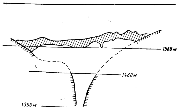
Рис. 134. Поперечный профиль ледника Мер-де-Гляс.
