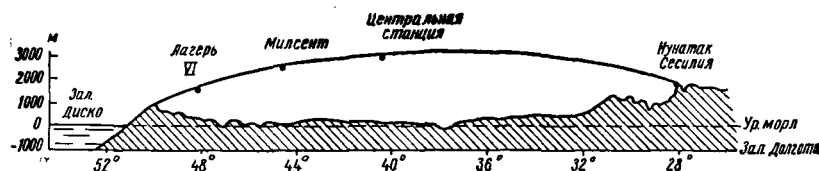
Рис. 44. Поперечный профиль Гренландского ледникового щита (по Хольцшереру)
