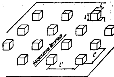
Рис. 66. Схема неровностей ледникового ложа (по Вэртману)
