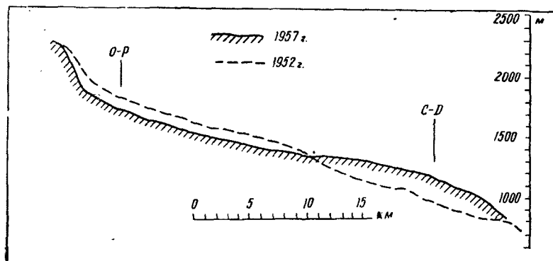
Рис. 108. Продольные профили поверхности ледника Малдров в 1952 и 1957 гг. (по О. Посту)
