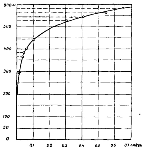
Рис. 13. Скорость истечения льда (см/сек) из отверстия цилиндра при различных давлениях, выраженных в толщине (м) слоя льда (по Г. Гессу)
