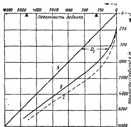
Рис. 45. Горизонтальные давления на разных глубинах, выраженные в толщине слоя льда (по Р. Кёхлину):
