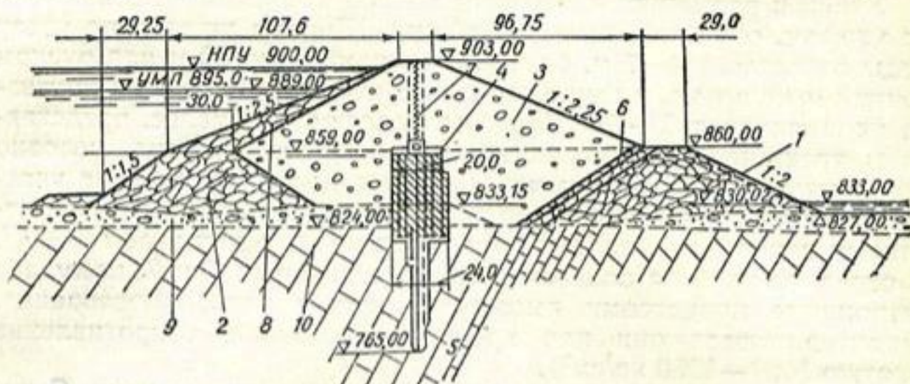
Р и с. 22. Поперечный разрез по Атбашинской плотине.
