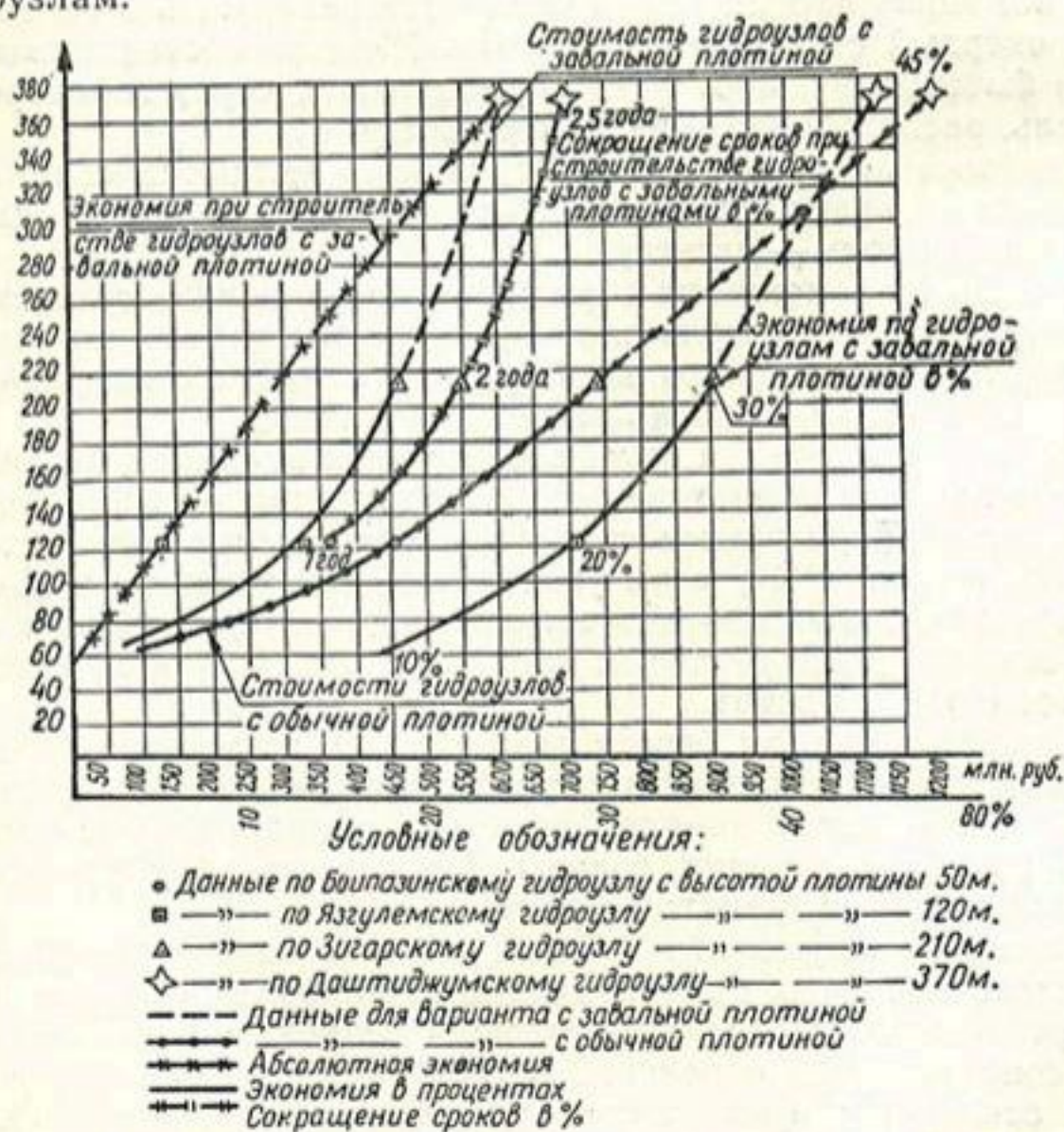
Р и с. 23. График эффективности возведения гидроузлов с завальными плотинами.
