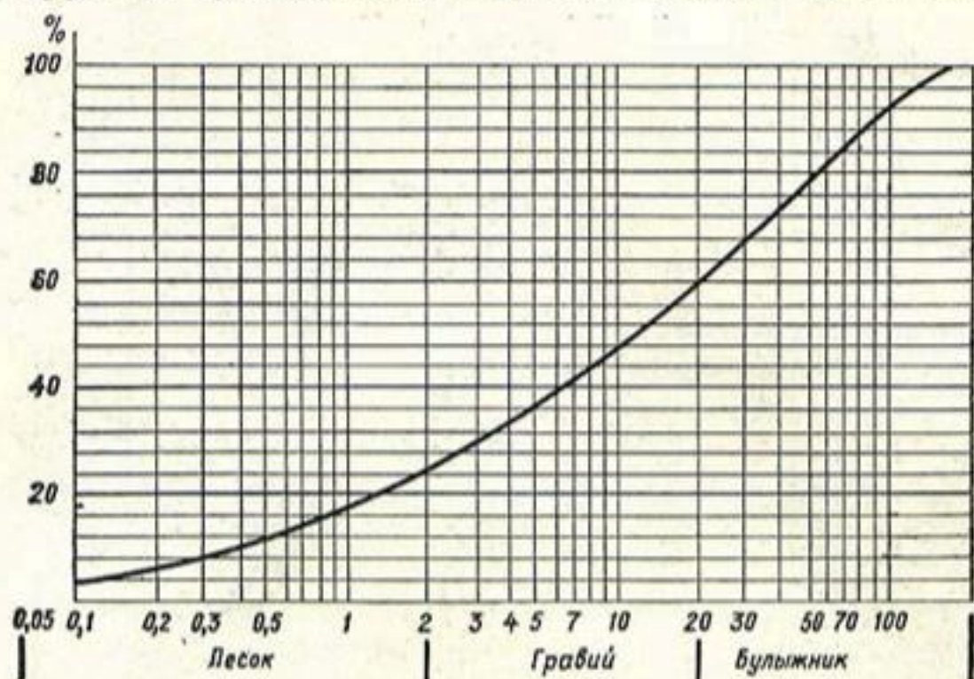
Рис. 14. Предельная кривая грансостава грунта тела Орто-токойской плотины.
