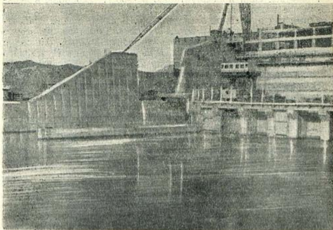
Р и с. 33. Головная ГЭС на р. Вахше. Вид на низовую правобережную стенку, выполненную с применением армо- панелей.
