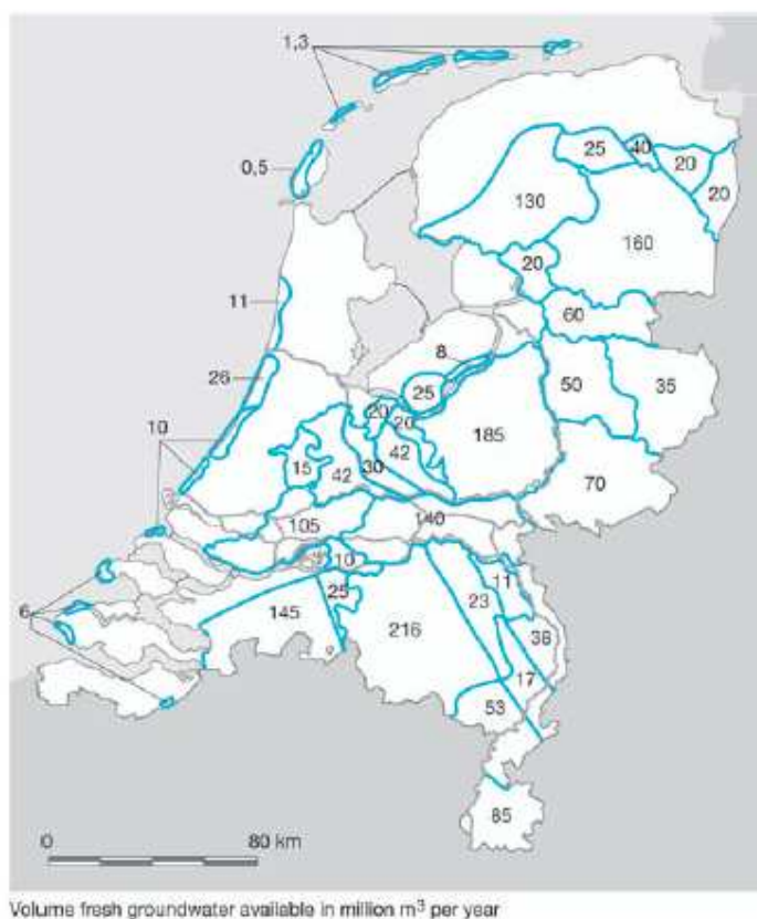
Рисунок 10.3.1 Расчётный объём пресных подземных вод в Нидерландах на регион в год (Источник: Ministerie van Verkeer en Waterstaat, 1985)
