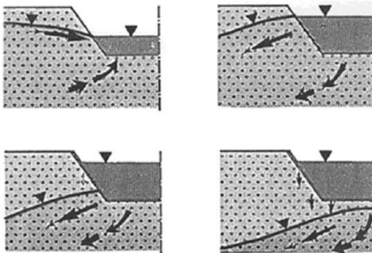
Рисунок 10.2.2 \delta^{18}O в речной воде и соответствующий уровень \delta^{18}O в близлежащих подземных водах; снижение значений \delta^{18}O обусловлено таянием снега в летний период
