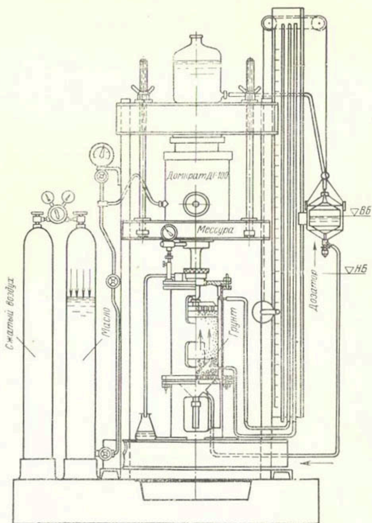
Рис. 2. Схема вертикального фильтрационно-компрессионного прибора.
