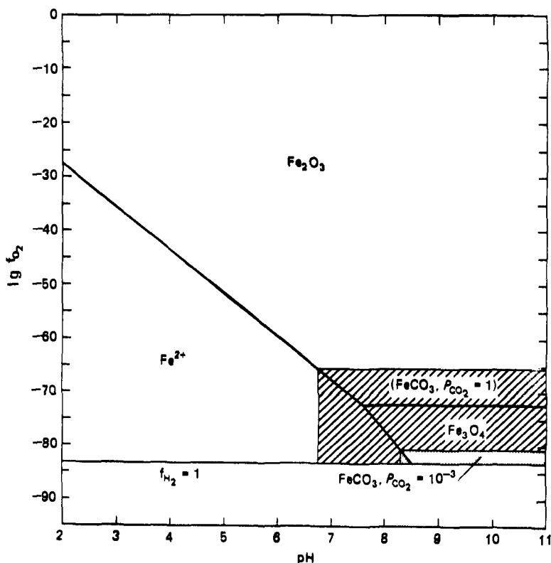
Р и с. 11.13. Зависимость соотношений устойчивости в системе \text{Fe} - \text{O} - \text{H}_2\text{O} - \text{CO}_2 при 25^\circ\text{C} от \lg f_{\text{O}_2} и pH. Заштрихованная область — поле устойчивости сидерита при P_{\text{CO}_2} = 1 атм, область с точками — поле устойчивости сидерита при P_{\text{CO}_2} = 10^{-3} атм. Границы твердое вещество/раствор построены для a_{\text{Fe}^{2+}} = 10^{-6} .
