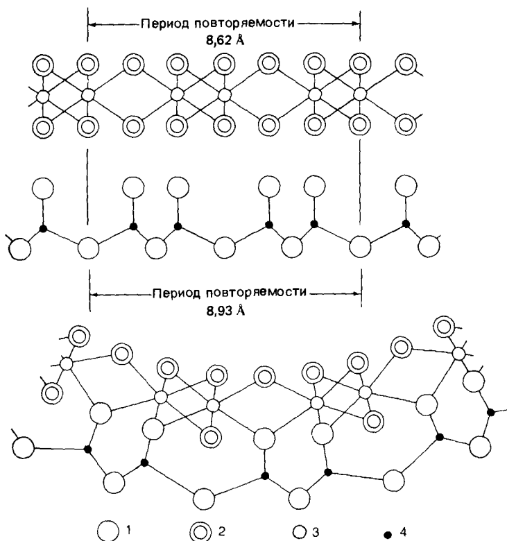
Р и с. 4.4. Схема, показывающая, как несогласованность между октаэдрическим и тетраэдрическим слоями вызывает изгиб решетки, приводящий к трубчатой структуре гаптуазита. 1 — кислород; 2 — гидроксип; 3 — алюминий; 4 — кремний.
