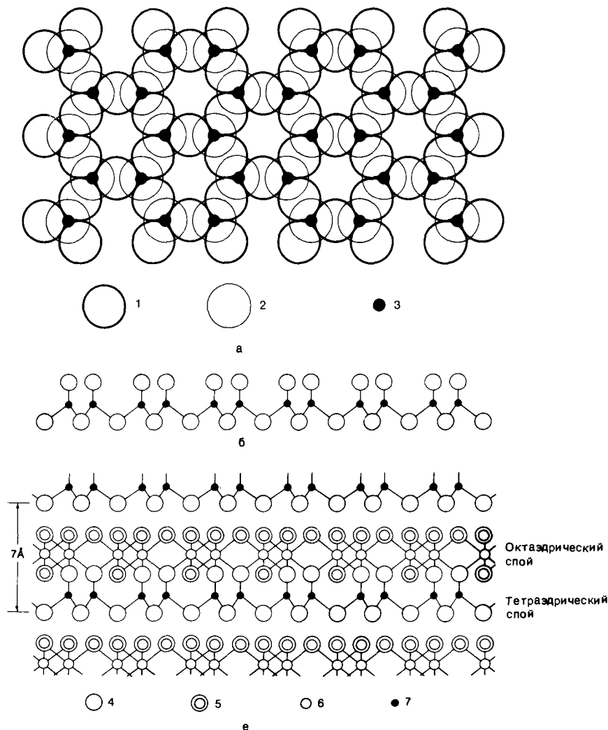
Р и с. 4.3. Структура каолинита. а — тетраздрический слой (вид сверху). Отметим, что ионы кислорода в основании слоя расположены по закону плотнейшей упаковки, но с некоторыми вакансиями; б — поперечное сечение тетраздрического слоя; в — поперечное сечение структуры каолинита, показывающее, что кислород в вершинах тетраэдров замещает некоторые гидроксил-ионы в структуре гиббсита. 1 — кислород в основании тетраэдров; 2 — кислород в вершинах тетраэдров; 3 — кремний; 4 — ионы кислорода; 5 — ионы гидроксила; 6 — алюминий; 7 — кремний.
