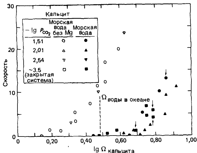
Р и с. 6.11. Зависимость скорости роста кальцита (в произвольных единицах) от степени пересыщения относительно кальцита. \Omega — произведение активностей ионов /K_{\text{кальцит}} . Символы такие же, как на рис. 6.10 (по Бернеру [23]).
