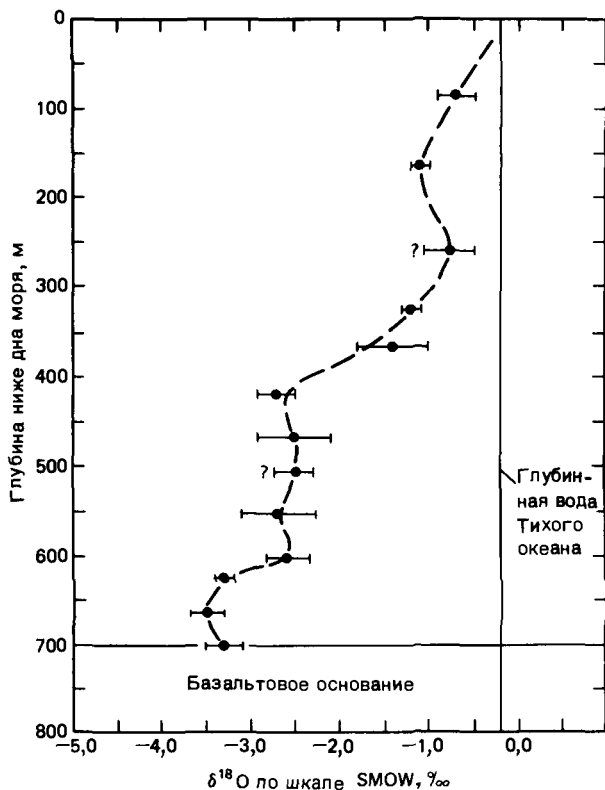
Р и с. 15.6. \delta^{18}\text{O} поровых вод со станции 323 Проекта глубоководного морского бурения. Общее снижение значения \delta^{18}\text{O} (площадь между кривой и линией глубинной воды Тихого океана) можно использовать для оценки имевшей место реакции (по Лоренсу и др. [220]).
