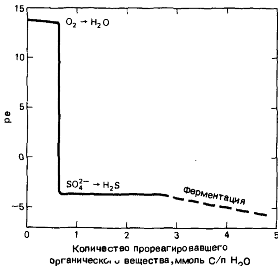
Рис. 12.2. Изменение p_e пресной воды (исходные содержания \text{O}_2 \approx 10 \text{ мг/л} , \text{SO}_4^{2-} = 96 \text{ мг/л} ) в зависимости от количества разложившегося органического вещества (C). Реакции, включающие соединения азота, создают лишь небольшую буферность между уровнями \text{O}_2/\text{H}_2\text{O} и \text{SO}_4^{2-}/\text{H}_2\text{S} . Значение pH предполагается постоянным, равным 7,0.
