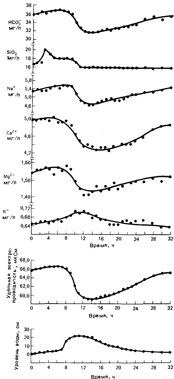
Р и с. 8.13. Изменение химического состава и уровня воды в реке Норт-Форк — притоке реки Шошоун после пивня 20 июля 1973 г. (по Мипперу и Драйверу [242], представлено Американским геологическим обществом).
