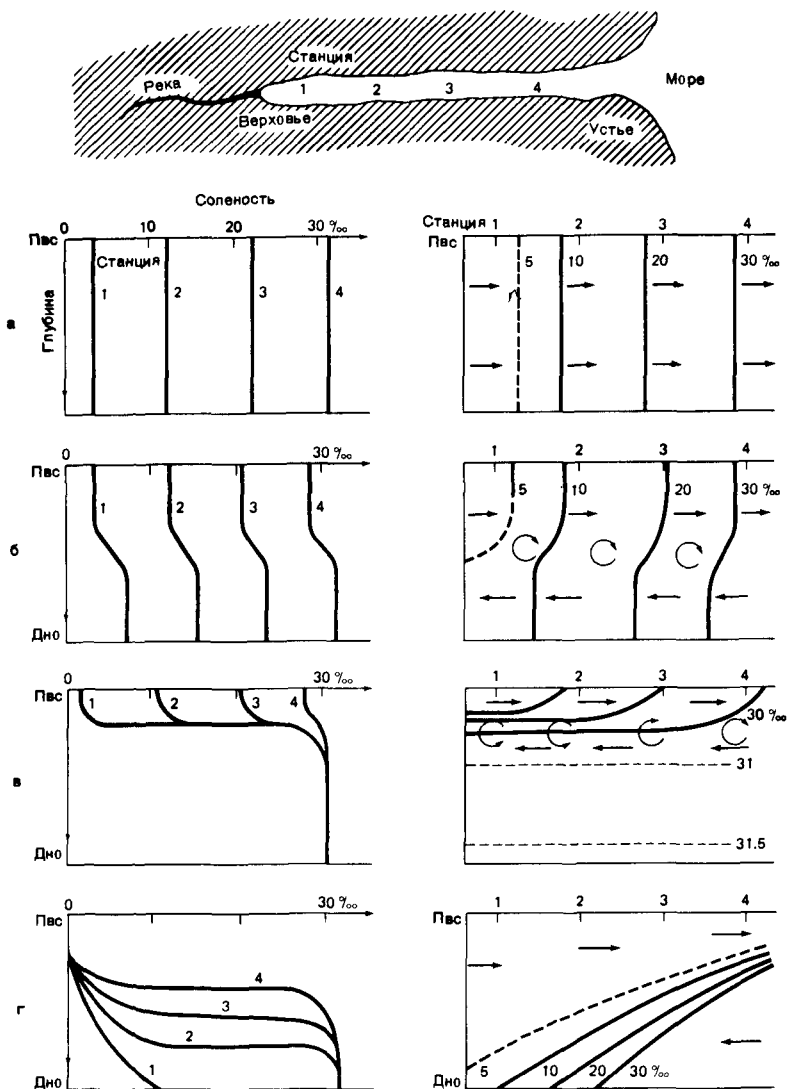
Р и с. 10.3. Типичные профили соленость — глубина в эстуарии вертикального смешения (а), слабостратифицированном (б), высокостратифицированном (в), с солевым клином (г). Контуры справа — соленость (в г/кг); Пвс — поверхность (по Пикарду [270]).
