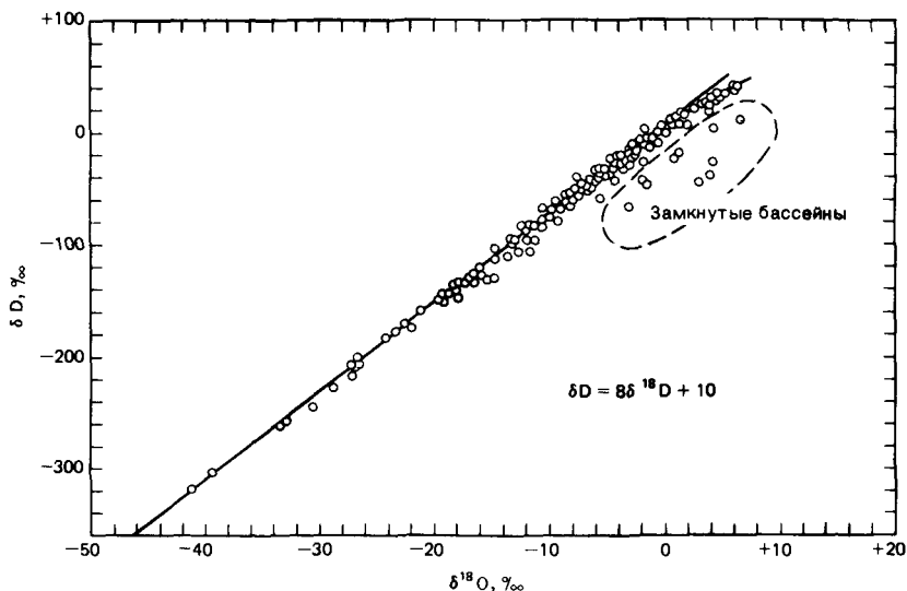
Р и с. 15.1. Изменения концентраций дейтерия и ^{18}O в реках, озерах, дождевых водах и в снегу (по Крейгу [74]).
