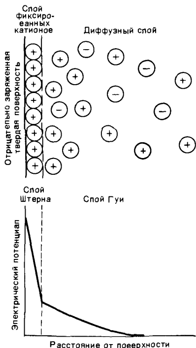
Р и с. 4.11. Схема неподвижного слоя Штерна и диффузного слоя Гуи.
