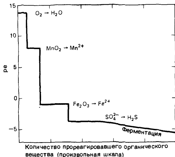
Р и с. 12.3. Изменение E_h пресной воды в контакте с осадком в зависимости от количества разложившегося органического вещества. Длины различных горизонтальных участков являются произвольными и зависят от количеств участвующих в реакции твердых фаз. Значение pH предполагается постоянным и равным 7,0.
