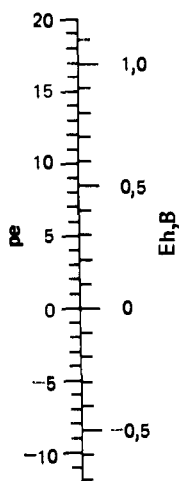
Р и с. 11.12. Сравнение шкал рН и Eh при 25°C.
