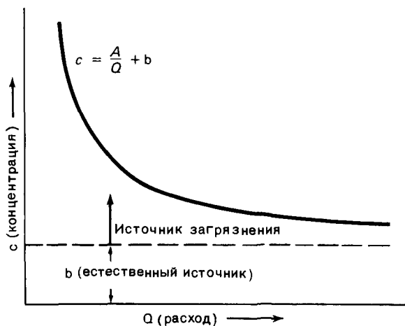
Рис. 8.15. Теоретическая зависимость концентрации растворенного вещества от расхода реки для веществ, содержания которых обусловлены загрязнением. A — антропогенное поступление в единицу времени (по Дейвису и Цобристу [78]).
