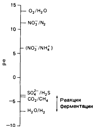
Р и с. 12.1. Приближенные значения p_e , соответствующие различным редокс-реакциям в водах при \text{pH} = 7 и 25^\circ\text{C} .
