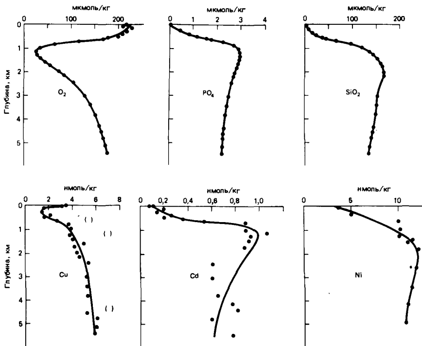
Р и с. 10.4. Профили кислорода, фосфата, кремнезема, меди и кадмия по данным GEOSECS, станция 226, и никеля, станция 204 (по Бойлю, Шчлатеру и Эдмонду [40]; Бойлю и др. [39]; Шчлатеру и др. [300]). Растущий фитопланктон в поверхностных слоях продуцирует O 2 и снижает содержание в воде биогенных элементов и рассеянных металлов. Процессы разложения ниже фотической зоны сопровождаются потреблением O 2 и переходом в воду биогенных элементов и рассеянных металлов. Профиль меди указывает на наличие ее источников у самой поверхности (атмосферный перенос) и в осадках. Заметьте, что концентрации крайне низкие ( 1 \text{ нмоль/кг} \approx 50 \cdot 10^{-6} \text{ млн}^{-1} ). Скобки указывают на предполагаемое загрязнение.
