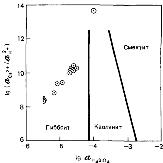
Р и б. 8.4. Пробы вод из ледникового района Южных Каскадных гор (по Рейнольдсу и Джонсону [286]), нанесенные на диаграмму устойчивости \lg(a_{Ca^{2+}}/a_{H^+}^2) - \lg a_{H_4SiO_4} . Половины кружков — содержания кремнезема ниже предела чувствительности аналитического метода (0,2 мг/л).
