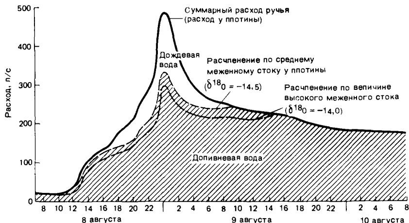
Р и с. 15.4. Сток Уилсон-Крик, расщепленный на дождевую воду и доливневой сток по данным по ^{18}\text{O} . Пунктирная линия показывает, как сказываются различные предположения об изотопном составе доливневой воды (по Фрицу и др. [115]).
