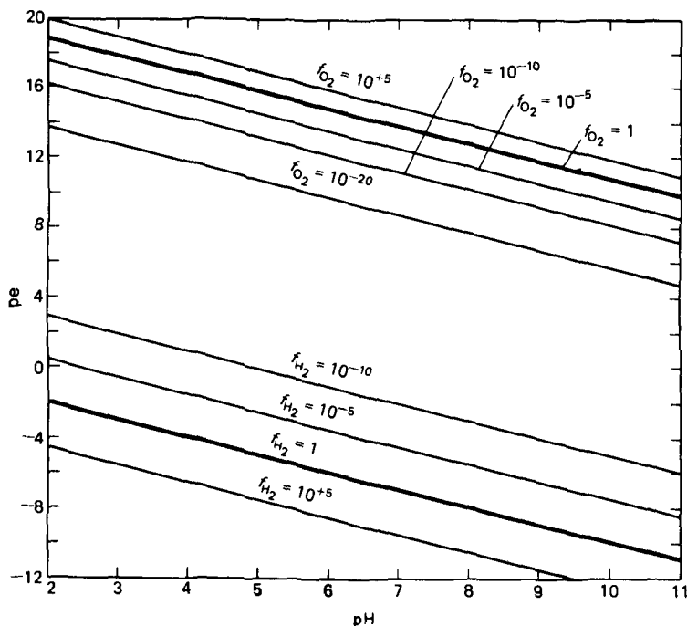
Р и с. 11.3. Линии равных петучестей кислорода и водорода в зависимости от p_e и pH при 25^\circ C .
