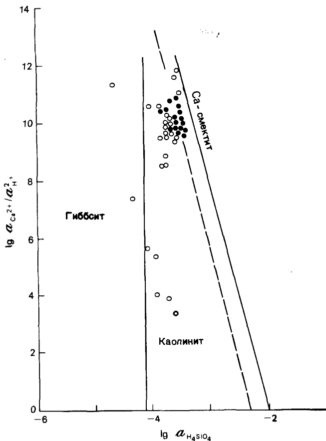
Р и с. 8.6. Данные о системе реки Рио-Танама на диаграмме активностей для системы CaO - Al_2O_3 - SiO_2 - H_2O при 25^\circ C . Поля устойчивости даны по Хелгесону [152]. Пунктирная линия основана на значениях K , предложенных Нортонном. Черные кружки означают, что пробы осадков связаны с водой, содержавшей смектит и каолинит (по Нортону [254]).
