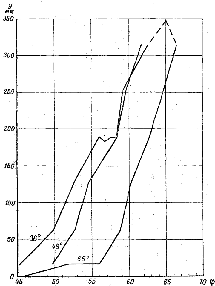
Рис. 23. Изменение среднегодового стока рек в зависимости от широты.
