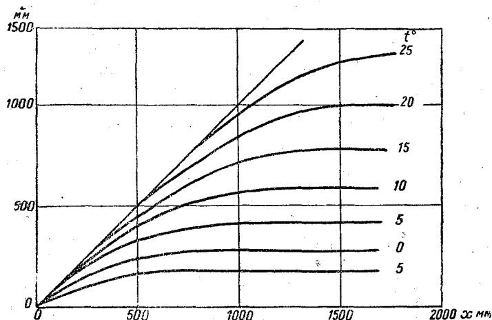
Рис. 11. Зависимость годовой суммы испарения ( z ) с поверхности речных бассейнов от годовых сумм атмосферных осадков ( x ) и среднегодовых температур воздуха ( t ) (по В. Вундту).
