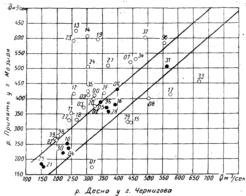
Рис. 29. График зависимости между среднегодовыми расходами р. Припяти у г. Мозыря и р. Десны у г. Чернигова.
