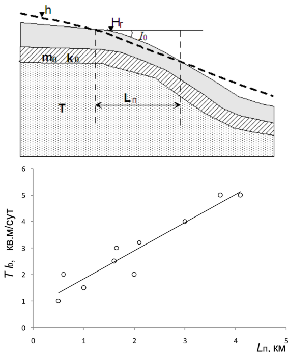
Рис. 1.3. Принципиальная схема формирования участка поглощения поверхностных вод и зависимость его протяженности L_{\text{п}} от соотношения проводимости пласта под рекой T и уклона поверхности воды в реке I_0
