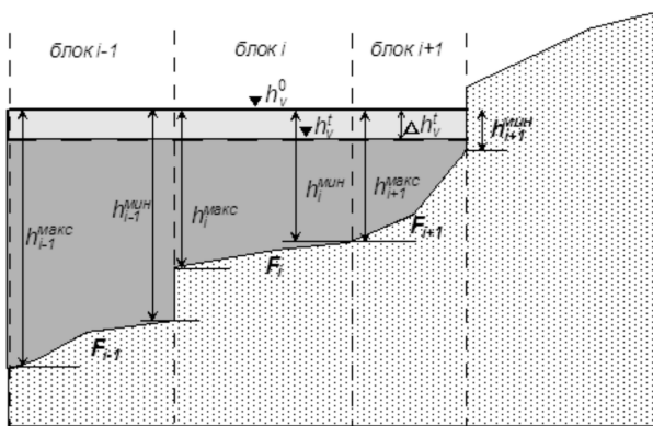
Рис. 5.2. Расчетная схема изменения площади дна водоема F в зависимости от его глубины h_v в границах блока модели
