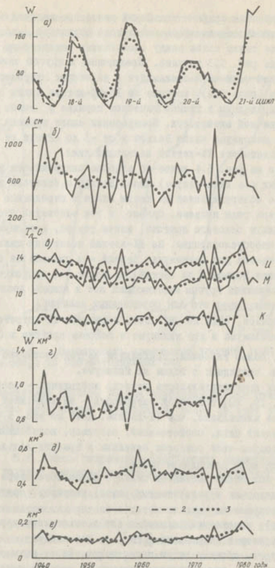
Рис. 5.3. Хронологический ход чисел Вольфа (а), амплитуды колебаний уровня (А) Сарезского озера (б), средней летней температуры воздуха на метеостанции Ирхт (И), Мургаб (М) и Каракуль (К) (в), бокового притока в Сарезское озеро (г), стока рек Мургаб (п. Мургаб) (д) и Лянгар (п. "Устье") (е) за 1940-1980 гг.: 1 - годовые значения, 2 - средние летние, 3 - скользящие пятилетние средние
