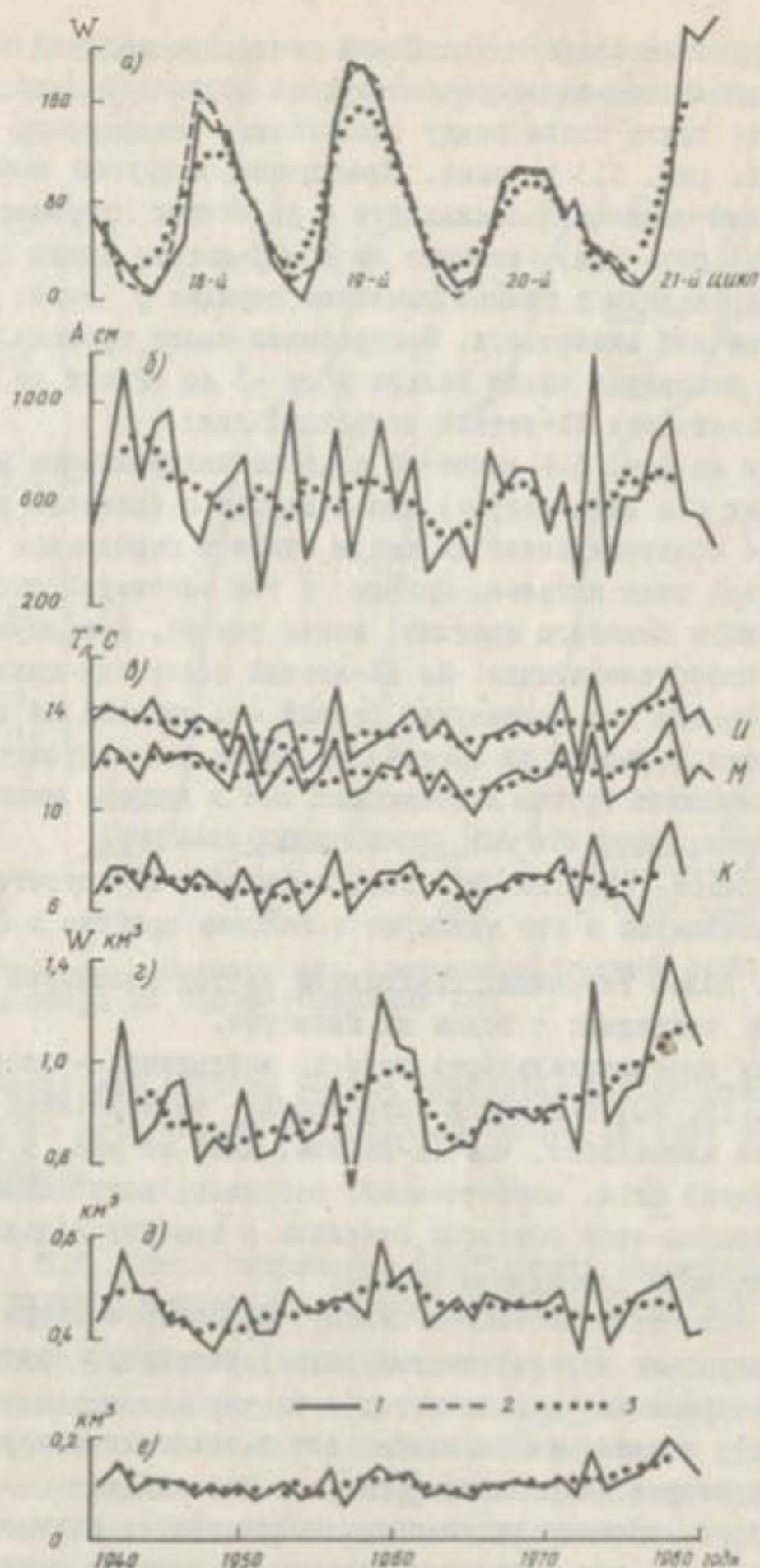
Рис. 5.3. Хронологический ход чисел Вольфа (а), амплитуды колебаний уровня (А) Сарезского озера (б), средней летней температуры воздуха на метеостанции Иркут (И), Мургаб (М) и Каракуль (К) (в), стокового притока в Сарезское озеро (г), стока рек Мургаб (п. Мургаб) (д) и Лянгар (п. "Устье") (е) за 1940-1980 гг.: 1 — годовые значения, 2 — средние летние, 3 — скользящие пятилетние средние
